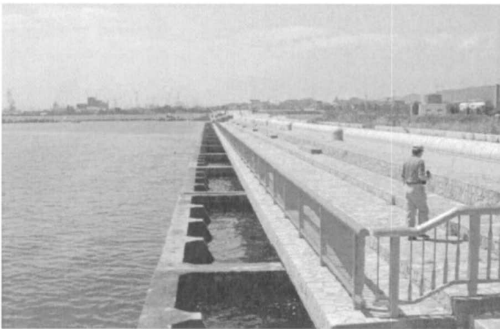
圖 5.14 面海視野的延伸彰顯了海洋魅力
