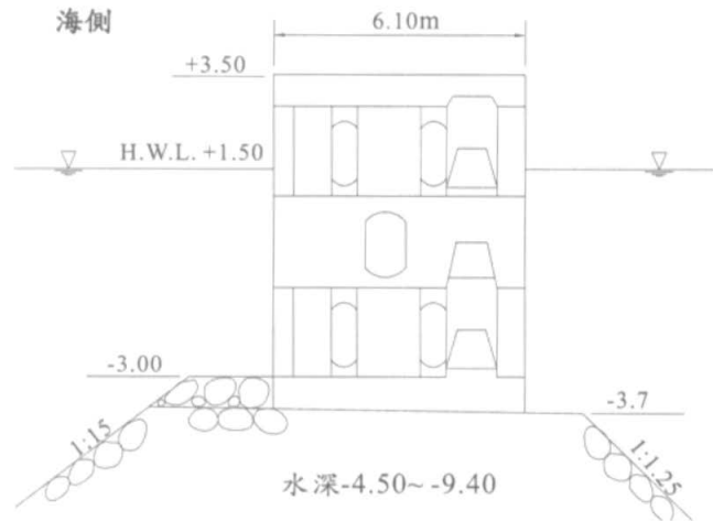
圖 4.7 混凝土塊堤設計斷面圖
