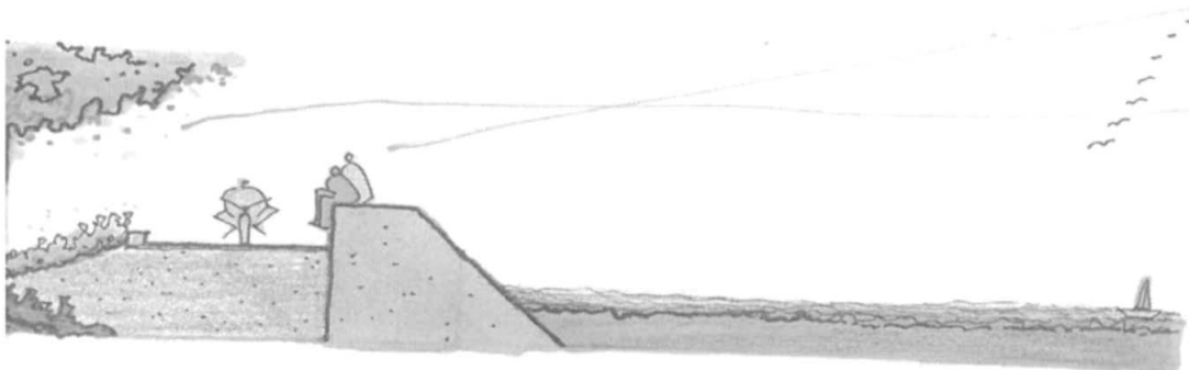
圖 5.12-b 海堤陸側部份提高道路覆土深度可增加視覺可及性
