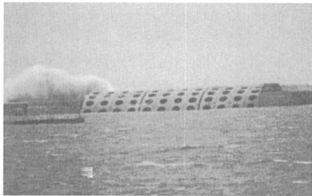
圖 4.8 開孔式新型防波堤
