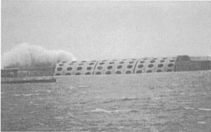
圖 2.27 開孔式新型防波堤
