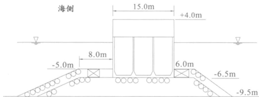
圖 4.9 合成堤設計斷面圖
