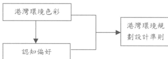
圖 6.7 研究架構圖
