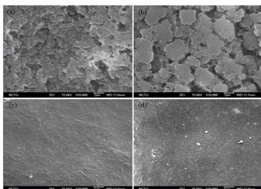
Fig. 3. SEM images of the SQI x film: (a) SQI 5 (b) SQI 1 (c) SQI 0.1 (d) SQI 0.01 .
