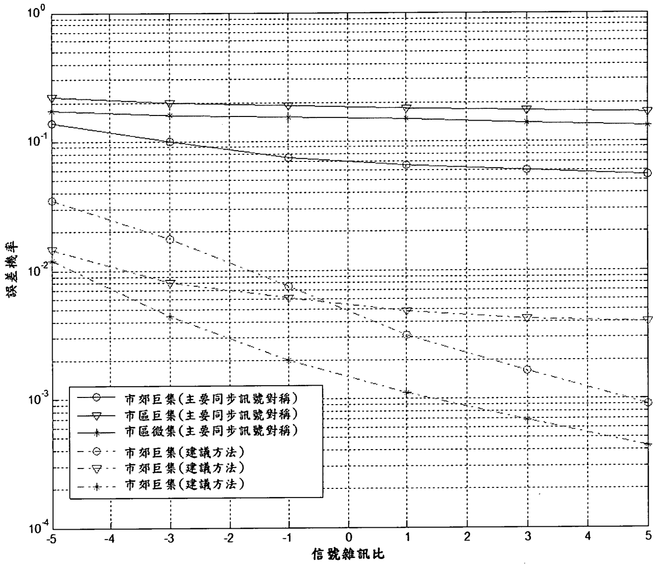
不同頻道之 N_{ID}^{cell} 偵測
