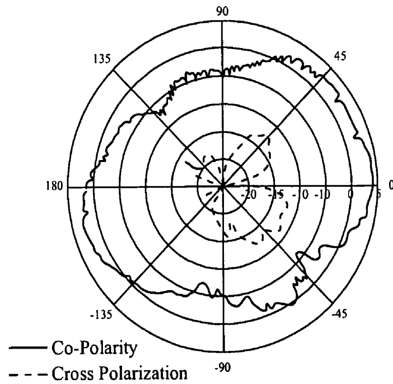
H-Plane
