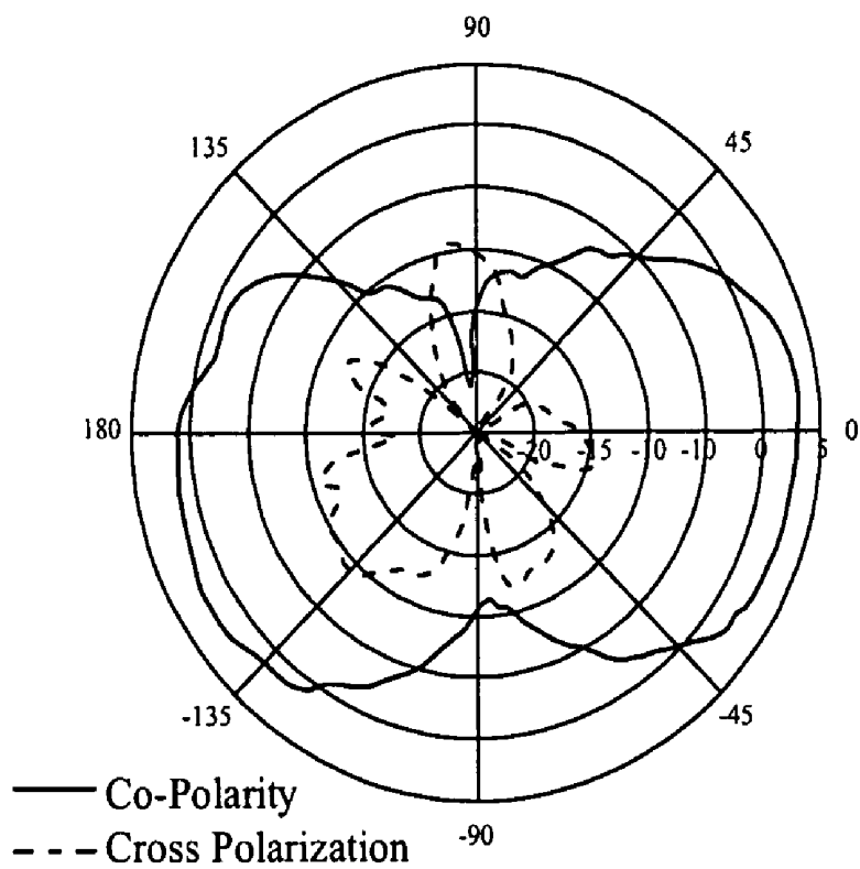
E-Plane
