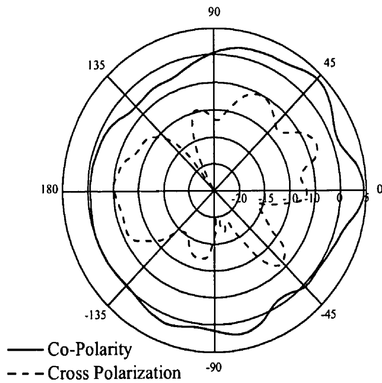
H-Plane
