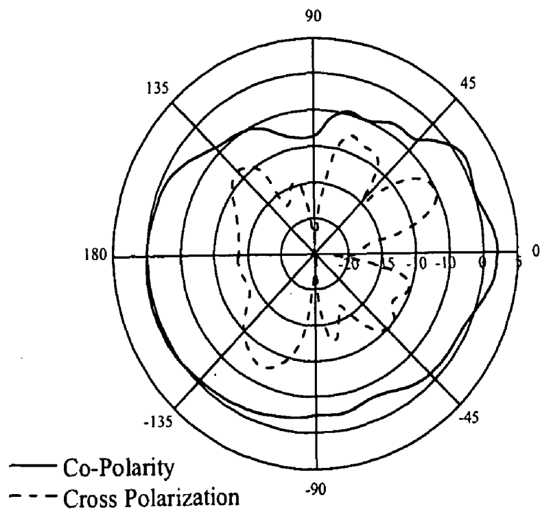
H-Plane
