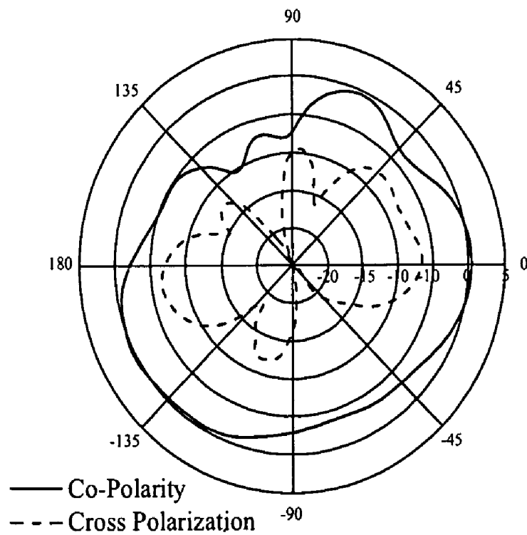
H-Plane
