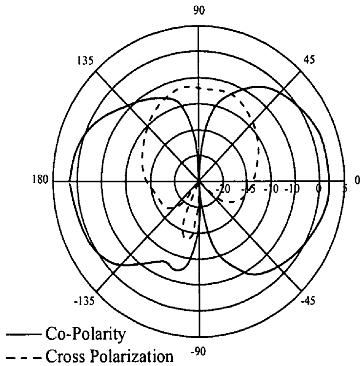
E-Plane
