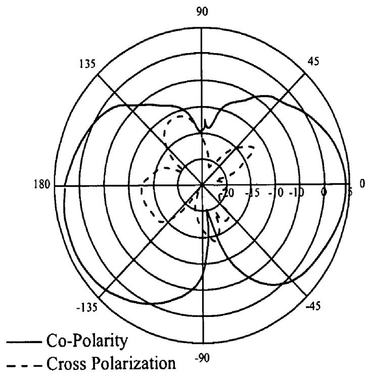
E-Plane
