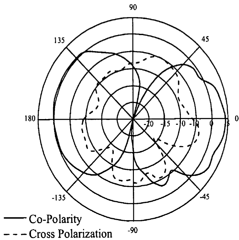
E-Plane
