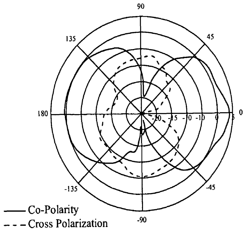
E-Plane
