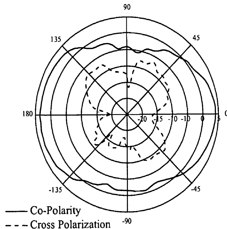
H-Plane
