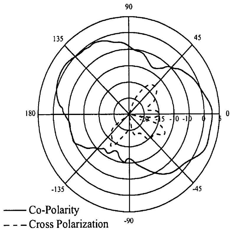
E-Plane
