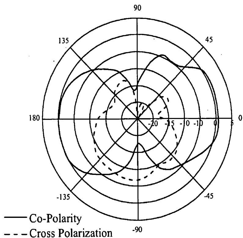
E-Plane
