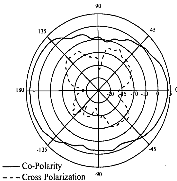
H-Plane
