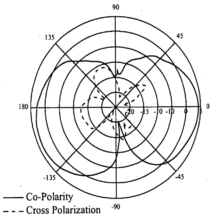
E-Plane
