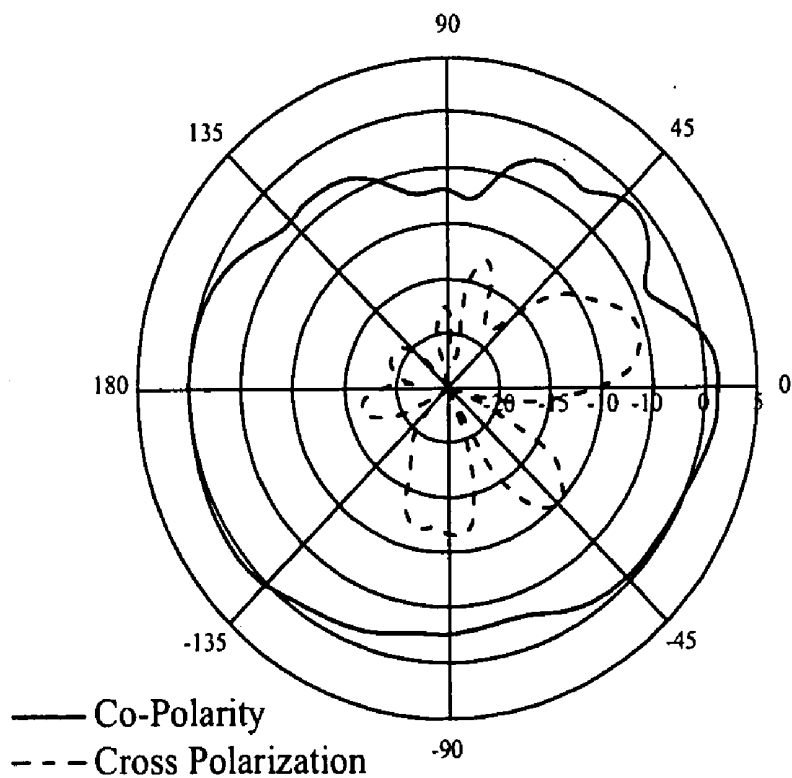
H-Plane
