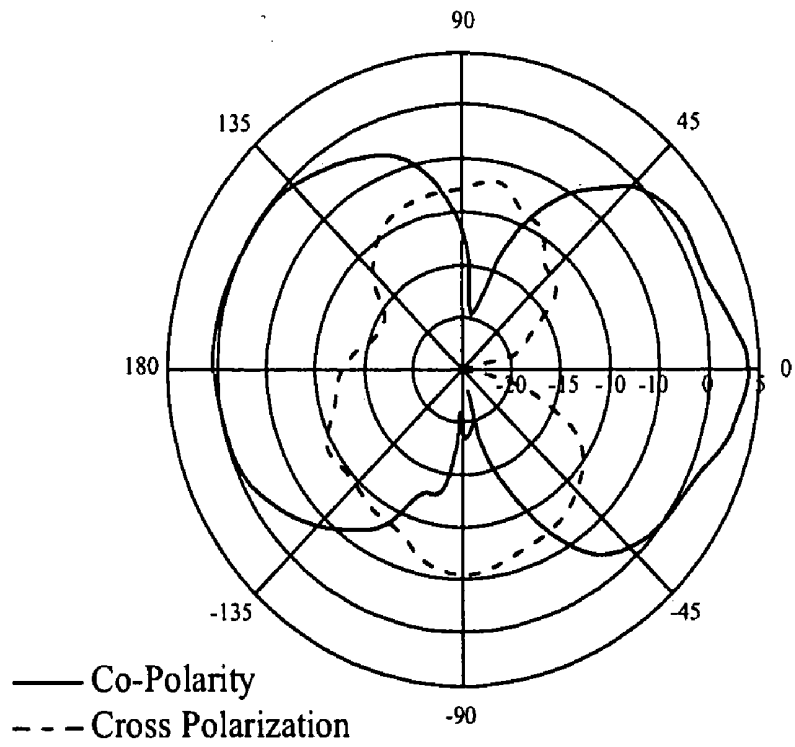
E-Plane
