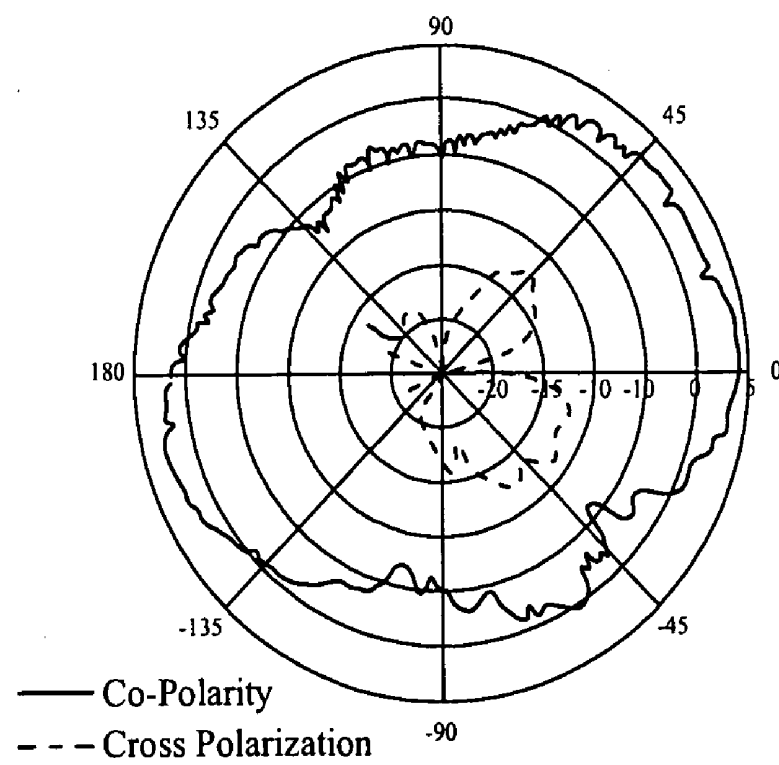
H-Plane
