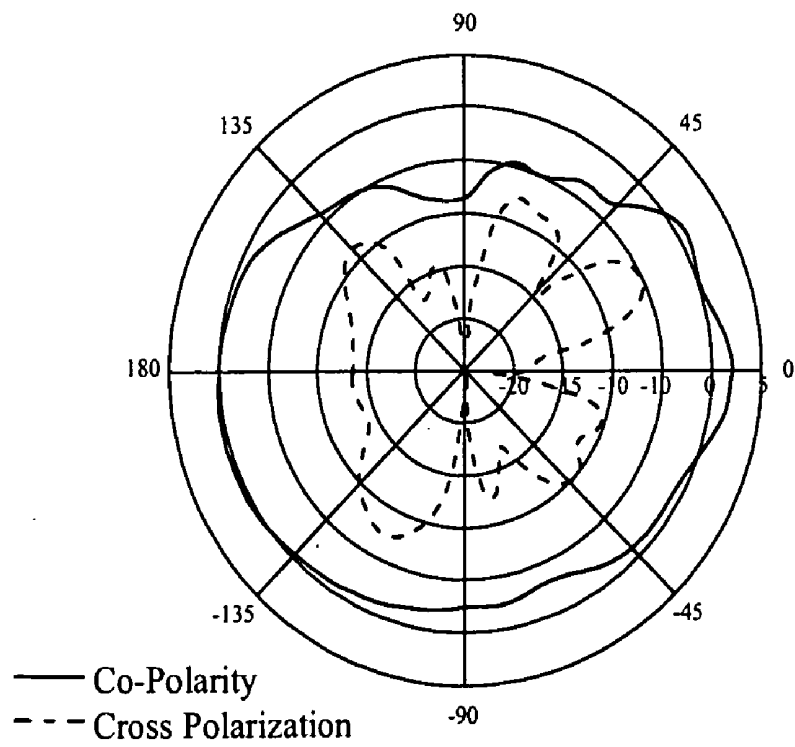
H-Plane
