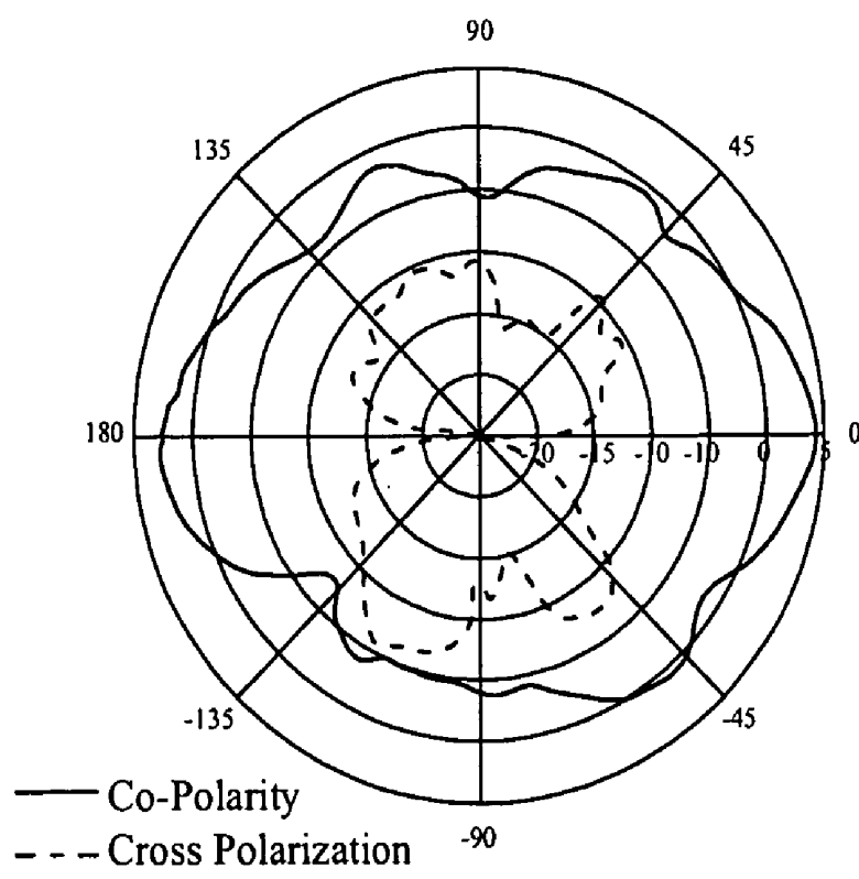
H-Plane
