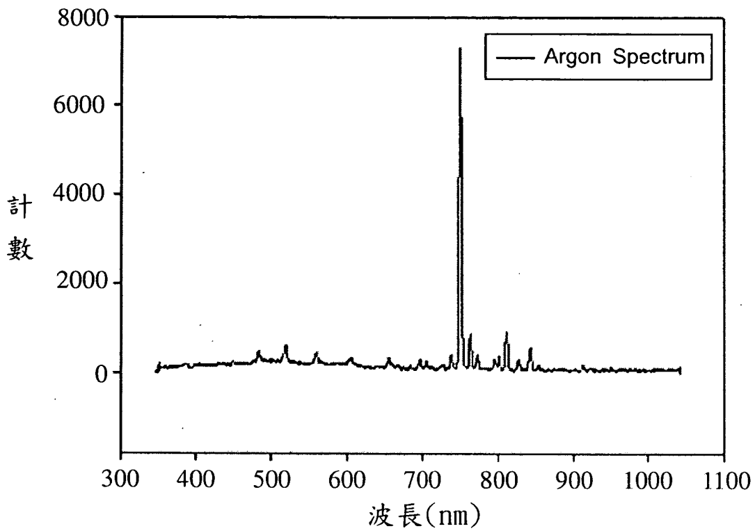
氬氣電漿氣泡光譜量測
