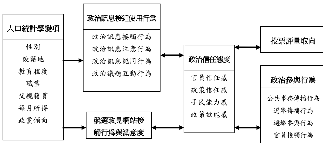
圖 11 研究架構圖
