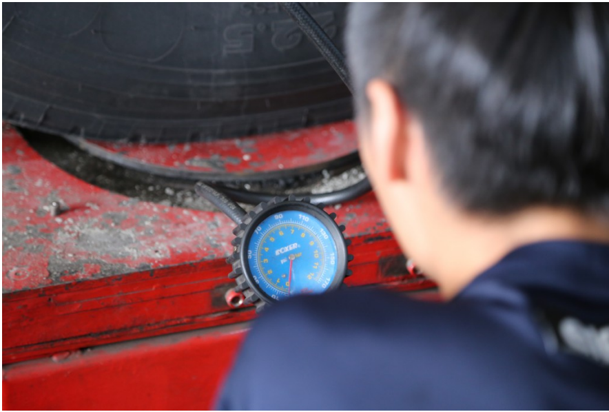
因擔心司機並未做好檢查，使胎輪磨耗，每一台車皆需測量胎壓。 (照片來源／麻愷垣攝)
