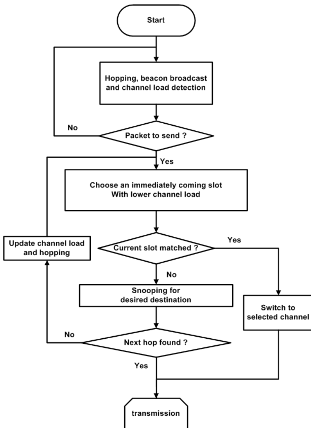
圖 4-5 System flow chart
