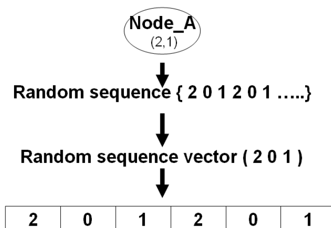
圖 4-1 Simple random sequence
