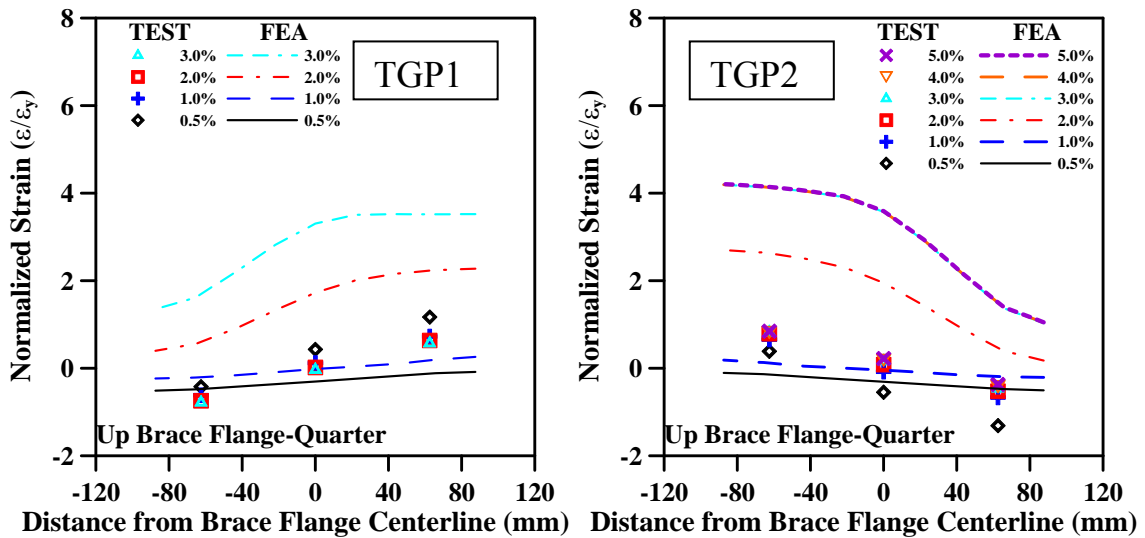
圖 5.17 2 組試體斜撐 1/4 長度下翼板實驗與分析之軸向應變分佈
