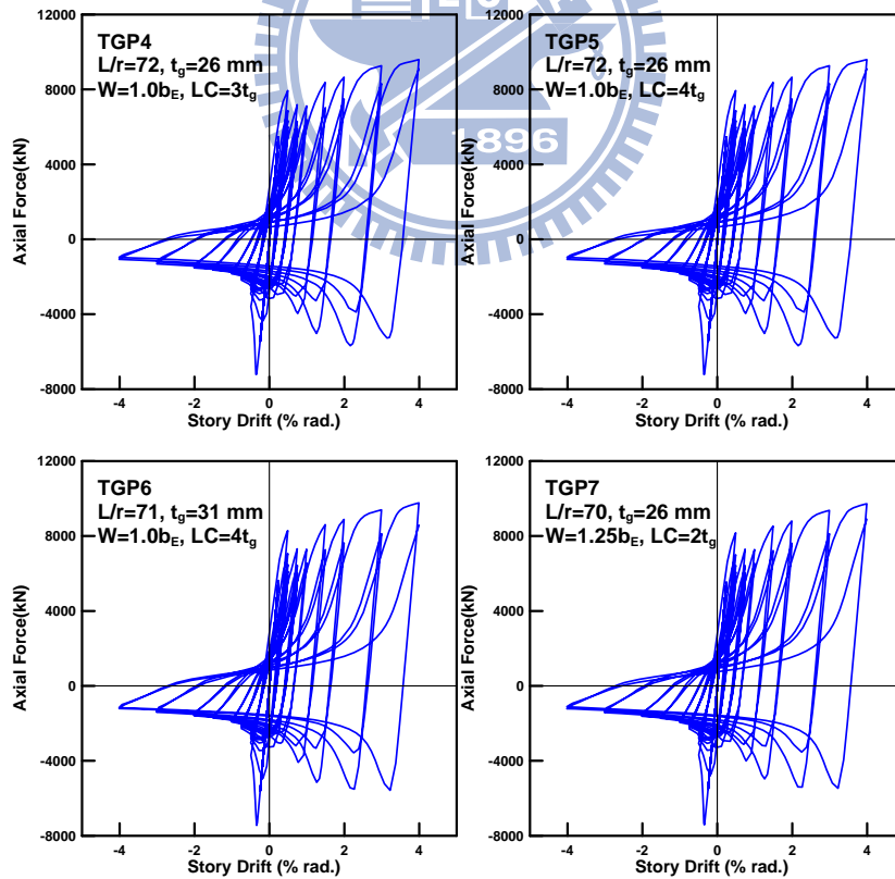
圖 3.25 4 組模型之軸向載重與層間位移角關係圖 (參數 LC 與 W )
