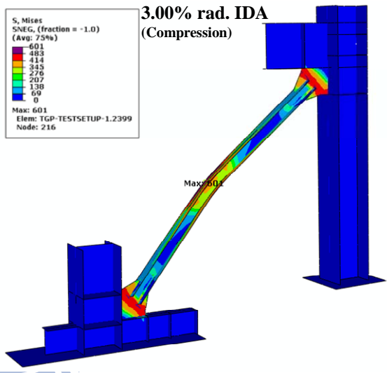
圖 5.7 試體 TGP1 之斜撐構材試驗行為與分析結果比較 (續)
