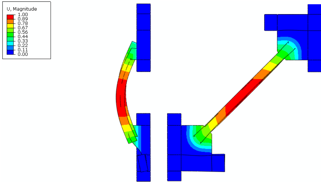
圖 3.11 典型斜撐構材挫屈模態 (Mode 1)
