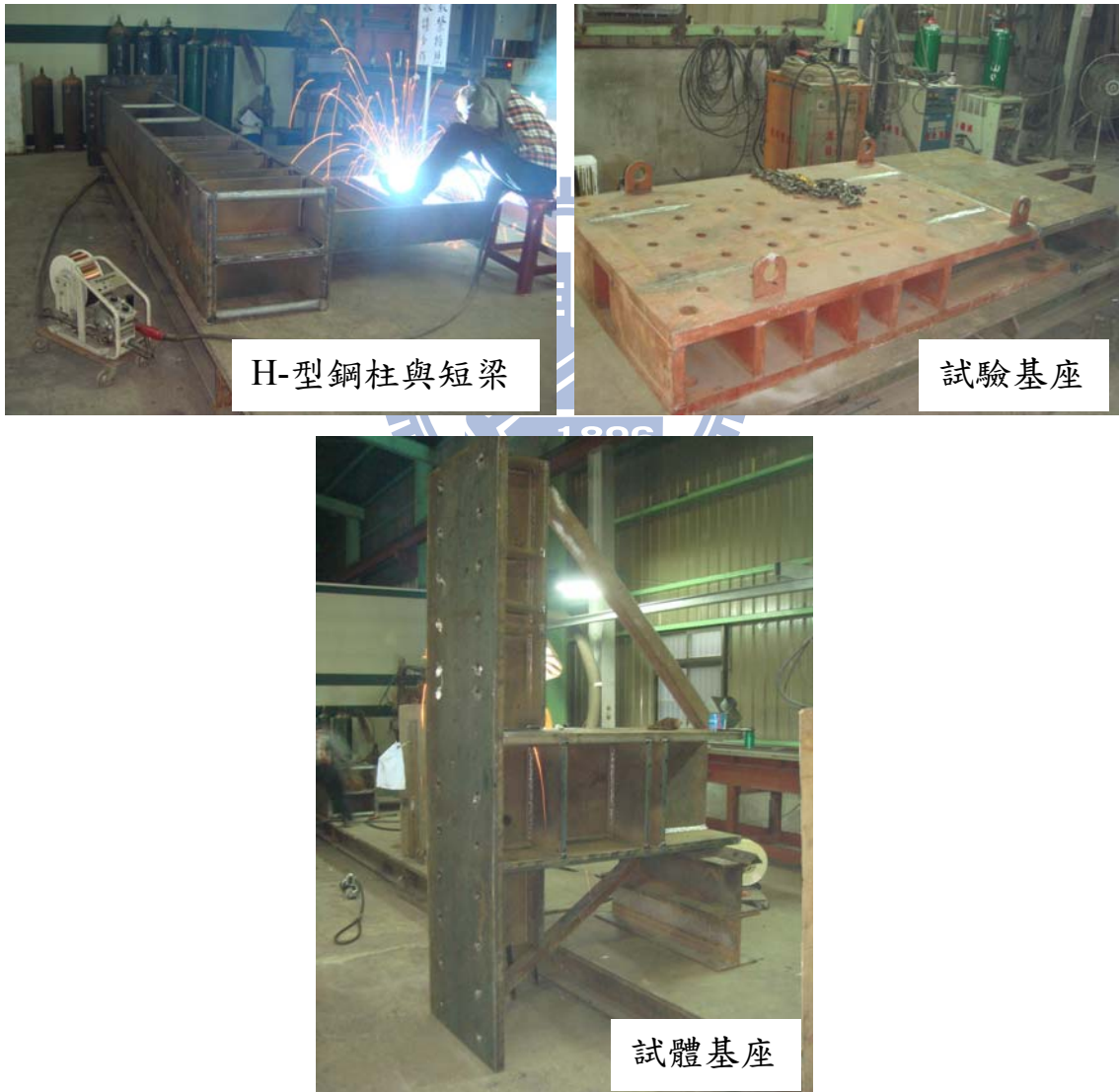
圖 4.21 試驗構架之各部位銲接與組裝
