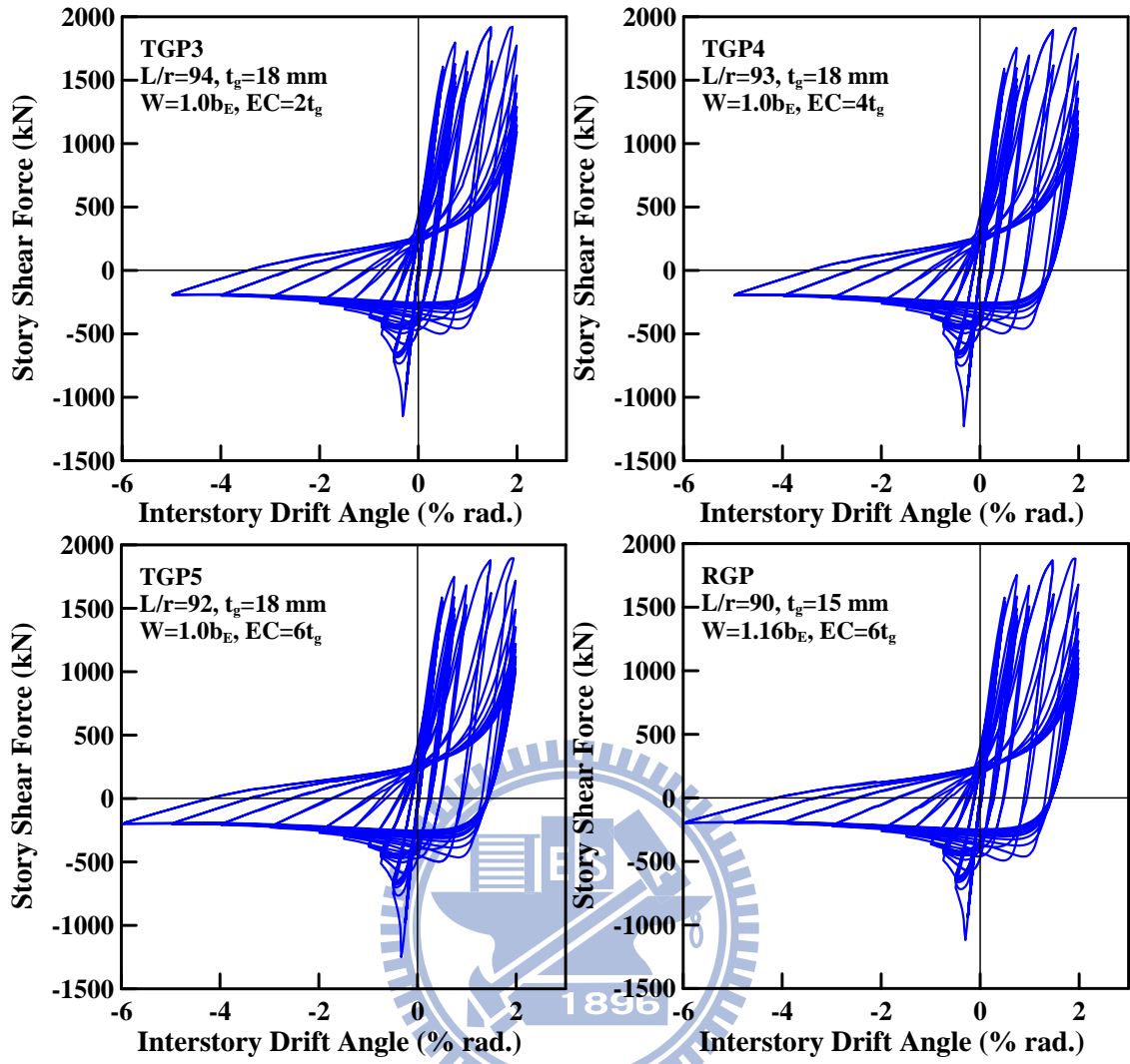
圖 4.63 EC 系列試體之層間剪力-層間位移角關係圖
