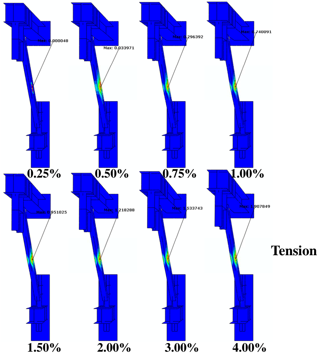
圖 5.21 試體 TGP1 數值模型斜撐構材之等值塑性應變分佈 (受拉)
