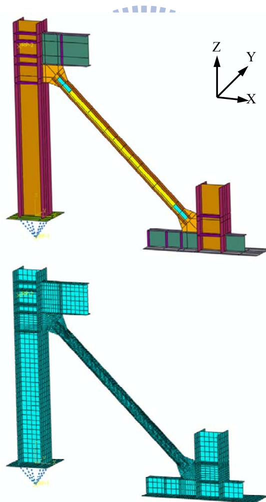
圖 5.1 分析模型與網格圖
