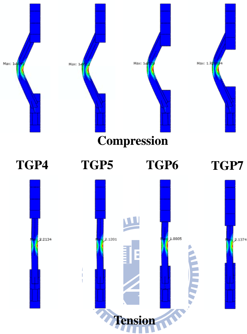
圖 3.23 4 組模型之斜撐構材 PEEQ 分佈圖 (4% 弧度 IDA)
