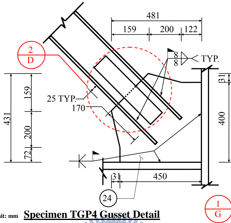
圖 4.16 試體 TGP4 接合板接合細部圖
