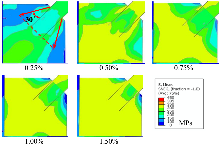
圖 2.22 具 2t 偏移矩形接合板之等值應力分佈圖 (陳誠直等人, 2009)
