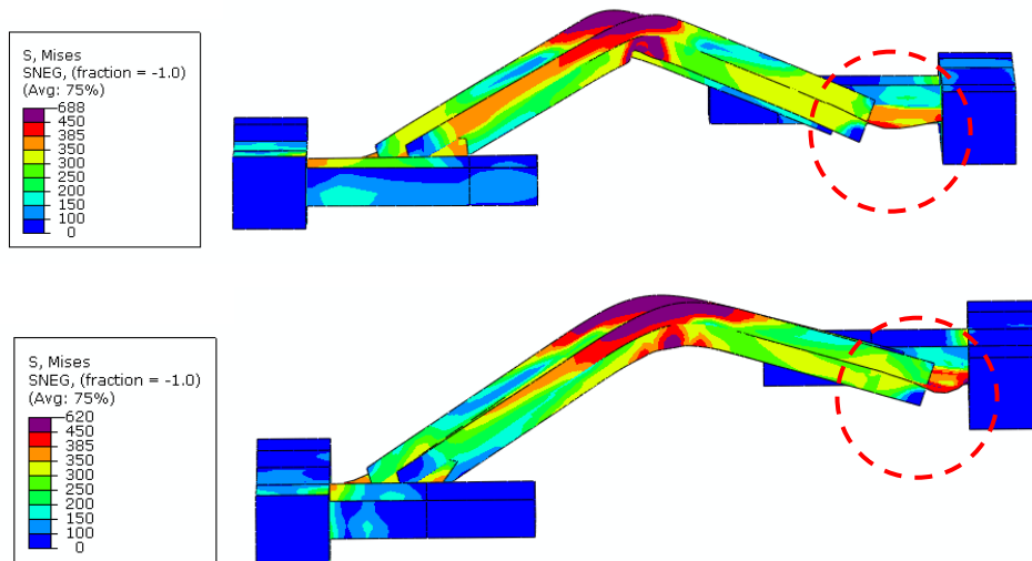
圖 3.35 模型 RGP 與模型 TGP1 產生接合板挫屈 (4%層間位移角)
