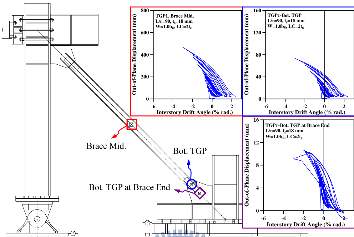
圖 4.66 試體 TGP1 斜撐端部至中央各測點之面外變形量
