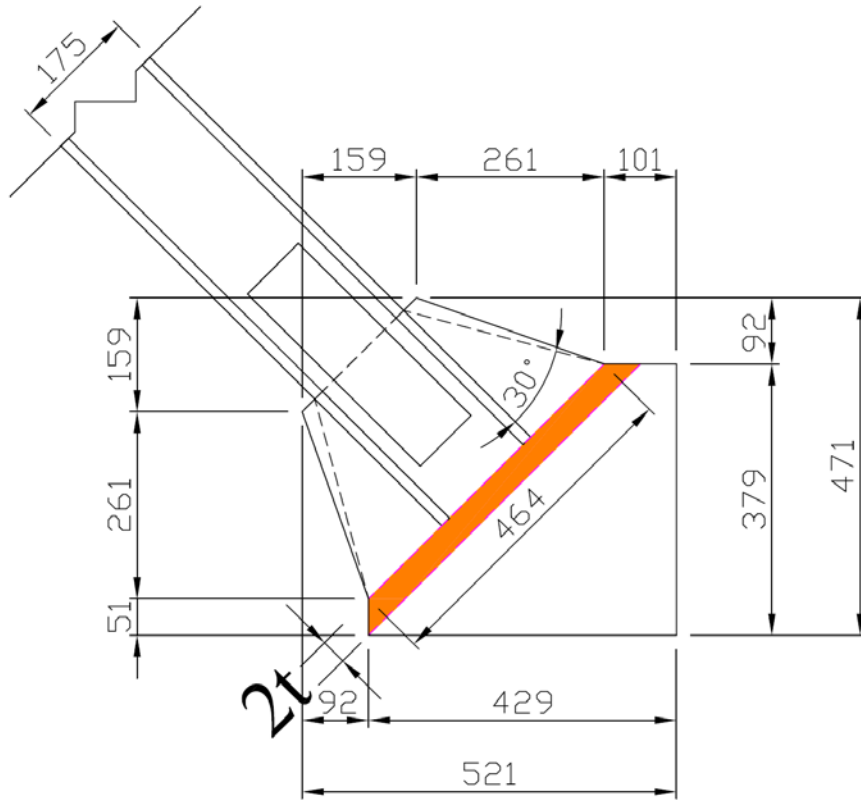
圖 4.2 試體 TGP1 接合板尺寸圖
