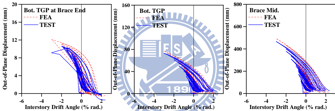
圖 5.5 試體 TGP1 實驗與分析之各測點面外變形量-層間位移關係圖比較
