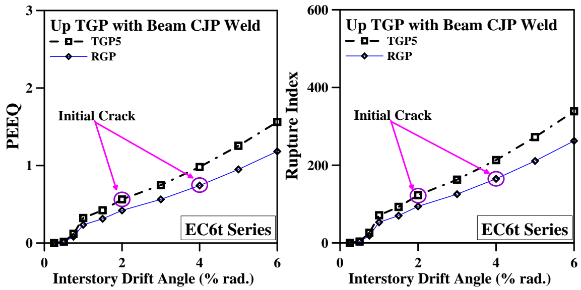
圖 5.30 EC6t 系列 2 組試體 PEEQ 與 RI 之分佈情形
