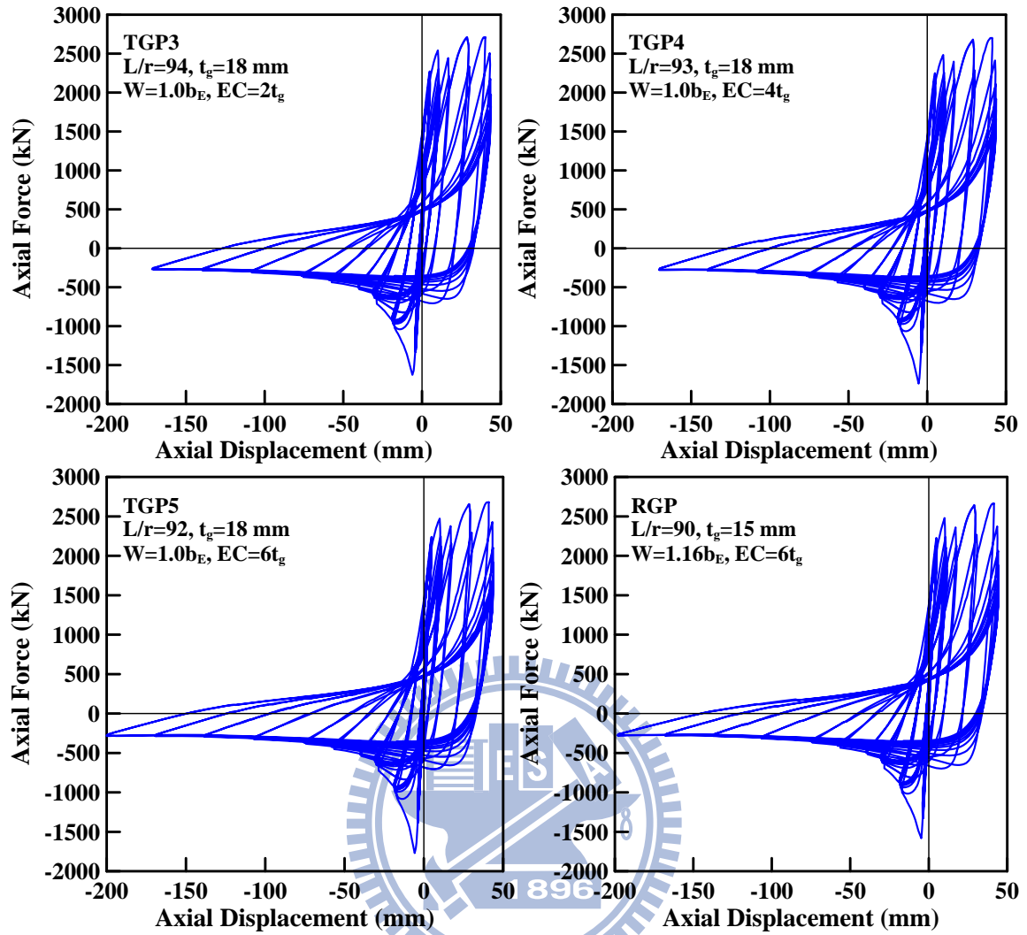
圖 4.64 EC 系列試體之軸力-軸向變位關係圖
