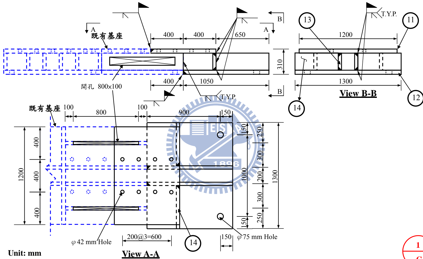
圖 4.29 試驗基座設計圖
