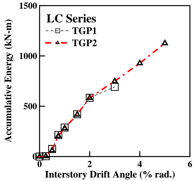
圖 4.77 LC 系列試體能量累積-層間位移角關係圖
