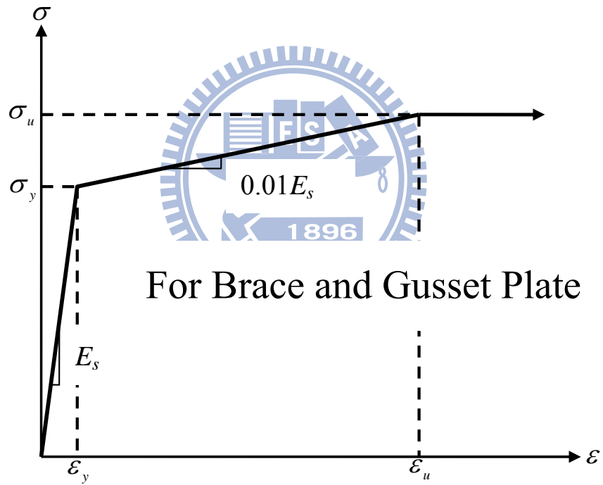
圖 3.8 鋼材之三線性應力-應變關係
