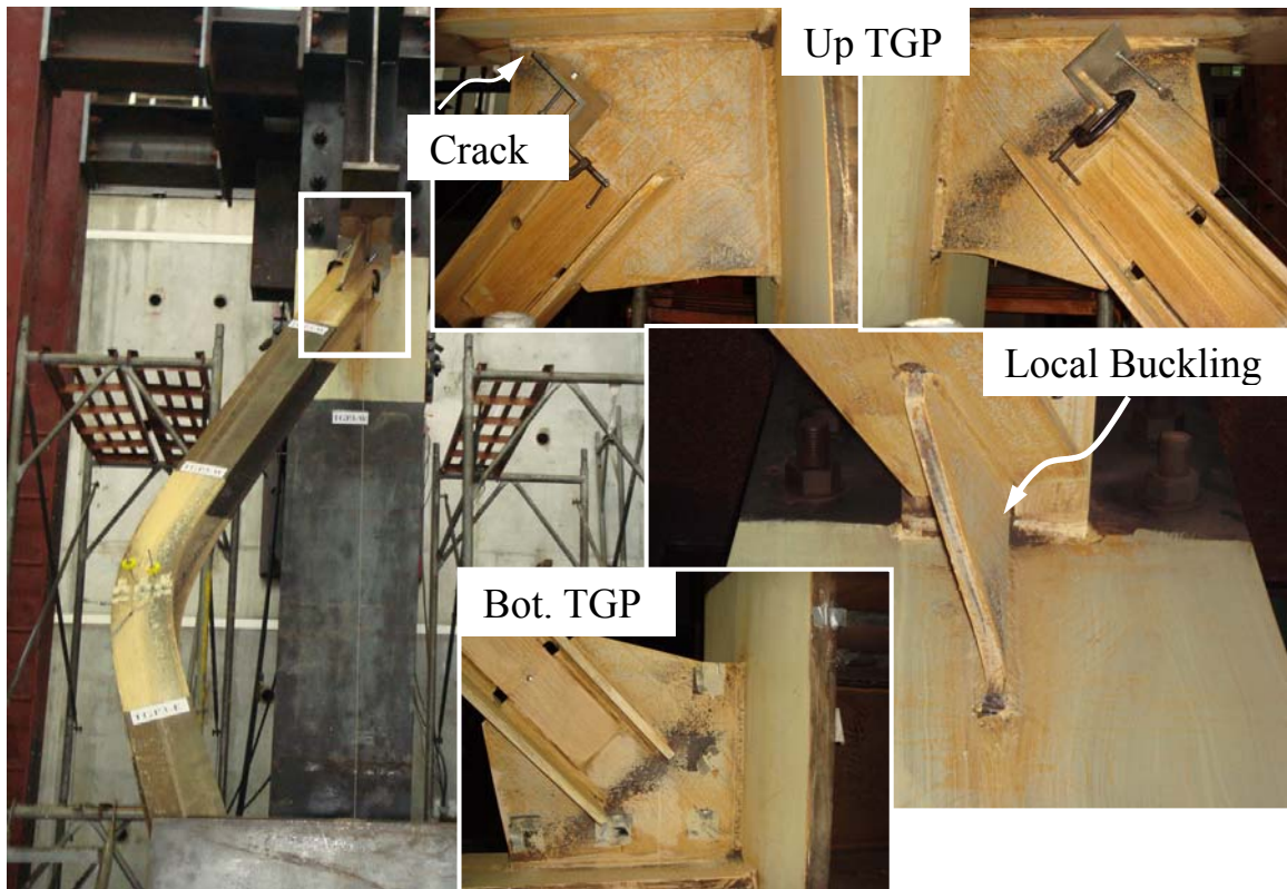
圖 4.50 試體 TGP3 最終破壞行為 (5% 弧度 IDA)
