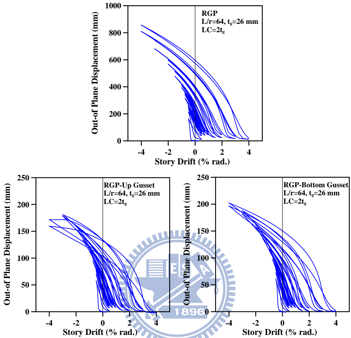
圖 3.36 模型 RGP 之斜撐構材與接合板之面外變形與層間位移角關係圖
