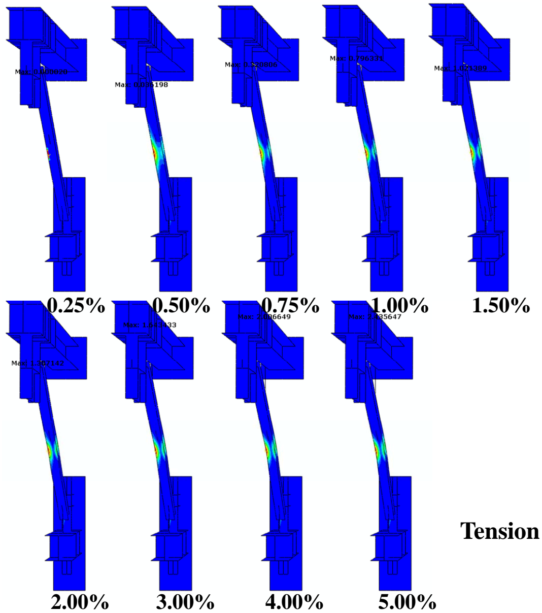
圖 5.23 試體 TGP2 數值模型斜撐構材之等值塑性應變分佈 (受拉)
