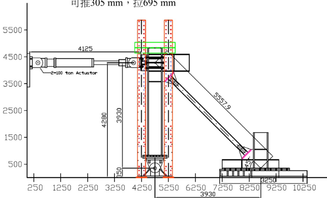
圖 4.24 載重試驗設置之俯視與正視圖
