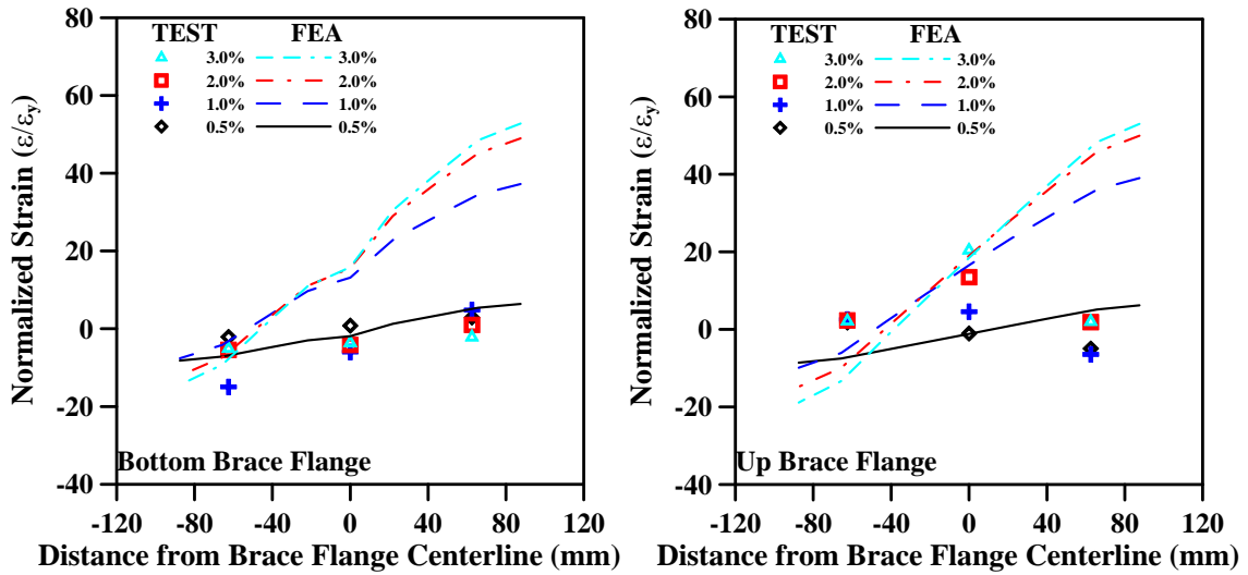
圖 5.15 試體 TGP1 斜撐中央處翼板實驗與分析之軸向應變分佈
