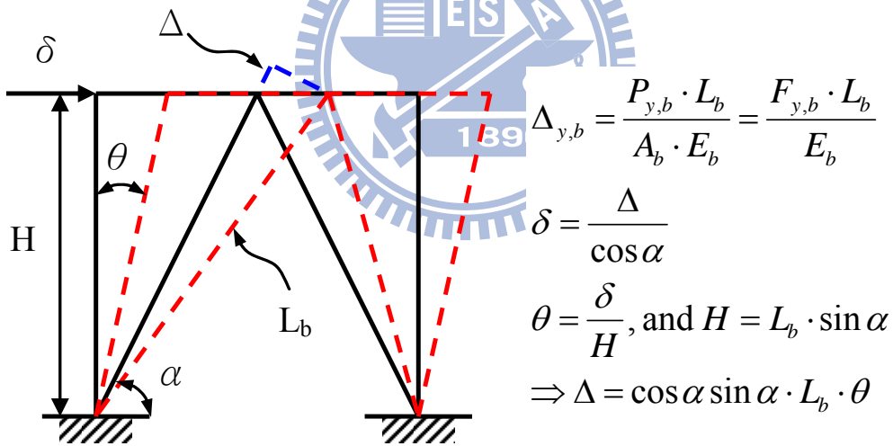
圖 3.4 層間位移角與斜撐構材軸向變形量之關係圖
