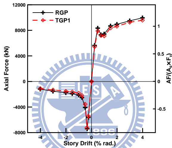
圖 3.34 模型 RGP 與模型 TGP1 之強度包絡線圖
