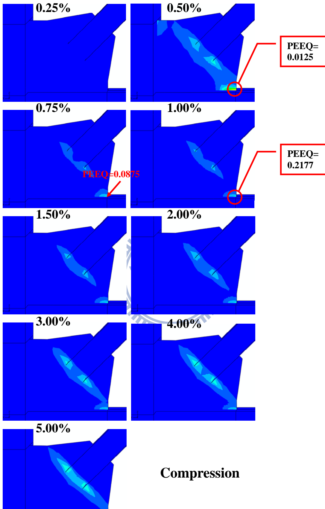
圖 5.25 試體 TGP2 數值模型梯形接合板之等值塑性應變分佈
