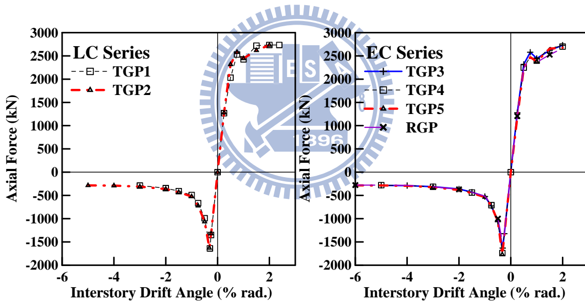
圖 4.65 具不同偏移區域型式之接合板與斜撐構材軸向強度包絡線圖
