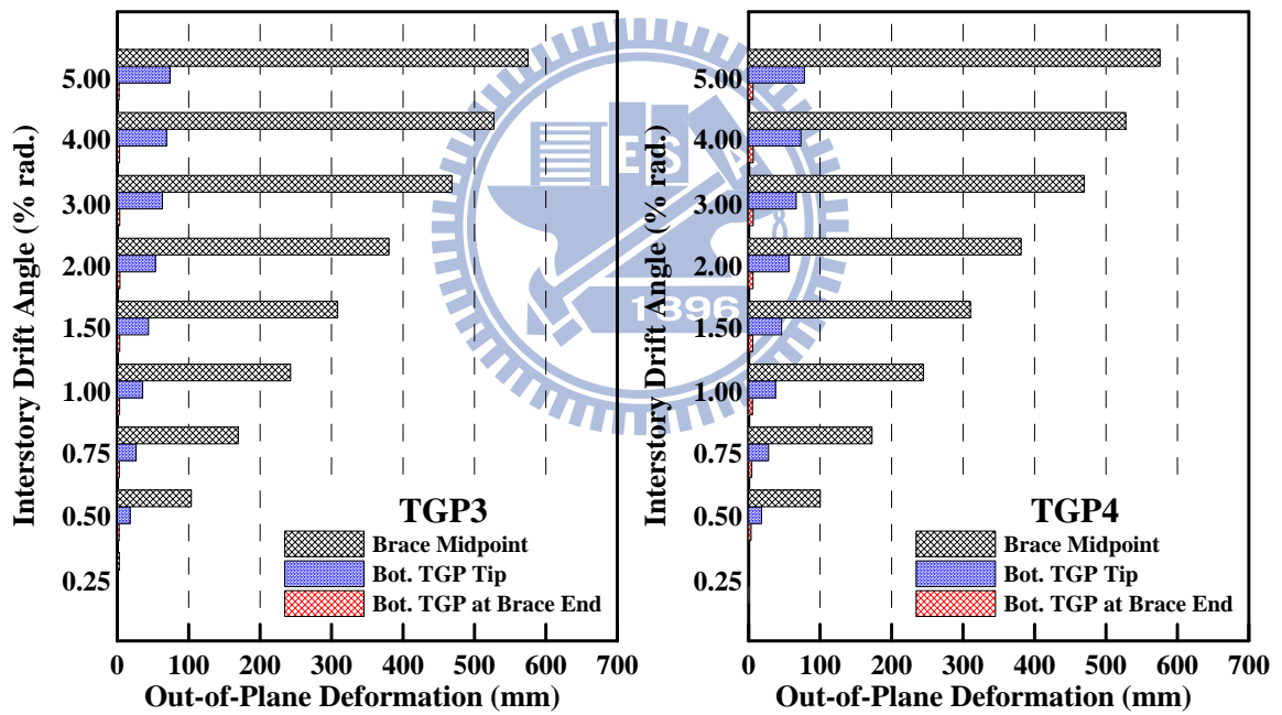
圖 4.73 試體 TGP3 與試體 TGP4 之各測點面外變形量變化
