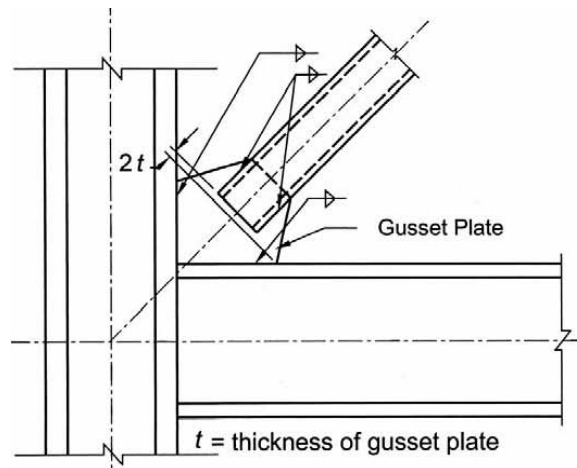
圖 1.5 面外挫屈之斜撐與接合板接合細節 (AISC 2005b)
