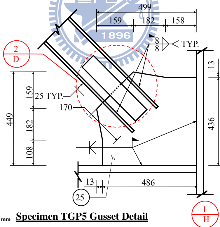
圖 4.17 試體 TGP5 接合板接合細部圖
