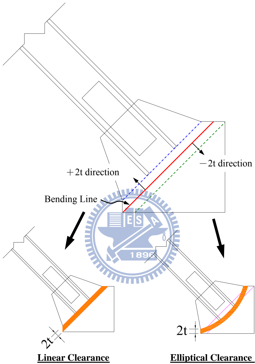
圖 4.1 不同偏移區域設計概念
