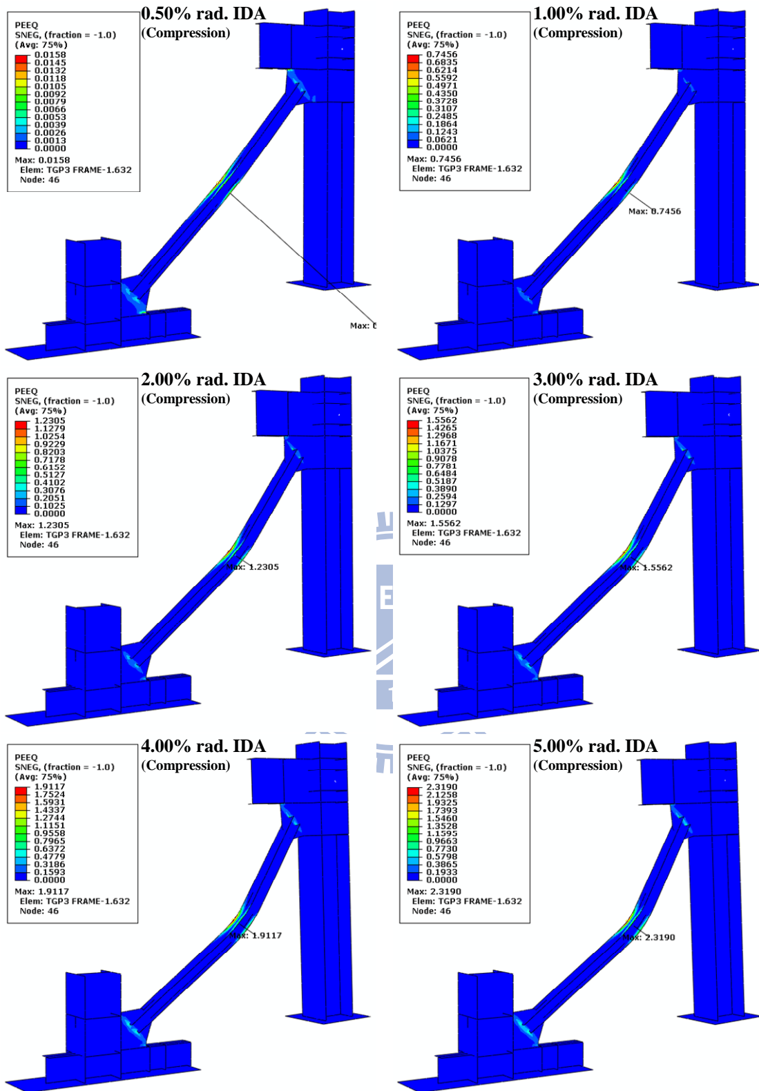
圖 5.10 試體 TGP2 斜撐構材分析模型之 PEEQ 分佈
