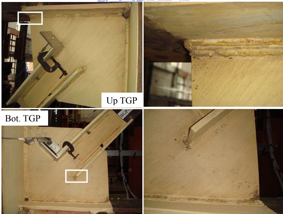
圖 4.59 試體 RGP 之上接合板與梁接合銲道開裂情況 (4% 弧度 IDA)
