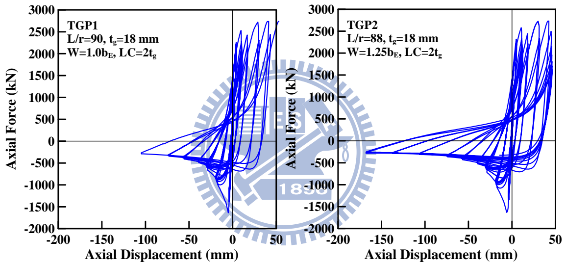
圖 4.62 LC 系列試體之軸力-軸向變位關係圖
