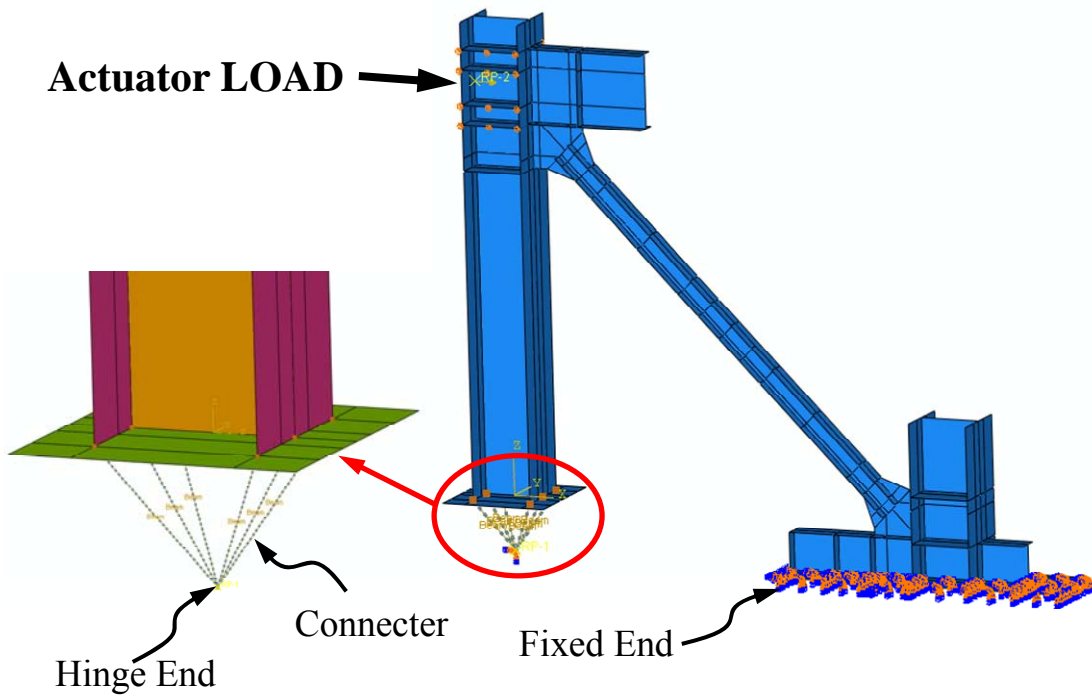
圖 5.2 分析模型之邊界條件設定
