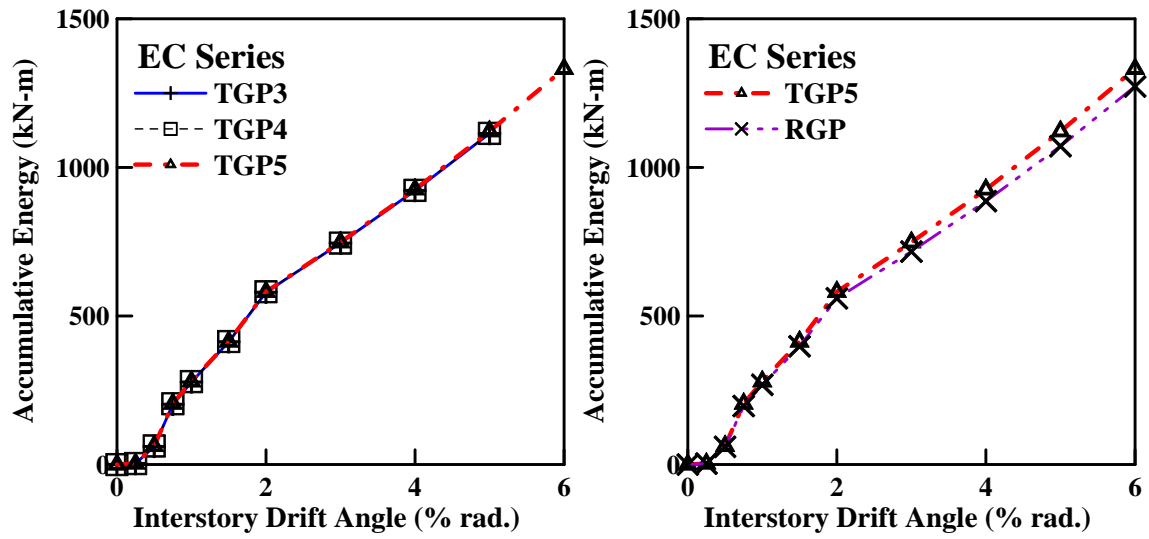
圖 4.79 EC 系列試體能量累積-層間位移角關係圖
