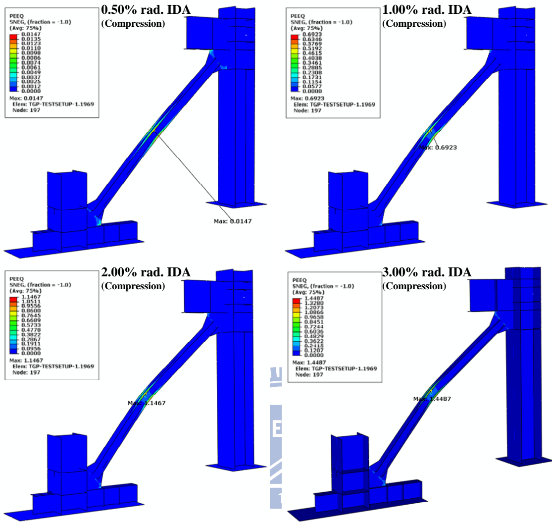
圖 5.8 試體 TGP1 斜撐構材分析模型之 PEEQ 分佈
