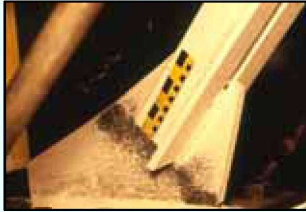
圖 2.1 含 2t 鉸區域長度之接合板凹折變形情況 (Astaneh-Asl et al. 1982)
