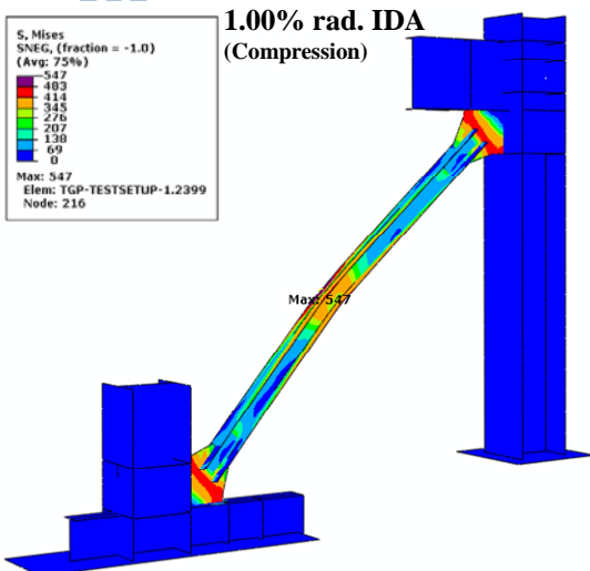
圖 5.7 試體 TGP1 之斜撐構材試驗行為與分析結果比較
