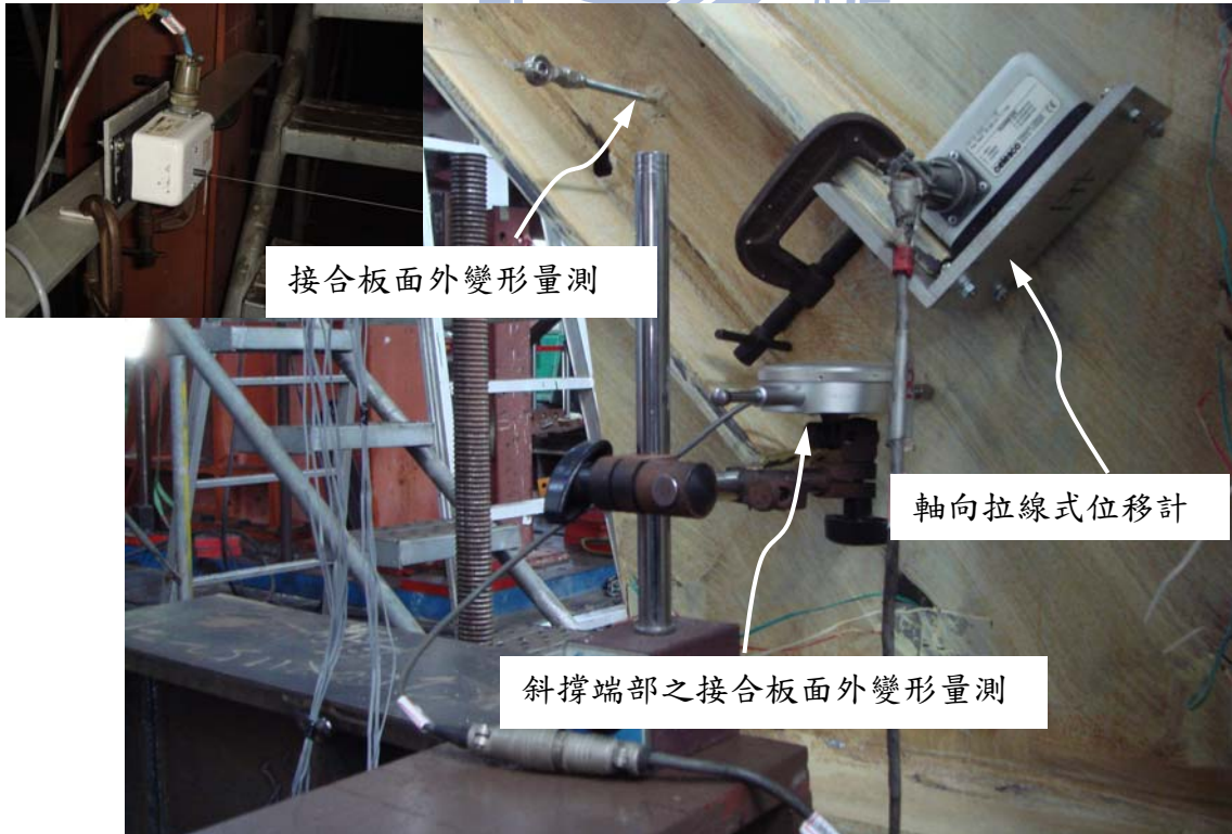
圖 4.35 斜撐與接合板各儀器架設實況
