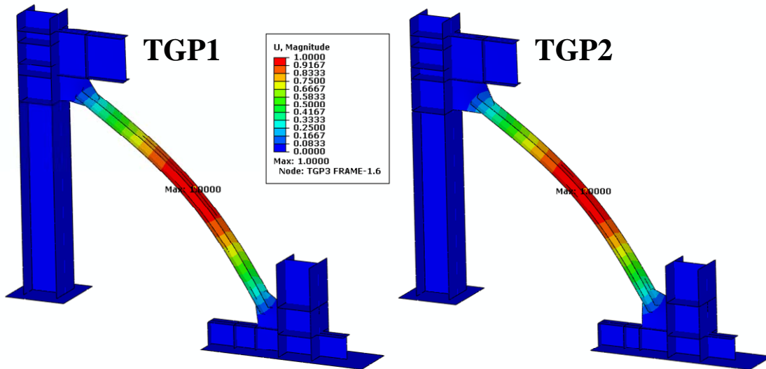
圖 5.3 試體 TGP1 與試體 TGP2 之挫屈模態 (Mode 1)
