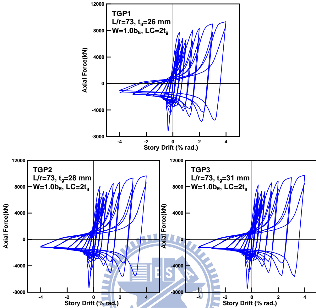
圖 3.16 3 組模型之軸向載重與層間位移角關係圖 (參數 \beta_j )
