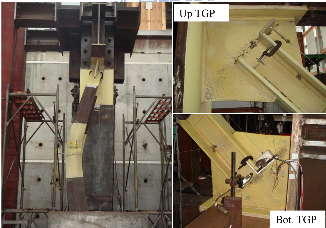
圖 4.55 斜撐挫屈與接合板凹折情形 (1% 弧度 IDA)
