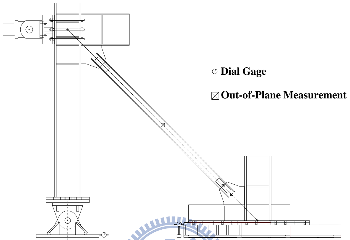
圖 4.34 試體與基座量測儀器架設圖
