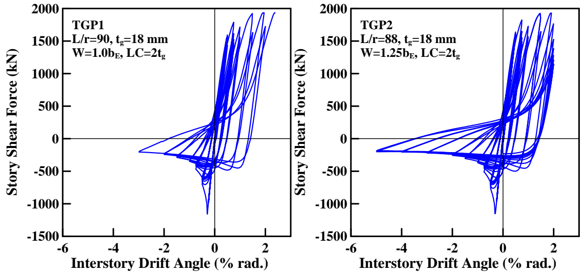
圖 4.61 LC 系列試體之層間剪力-層間位移角關係圖
