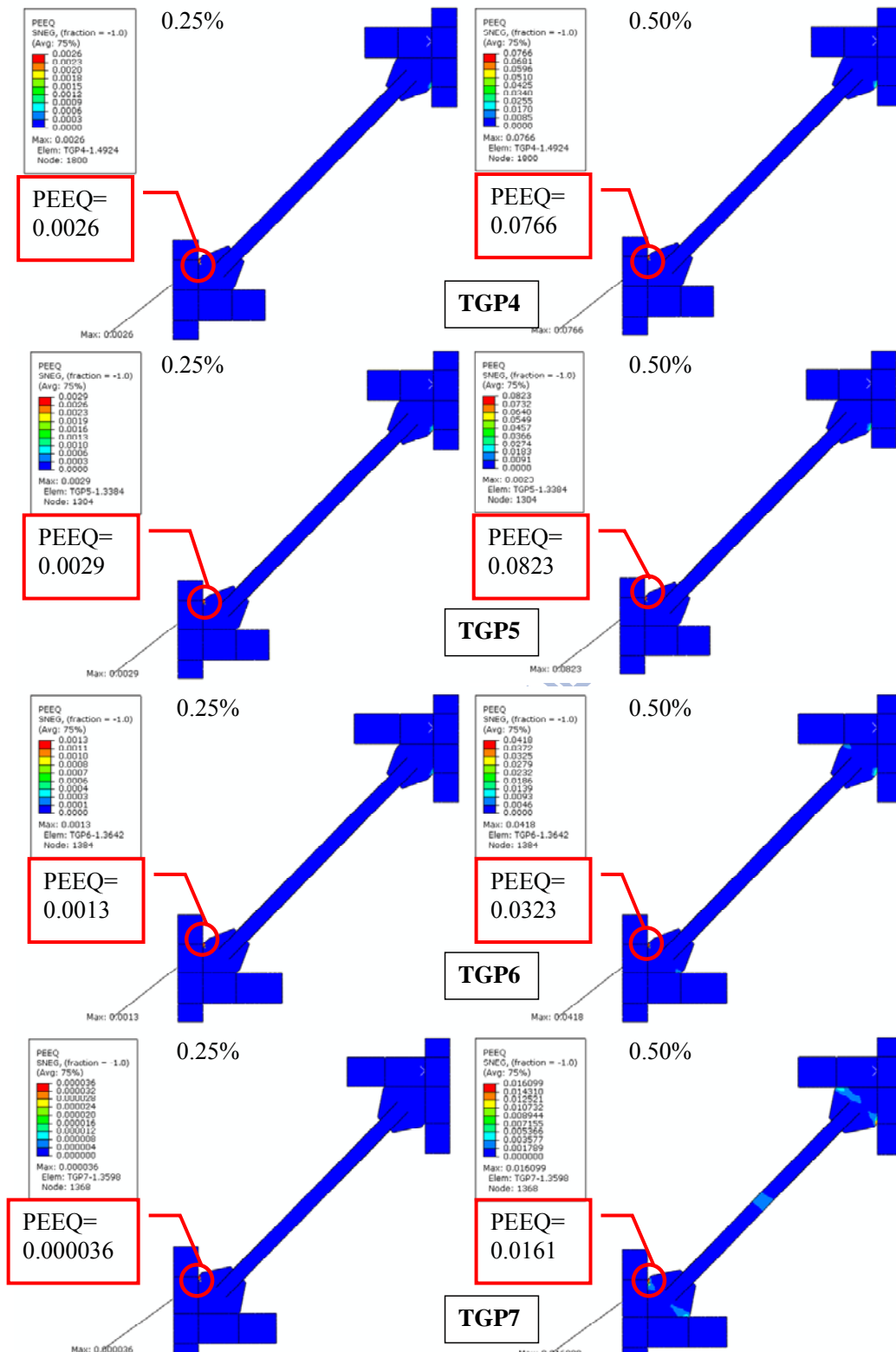
圖 3.22 模型 TGP4、模型 TGP5、模型 TGP6 與模型 TGP7 之接合板 PEEQ 分佈圖
