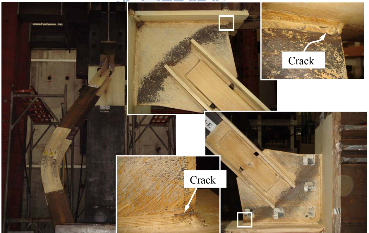
圖 4.53 試體 TGP4 最終破壞行為 (5% 弧度 IDA)
