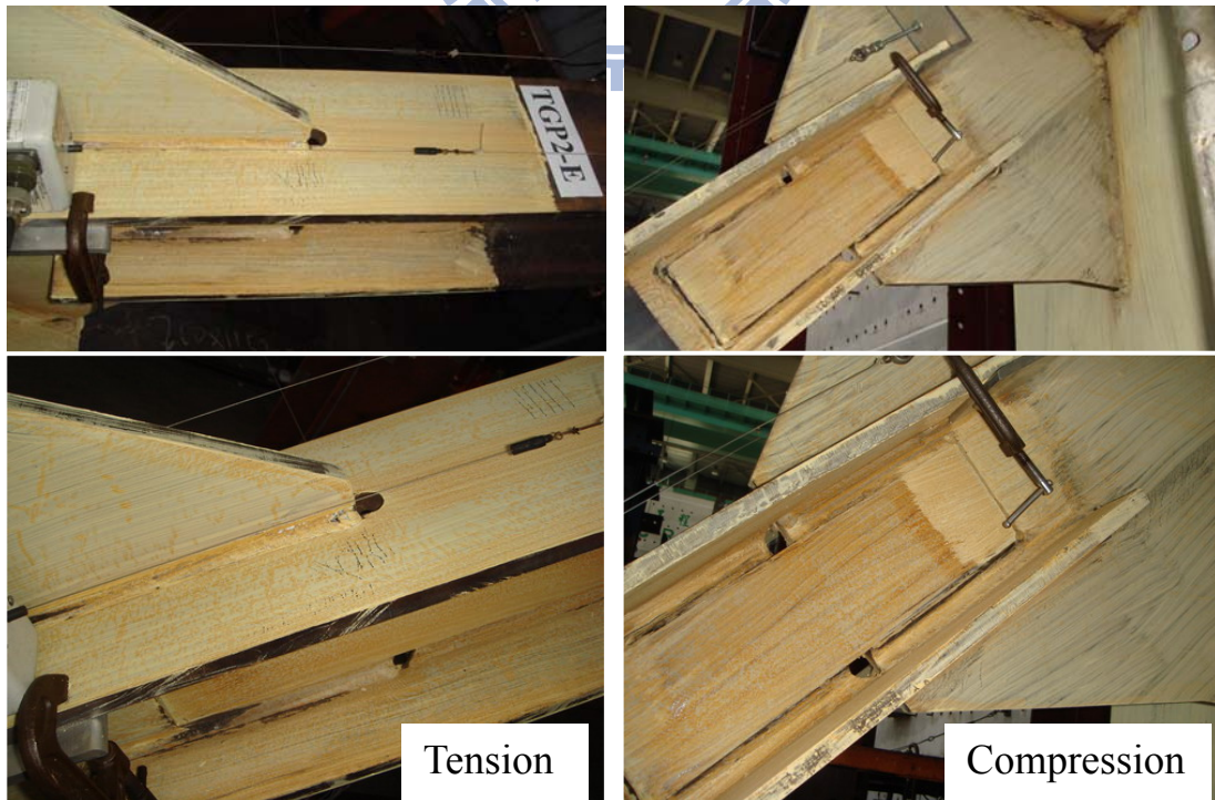
圖 4.45 斜撐與接合板之受力情況 (0.25% 弧度 IDA)
