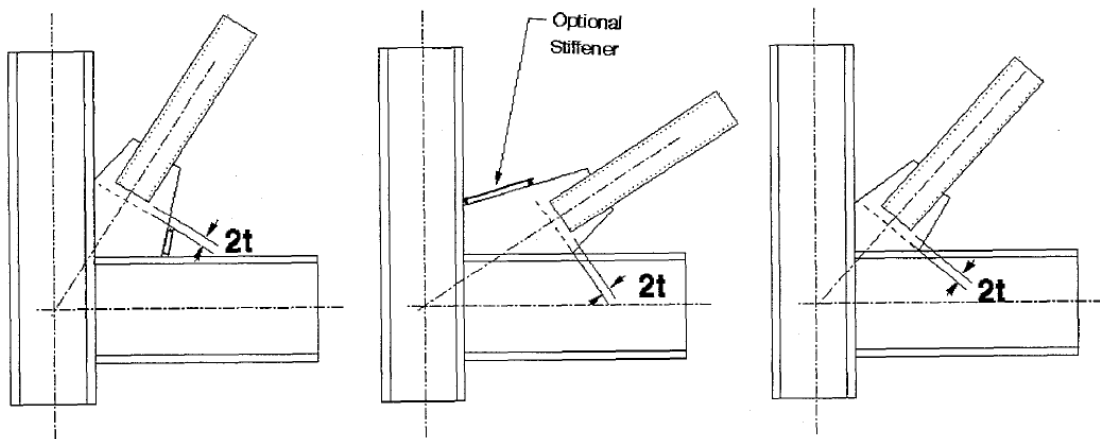
圖 2.3 接合板之 2t 設置示意圖 (Astaneh et al. 1982)
