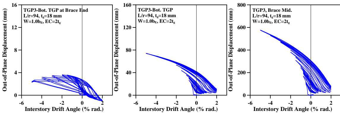
圖 4.68 試體 TGP3 斜撐端部至中央各測點之面外變形量
