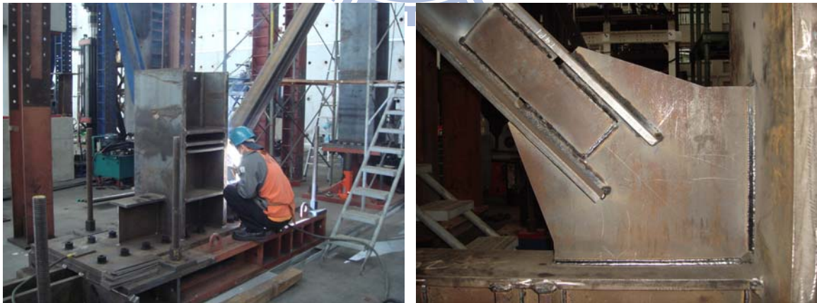
圖 4.23 接合板與梁、柱桿件模擬現地銲接施工與完成圖
