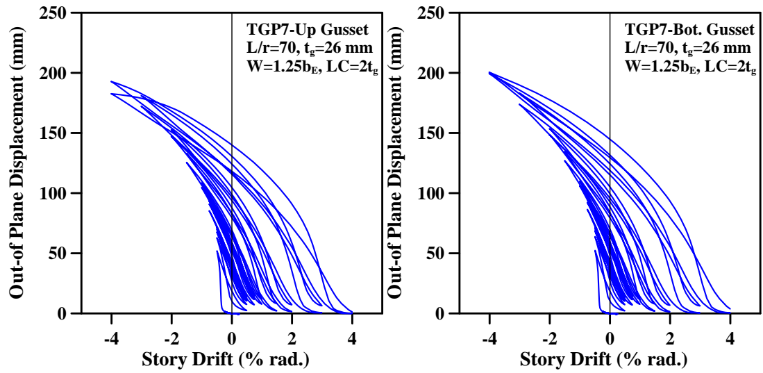
圖 3.29 參數 W 下模型 TGP7 之接合板面外變形量與層間位移角關係圖
