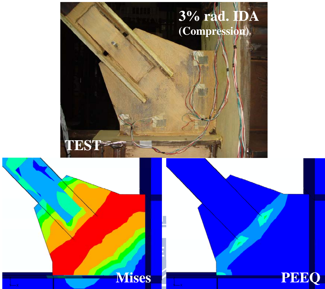
圖 5.11 試體 TGP1 之梯形接合板實驗與分析之行為比較
