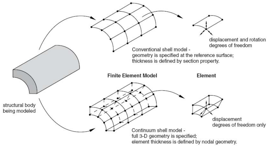
圖 3.7 ABAQUS 結構體轉置殼元素建模示意圖
