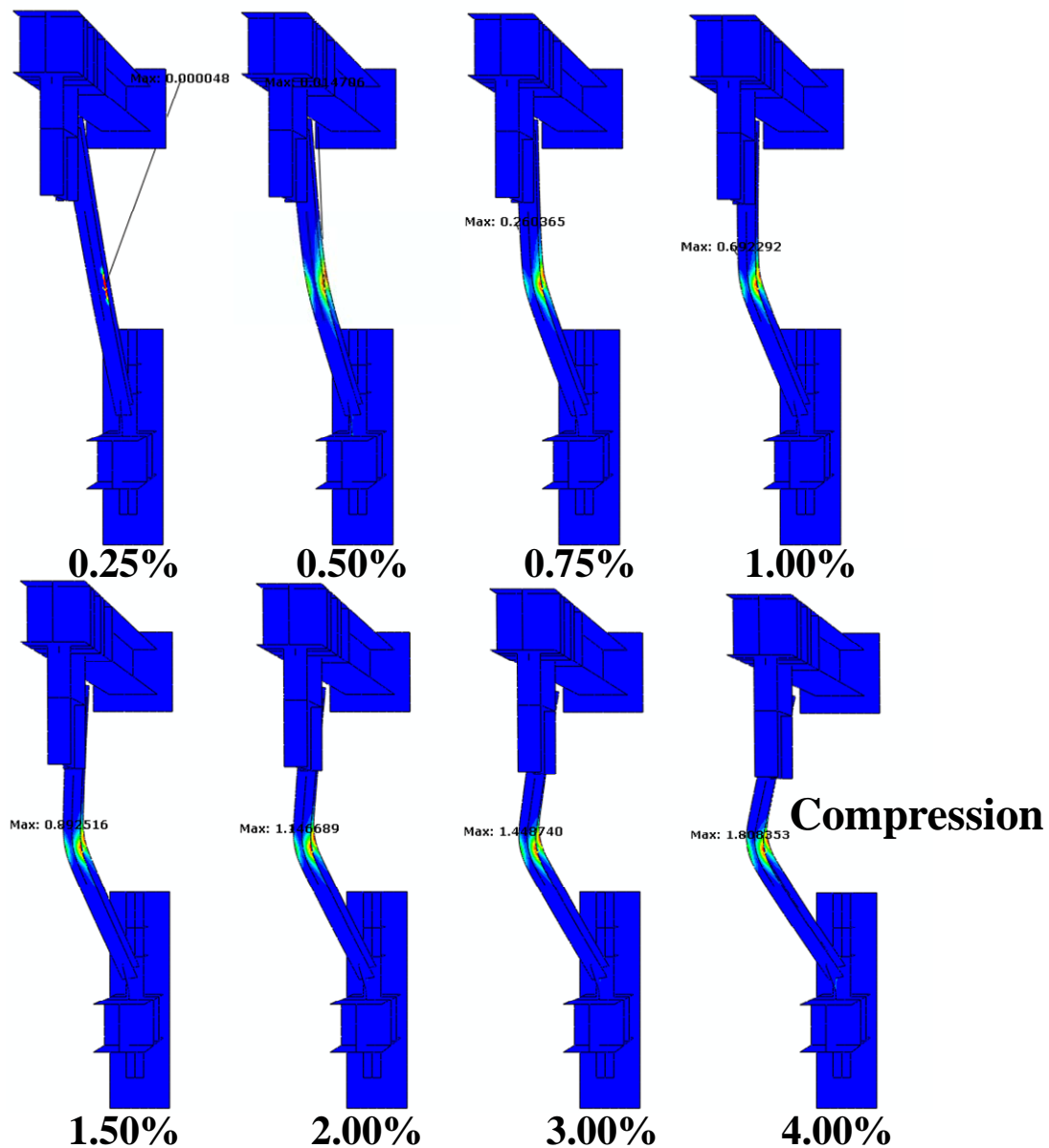
圖 5.20 試體 TGP1 數值模型斜撐構材之等值塑性應變分佈 (受壓)
