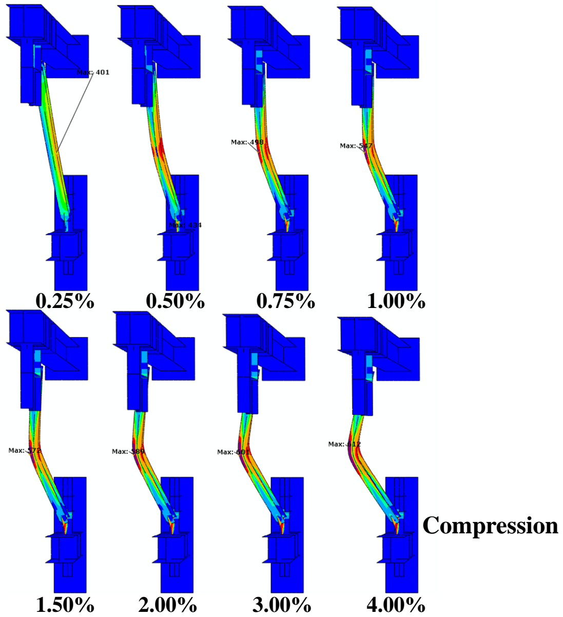
圖 5.13 試體 TGP1 之數值模型斜撐構材等值應力分佈
