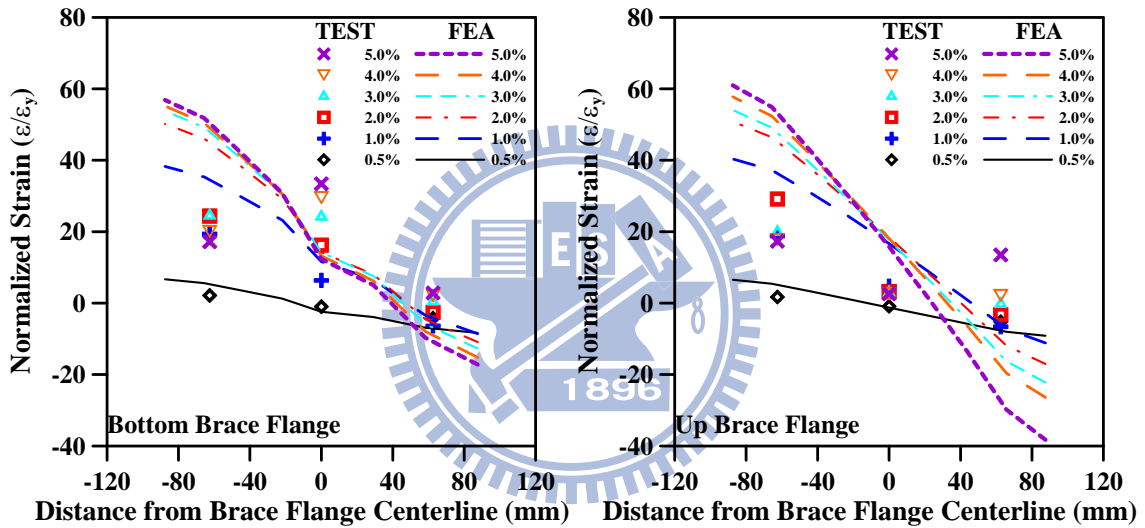
圖 5.16 試體 TGP2 斜撐中央處翼板實驗與分析之軸向應變分佈
