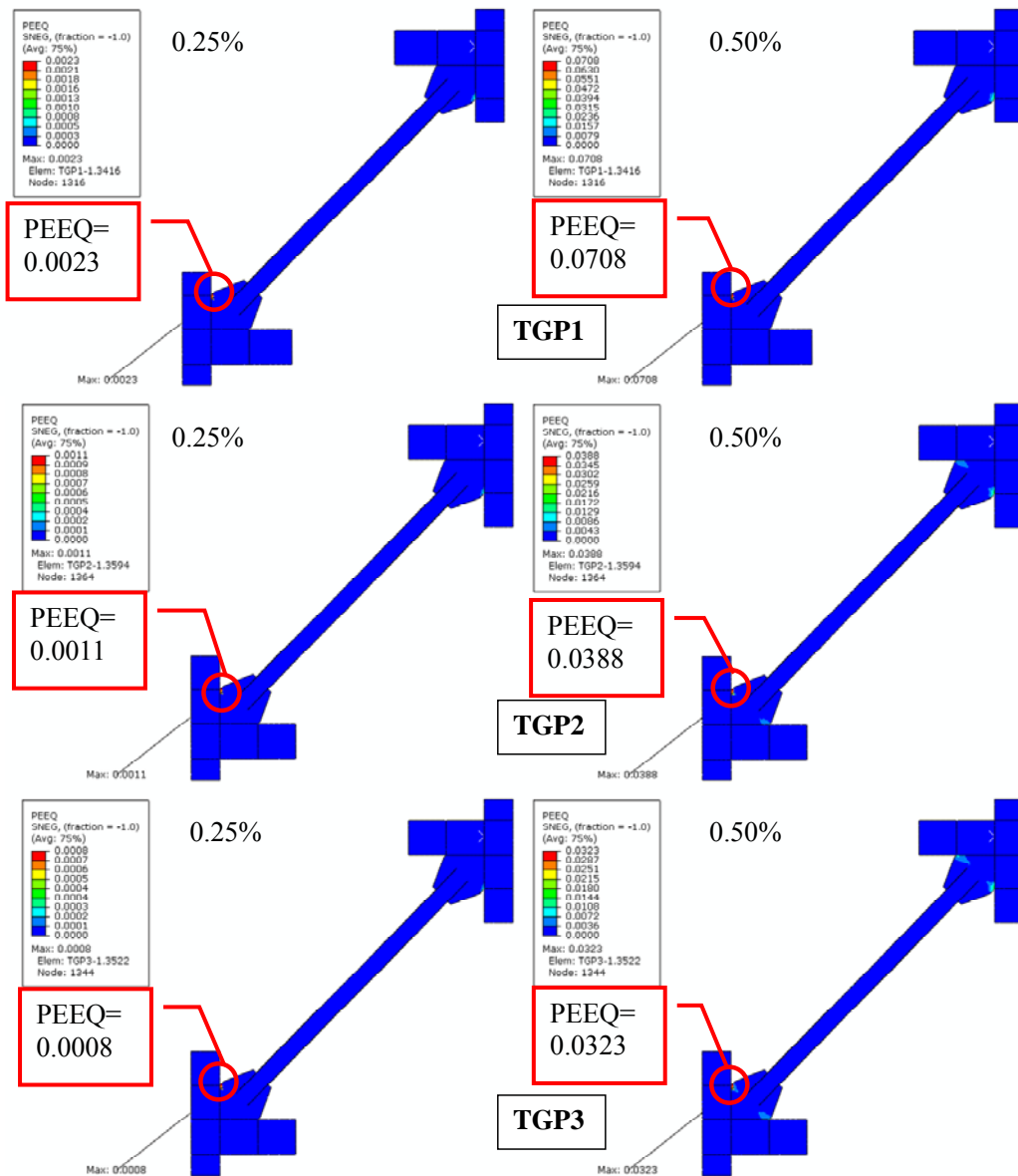
圖 3.13 模型 TGP1、模型 TGP2 與模型 TGP3 之接合板 PEEQ 分佈圖 (Compression)
