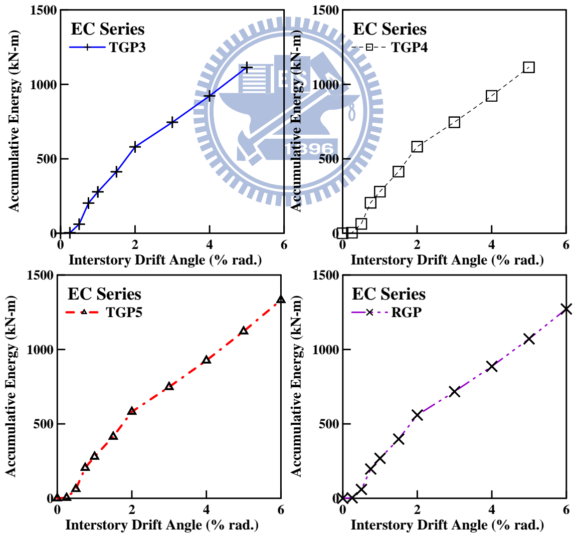
圖 4.78 4 組具 EC 之試體能量累積-層間位移角關係圖
