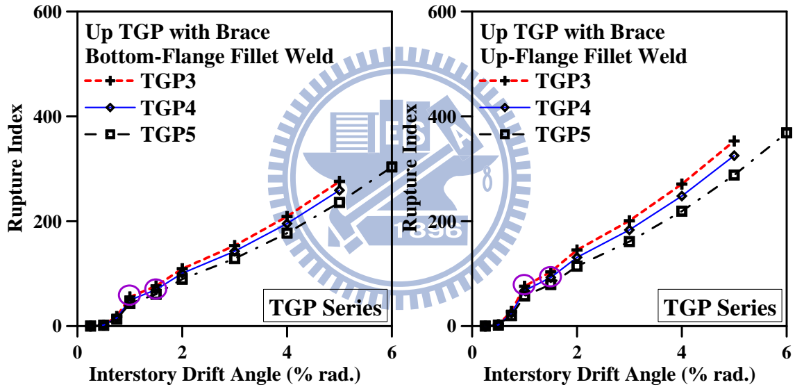
圖 5.29 與斜撐翼板填角銲道處之梯形接合板初始開裂 RI 分佈
