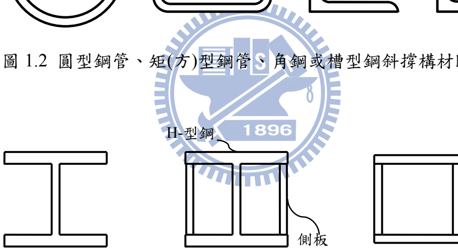
圖 1.3 H 型鋼、H 型鋼加側板與箱型斜撐構材斷面
