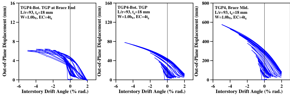
圖 4.69 試體 TGP4 斜撐端部至中央各測點之面外變形量
