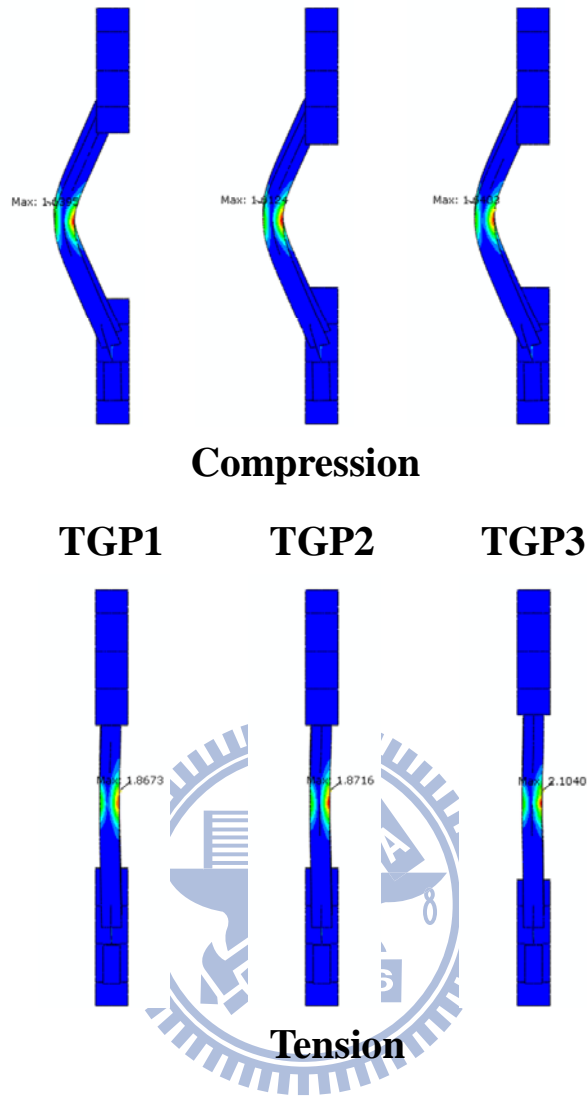
圖 3.14 模型 TGP1、模型 TGP2 與模型 TGP3 之斜撐構材 PEEQ 分佈圖
