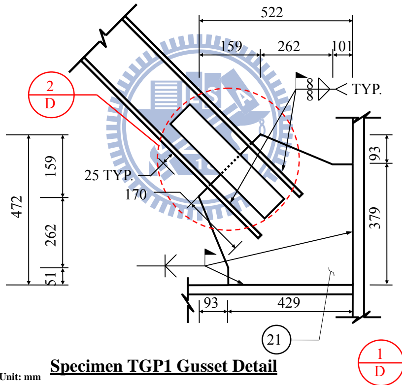
圖 4.11 試體 TGP1 接合板接合細部圖
