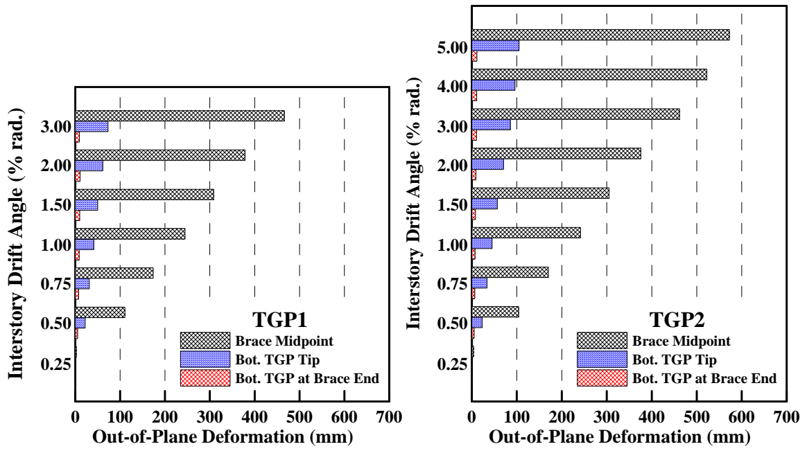
圖 4.72 試體 TGP1 與試體 TGP2 之各測點面外變形量變化
