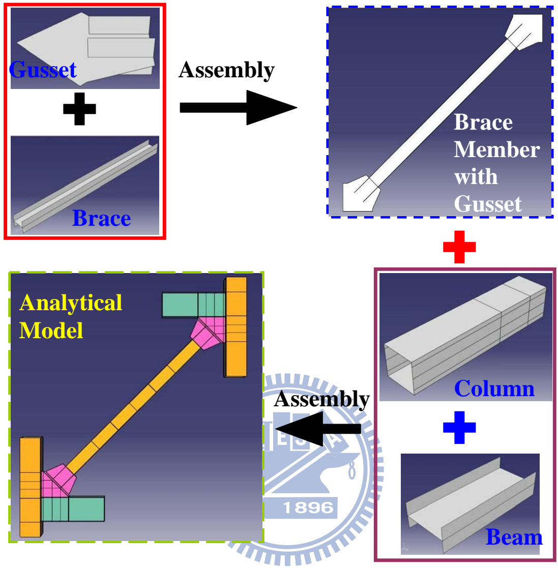
圖 3.2 分析模型組裝之步驟
