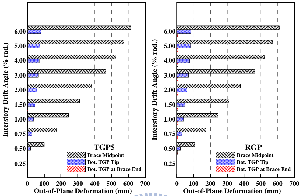
圖 4.74 試體 TGP5 與試體 RGP 之各測點面外變形量變化
