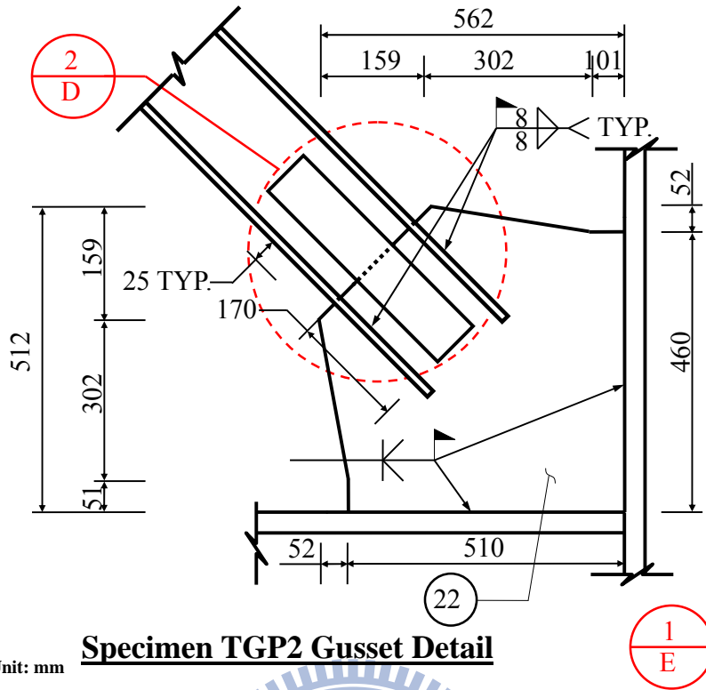
圖 4.14 試體 TGP2 接合板接合細部圖
