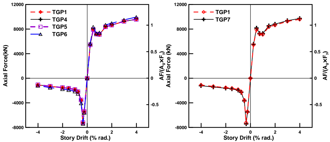
圖 3.26 4 組模型之強度包絡線圖 (參數 LC 與 W )
