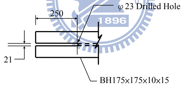
圖 4.12 梯形接合板與斜撐構材之淨斷面加勁細部
