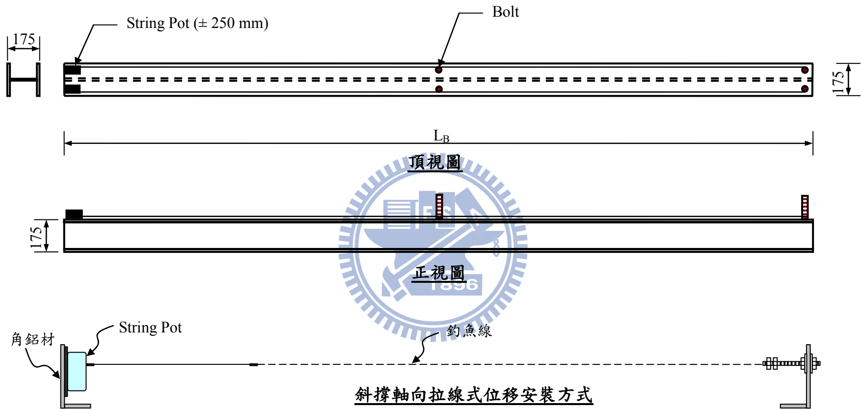
圖 4.33 斜撐軸向變形之拉線式位移計設置圖
