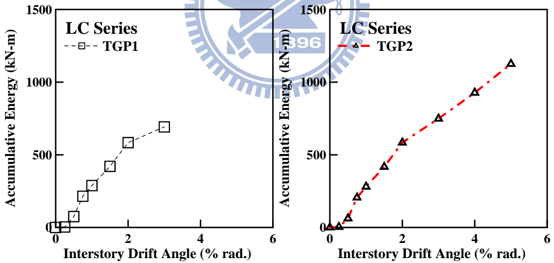
圖 4.76 試體 TGP1 與試體 TGP2 能量累積-層間位移角關係圖
