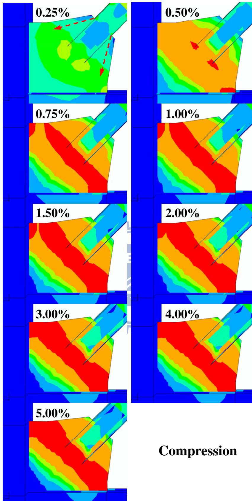
圖 5.19 試體 TGP2 之數值模型於梯形接合板等值應力分佈
