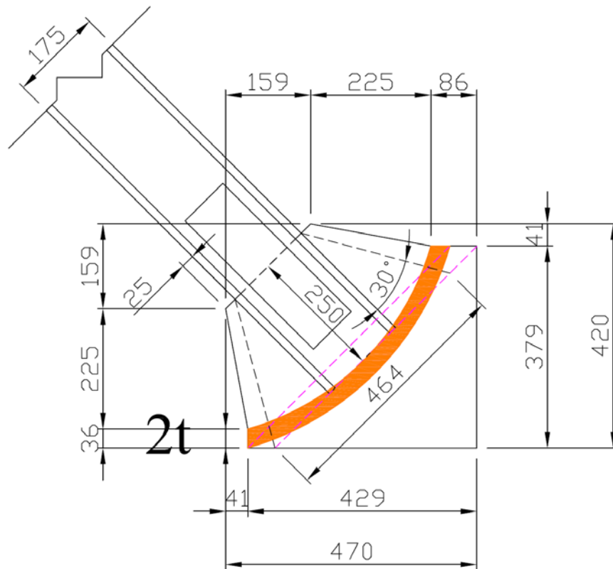
圖 4.4 試體 TGP3 接合板尺寸圖
