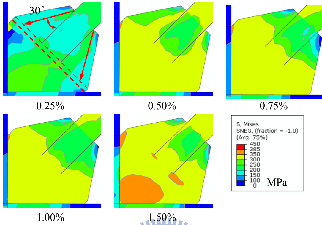
圖 3.21 模型 TGP7 之等值應力分佈圖
