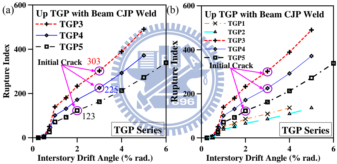
圖 5.27 與梁接合開槽銲道處之梯形接合板初始開裂 RI 分佈
