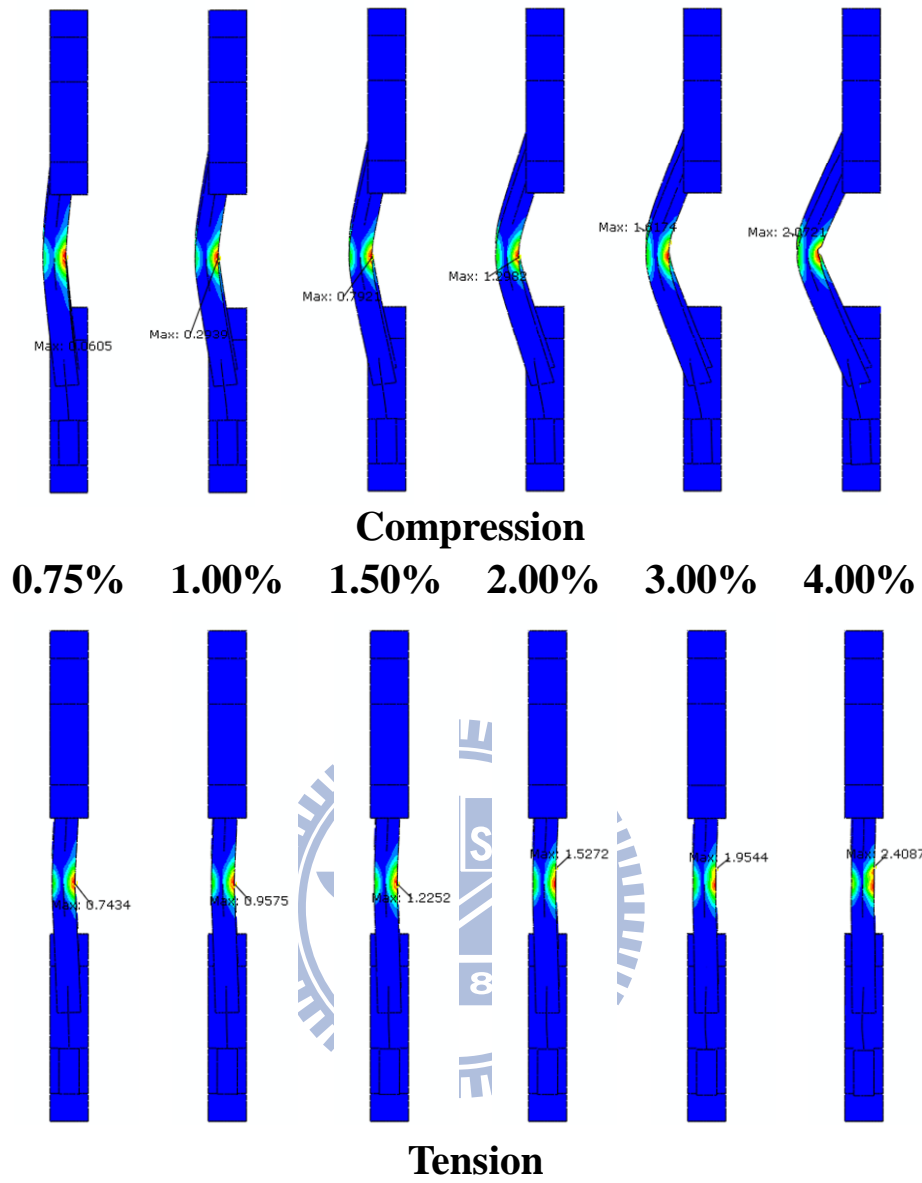
圖 3.32 模型 RGP 斜撐構材 PEEK
