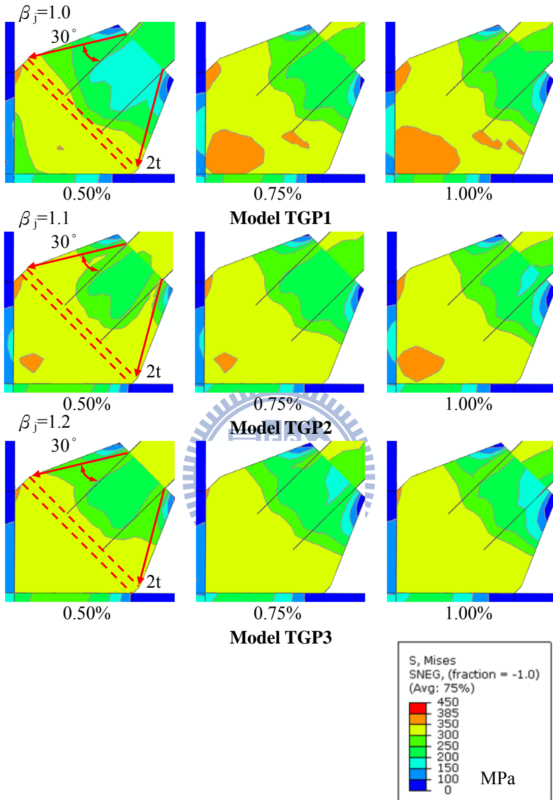
圖 3.12 模型 TGP1、模型 TGP2 與模型 TGP3 之等值應力分佈圖
