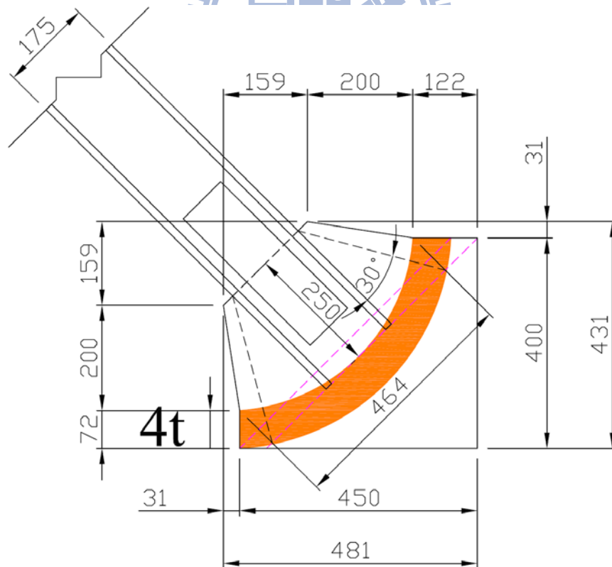
圖 4.5 試體 TGP4 接合板尺寸圖
