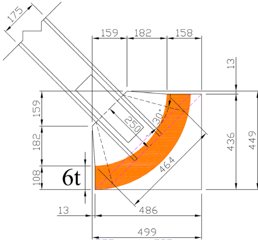
圖 4.6 試體 TGP5 接合板尺寸圖
