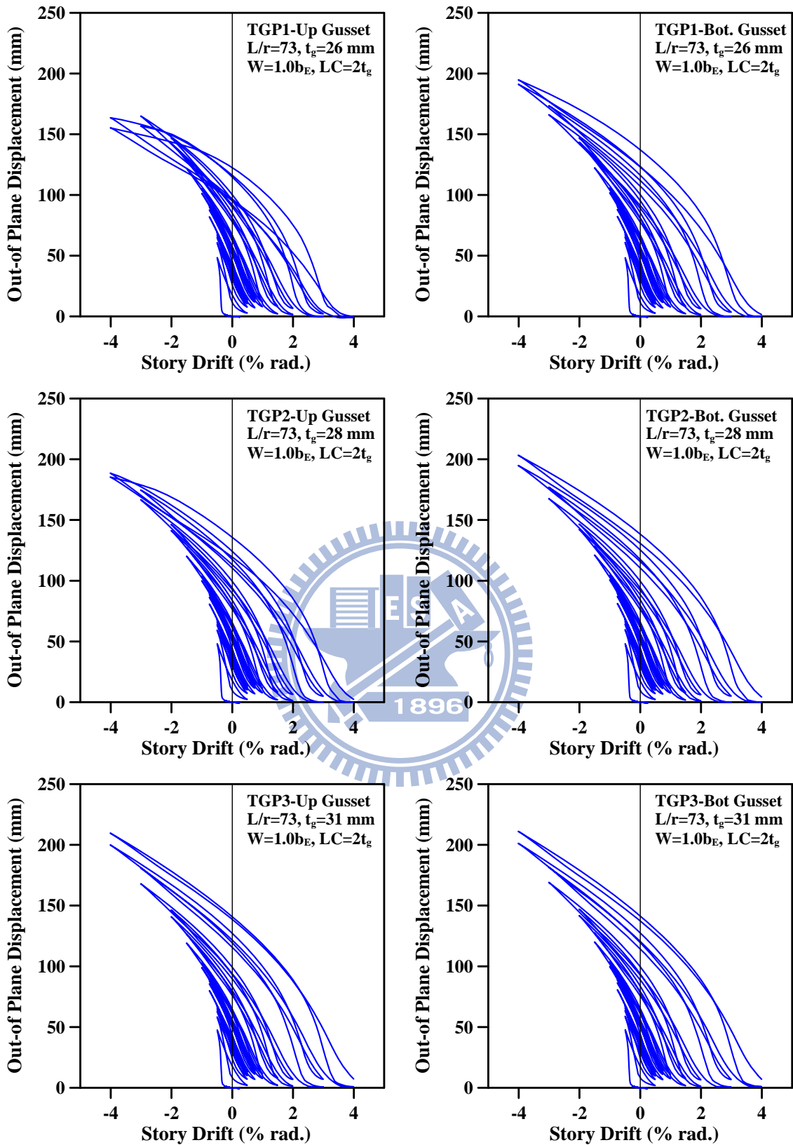
圖 3.19 參數 \beta_j 下 3 組模型之接合板面外變形量與層間位移角關係圖
