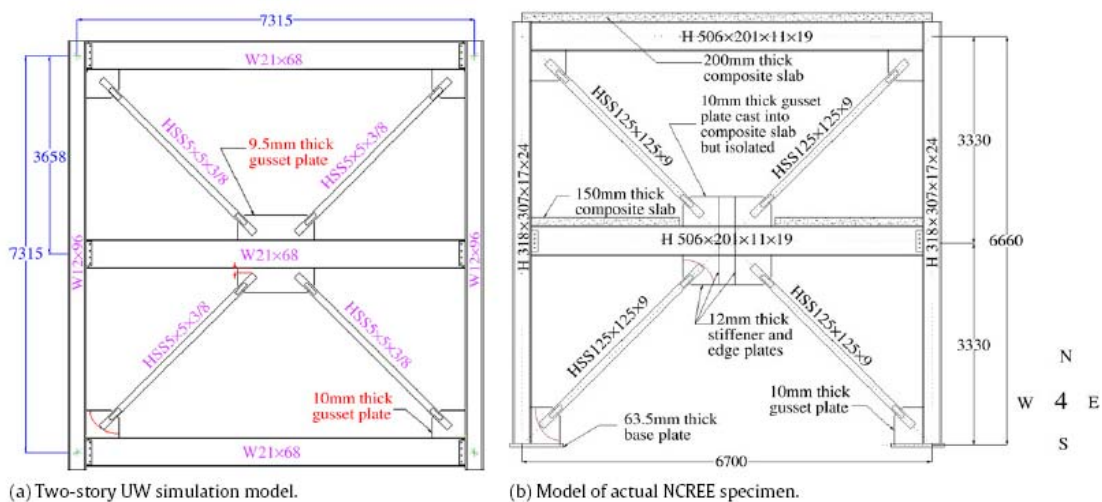
圖 2.8 二層樓 X 型斜撐構架圖
