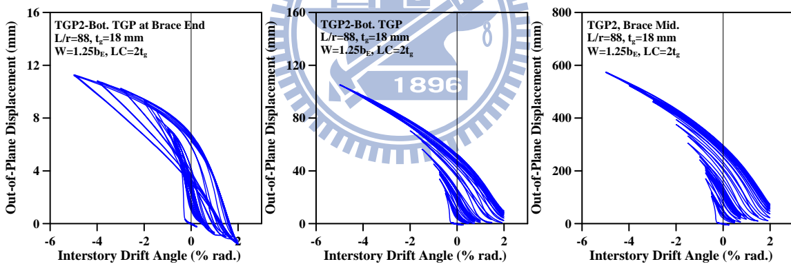
圖 4.67 試體 TGP2 斜撐端部至中央各測點之面外變形量
