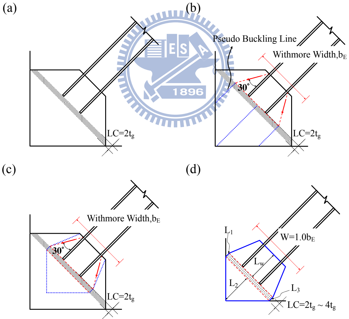
圖 2.23 梯形接合板之設計概念
