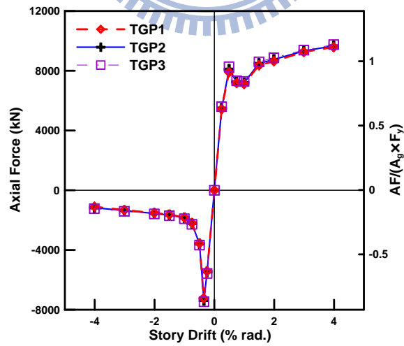
圖 3.17 3 組模型之強度包絡線圖 (參數 \beta_j )
