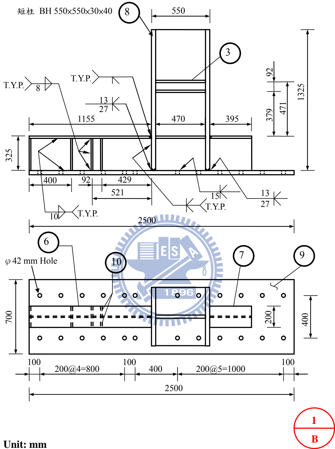
圖 4.28 試驗試體基座設計圖
