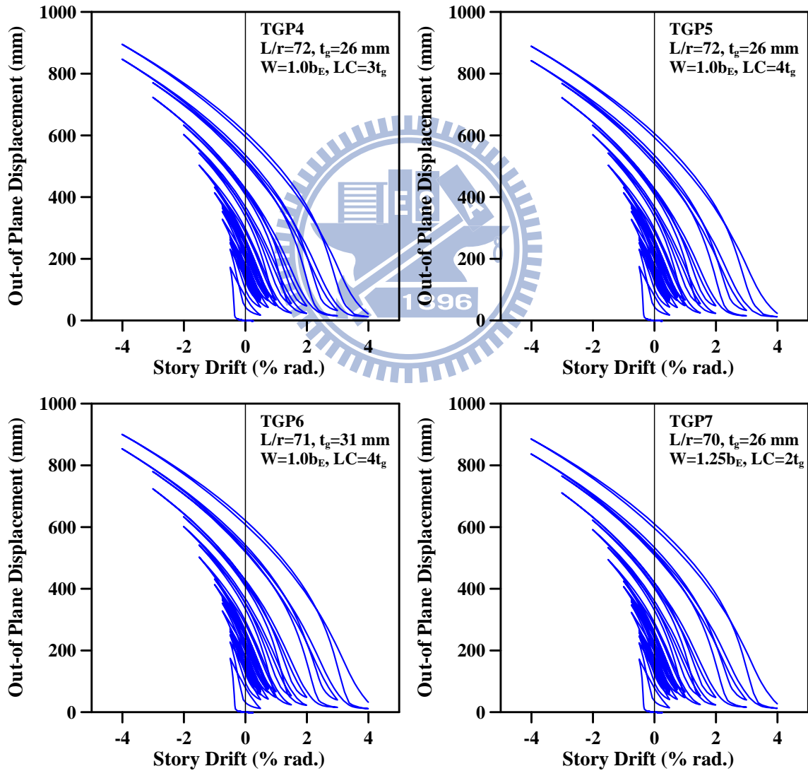
圖 3.27 參數 LC 與 W 下 4 組模型之斜撐構材面外變形量與層間位移角關係圖
