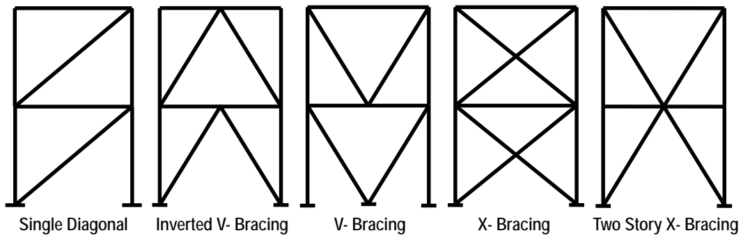
圖 1.1 一般常見的同心斜撐構架型式
