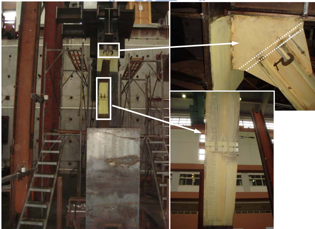
圖 4.40 斜撐中央與接合板凹折區域之石膏剝落情形 (0.75% 弧度 IDA)
