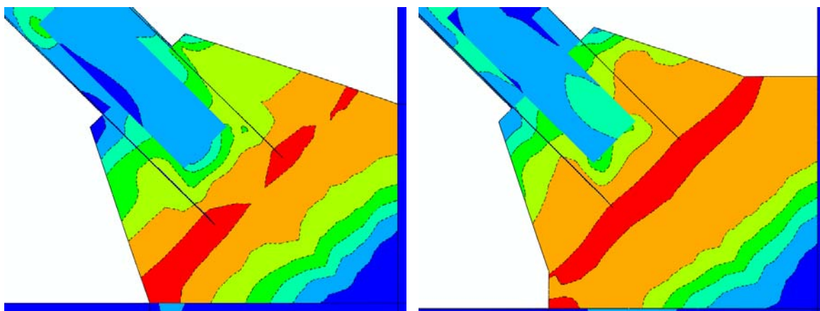
圖 3.37 採錐形與梯形接合板之等值應力圖
