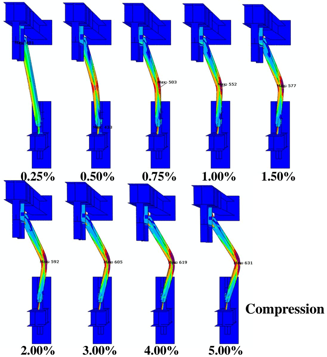
圖 5.14 試體 TGP2 之數值模型斜撐構材等值應力分佈
