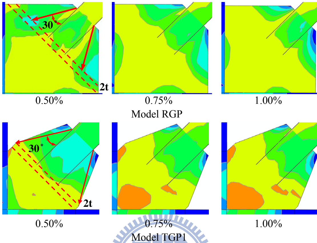
圖 3.30 模型 RGP 與模型 TGP1 之等值應力分佈圖
