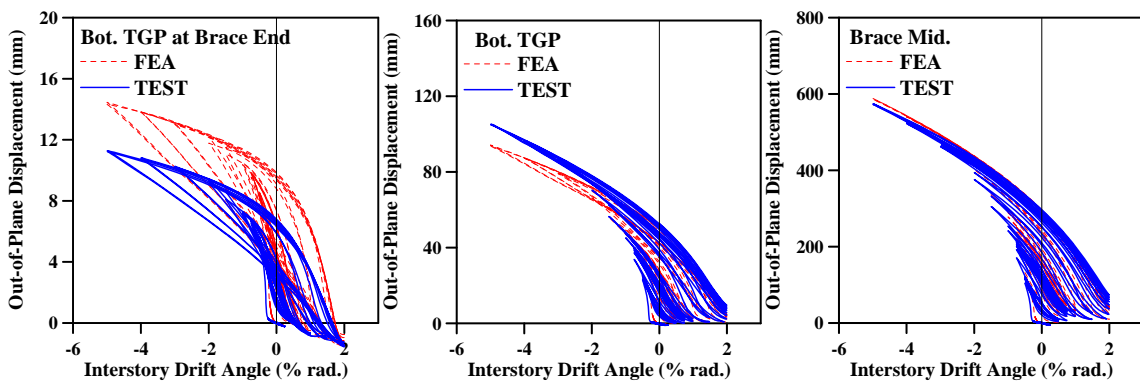
圖 5.6 試體 TGP2 實驗與分析之各測點面外變形量-層間位移關係圖比較
