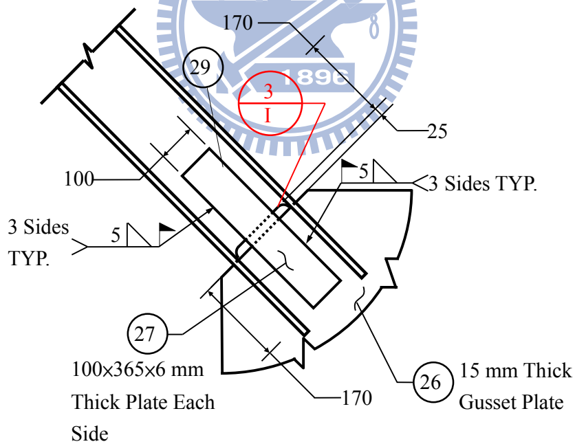
圖 4.18 試體 RGP 合板接合細部圖
