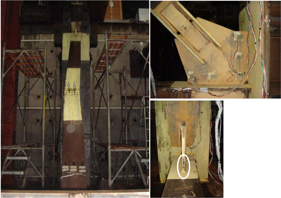
圖 4.43 試體 TGP1 最終變形情況 (3% 弧度 IDA)
