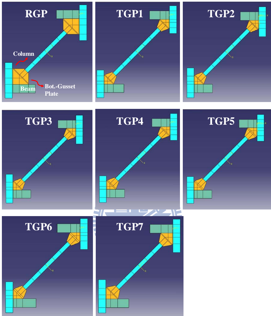
圖 3.10 8 組有限分析模型
