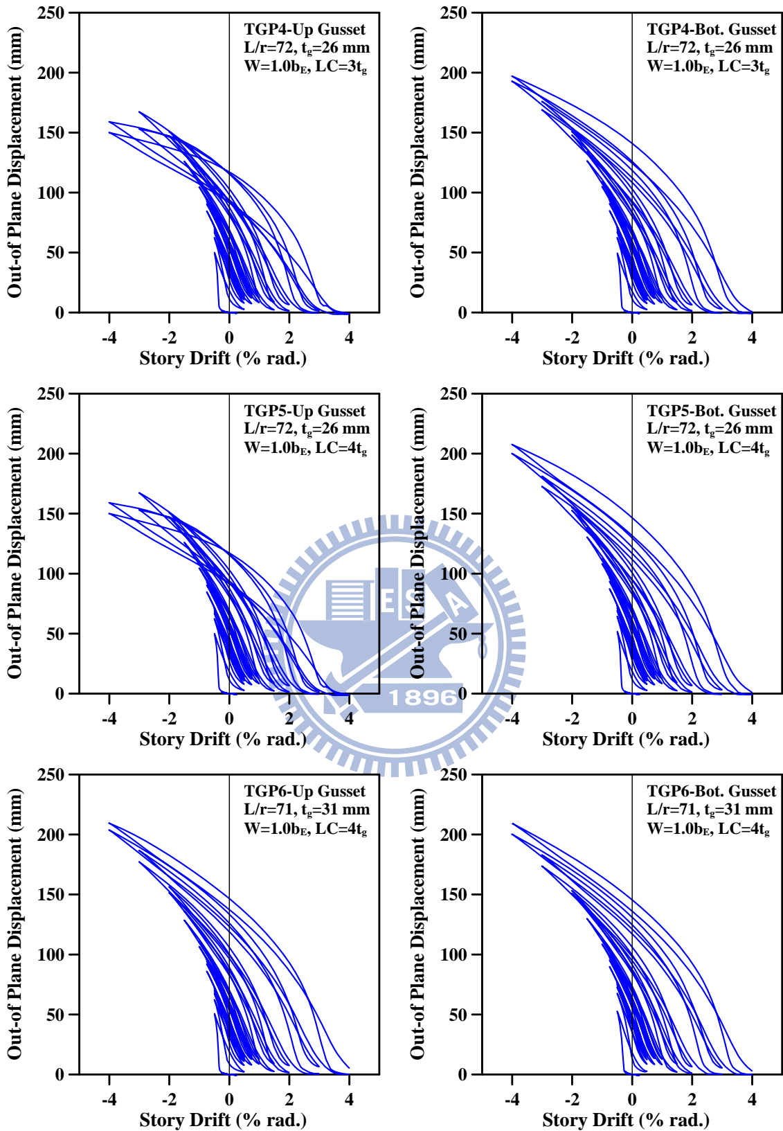
圖 3.28 參數 LC 下 3 組模型之接合板面外變形量與層間位移角關係圖
