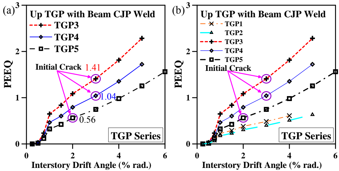
圖 5.26 與梁接合開槽銲道處之梯形接合板初始開裂 PEEQ 分佈
