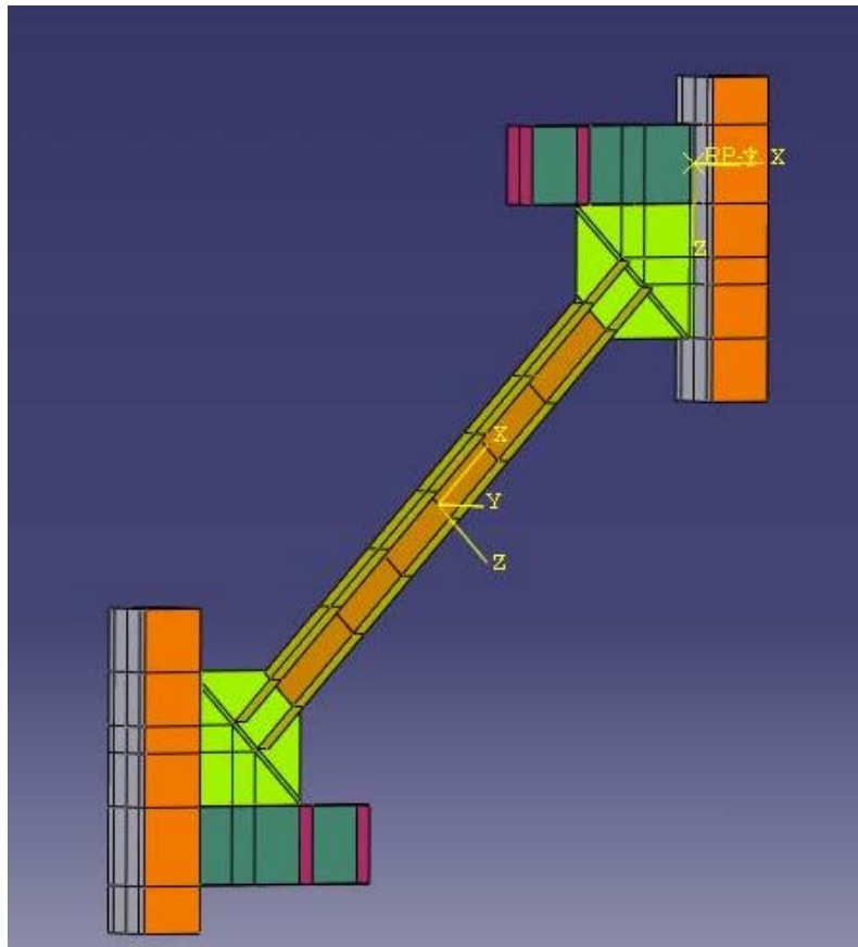
圖 3.1 斜撐構材含接合板之分析模型
