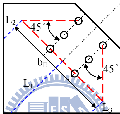
圖 2.16 Modified Thornton Method 有效寬度示意圖
