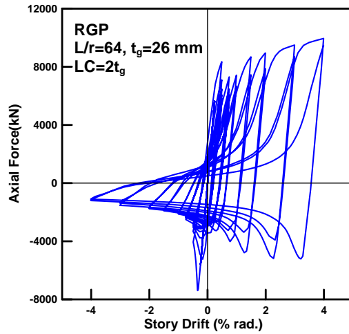
圖 3.33 模型 RGP 之軸向載重與層間位移角關係圖 (接合板形狀影響)
