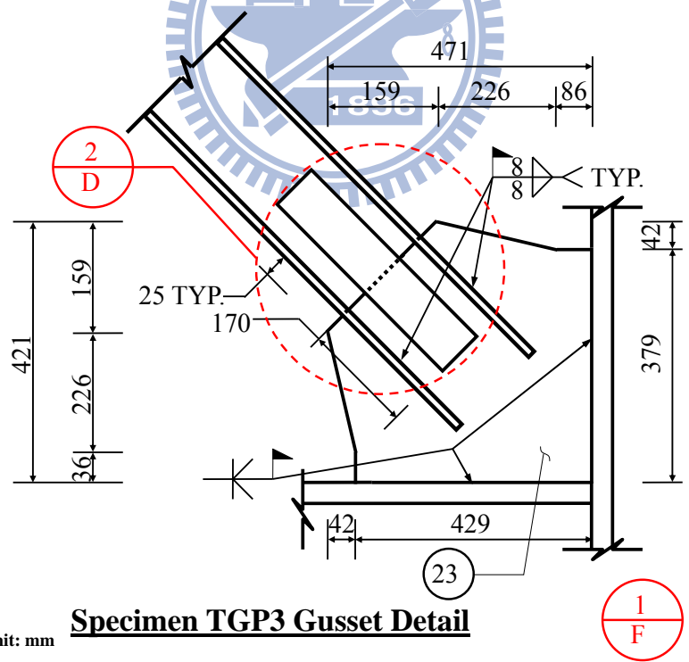
圖 4.15 試體 TGP3 接合板接合細部圖
