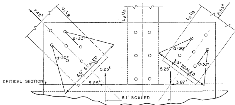
圖 2.12 接合板有效寬度之概念 (Whitmore 1952)
