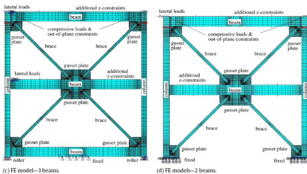
圖 2.9 斜撐構架之分析模型 (Yoo et al. 2009)
