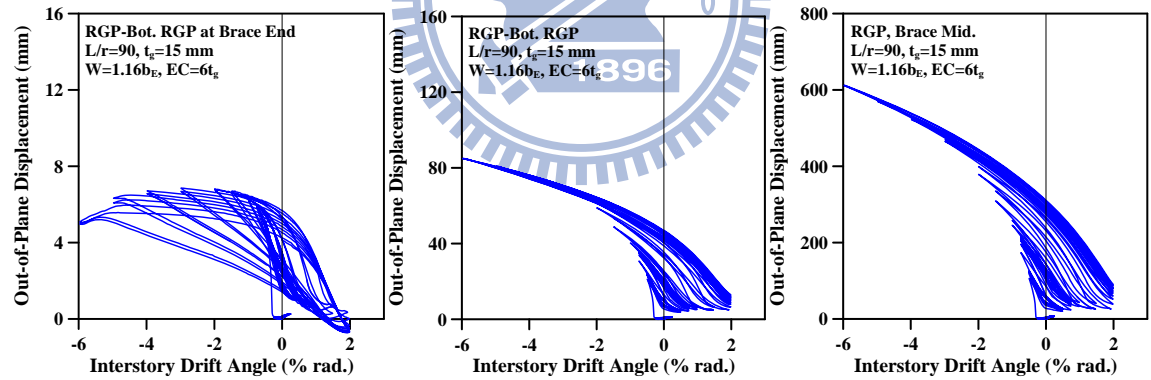
圖 4.71 試體 RGP 斜撐端部至中央各測點之面外變形量
