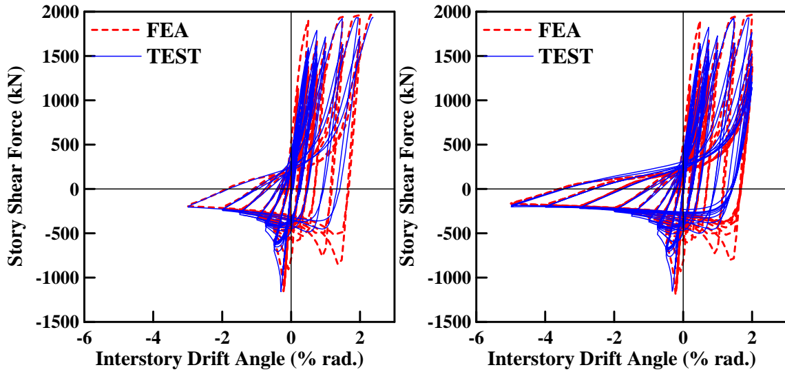
圖 5.4 試體 TGP1 與試體 TGP2 實驗與分析之層間剪力-層間位移關係圖比較
