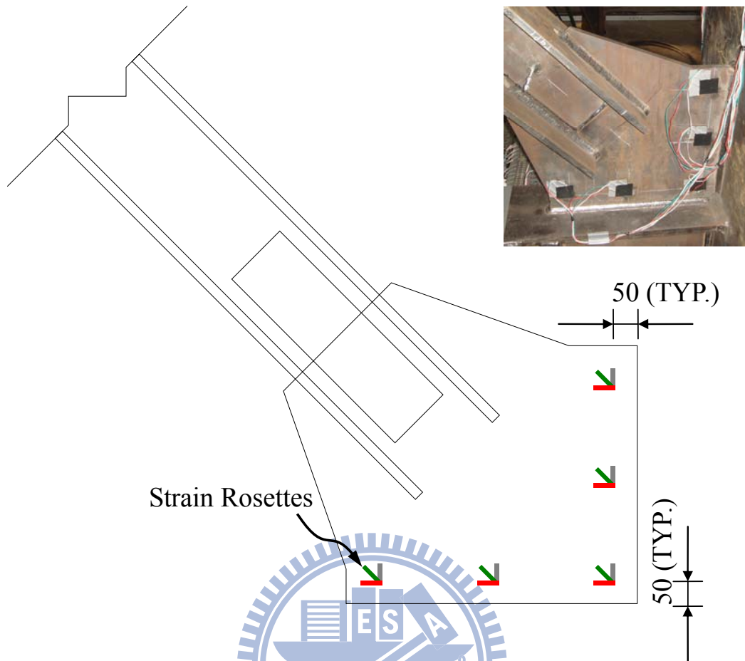
圖 4.37 接合板之 3 軸應變計黏貼位置圖
