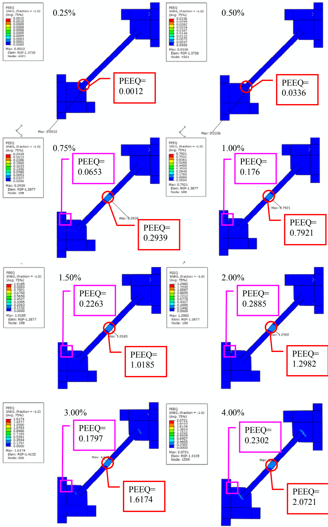
圖 3.31 模型 RGP 之 PEEQ 分佈圖 (Compression)
