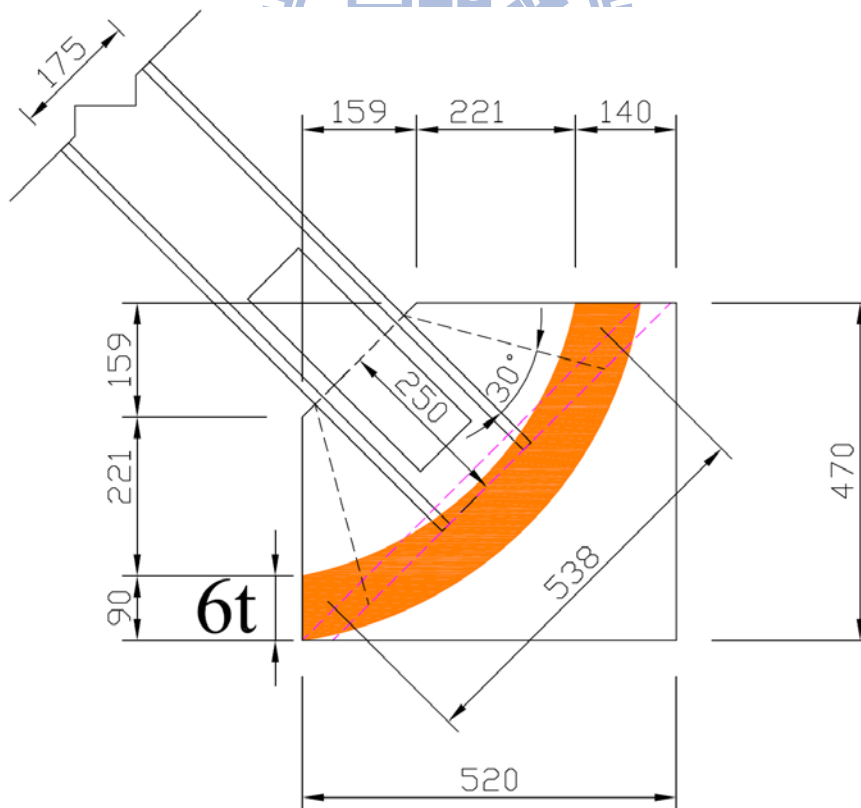
圖 4.7 試體 RGP 接合板尺寸圖
