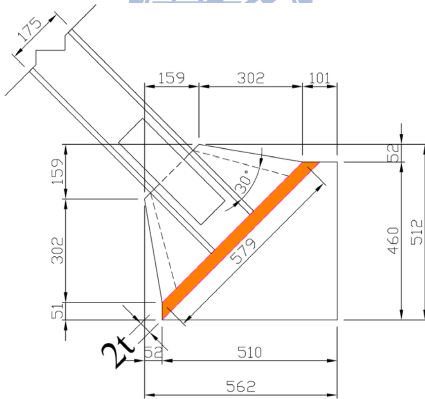
圖 4.3 試體 TGP2 接合板尺寸圖
