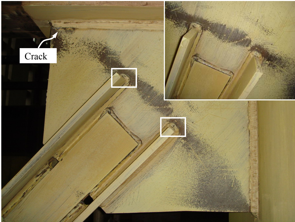
圖 4.56 上接合板於應力集中處之母材開裂情形 (1.5% 弧度 IDA)
