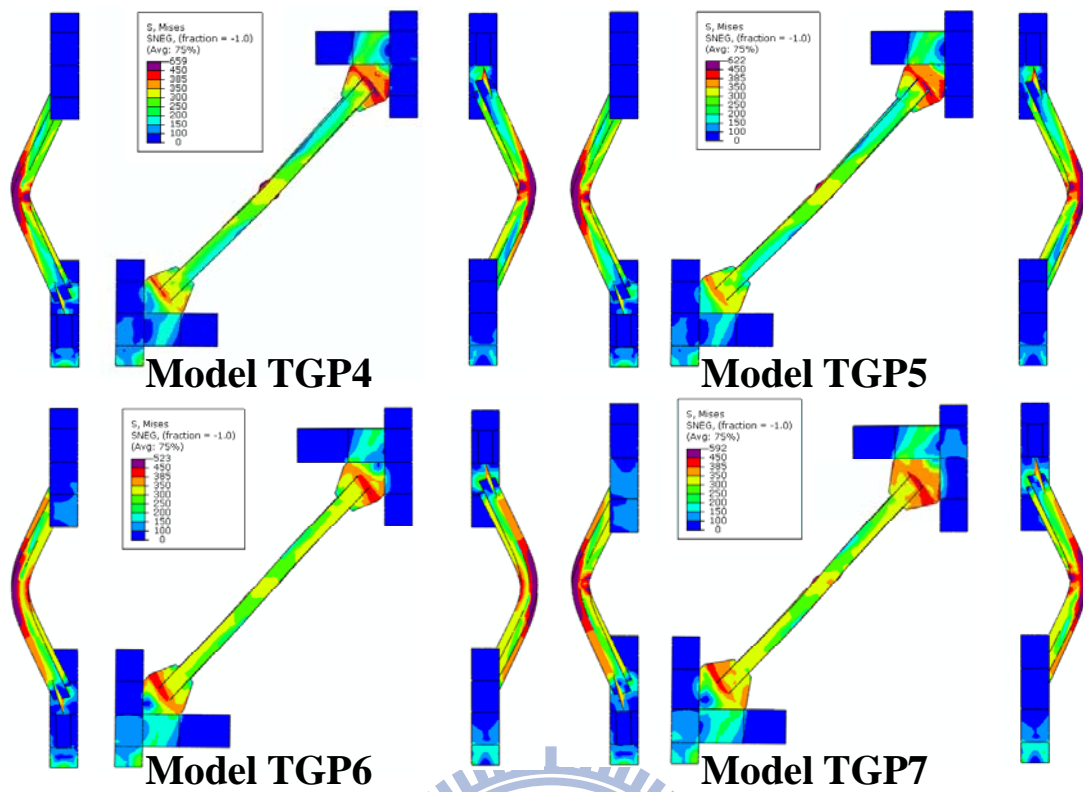
圖 3.24 4 組模型之挫屈行為 (參數 LC 與 W )
