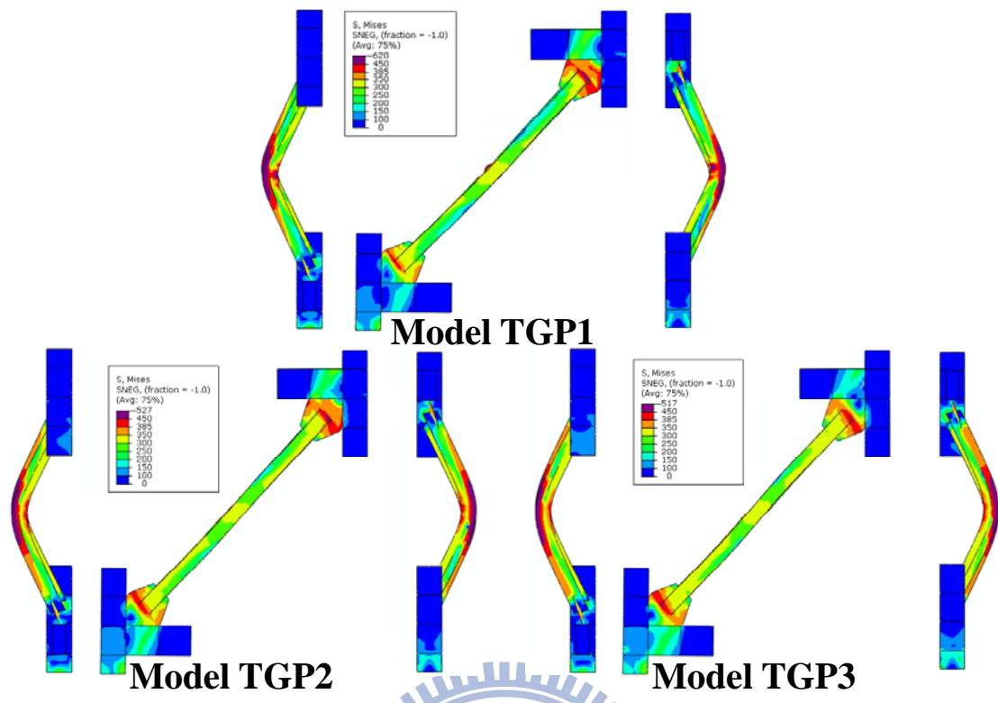
圖 3.15 3 組模型之挫屈行為 (參數 \beta_j )
