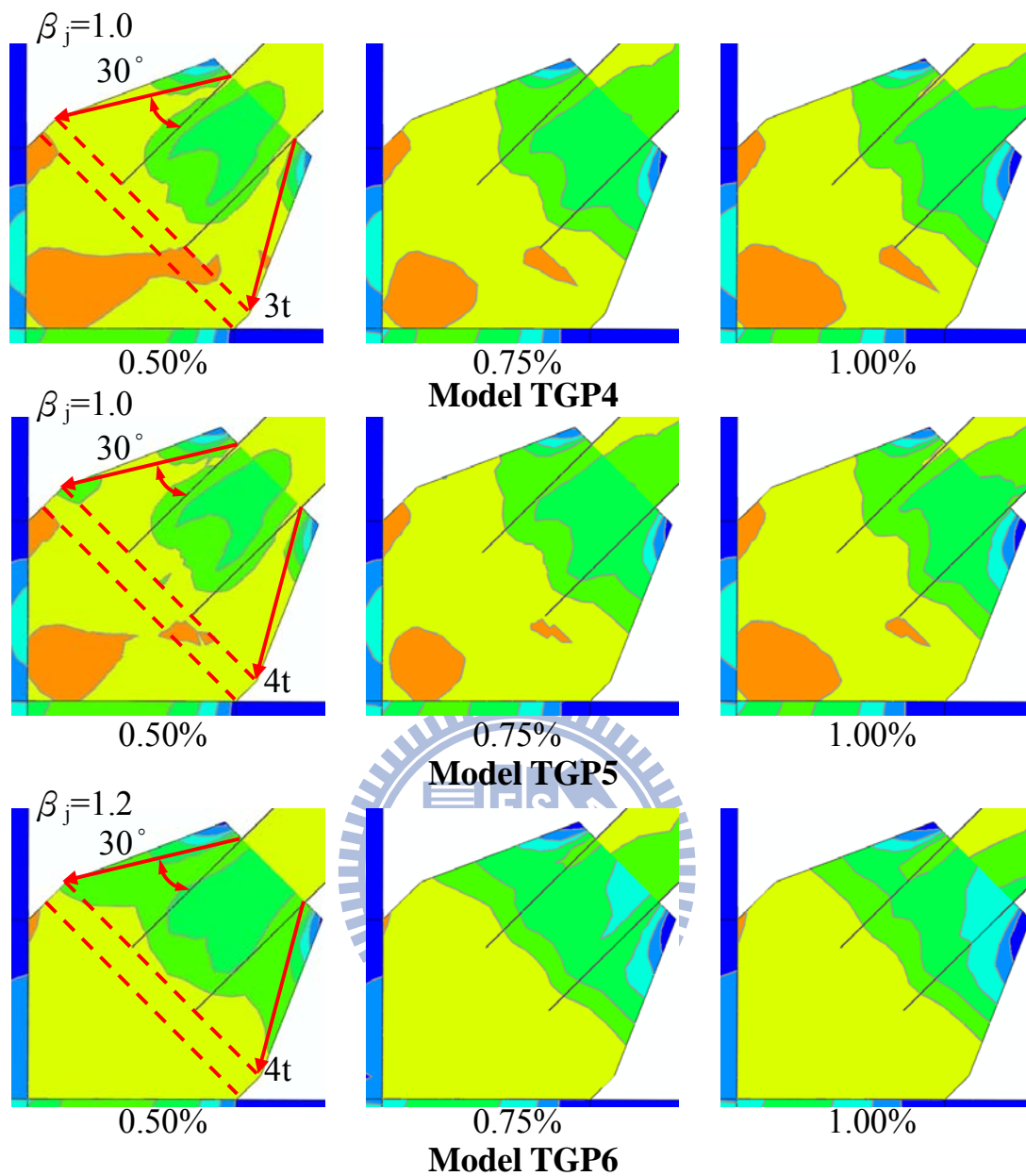
圖 3.20 模型 TGP4、模型 TGP5 與模型 TGP6 之等值應力分佈圖
