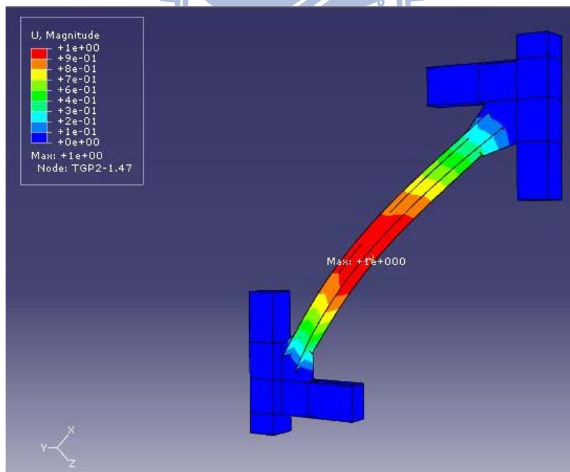
圖 3.6 模型挫屈模態分析結果 (Mode 1)
