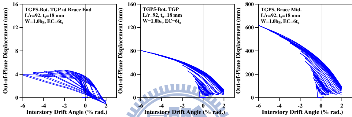
圖 4.70 試體 TGP5 斜撐端部至中央各測點之面外變形量
