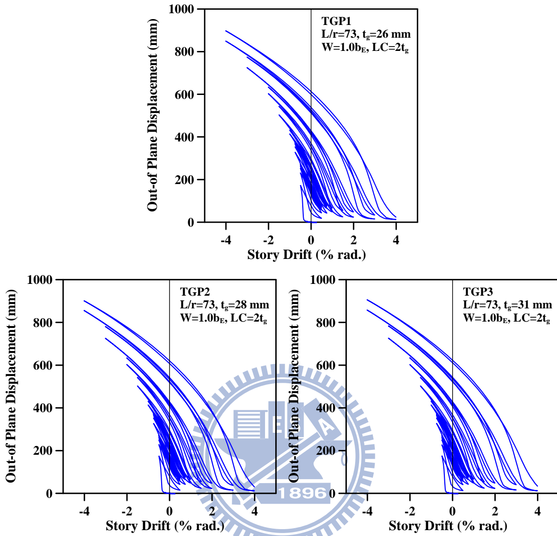
圖 3.18 參數 \beta_j 下 3 組模型之斜撐構材面外變形量與層間位移角關係圖
