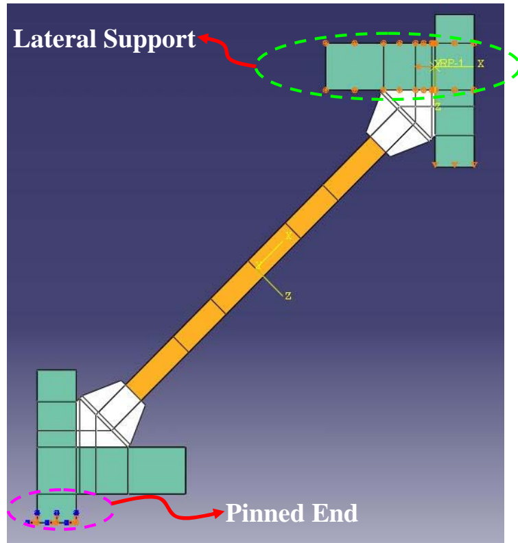
圖 3.5 模型之邊界與載重施載
