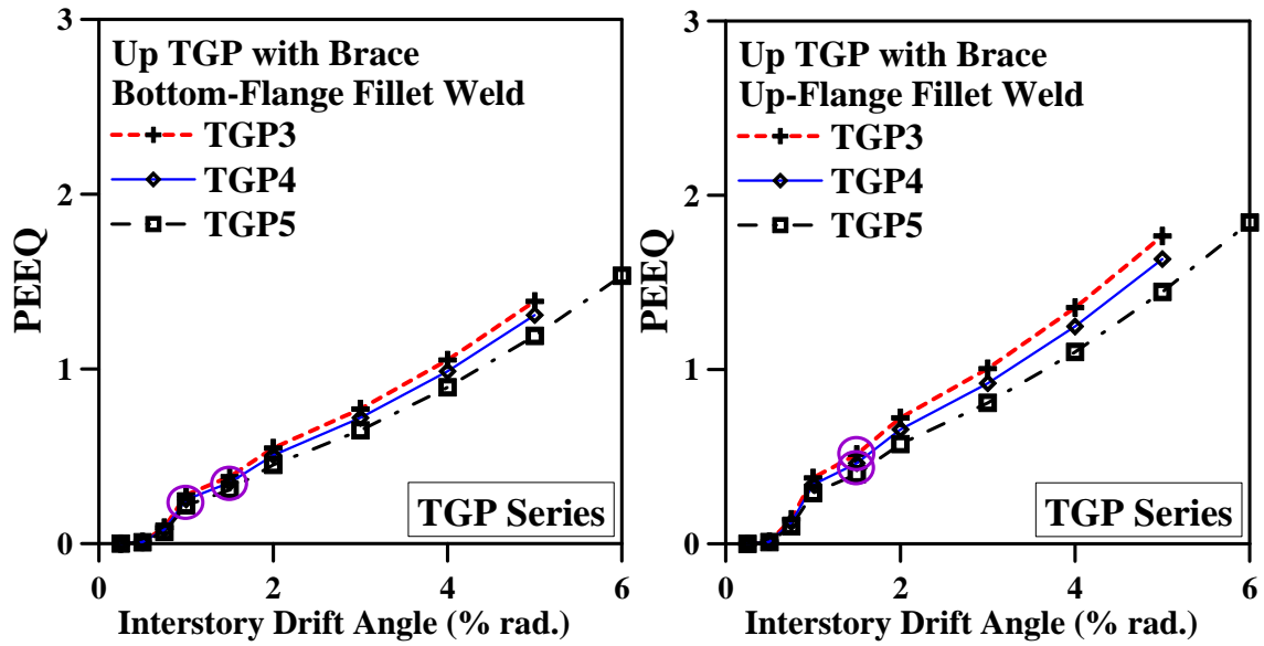
圖 5.28 與斜撐翼板填角銲道處之梯形接合板初始開裂 PEEQ 分佈
