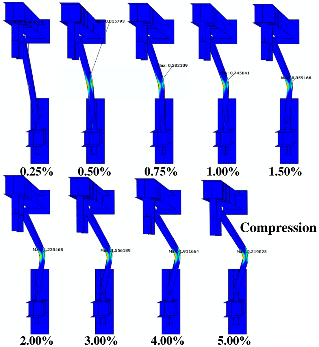
圖 5.22 試體 TGP2 數值模型斜撐構材之等值塑性應變分佈 (受壓)
