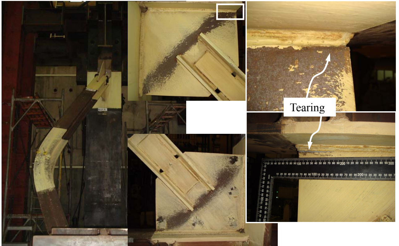
圖 4.60 試體 RGP 最終破壞行為 (6% 弧度 IDA)
