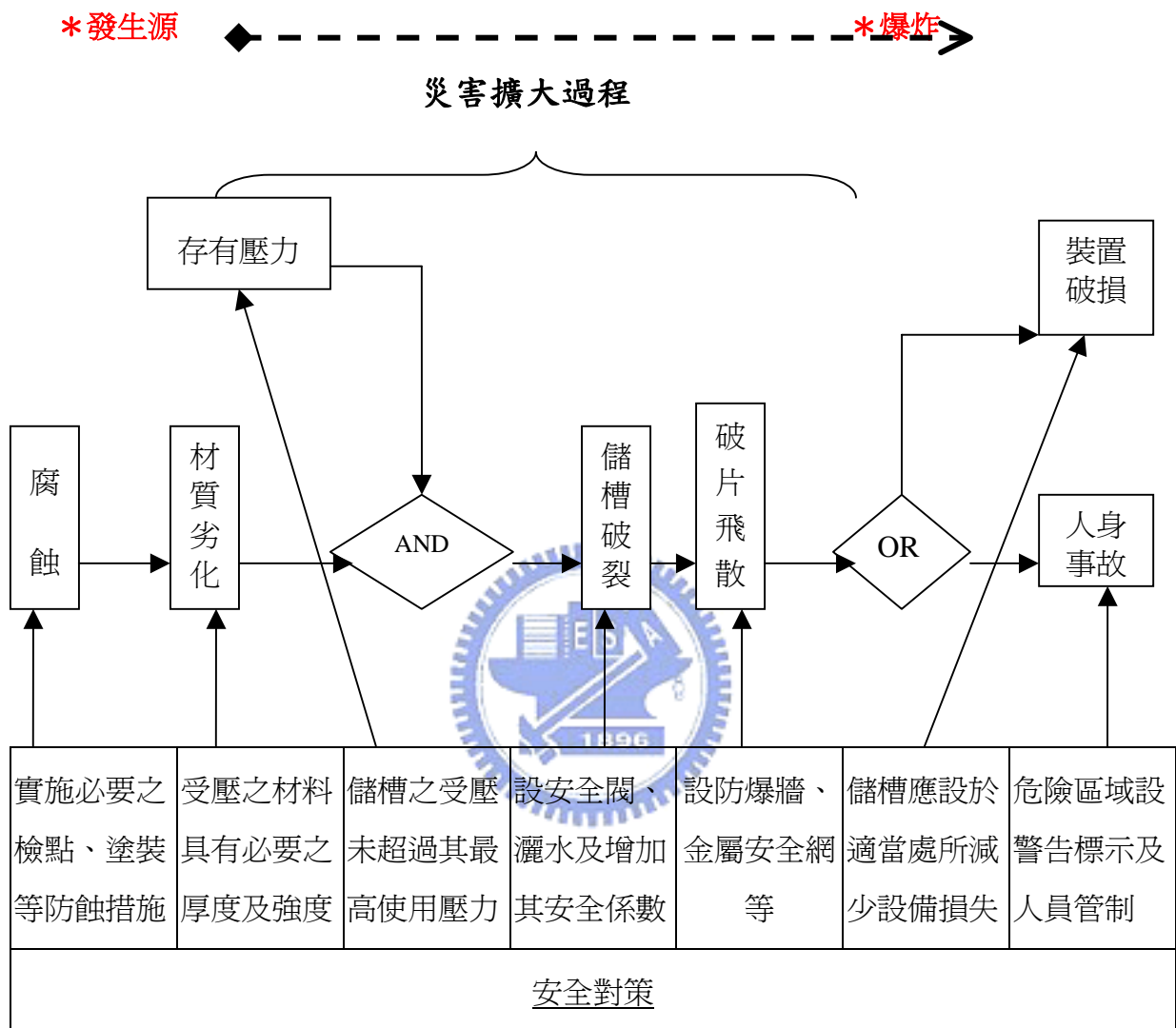
圖 4 壓力容器異常狀況流程分析圖
