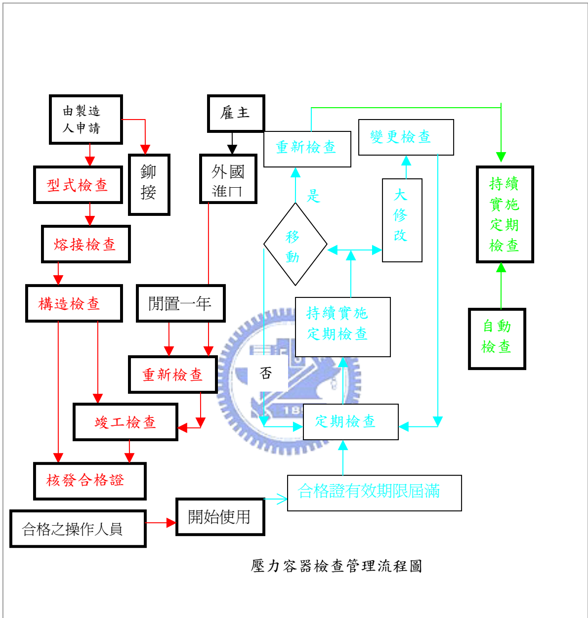
圖1 壓力容器檢查示意圖
