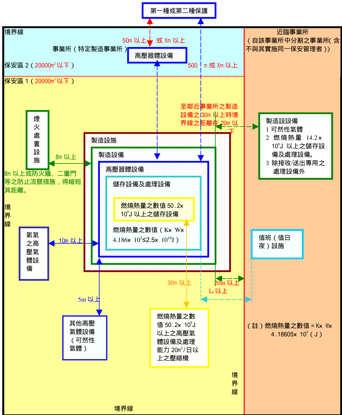
圖 6、保安距離及設備間距離之圖示
