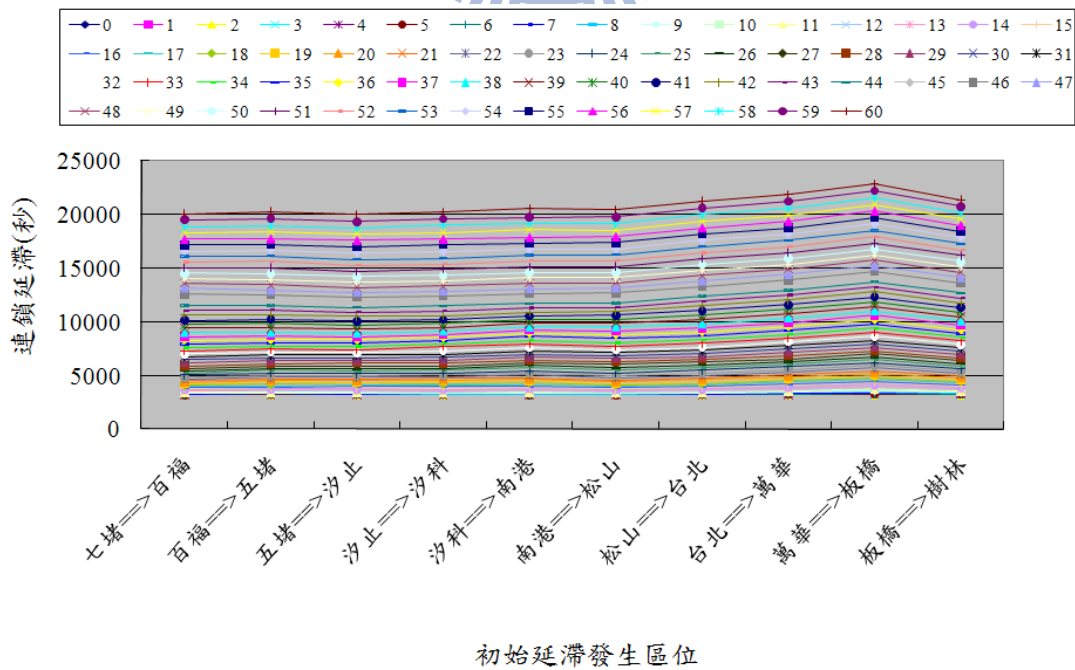
圖 5-8 同時採取二運轉調度策略下二末端車站之連鎖延滯
