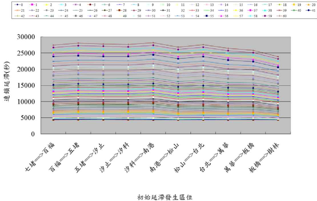
圖 5-7 無運轉調度策略下二末端車站之連鎖延滯
