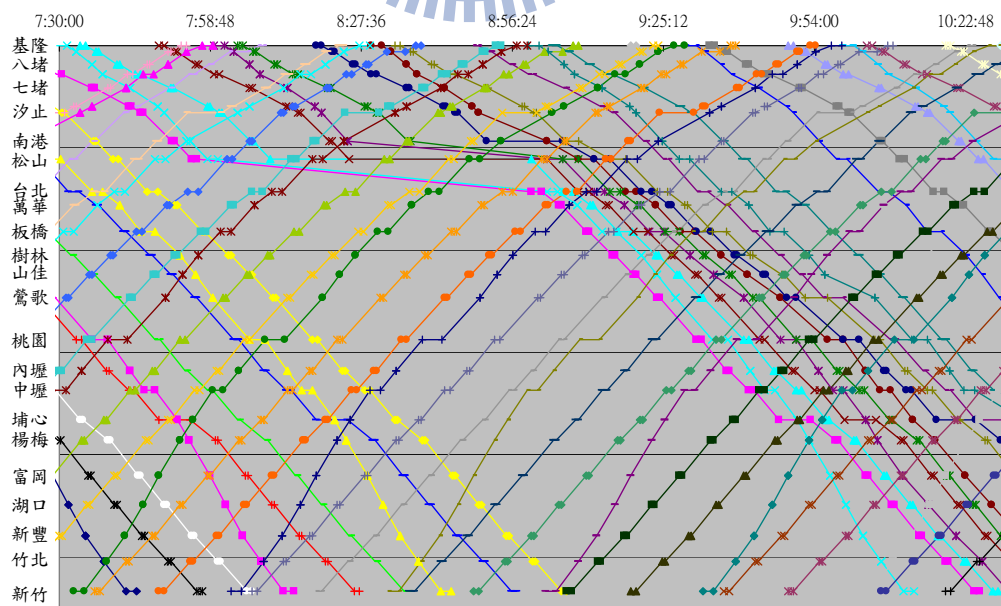
圖 3-18 模擬班表時空圖(初始延滯持續 3,600 秒)
