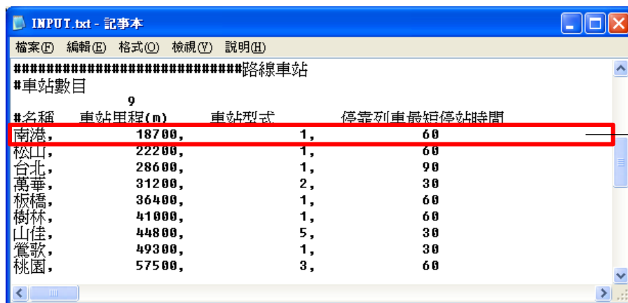
附圖 3 路線車站輸入格式
