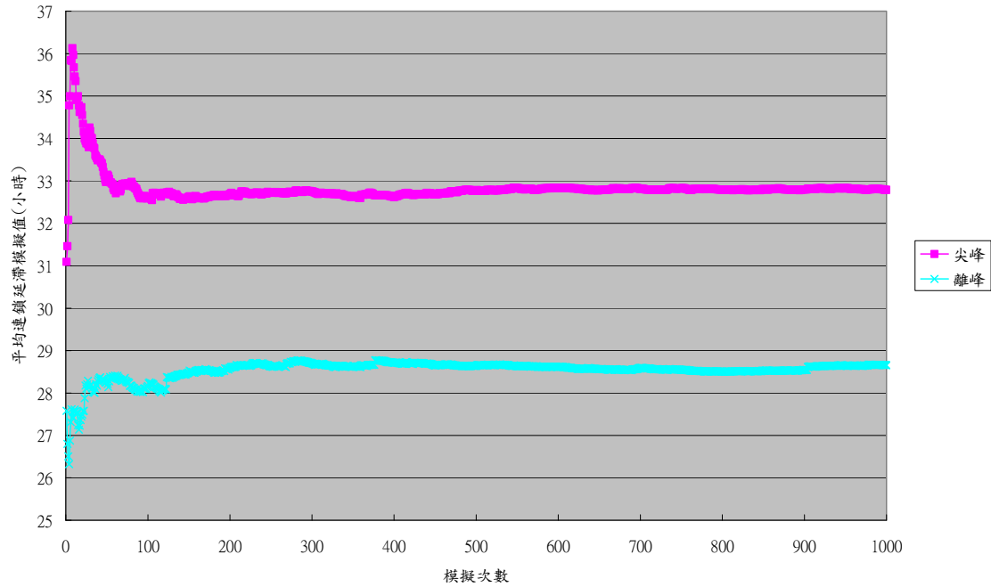
圖 6-12 七堵及新竹二末端車站之平均連鎖延滯模擬值與模擬次數關係
