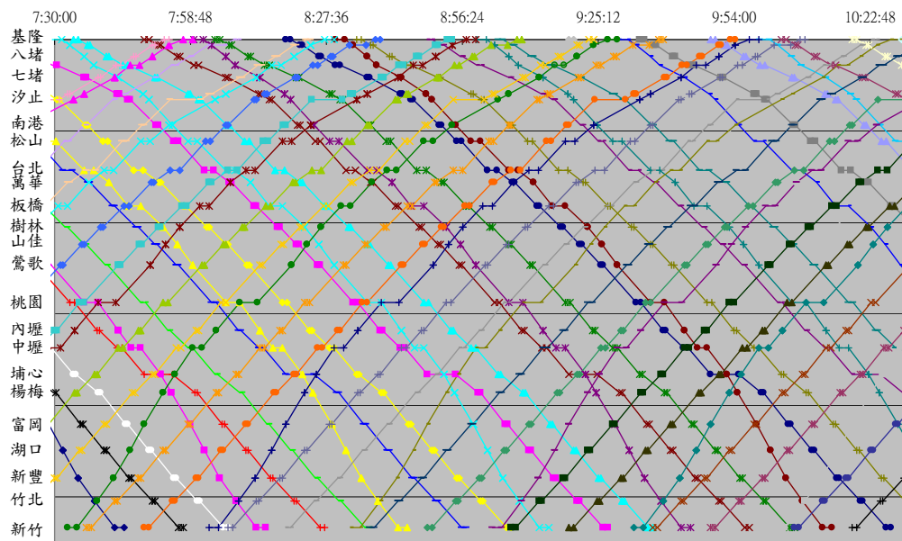
圖 3-17 原訂班表時空圖
