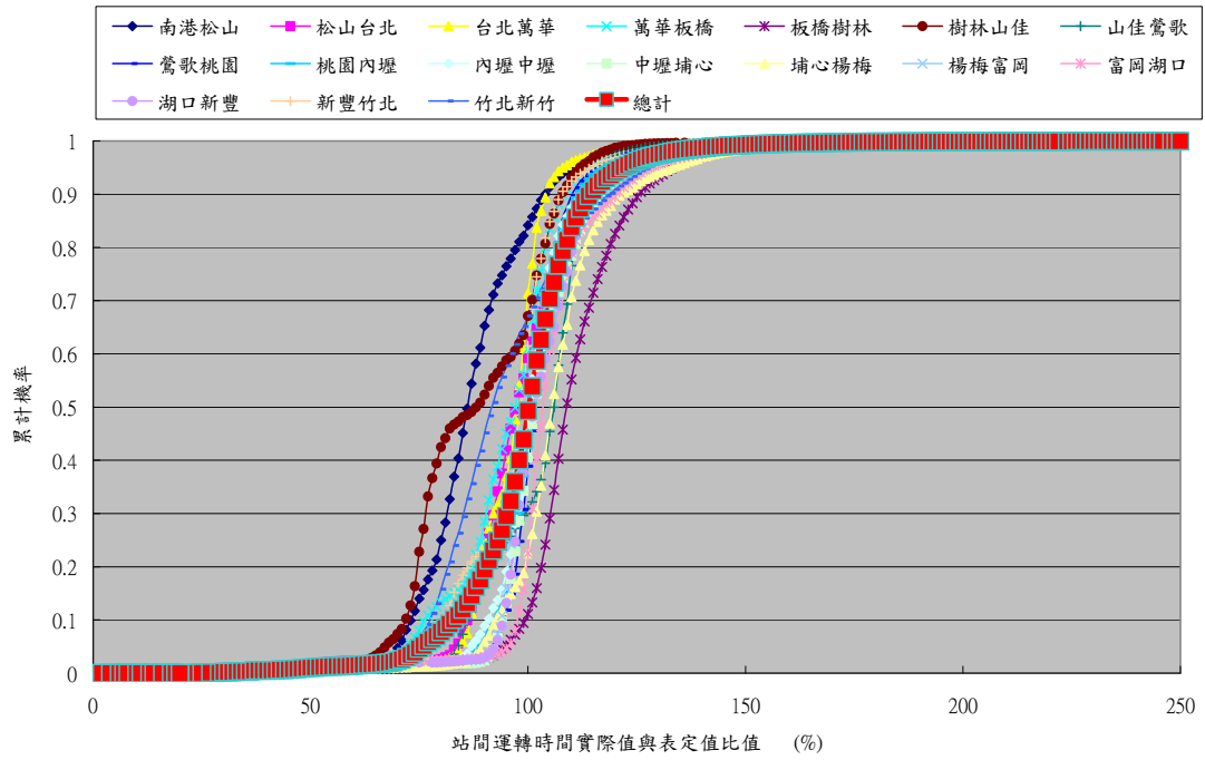
圖 6-2 通勤電聯車之站間運轉時間分佈圖
