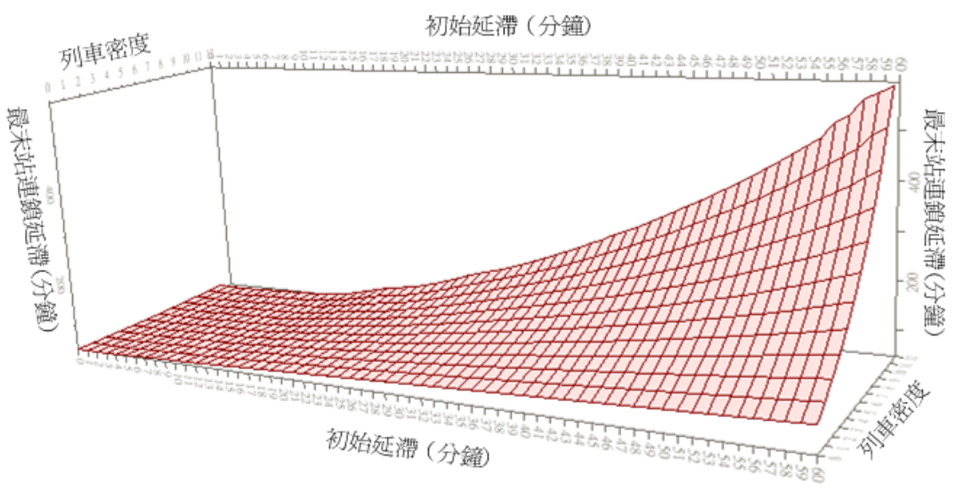
圖 4-14 同時採取二種調度策略下列車密度/初始延滯/連鎖延滯(平均值)之關係圖
