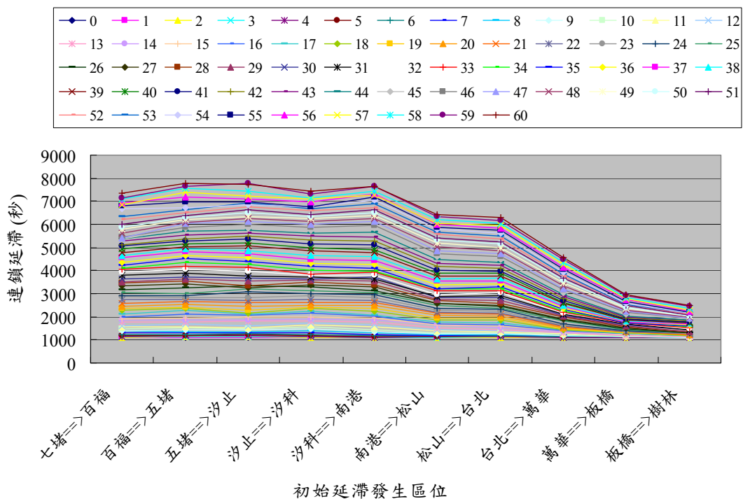
圖 5-9 同時採取二運轉調度策略下二末端車站之連鎖延滯降低
