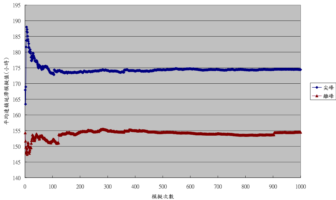
圖 6-11 所有車站之平均連鎖延滯模擬值與模擬次數關係
