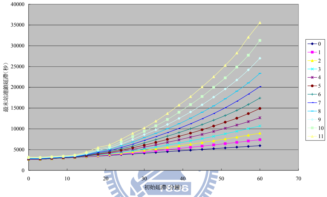
圖 4-13 各種列車密度情境下初始延滯與連鎖延滯關係圖
