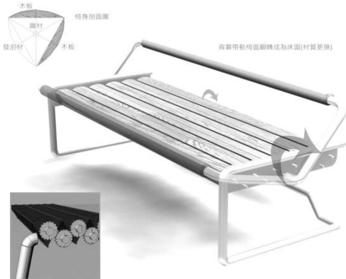
圖 77 材質與機構示意
