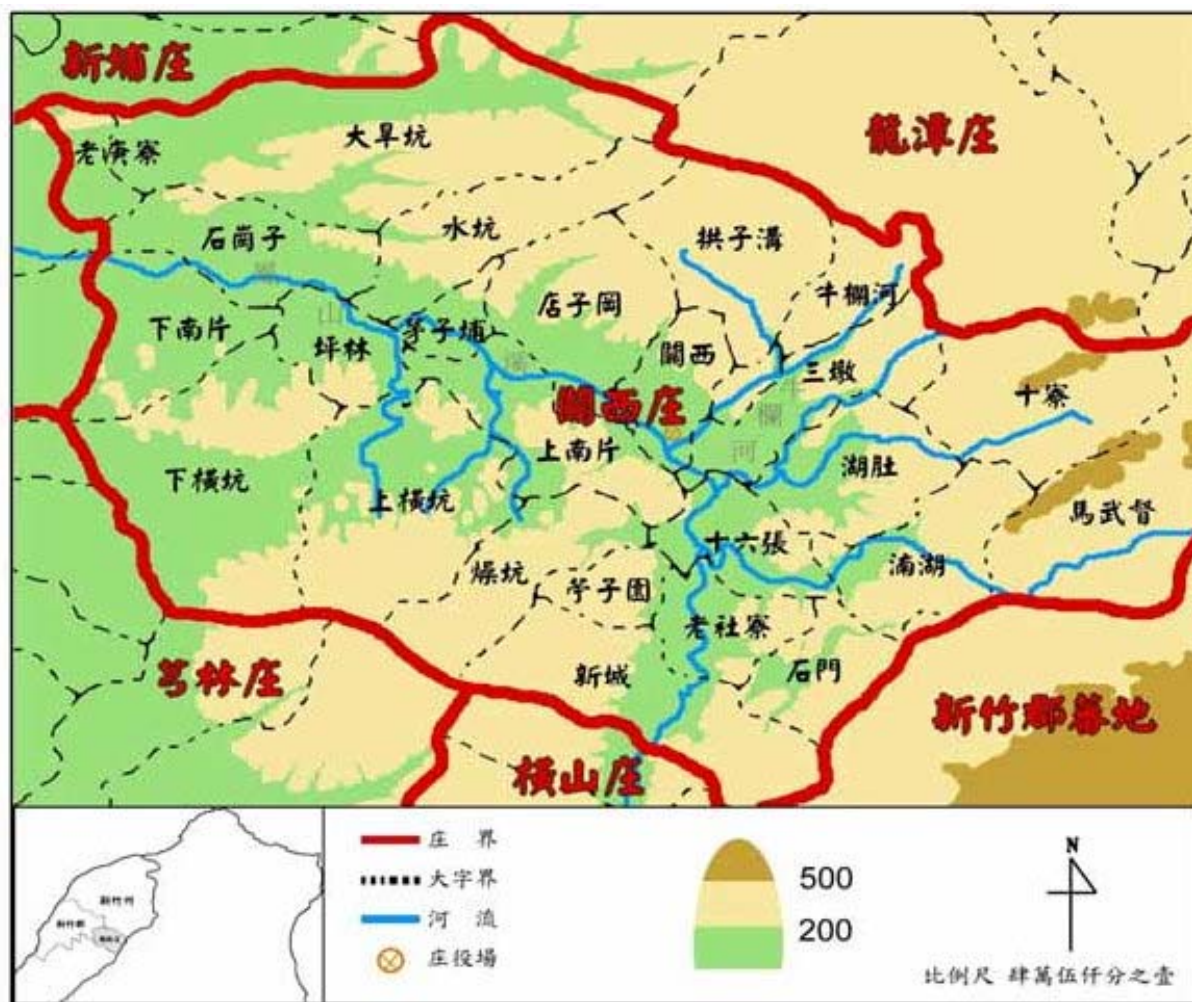
圖3.1 西元1924 年關西庄行政區劃
