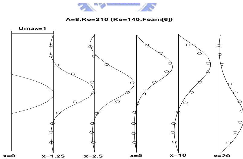
圖 4.8 管道中心截面之速度分佈曲線和實驗數據(Fearn 等人[6])的比
