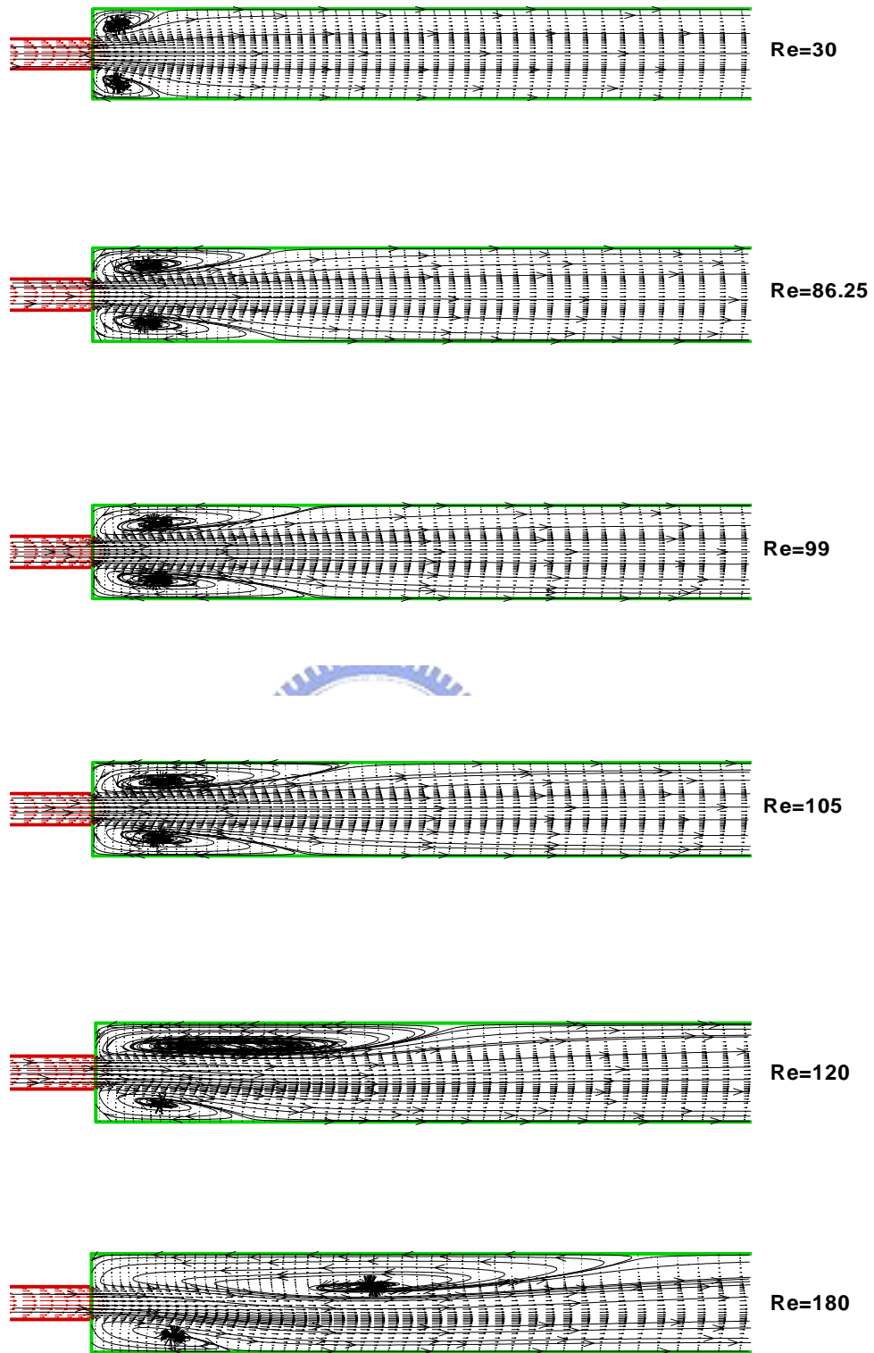
圖 4.14 A=1 ,不同雷諾數時,管道中心截面之速度場流線圖
