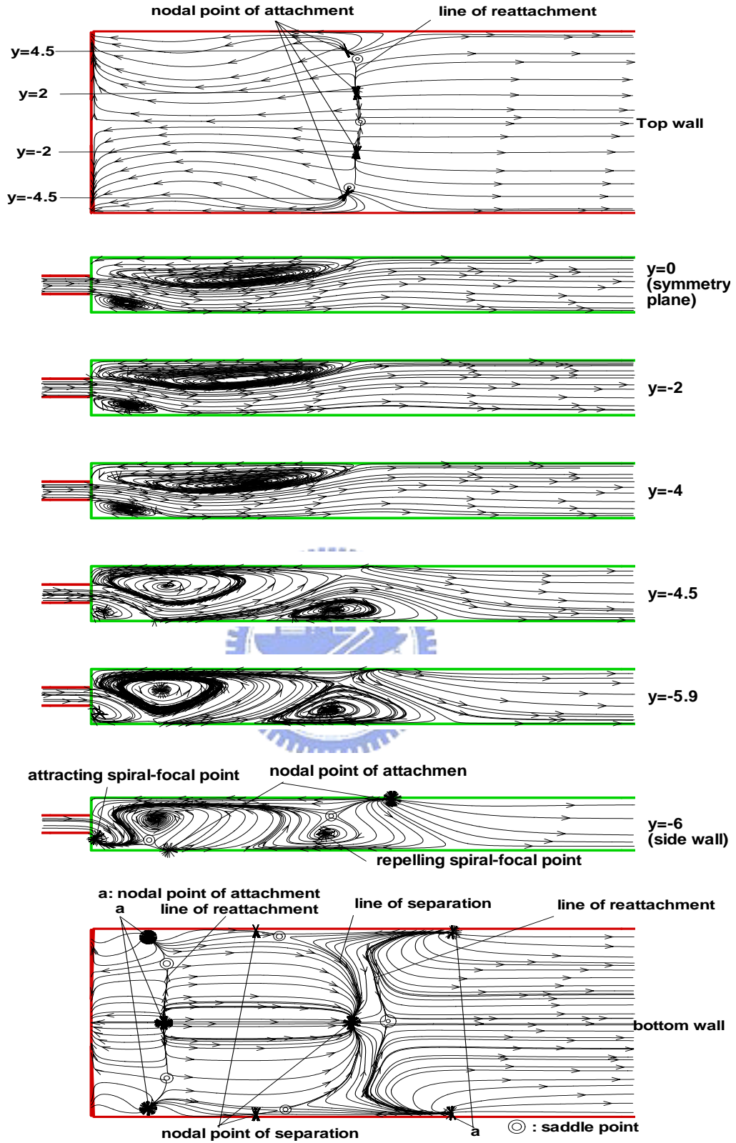
圖 4.23 A=4, Re=150 管道不同截面之流線圖
