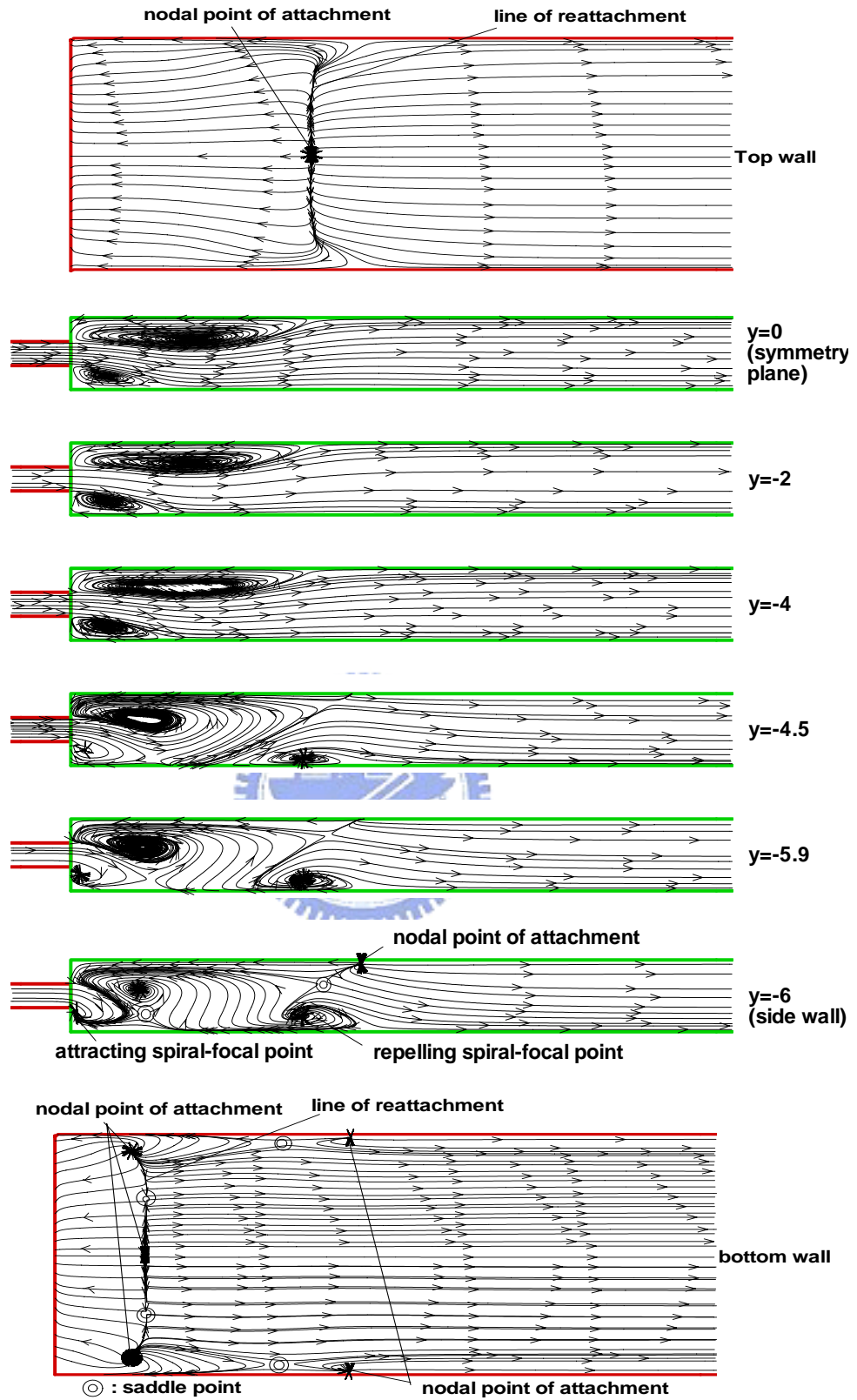
圖 4.22 A=4, Re=90 管道不同截面之流線圖
