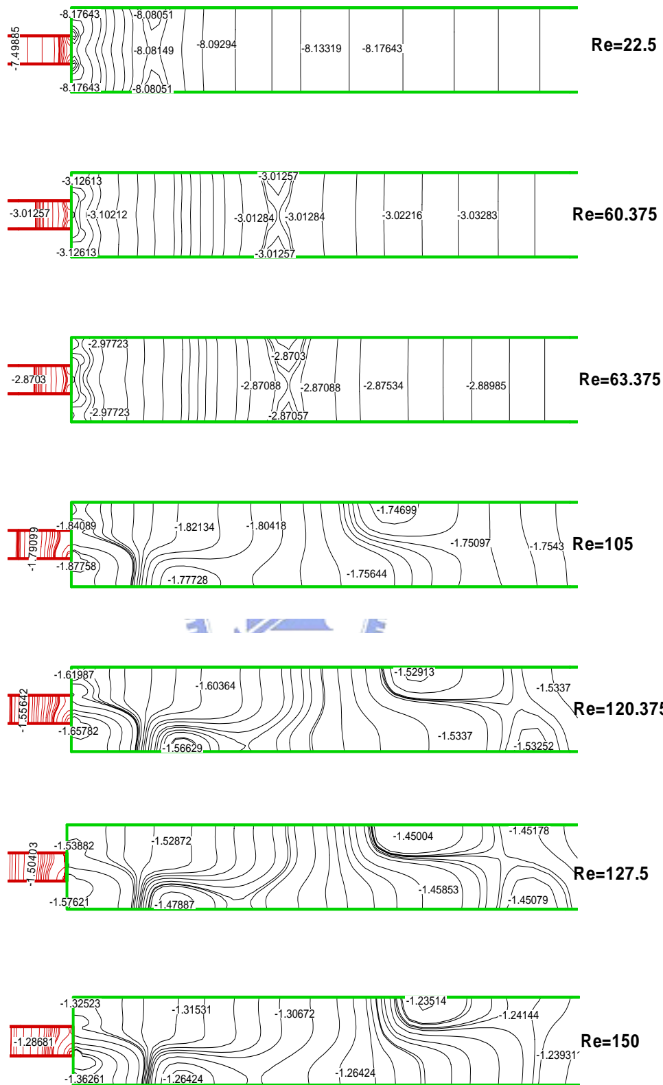
圖 4.26 A=8,不同雷諾數時,管道中心截面之壓力等值線分佈圖
