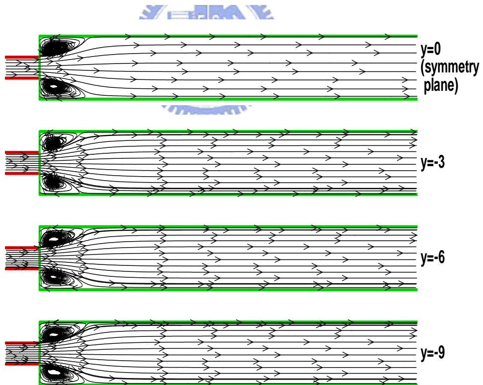
圖 4.27-1 A=8, Re=40 管道不同截面之流線圖
