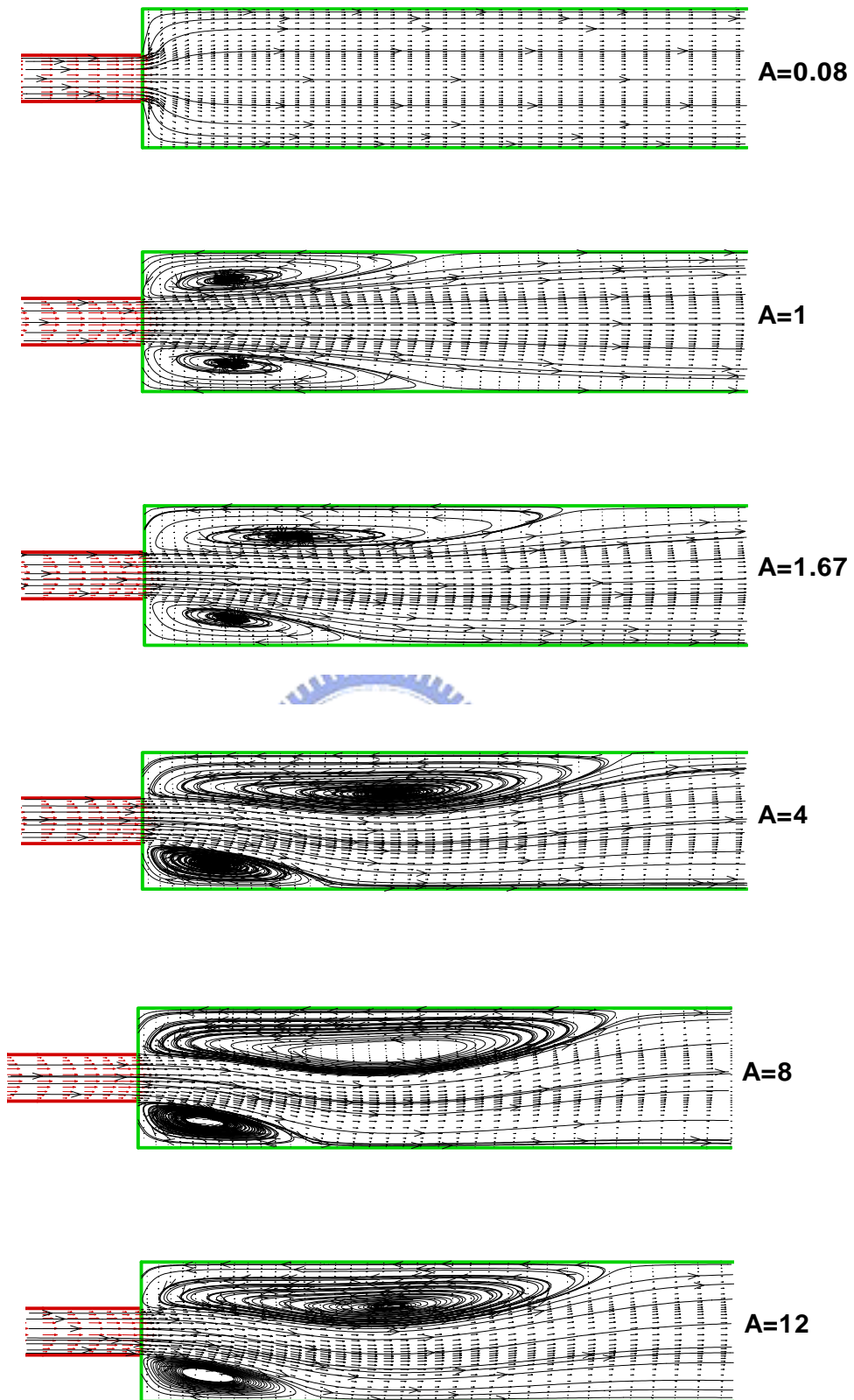
圖 4.31 Re=90 ,不同高寬比時,管道中心截面之迴流大小
