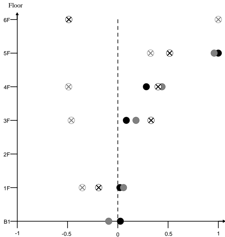
水平向第五模態
