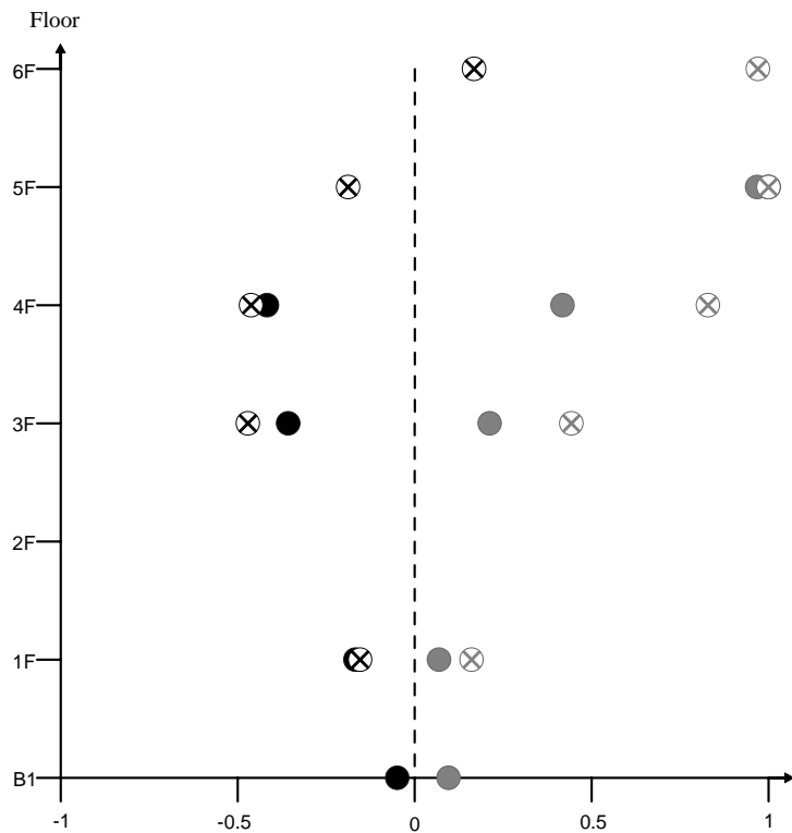
水平向第六模態
