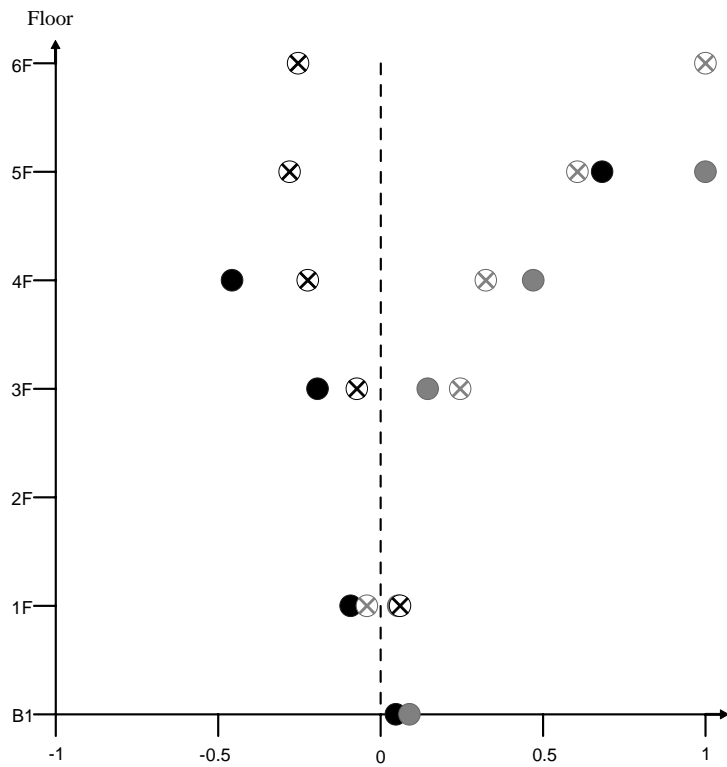
水平向第四模態
