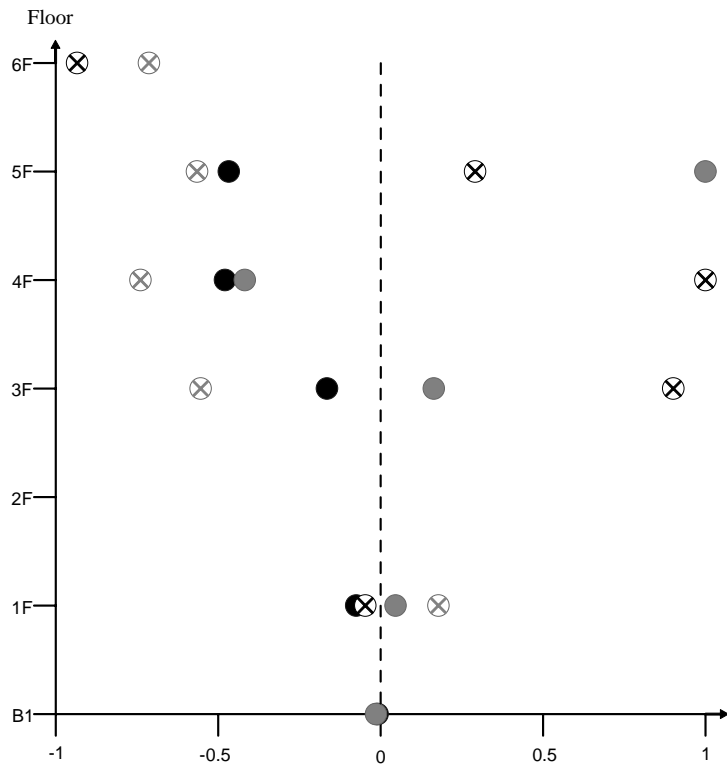
水平向第九模態
