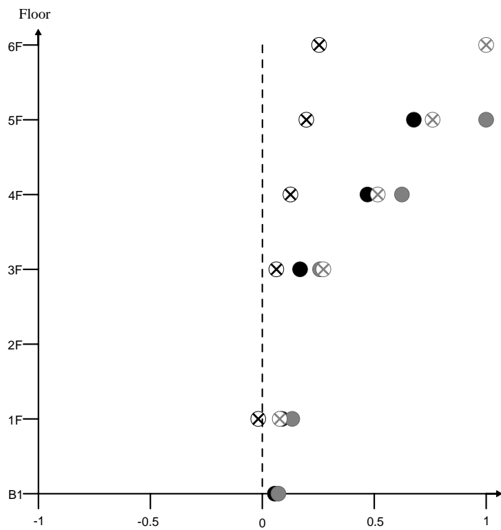
水平向第二模態
