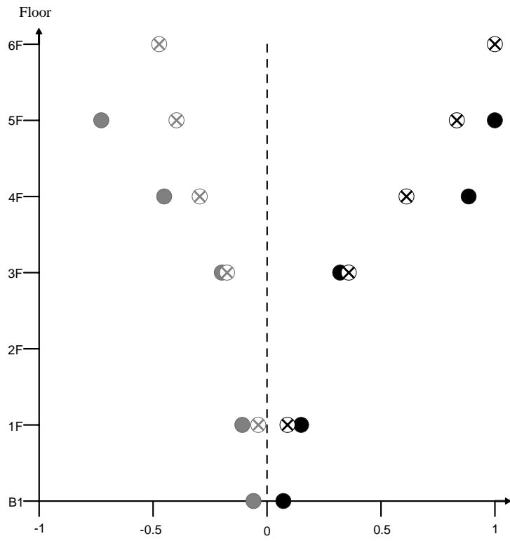
水平向第一模態
