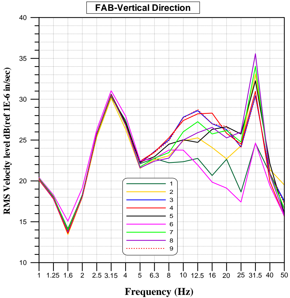
圖 4.40 穿孔格子樑版垂直向 RMS 比較
