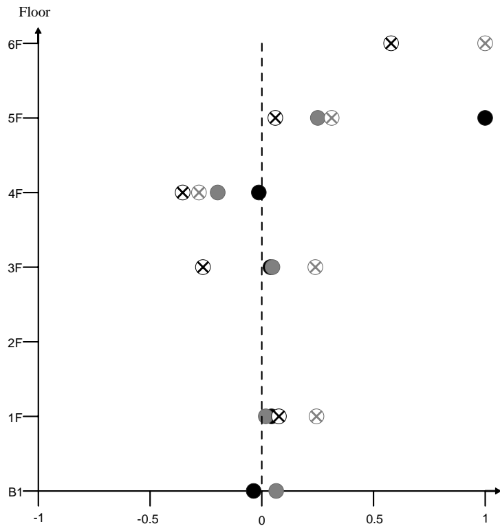
水平向第七模態
