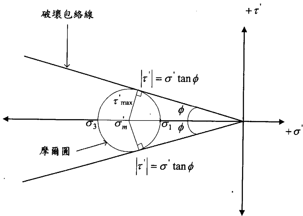
圖 2.2 摩爾圓-破壞包絡線關係示意圖(無凝聚力土壤)
