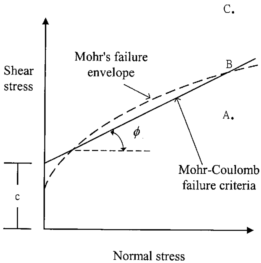
圖 2.1 摩爾破壞包絡線及摩爾-庫倫破壞準則概念
