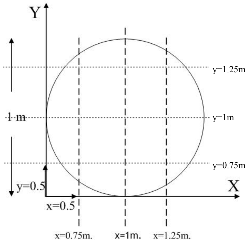
圖 3.6(a) 有限解析法圓形模擬區域測試示意圖
