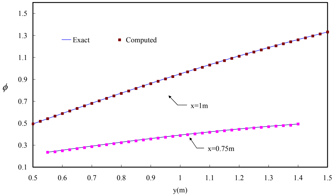
圖 3.7(b) 有限解析法圓形模擬區域測試模擬結果(A=15、B=15)
