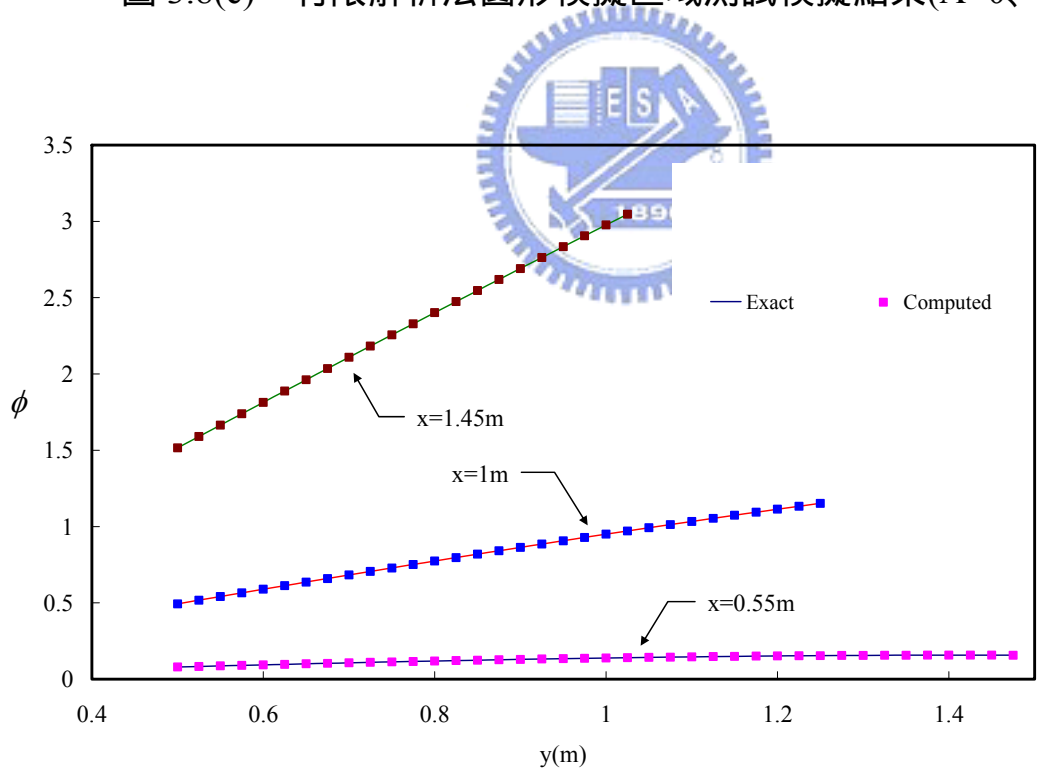
圖 3.8(c) 有限解析法圓形模擬區域測試模擬結果(A=0、B=15)
