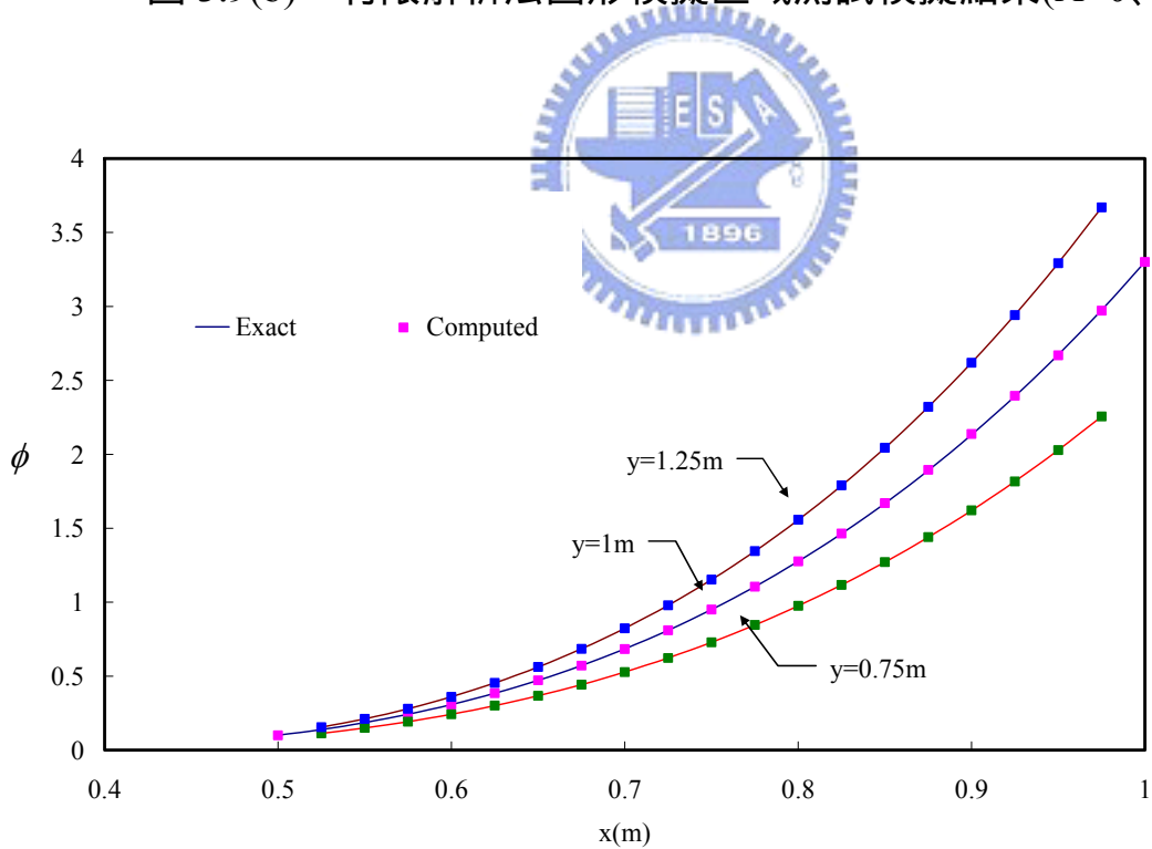
圖 3.9(b) 有限解析法圓形模擬區域測試模擬結果(A=0、B=0)
