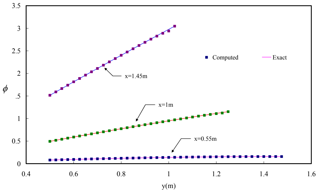
圖 3.8(a) 有限解析法梯形模擬區域測試模擬結果(A=0、B=15)
