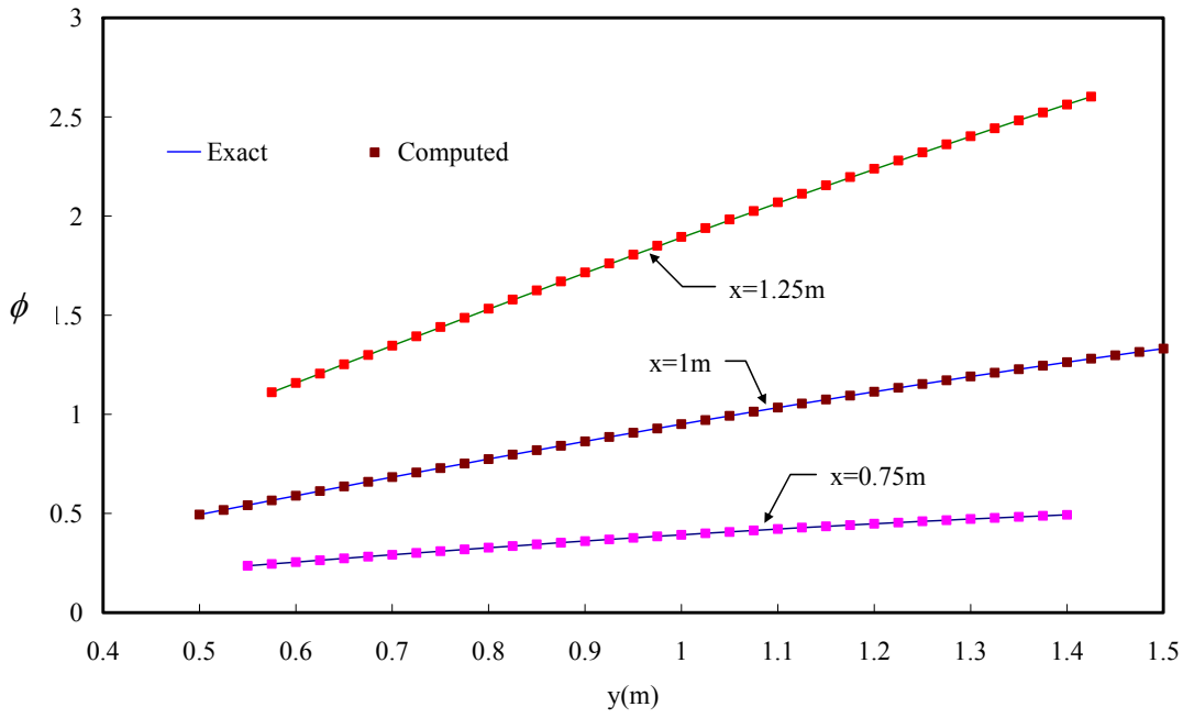
圖 3.9(b) 有限解析法圓形模擬區域測試模擬結果(A=0、B=0)
