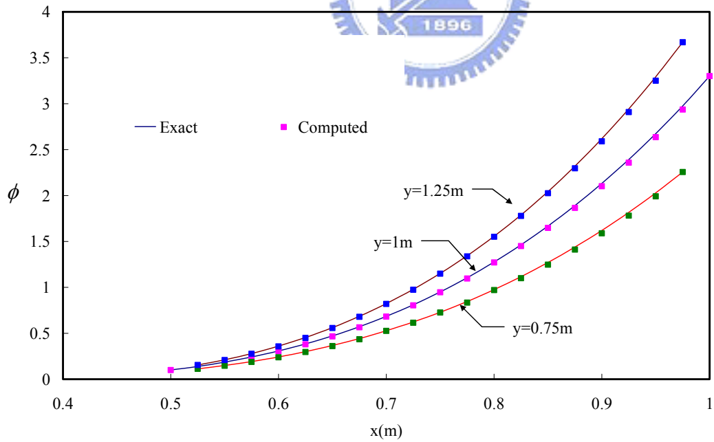
圖 3.7(c) 有限解析法圓形模擬區域測試模擬結果(A=15、B=15)
