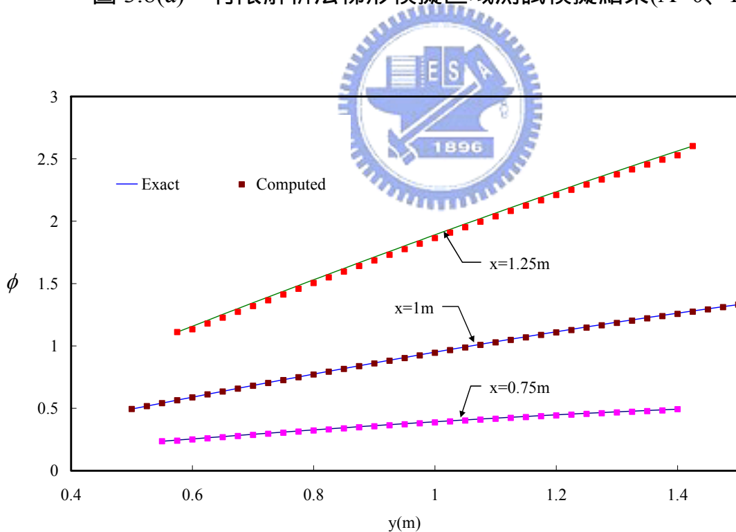
圖 3.8(a) 有限解析法梯形模擬區域測試模擬結果(A=0、B=15)
