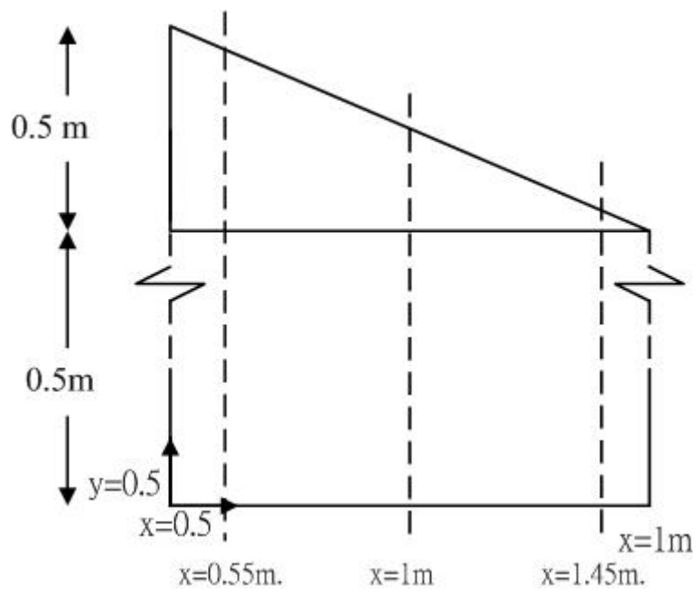
圖 3.5 有限解析法梯形模擬區域測試示意圖
