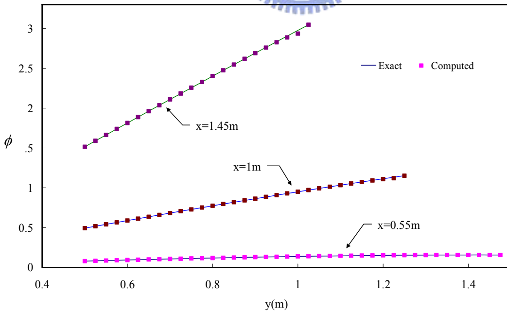
圖 3.7(a) 有限解析法梯形模擬區域測試模擬結果(A=15、B=15)
