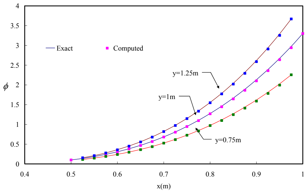
圖 3.8(c) 有限解析法圓形模擬區域測試模擬結果(A=0、B=15)
