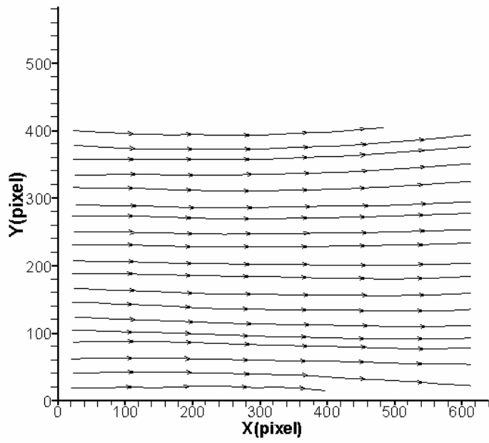
圖 4-81 案例 VI 位置 A 之速度流線分佈圖
