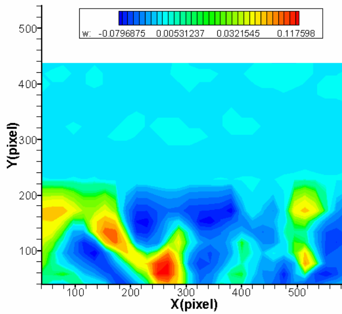
圖 4-112 案例 VII 位置 C 之渦度場圖
