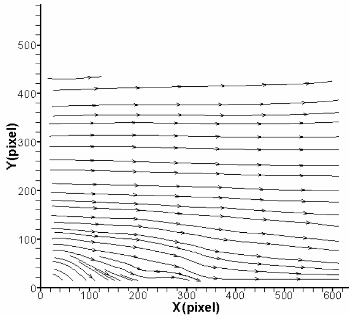
圖 4-76 案例 V 位置 C 之速度流線分佈圖
