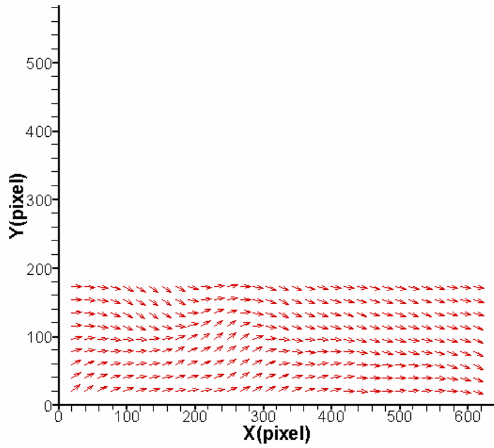
圖 4-115 案例 VII 位置 D 下半部之速度向量放大分佈圖
