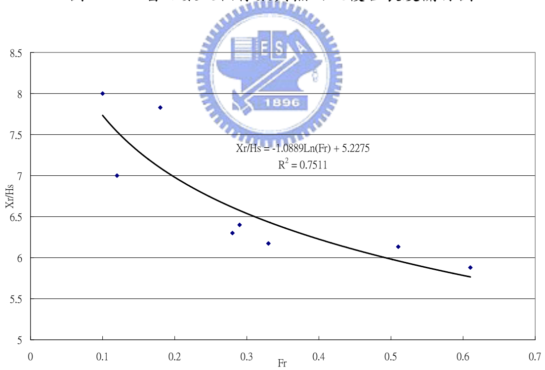
圖 4-139 雷諾數及福祿數與無因次複合長度關係圖
