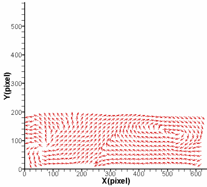
圖 4-105 案例 VII 位置 B 下半部之速度向量放大分佈圖
