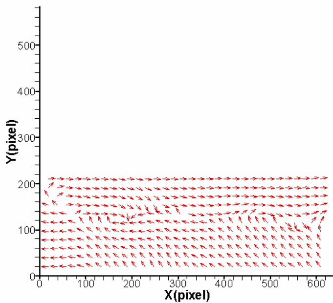
圖 4-130 案例 VIII 位置 C 下半部之速度向量放大分佈圖
