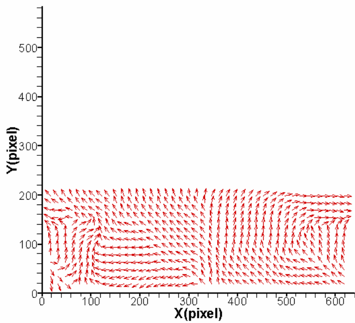
圖 4-125 案例 VIII 位置 B 下半部之速度向量放大分佈圖
