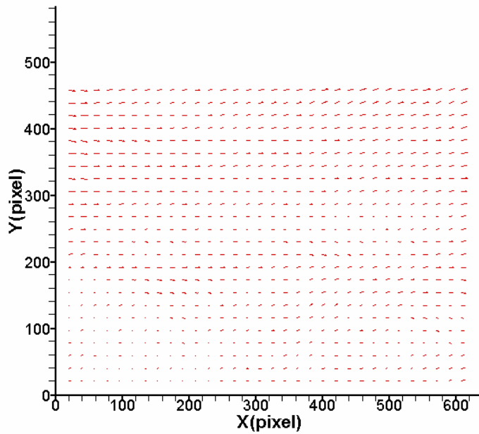
圖 4-134 案例 VIII 位置 D 之速度向量分佈圖
