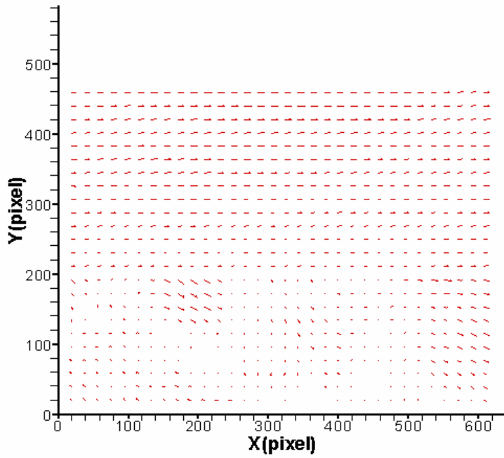
圖 4-89 案例 VI 位置 C 之速度向量分佈圖
