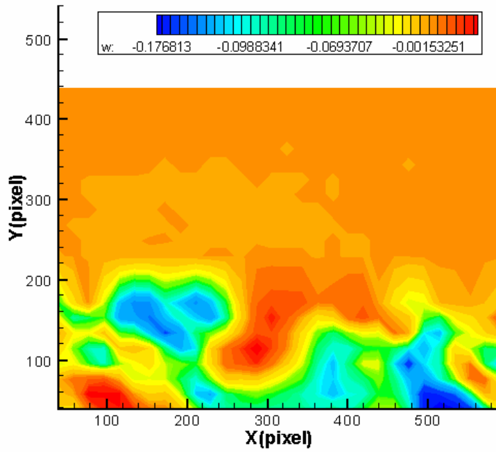
圖 4-97 案例 VI 位置 D 之渦度場圖
