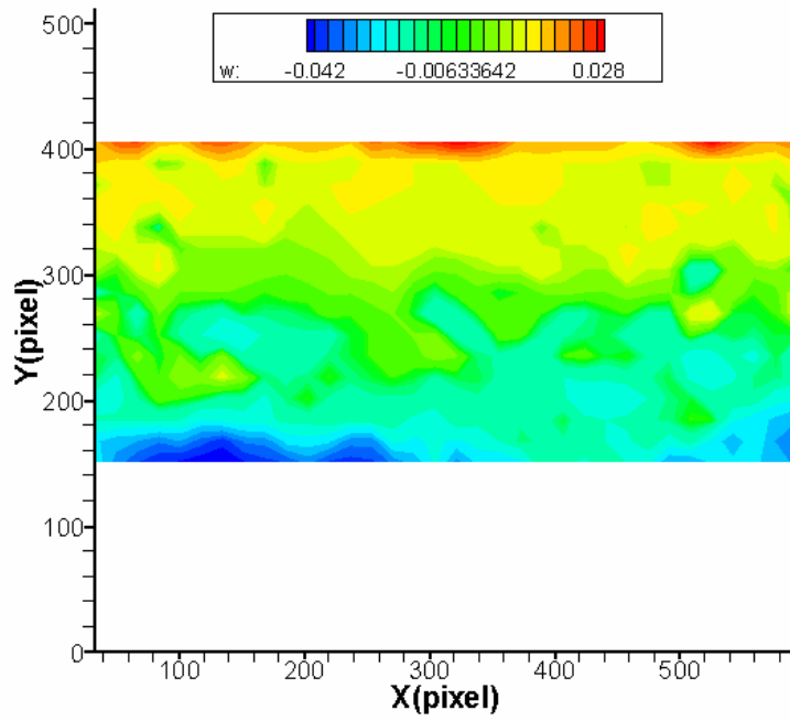
圖 4-67 案例 V 位置 A 之渦度場圖
