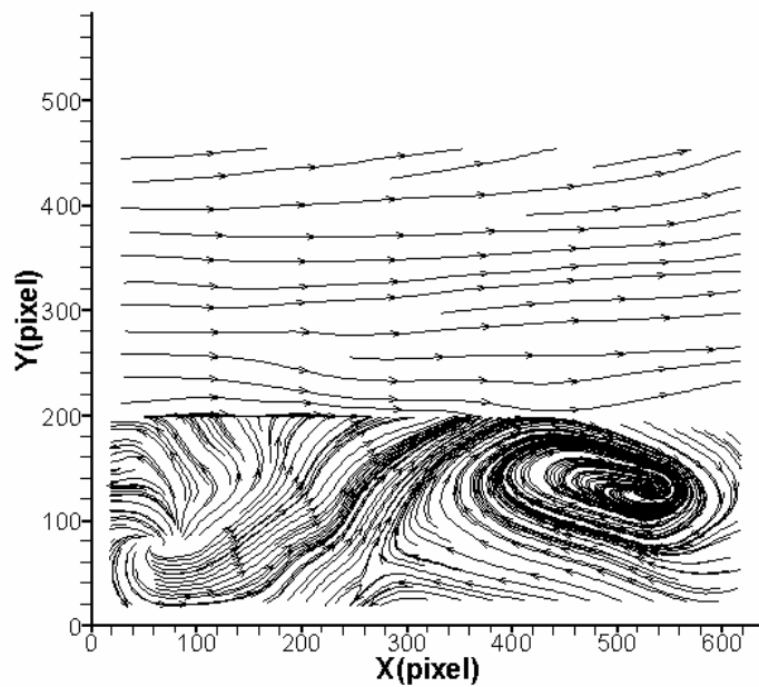
圖 4-106 案例 VII 位置 B 之速度流線分佈圖
