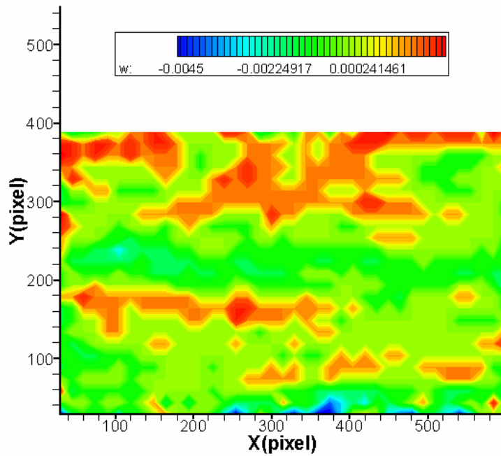
圖 4-82 案例 VI 位置 A 之渦度場圖
