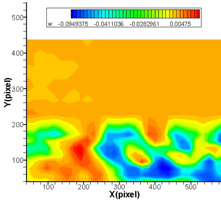
圖 4-117 案例 VII 位置 D 之渦度場圖
