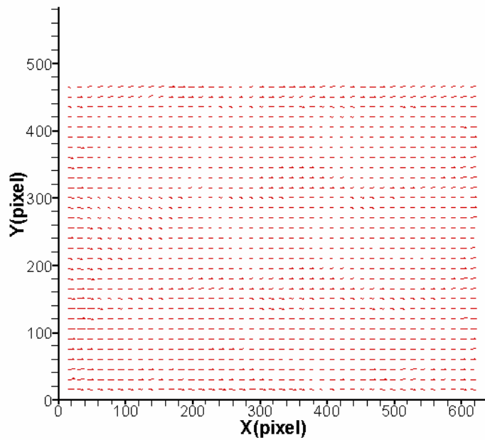
圖 4-100 案例 VII 位置 A 之速度向量分佈圖
