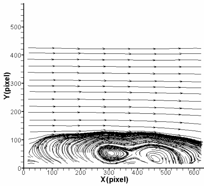
圖 4-71 案例 V 位置 B 之速度流線分佈圖
