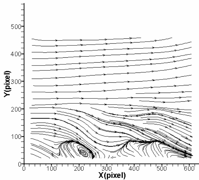
圖 4-96 案例 VI 位置 D 之速度流線分佈圖
