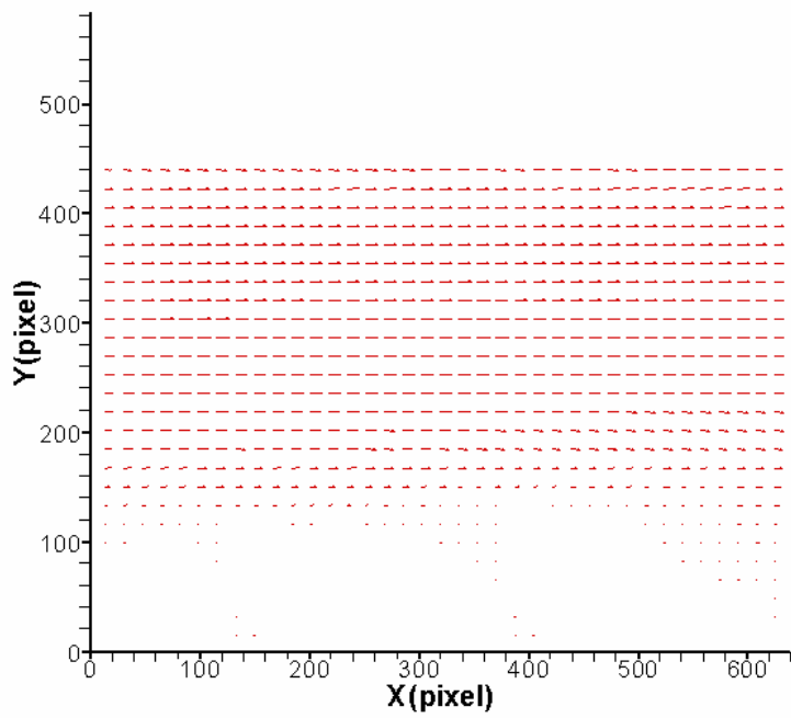
圖 4-69 案例 V 位置 B 之速度向量分佈圖
