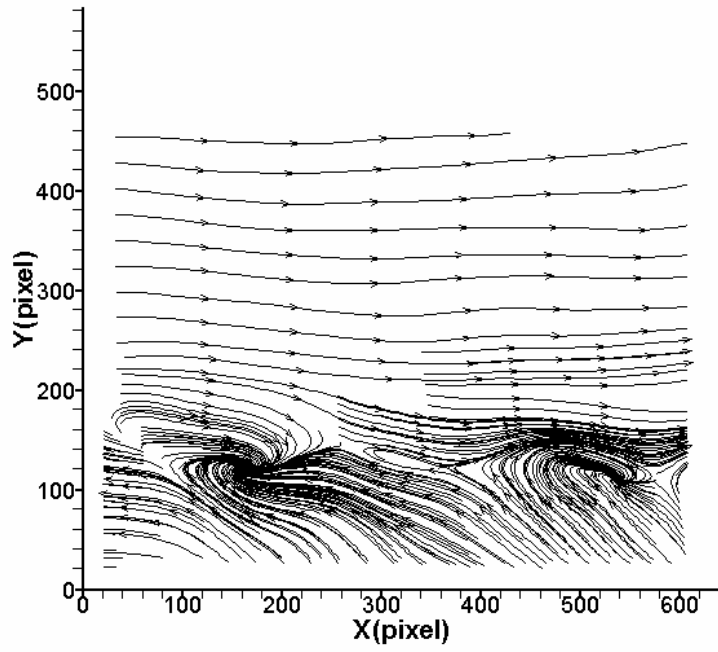
圖 4-131 案例 VIII 位置 C 之流線分佈圖
