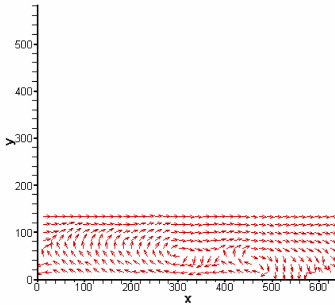
圖 4-70 案例 V 位置 B 下半部之速度向量放大分佈圖
