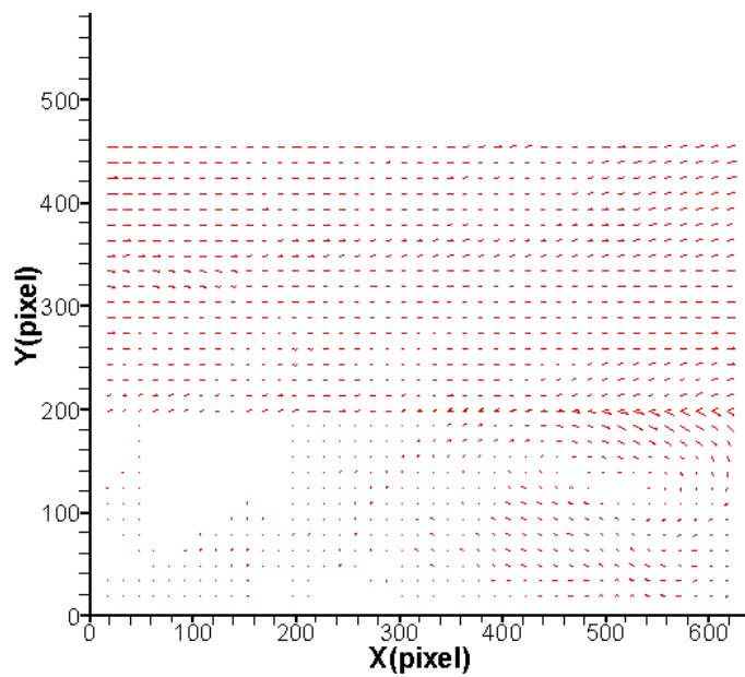
圖 4-104 案例 VII 位置 B 之速度向量分佈圖
