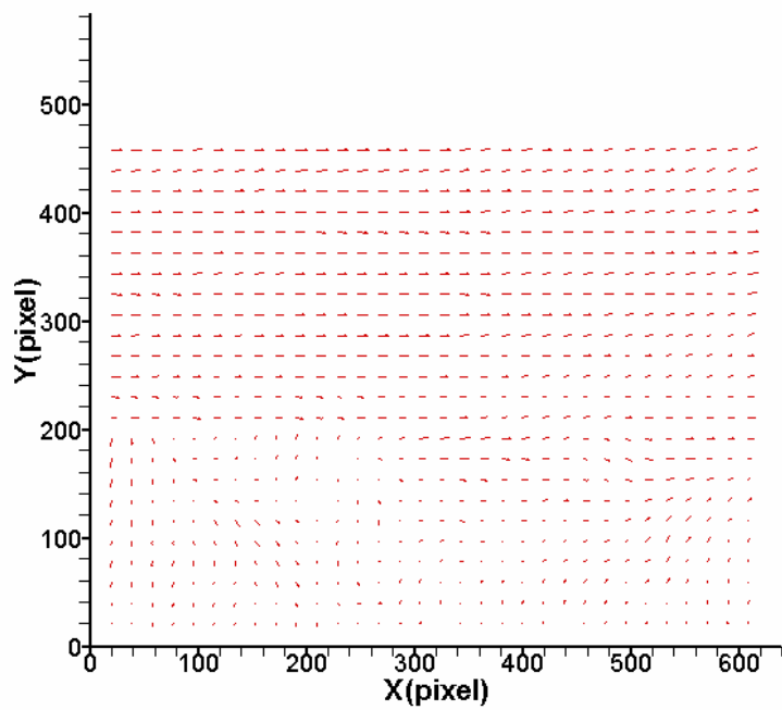
圖 4-109 案例 VII 位置 C 之速度向量分佈圖
