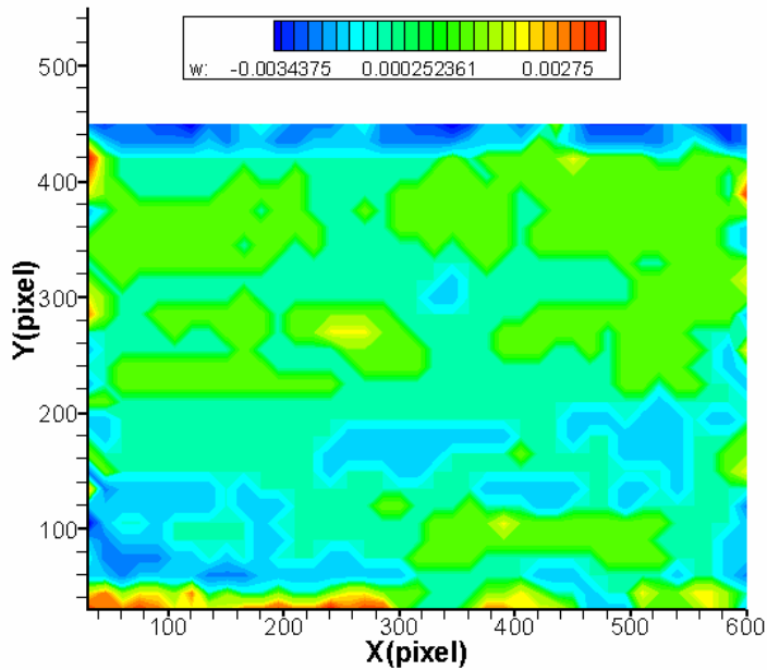
圖 4-122 案例 VIII 位置 A 之渦度場圖
