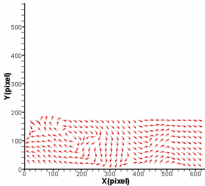
圖 4-90 案例 VI 位置 C 下半部之速度向量放大分佈圖
