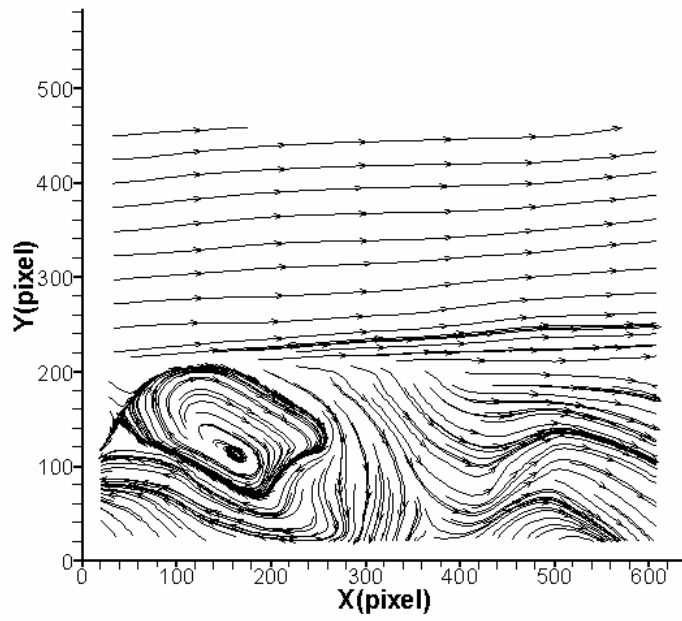
圖 4-91 案例 VI 位置 C 之速度流線分佈圖
