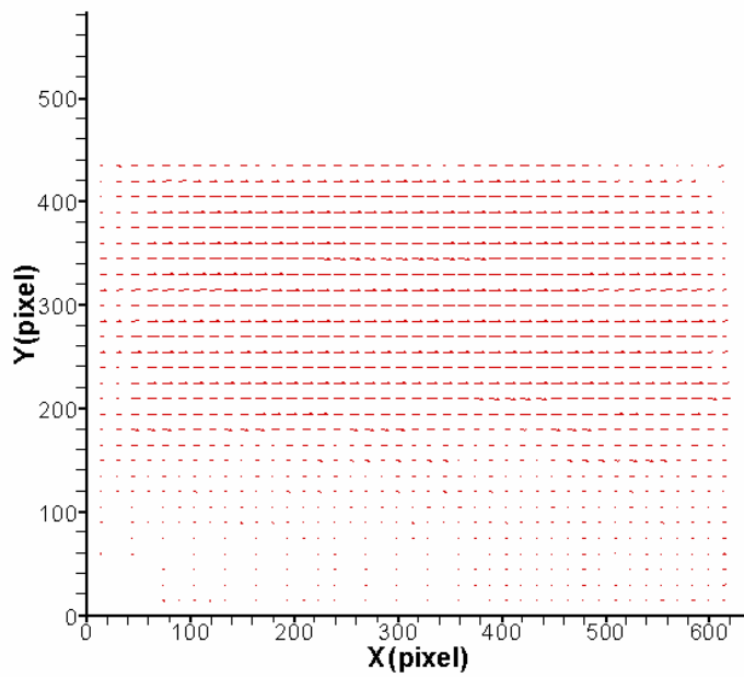
圖 4-74 案例 V 位置 C 之速度向量分佈圖圖
