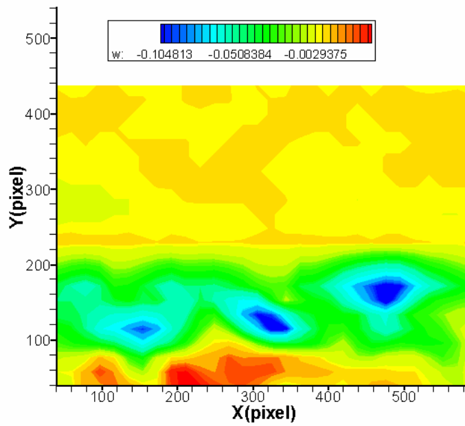
圖 4-132 案例 VIII 位置 C 之渦度場圖
