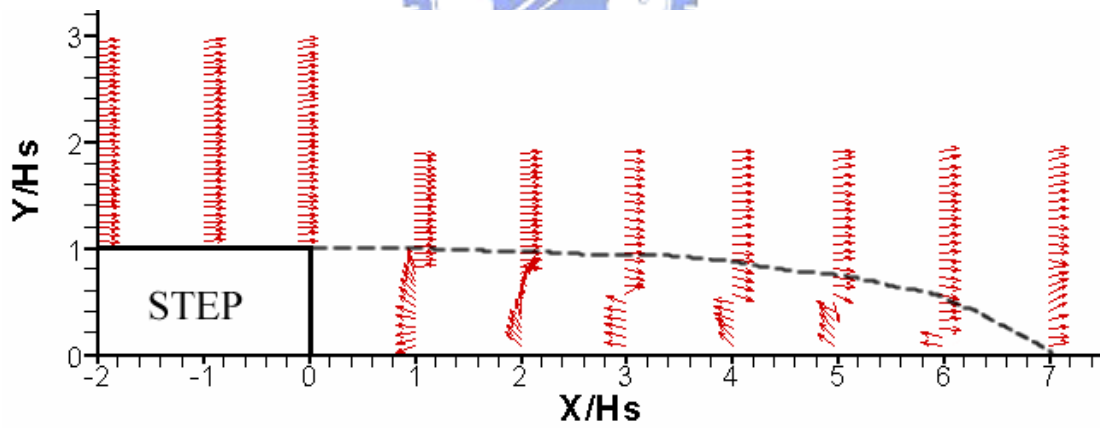
圖 4-138 案例 VIII 速度向量剖面圖
