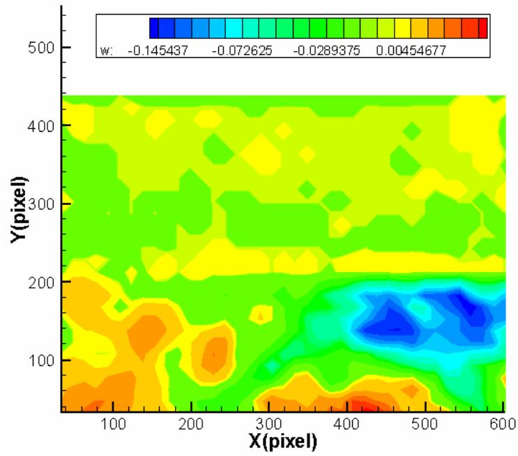
圖 4-107 案例 VII 位置 B 之渦度場圖
