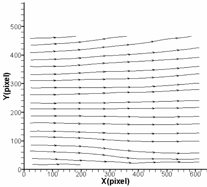
圖 4-121 案例 VIII 位置 A 之速度流線分佈圖
