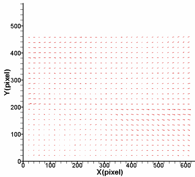
圖 4-114 案例 VII 位置 D 之速度向量分佈圖
