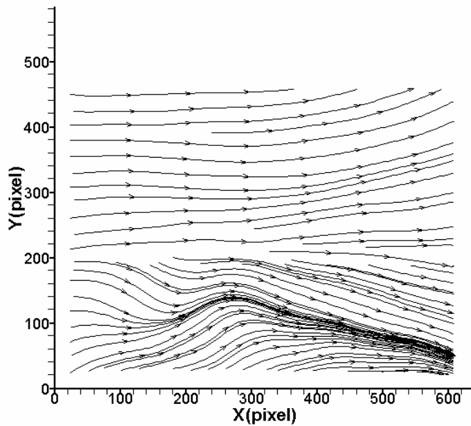
圖 4-116 案例 VII 位置 D 之速度流線分佈圖
