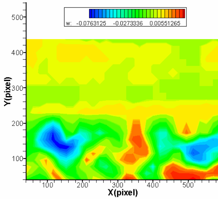
圖 4-137 案例 VIII 位置 D 之渦度場圖
