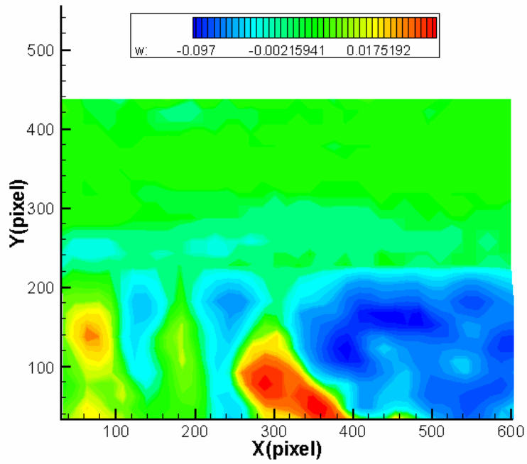
圖 4-87 案例 VI 位置 B 之渦度場圖
