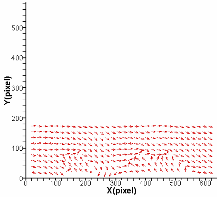
圖 4-95 案例 VI 位置 D 下半部之速度向量放大分佈圖
