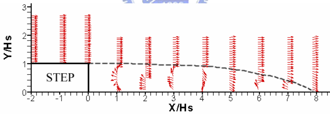
圖 4-98 案例 VI 速度向量剖面圖
