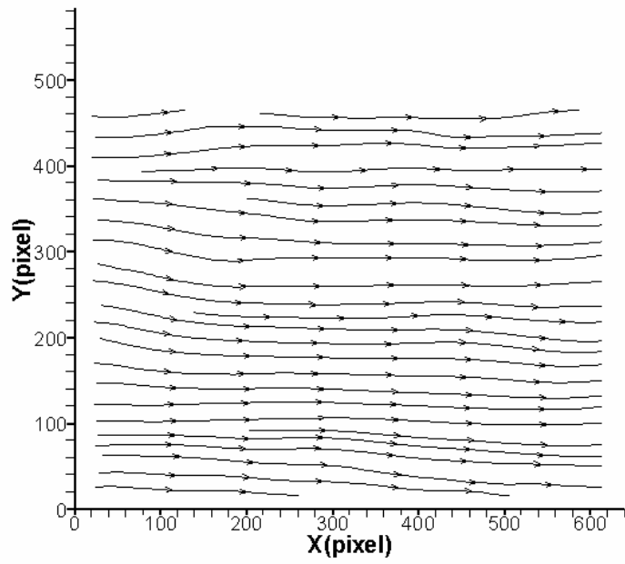
圖 4-101 案例 VII 位置 A 之速度流線分佈圖
