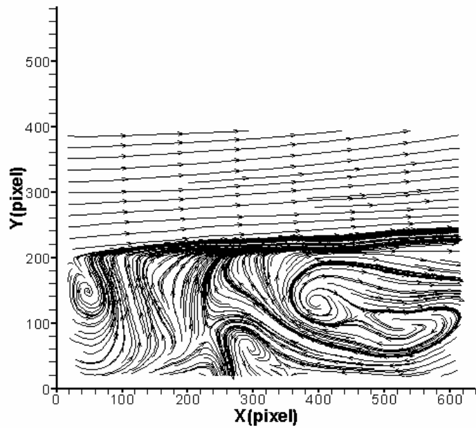
圖 4-86 案例 VI 位置 B 之速度流線分佈圖
