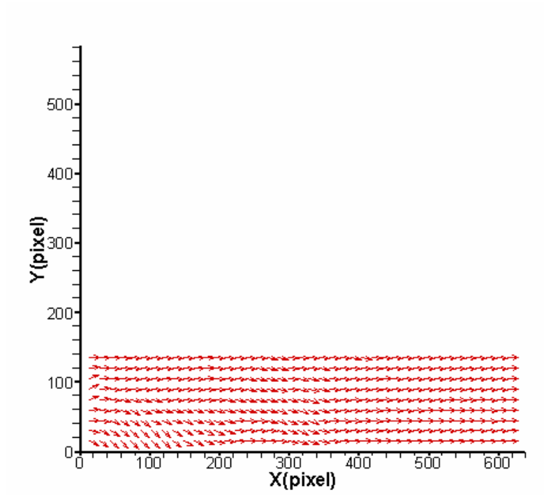
圖 4-75 案例 V 位置 C 下半部之速度向量放大分佈圖
