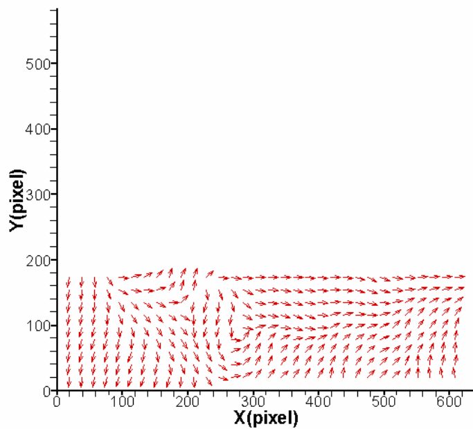
圖 4-110 案例 VII 位置 C 下半部之速度向量放大分佈圖
