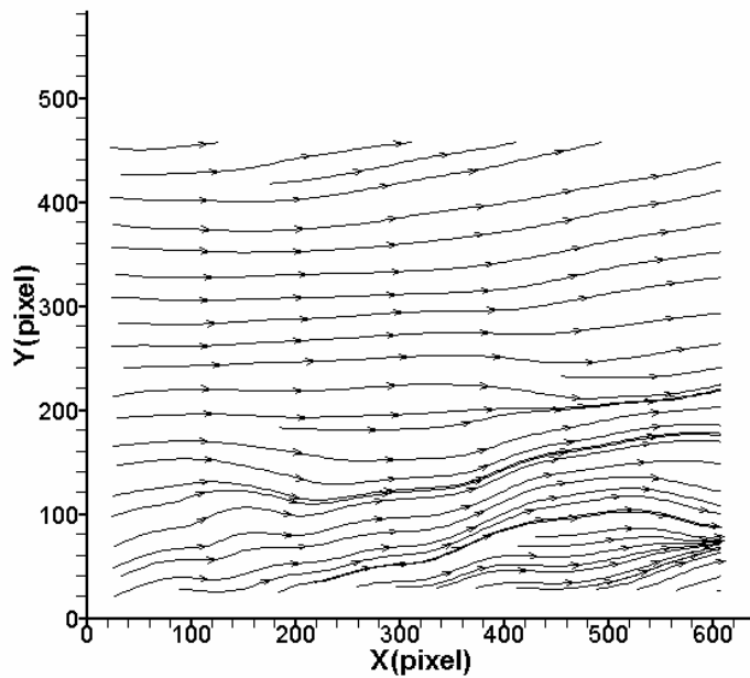
圖 4-136 案例 VIII 位置 D 之流線分佈圖
