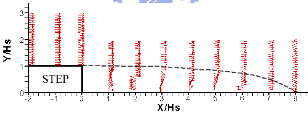
圖 4-118 案例 VII 速度向量剖面圖
