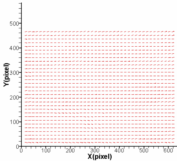
圖 4-120 案例 VIII 位置 A 之速度向量分佈圖
