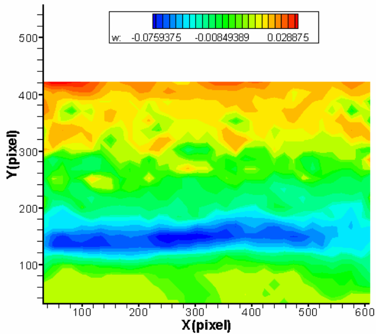
圖 4-72 案例 V 位置 B 之渦度場圖
