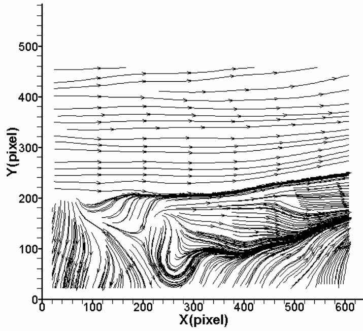
圖 4-111 案例 VII 位置 C 之速度流線分佈圖
