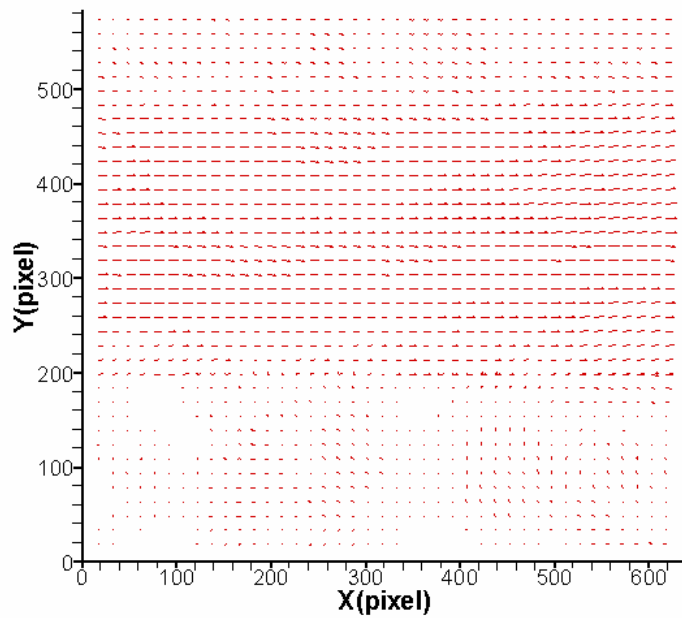
圖 4-124 案例 VIII 位置 B 之速度向量分佈圖
