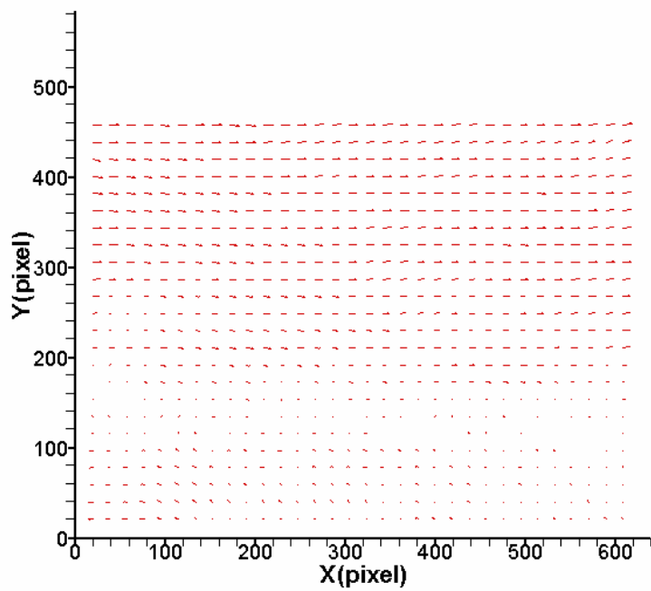
圖 4-129 案例 VIII 位置 C 之速度向量分佈圖
