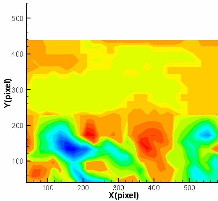
圖 4-92 案例 VI 位置 C 之渦度場圖
