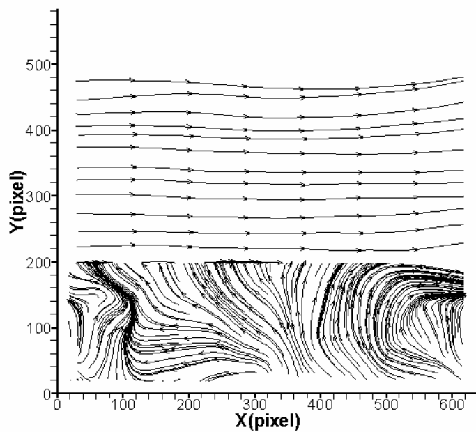
圖 4-126 案例 VIII 位置 B 之流線分佈圖
