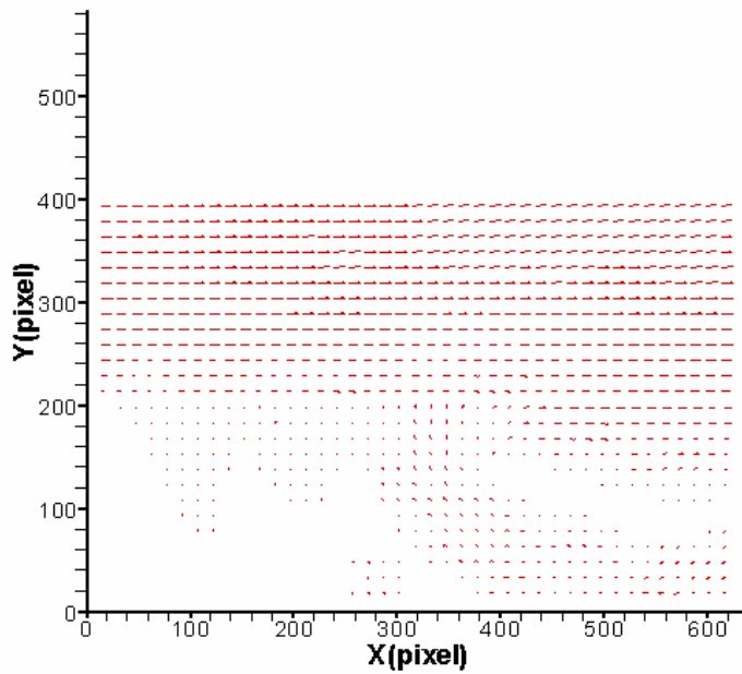
圖 4-84 案例 VI 位置 B 之速度向量分佈圖
