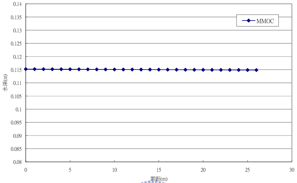
圖 5.4 定量流於合流支渠水深沿程圖
