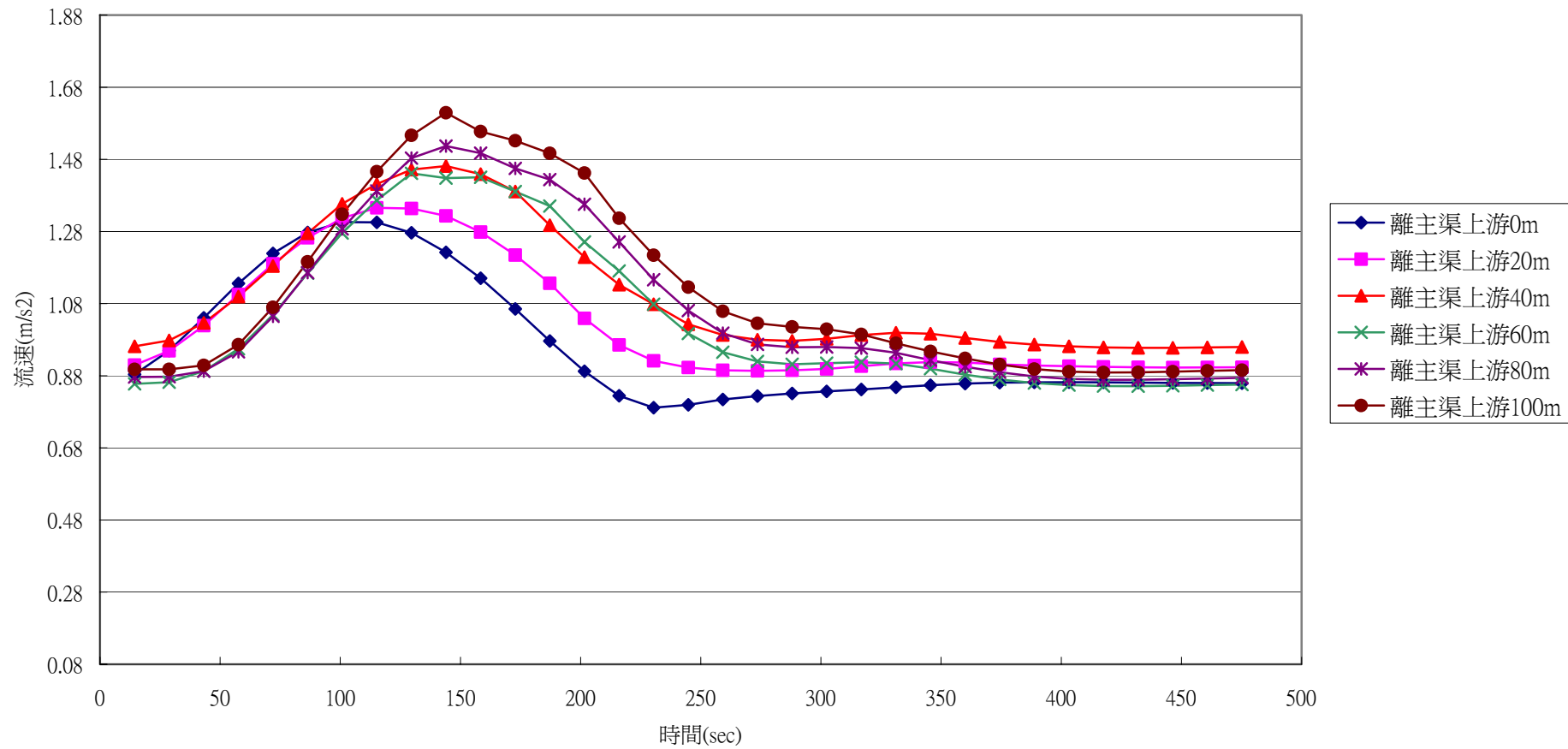
圖 5.19 非矩形渠道主渠流速延時歷線圖
