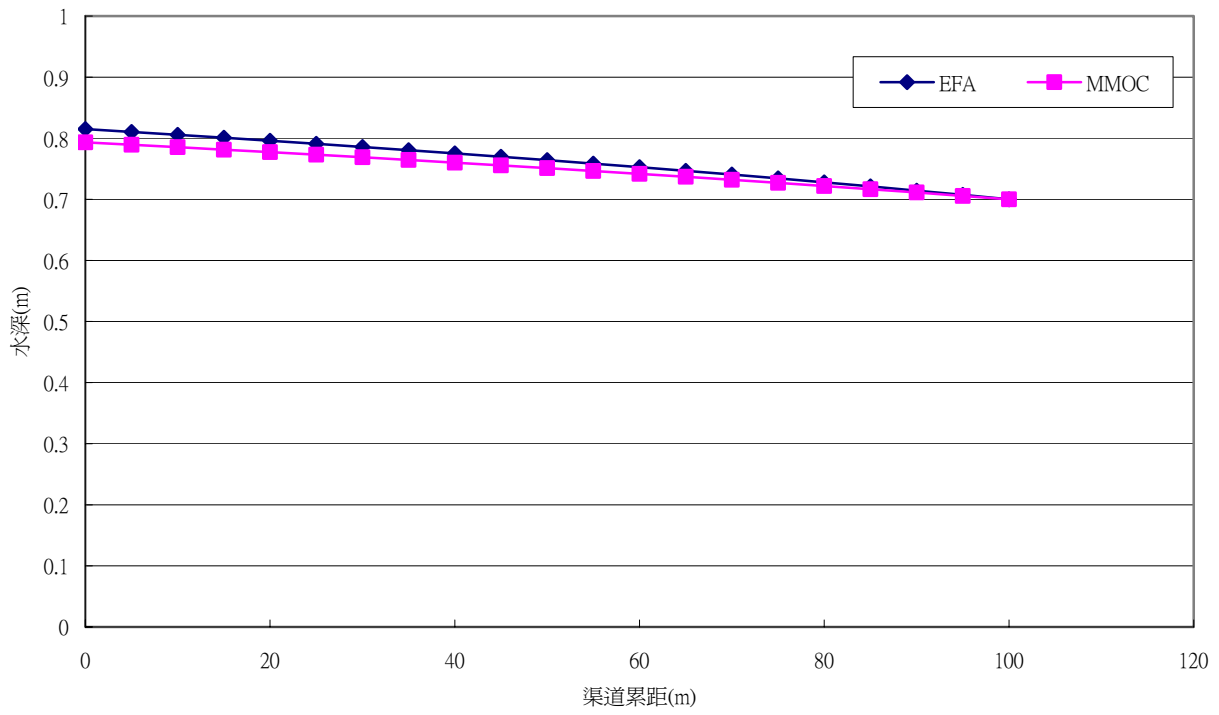
圖 5.11 定量流於分流支渠水深沿程圖
