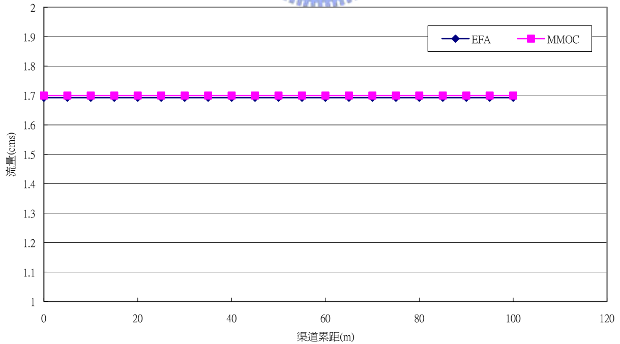
圖 5.12 定量流於分流支渠流量沿程圖
