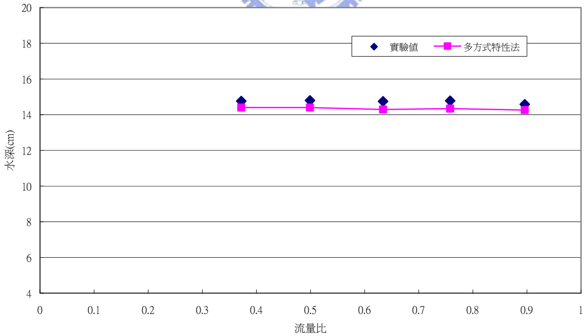
圖 4.11 交匯角度 30 度支流上游水深比較圖
