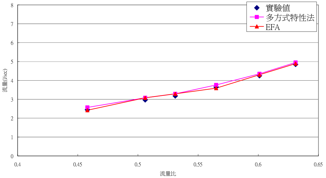
圖 4.17 分流角度 90 度主流下游流量比較圖
