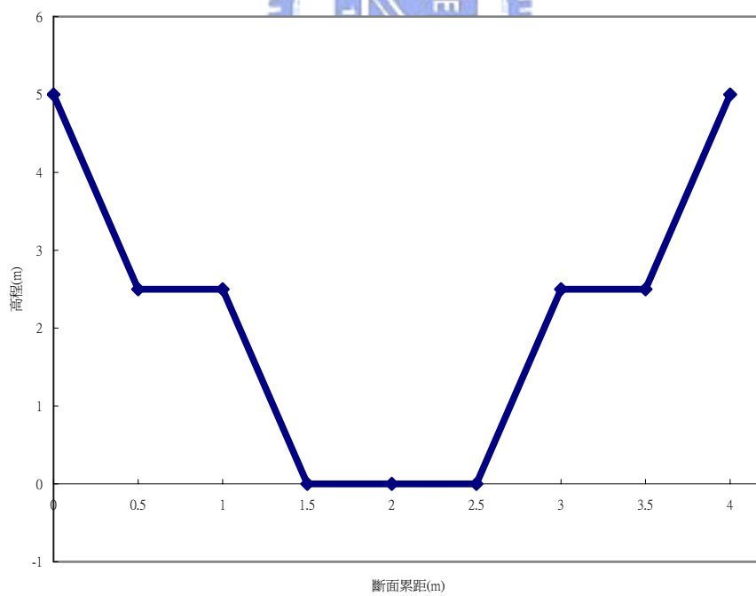
圖 5.17 主渠下游斷面圖
