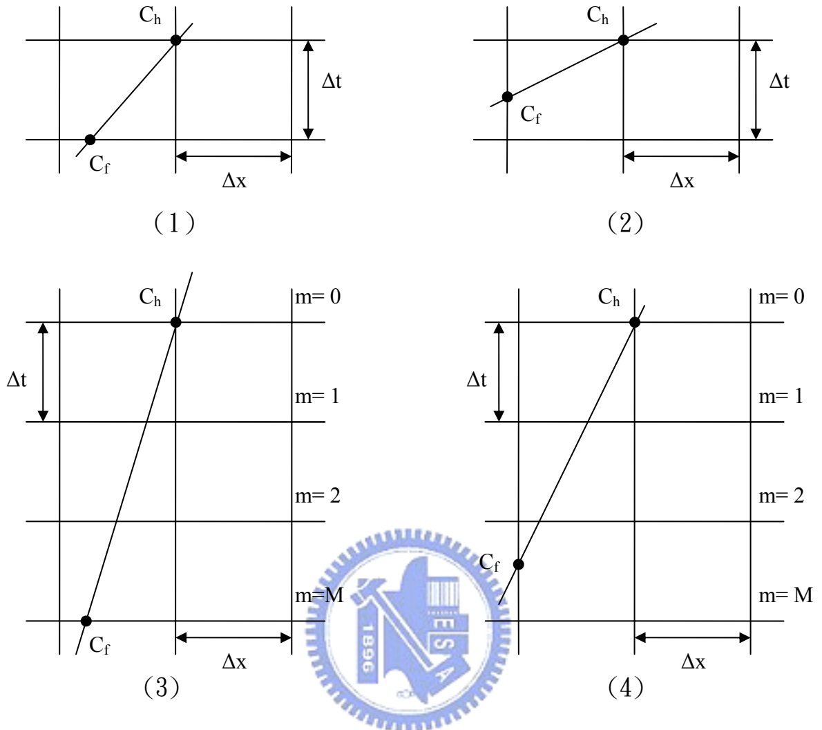
圖 3.1 各特性法之示意圖：(1) 顯式法；(2) 隱式法；(3) 空間延後法；(4) 時間延後法。
