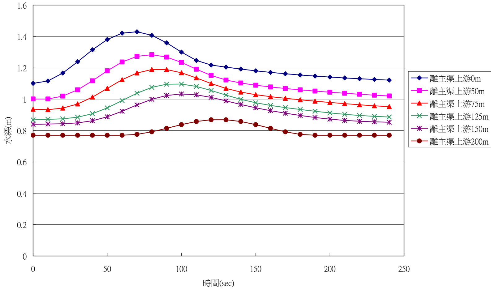
圖 5.15 分流主渠水深延時歷線圖
