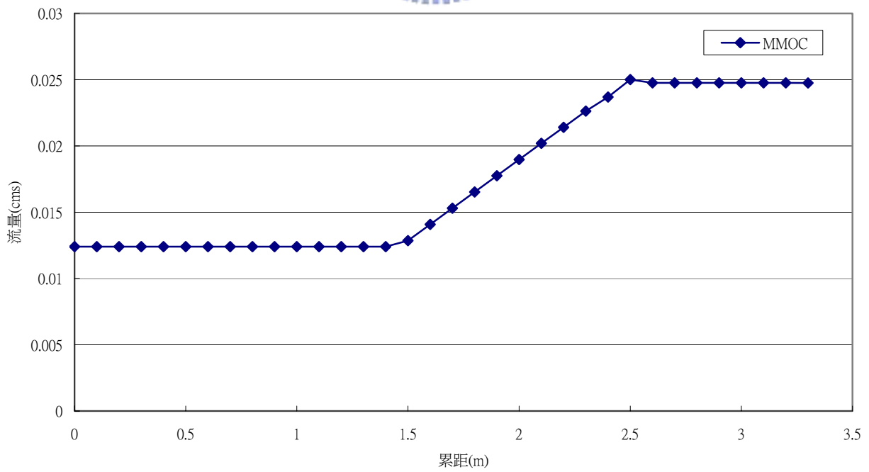
圖 5.3 定量流於合流主渠流量沿程圖
