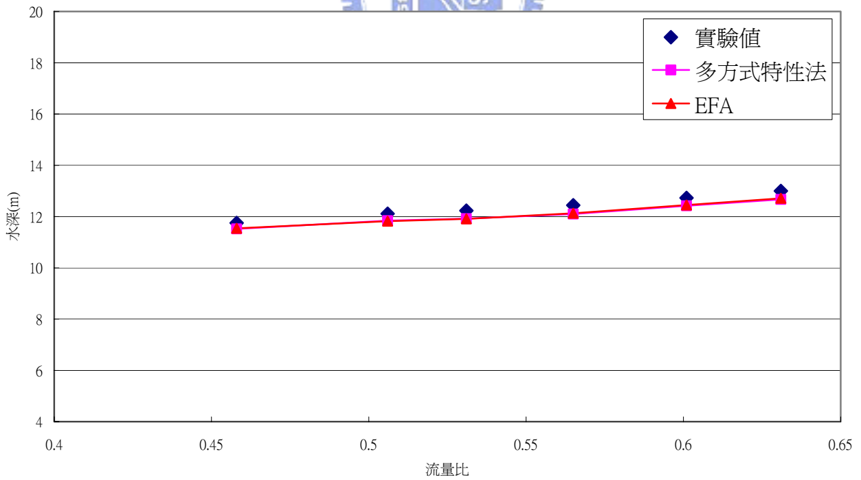
圖 4.18 分流角度 90 度主流上游水深比較圖
