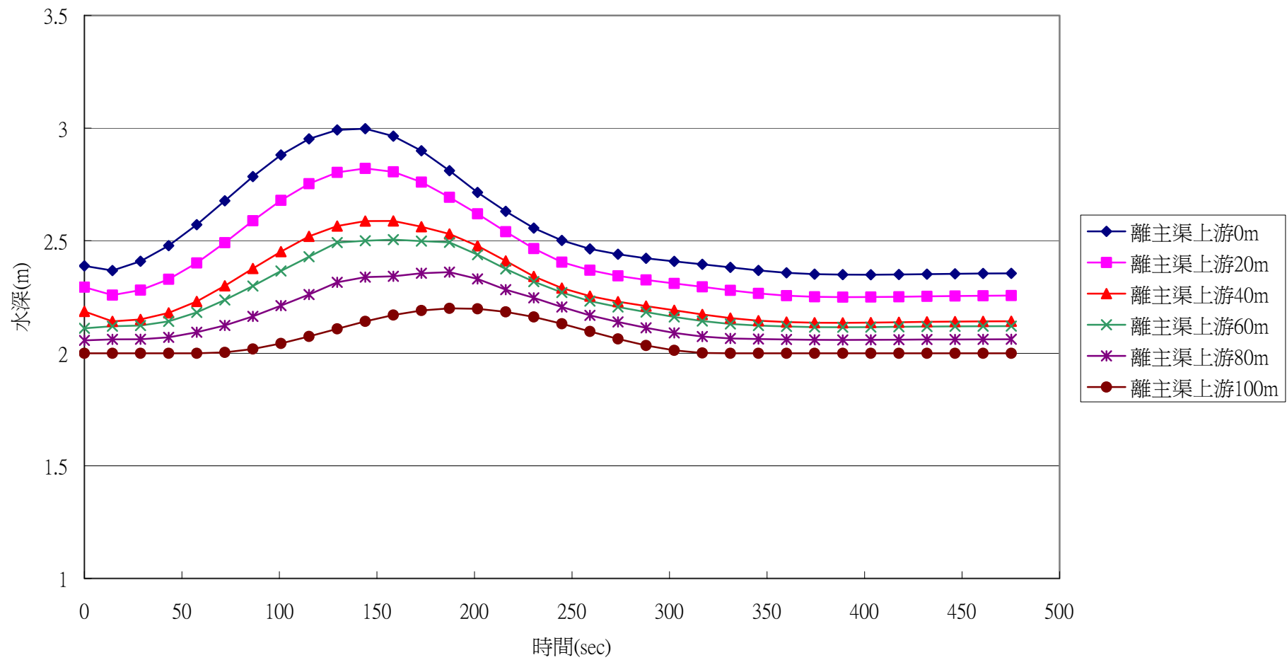
圖 5.20 非矩形渠道主渠水深延時歷線圖
