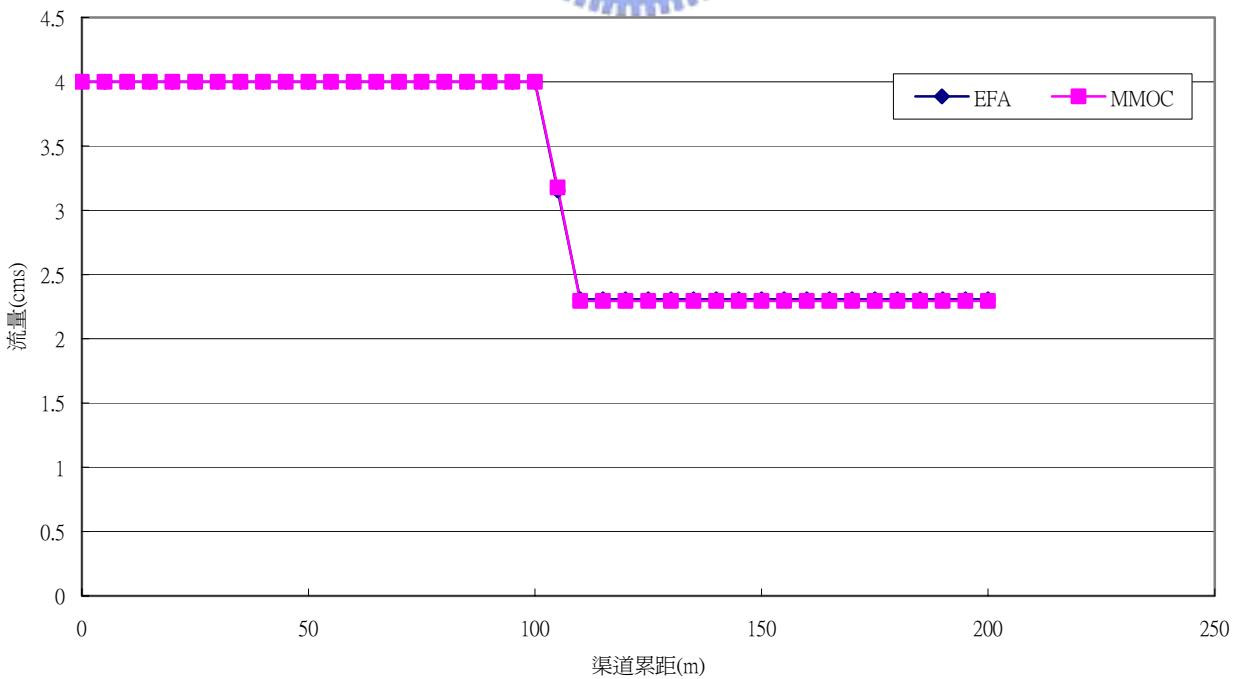
圖 5.10 定量流於分流主渠流量沿程圖
