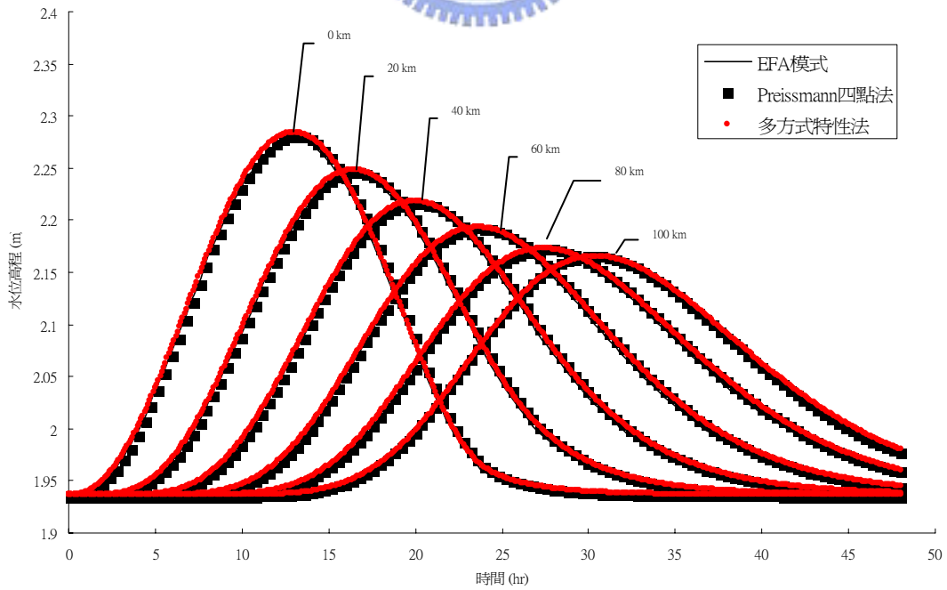
圖 4.3 單一渠道水位延時歷線圖
