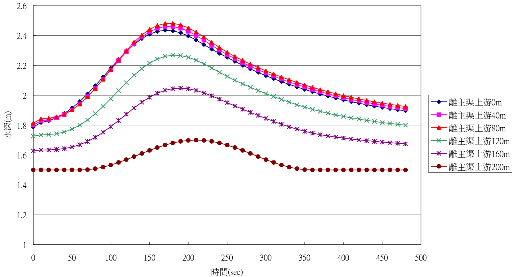
圖 5.8 合流主渠水深延時歷線圖
