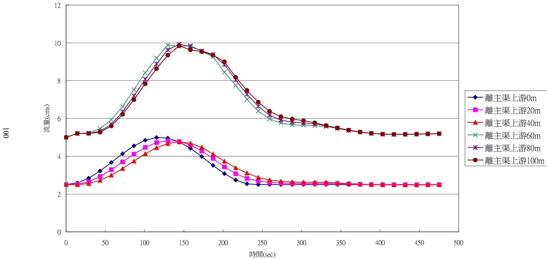
圖 5.18 非矩形渠道主渠流量延時歷線圖
