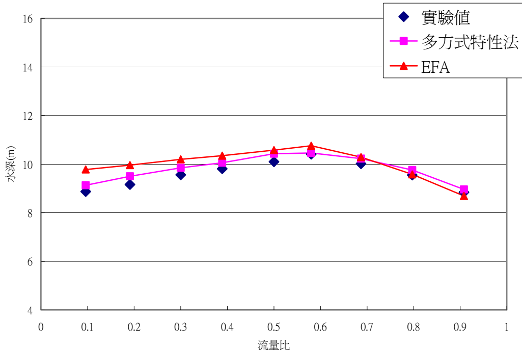
圖 4.6 交匯角度 45 度主流上游水深比較圖
