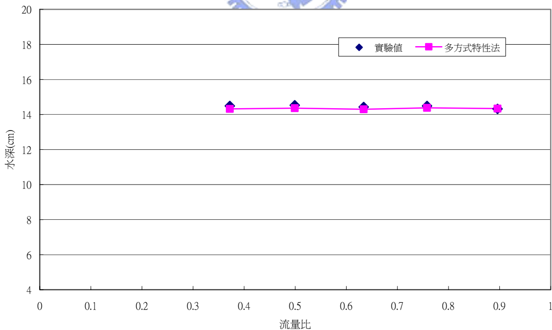
圖 4.10 交匯角度 30 度主流上游水深比較圖
