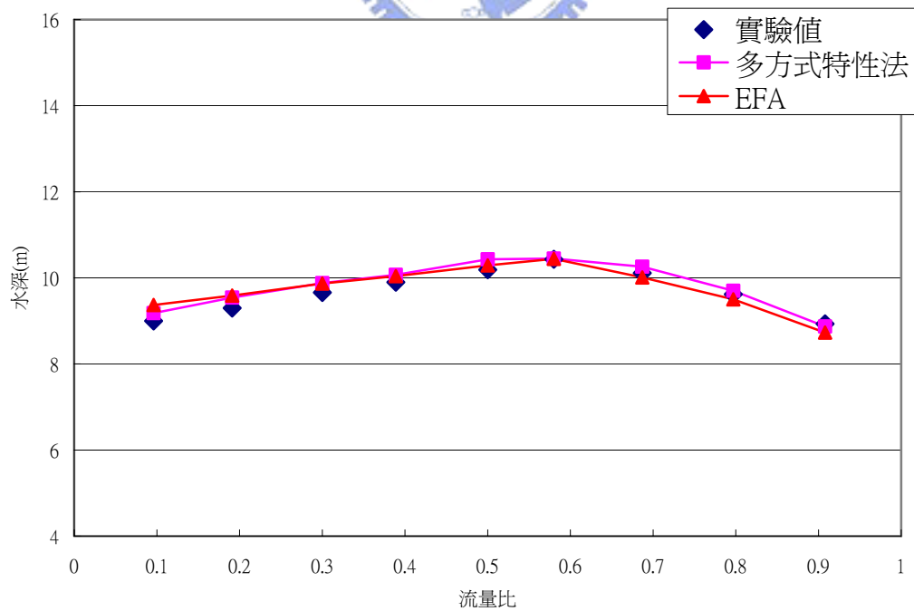
圖 4.7 交匯角度 45 度支流上游水深比較圖
