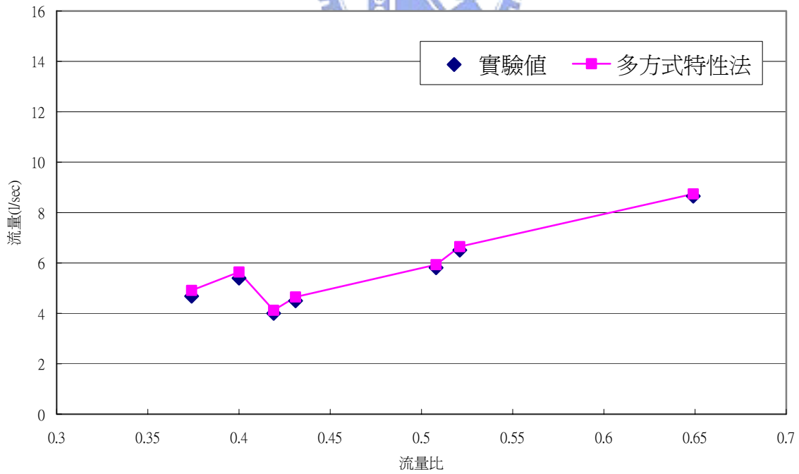
渠寬比 1/3
