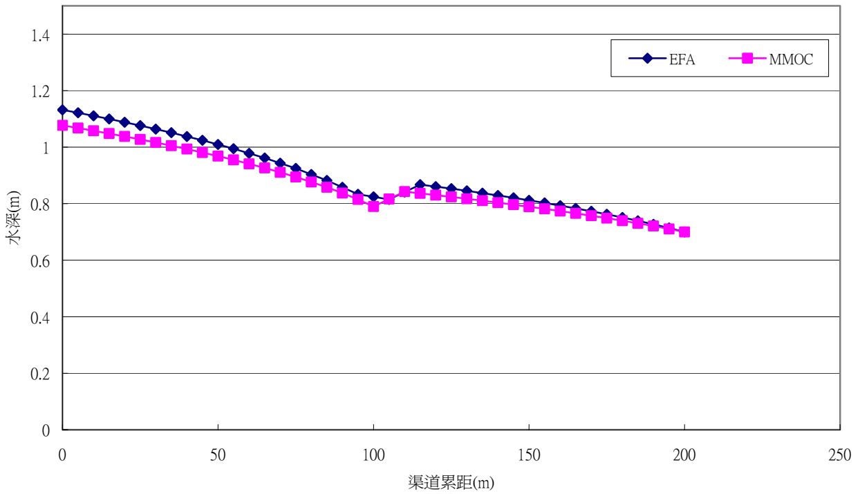
圖 5.9 定量流於分流主渠水深沿程圖
