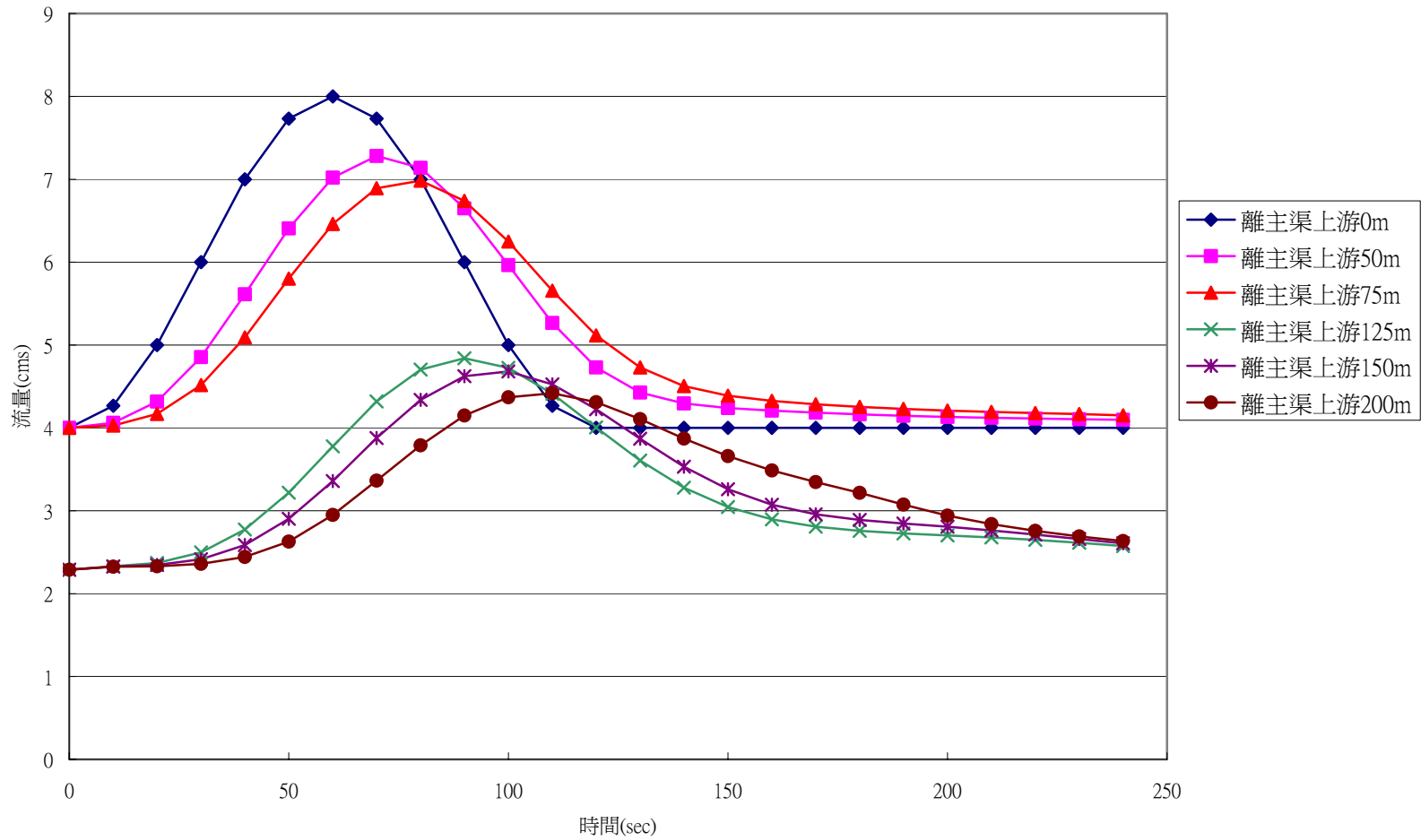
圖 5.13 分流主渠流量延時歷線圖
