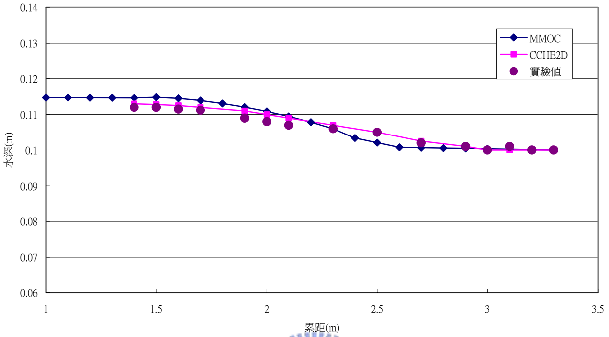
圖 5.2 定量流於合流主渠水深沿程圖
