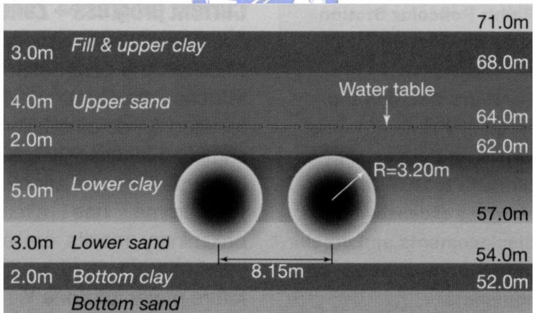
圖 3-12 Bucharest 捷運 Line 4 延伸線隧道工程 地層剖面圖
