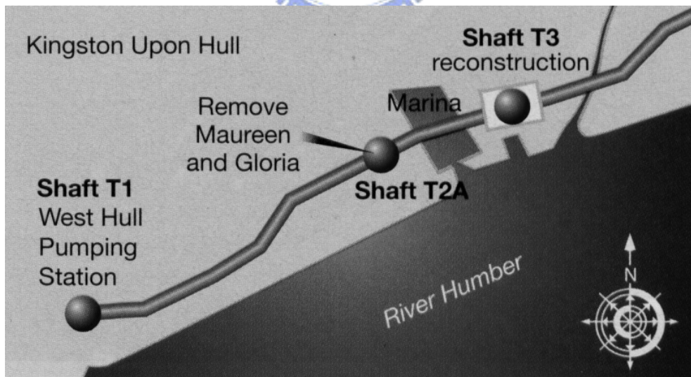
圖 3-9 另外開工作井移除潛盾機
