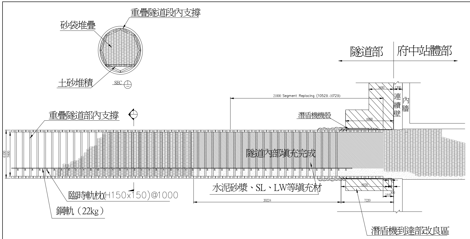
圖 5-25 隧道兩側砂包及袋裝水泥包堆積情形
