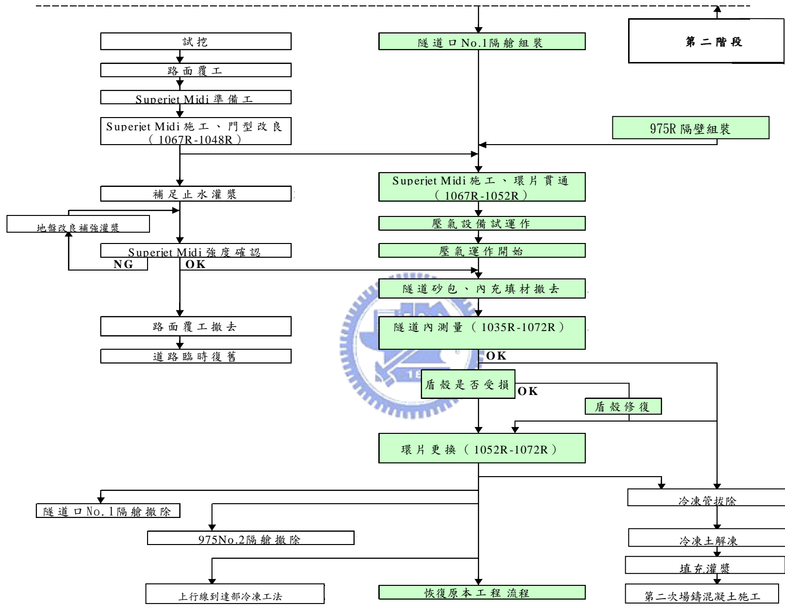
圖 5-40 (b) 整體復舊工程施工流程圖 (摘自 大陸工程, 2003)
