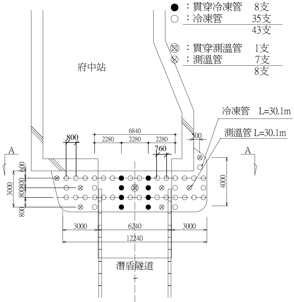
圖 5-41 隧道洞口復原部垂直冷凍管配置圖 (摘自 大陸工程, 2003)
