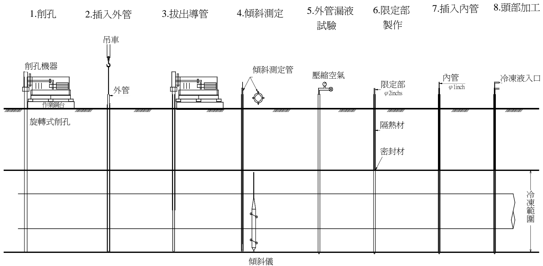
圖 5-43 垂直冷凍管之埋設順序 (摘自 大陸工程, 2003)
