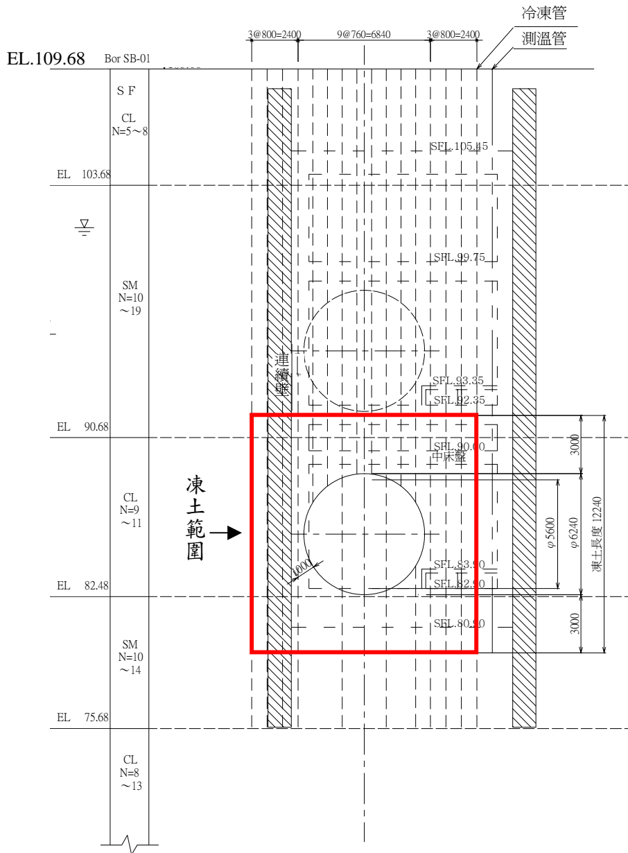
圖 5-42 隧道洞口 A-A 斷面圖 (摘自 大陸工程，2003)
