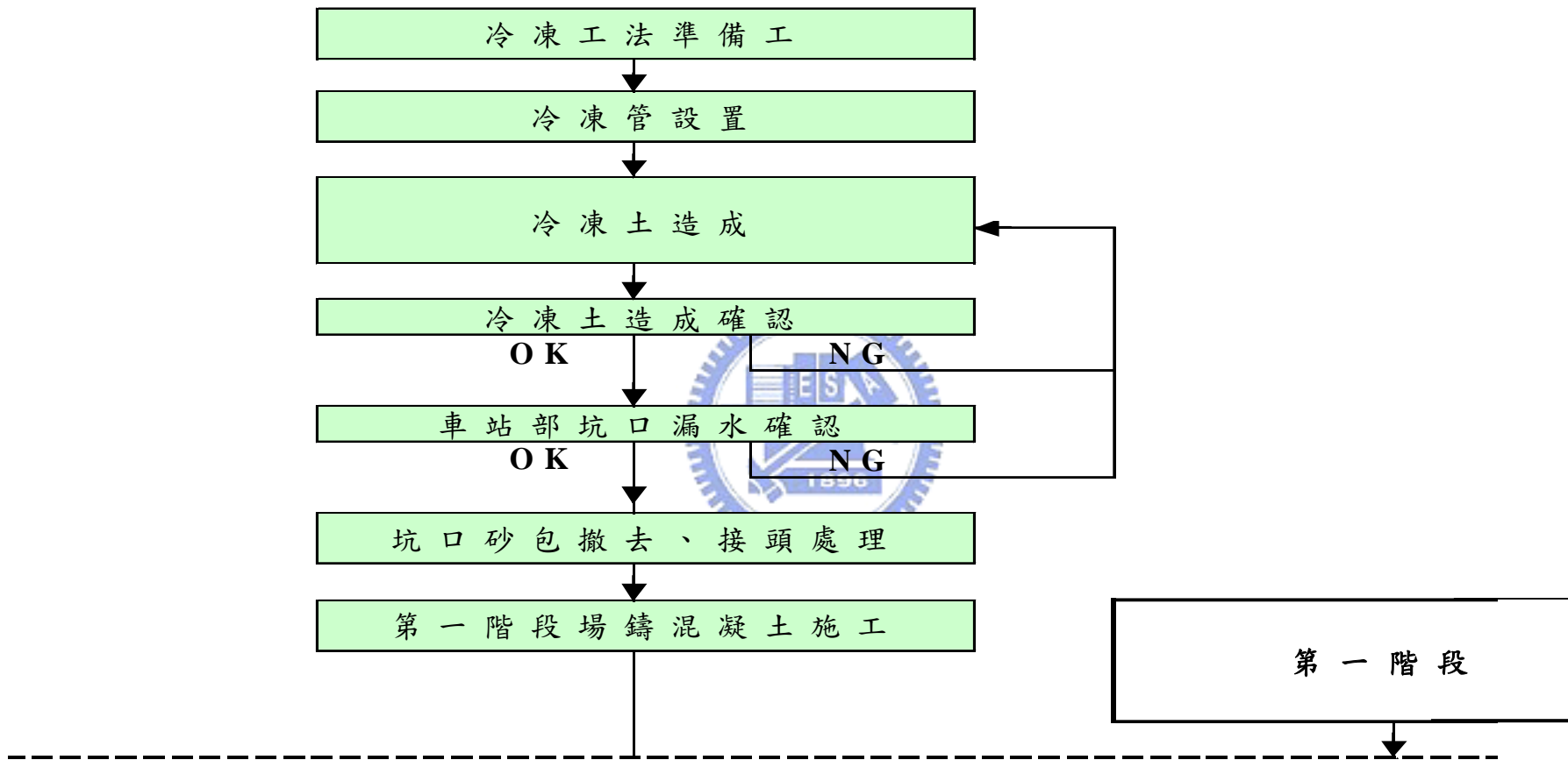
圖 5-40 (a) 整體復舊工程施工流程圖 (摘自 大陸工程，2003)
