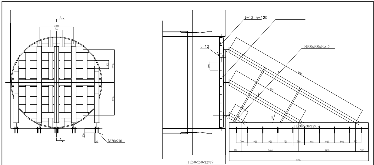
圖 5-55 NO.1 隔艙壁設置圖 (摘自 大陸工程，2003)
