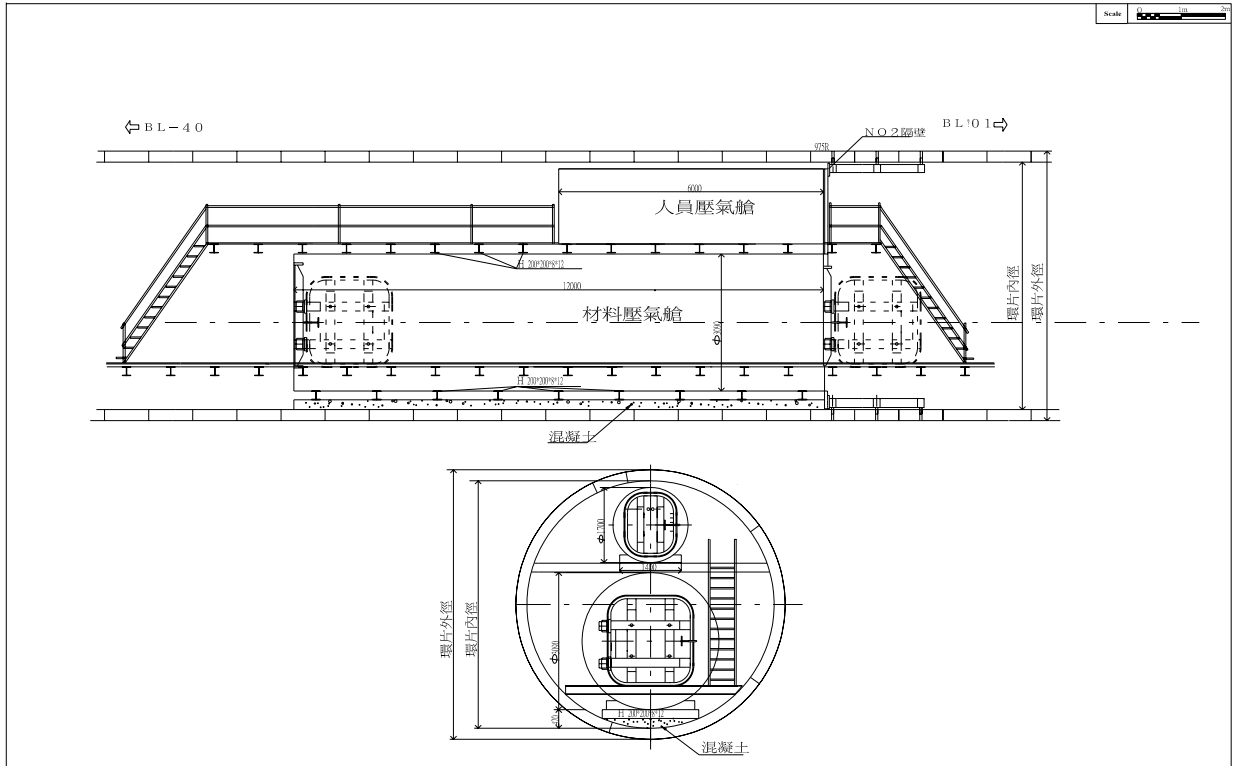
圖 5-57 NO.2 隔艙壁及氣閘室設置圖 (摘自 大陸工程，2003)
