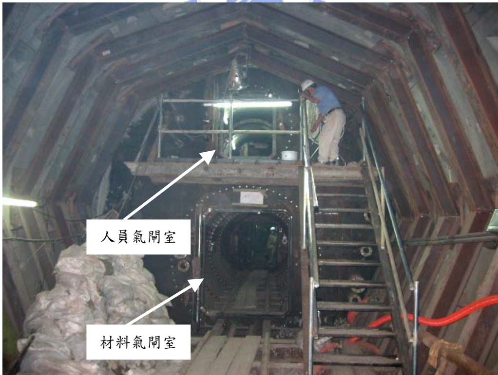
圖 5-58 壓氣工法 NO.2 隔艙組裝完成 (摘自 大陸工程，2003)
