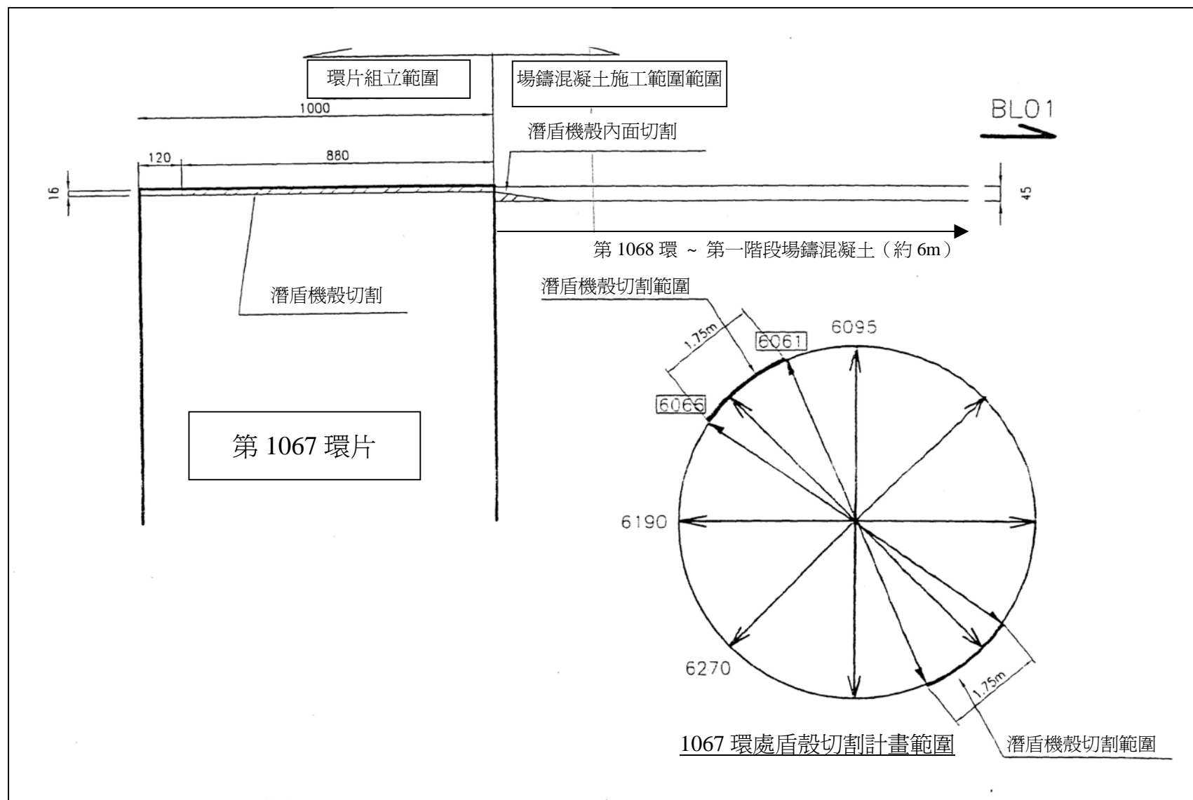
圖 5-62 第 1067 環環片切割範圍圖 (摘自 大陸工程, 2004)
