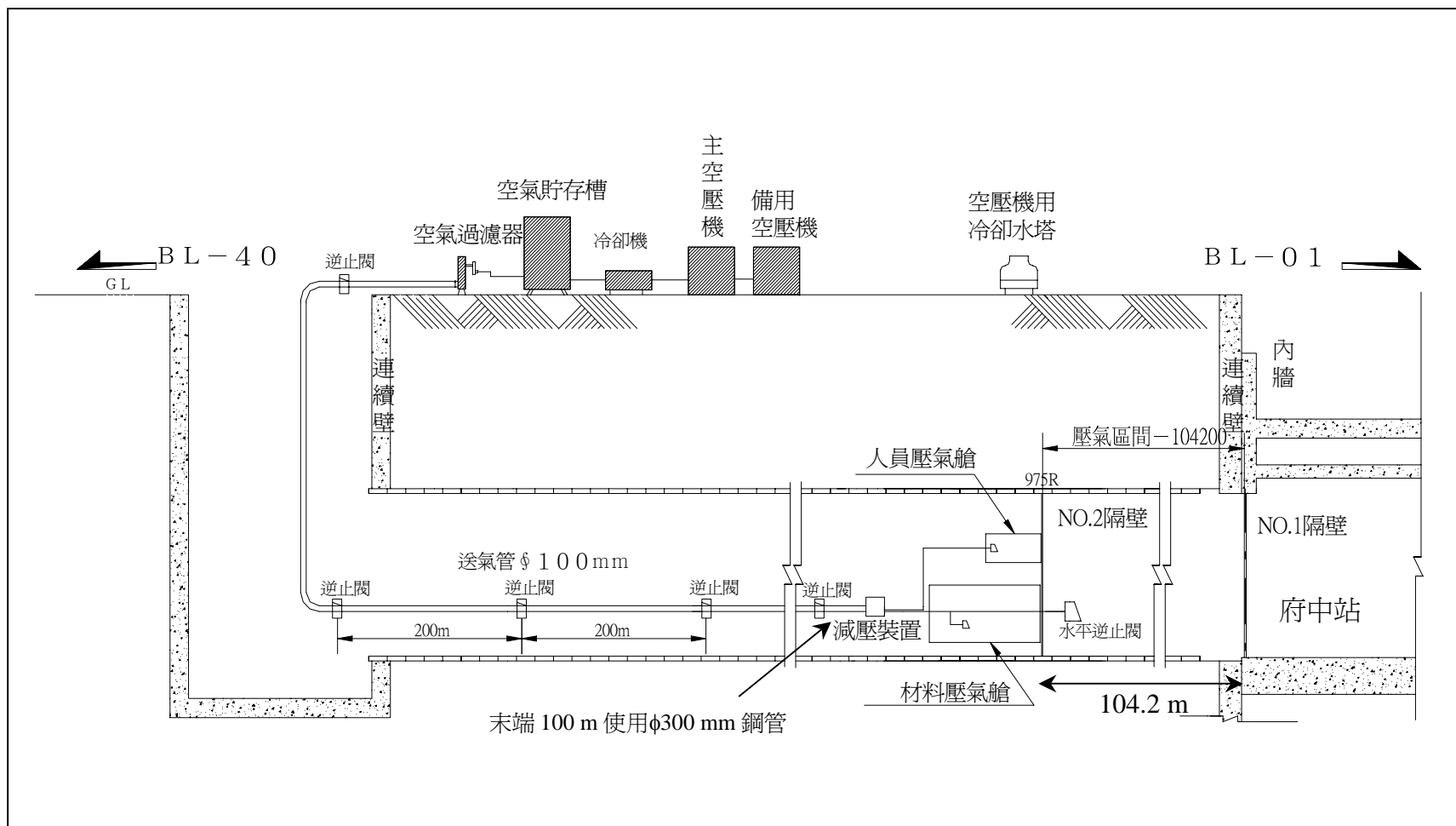
圖 5-54 壓氣設備配置圖 (摘自 大陸工程, 2003)
