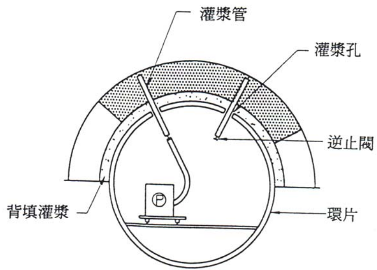
圖 7-13 二次灌漿示意圖
