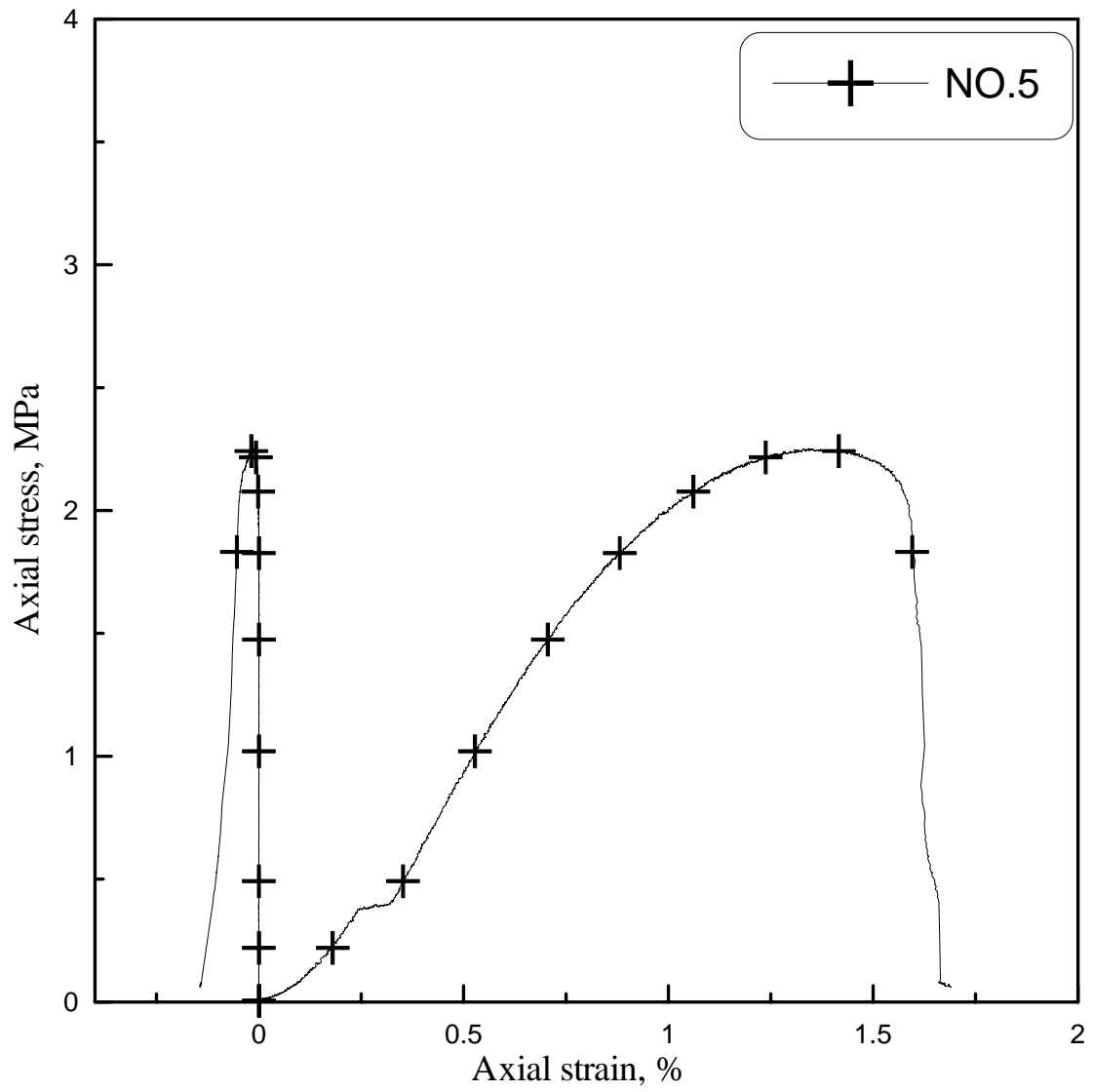
NO.5 全應力應變曲線
