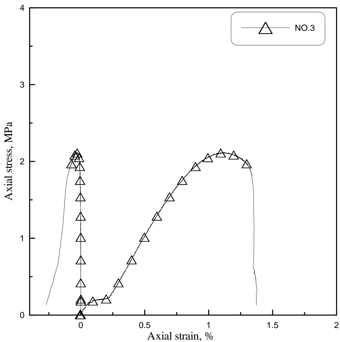
NO.3 全應力應變曲線
