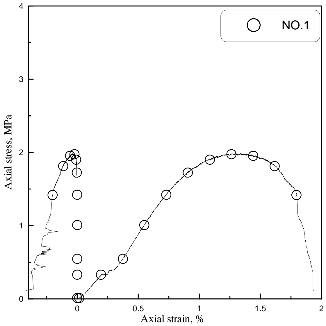
NO.1 全應力應變曲線
