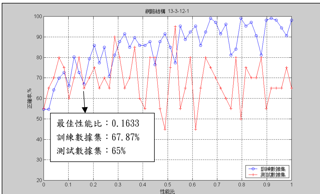
圖 E17、二層隱藏層三及十二個神經元網路訓練結果
