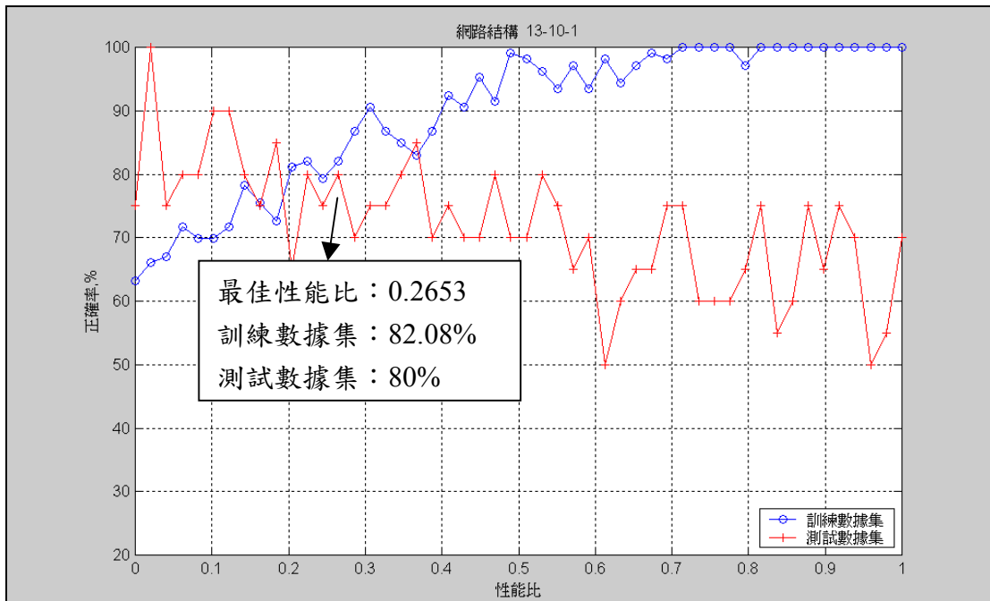
圖 E11、一層隱藏層十個神經元網路訓練結果
