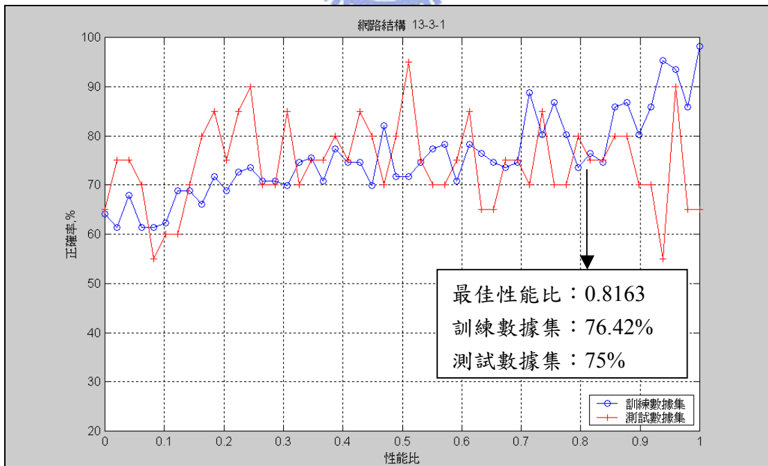
圖 E4、一層隱藏層三個神經元網路訓練結果
