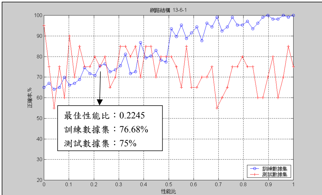
圖 E7、一層隱藏層六個神經元網路訓練結果
