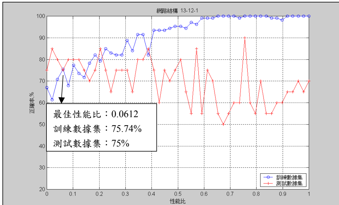
圖 E13、一層隱藏層十二個神經元
