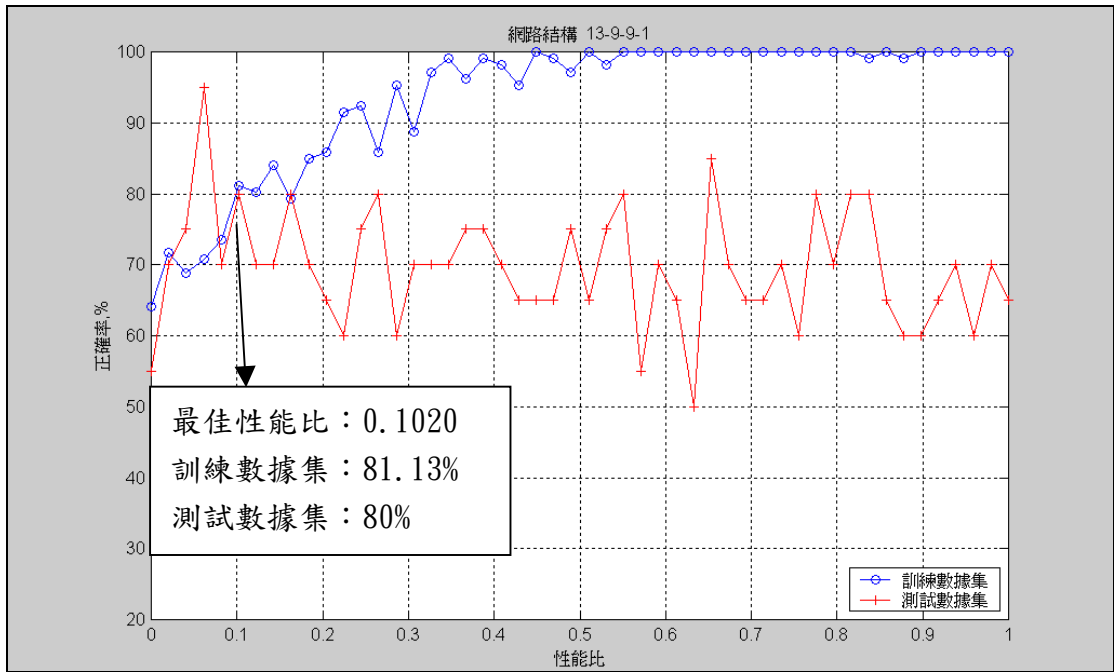
圖 E24、二層隱藏層九及九個神經元網路訓練結果
