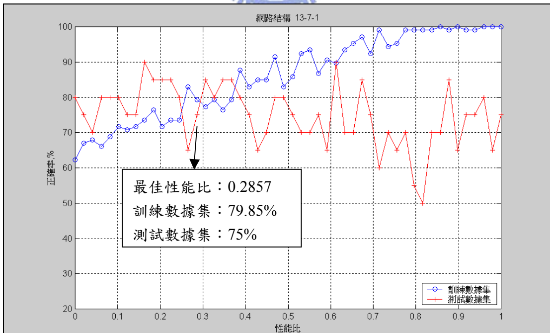
圖 E8、一層隱藏層七個神經元網路訓練結果
