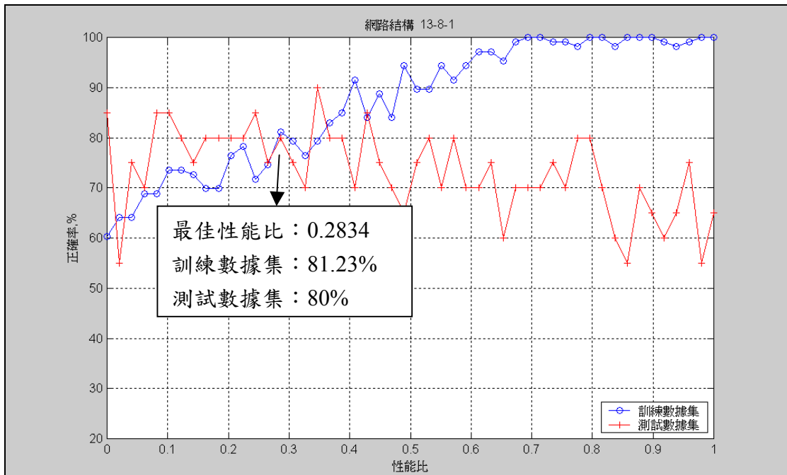
圖 E9、一層隱藏層八個神經元網路訓練結果
