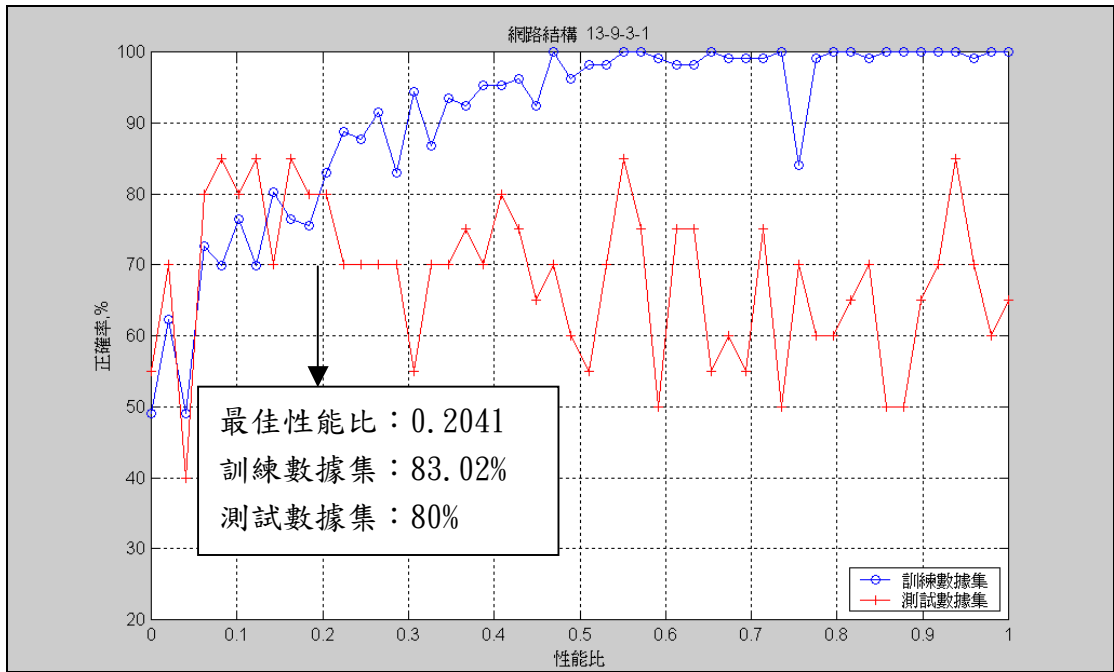
圖 E22、二層隱藏層九及三個神經元網路訓練結果
