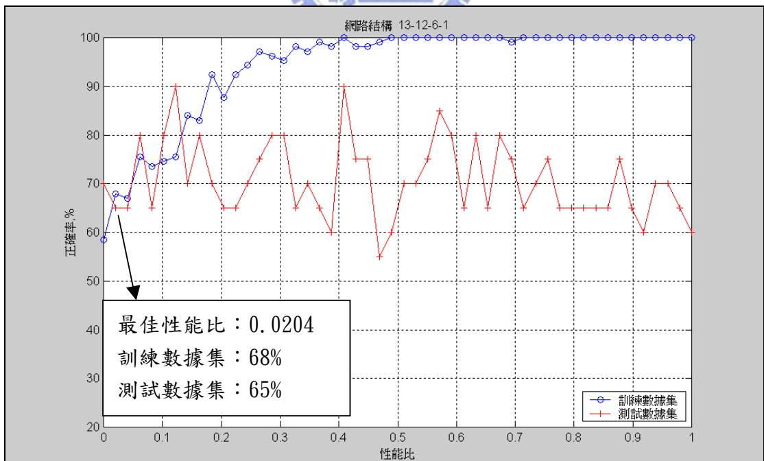
圖 E27、二層隱藏層十二及六個神經元網路訓練結果
