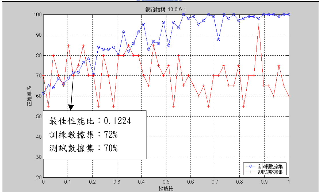
圖 E19、二層隱藏層六及六個神經元網路訓練結果
