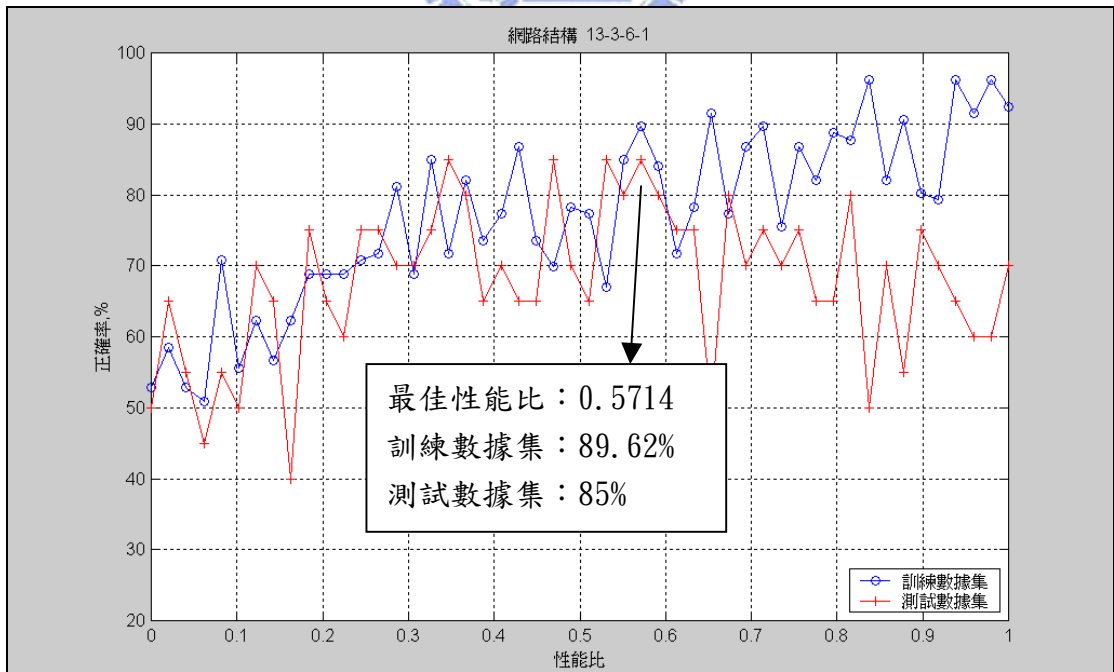
圖 E15、二層隱藏層三及六個神經元網路訓練結果
