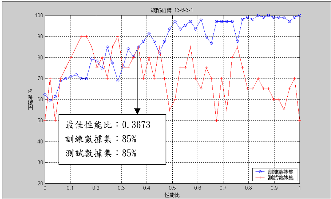
圖 E18、二層隱藏層六及三個神經元網路訓練結果
