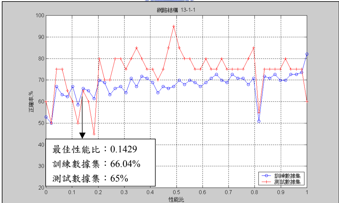
圖 E2、一層隱藏層一個神經元網路訓練結果
