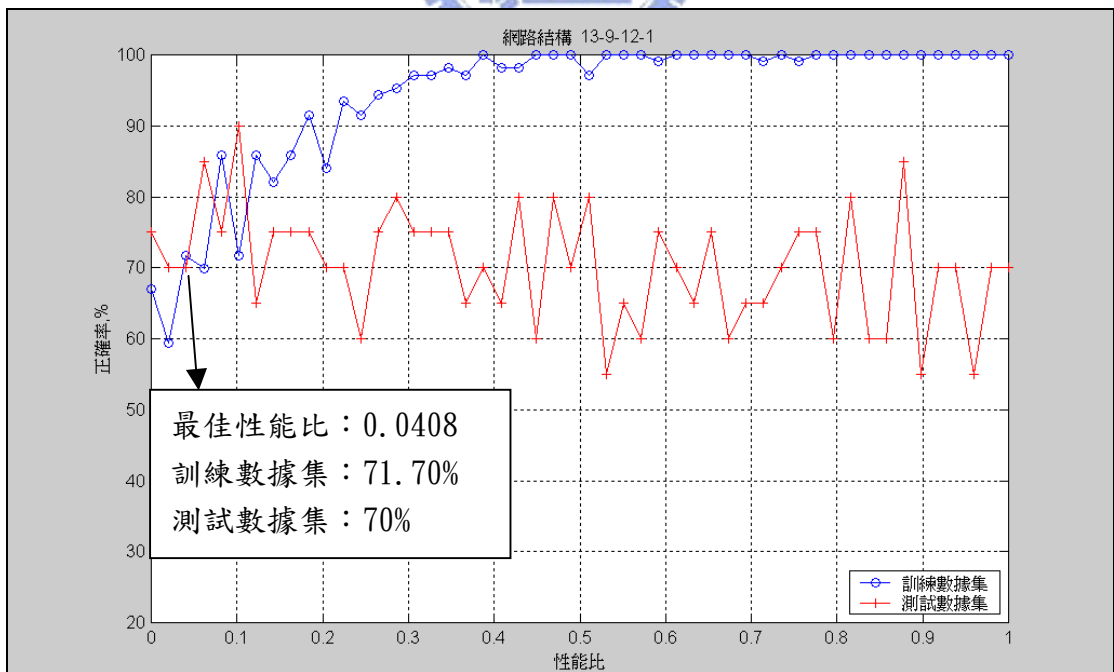
圖 E25、二層隱藏層九及十二個神經元網路訓練結果
