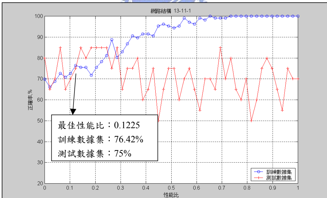
圖 E12、一層隱藏層十一個神經元
