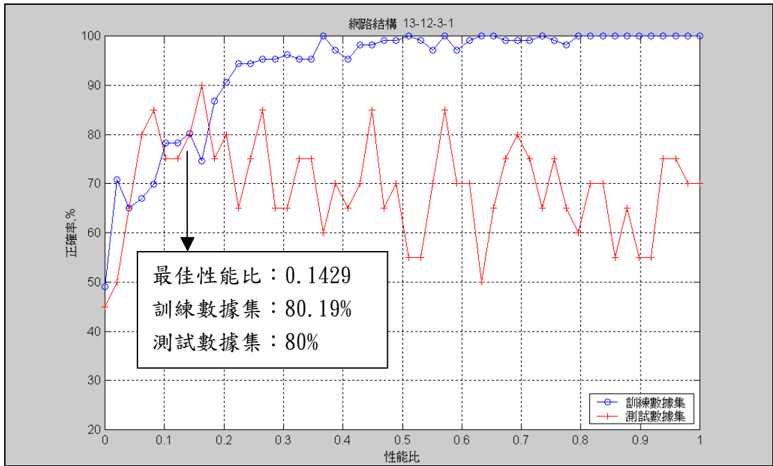
圖 E26、二層隱藏層十二及三個神經元網路訓練結果
