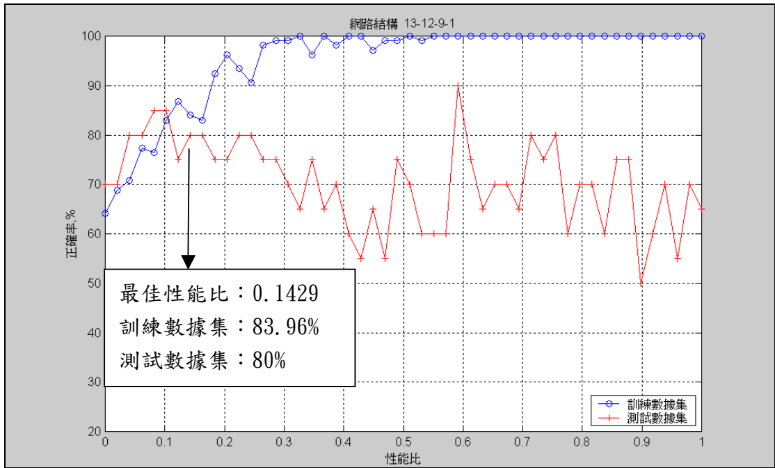
圖 E28、二層隱藏層十二及九個神經元網路訓練結果
