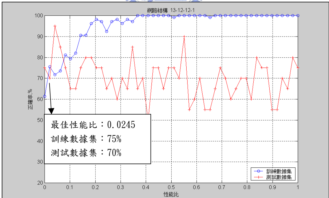
圖 E29、二層隱藏層十二及十二個神經元網路訓練結果
