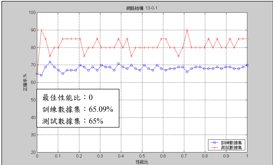
圖 E1、無隱藏層網路訓練結果
