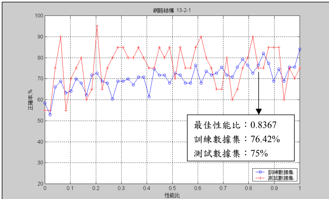
圖 E3、一層隱藏層二個神經元網路訓練結果
