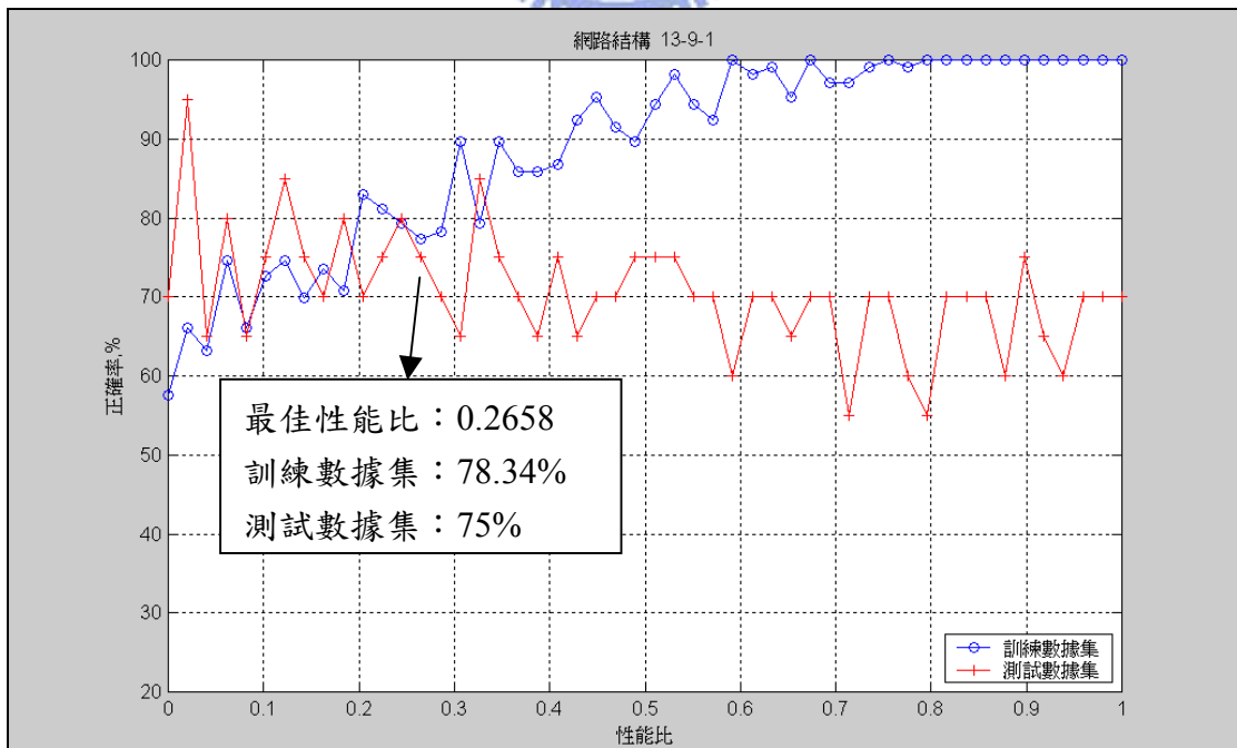
圖 E10、一層隱藏層九個神經元網路訓練結果
