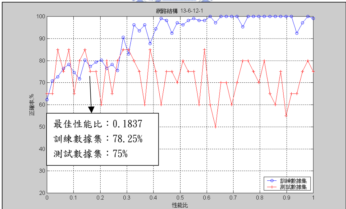
圖 E21、二層隱藏層六及十二個神經元網路訓練結果
