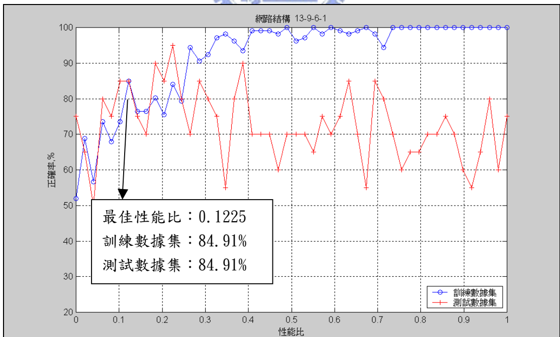
圖 E23、二層隱藏層九及六個神經元網路訓練結果
