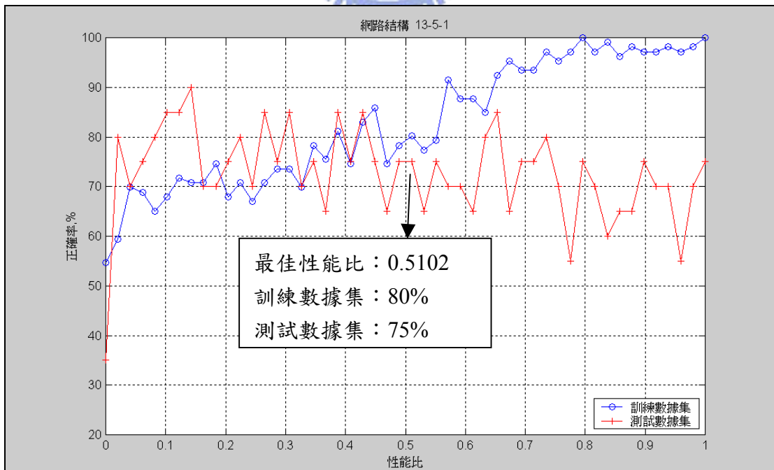
圖 E6、一層隱藏層五個神經元網路訓練結果
