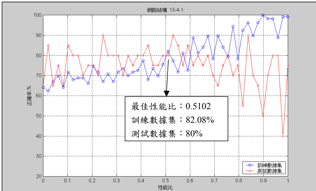
圖 E5、一層隱藏層四個神經元網路訓練結果
