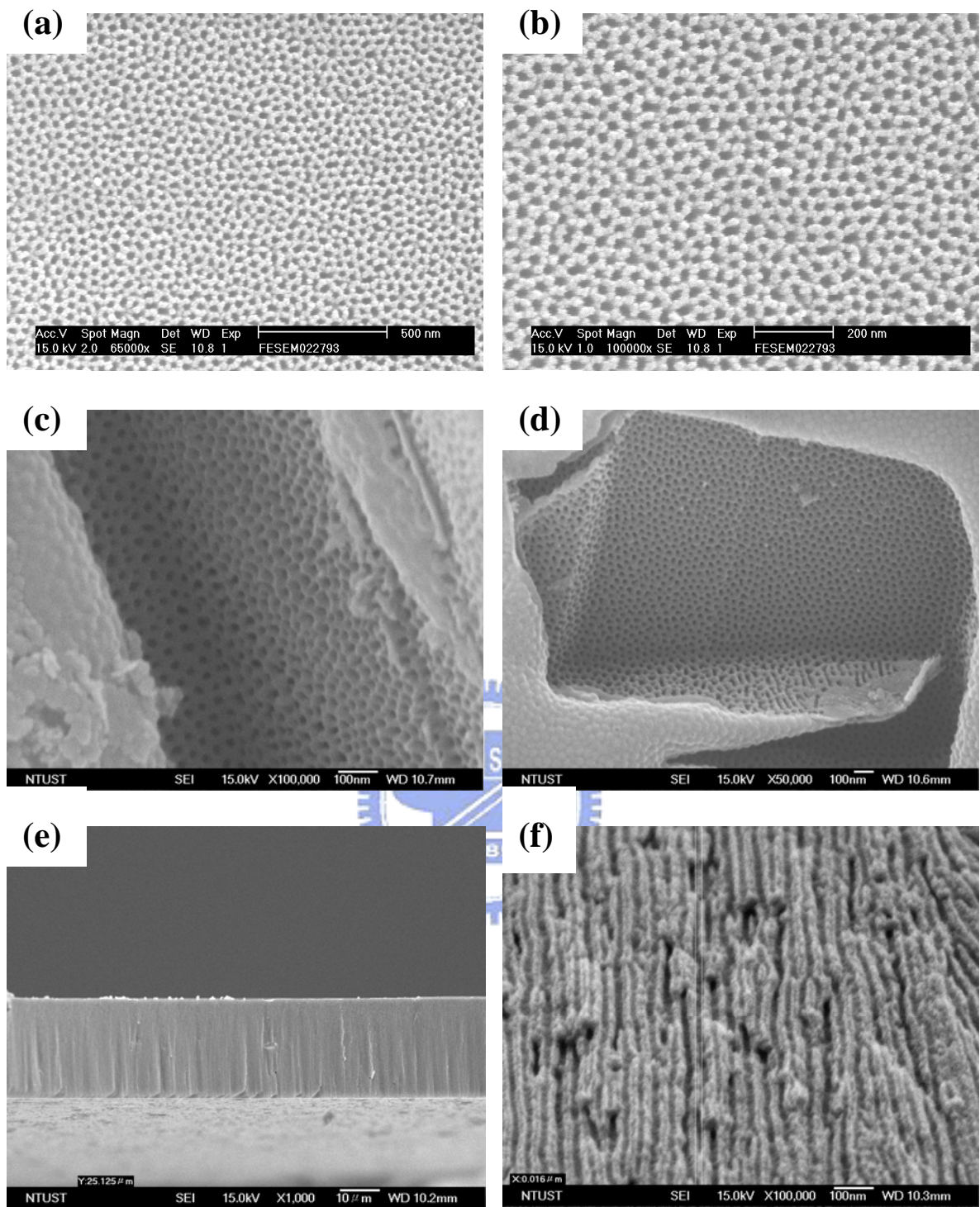
圖 4-11 硫酸( H_2SO_4 )AAO 之 SEM 俯視圖(a)~(d)和剖面圖(e)、(f)，倍率分別為(a) 65,000x (b) 100,000x (c) 100,000x (d) 50,000x (e) 10,000x (f) 50,000x。工作條件:電壓 10V, 溫度 5^{\circ}C , 時間 6hr,轉速 300rpm 和二次的陽極處理
