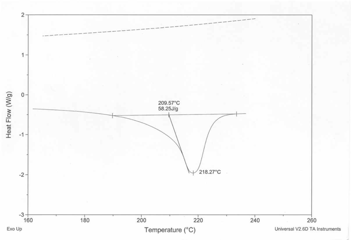
附圖 9. PBFBPOMe 之 DSC 圖
