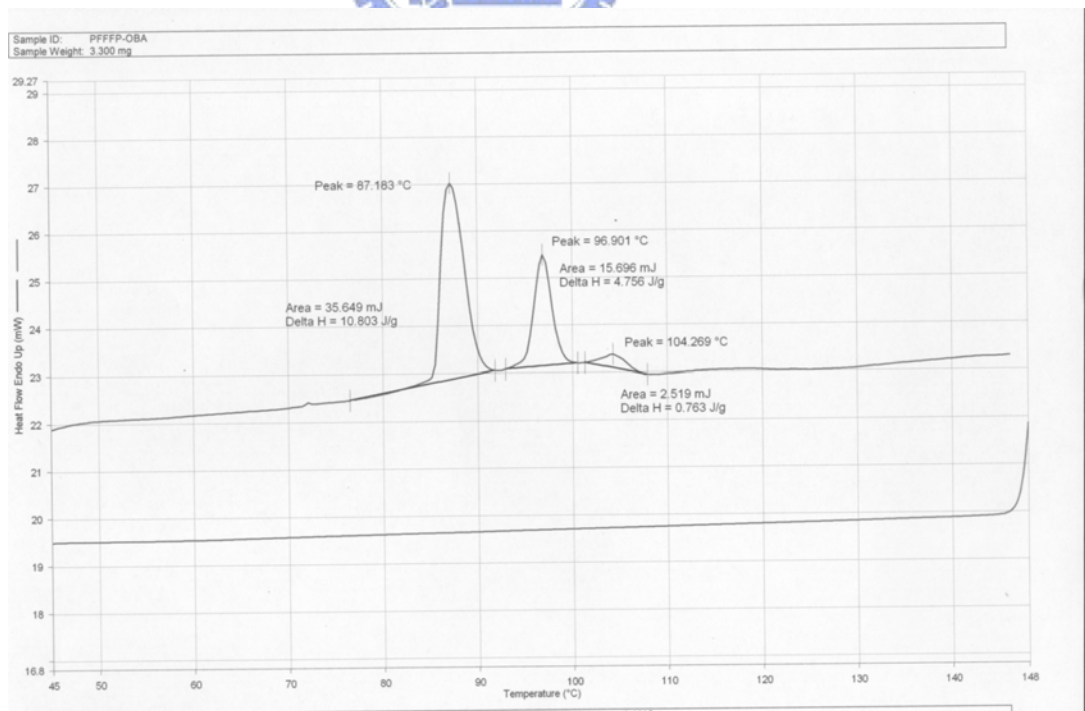
附圖 24. PFFFP-OBA 之 DSC 圖
