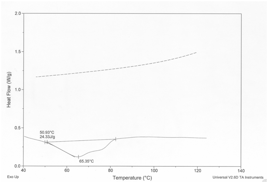
附圖 17. PFBPMe-THA 之 DSC 圖
