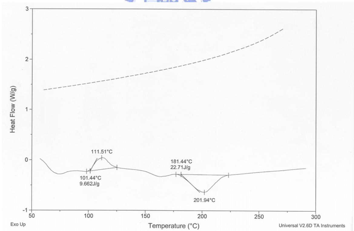
附圖 14. PFBPMe 之 DSC 圖
