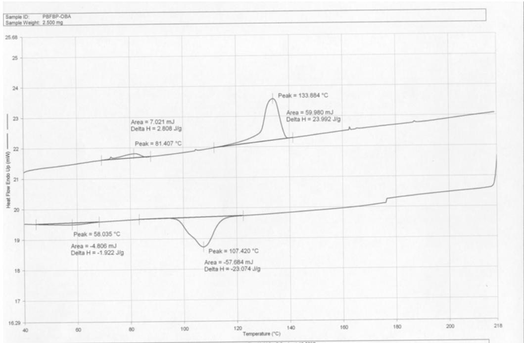
附圖 19. PBFBP-OBA 之 DSC 圖
