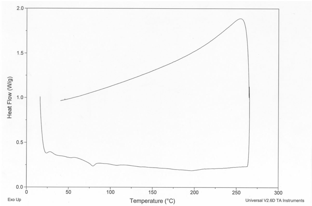
附圖 23. PFFFP 之 DSC 圖
