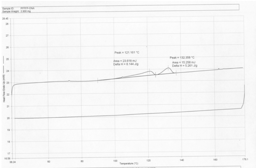
附圖 25. PFFFFP-ONA 之 DSC 圖
