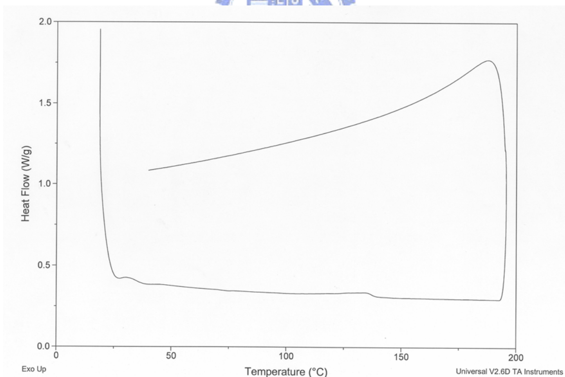
附圖 26. PFFFFP-THA 之 DSC 圖
