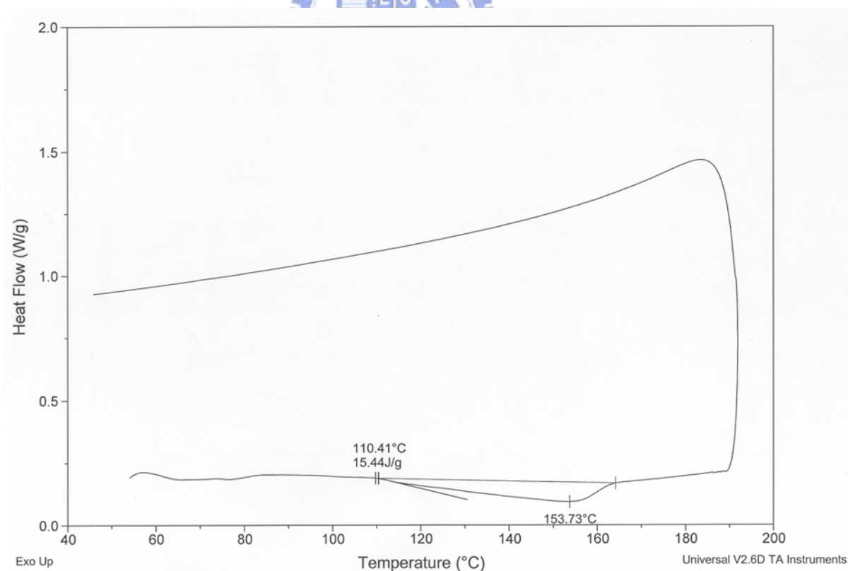
附圖 12. PBFBPOMe-THA 之 DSC 圖
