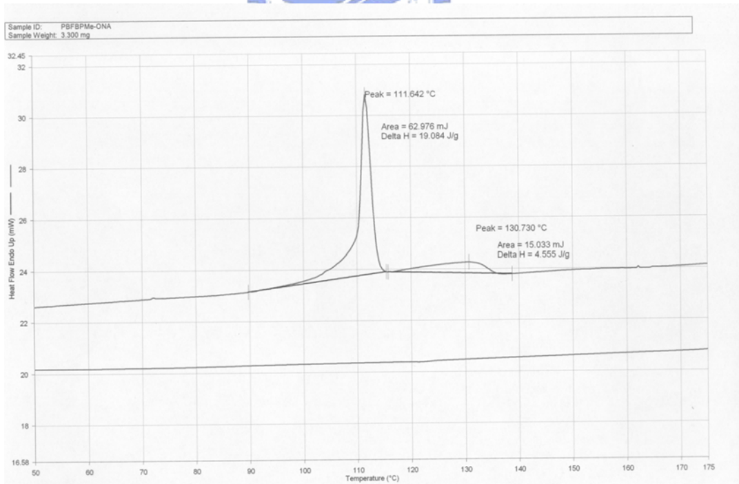
附圖 16. PFBPMe-ONA 之 DSC 圖
