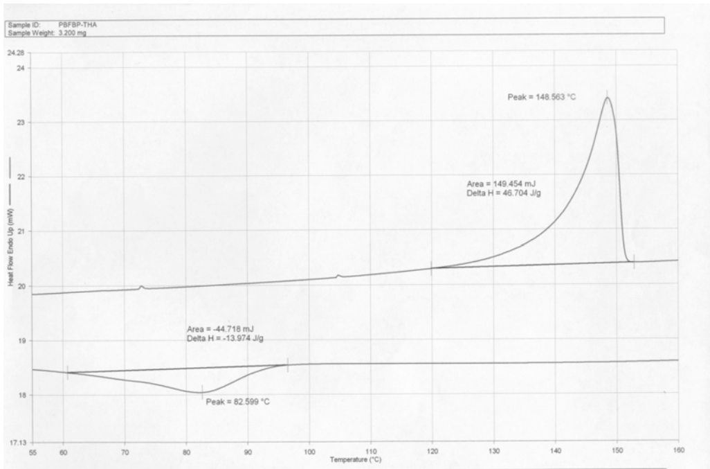
附圖 21. PBFBP-THA 之 DSC 圖
