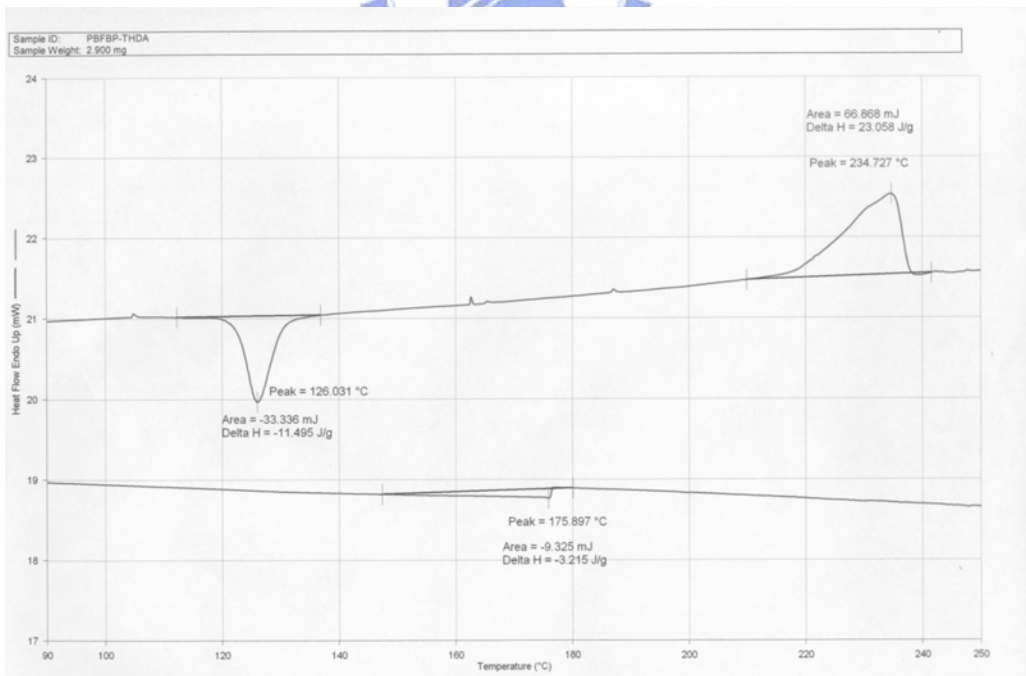
附圖 22. PBFBP-THDA 之 DSC 圖
