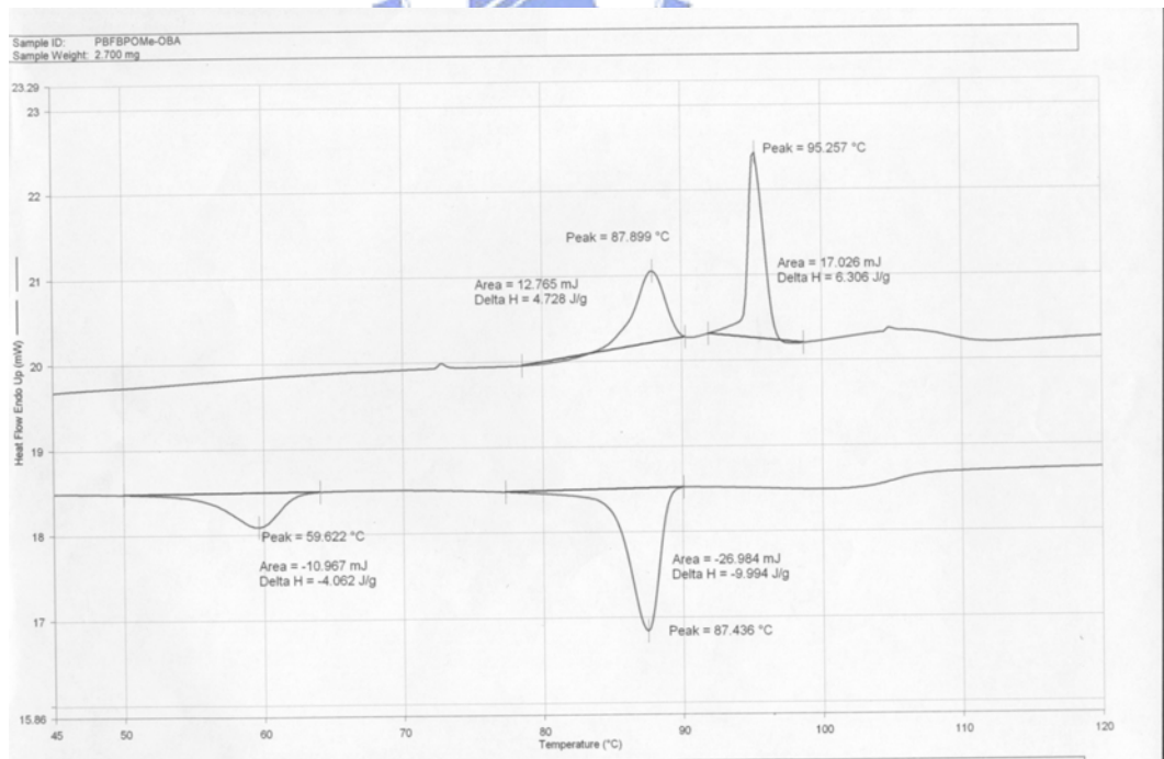
附圖 10. PBFBPOMe-OBA 之 DSC 圖
