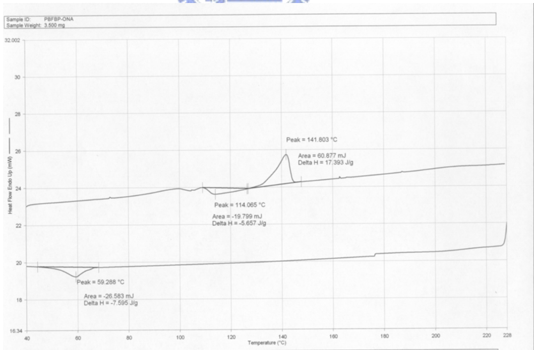
附圖 20. PBFBP-ONA 之 DSC 圖
