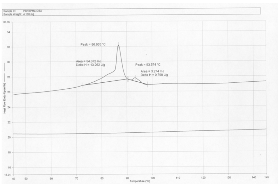
附圖 15. PFBPMe-OBA 之 DSC 圖
