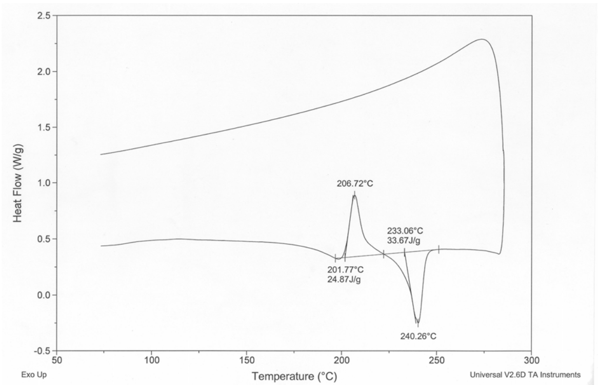
附圖 13. PFBPOMe-THDA 之 DSC 圖
