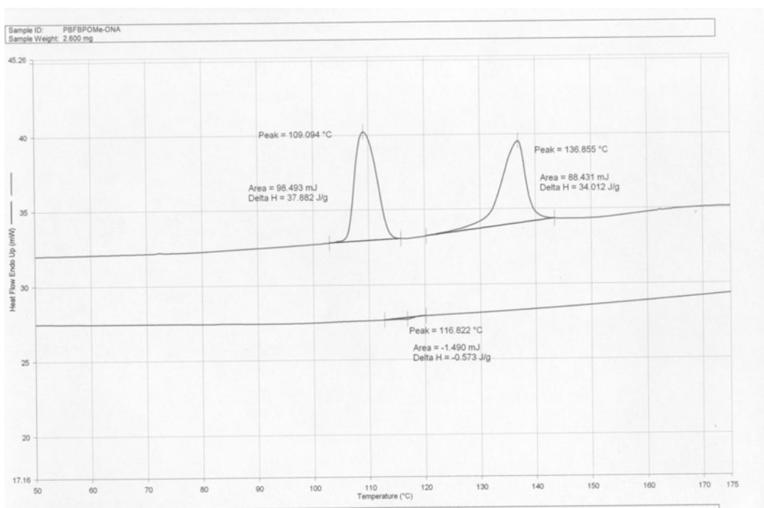
附圖 11. PBFBPOMe-ONA 之 DSC 圖
