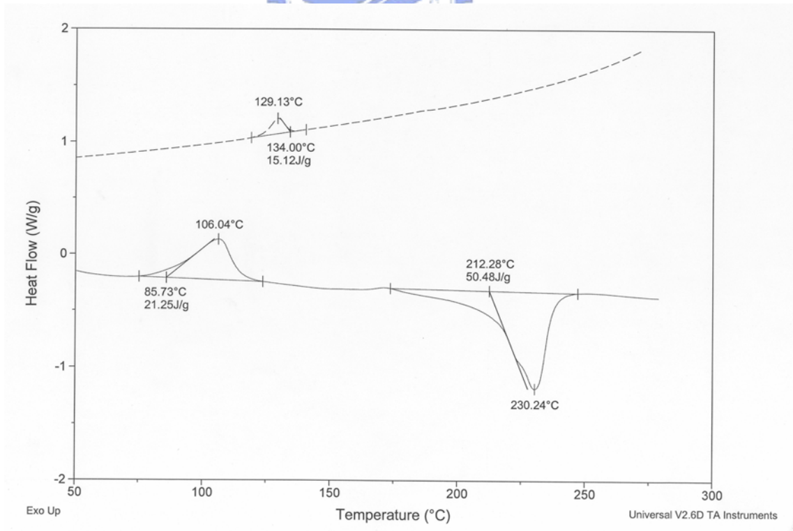
附圖 18. PFBFP 之 DSC 圖
