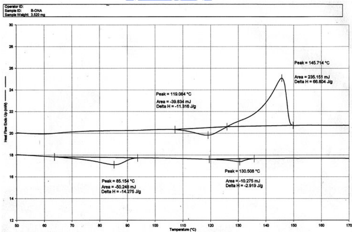
附圖 14 PFBFP3-ONA 之 DSC 圖
