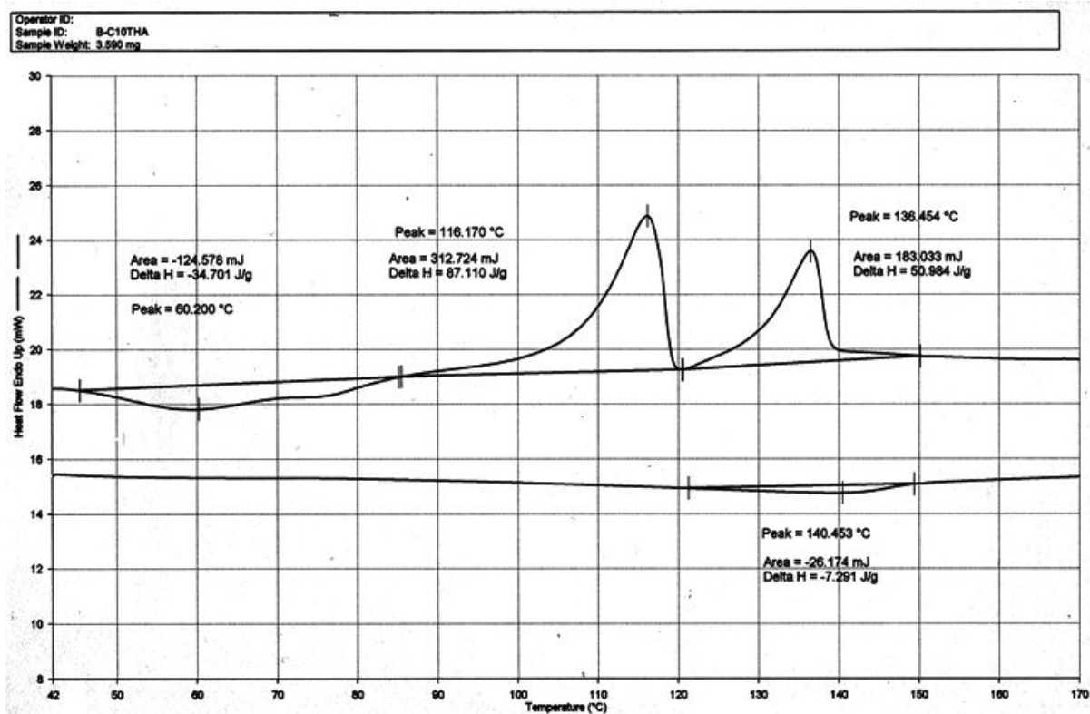
附圖 15 PFBFP3-THA 之 DSC 圖
