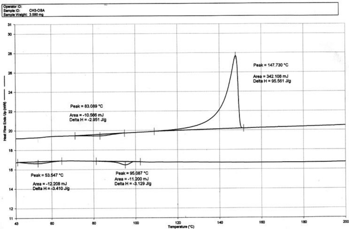
附圖 17 PFBFP3Me-OBA 之 DSC 圖
