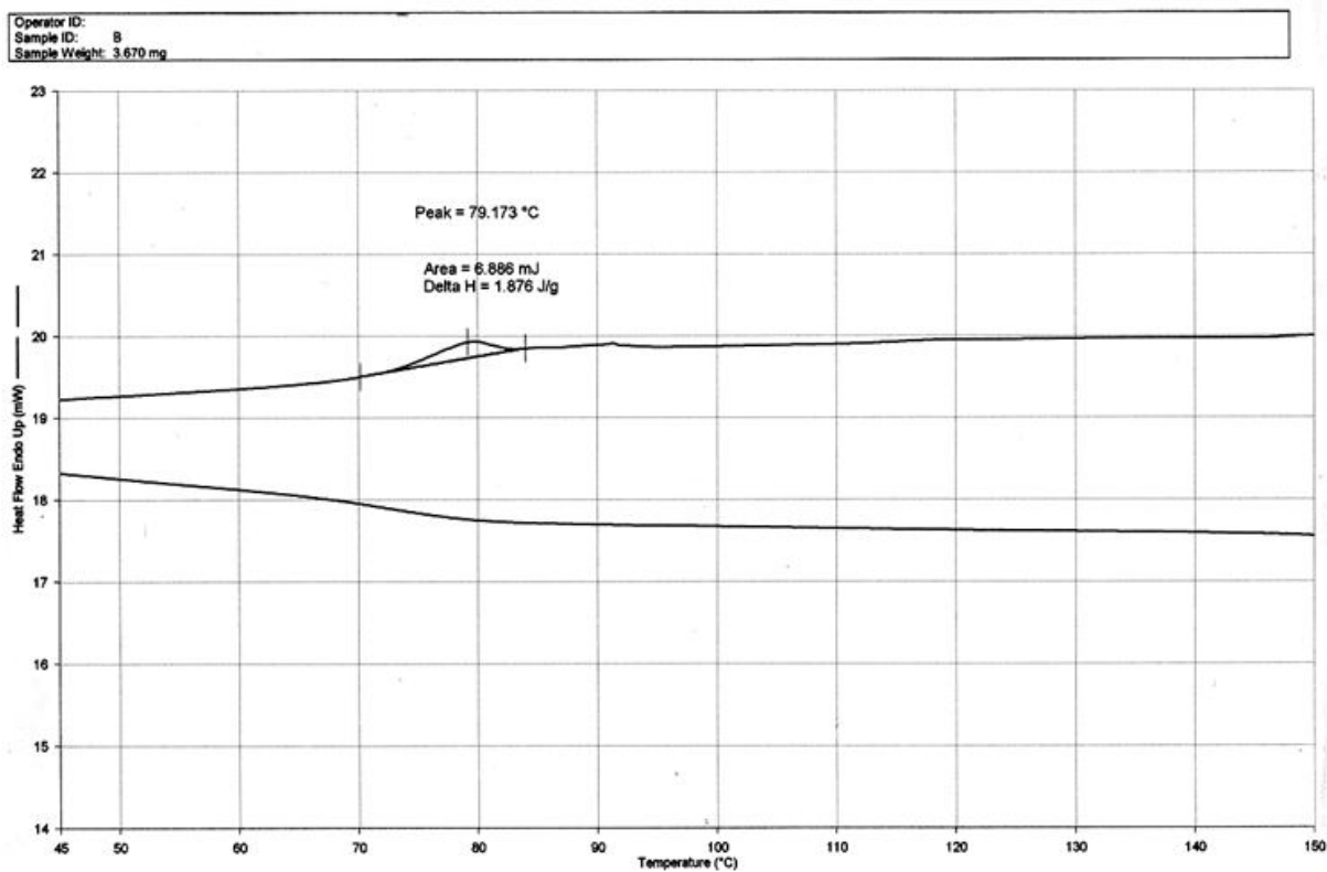
附圖 9 PFBFP3 之 DSC 圖
