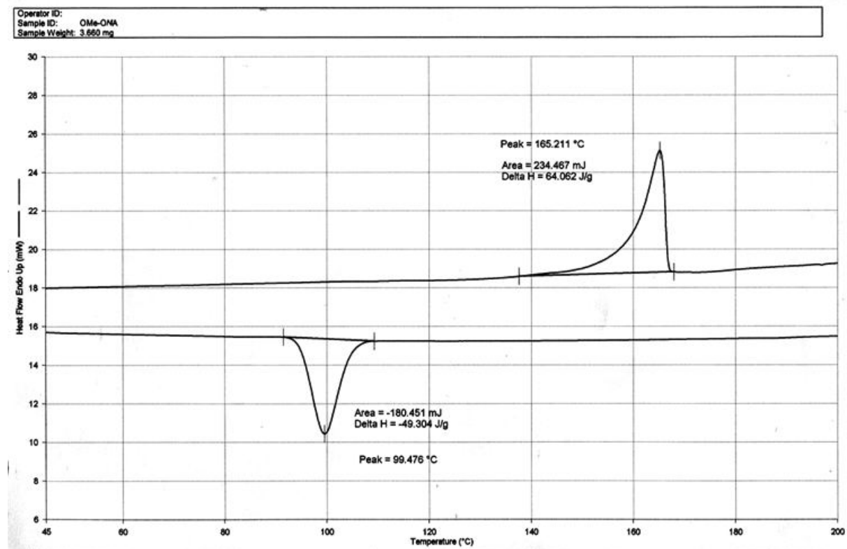
附圖 22 PFBFP30Me-ONA 之 DSC 圖
