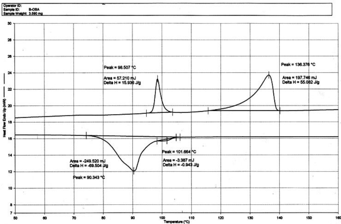
附圖 13 PFBFP3-OBA 之 DSC 圖
