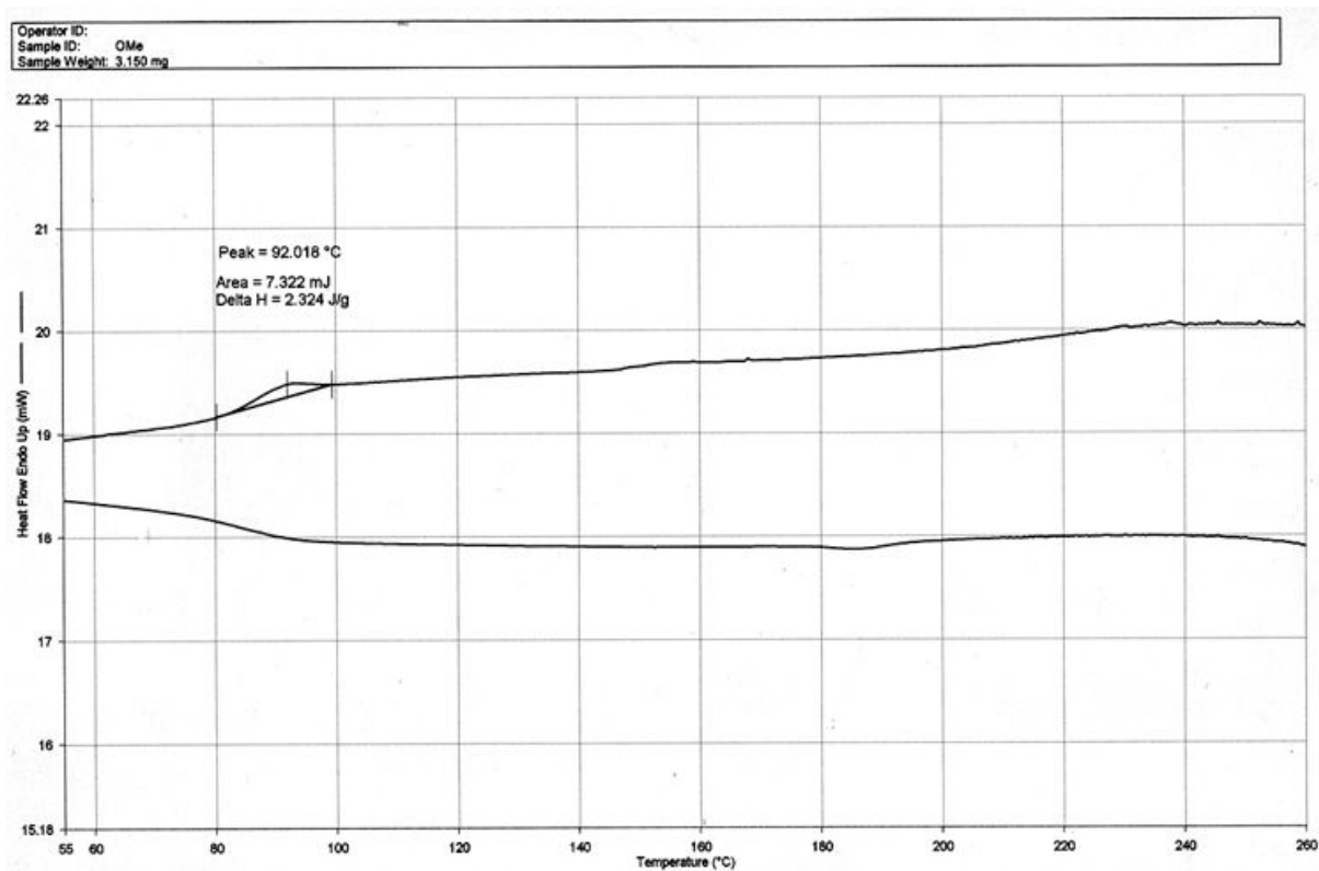
附圖 11 PFBFP3OMe 之 DSC 圖
