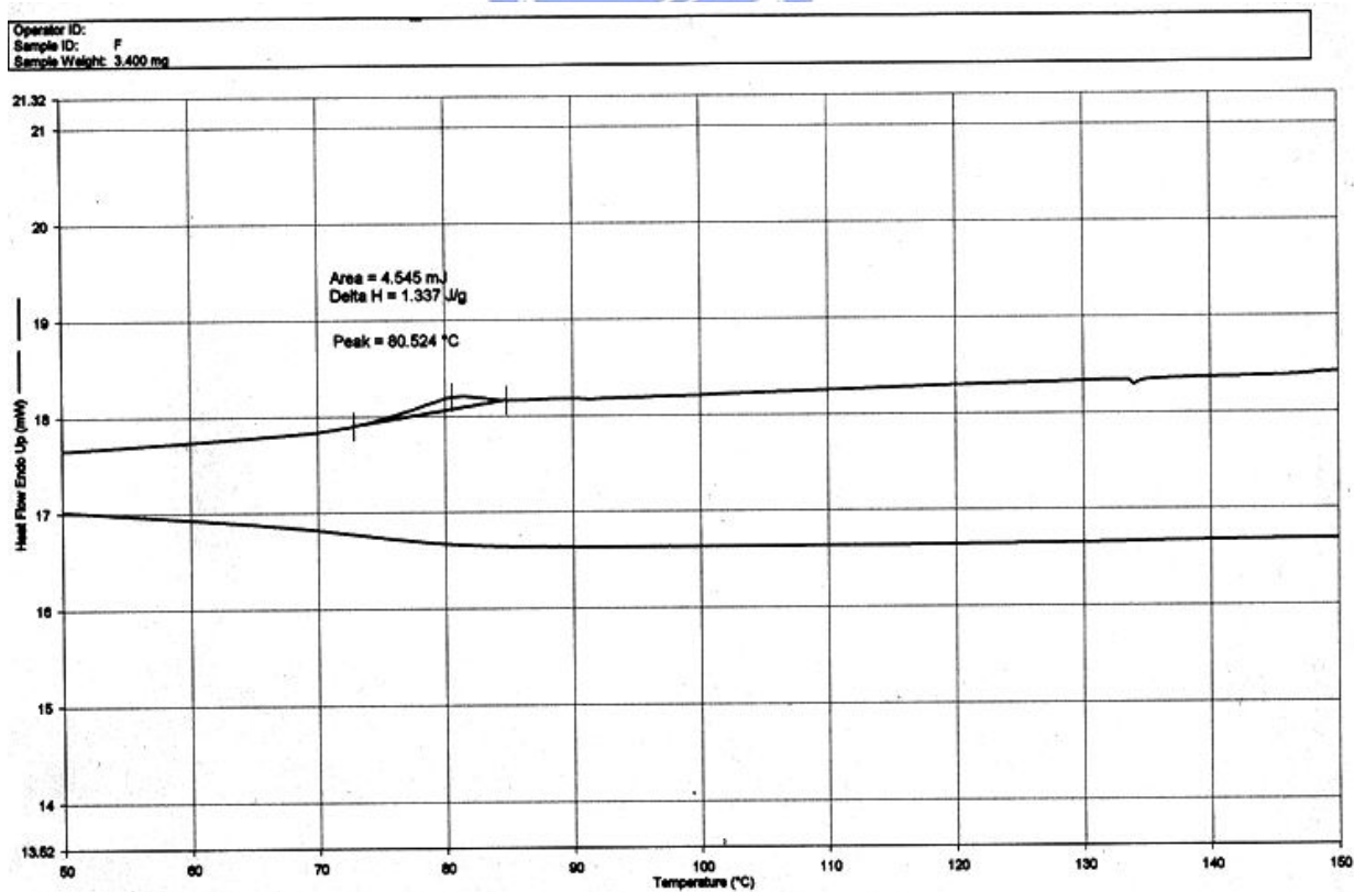
附圖 12 PFFFP3 之 DSC 圖
