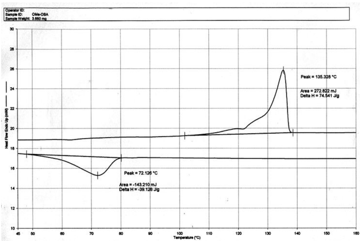
附圖 21 PFBFP30Me-OBA 之 DSC 圖
