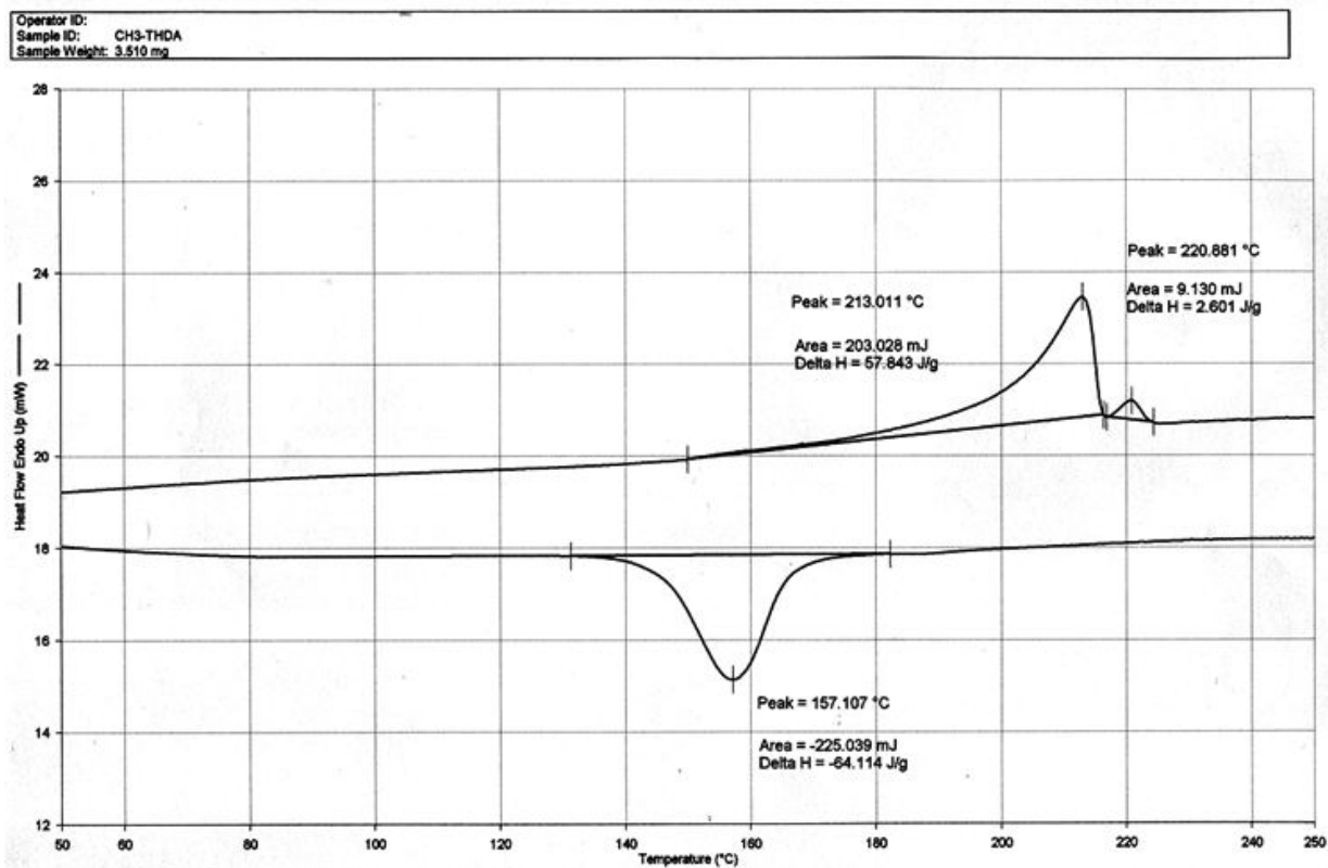
附圖 20 PFBFP3Me-THDA 之 DSC 圖
