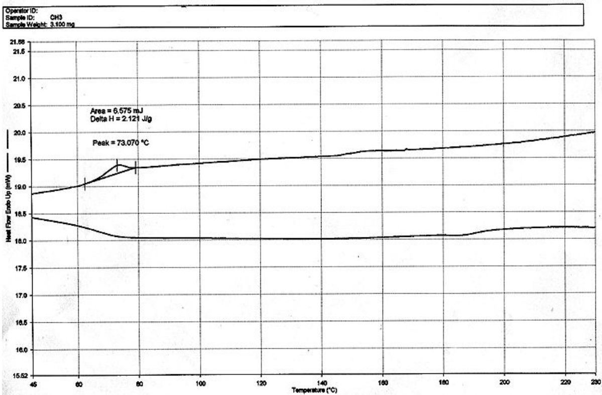
附圖 10 PFBFP3Me 之 DSC 圖
