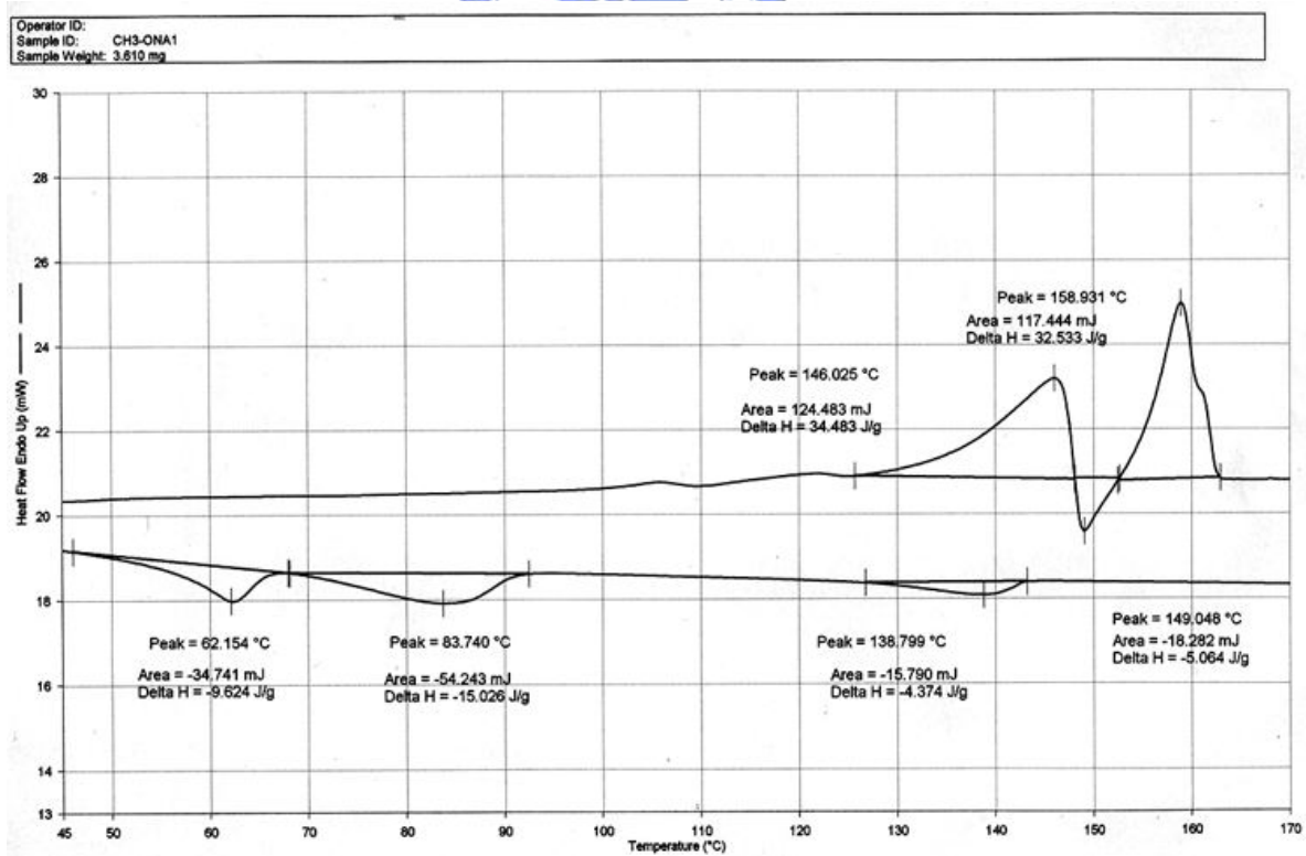
附圖 18 PFBFP3Me-ONA 之 DSC 圖
