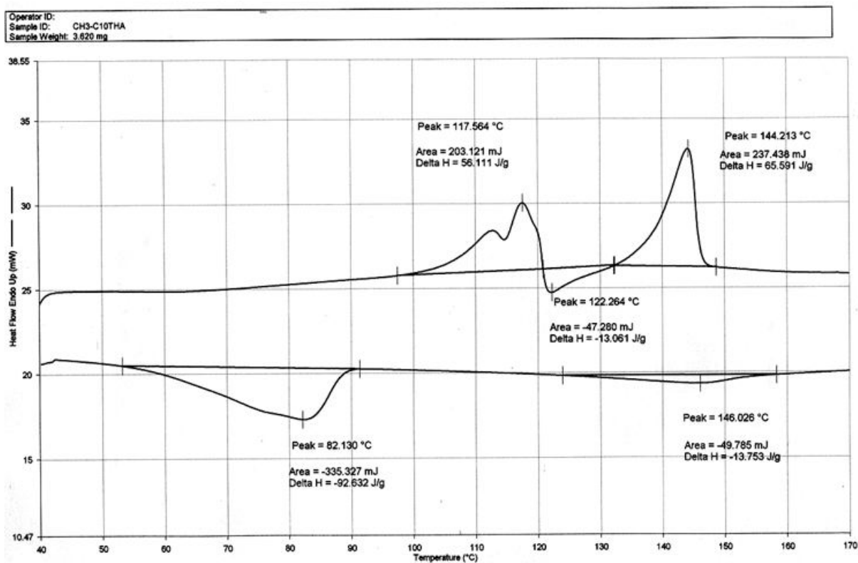
附圖 19 PFBFP3Me-THA 之 DSC 圖
