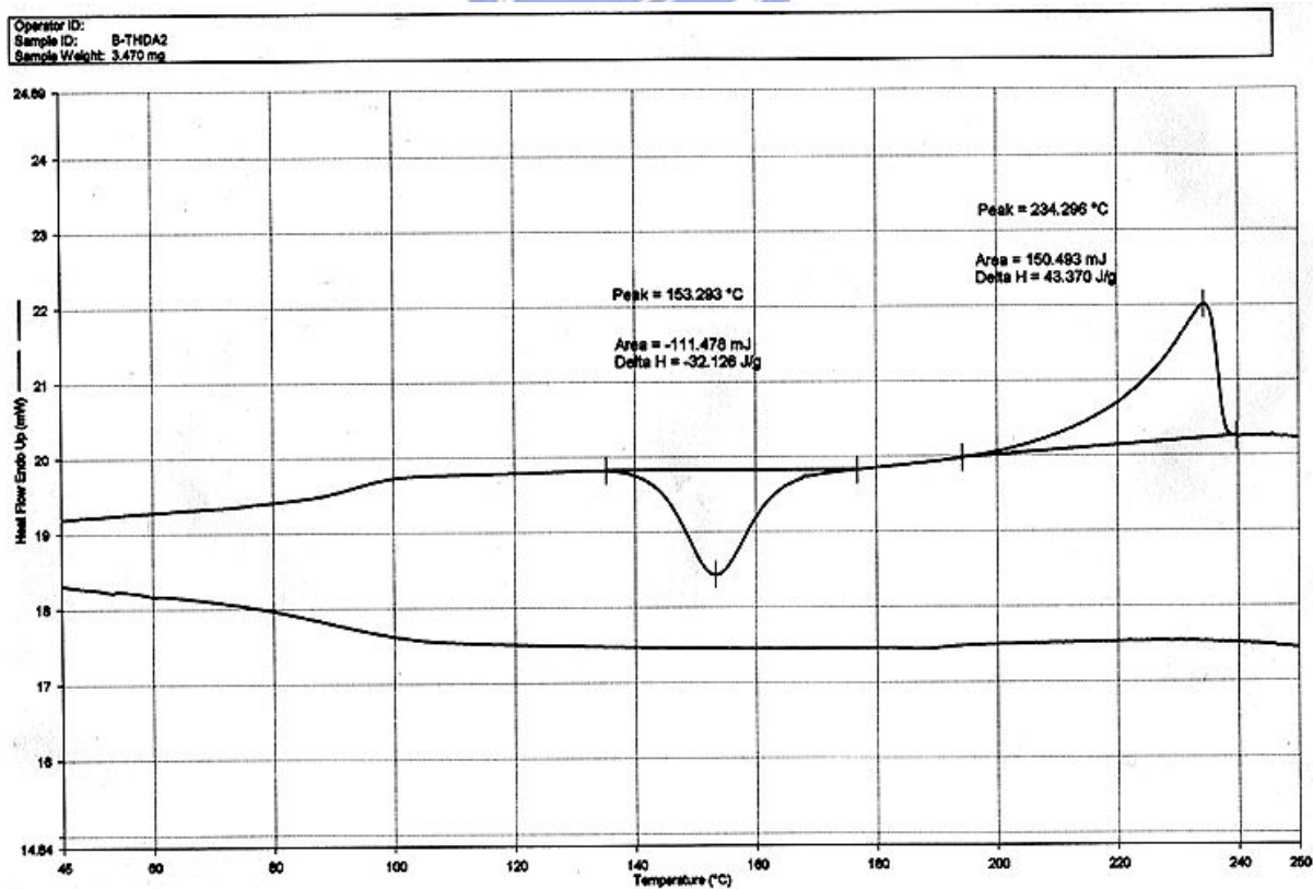
附圖 16 PFBFP3-THDA 之 DSC 圖
