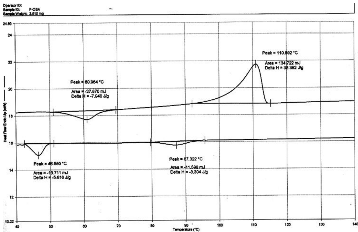
附圖 25 PFFFP3-OBA 之 DSC 圖
