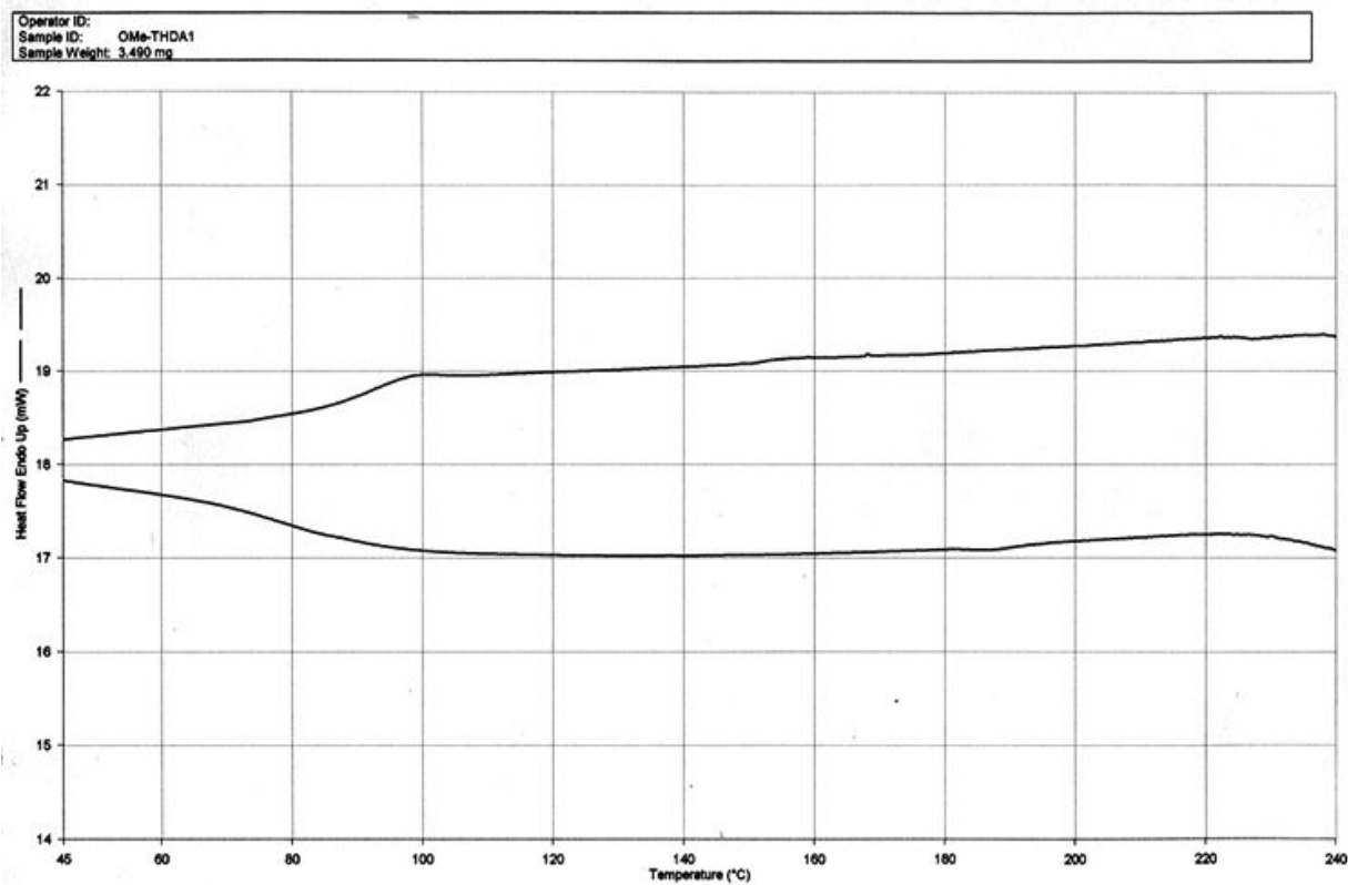
附圖 24 PFBFP30Me-THDA 之 DSC 圖
