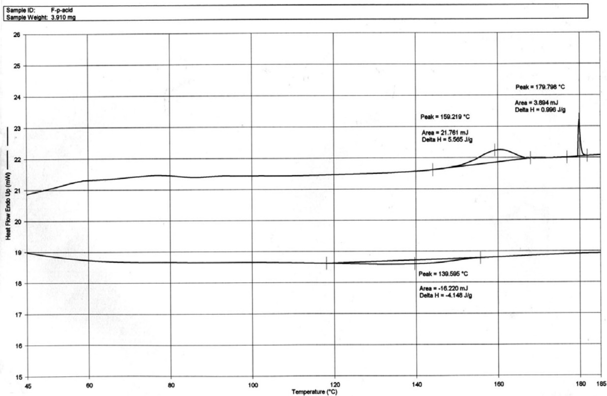
附圖 36 PFFFP3-PPA 第一次升溫及降溫之 DSC 圖
