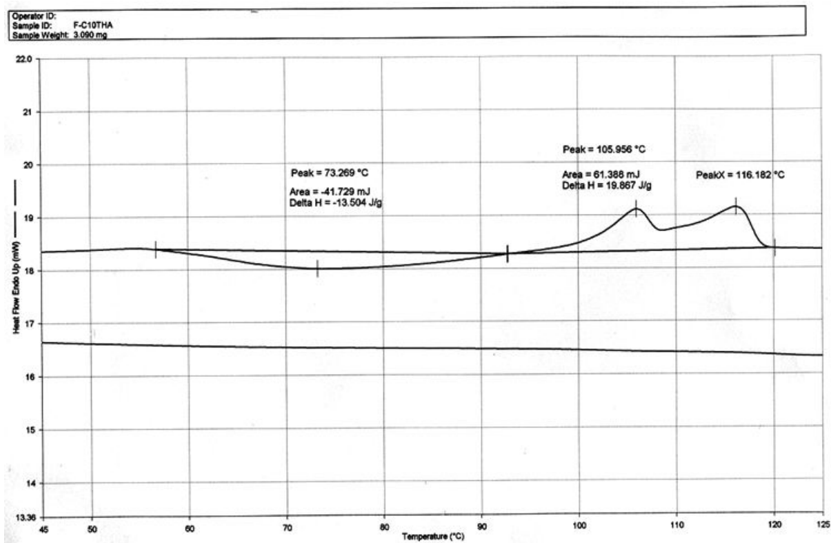
附圖 27 PFFFP3-THA 之 DSC 圖
