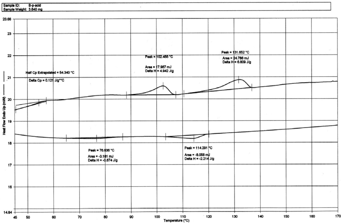
附圖 30 PFBFP3-PPA 第一次升溫及降溫之 DSC 圖
