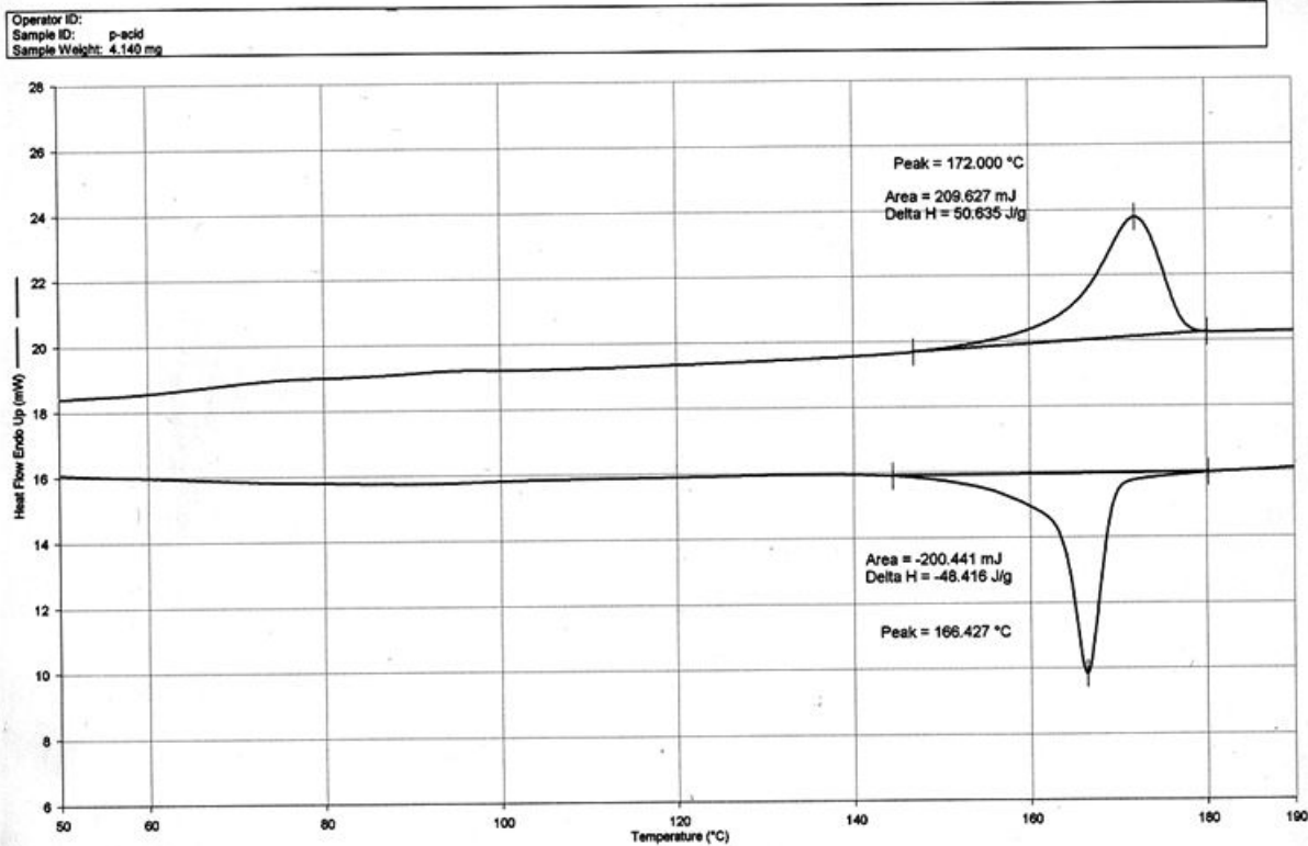
附圖 29 PPA 之 DSC 圖
