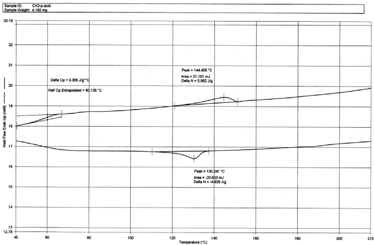
附圖 33 PFBFP3Me-PPA 第二次升溫及降溫之 DSC 圖
