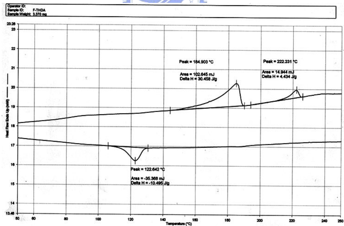
附圖 28 PFFFP3-THDA 之 DSC 圖
