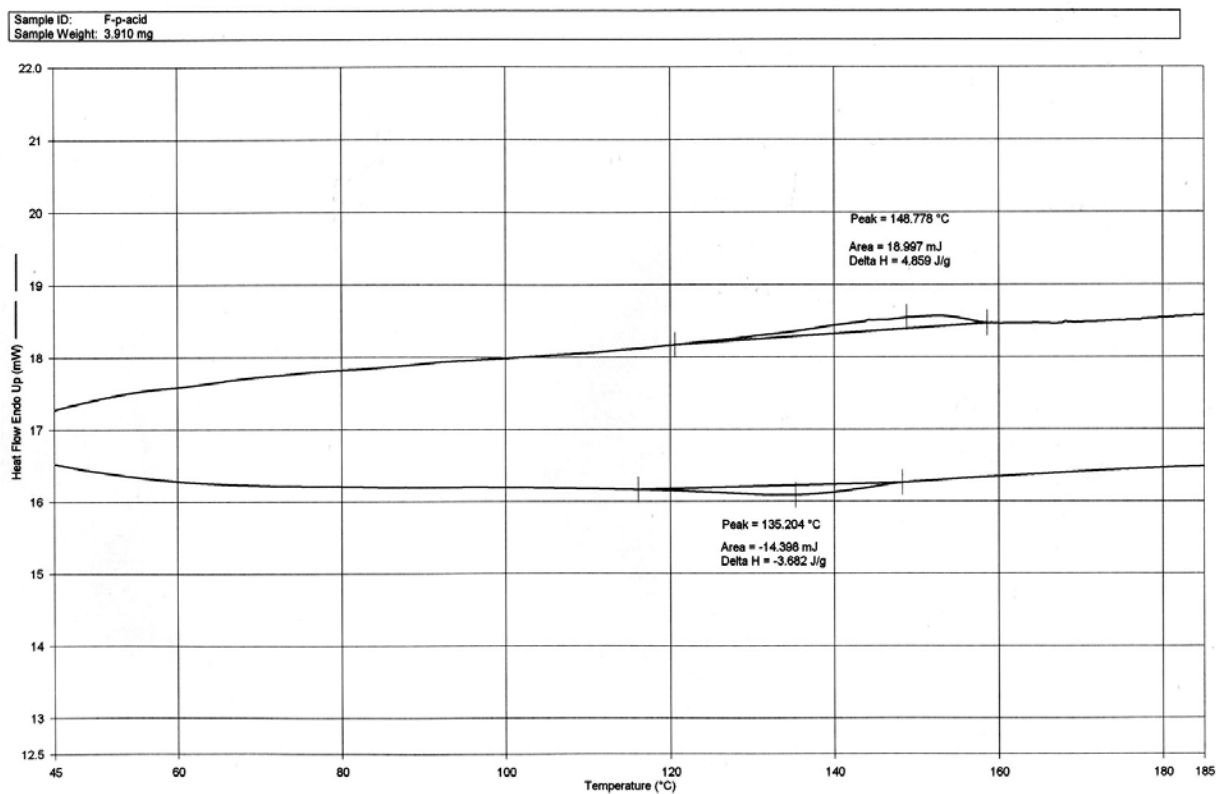
附圖 37 PFFFP3-PPA 第二次升溫及降溫之 DSC 圖
