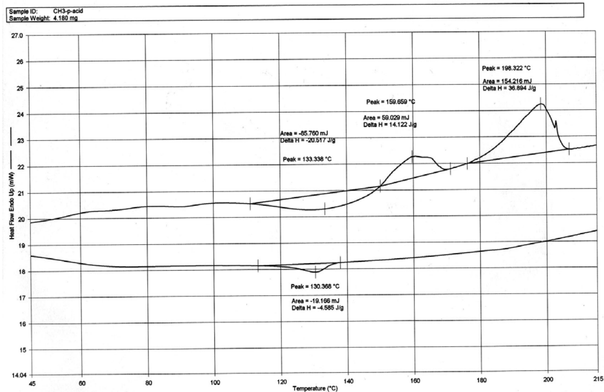
附圖 32 PFBFP3Me-PPA 第一次升溫及降溫之 DSC 圖
