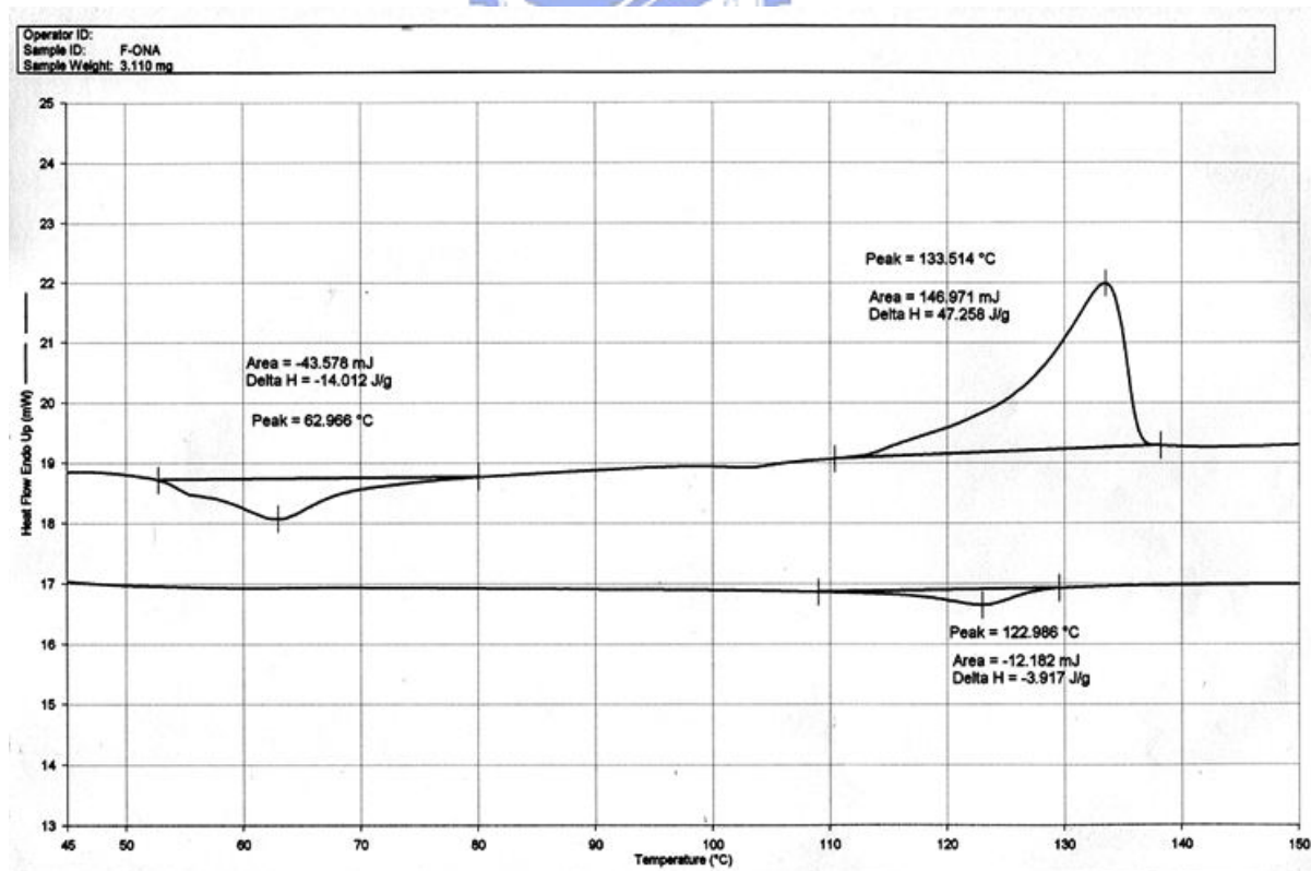
附圖 26 PFFFP3-ONA 之 DSC 圖
