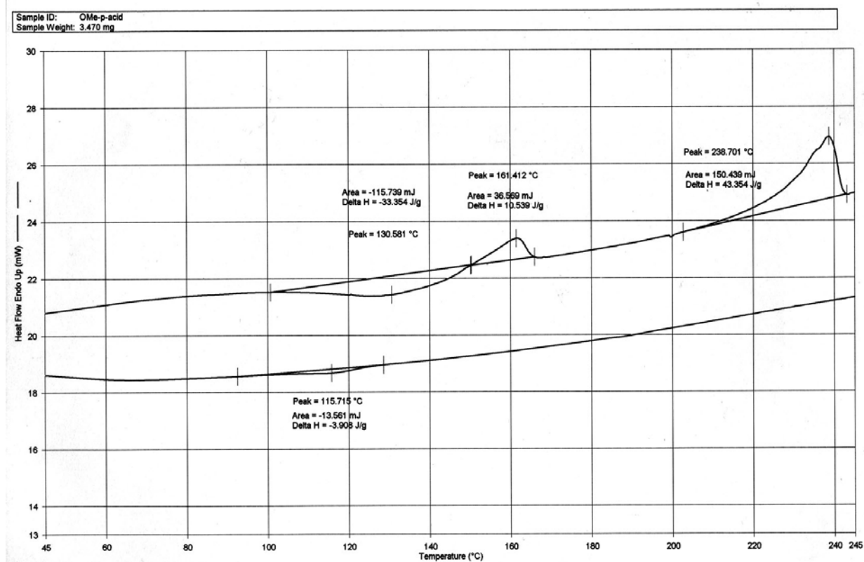
附圖 34 PFBFP3OMe-PPA 第一次升溫及降溫之 DSC 圖
