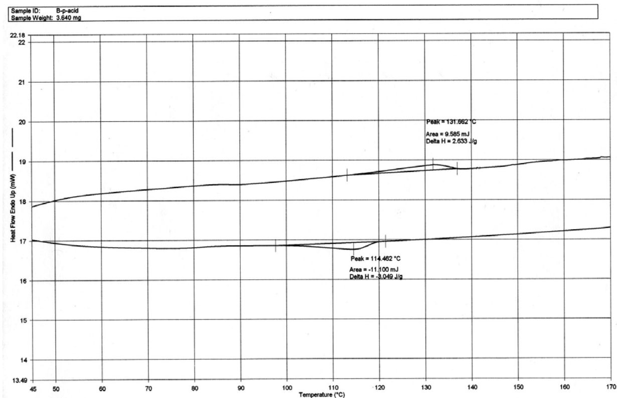
附圖 31 PFBFP3-PPA 第二次升溫及降溫之 DSC 圖
