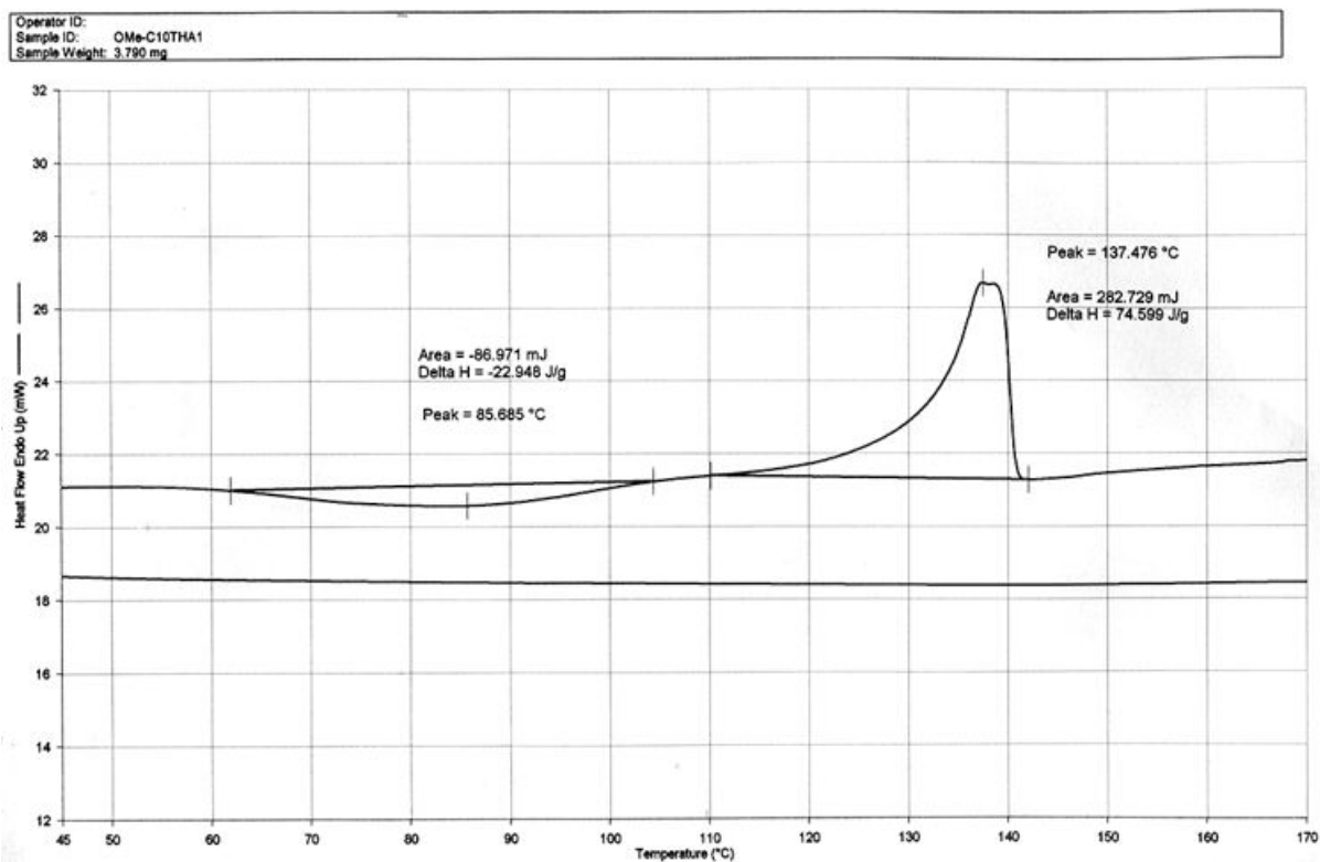
附圖 23 PFBFP30Me-THA 之 DSC 圖
