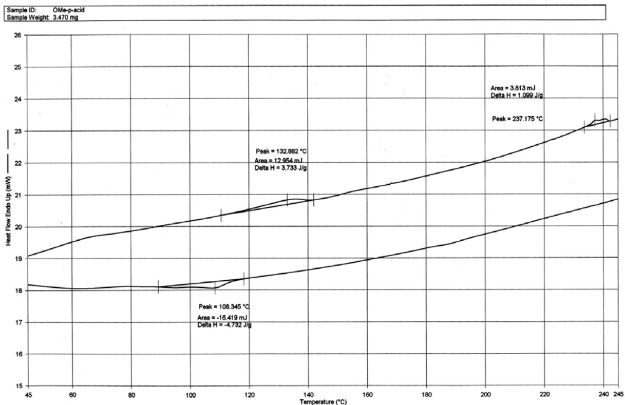
附圖 35 PFBFP3OMe-PPA 第二次升溫及降溫之 DSC 圖
