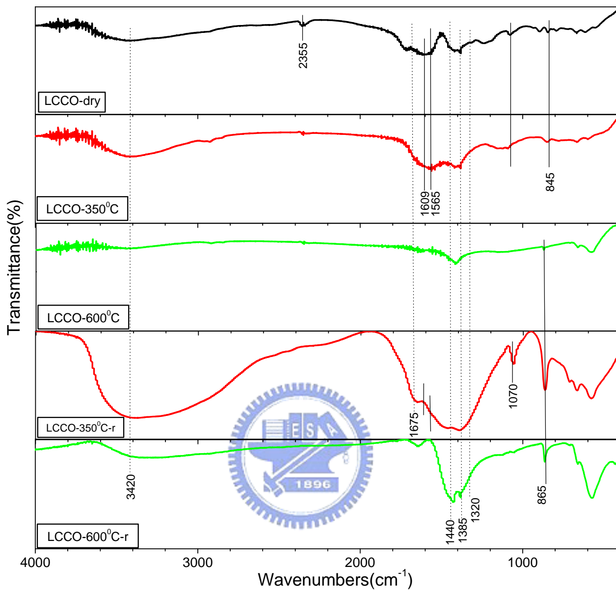
(附)圖 1-7 LCCO化合物經 \text{H}_2\text{O}_2 分解反應前後之IR光譜圖
