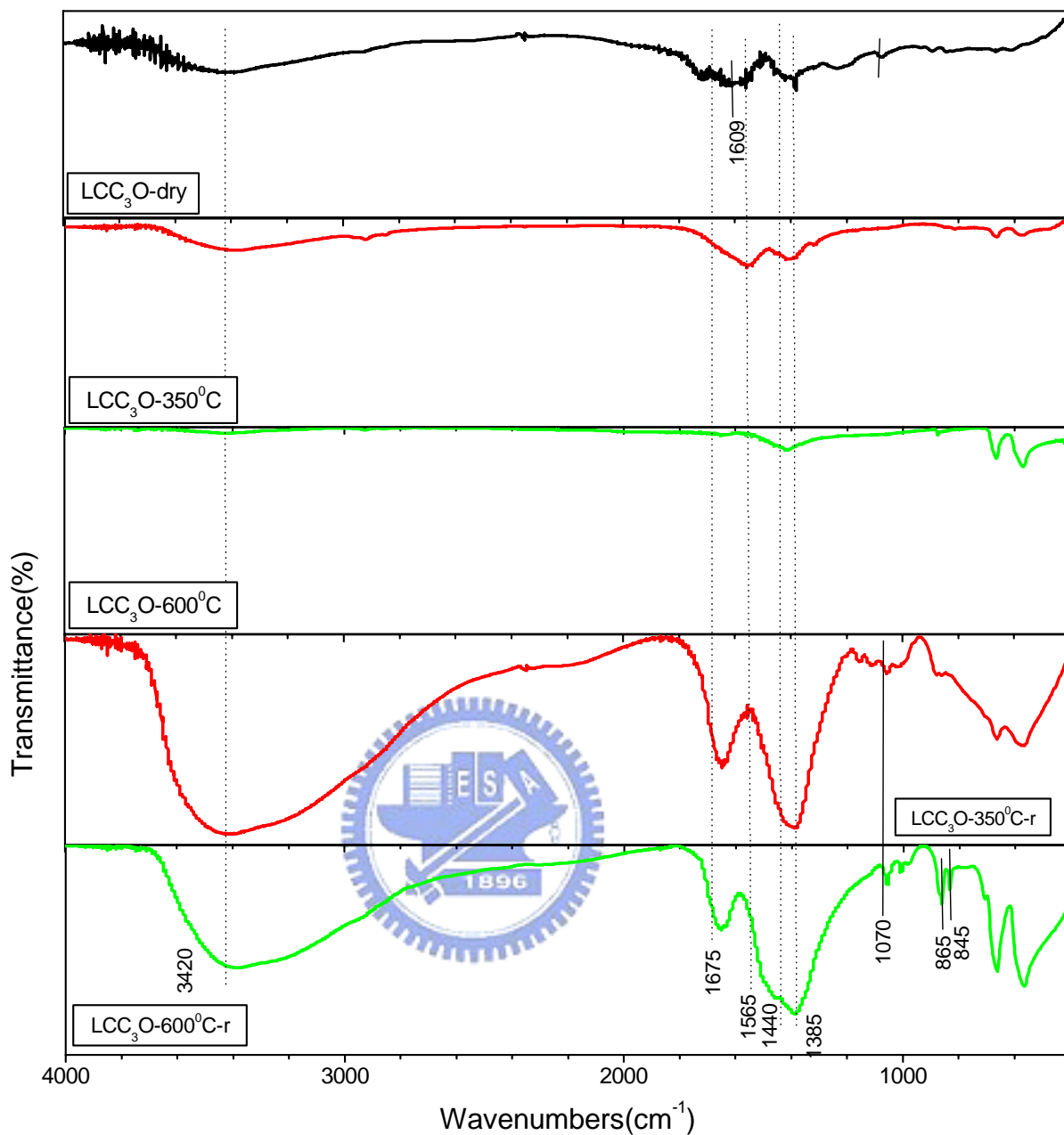
(附)圖 1-9 LCC 3 O化合物經H 2 O 2 分解反應前後之IR光譜圖
