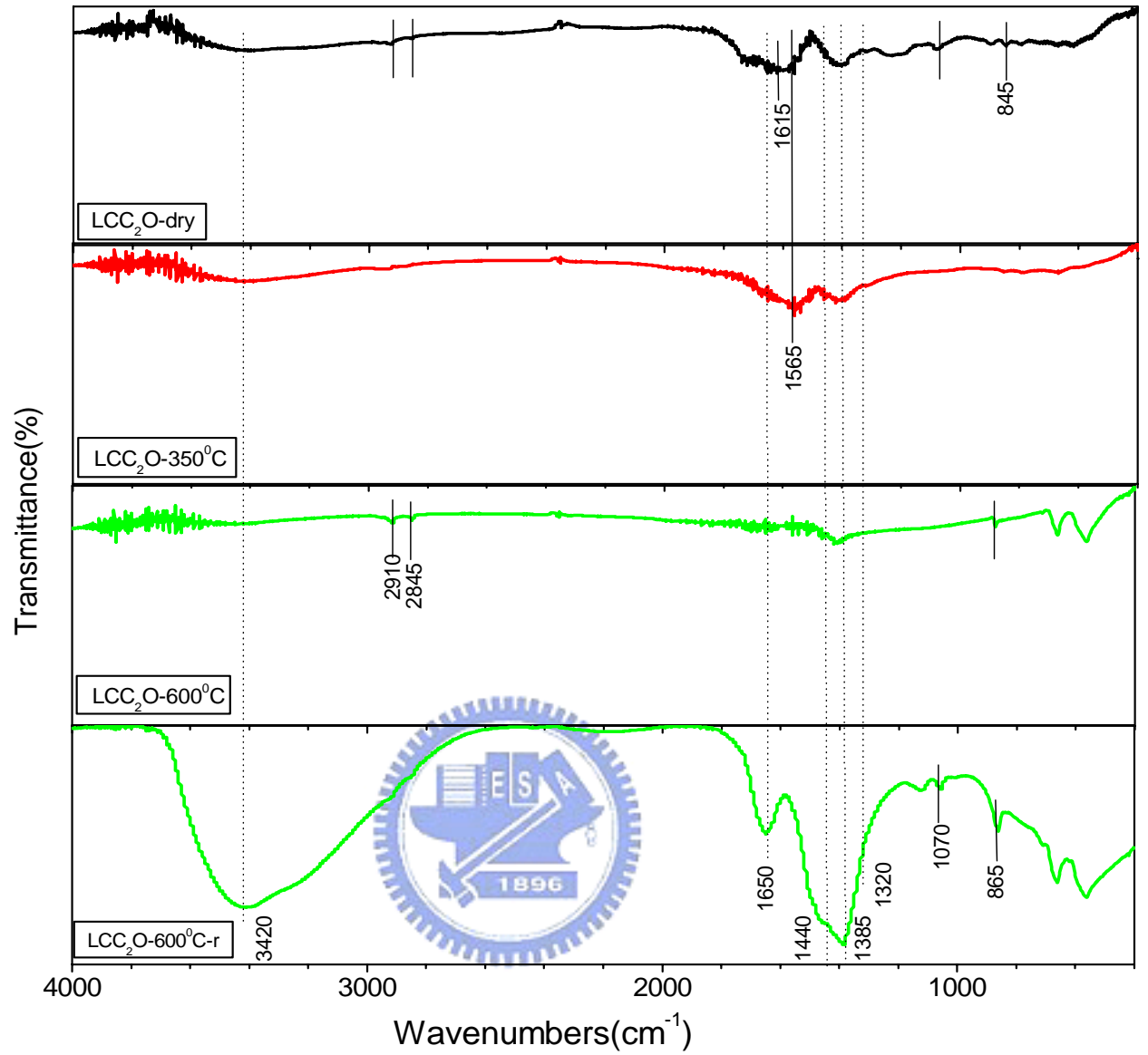
(附)圖 1-8 LCC 2 O化合物經H 2 O 2 分解反應前後之IR光譜圖
