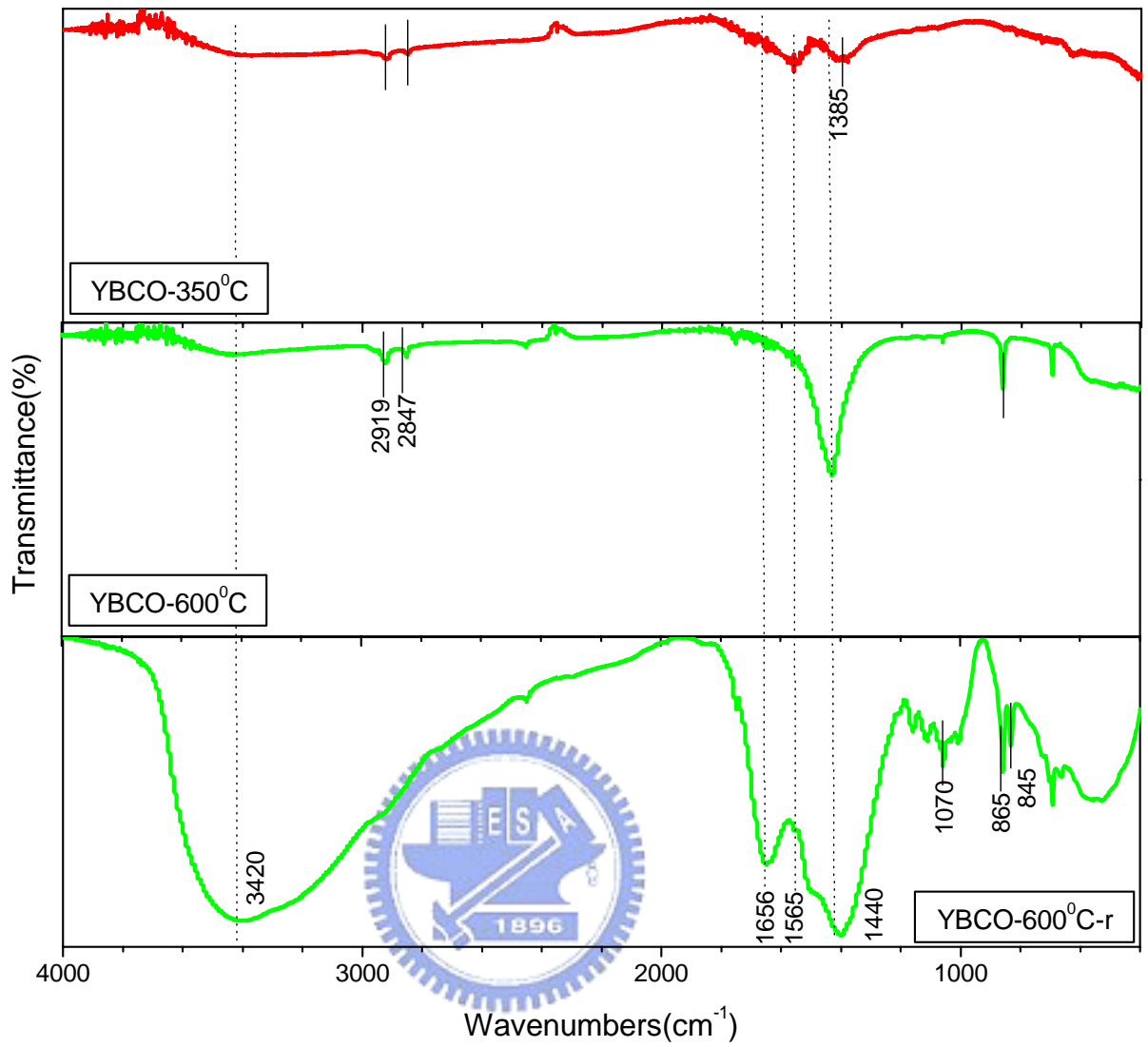
(附)圖 1-10 YBCO化合物經 \text{H}_2\text{O}_2 分解反應前後之IR光譜圖
