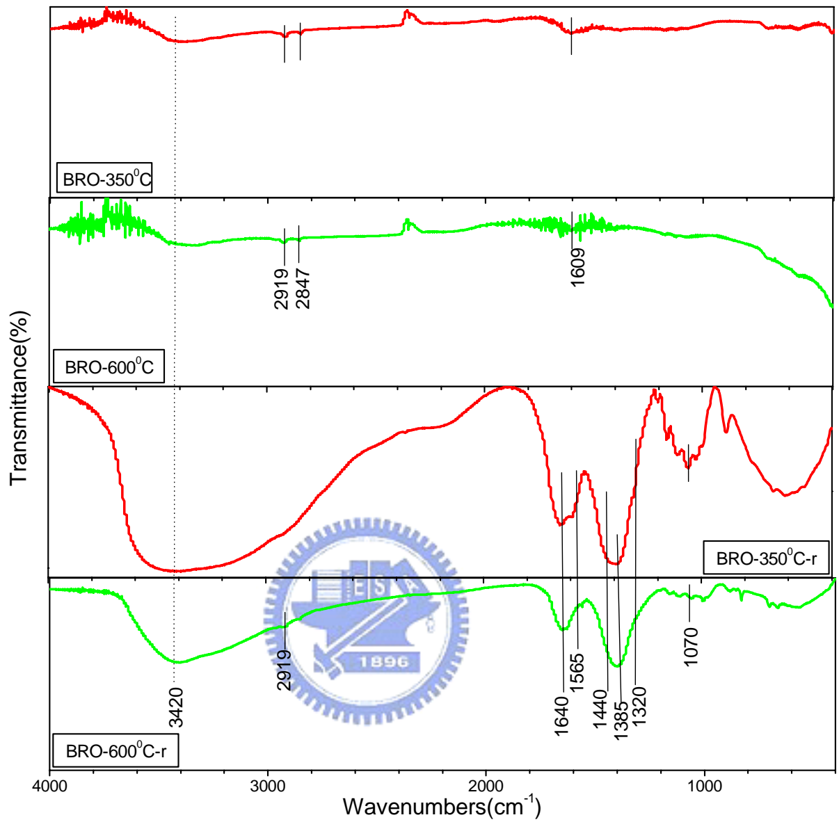
(附)圖 1-11 BRO化合物經H 2 O 2 分解反應前後之IR光譜圖
