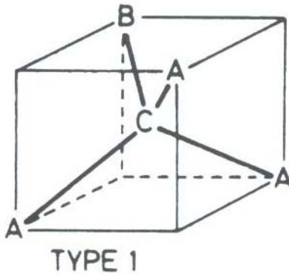
Fig. 3.1a The CuPt-type structure; A · B : group III element; C : group V element.
