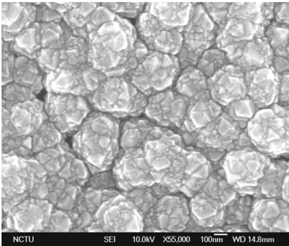
圖 4-37 試片 D-1 低密度鑽石形貌
