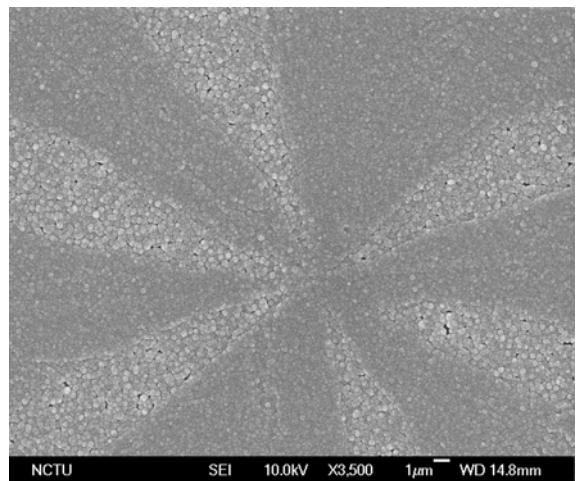
圖 4-36 試片 D-1 鑽石花瓣圖形
