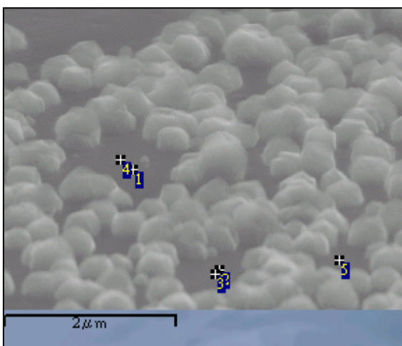
圖 4-17 試片 B-2 高密度分析點
