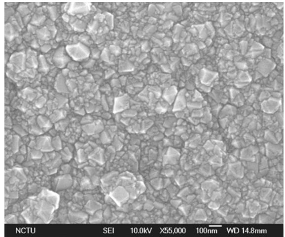
圖 4-38 試片 D-1 高密度鑽石形貌
