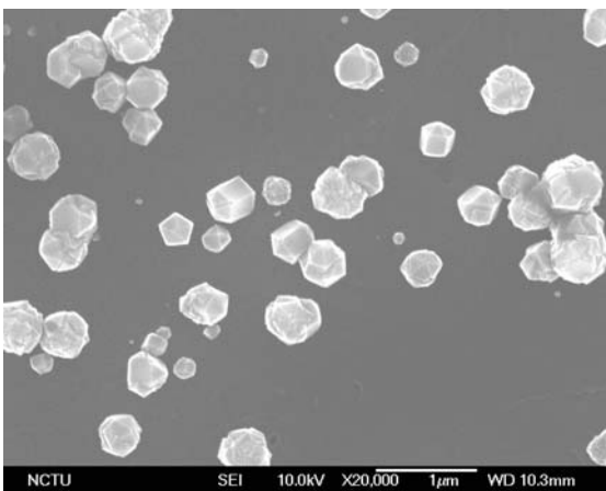
圖 4-5 試片 B 高密度鑽石形貌
