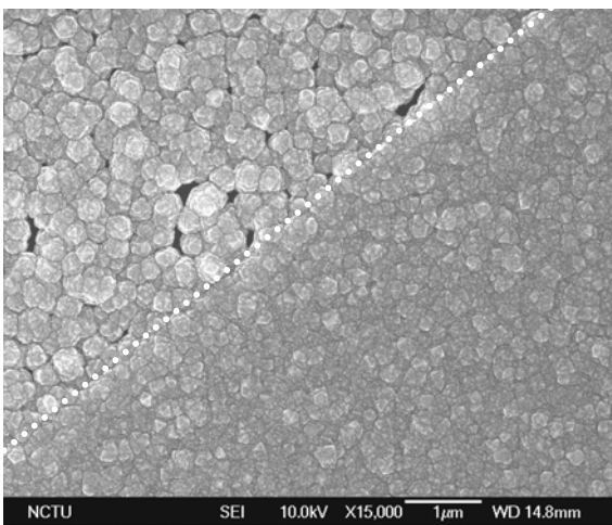
圖 4-39 晶界兩邊鑽石形貌差異
