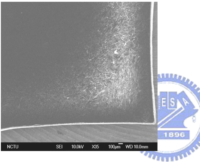
圖 4-3 試片 B 的邊緣圖
