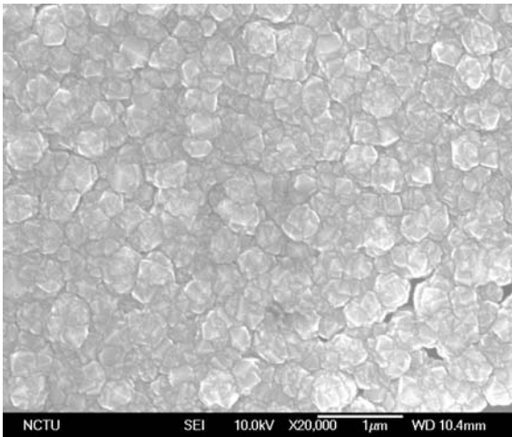
圖 4-25 試片 C 高密度鑽石形貌
