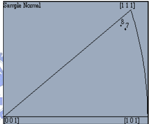
圖 4-34 六邊形區域砂方位分佈
