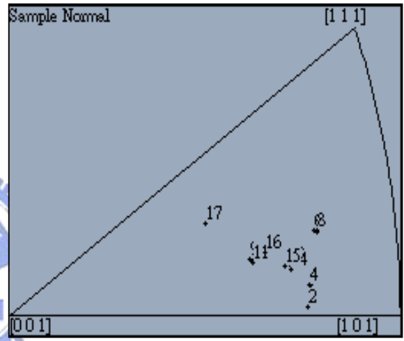
圖 4-10 試片 B-2 矽方位分佈圖
