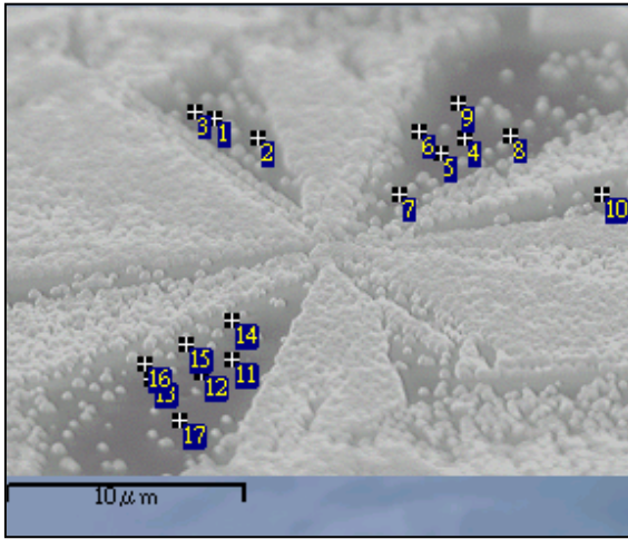
圖 4-31 試片 C-4 低密度分析點
