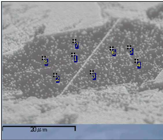
圖 4-33 六邊形低密度區域分析點
