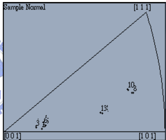
圖 4-22 試片 B-4 左下的方位分佈
