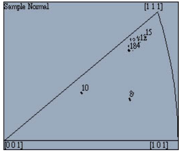
圖 4-8 試片 B-1 矽方位分佈圖
