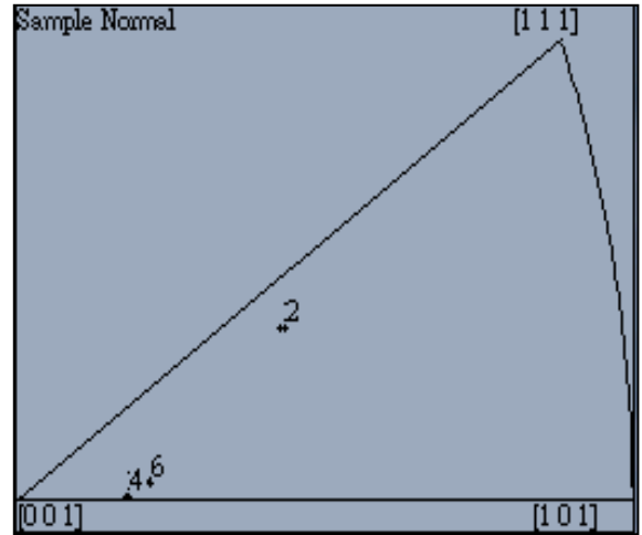
圖 4-14 試片 B-1 右上的方位分佈
