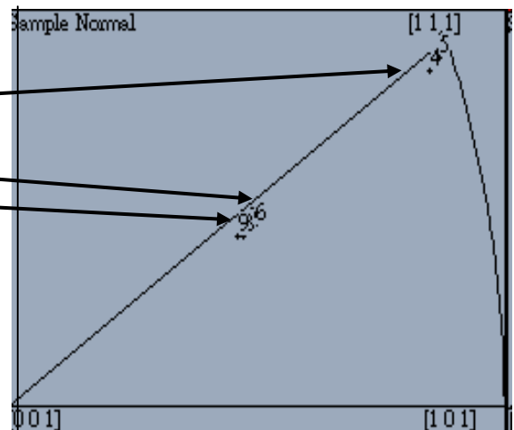
圖 4-42 鑽石成核趨勢與矽方位關係
