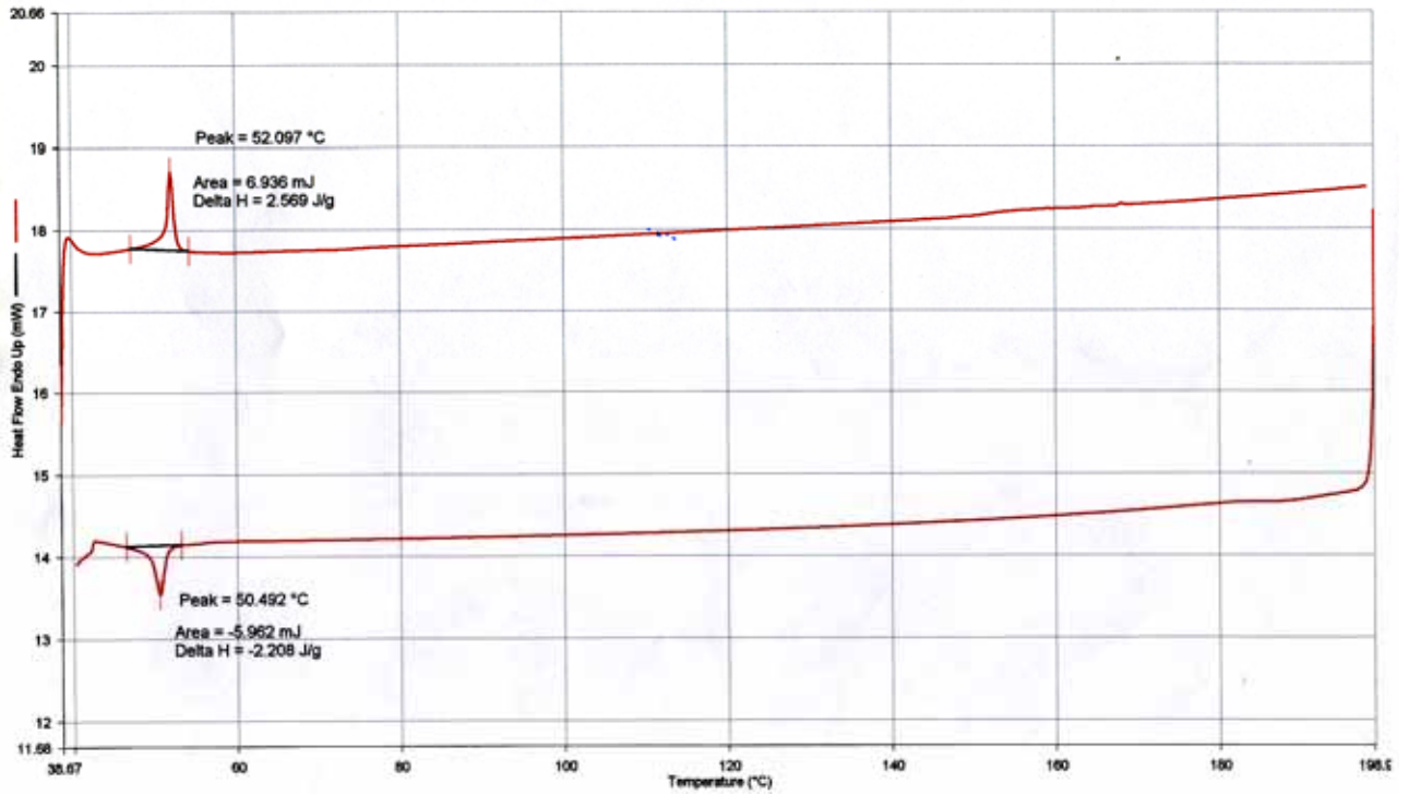
附圖 14. PDMB3OC10MA third heating-cooling 之 DSC 圖
