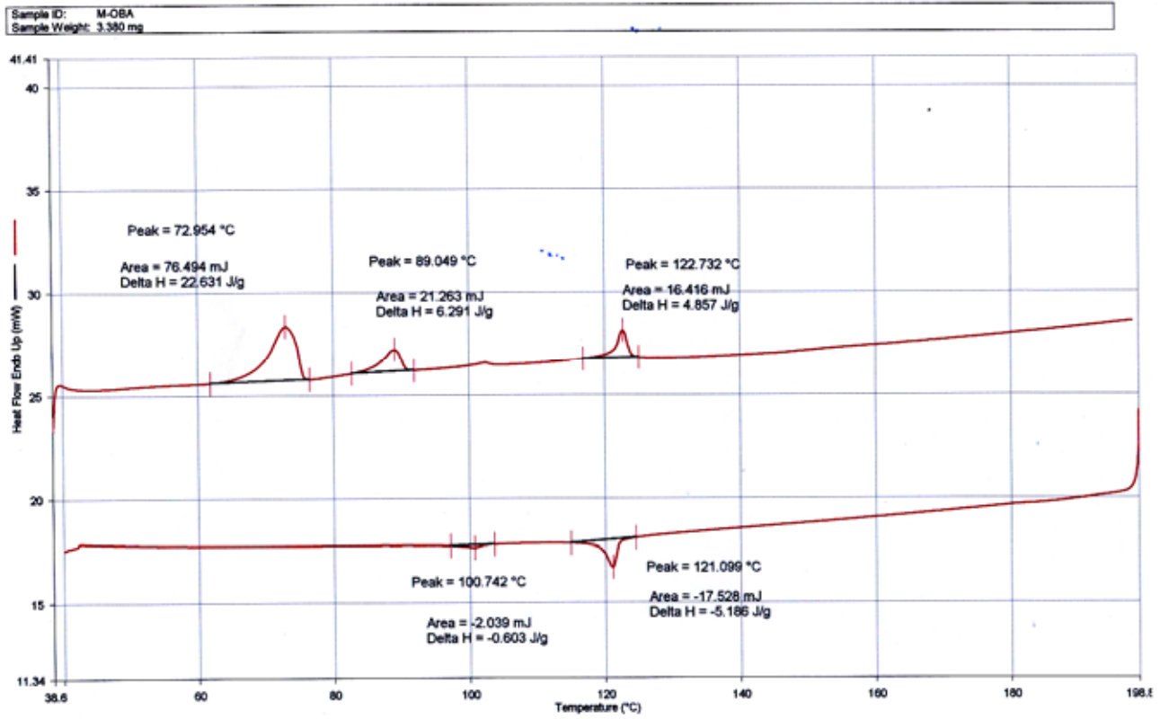
附圖 20. PDMB3OC10MA-OBA third heating-cooling 之 DSC 圖
