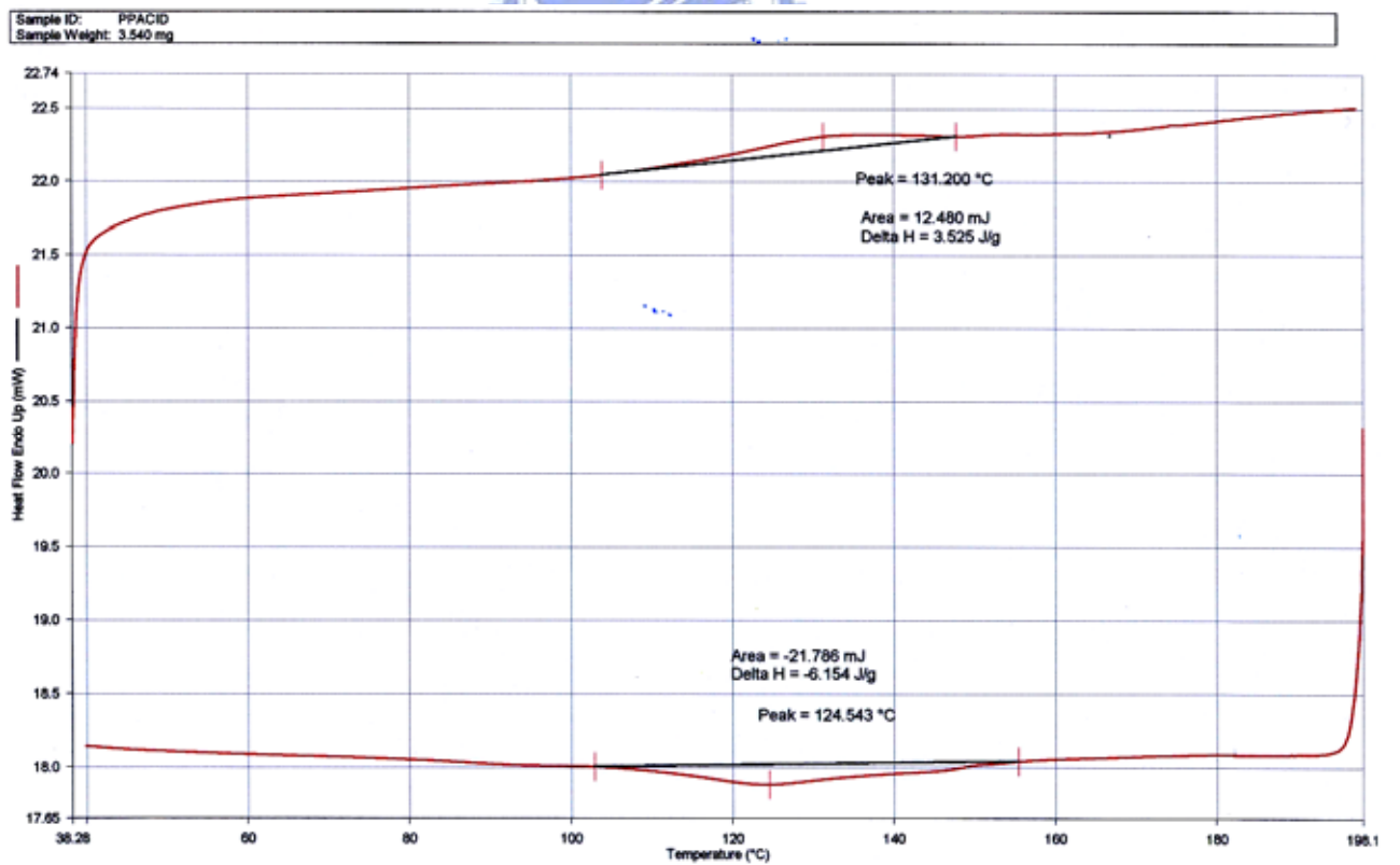
附圖 31. PDMB3OC10MA-p-PC 10 BA second heating-cooling 之 DSC 圖
