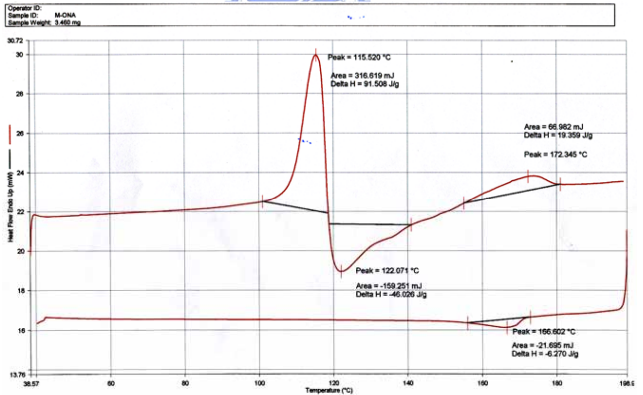
附圖 21. PDMB3OC10MA-ONA first heating-cooling 之 DSC 圖
