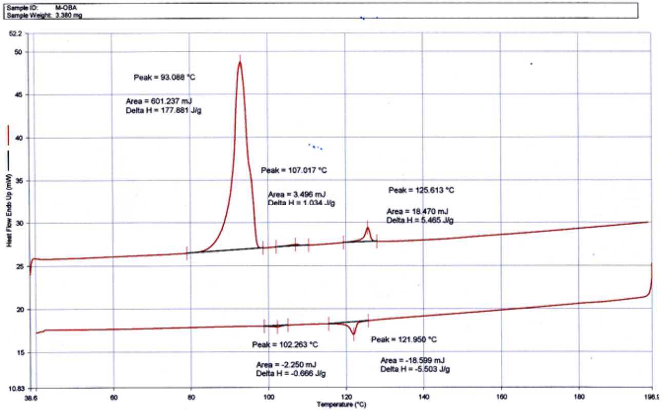
附圖 18. PDMB3OC10MA-OBA first heating-cooling 之 DSC 圖
