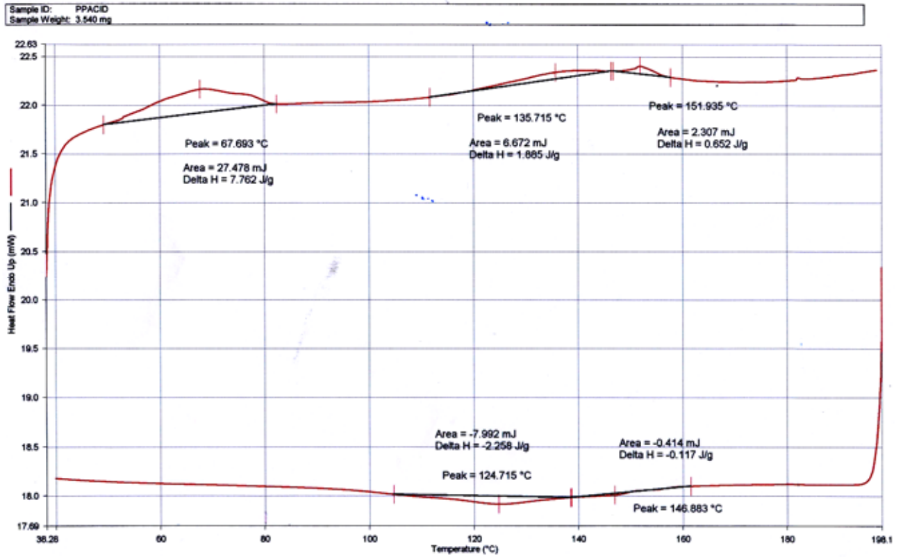
附圖 30. PDMB3OC10MA-p-PC 10 BA first heating-cooling 之 DSC 圖
