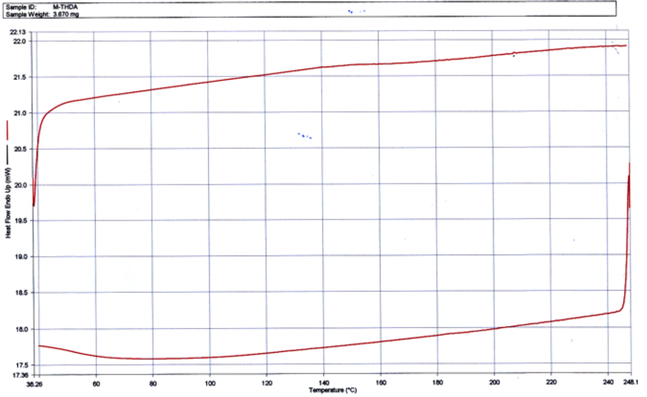
附圖 16. PDMB3OC10MA-THDA second heating-cooling 之 DSC 圖
