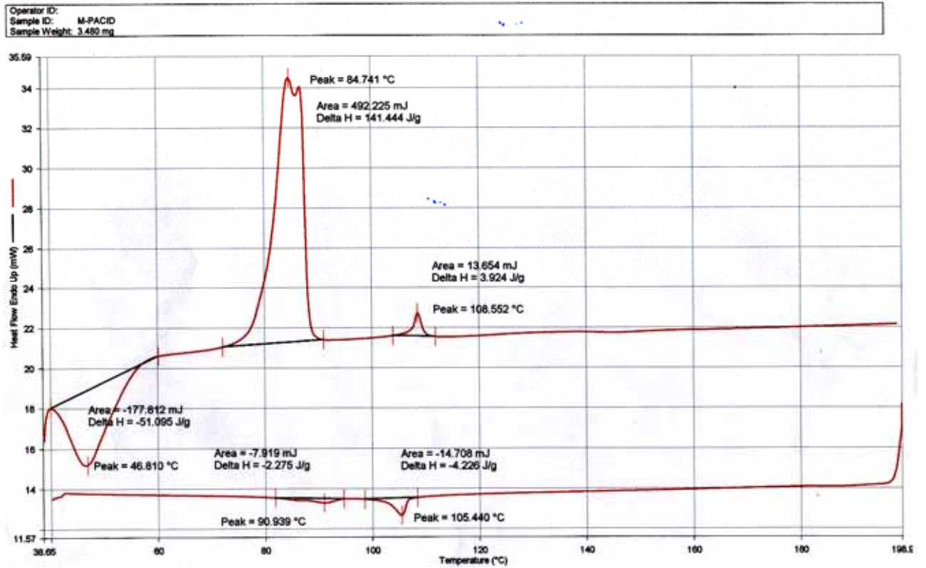
附圖 25. PDMB3OC10MA-p-MC 10 BA second heating-cooling 之 DSC 圖
