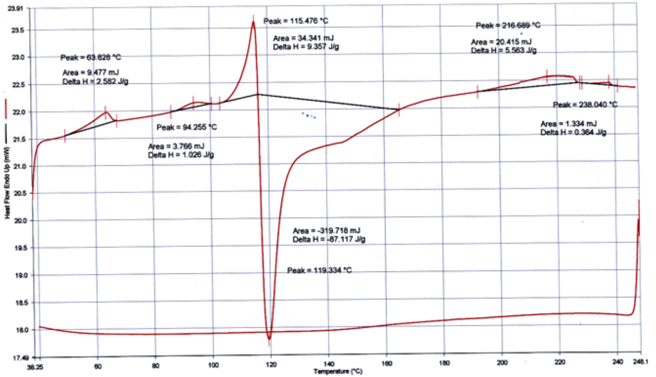
附圖 15. PDMB3OC10MA-THDA first heating-cooling 之 DSC 圖
