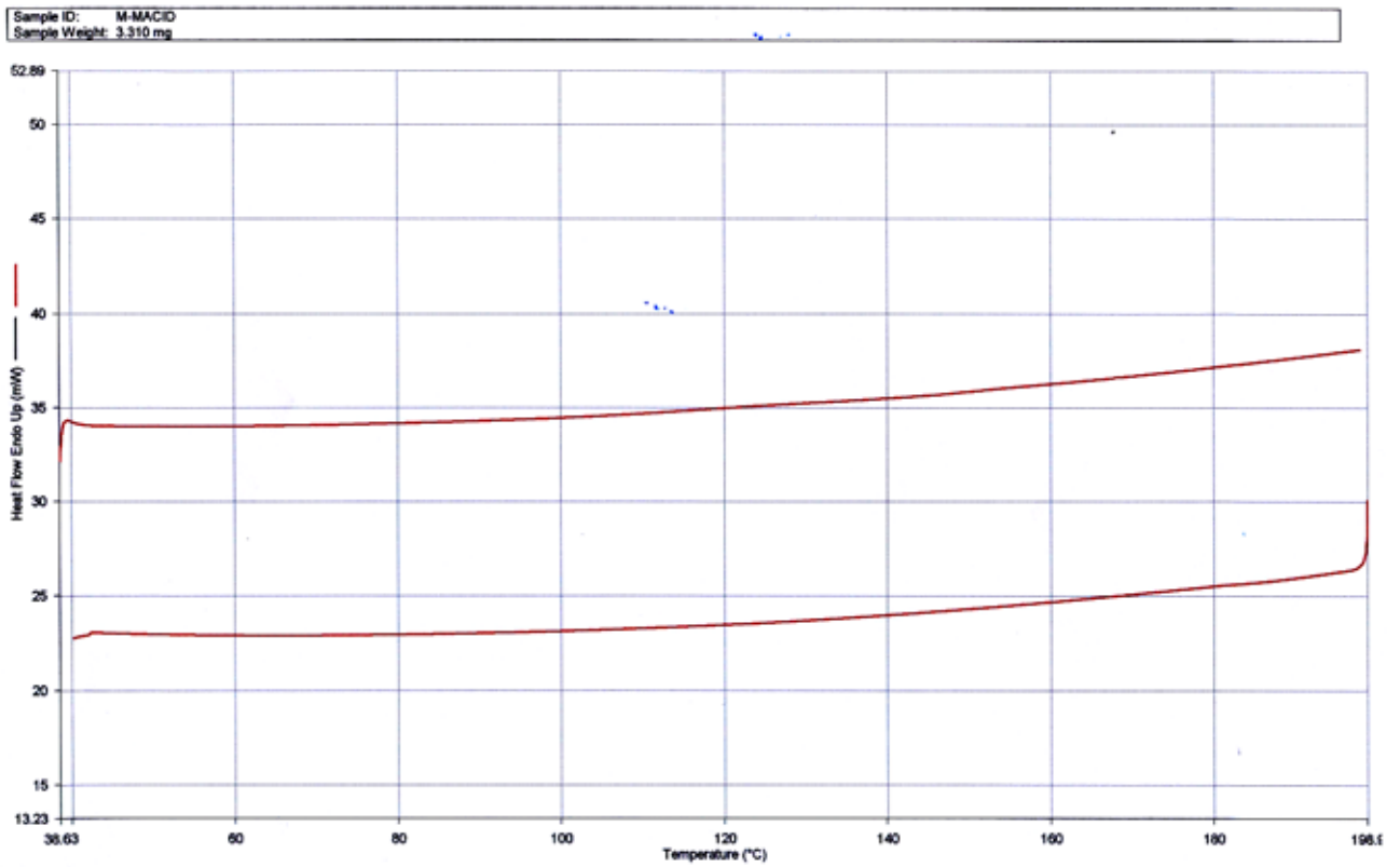
附圖 28. PDMB3OC10MA-m-MC 10 BA second heating-cooling 之 DSC 圖
