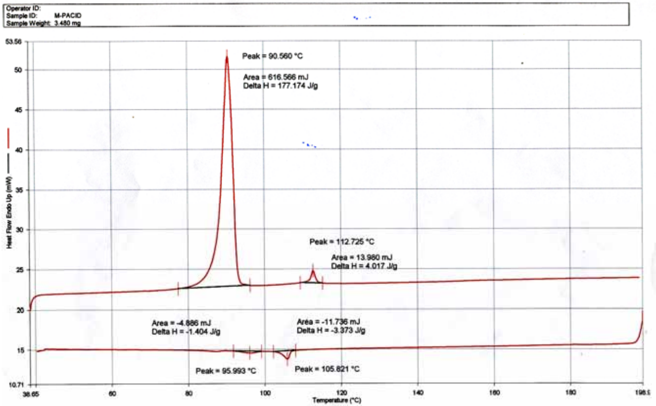
附圖 24. PDMB3OC10MA-p-MC 10 BA first heating-cooling 之 DSC 圖
