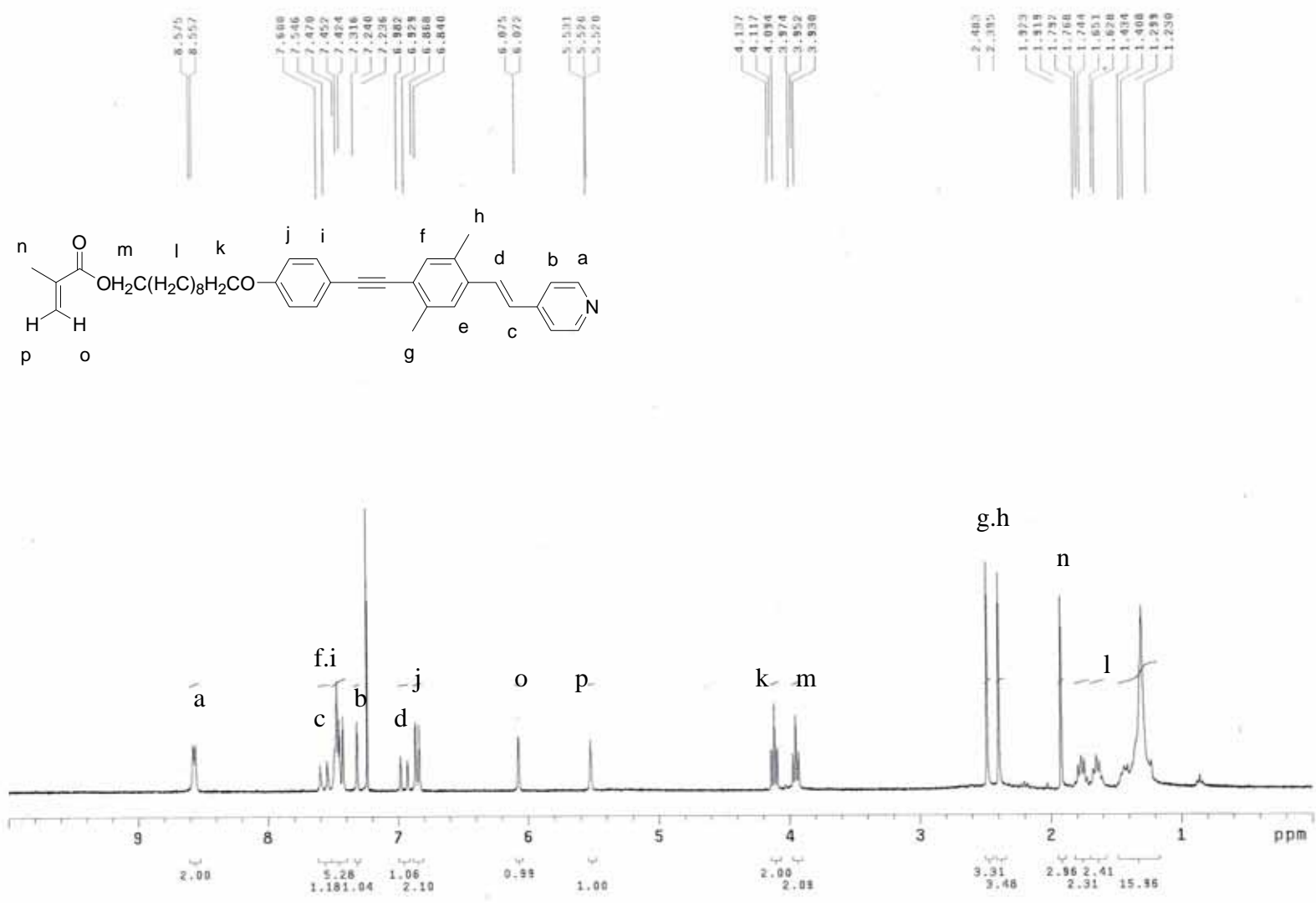
附圖 4. PDMB3OC10MA 之 1 H-NMR 圖
