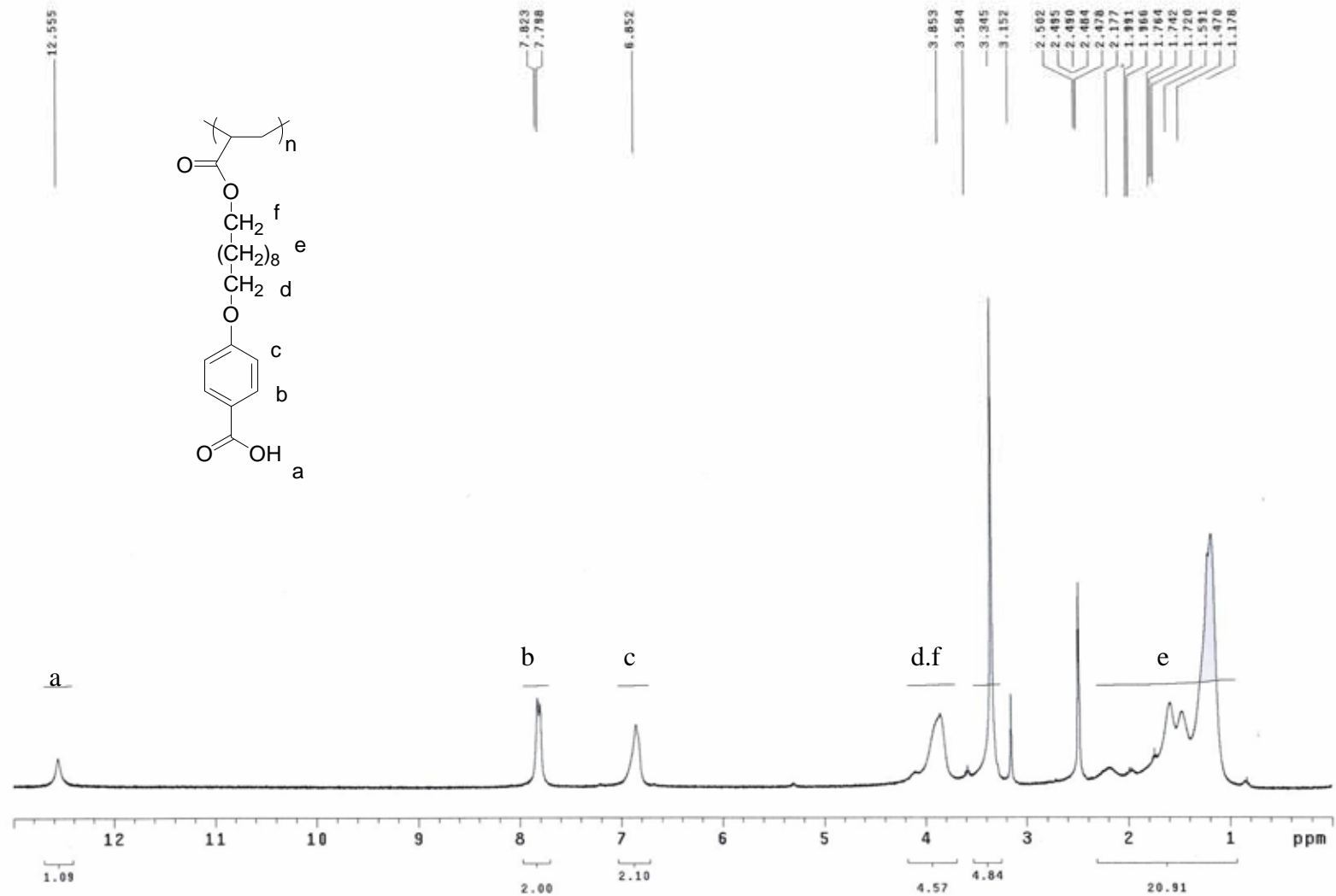
附圖 8. p-PC 10 BA 之 ^1\text{H-NMR} 圖
