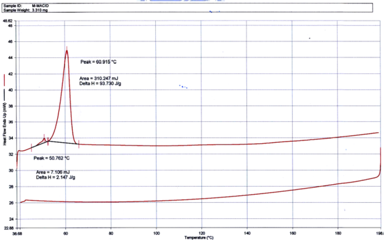
附圖 27. PDMB3OC10MA-m-MC 10 BA first heating-cooling 之 DSC 圖
