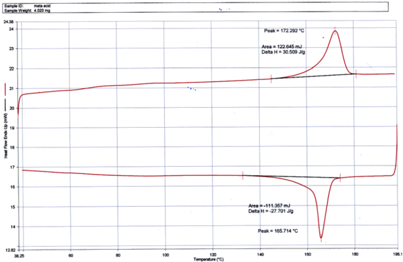
附圖 10. p-PC 10 BA 之 DSC 圖
