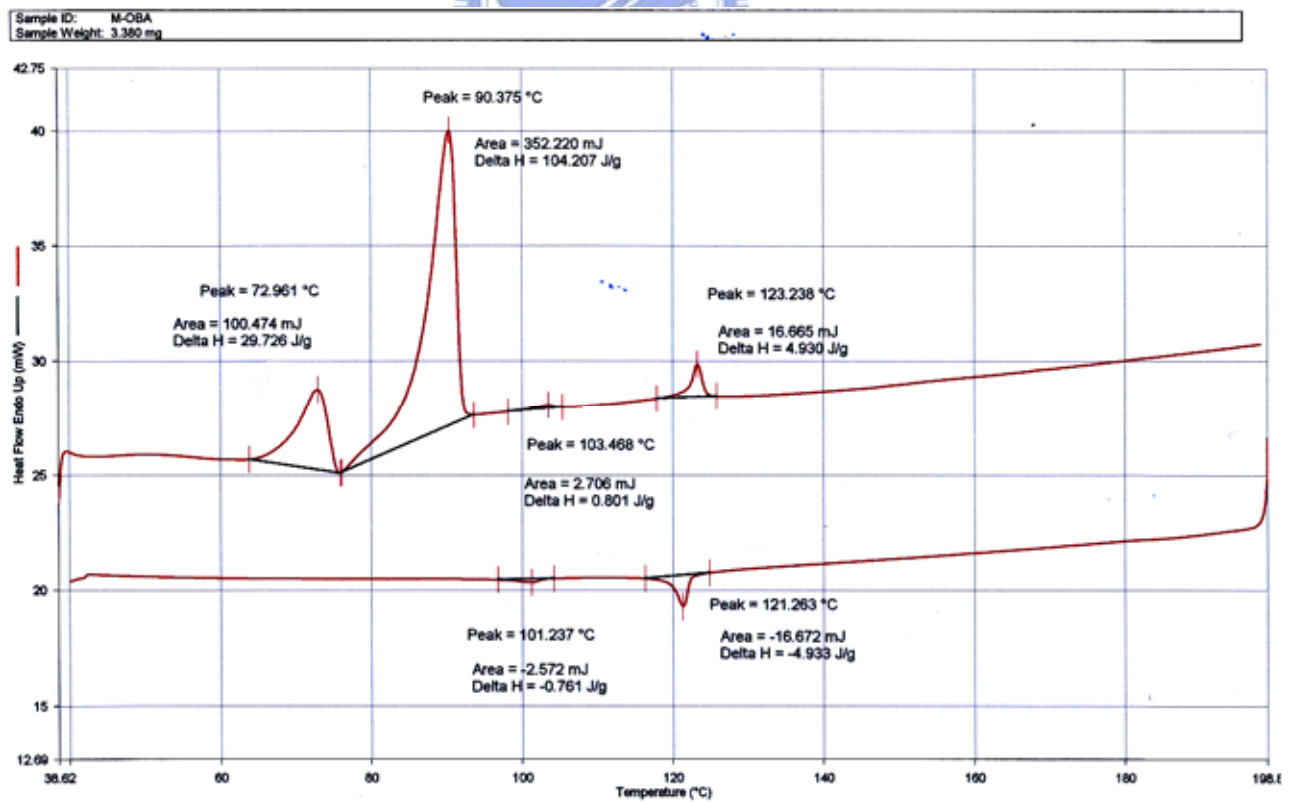
附圖 19. PDMB3OC10MA-OBA second heating-cooling 之 DSC 圖
