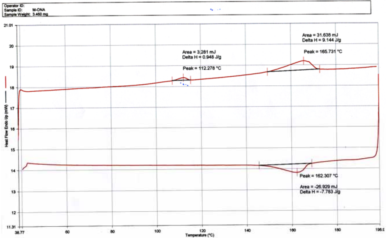
附圖 23. PDMB3OC10MA-ONA third heating-cooling 之 DSC 圖
