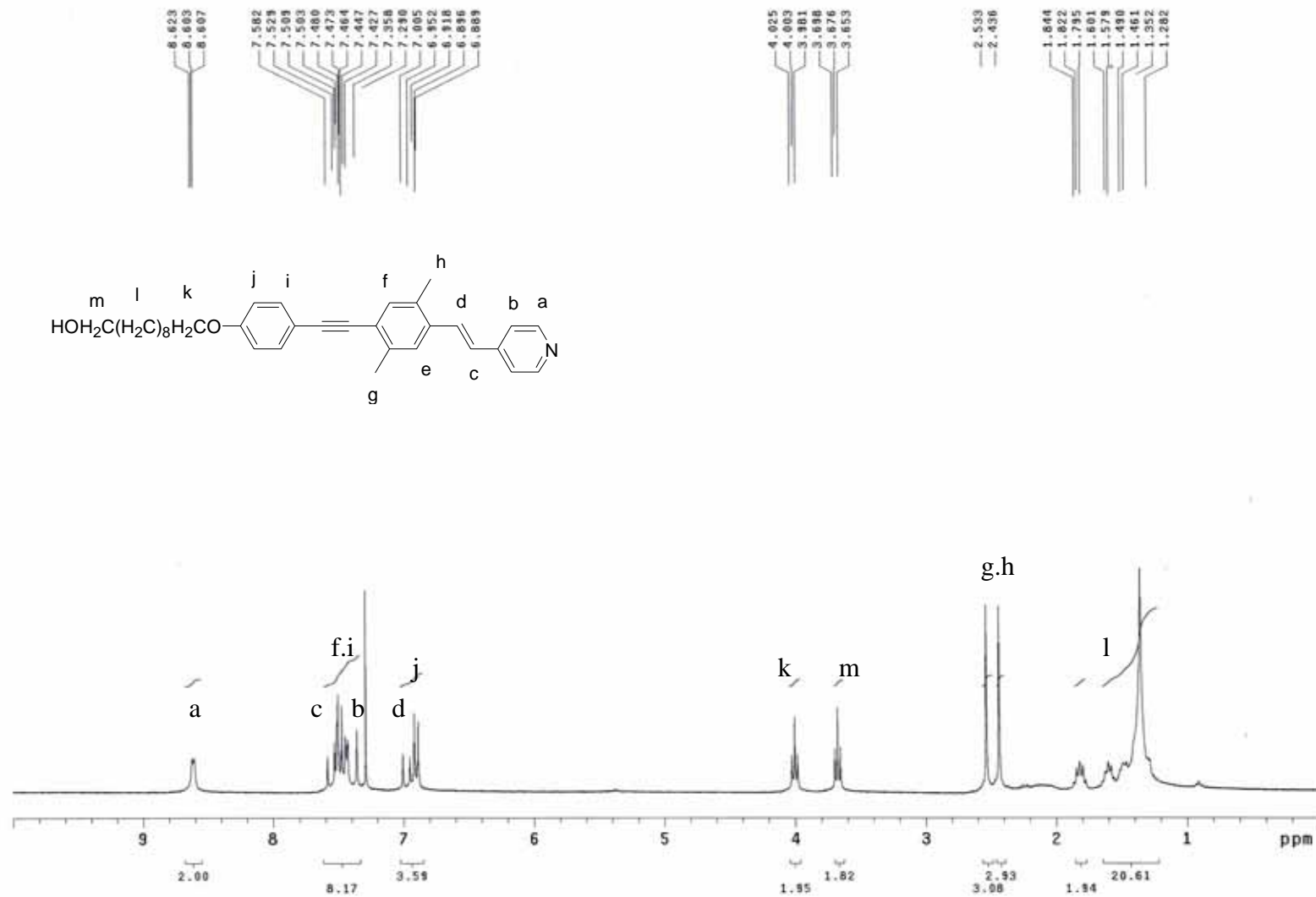
附圖 3. PDMB3OC10OH 之 1 H-NMR 圖
