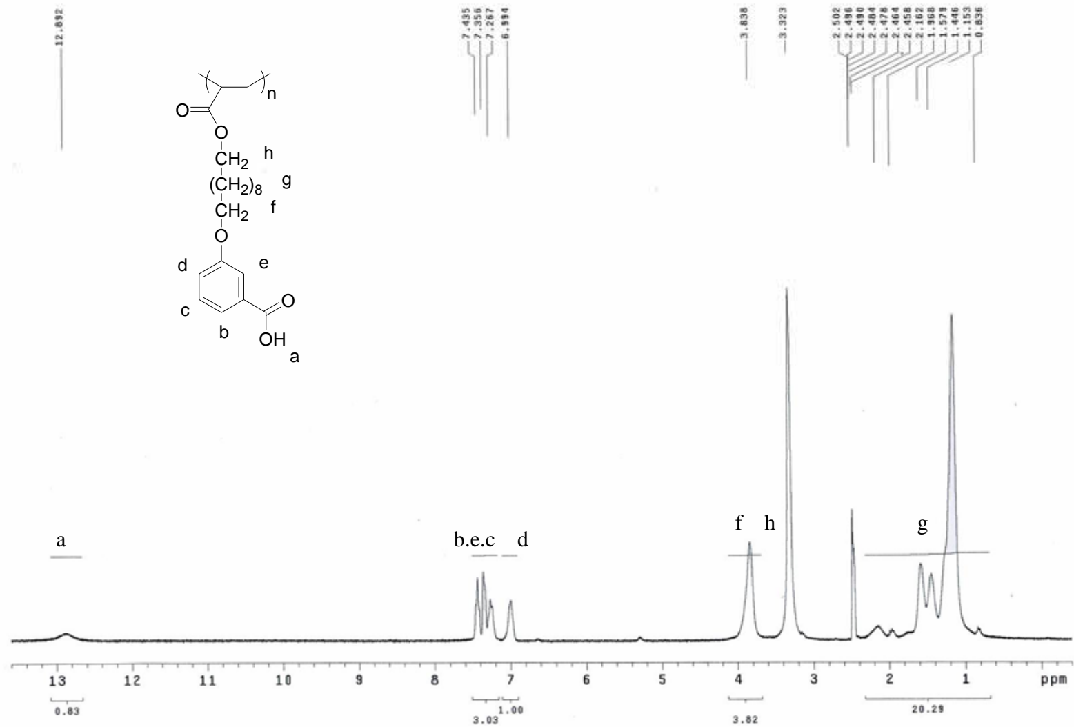
附圖 9. m-PC 10 BA 之 1 H-NMR 圖
