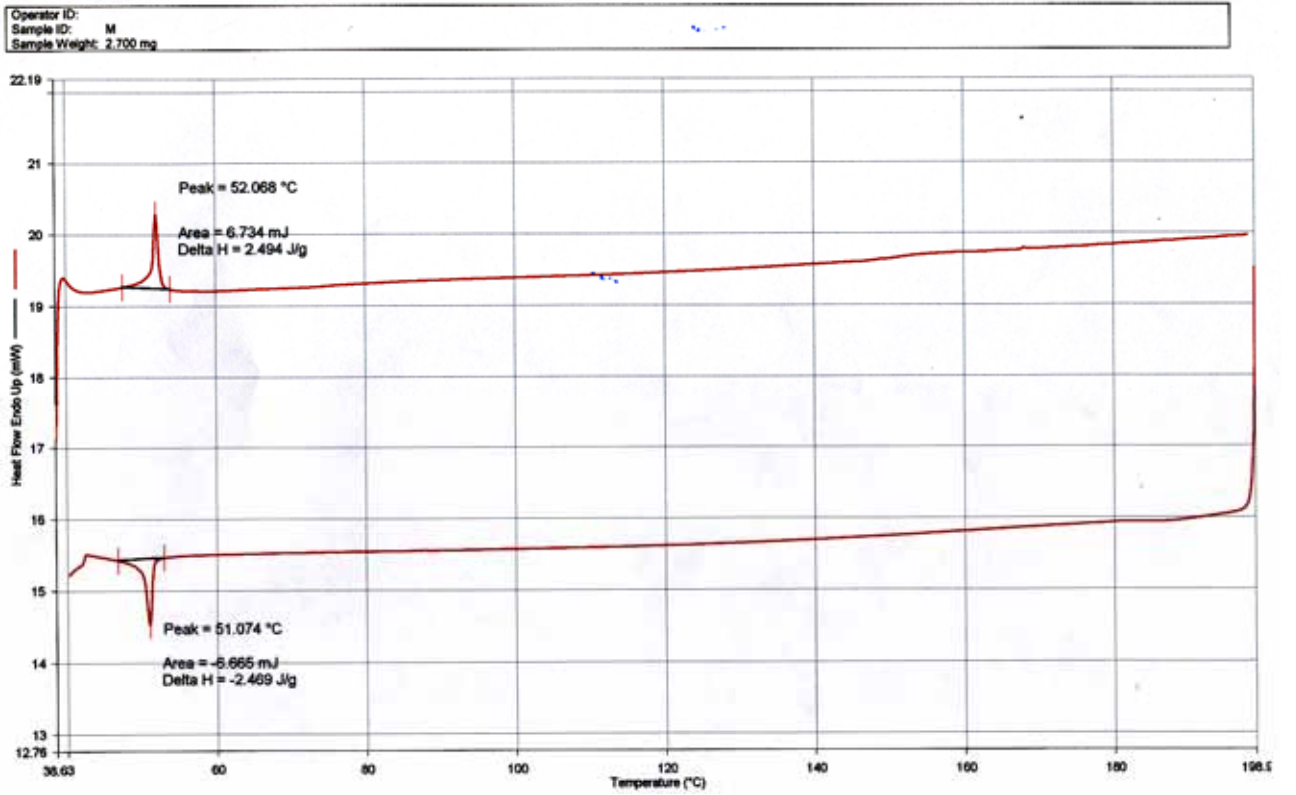
附圖 13. PDMB3OC10MA second heating-cooling 之 DSC 圖
