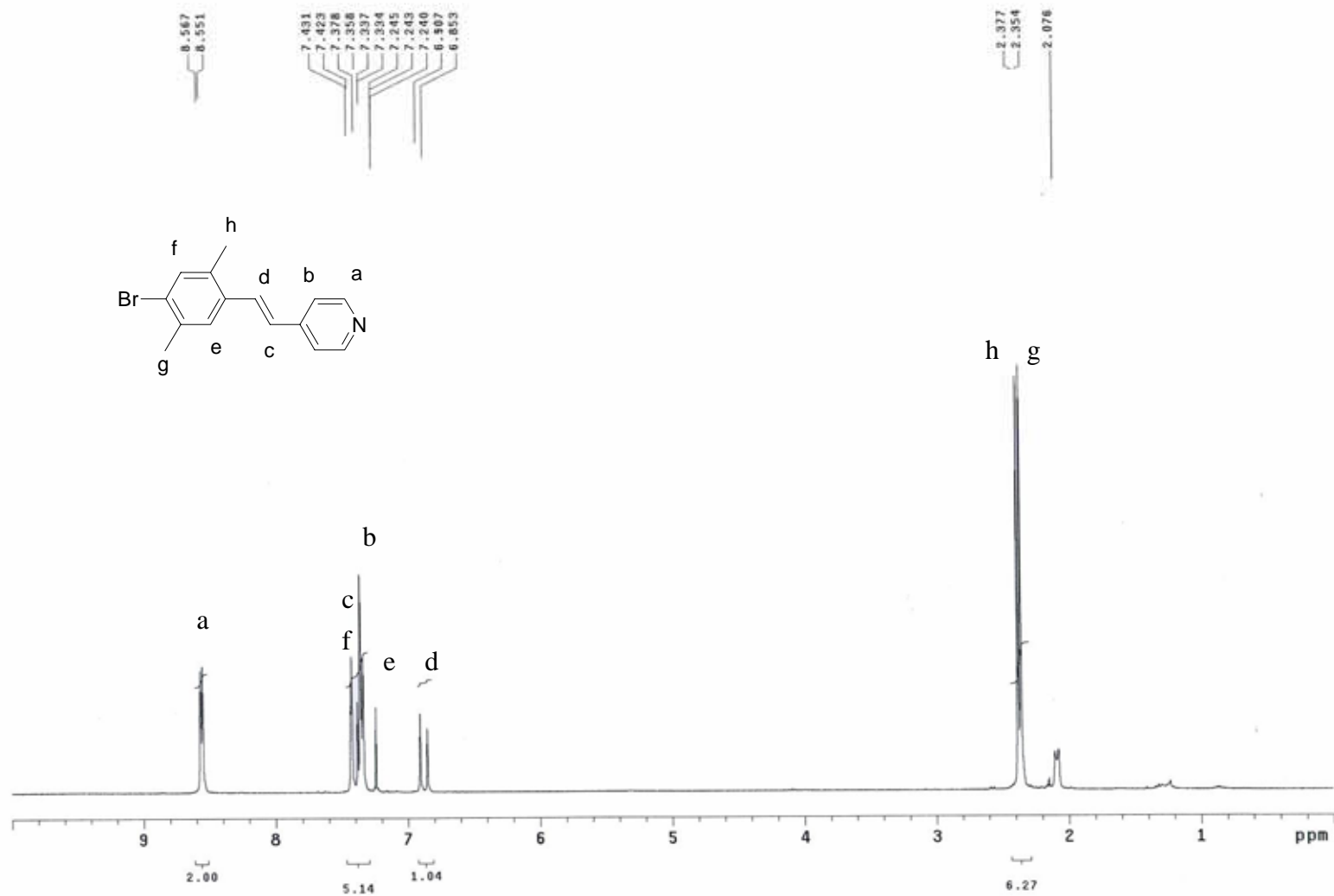
附圖 1.PDMBr 之 1 H-NMR 圖
