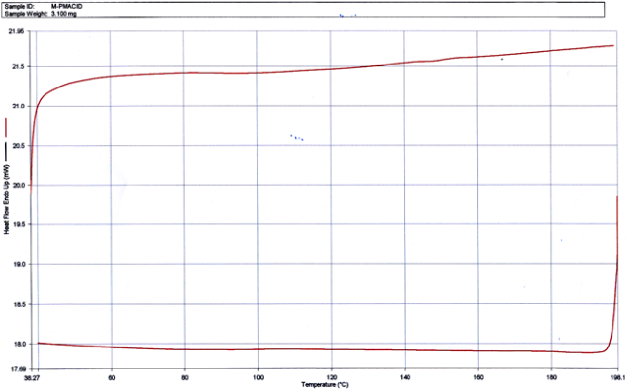
附圖 35. PDMB3OC10MA-m-PC 10 BA third heating-cooling 之 DSC 圖
