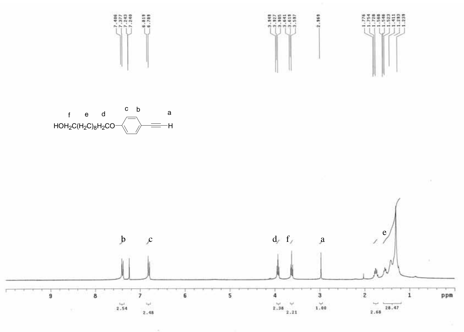
附圖 2. B3OC10OH 之 1 H-NMR 圖
