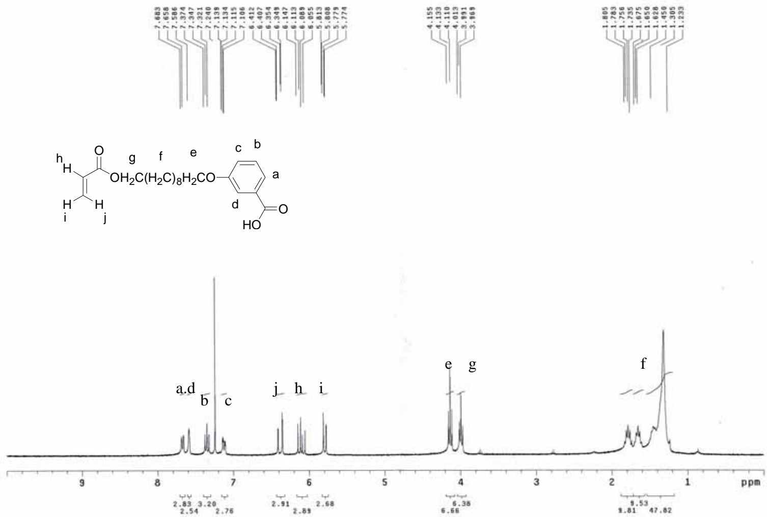
附圖 7. m-MC 10 BA 之 1 H-NMR 圖
