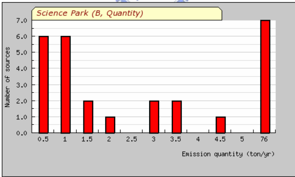
附圖 1.2 案例區污染物 B 之各濃度區間排放源數量分析圖
