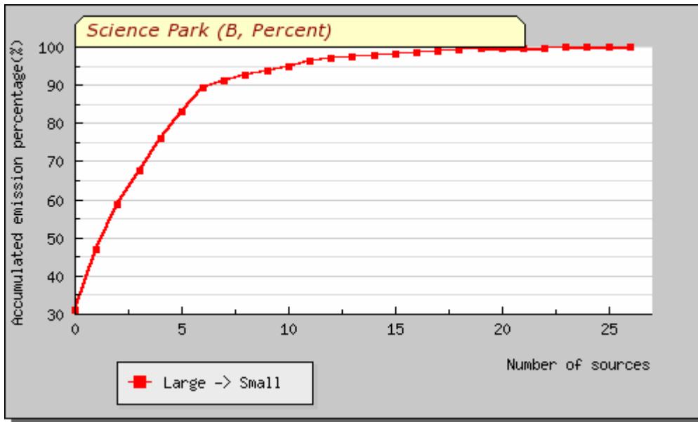
附圖 1.1 案例區污染物 B 之累積排放百分率圖
