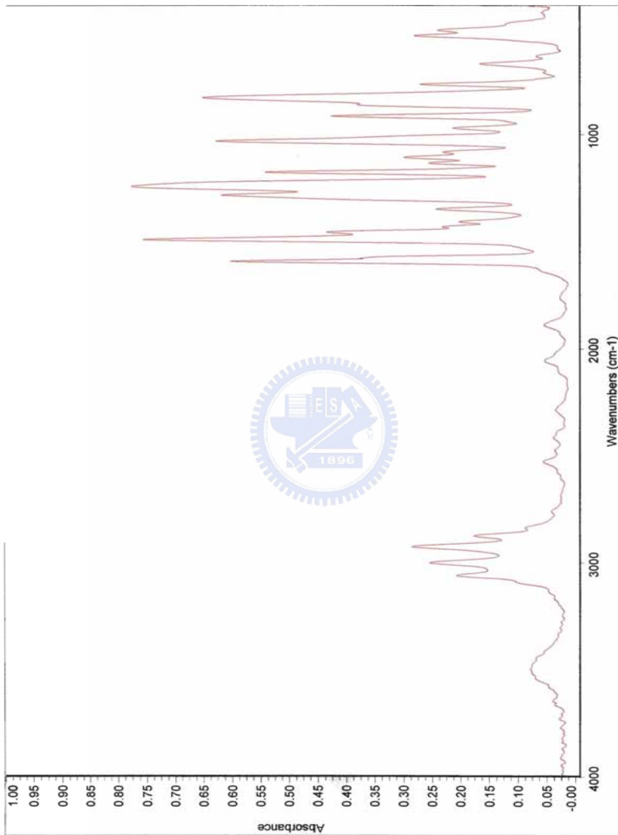
Figure3-3. Epoxy 的紅外線光譜
