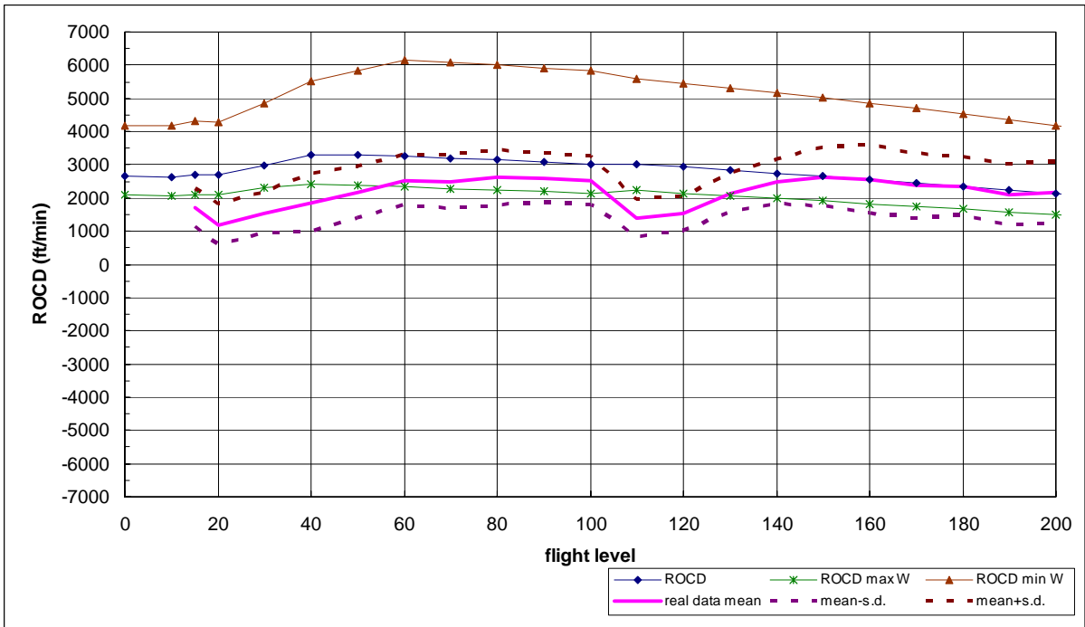
圖 7.51 B744 型機平均爬升飛航軌跡、爬升率圖(含標準差)
