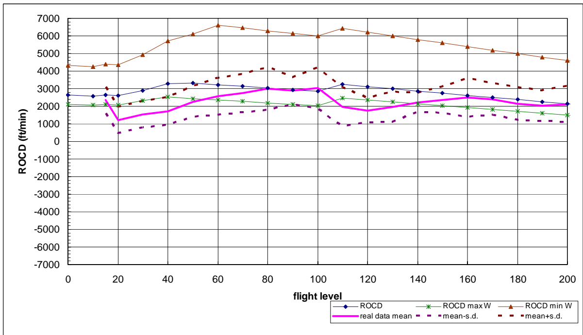
圖 7.59 MD11 型機平均爬升飛航軌跡、爬升率圖(含標準差)
