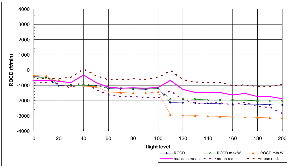
圖 7.46 A330 型機平均下降飛航軌跡、下降率圖(含標準差)
