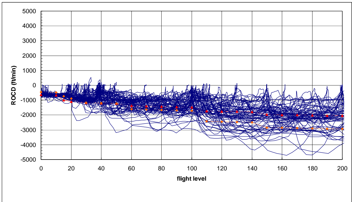
圖 7.36 B767 型機實際雷達資料下降飛航軌跡、下降率圖
