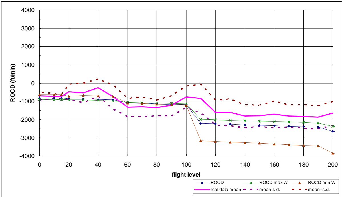
圖 7.52 B744 型機平均下降飛航軌跡、下降率圖(含標準差)
