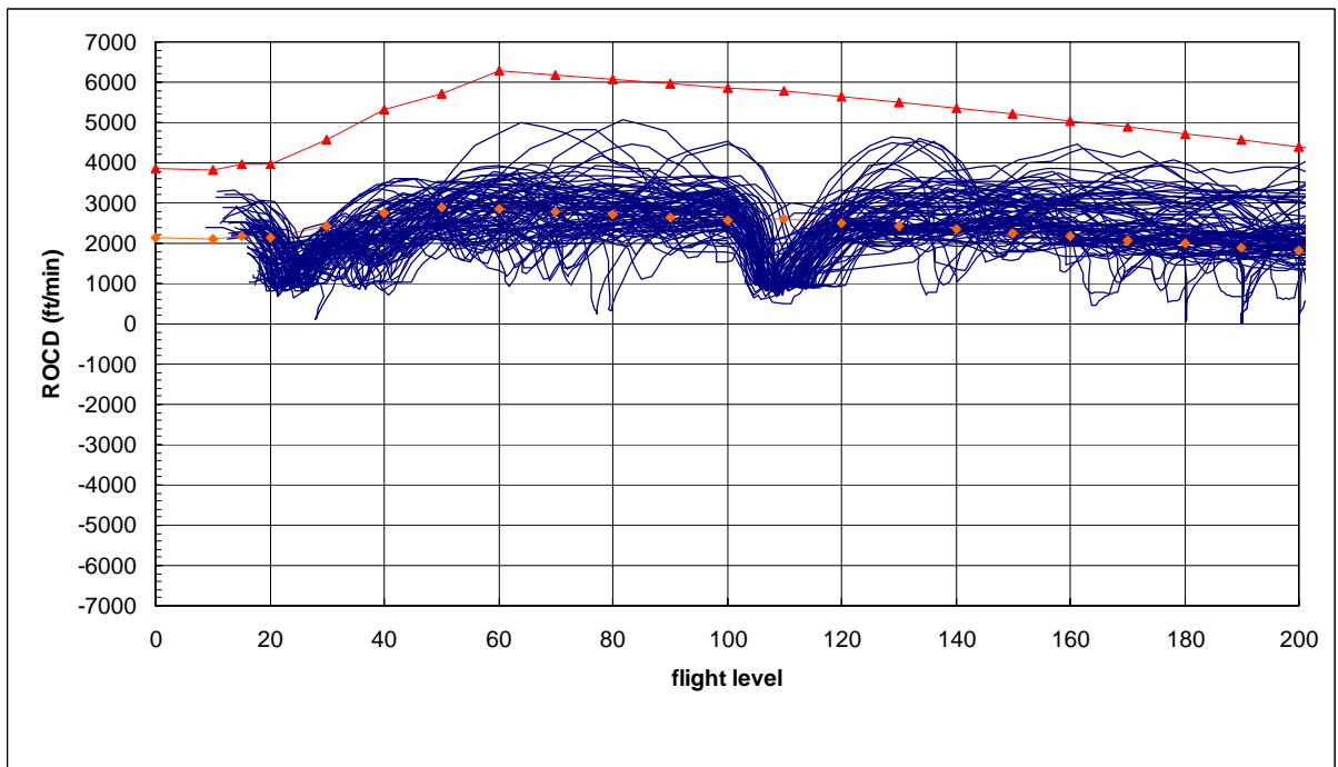
圖 7.29 B738 型機實際雷達資料爬升飛航軌跡、爬升率圖
