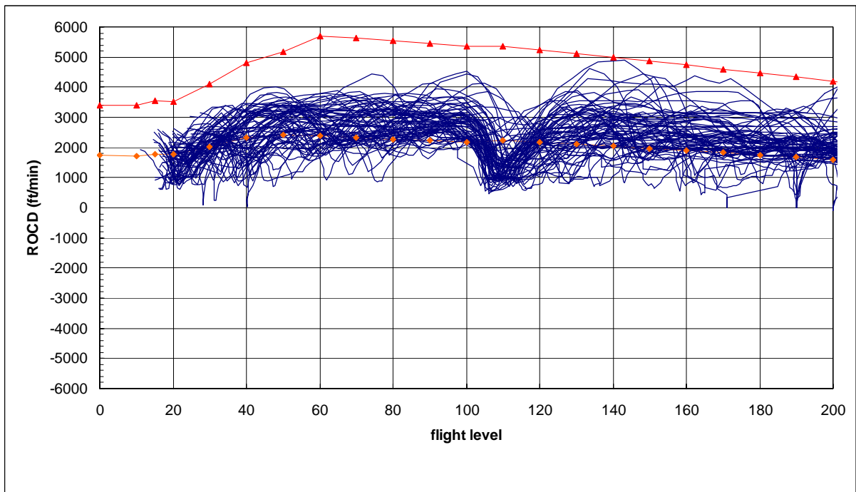
圖 7.33 B757 型機實際雷達資料爬升飛航軌跡、爬升率圖
