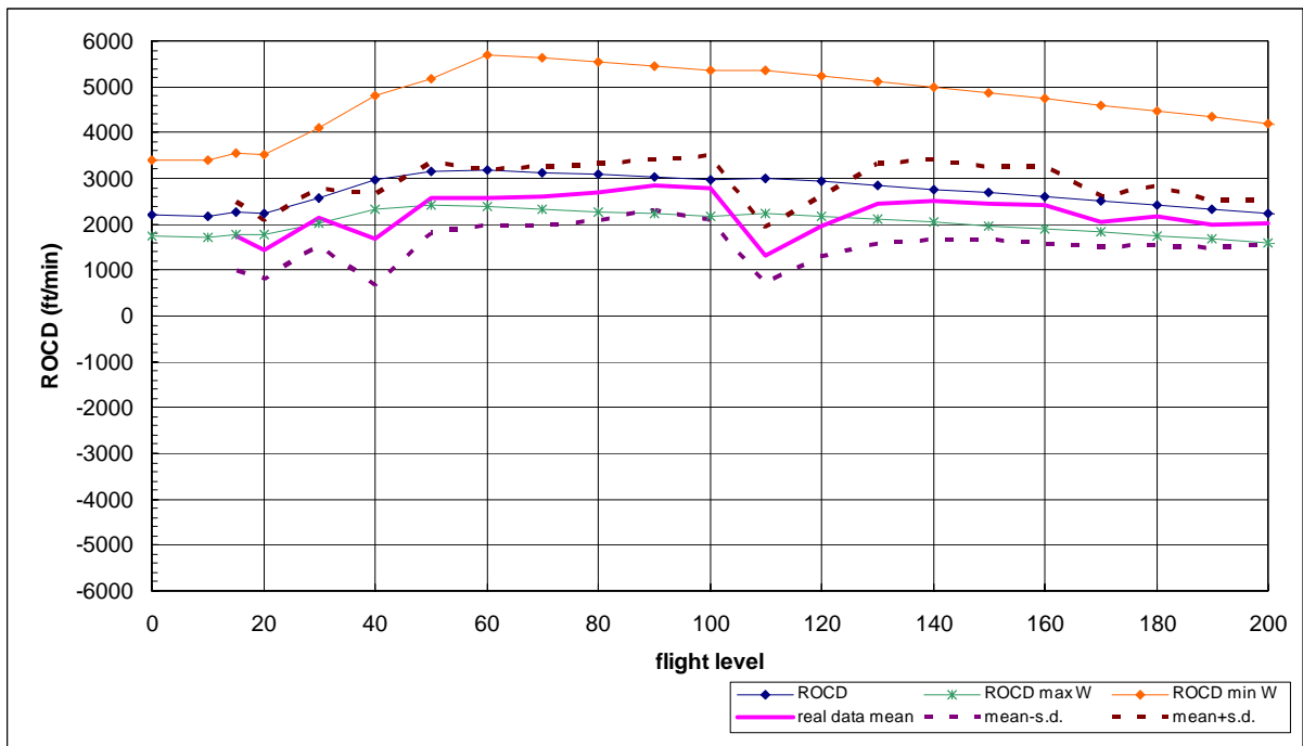
圖 7.53 B757 型機平均爬升飛航軌跡、爬升率圖(含標準差)
