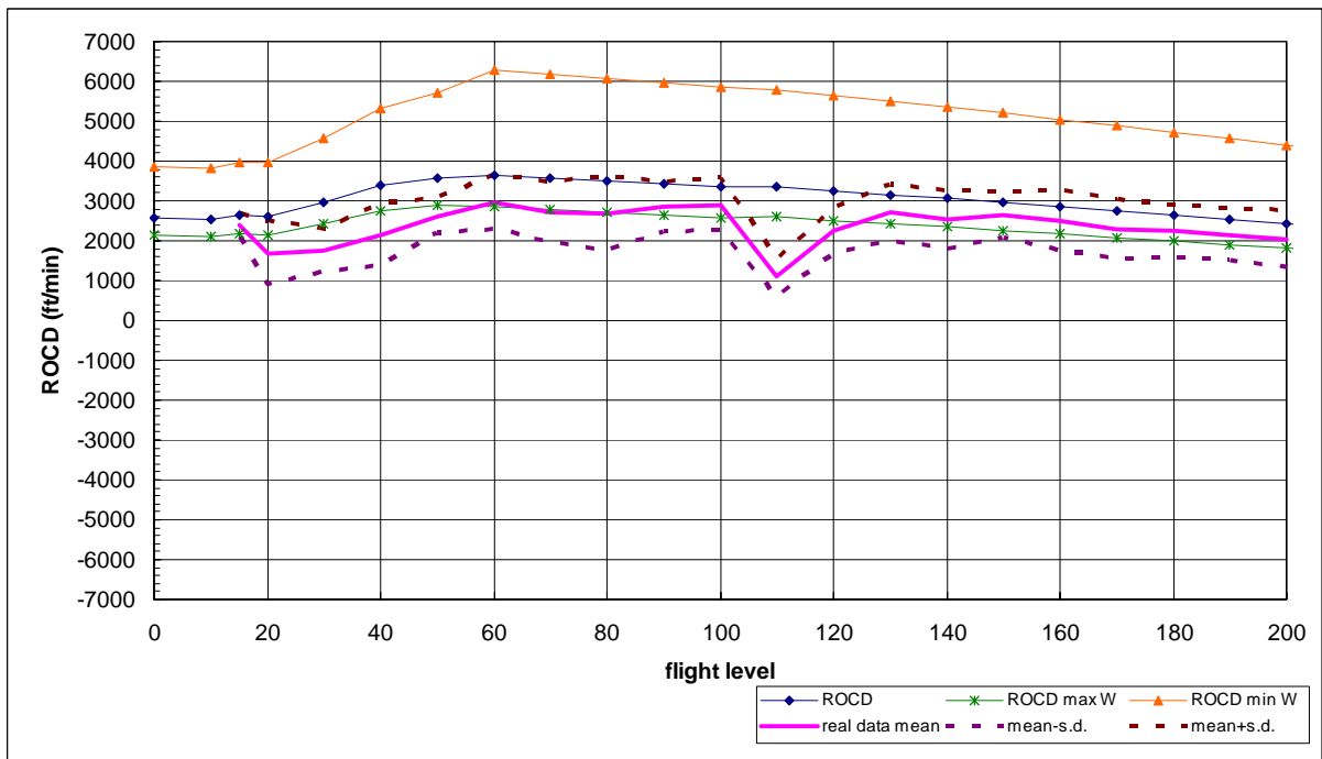
圖 7.49 B738 型機平均爬升飛航軌跡、爬升率圖(含標準差)
