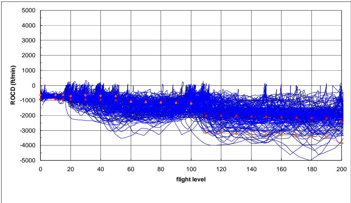
圖 7.32 B747 型機實際雷達資料下降飛航軌跡、下降率圖
