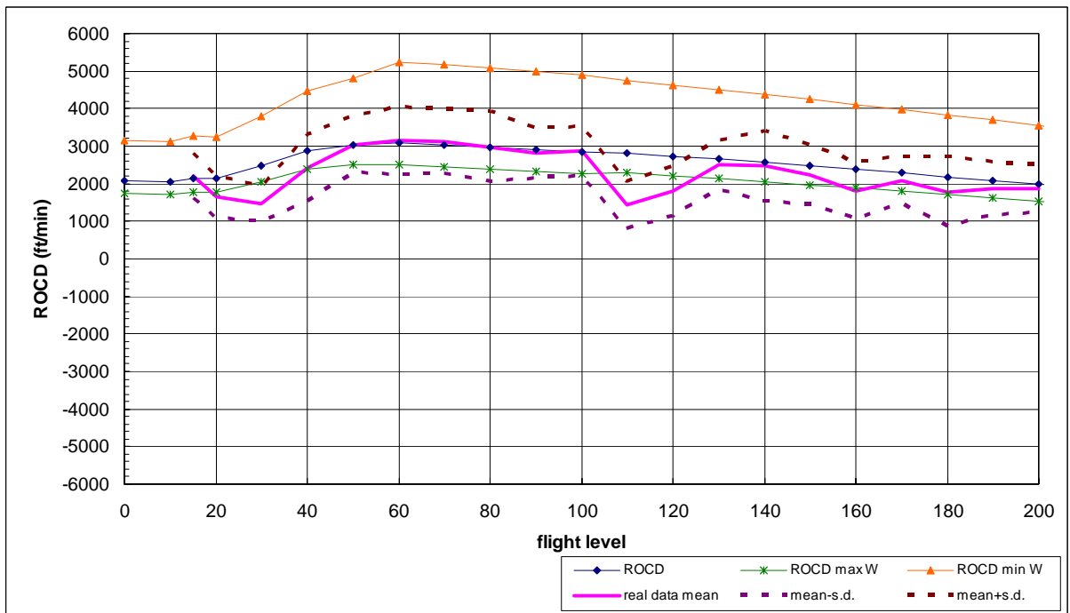
圖 7.43 A321 型機平均爬升飛航軌跡、爬升率圖(含標準差)
