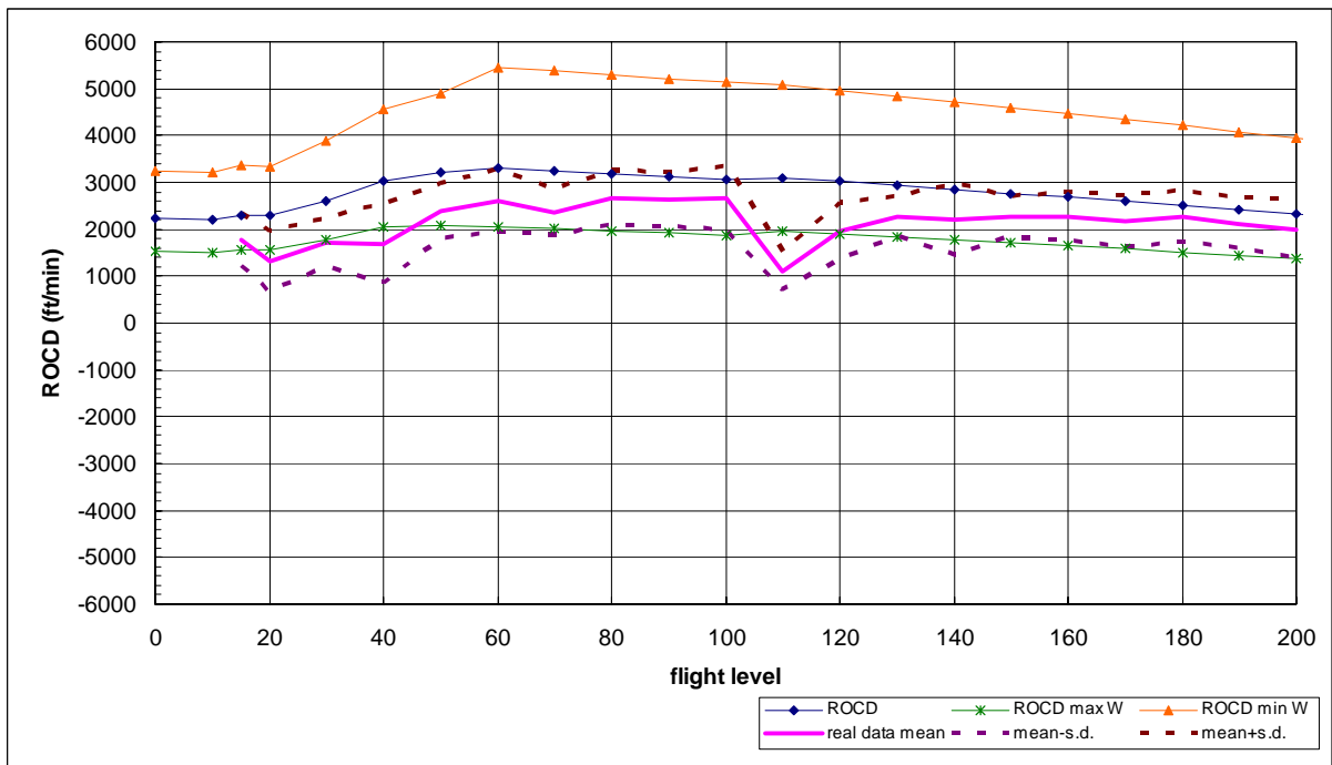
圖 7.57 B777 型機平均爬升飛航軌跡、爬升率圖(含標準差)
