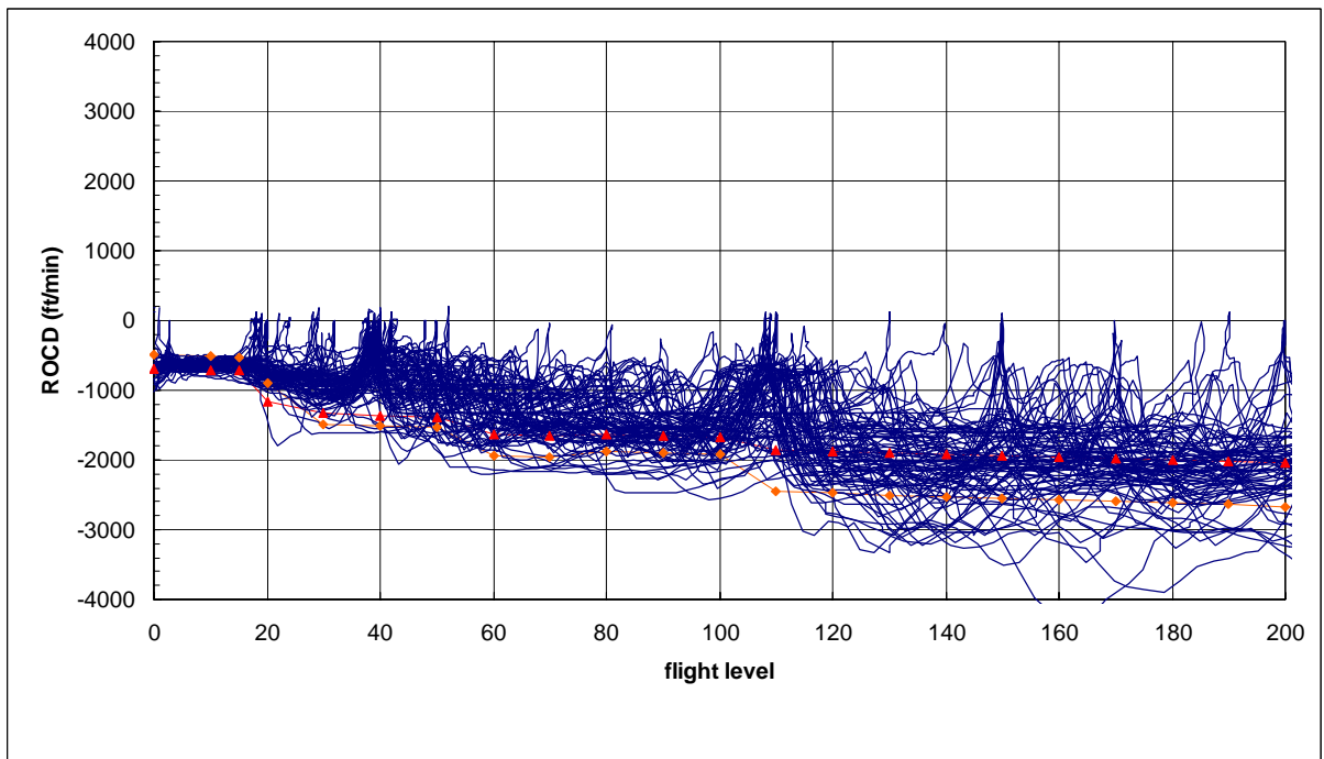
圖 7.22 A306 型機實際雷達資料下降飛航軌跡、下降率圖
