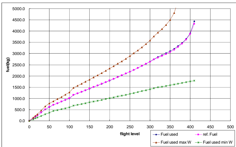
圖 7.15 BADA B767 型機爬升飛航軌跡、爬升率、油耗圖
