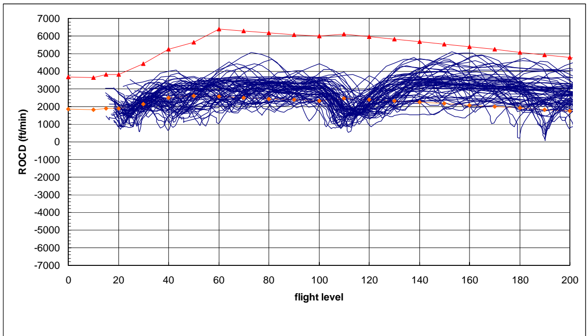
圖 7.35 B767 型機實際雷達資料爬升飛航軌跡、爬升率圖
