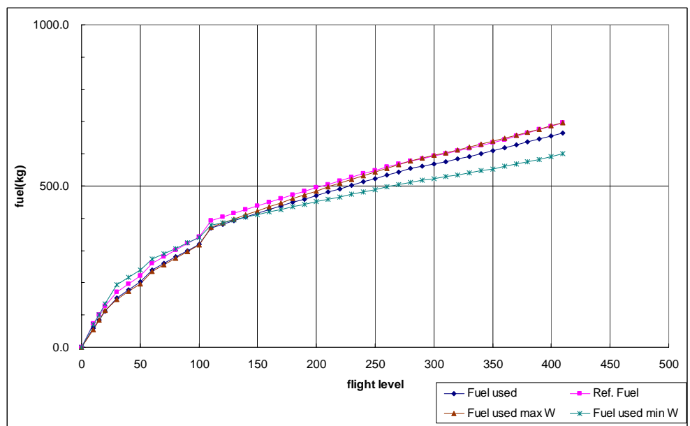
圖 7.6 BADA A330 型機下降飛航軌跡、下降率、油耗圖
