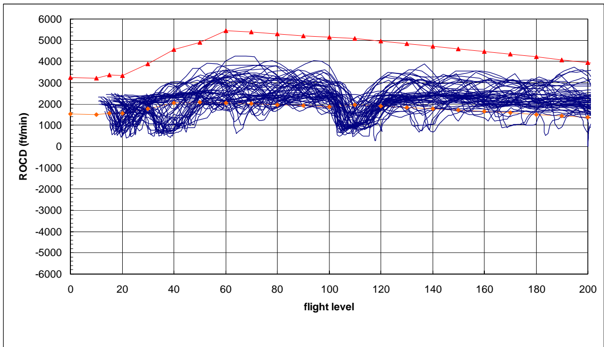
圖 7.37 B777 型機實際雷達資料爬升飛航軌跡、爬升率圖
