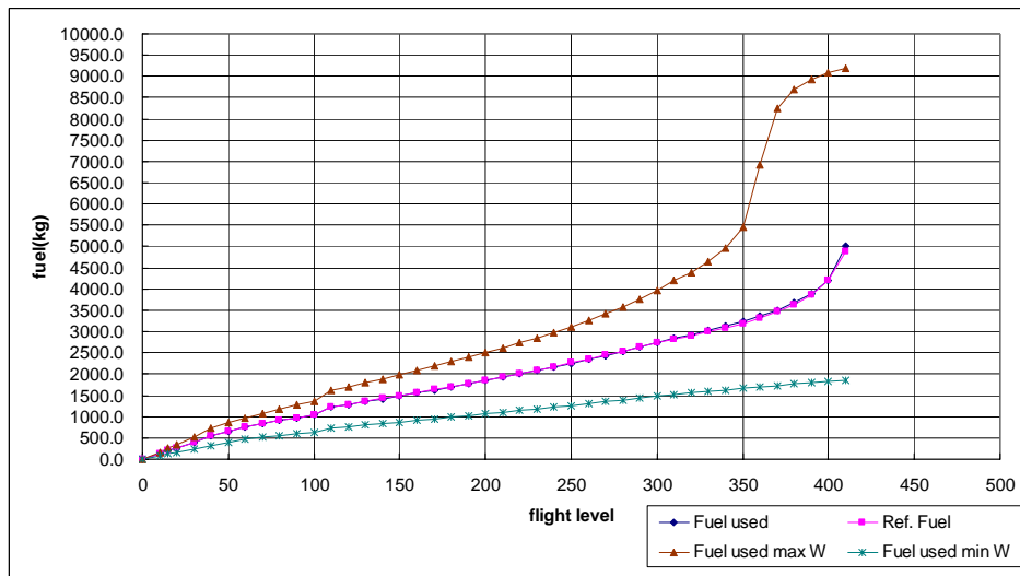
圖 7.1 BADA A306 型機爬升飛航軌跡、爬升率、油耗圖
