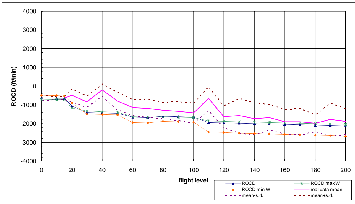
圖 7.42 A306 型機平均下降飛航軌跡、下降率圖(含標準差)
