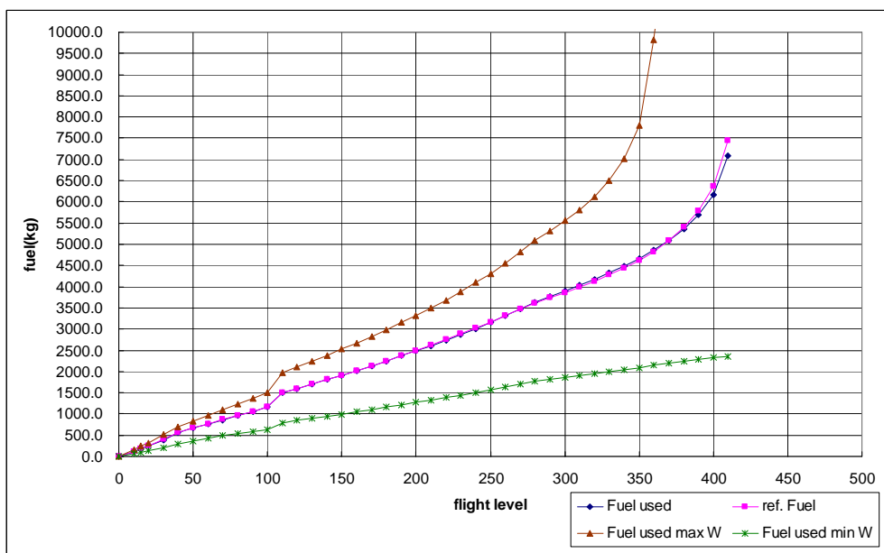
圖 7.19 BADA MD11 型機爬升飛航軌跡、爬升率、油耗圖
