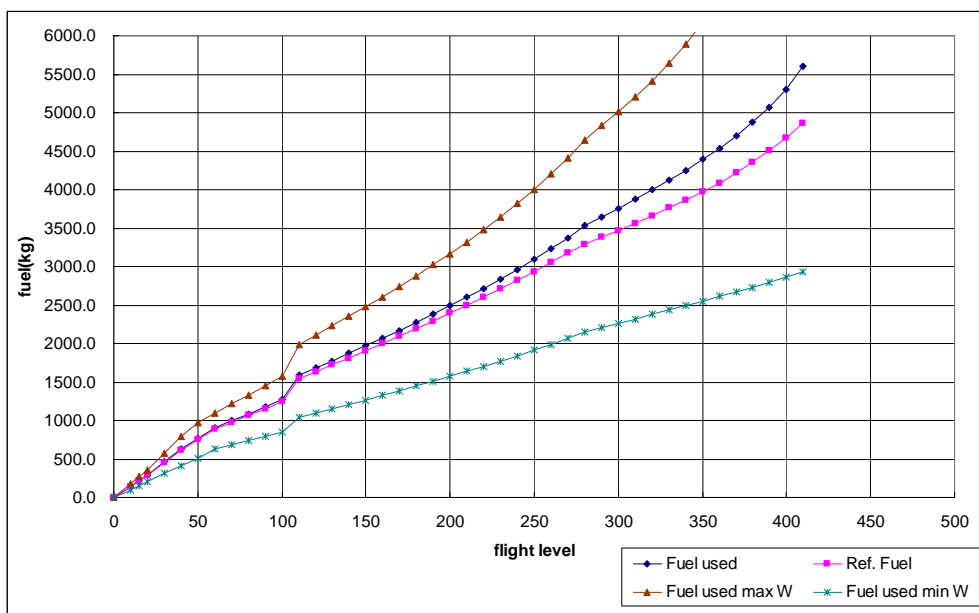
圖 7.5 BADA A330 型機爬升飛航軌跡、爬升率、油耗圖
