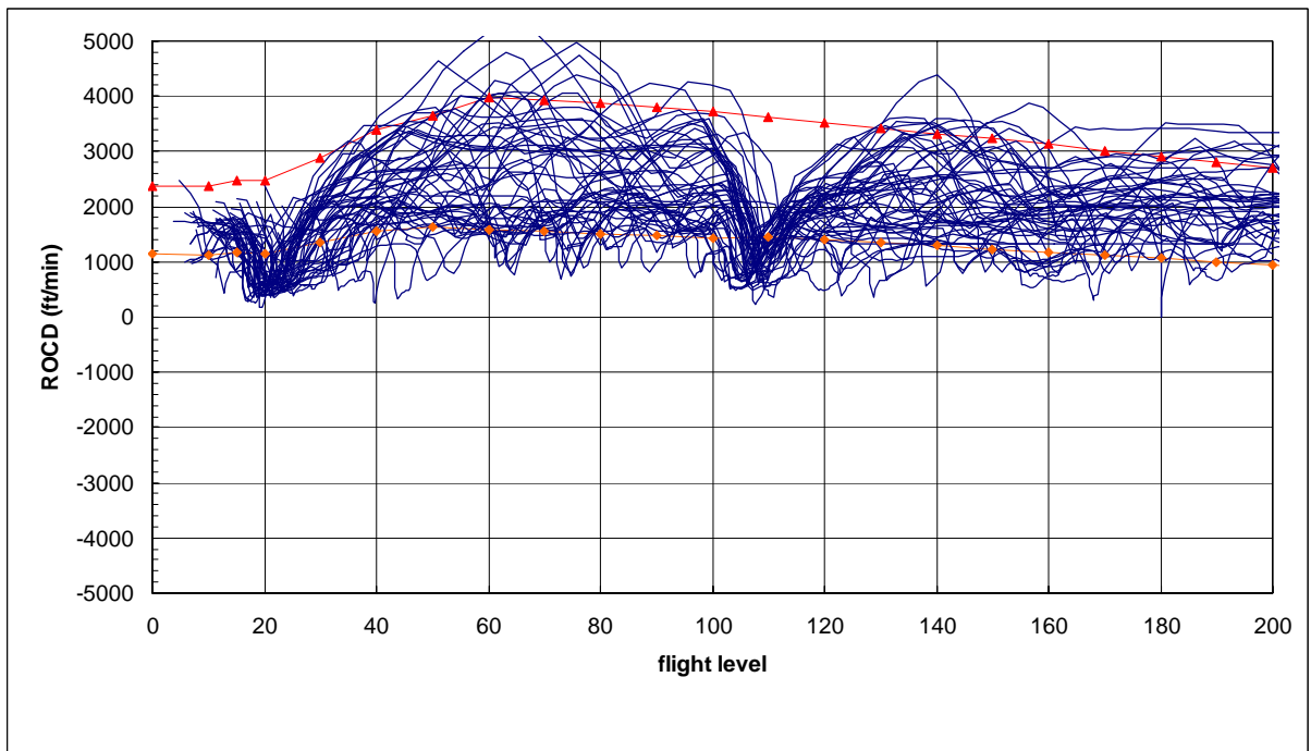
圖 7.27 A340 型機實際雷達資料爬升飛航軌跡、爬升率圖
