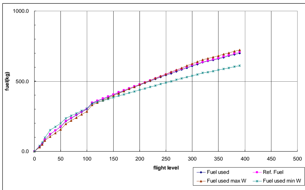
圖 7.8 BADA A340 型機下降飛航軌跡、下降率、油耗圖
