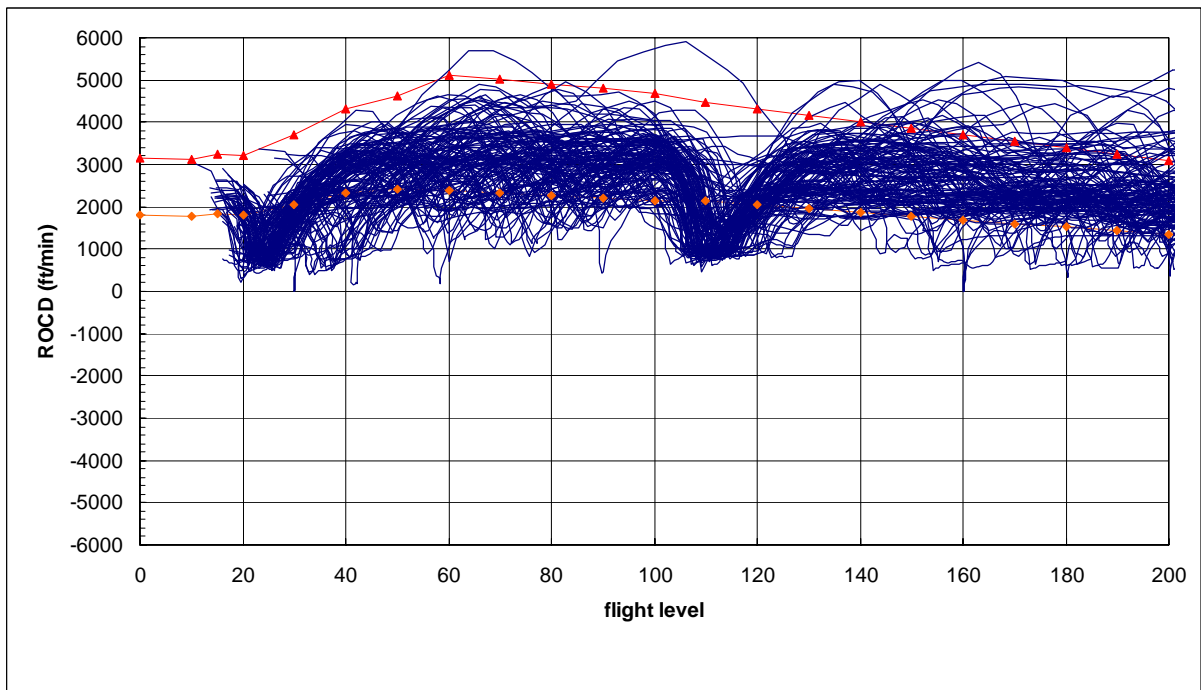
圖 7.25 A330 型機實際雷達資料爬升飛航軌跡、爬升率圖
