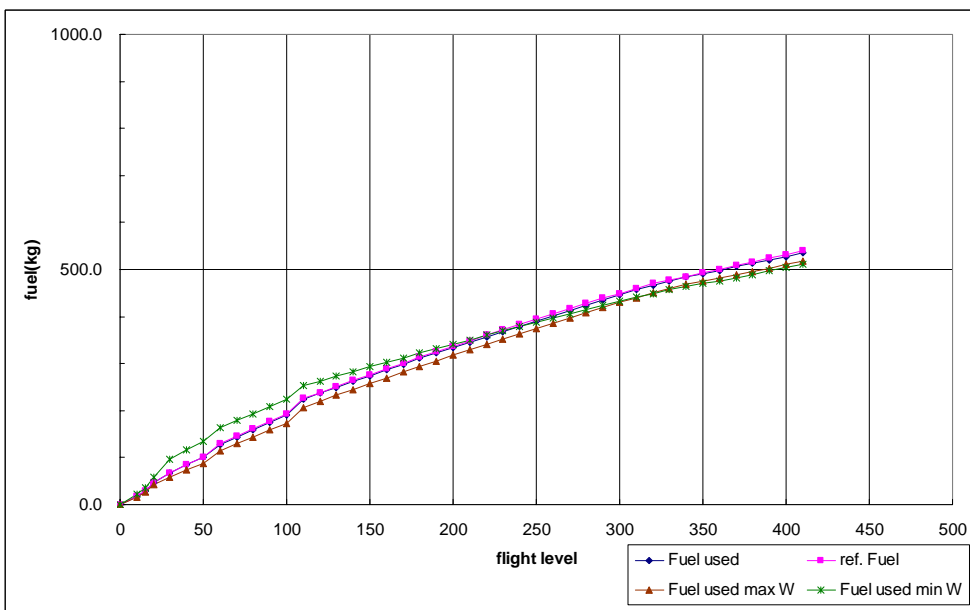
圖 7.20 BADA MD11 型機下降飛航軌跡、下降率、油耗圖
