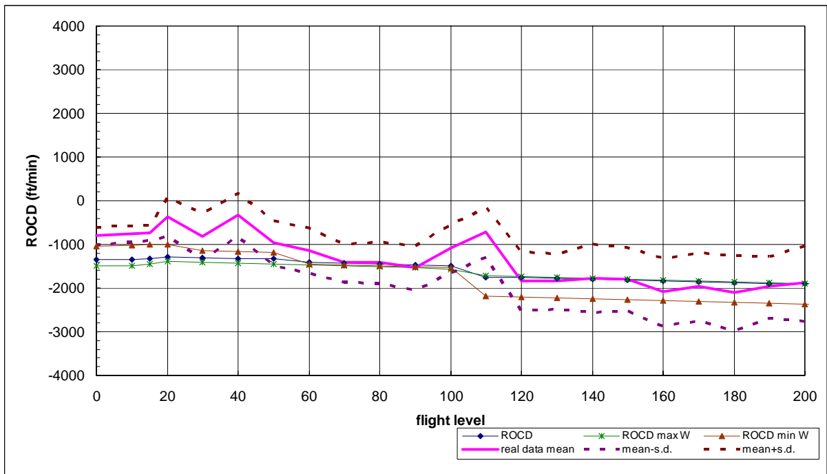
圖 7.60 MD11 型機平均下降飛航軌跡、下降率圖(含標準差)
