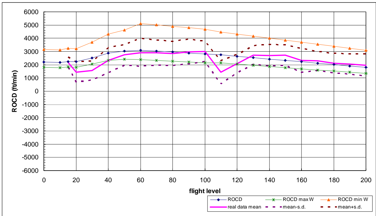
圖 7.45 A330 型機平均爬升飛航軌跡、爬升率圖(含標準差)
