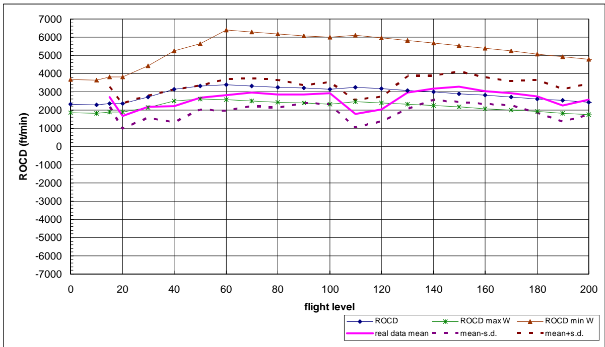
圖 7.55 B767 型機平均爬升飛航軌跡、爬升率圖(含標準差)
