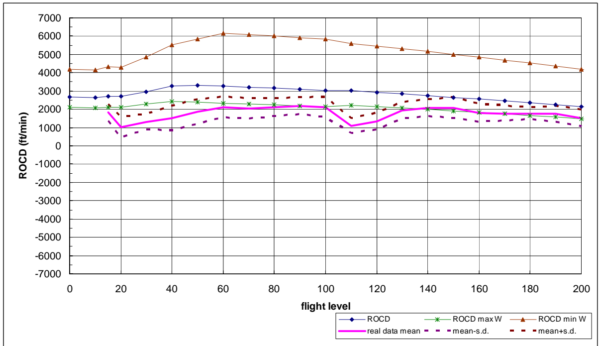
圖 7.61 B744 型機長程(long haul)平均爬升飛航軌跡、爬升率圖(含標準差)
