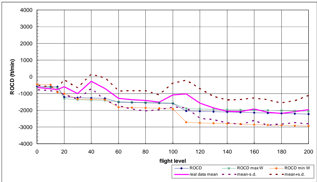
圖 7.54 B757 型機平均下降飛航軌跡、下降率圖(含標準差)
