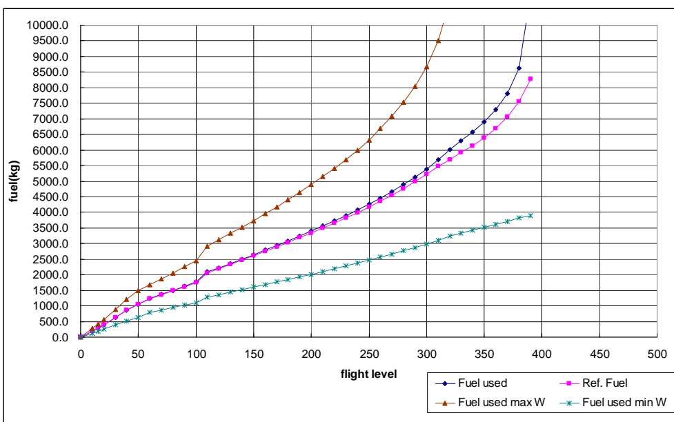
圖 7.7 BADA A340 型機爬升飛航軌跡、爬升率、油耗圖
