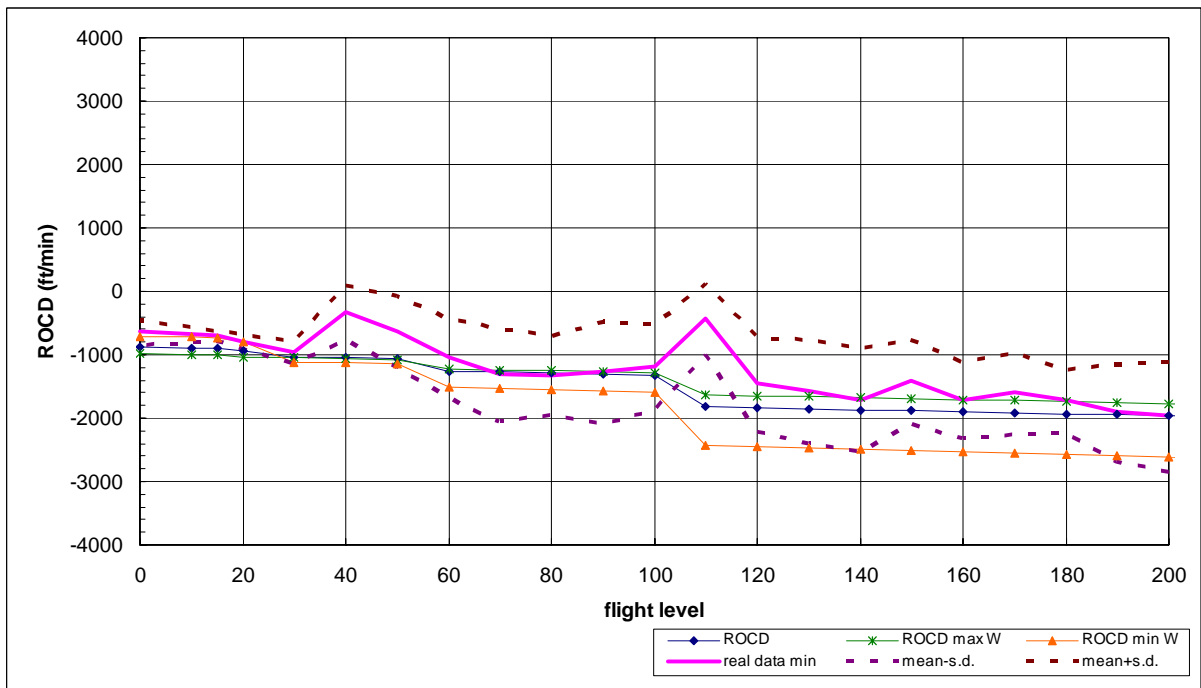
圖 7.48 A340 型機平均下降飛航軌跡、下降率圖(含標準差)
