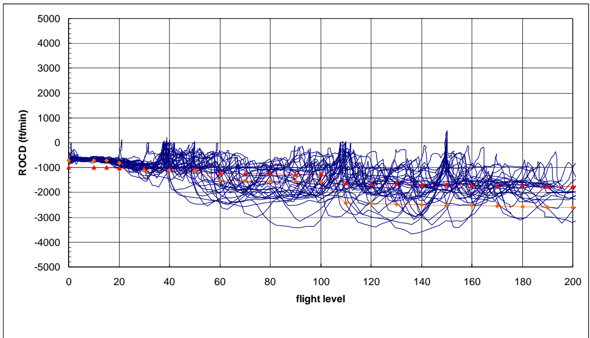
圖 7.28 A340 型機實際雷達資料下降飛航軌跡、下降率圖
