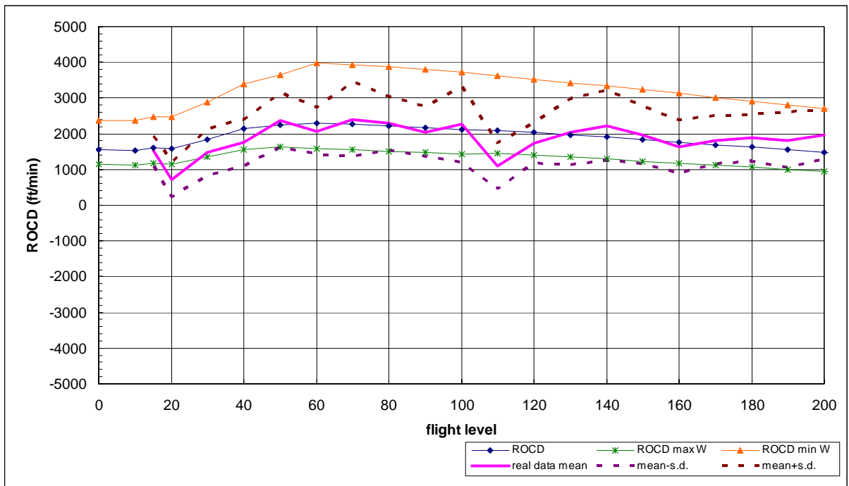
圖 7.47 A340 型機平均爬升飛航軌跡、爬升率圖(含標準差)
