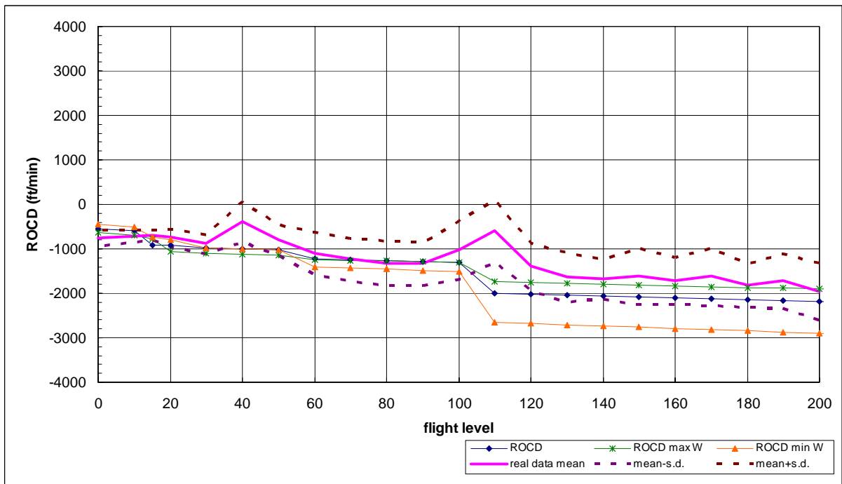
圖 7.58 B777 型機平均下降飛航軌跡、下降率圖(含標準差)
