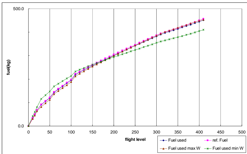
圖 7.16 BADA B767 型機下降飛航軌跡、下降率、油耗圖
