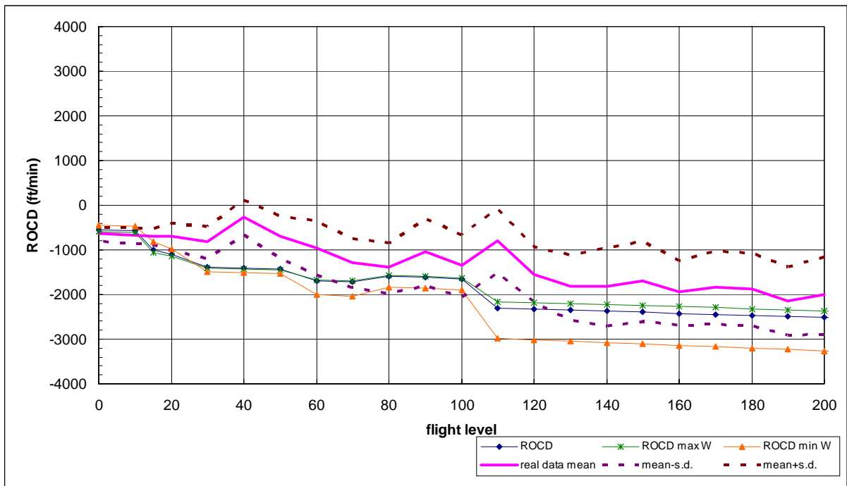
圖 7.44 A321 型機平均下降飛航軌跡、下降率圖(含標準差)
