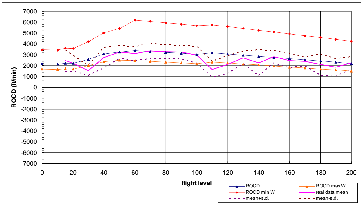
圖 7.41 A306 型機平均爬升飛航軌跡、爬升率圖(含標準差)
