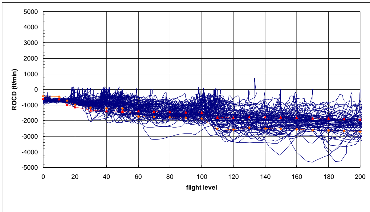
圖 7.30 B738 型機實際雷達資料下降飛航軌跡、下降率圖
