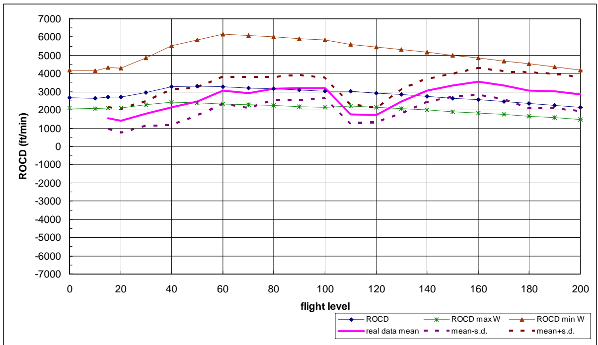
圖 7.62 B744 型機短程(short range)平均爬升飛航軌跡、爬升率圖(含標準差)
