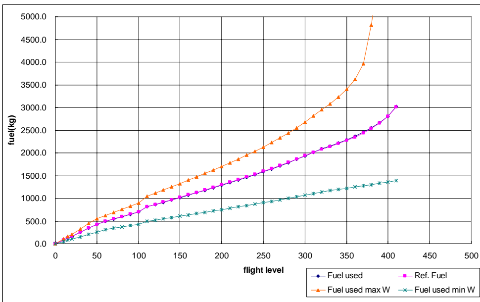
圖 7.13 BADA B752 型機爬升飛航軌跡、爬升率、油耗圖
