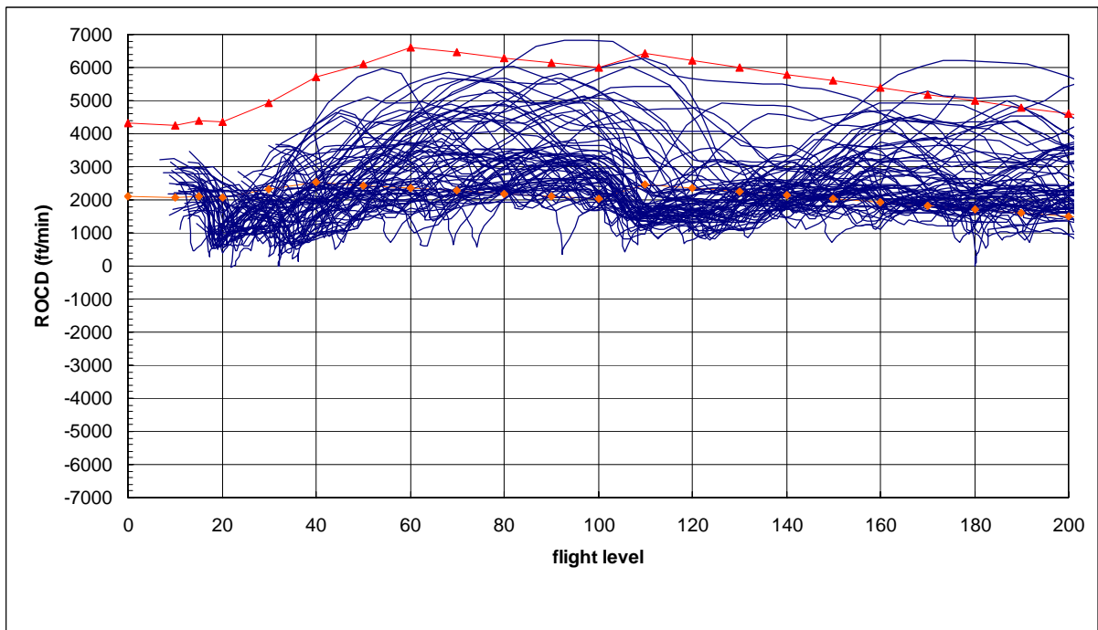
圖 7.39 MD11 型機實際雷達資料爬升飛航軌跡、爬升率圖
