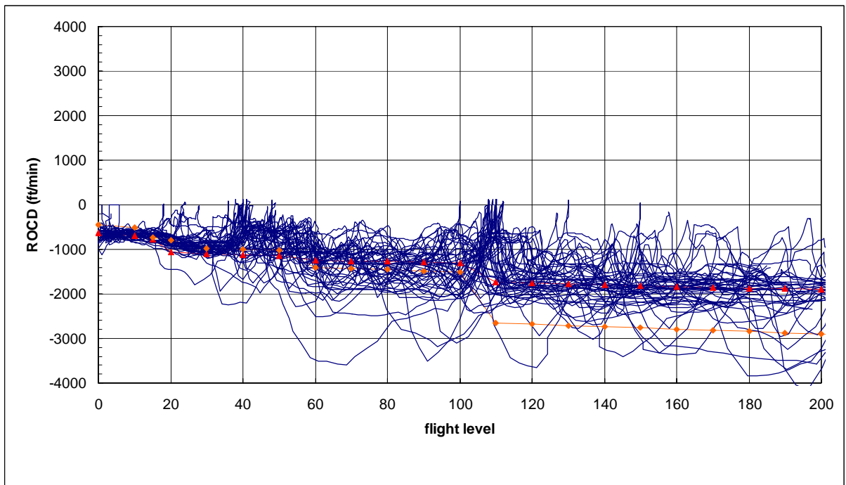
圖 7.38 B777 型機實際雷達資料下降飛航軌跡、下降率圖
