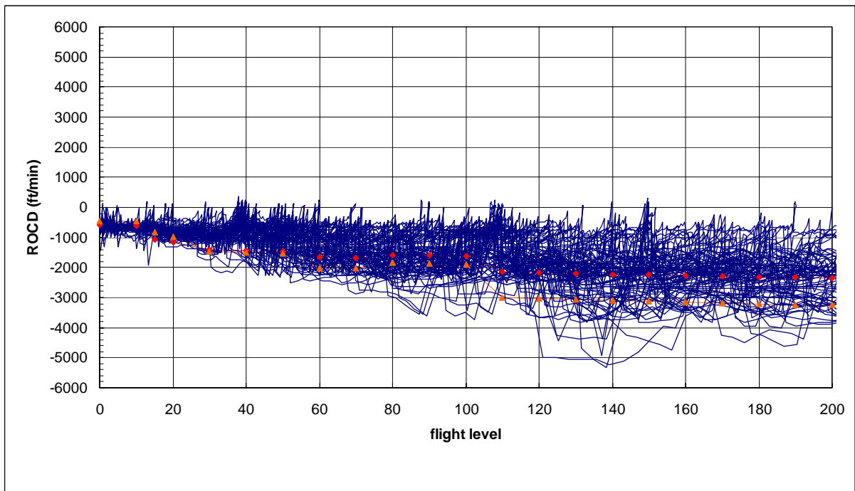
圖 7.24 A321 型機實際雷達資料下降飛航軌跡、下降率圖
