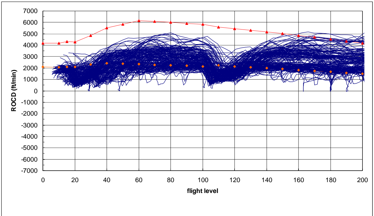
圖 7.31 B747 型機實際雷達資料爬升飛航軌跡、爬升率圖
