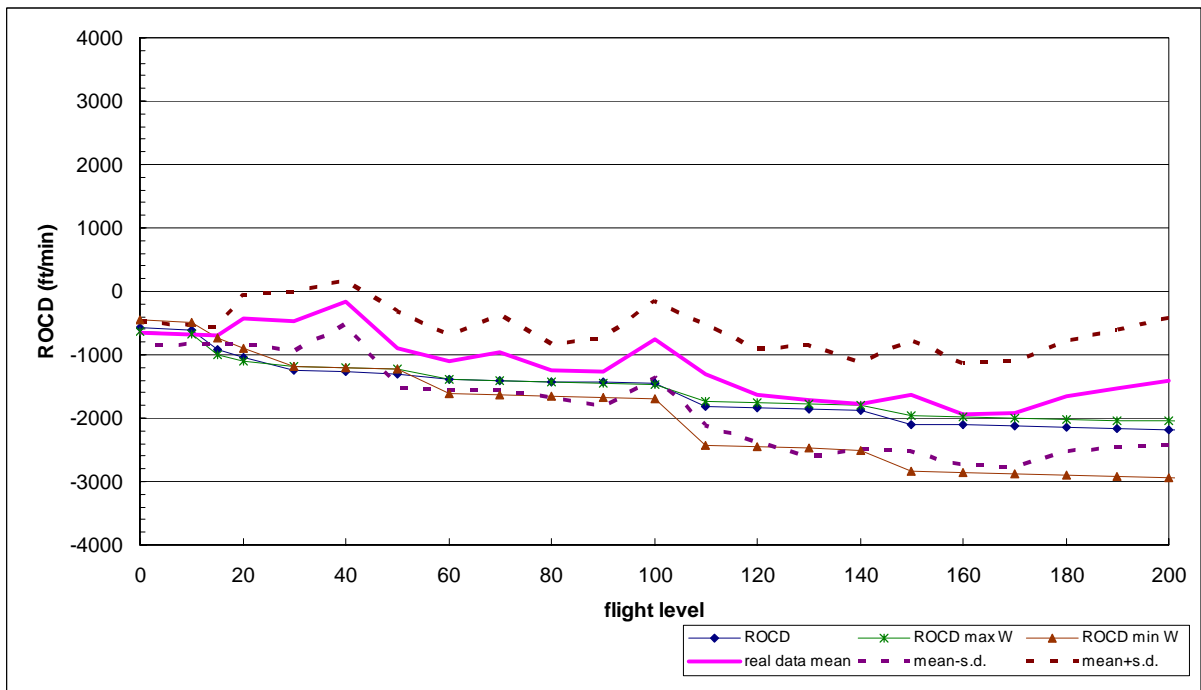
圖 7.56 B767 型機平均下降飛航軌跡、下降率圖(含標準差)
