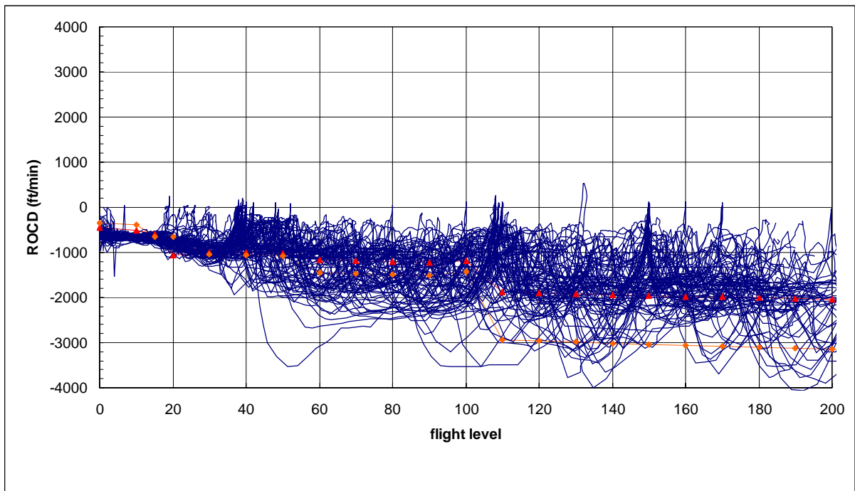
圖 7.26 A330 型機實際雷達資料下降飛航軌跡、下降率圖
