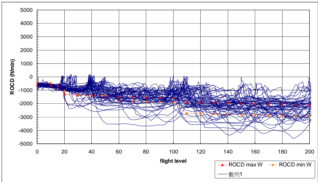
圖 7.34 B757 型機實際雷達資料下降飛航軌跡、下降率圖
