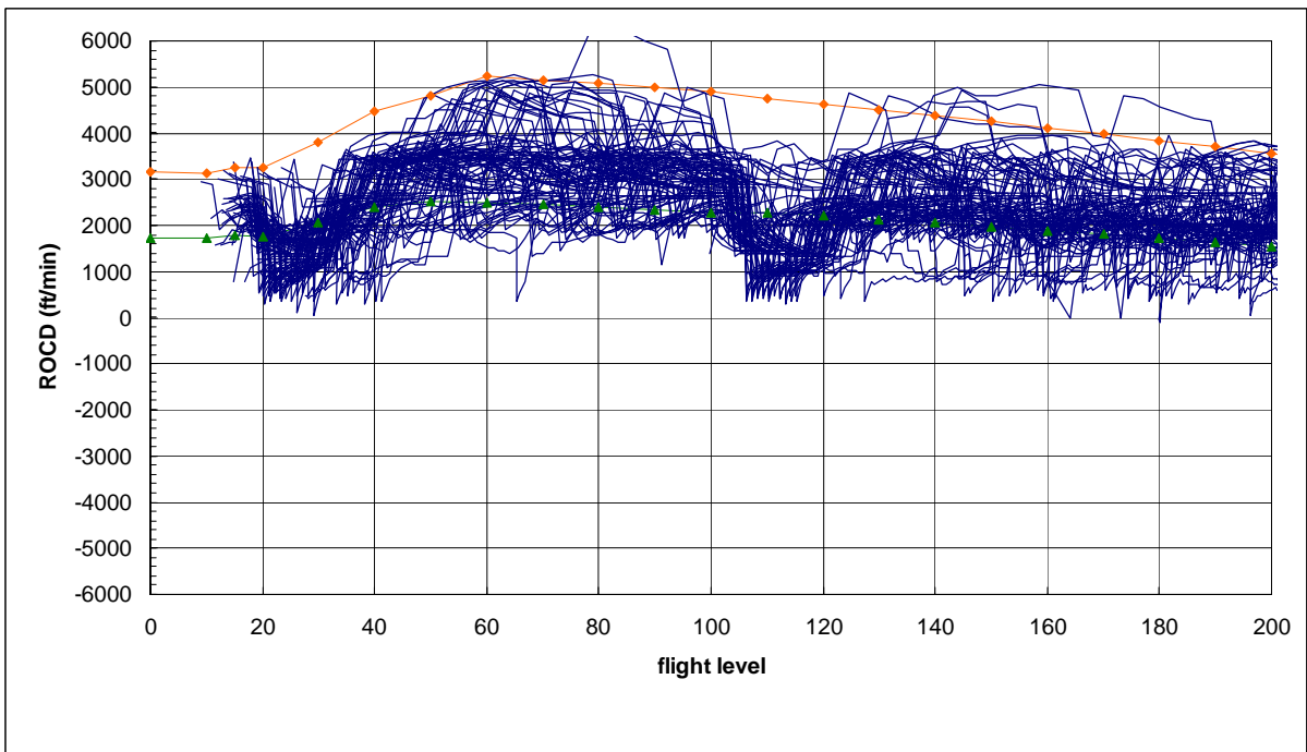
圖 7.23 A321 型機實際雷達資料爬升飛航軌跡、爬升率圖
