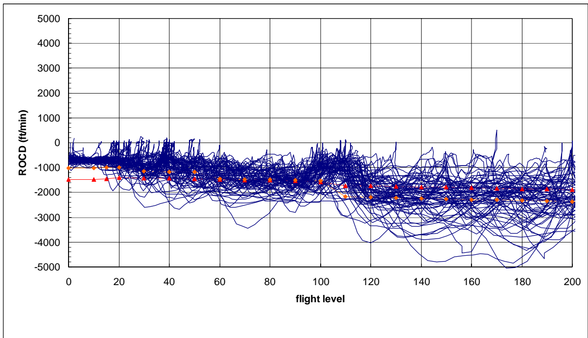
圖 7.40 MD11 型機實際雷達資料下降飛航軌跡、下降率圖
