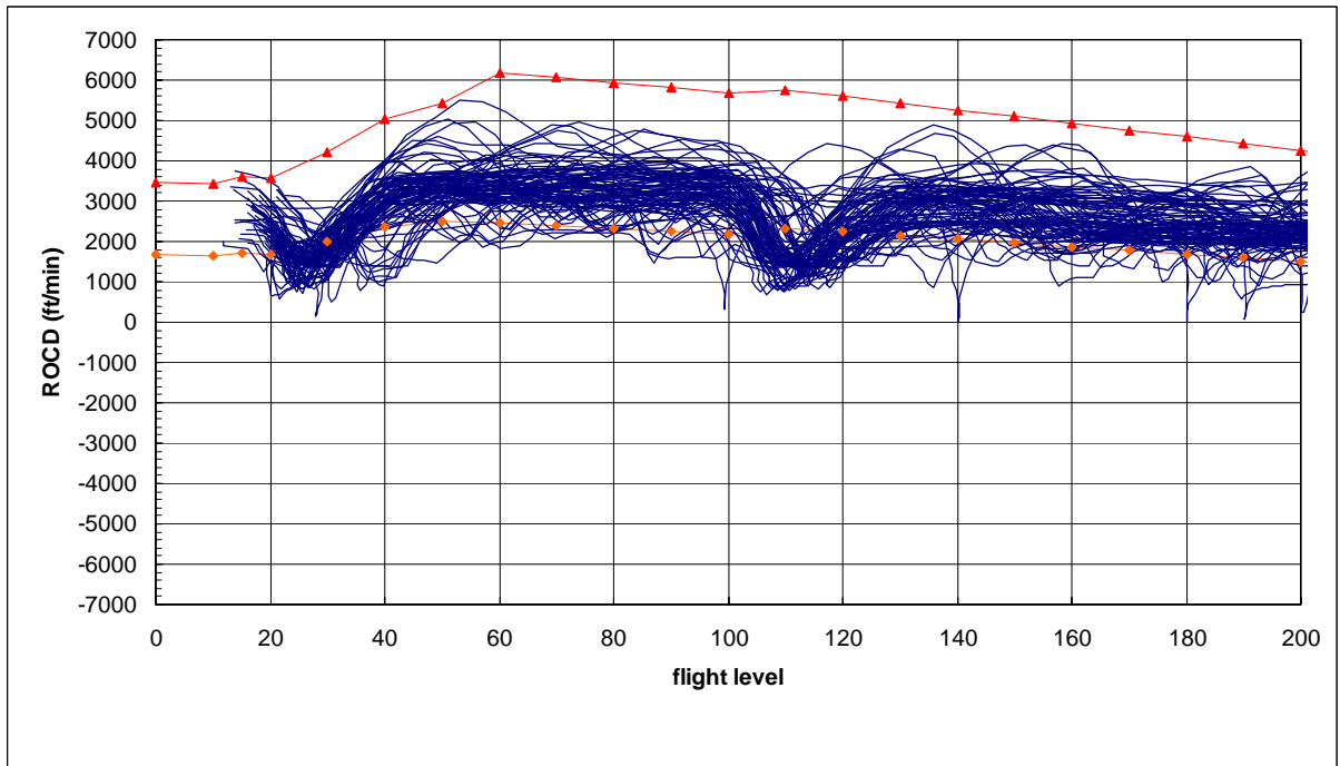
圖 7.21 A306 型機實際雷達資料爬升飛航軌跡、爬升率圖
