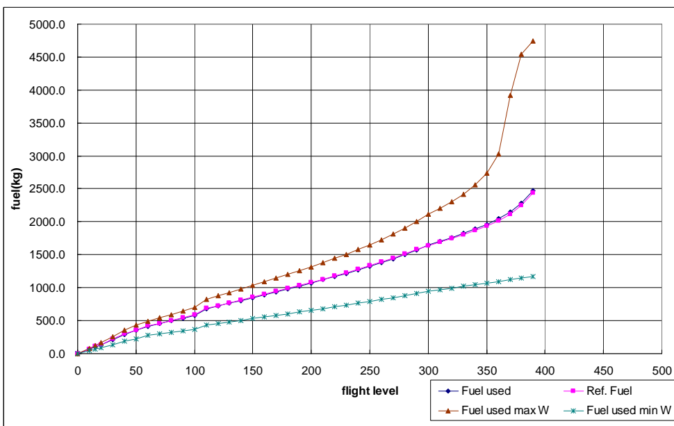
圖 7.3 BADA A321 型機爬升飛航軌跡、爬升率、油耗圖
