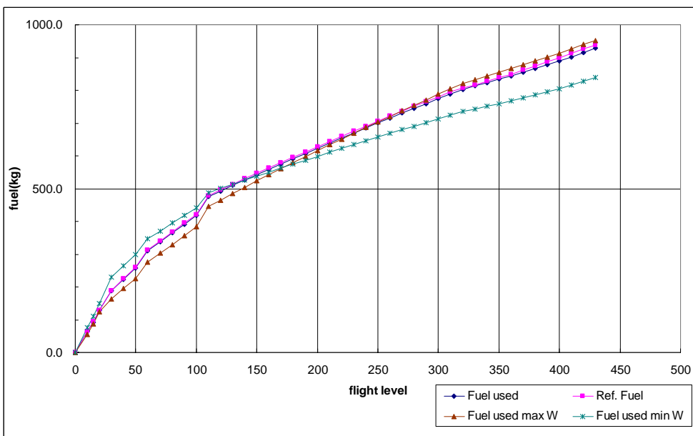
圖 7.18 BADA B777 型機下降飛航軌跡、下降率、油耗圖
