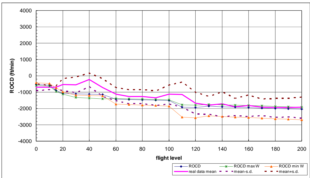
圖 7.50 B738 型機平均下降飛航軌跡、下降率圖(含標準差)
