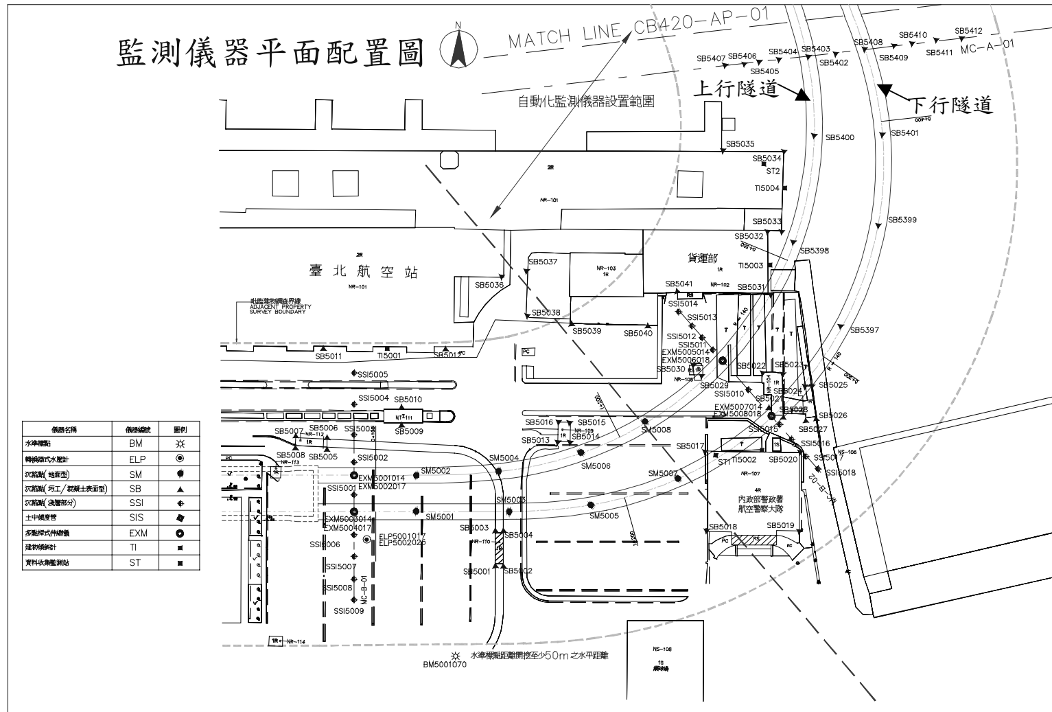
圖 4-17 (d) 監測儀器平面配置圖 (摘自 大陸工程, 2003e)
