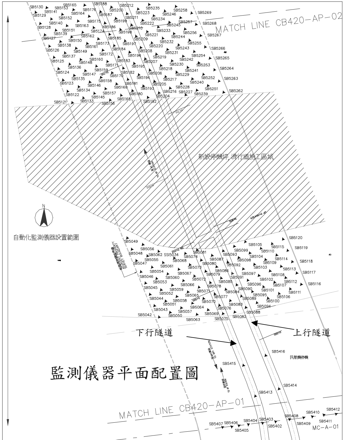
圖 4-17 (c) 監測儀器平面配置圖 (摘自大陸工程, 2003e)
