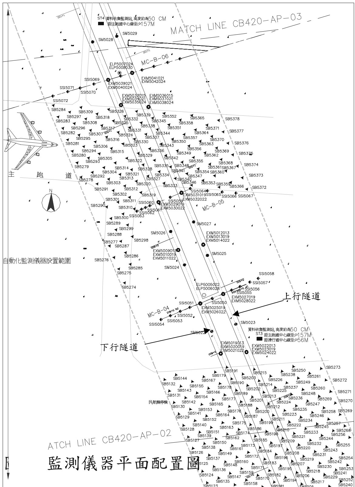
圖 4-17 (b) 監測儀器平面配置圖 (摘自大陸工程, 2003e)
