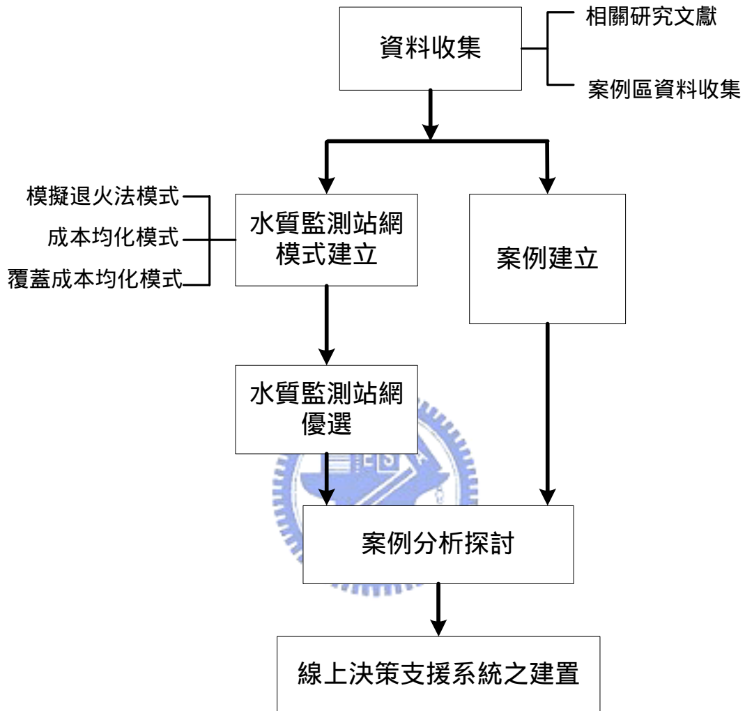
圖 3.1 研究流程圖
