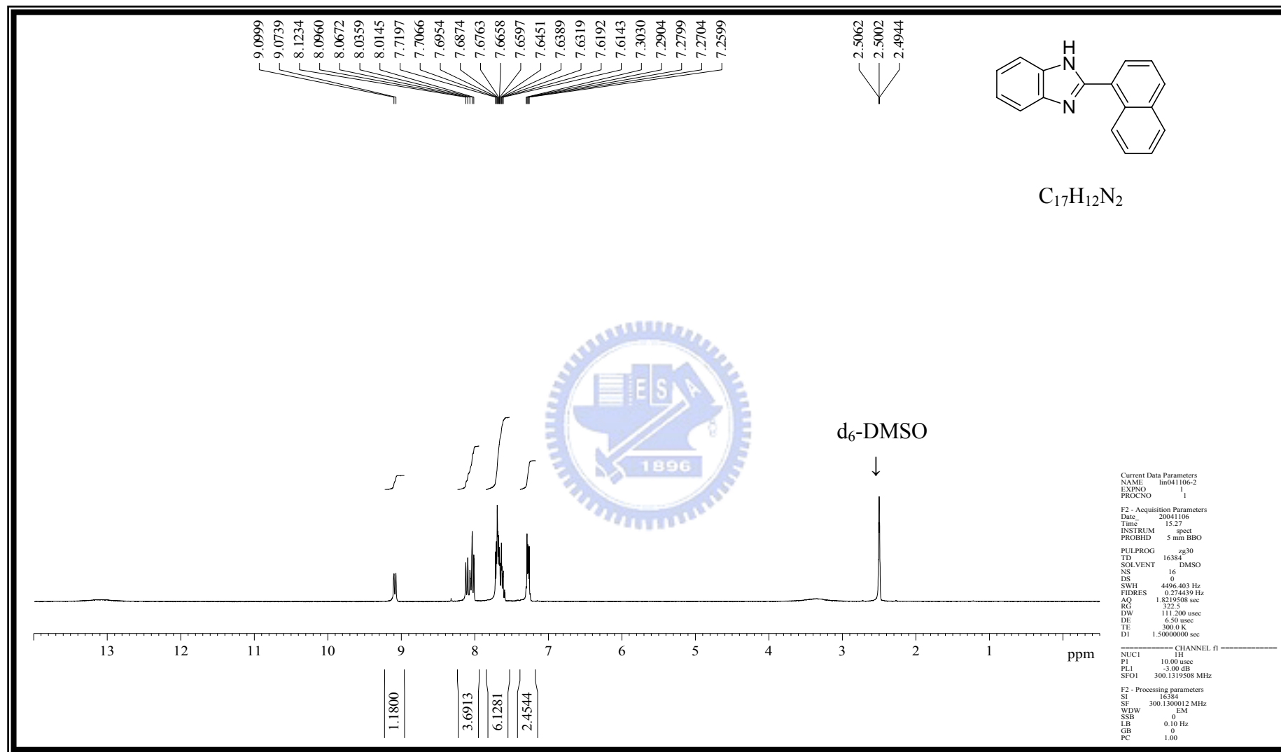
附圖 10 化合物 2-(1-naphthyl)-1H-benzo[d]imidazole, 61 之 ^1H -NMR (300 MHz, d_6 -DMSO) 光譜圖
