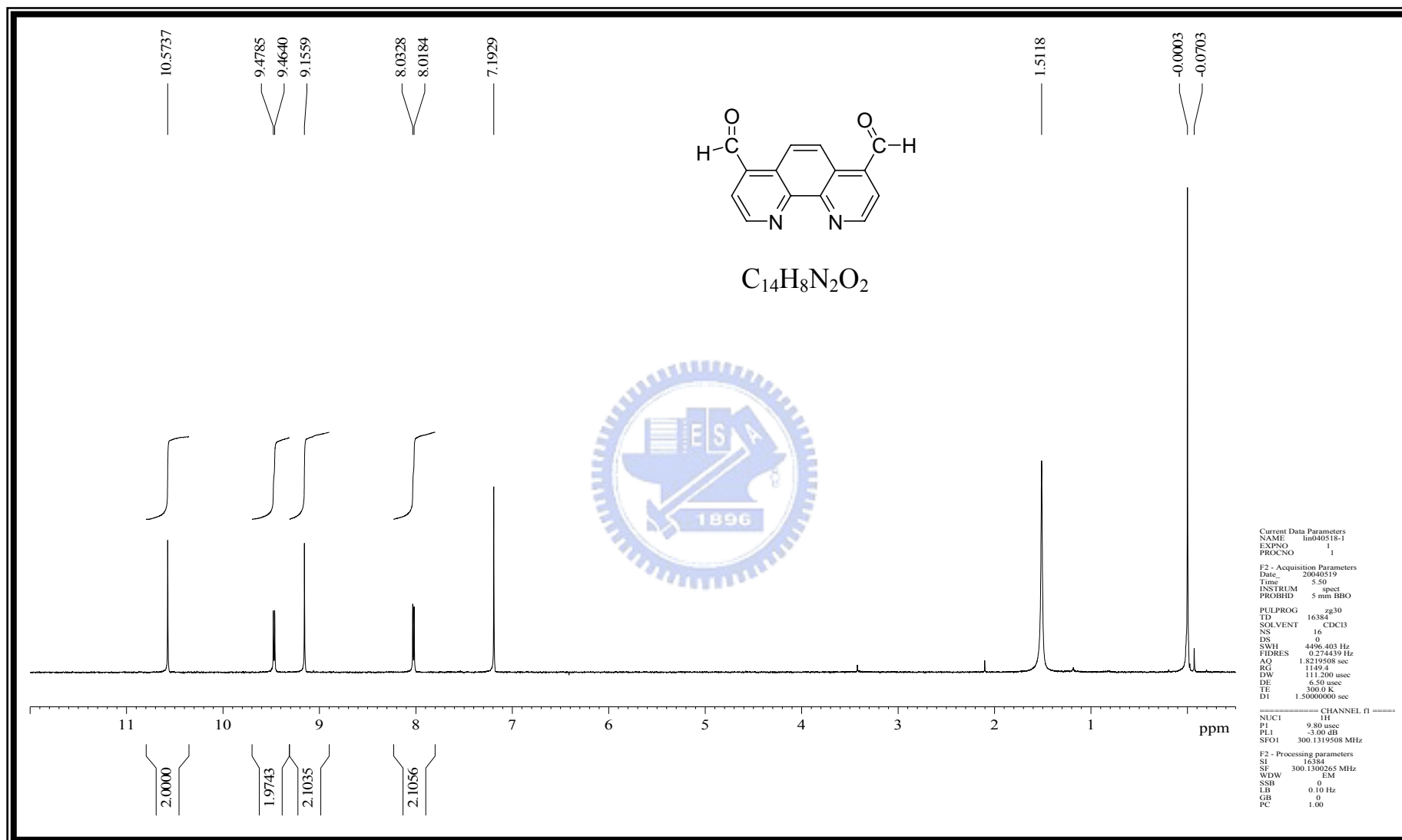
附圖 51 化合物 4,7-diformyl-1,10-phenanthroline, 97 之 ^1\text{H-NMR} (300 MHz, \text{CDCl}_3 ) 光譜圖
