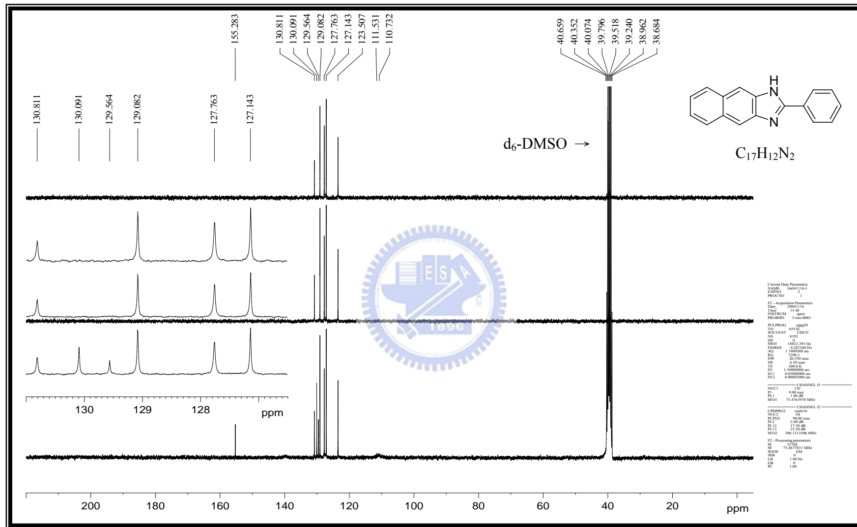
附圖 17 2-phenyl-1 H -naphtho[2,3- d ]imidazole, 63 之 DEPT- ^{13}C -NMR (75 MHz, d_6 -DMSO) 光譜圖
