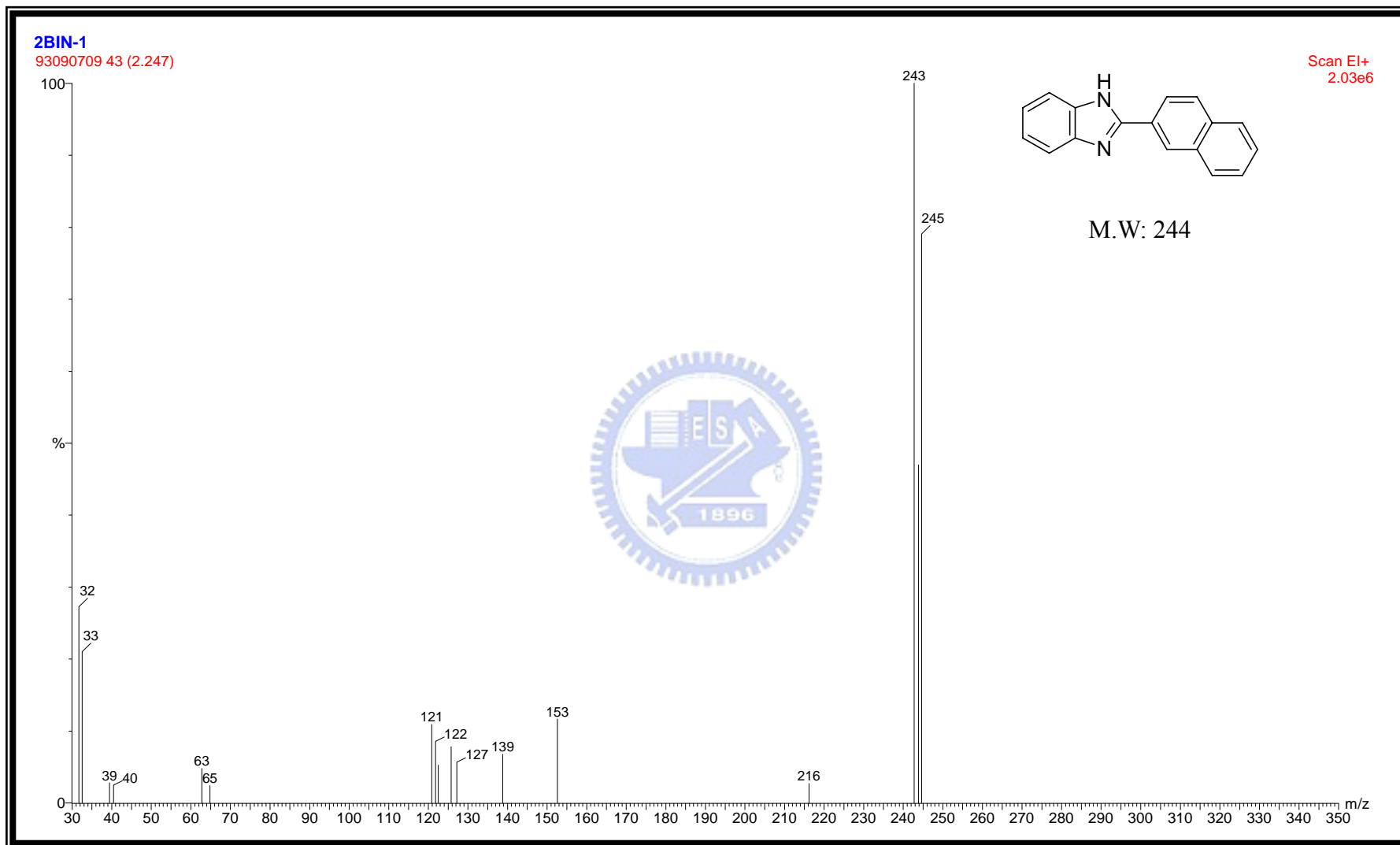
附圖 15 化合物 2-(2-naphthyl)-1H-benzo[d]imidazole, 62 之 EI 質譜圖
