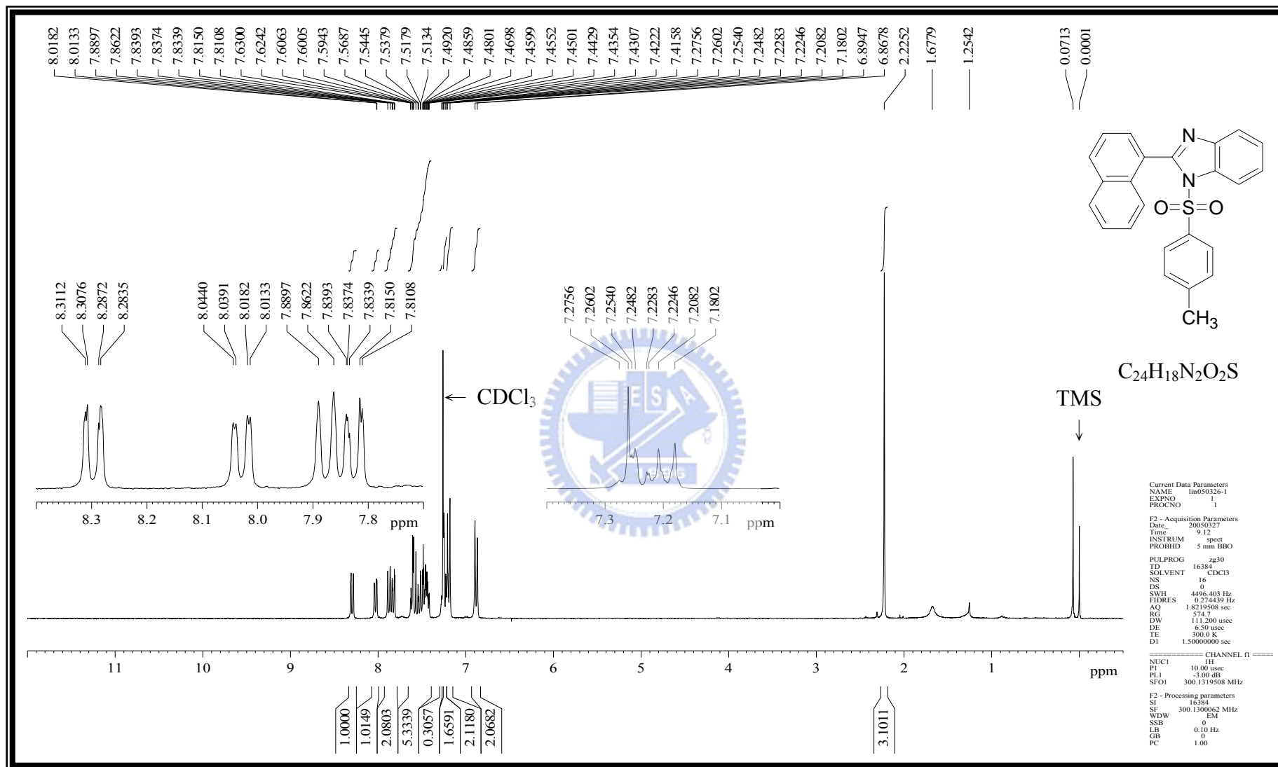
附圖 34 化合物 1-[(4-methylphenyl)sulfonyl]-2-(1-naphthyl)-1H-benzo[d]imidazole, 65 之 ^1\text{H-NMR} (300 MHz, \text{CDCl}_3 ) 光譜圖
