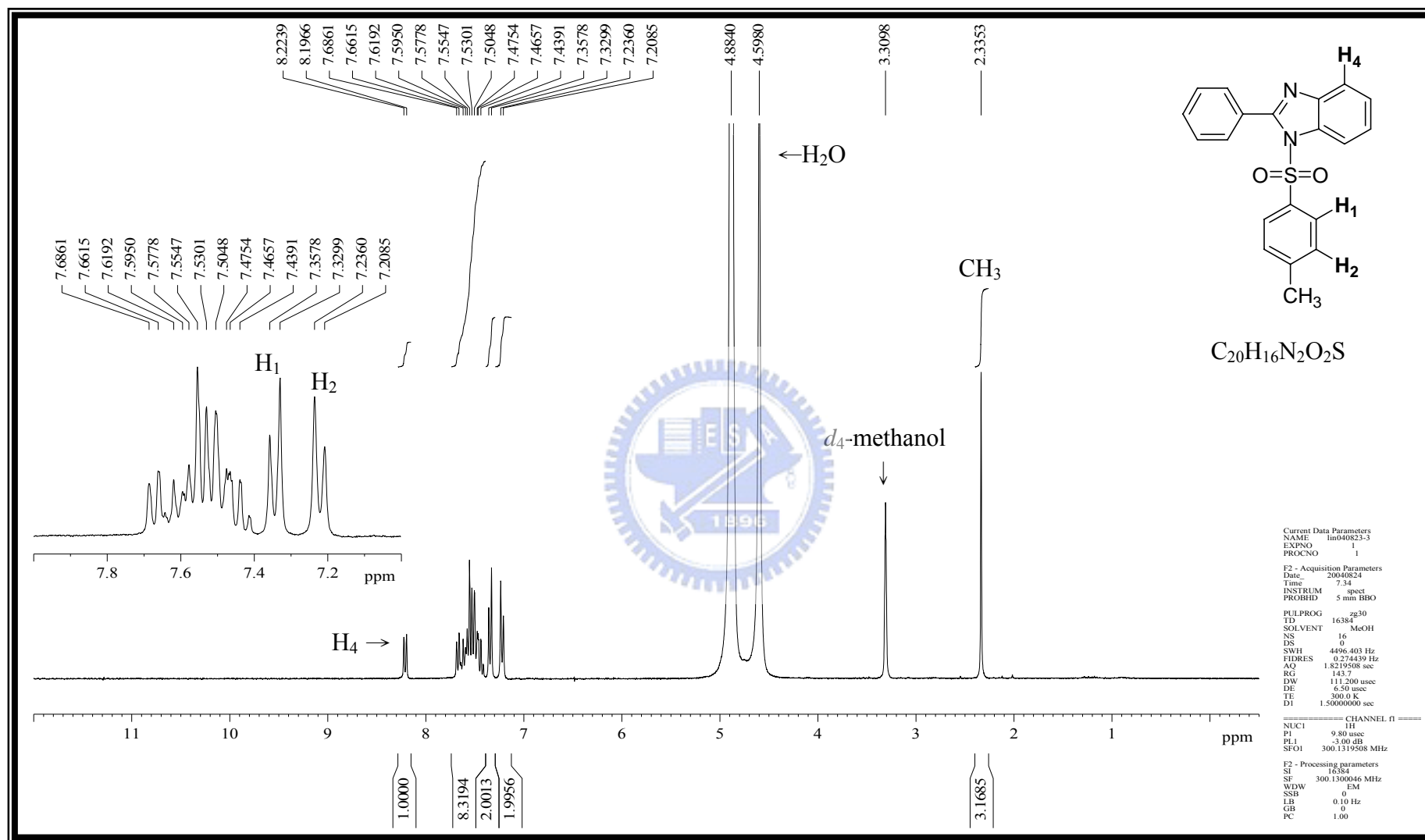
附圖 22 化合物 1-[(4-methylphenyl)sulfonyl]2-phenyl-1H-benzo[d]imidazole, 55 之 ^1\text{H-NMR} (300 MHz, d_4 -methanol) 光譜圖
