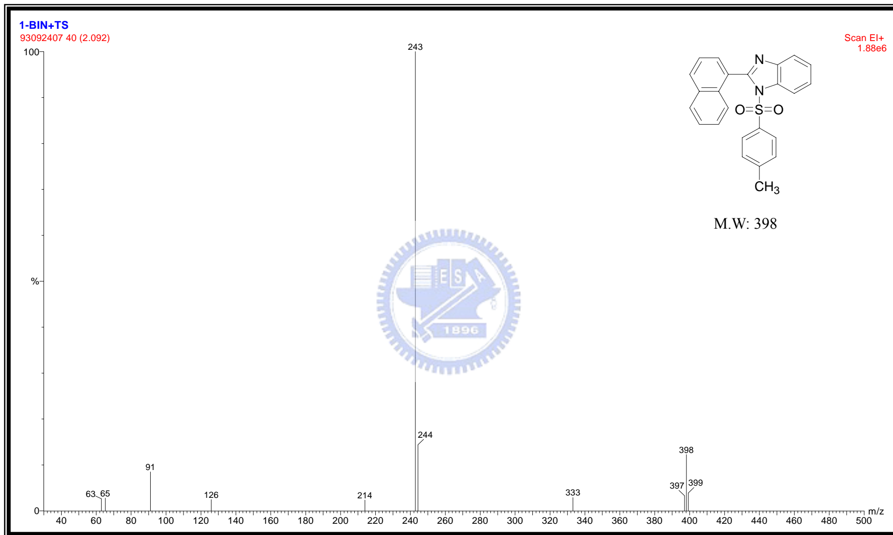
附圖 36 化合物 1-[(4-methylphenyl)sulfonyl]-2-(1-naphthyl)-1H-benzo[d]imidazole, 65 之 EI 質譜圖
