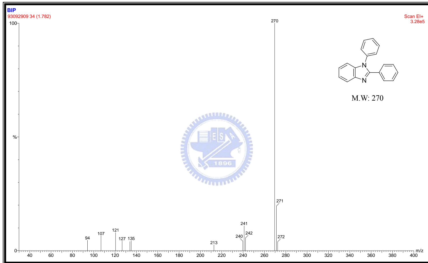
附圖 21 化合物 1,2-diphenyl-1H-benzo[d]imidazol, 64 之 EI 質譜圖
