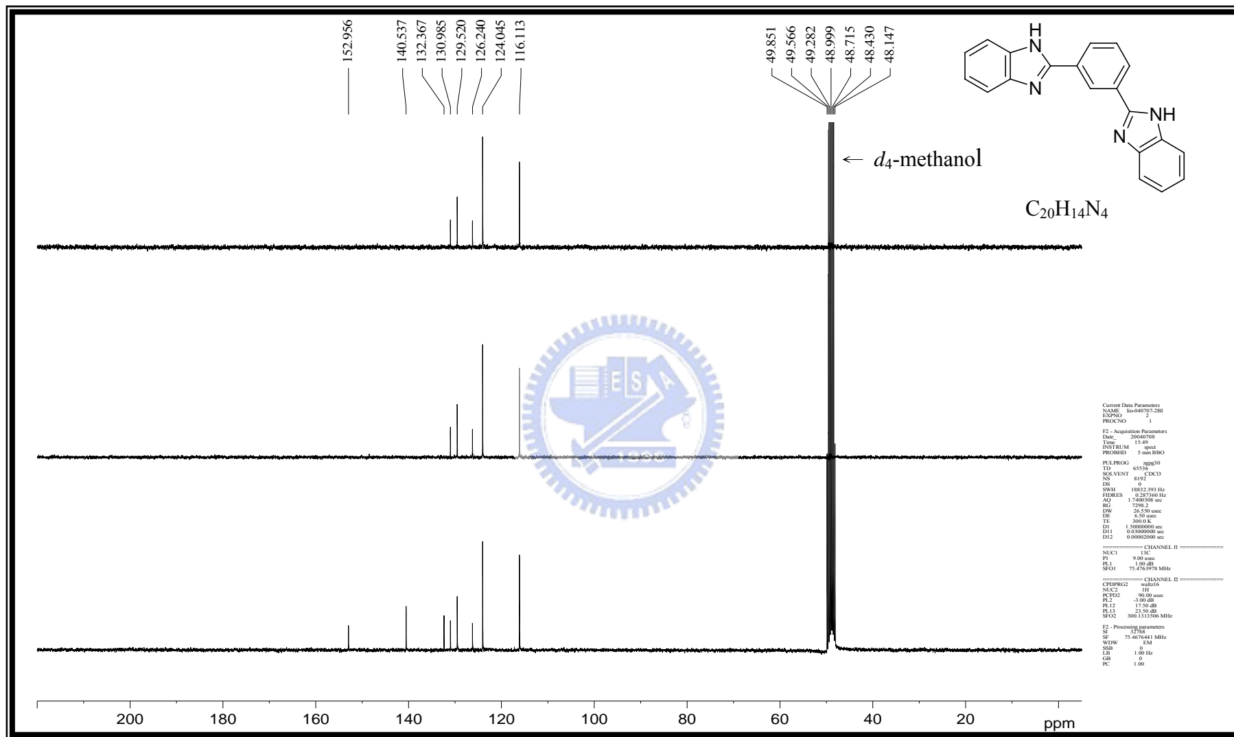
附圖 5 化合物 2-[3-(1H-benzo[d]imidazol-2-yl)phenyl]-1H-benzo[d]imidazole, 59 之 DEPT- ^{13}C -NMR (75 MHz, d_4 -methanol) 光譜圖
