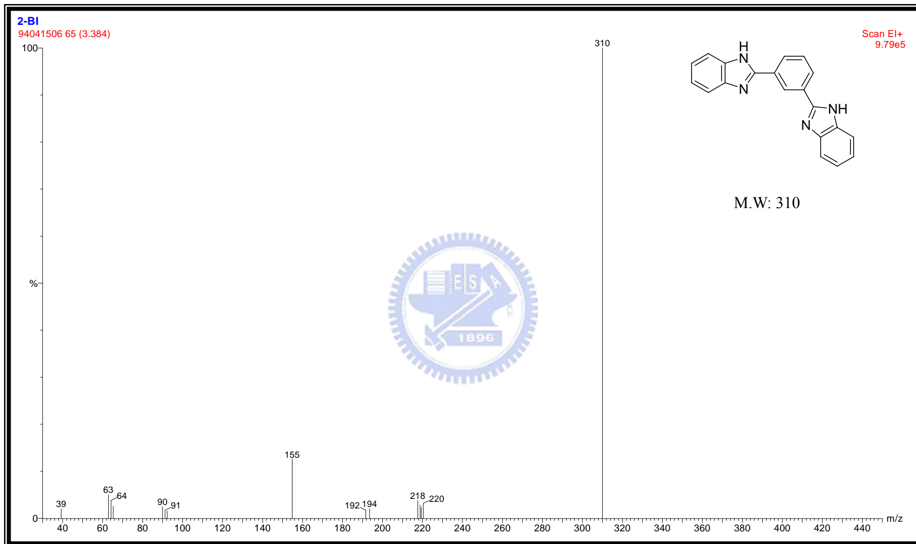
附圖 6 化合物 2-[3-(1 H -benzo[ d ]imidazol-2-yl)phenyl]-1 H -benzo[ d ]imidazole, 59 之 EI 質譜圖
