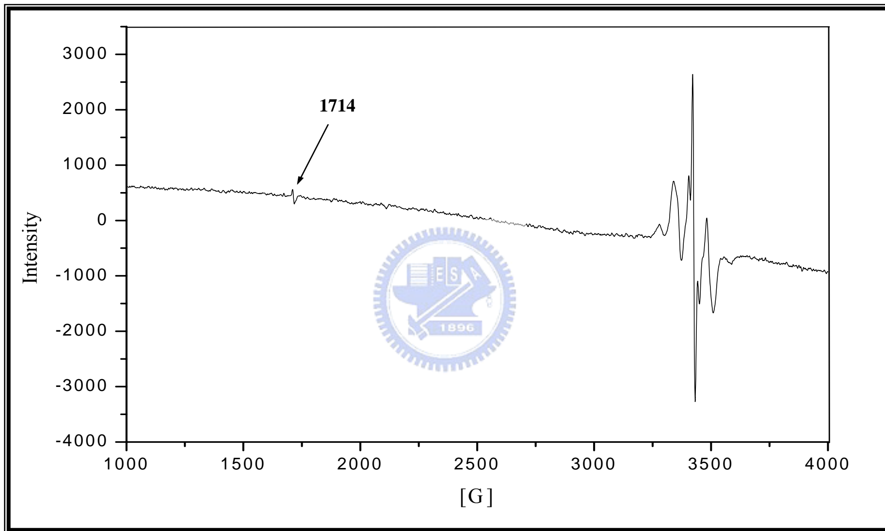
附圖 54 化合物 1-[(4-methylphenyl)sulfonyl]2-phenyl-1 H -benzo[ d ]imidazole, 55 照光後之 77 K EPR 光譜全圖
