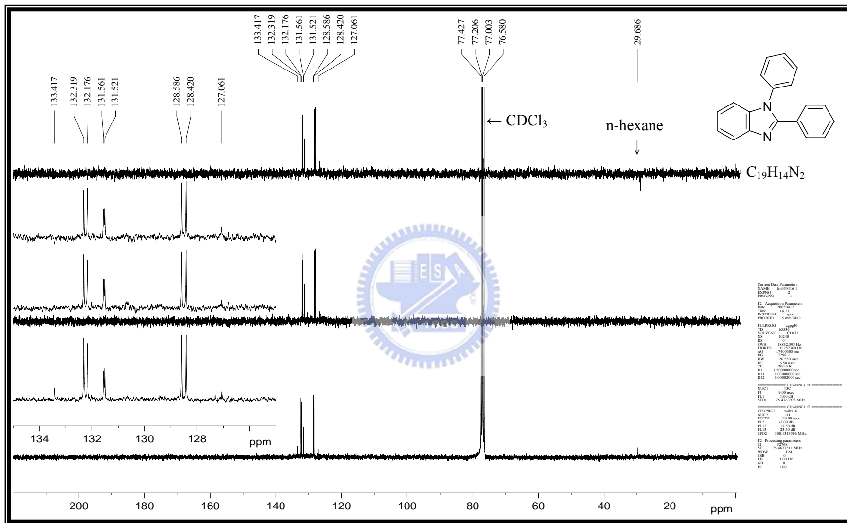
附圖 20 化合物 1,2-diphenyl-1H-benzo[d]imidazole, 64 之 DEPT- ^{13}C -NMR (75 MHz, CDCl_3 ) 光譜圖
