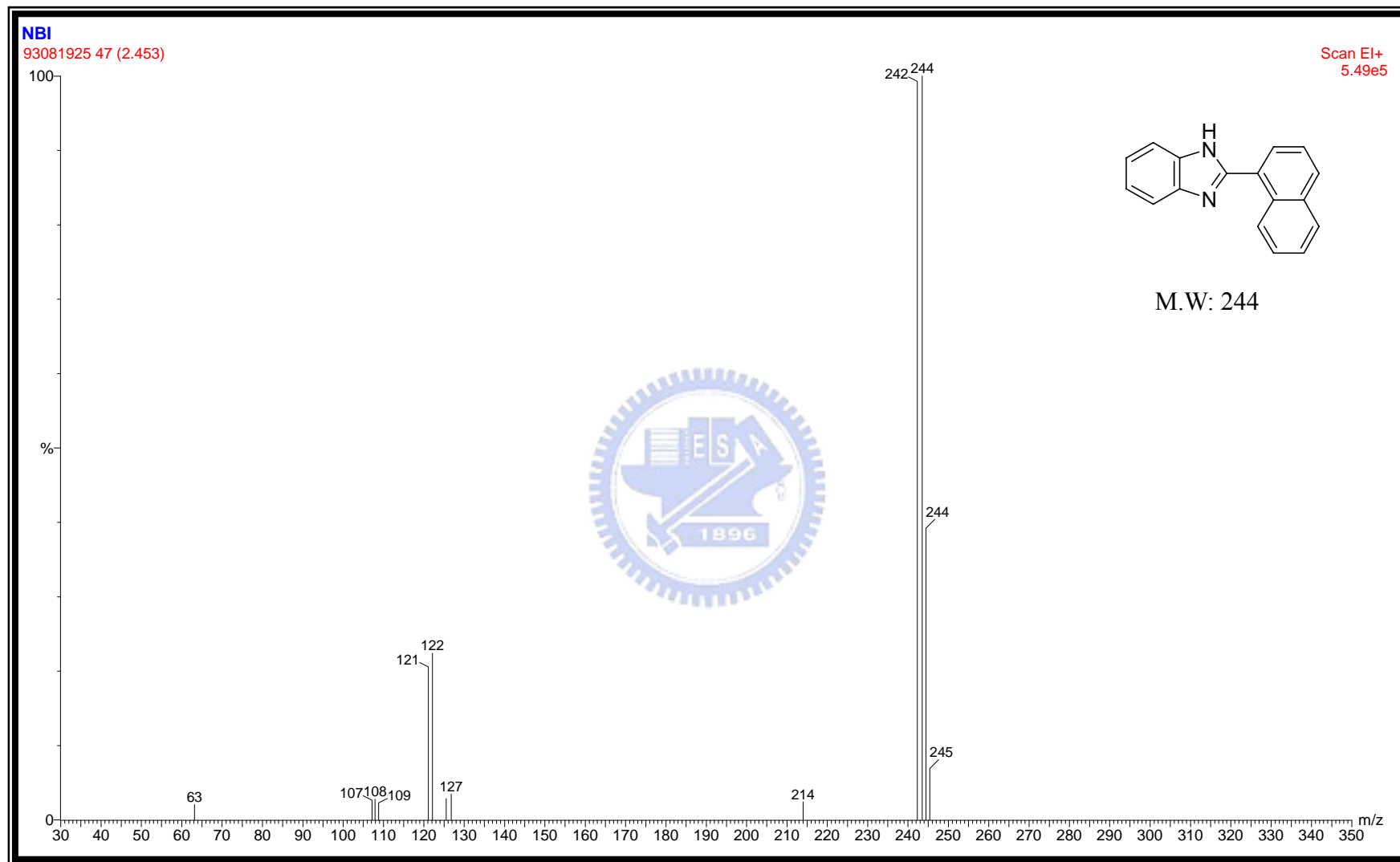
附圖 12 化合物 2-(1-naphthyl)-1H-benzo[d]imidazole, 61 之 EI 質譜圖
