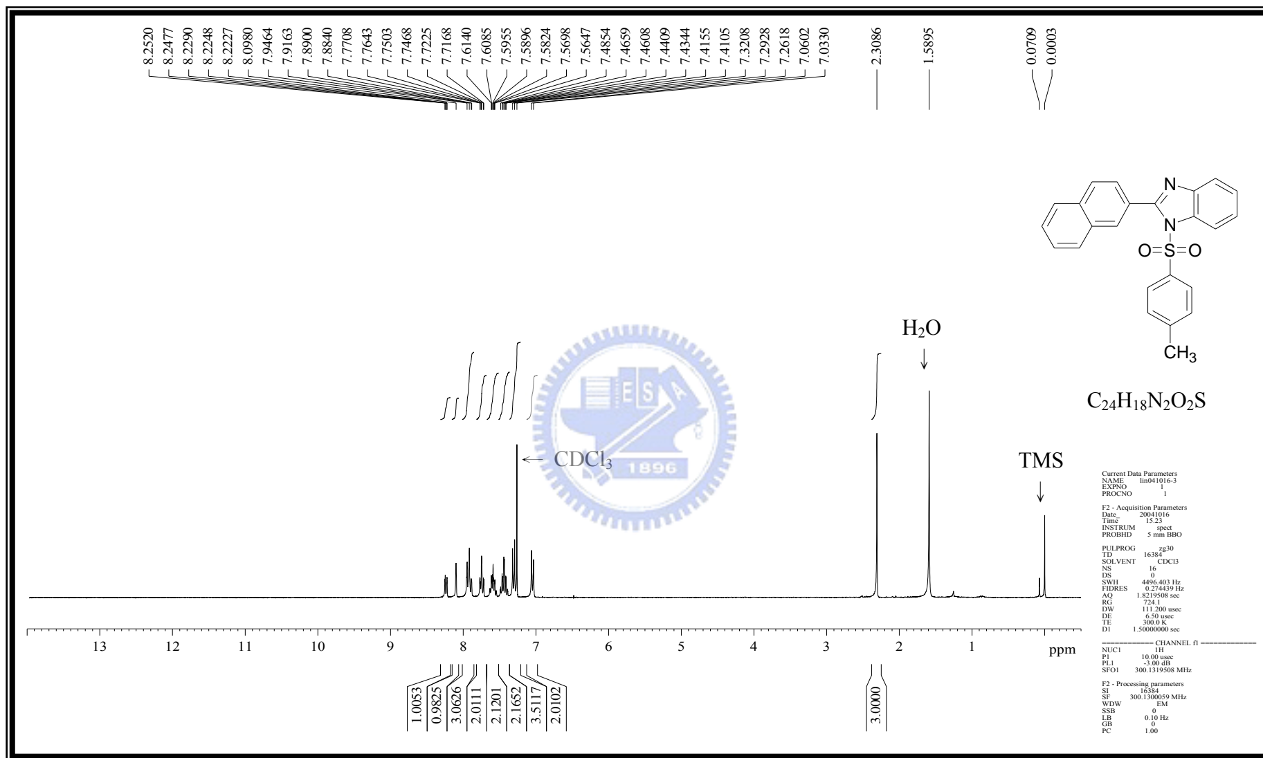
附圖 37 化合物 1-[(4-methylphenyl)sulfonyl]-2-(2-naphthyl)-1H-benzo[d]imidazole, 66 之 1 H-NMR (300 MHz, CDCl 3 ) 光譜圖
