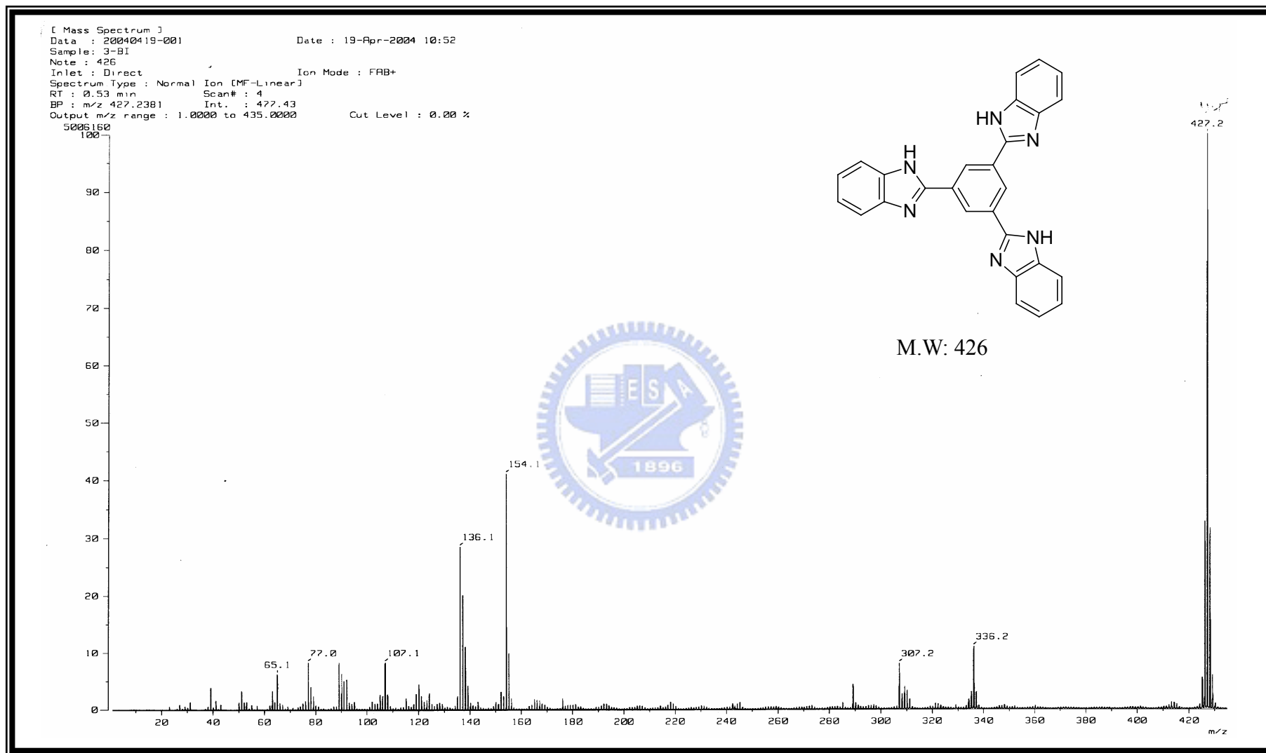
附圖 9 化合物 2-[3,5-di(1H-benzo[d]imidazol-2-yl)phenyl]-1H-benzo[d]-imidazole, 60 之 FAB 質譜圖
