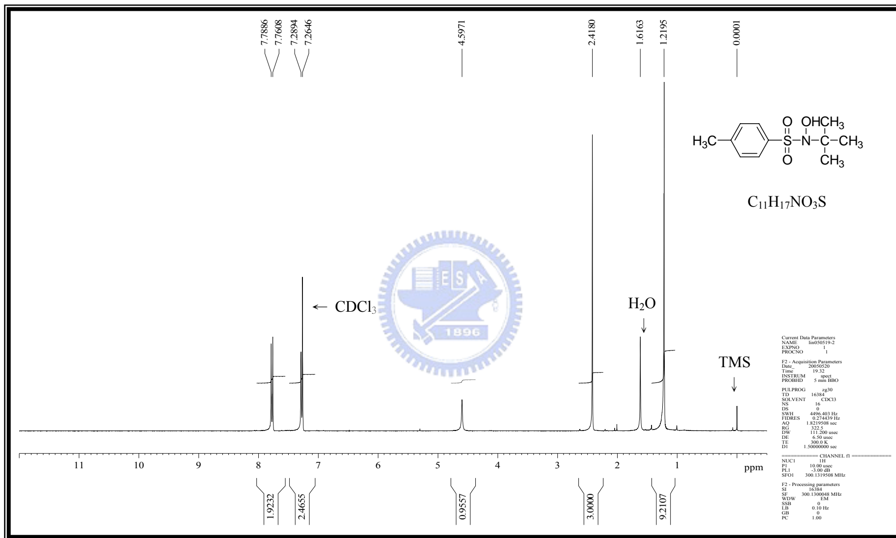
附圖 46 化合物 1-[(4-methylphenyl)sulfonyl]- N -( tert -butyl) hydroxylamine, Ts-MNP 之 ^1\text{H-NMR} (300 MHz, \text{CDCl}_3 ) 光譜圖
