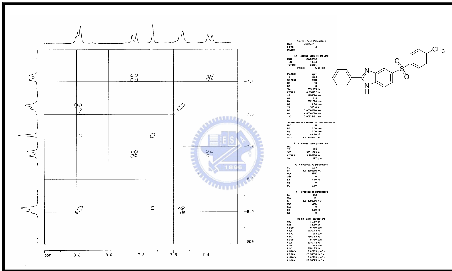
附圖 44 化合物 5-[(4-methylphenyl)sulfonyl]-2-phenyl-1H-benzo[d]imidazole, 73 之 H,H-COSY-NMR (300 MHz, d_6 -DMSO) 光譜圖
