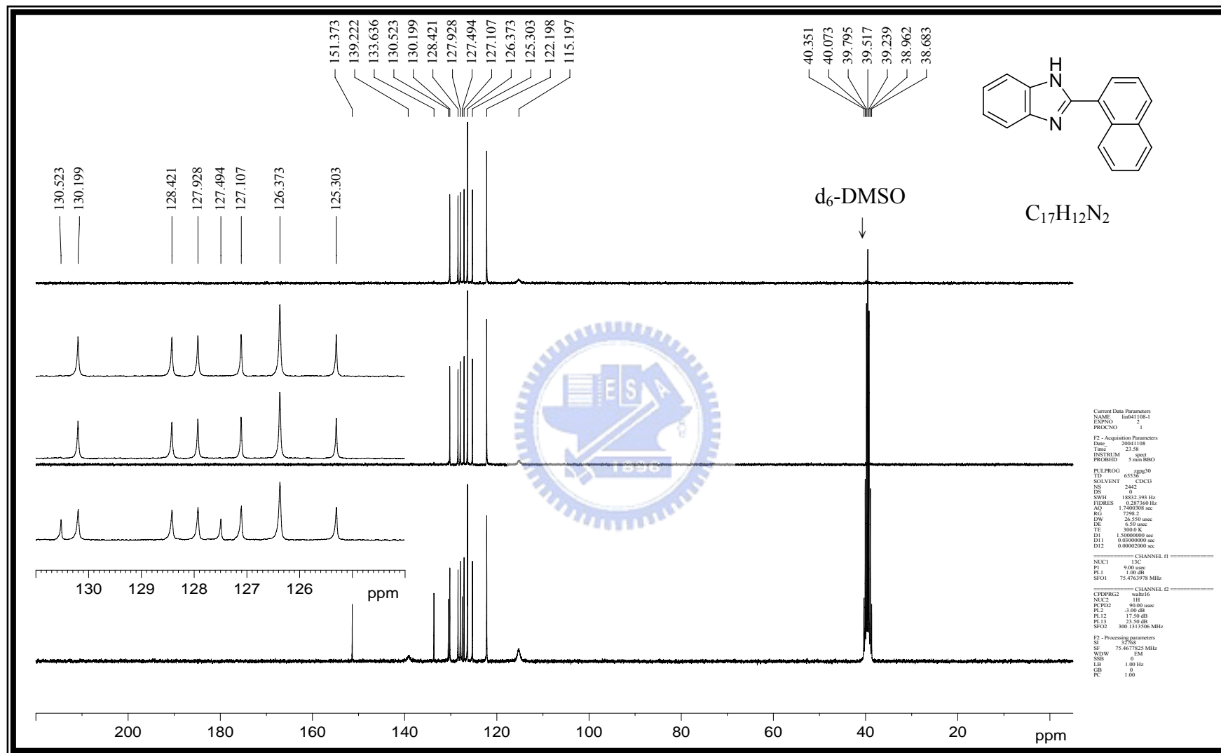
附圖 11 化合物 2-(1-naphthyl)-1H-benzo[d]imidazole, 61 之 DEPT- ^{13}C -NMR (75 MHz, d_6 -DMSO) 光譜圖
