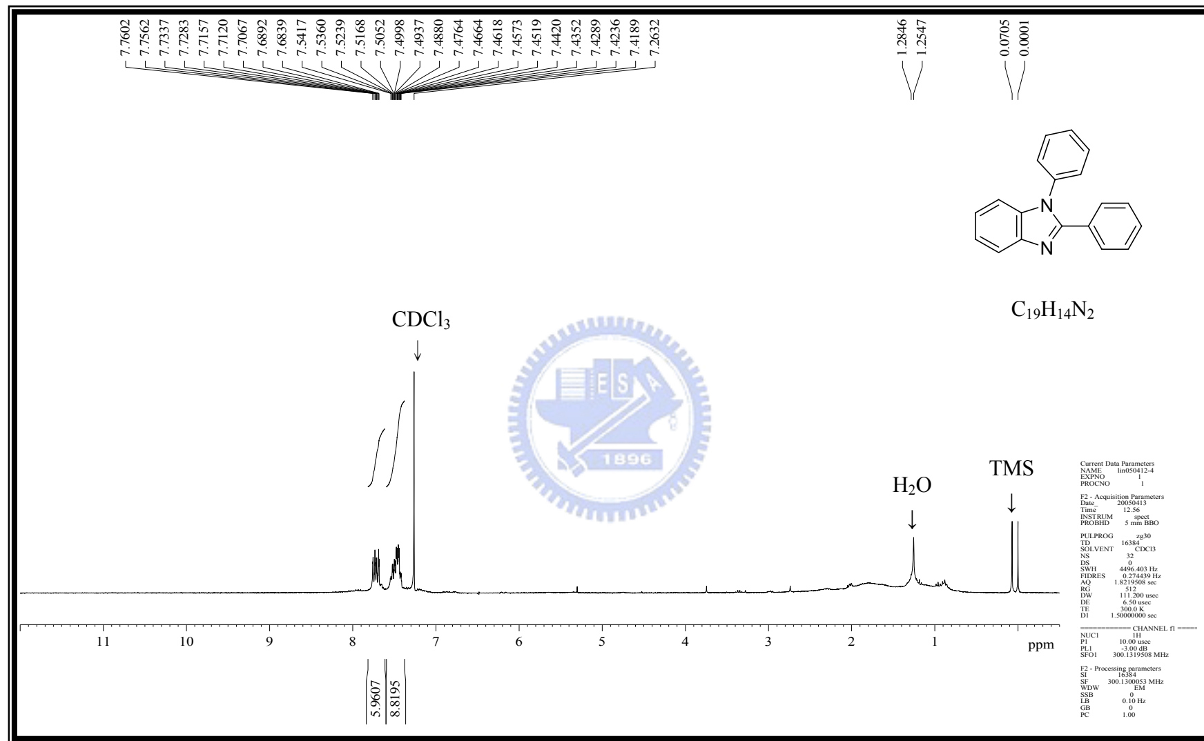
附圖 19 化合物 1,2-diphenyl-1H-benzo[d]imidazole, 64 之 1 H-NMR (300 MHz, CDCl 3 ) 光譜圖
