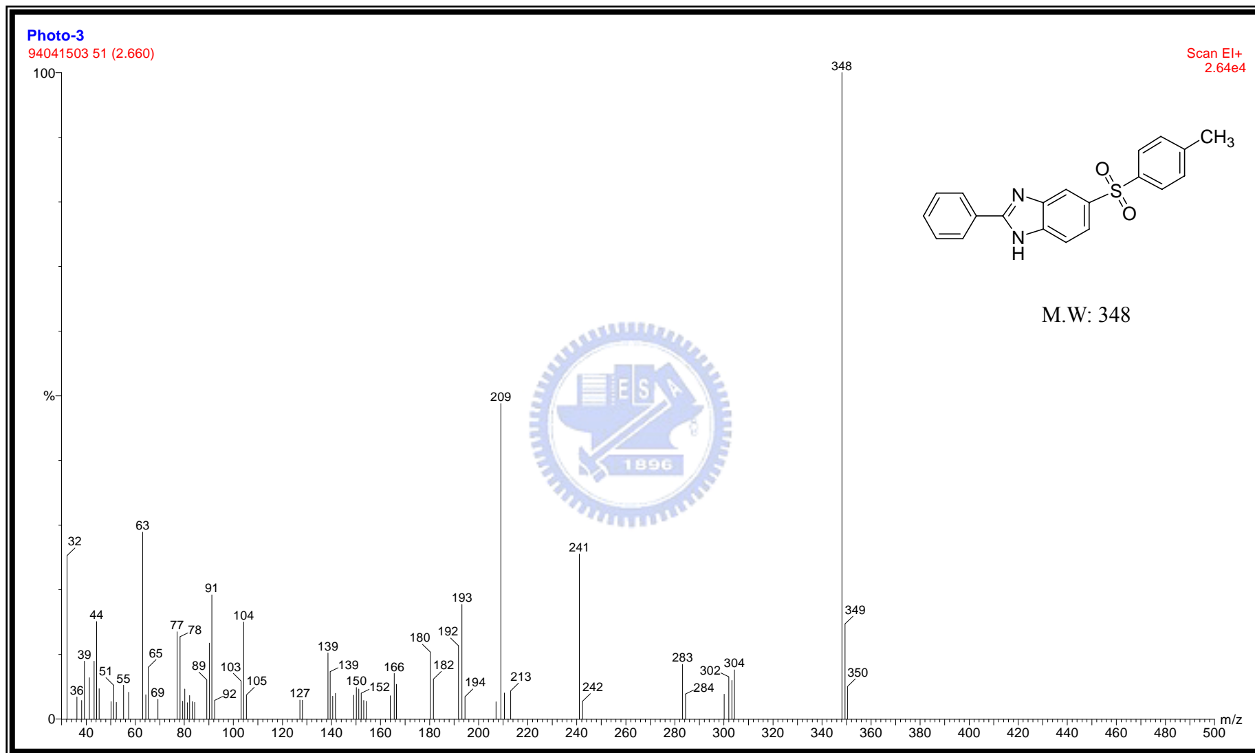
附圖 45 化合物 5-[(4-methylphenyl)sulfonyl]-2-phenyl-1H-benzo[d]imidazole, 73 之 EI 質譜圖
