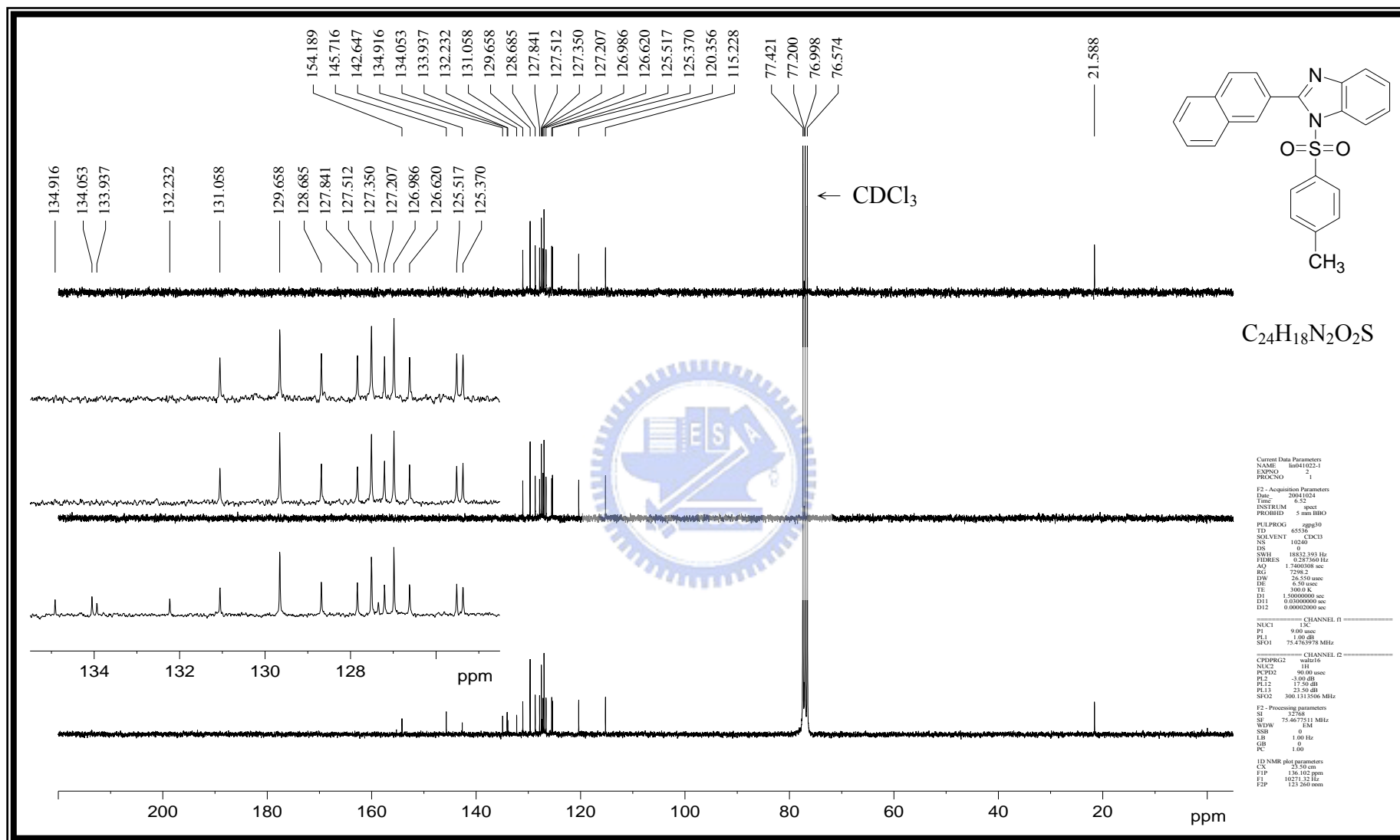
附圖 39 化合物 1-[(4-methylphenyl)sulfonyl]-2-(2-naphthyl)-1H-benzo[d]imidazole, 66 之 DEPT- ^{13}C -NMR (75 MHz, CDCl_3 ) 光譜圖
