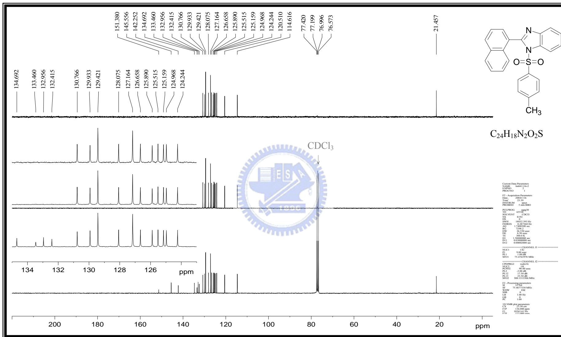
附圖 35 化合物 1-[(4-methylphenyl)sulfonyl]-2-(1-naphthyl)-1H-benzo[d]imidazole, 65 之 DEPT- ^{13}C -NMR (75 MHz, CDCl_3 ) 光譜圖
