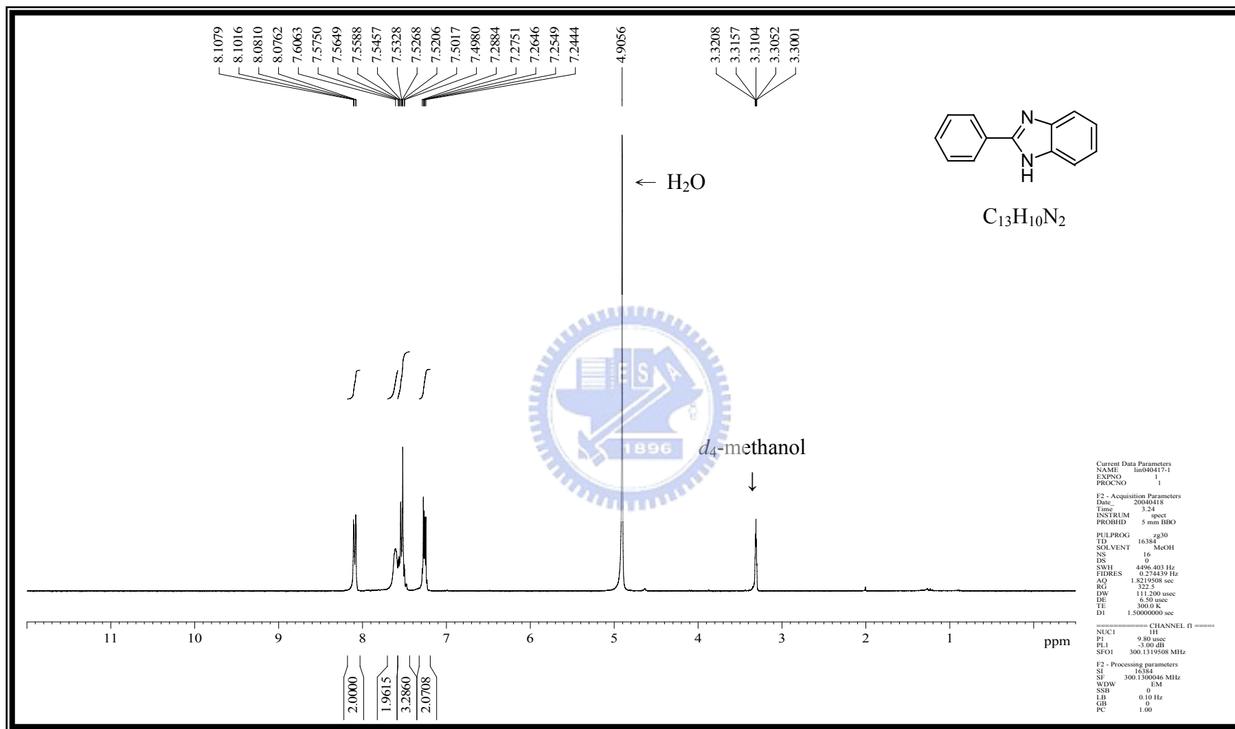
附圖 1 化合物 2-phenyl-1H-benzo[d]imidazole, 58 之 ^1\text{H-NMR} (300 MHz, d_4 -methanol) 光譜圖
