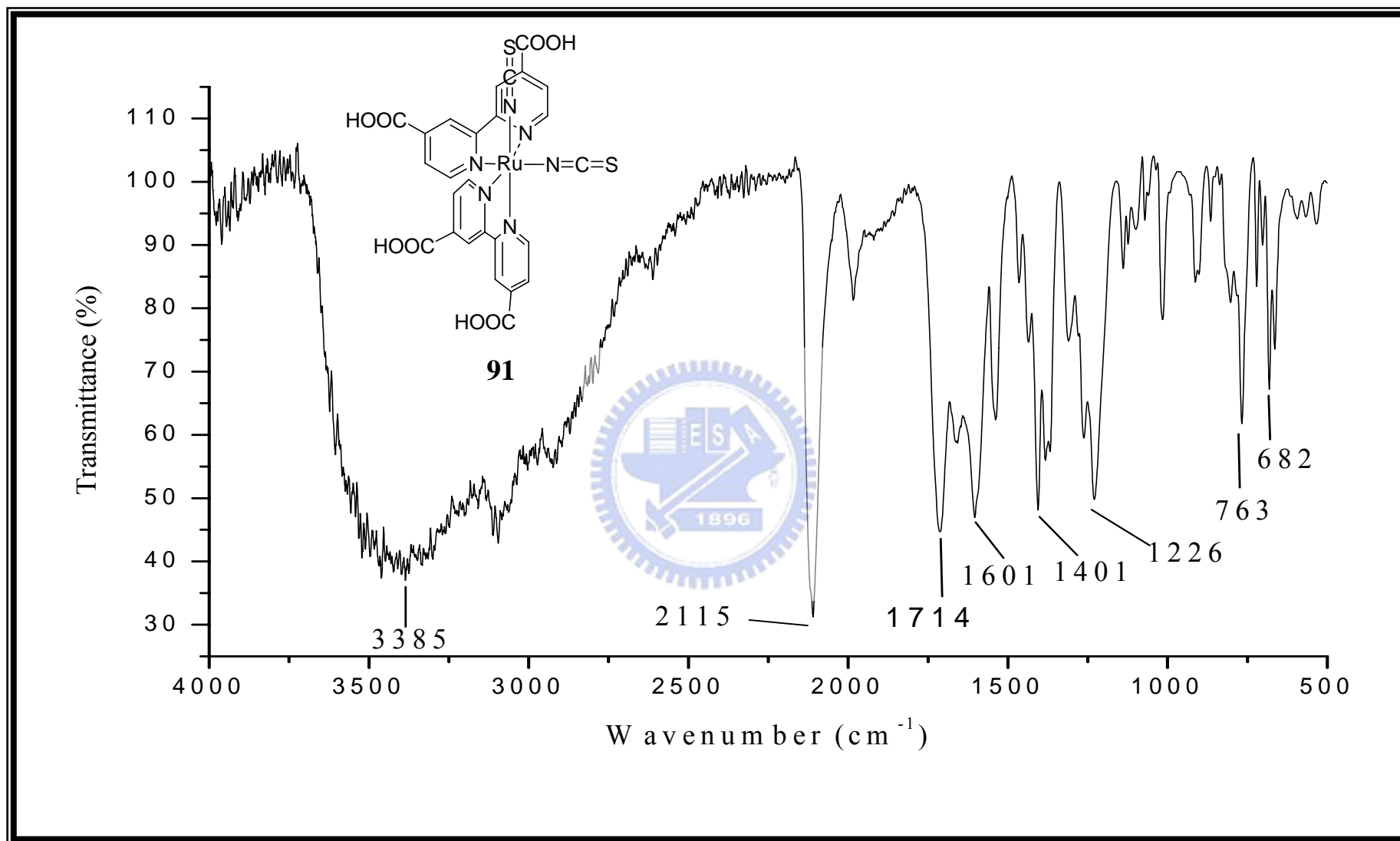
附圖 50 化合物 cis -di(thiocynato)bis(2,2'-bipyridyl-4,4'-dicarboxylate)ruthenium (II), 91 之 IR 光譜圖
