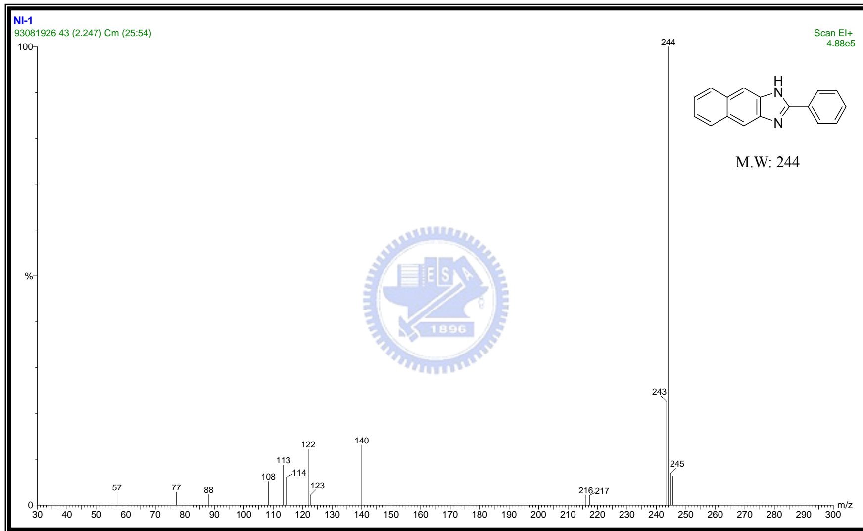
附圖 18 2-phenyl-1 H -naphtho[2,3- d ]imidazole, 63 之 EI 質譜圖
