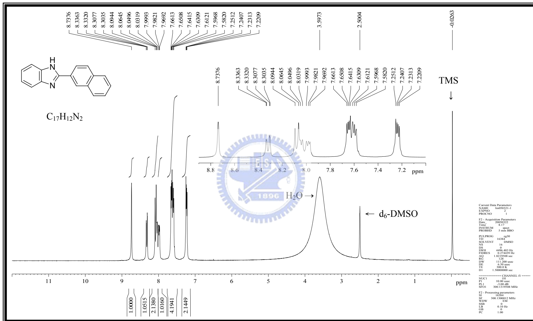
附圖 13 化合物 2-(2-naphthyl)-1H-benzo[d]imidazole, 62 之 ^1\text{H-NMR} (300 MHz, d_6 -DMSO) 光譜圖
