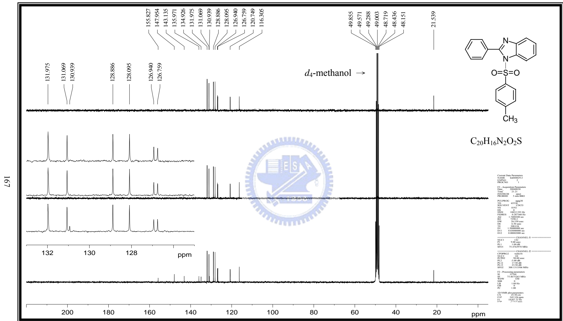
附圖 24 化合物 1-[(4-methylphenyl)sulfonyl]-2-phenyl-1H-benzo[d]imidazole, 55 之 DEPT- ^{13}C -NMR (75 MHz, d_4 -methanol) 光譜圖
