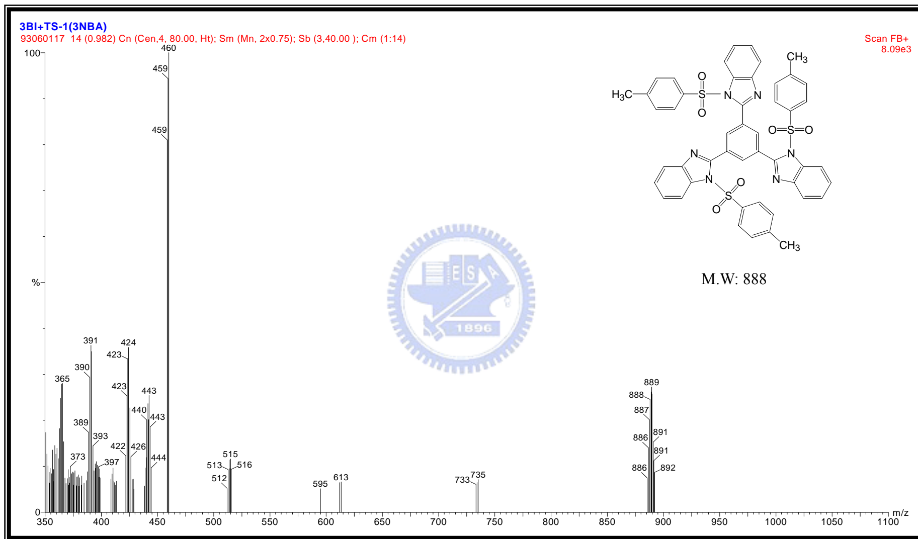
附圖 33 化合物 2-(3,5-di{1-[(4-methylphenyl)sulfonyl]-1 H -benzo[ d ]imidazol-2-yl }-phenyl)-1-[(4-methylphenyl)sulfonyl]-1 H -benzo[ d ]imidazole, 57 之 FAB 質譜圖
