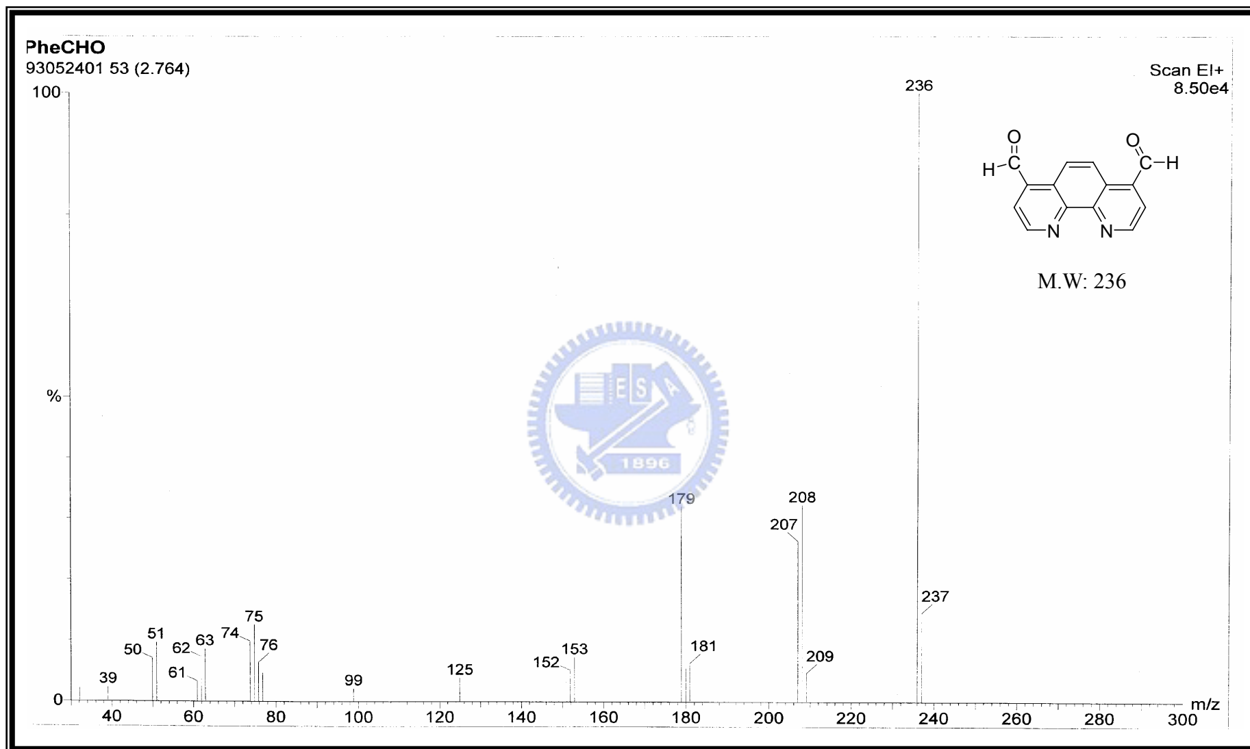
附圖 53 化合物 4,7-diformyl-1,10-phenanthroline, 97 之 EI 質譜圖
