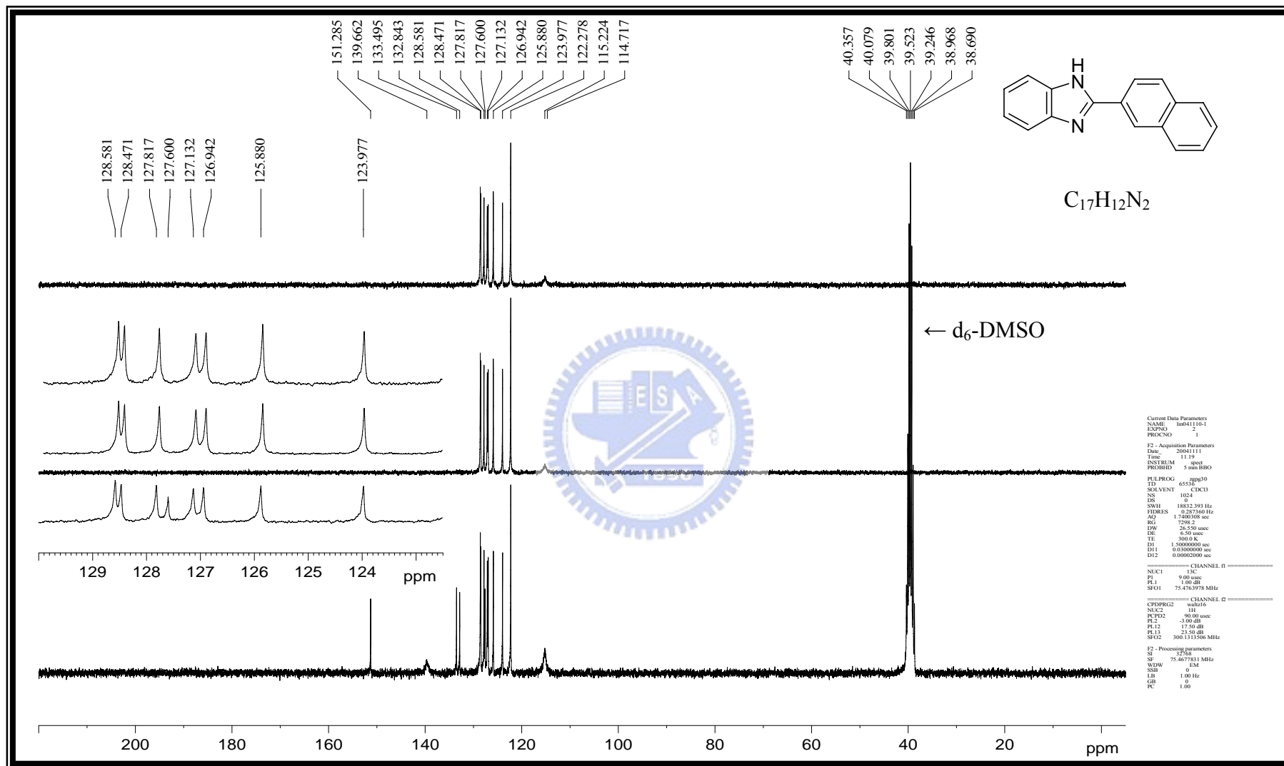
附圖 14 化合物 2-(2-naphthyl)-1H-benzo[d]imidazole, 62 之 DEPT- ^{13}C -NMR (75 MHz, d_6 -DMSO) 光譜圖
