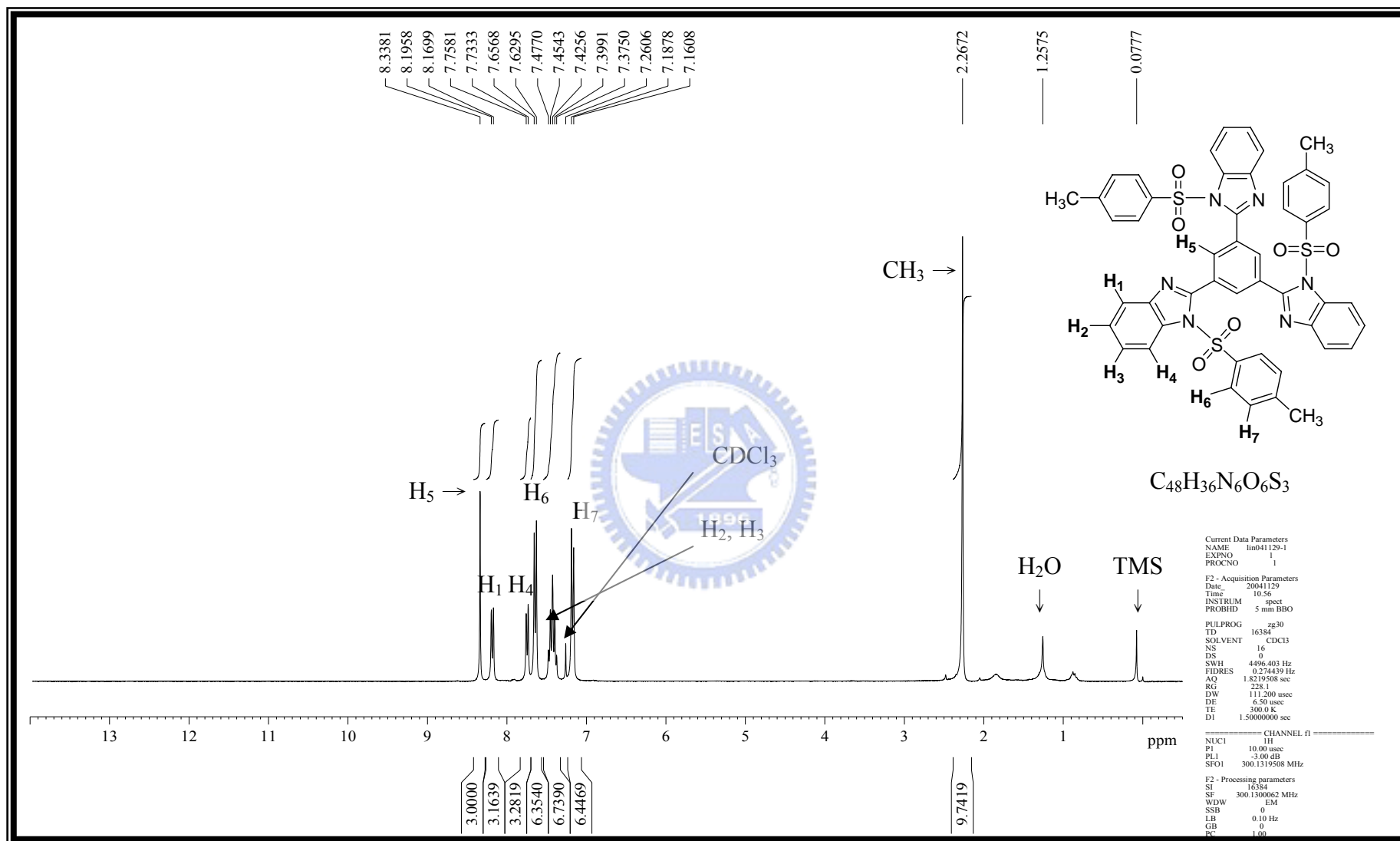
附圖 30 化合物 2-(3,5-di{1-[(4-methylphenyl)sulfonyl]-1 H -benzo[ d ]imidazol-2-yl }-phenyl)-1-[(4-methylphenyl)-sulfonyl]-1 H -benzo[ d ]imidazole, 57 之 1 H-NMR (300 MHz, CDCl 3 ) 光譜圖
