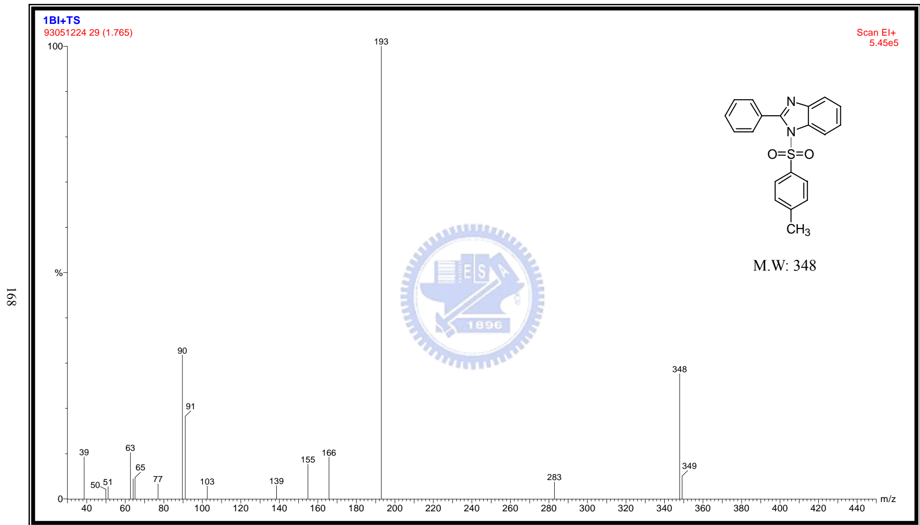
附圖 25 化合物 1-[(4-methylphenyl)sulfonyl]2-phenyl-1H-benzo[d]imidazole, 55 之 EI 質譜圖
