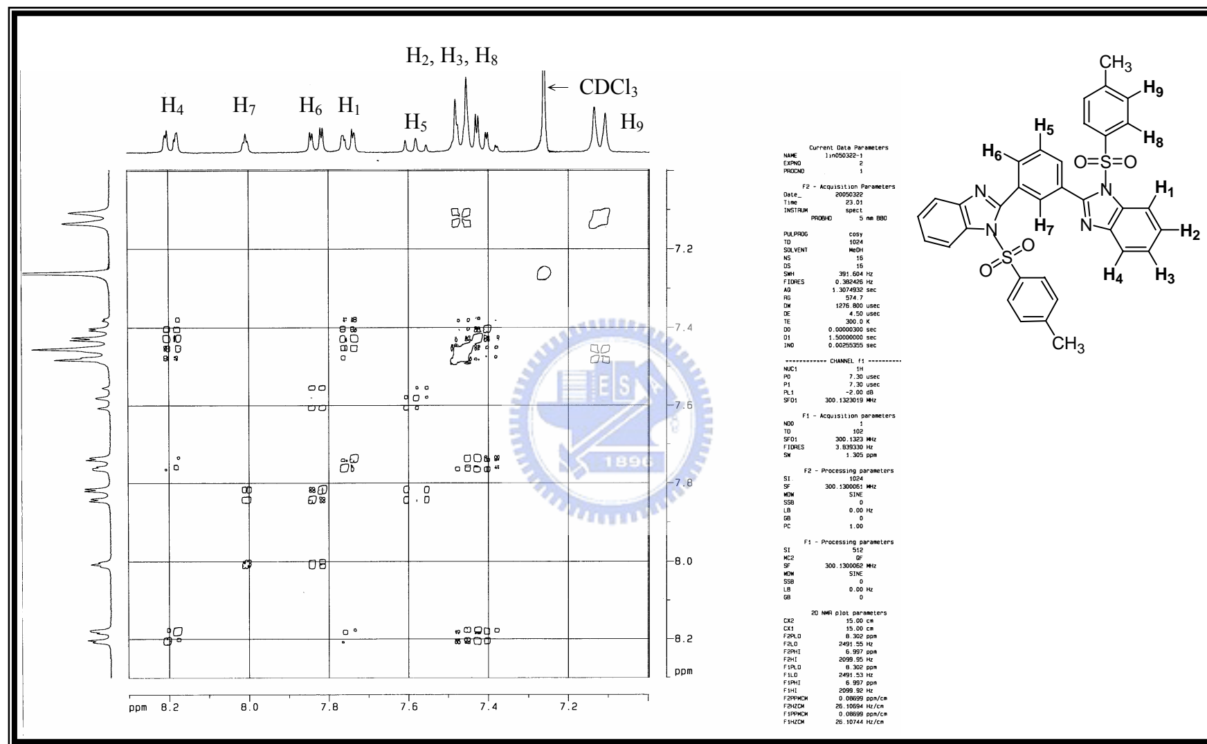
附圖 27 化合物 1-[4-methylphenylsulfonyl]-2-(3-{1-[4-methylphenylsulfonyl]-1 H -benzo[ d ]imidazol-2-yl}phenyl)-1 H -benzo[ d ]imidazole, 56 之 H,H-COSY-NMR (300 MHz, CDCl 3 ) 光譜圖
