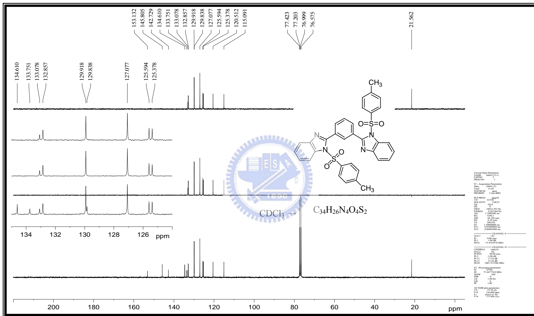
附圖 28 化合物 1-[(4-methylphenyl)sulfonyl]-2-(3-{1-[(4-methylphenyl)sulfonyl]-1 H -benzo[ d ]imidazol-2-yl}phenyl)-1 H -benzo[ d ]imidazole, 56 之 DEPT- ^{13}\text{C} -NMR (75 MHz, \text{CDCl}_3 ) 光譜圖
