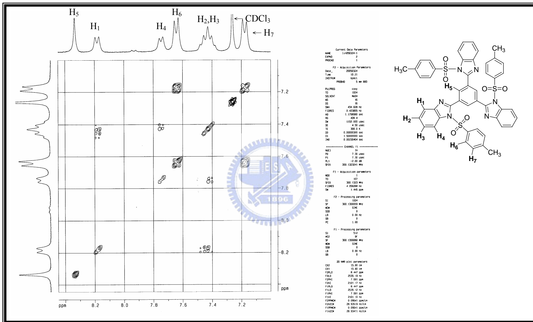
附圖 31 化合物 2-(3,5-di{1-[(4-methylphenyl)sulfonyl]-1 H -benzo[ d ]imidazol-2-yl }-phenyl)-1-[(4-methylphenyl)-sulfonyl]-1 H -benzo[ d ]imidazole, 57 之 H,H-COSY-NMR (300 MHz, CDCl 3 ) 光譜圖
