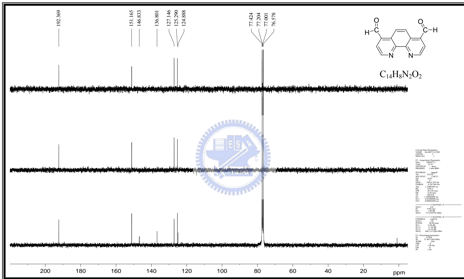
附圖 52 化合物 4,7-diformyl-1,10-phenanthroline, 97 之 DEPT- ^{13}C -NMR (75 MHz, CDCl_3 ) 光譜圖
