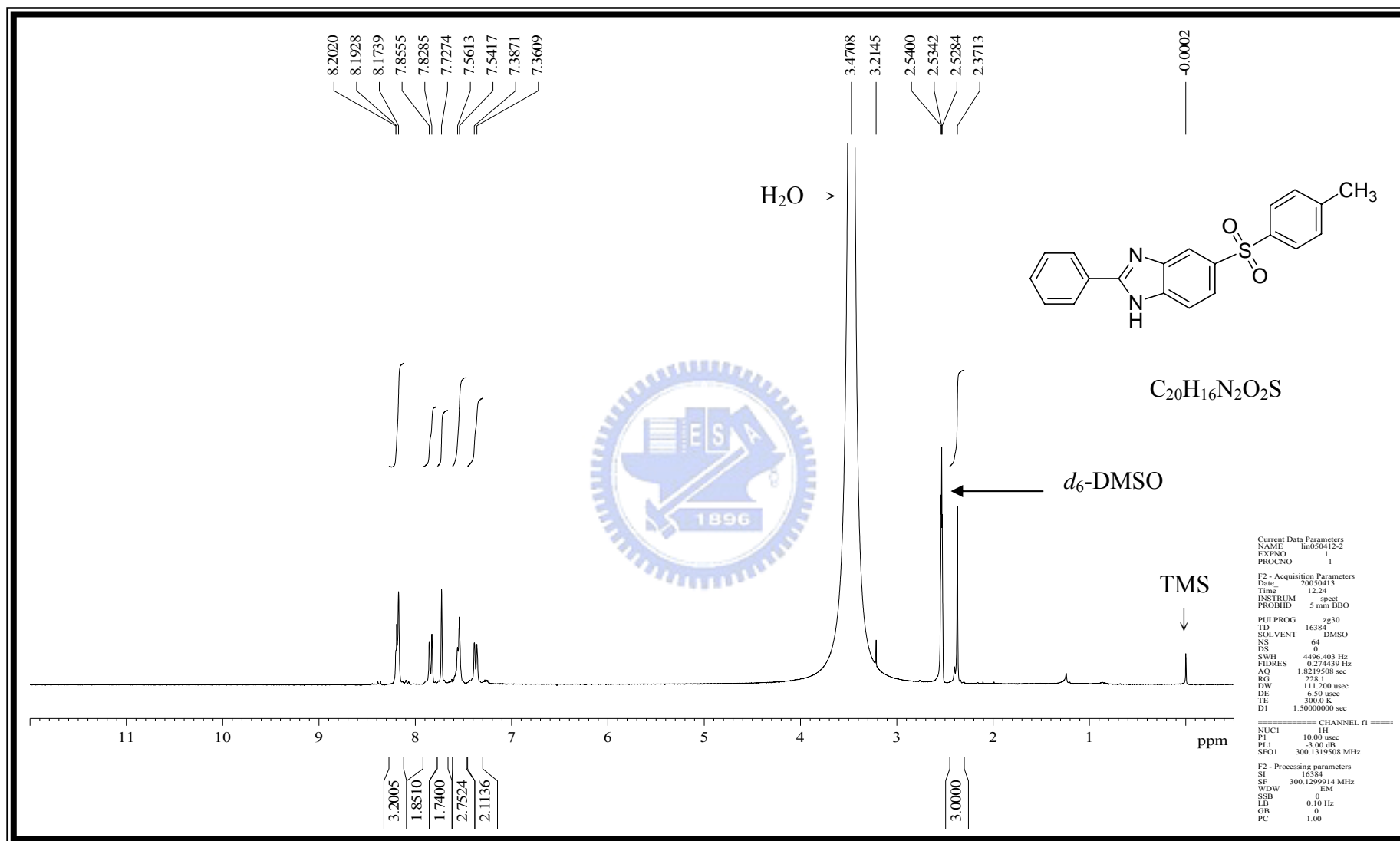
附圖 43 化合物 5-[(4-methylphenyl)sulfonyl]-2-phenyl-1H-benzo[d]imidazole, 73 之 ^1\text{H-NMR} (300 MHz, d_6 -DMSO) 光譜圖
