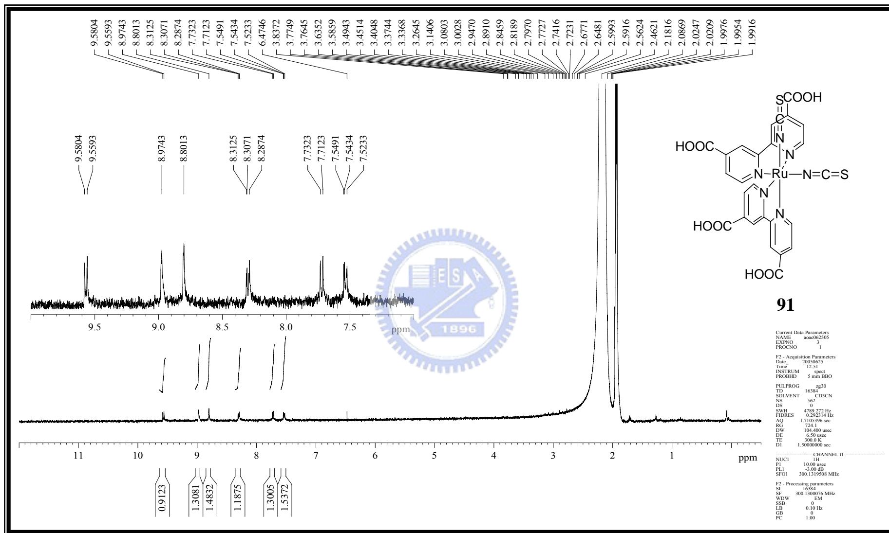
附圖 49 化合物 cis -di(thiocynato)bis(2,2'-bipyridyl-4,4'-dicarboxylate)ruthenium (II), 91 之 ^1\text{H-NMR} (300 MHz, \text{CD}_3\text{CN} ) 光譜圖
