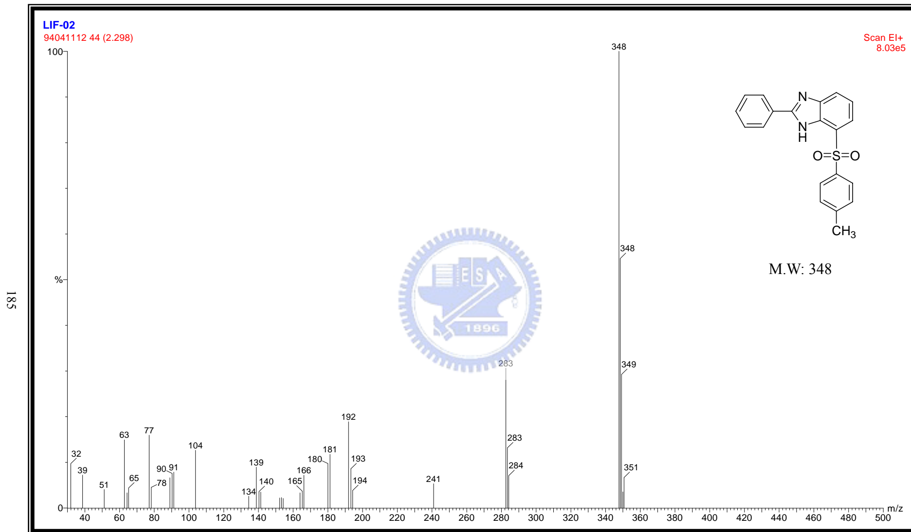
附圖 42 化合物 7-[(4-methylphenyl)sulfonyl]-2-phenyl-1H-benzo[d]imidazole, 72 之 EI 質譜圖
