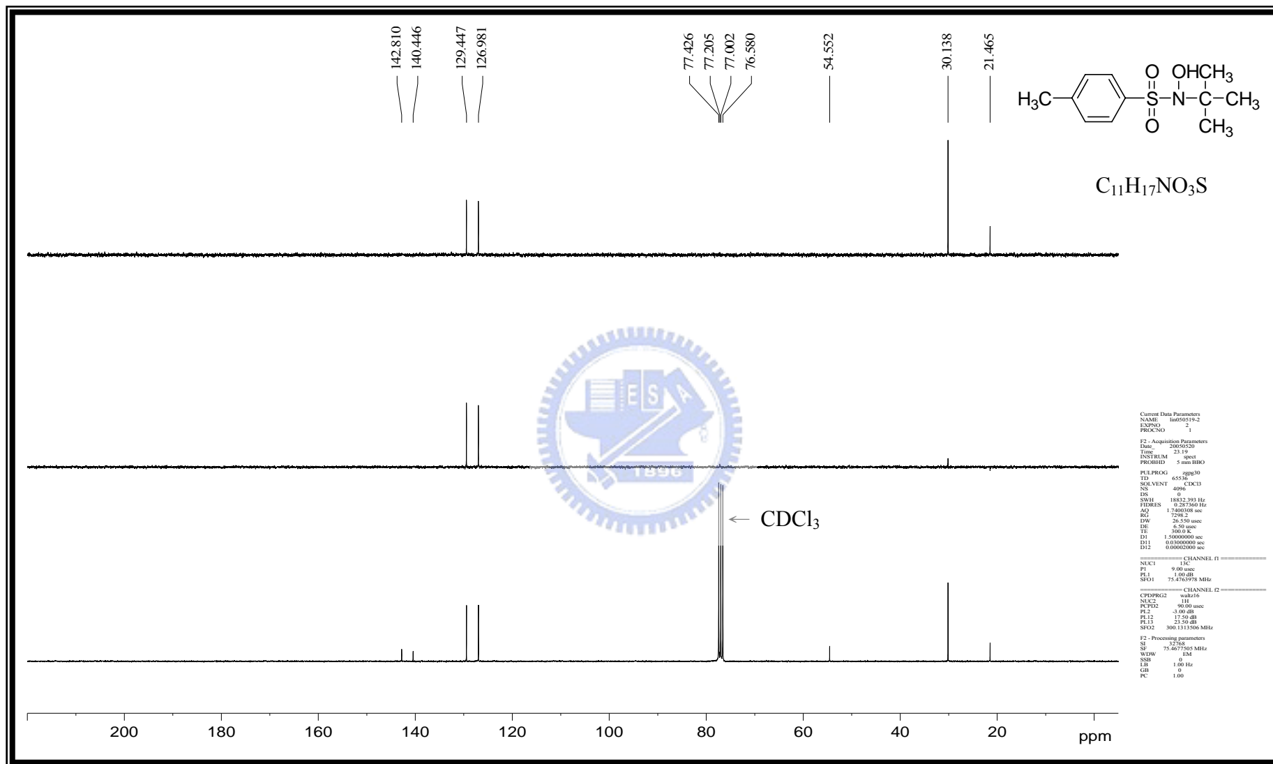
附圖 47 化合物 1-[(4-methylphenyl)sulfonyl]- N -( tert -butyl) hydroxylamine, Ts-MNP 之 DEPT- 13 C-NMR (75 MHz, CDCl 3 ) 光譜圖
