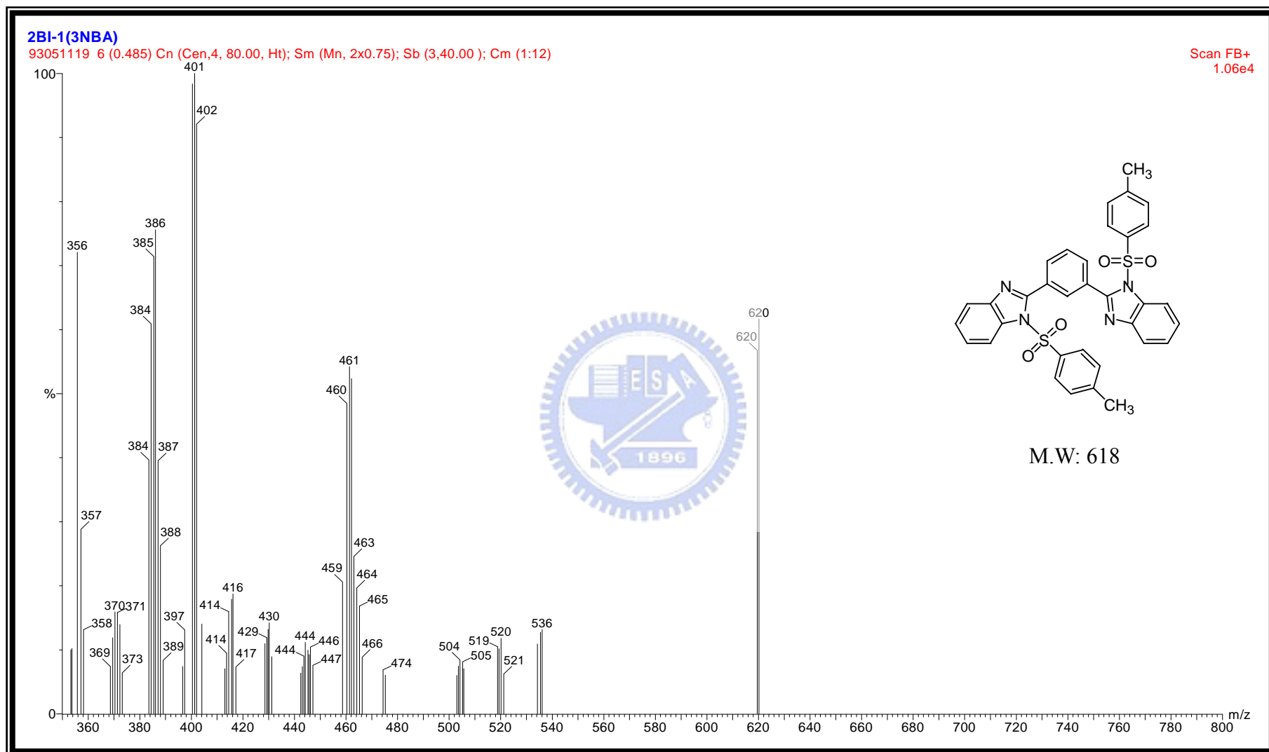
附圖 29 化合物 1-[(4-methylphenyl)sulfonyl]-2-(3-{1-[(4-methylphenyl)sulfonyl]-1H-benzo[d]imidazol-2-yl}phenyl)-1H-benzo[d]imidazole, 56 之 FAB 質譜圖
