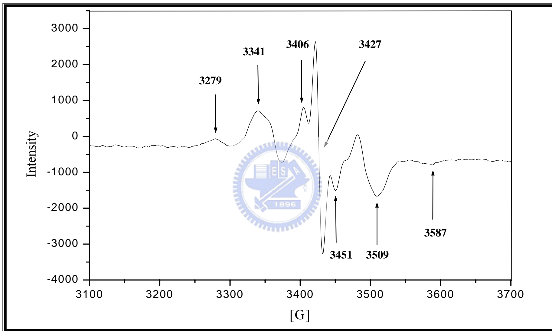
附圖 55 化合物 1-[(4-methylphenyl)sulfonyl]2-phenyl-1 H -benzo[ d ]imidazole, 55 照光後之 77 K EPR 光譜放大圖
