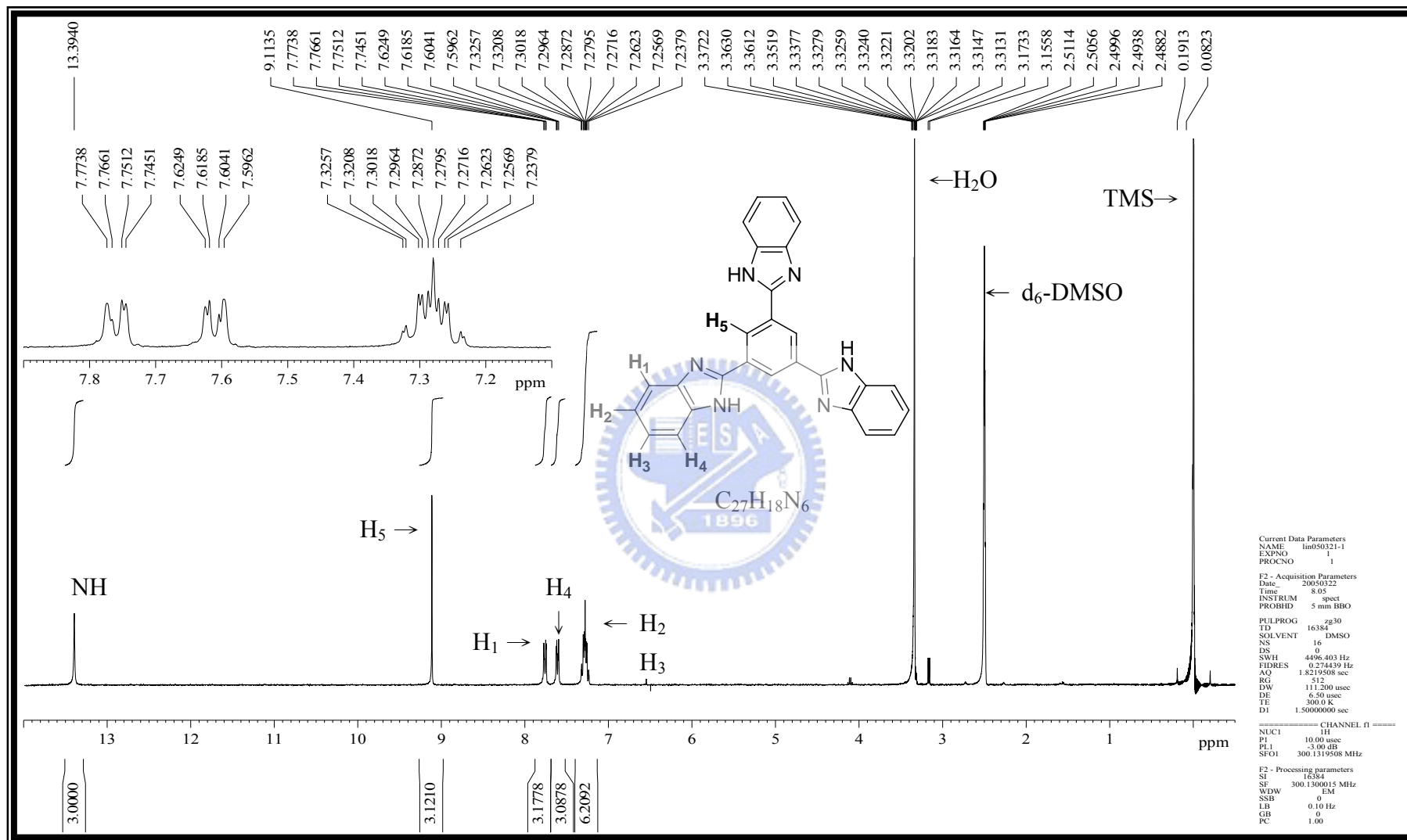
附圖 7 化合物 2-[3,5-di(1H-benzo[d]imidazol-2-yl)phenyl]-1H-benzo[d]imidazole, 60 之 1 H-NMR (300 MHz, d 6 -DMSO) 光譜圖
