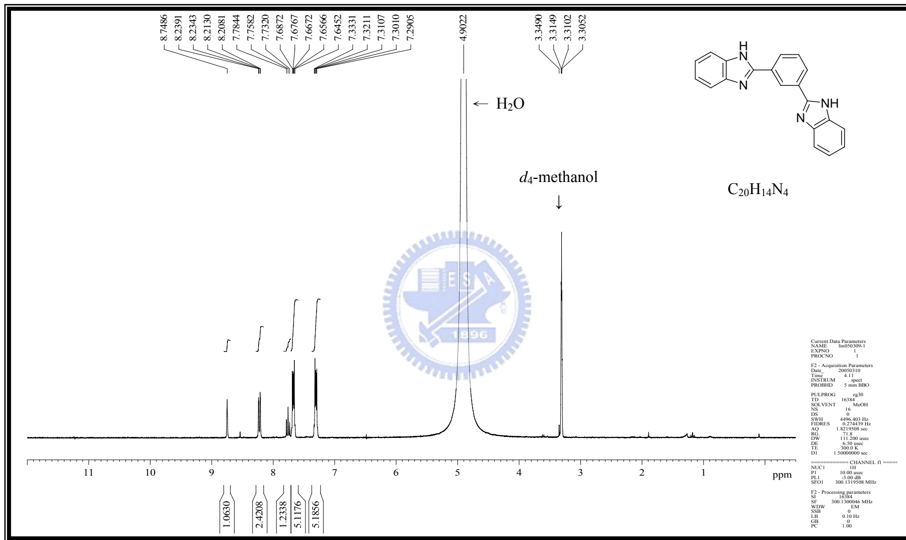
附圖 4 化合物 2-[3-(1H-benzo[d]imidazol-2-yl)phenyl]-1H-benzo[d]imidazole, 59 之 ^1\text{H-NMR} (300 MHz, d_4 -methanol) 光譜圖
