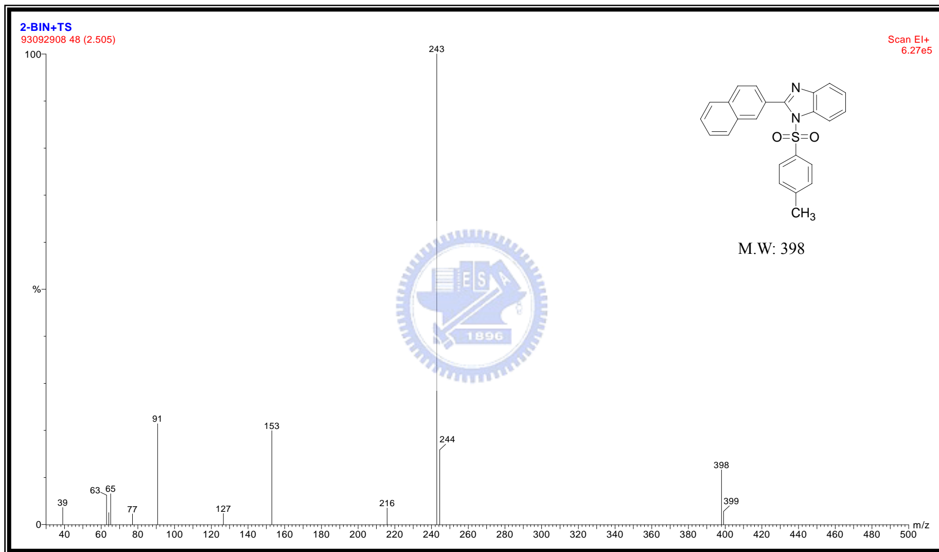
附圖 40 化合物 1-[(4-methylphenyl)sulfonyl]-2-(2-naphthyl)-1H-benzo[d]imidazole, 66 之 EI 質譜圖
