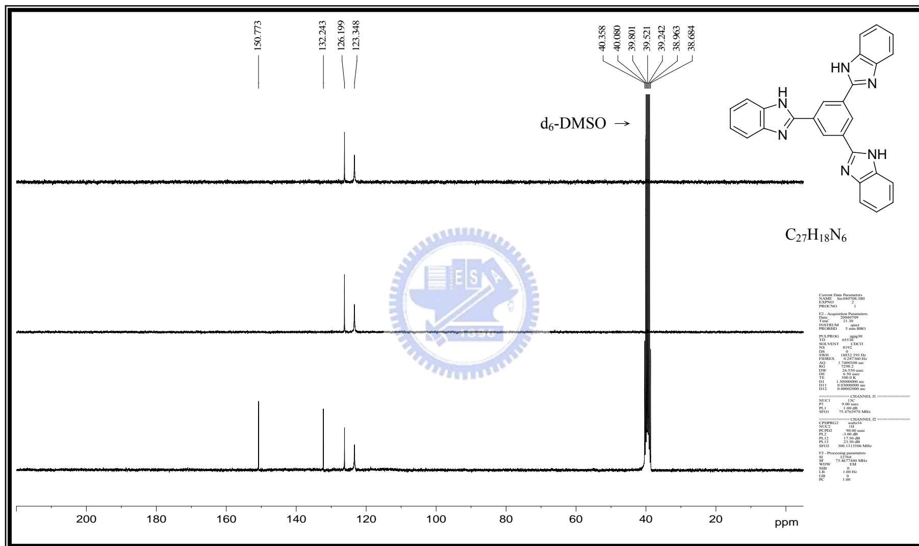
附圖 8 化合物 2-[3,5-di(1H-benzo[d]imidazol-2-yl)phenyl]-1H-benzo[d]-imidazole, 60 之 DEPT- ^{13}C -NMR (75 MHz, d_6 -DMSO) 光譜圖
