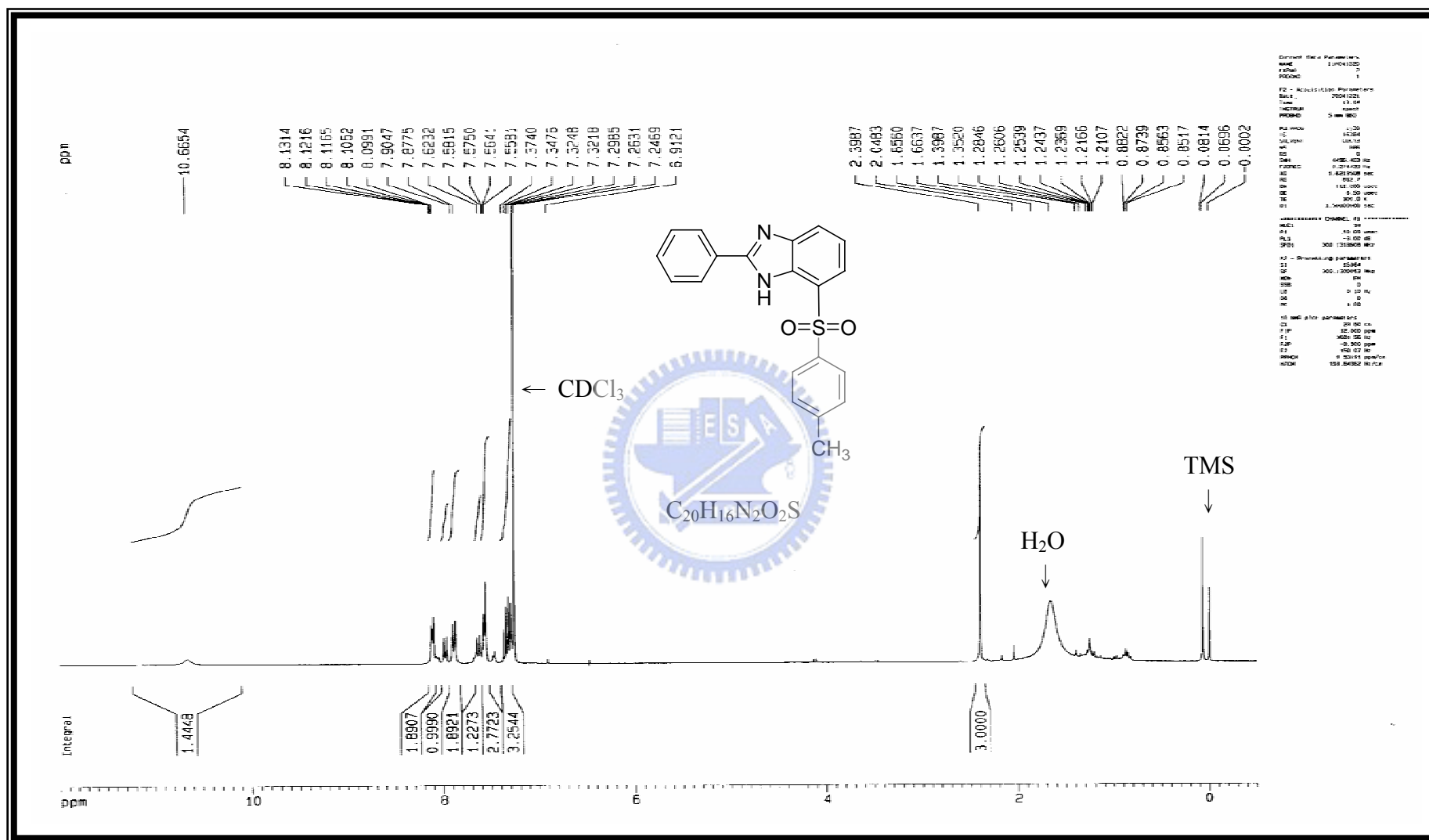
附圖 41 化合物 7-[(4-methylphenyl)sulfonyl]-2-phenyl-1 H -benzo[ d ]imidazole, 72 之 1 H-NMR (300 MHz, CDCl 3 ) 光譜圖
