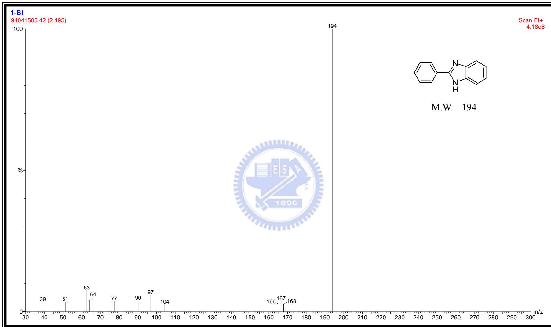
附圖 3 化合物 2-phenyl-1H-benzo[d]imidazole, 58 之 EI 質譜圖
