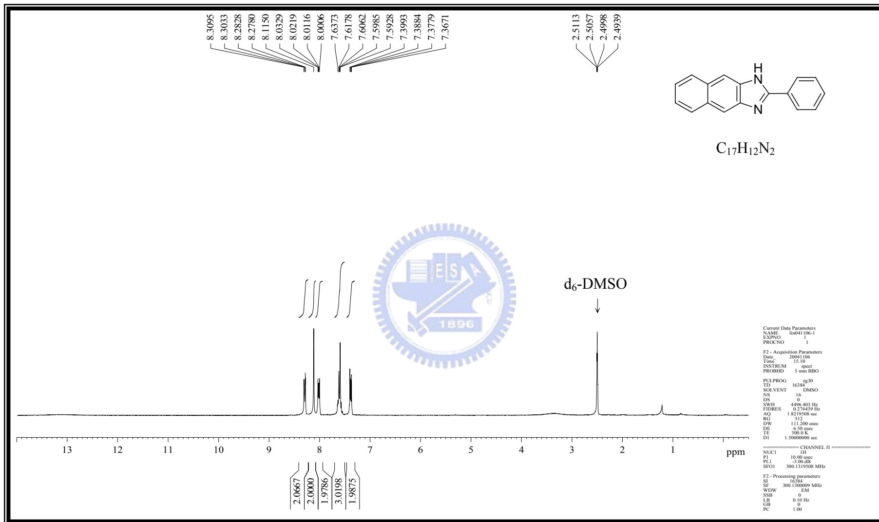
附圖 16 2-phenyl-1 H -naphtho[2,3- d ]imidazole, 63 之 ^1\text{H} -NMR (300 MHz, d_6 -DMSO) 光譜圖
