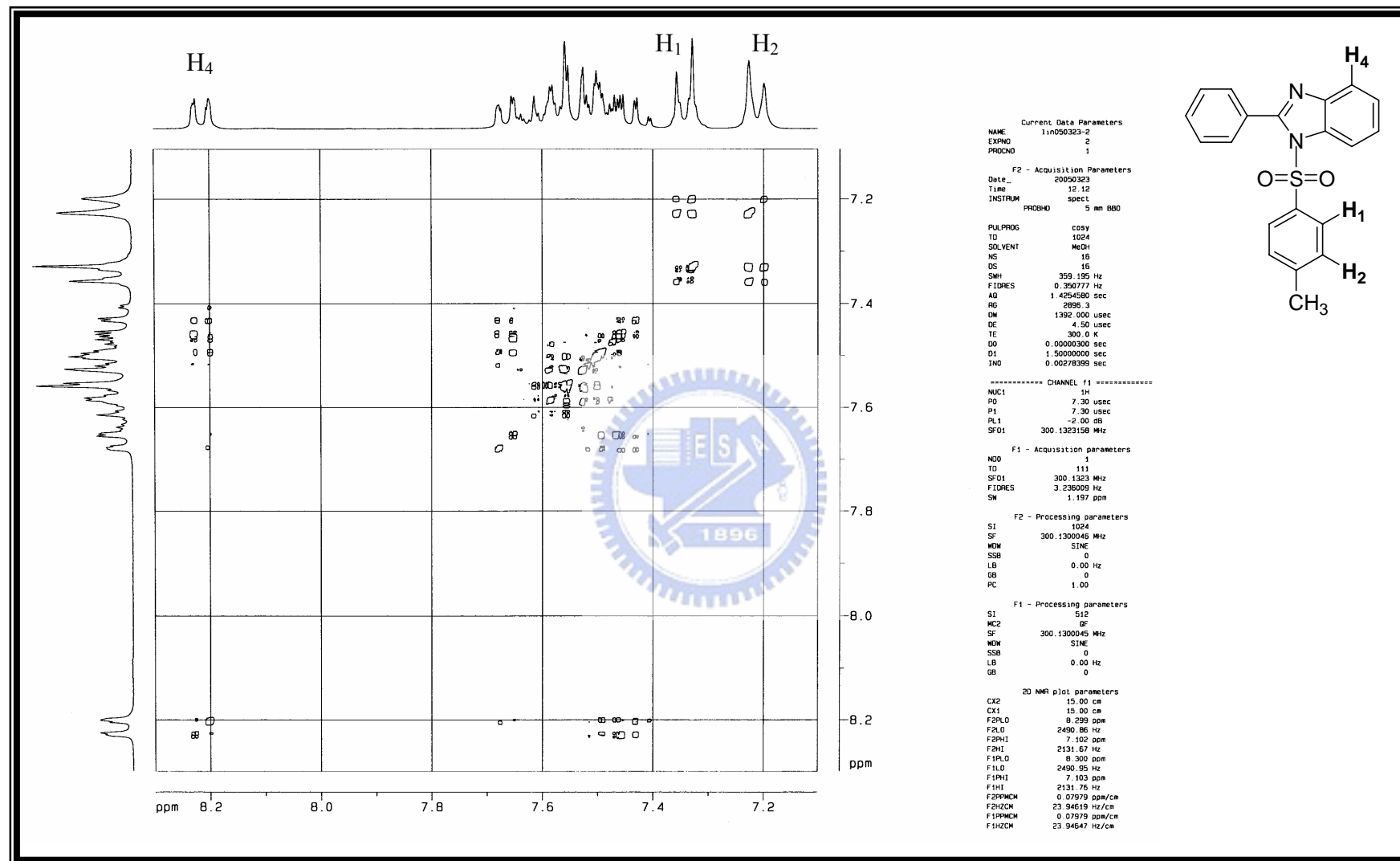
附圖 23 化合物 1-[(4-methylphenyl)sulfonyl]-2-phenyl-1H-benzo[d]imidazole, 55 之 H,H-COSY-NMR (300 MHz, d_4 -methanol) 光譜圖
