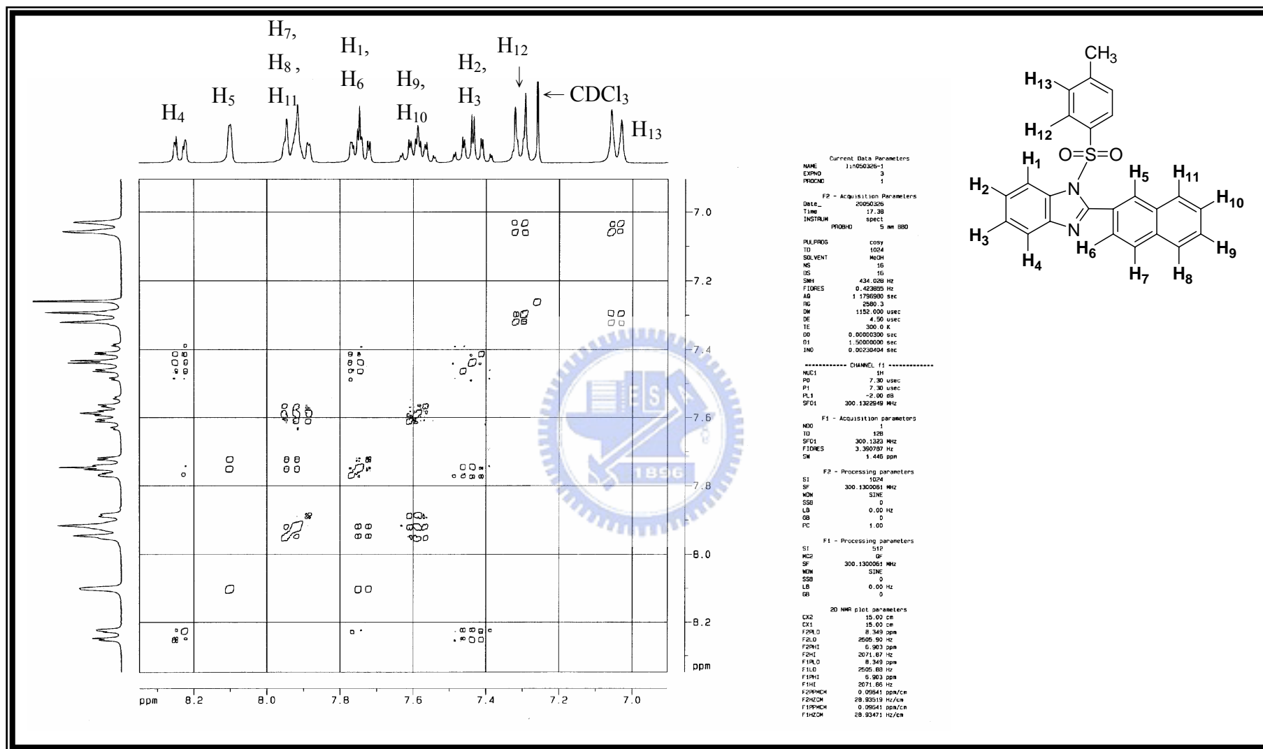
附圖 38 化合物 1-[(4-methylphenyl)sulfonyl]-2-(2-naphthyl)-1H-benzo[d]imidazole, 66 之 H,H-COSY-NMR (300 MHz, CDCl 3 ) 光譜圖
