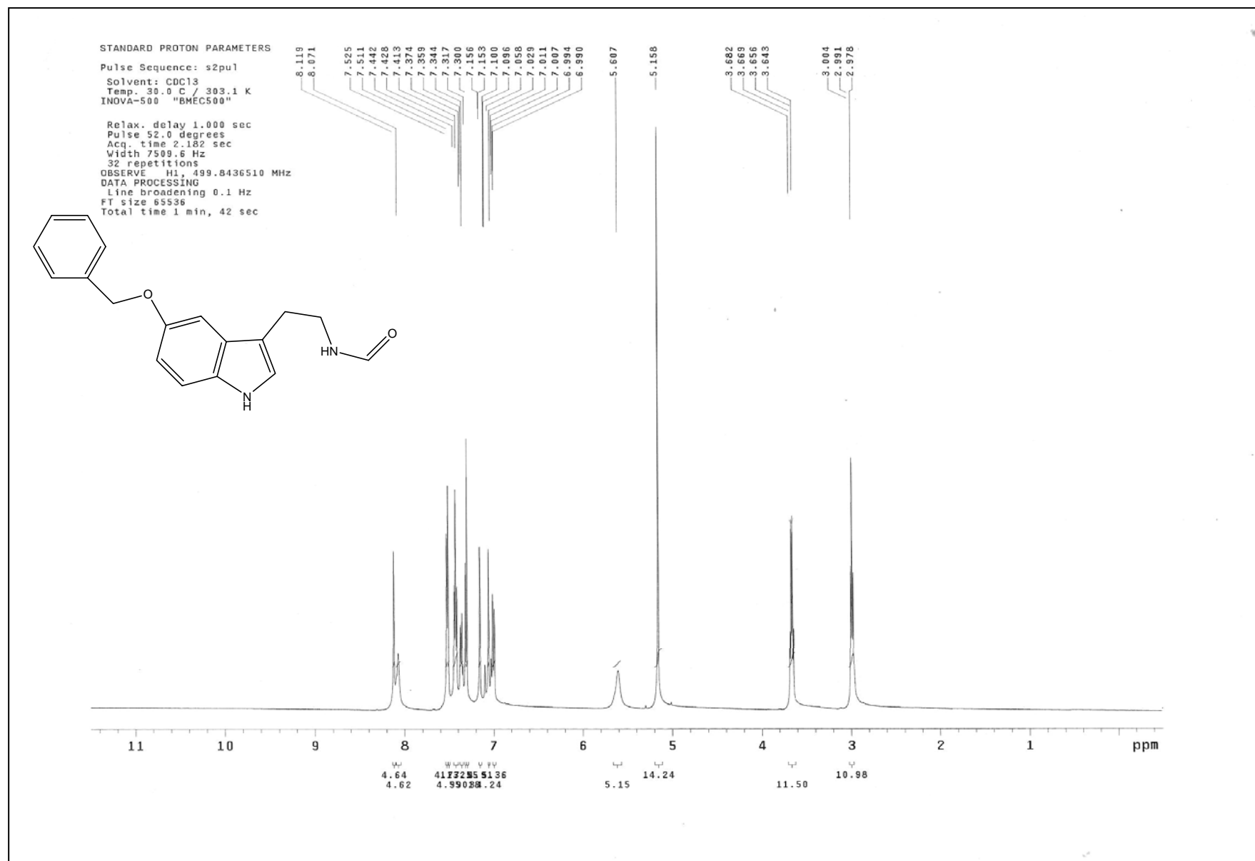
圖 10 化合物 36 之 1 H核磁共振光譜圖
