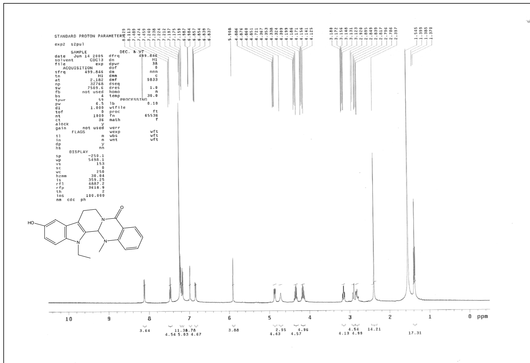
圖 25 化合物 51 之 1 H核磁共振光譜圖
