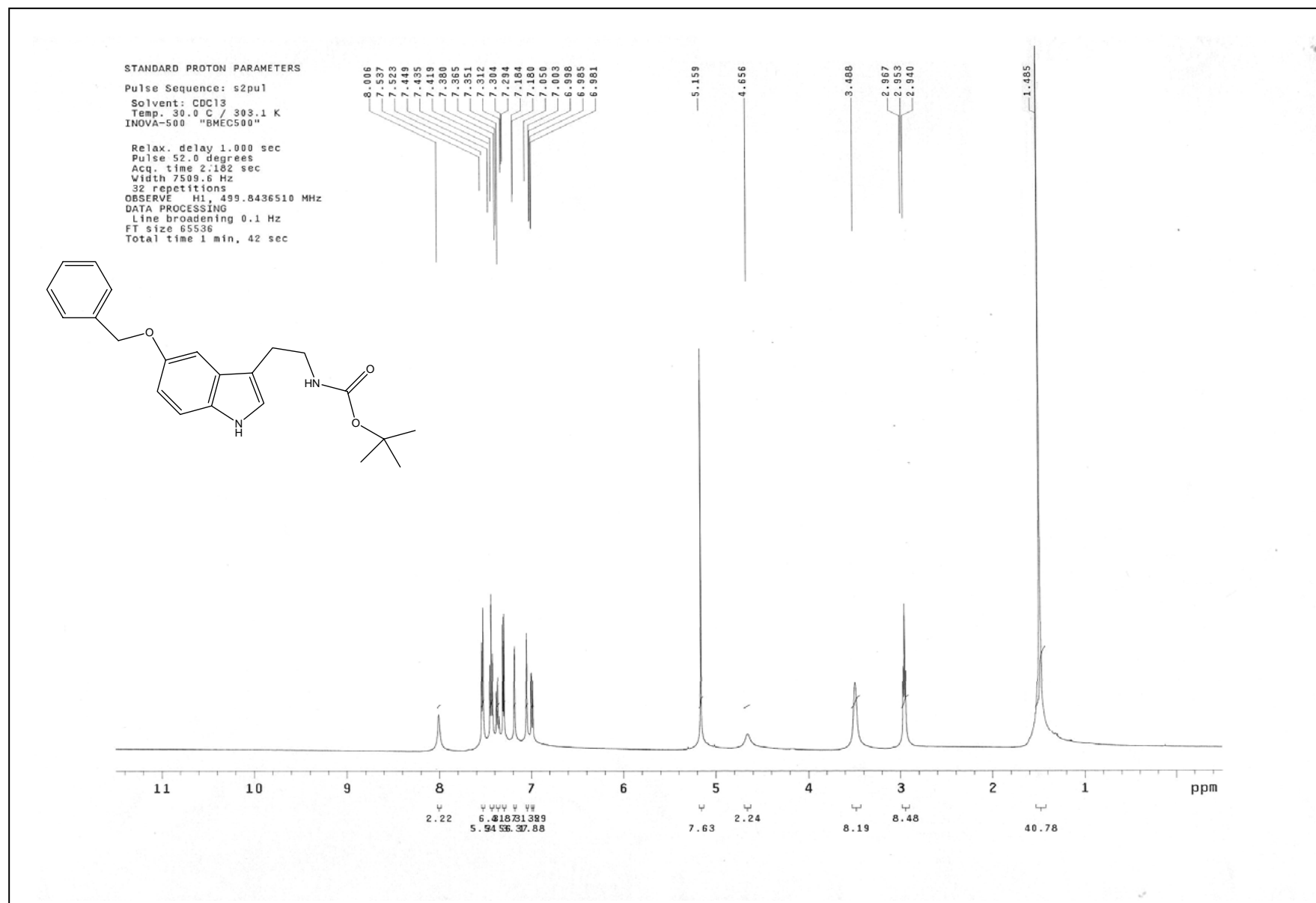
圖 9 化合物 34 之 1 H核磁共振光譜圖
