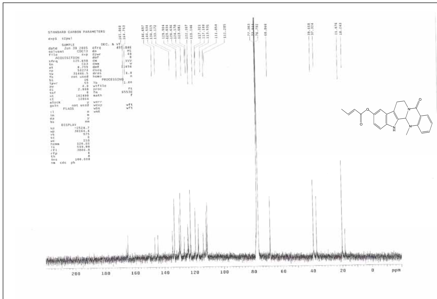
圖 38 化合物 48 之 ^{13}\text{C} 核磁共振光譜圖
