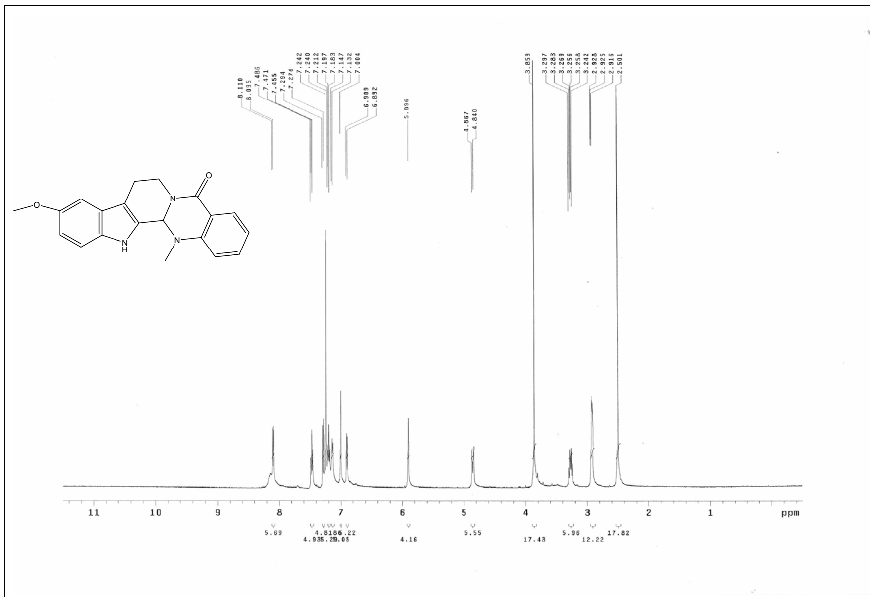
圖 8 化合物 32 之 1 H核磁共振光譜圖
