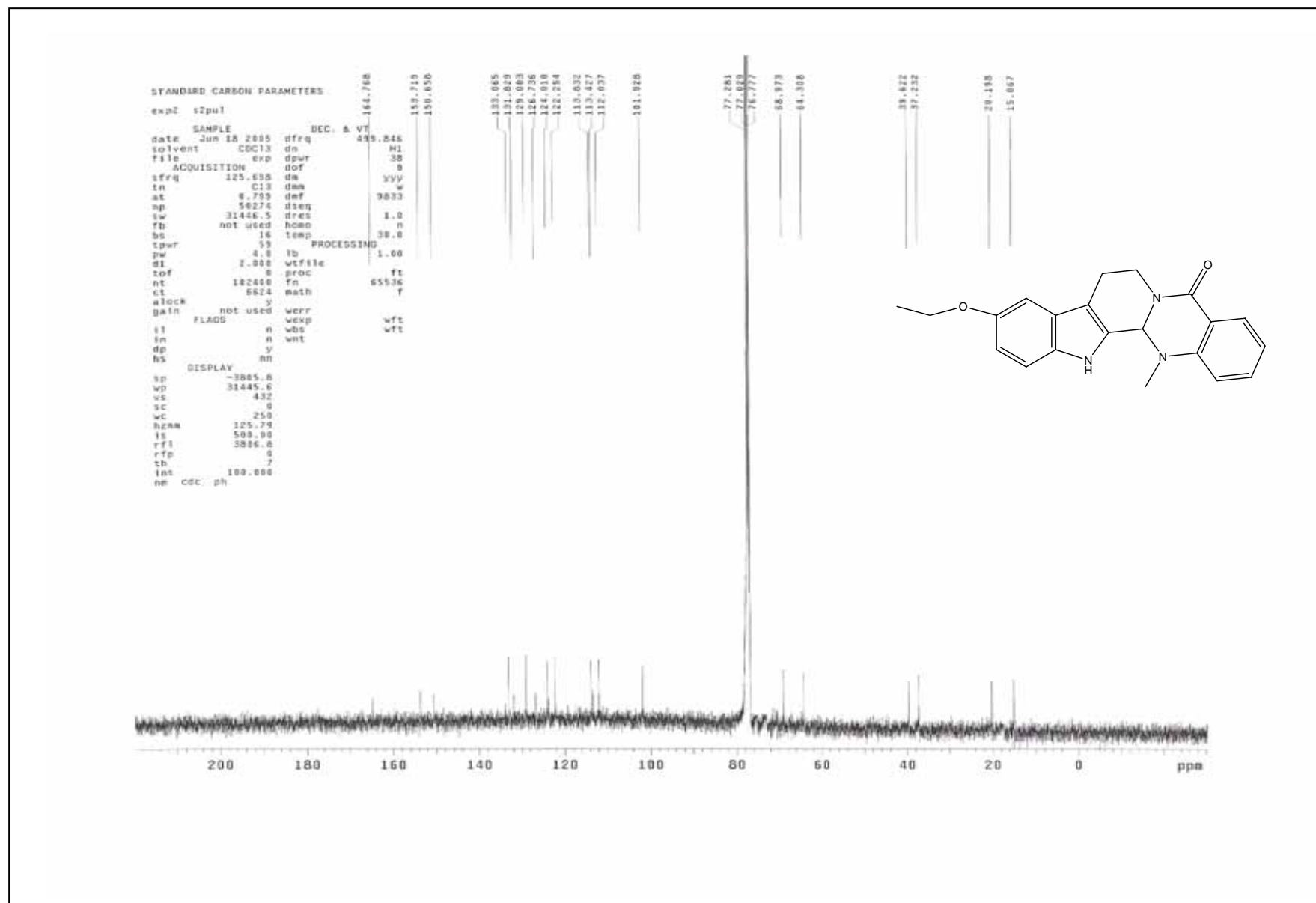
圖 30 化合物 39 之 ^{13}\text{C} 核磁共振光譜圖
