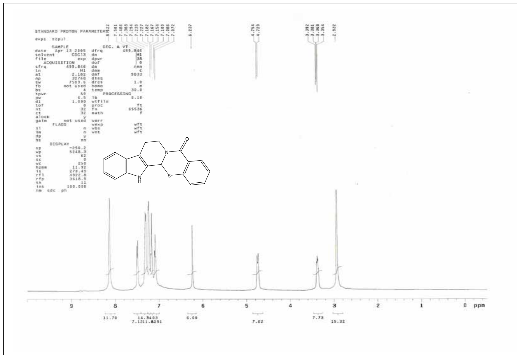
圖 19 化合物 44 之 1 H核磁共振光譜圖
