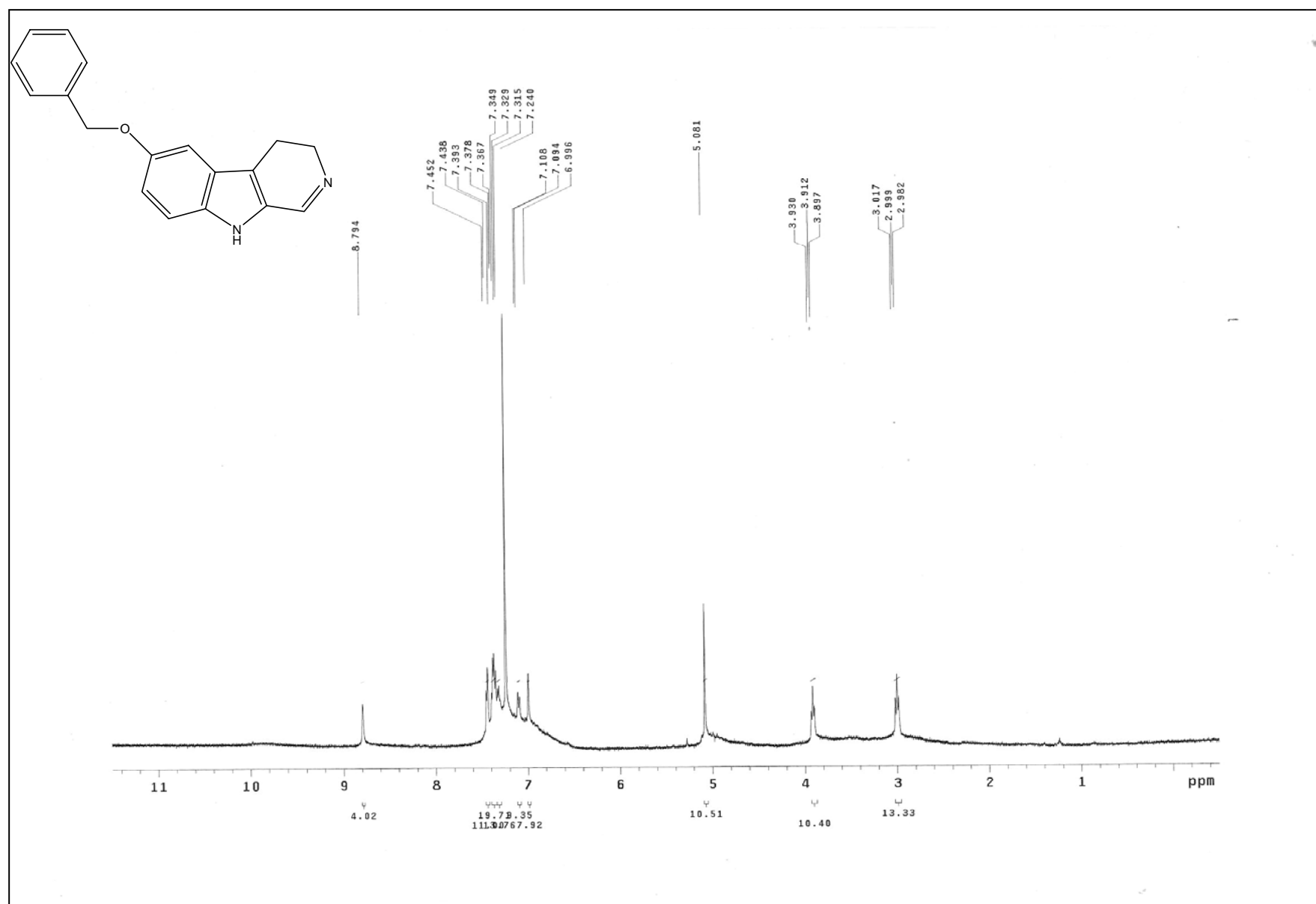
圖 11 化合物 37 之 1 H核磁共振光譜圖
