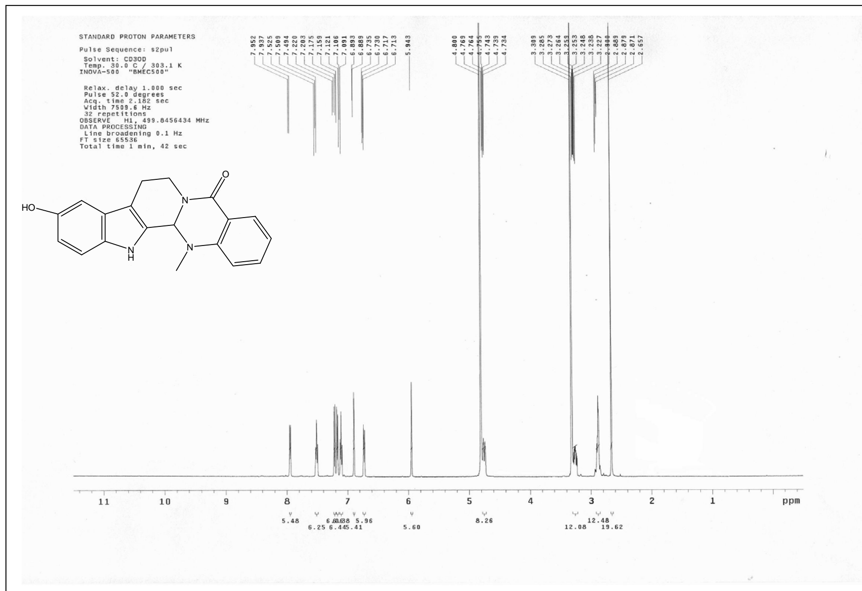
圖 13 化合物 33 之 1 H核磁共振光譜圖
