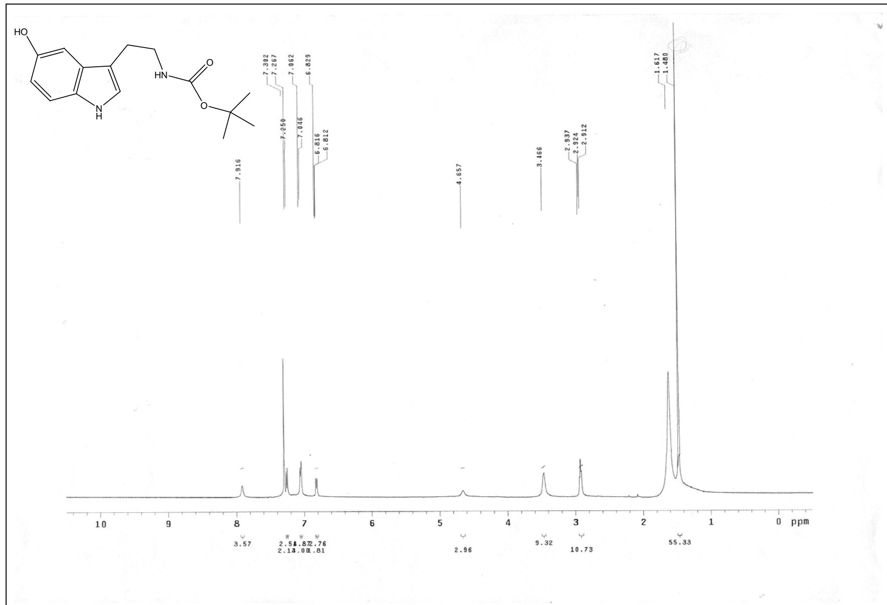
圖 4 化合物 27 之 1 H核磁共振光譜圖
