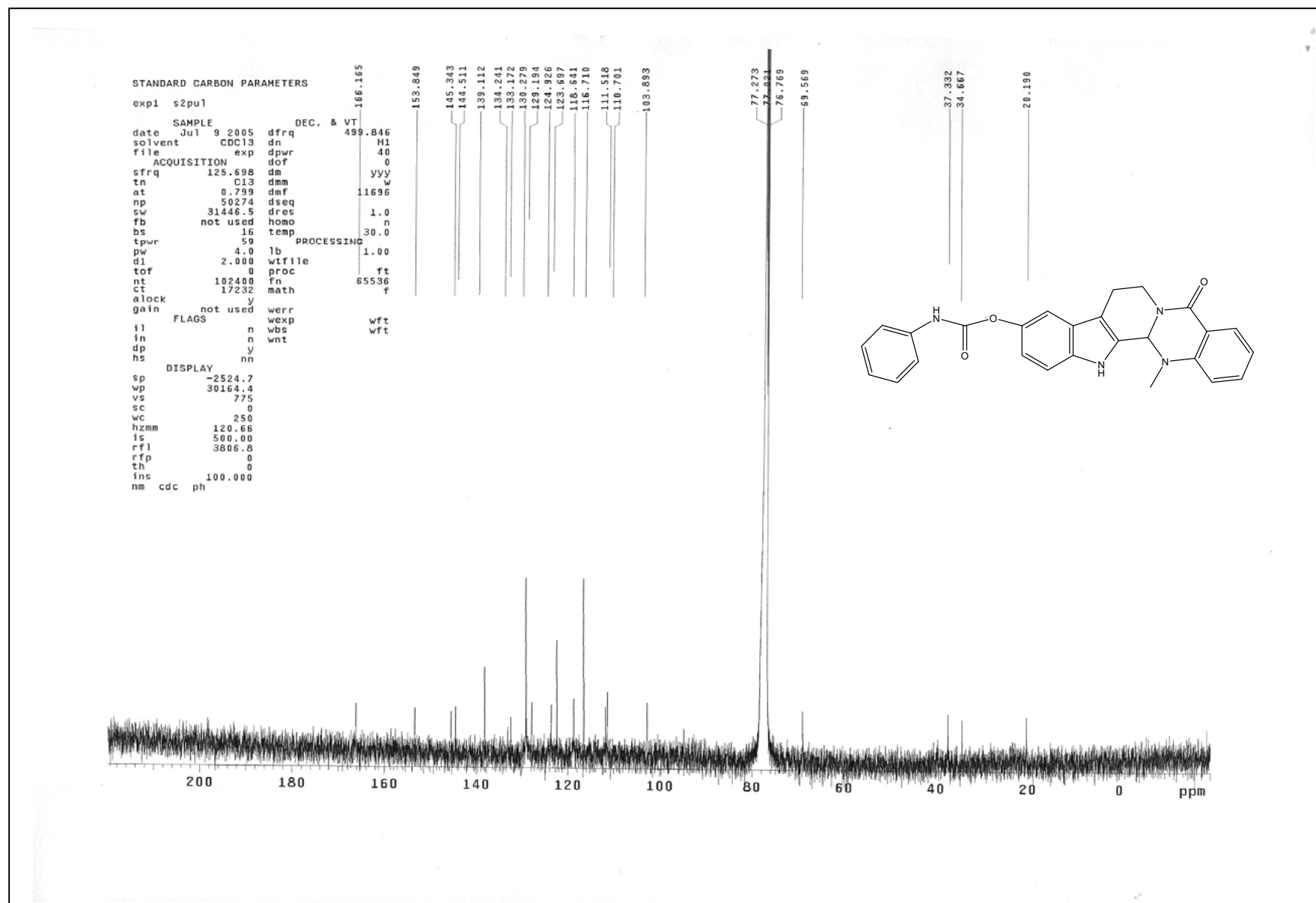
圖 37 化合物 46 之 ^{13}\text{C} 核磁共振光譜圖
