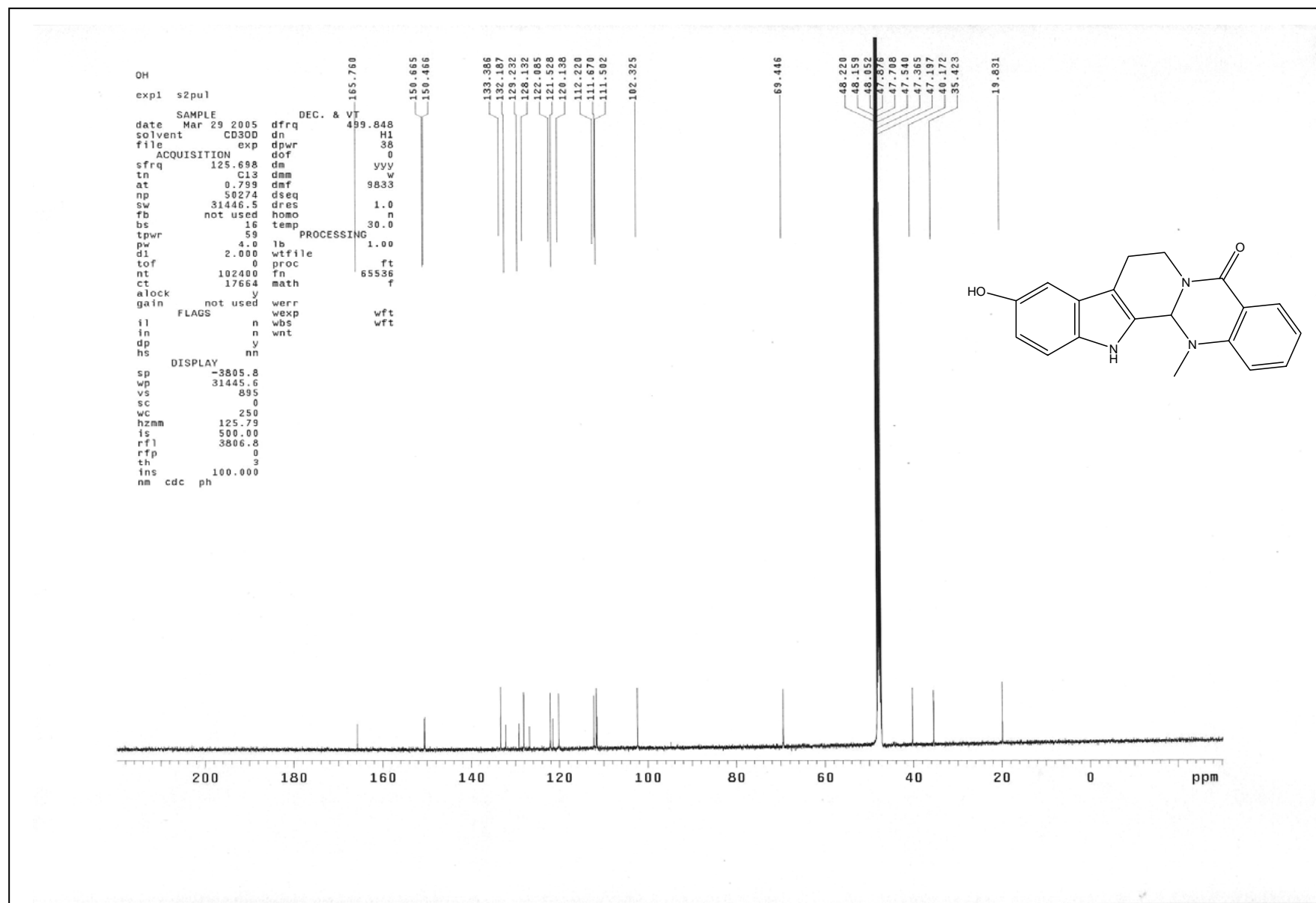
圖 28 化合物 33 之 ^{13}\text{C} 核磁共振光譜圖
