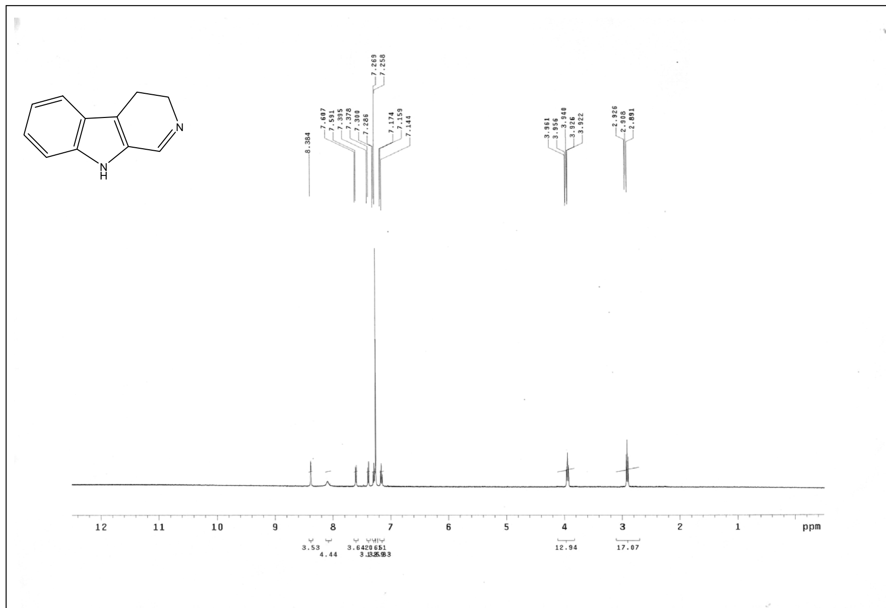
圖 2 化合物 9 之 1 H核磁共振光譜圖
