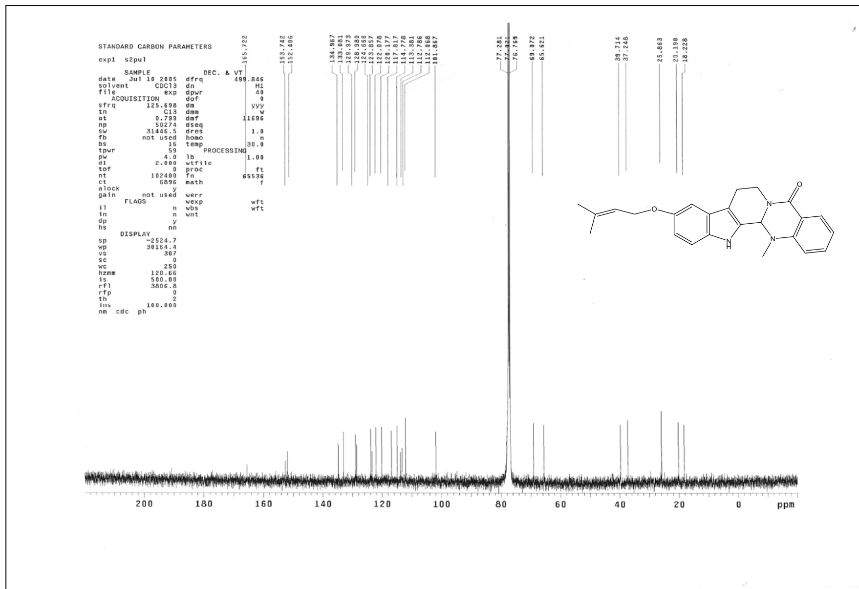
圖 34 化合物 43 之 ^{13}\text{C} 核磁共振光譜圖
