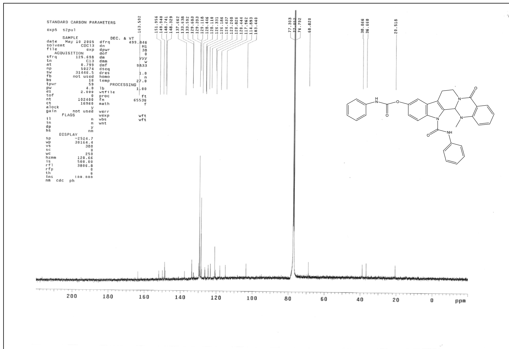
圖 43 化合物 53 之 ^{13}\text{C} 核磁共振光譜圖
