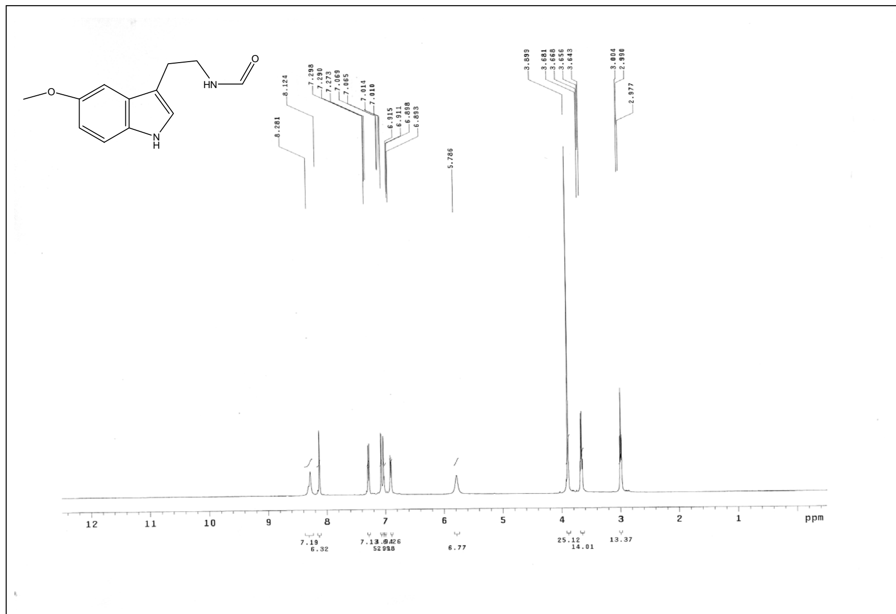
圖 6 化合物 30 之 1 H核磁共振光譜圖
