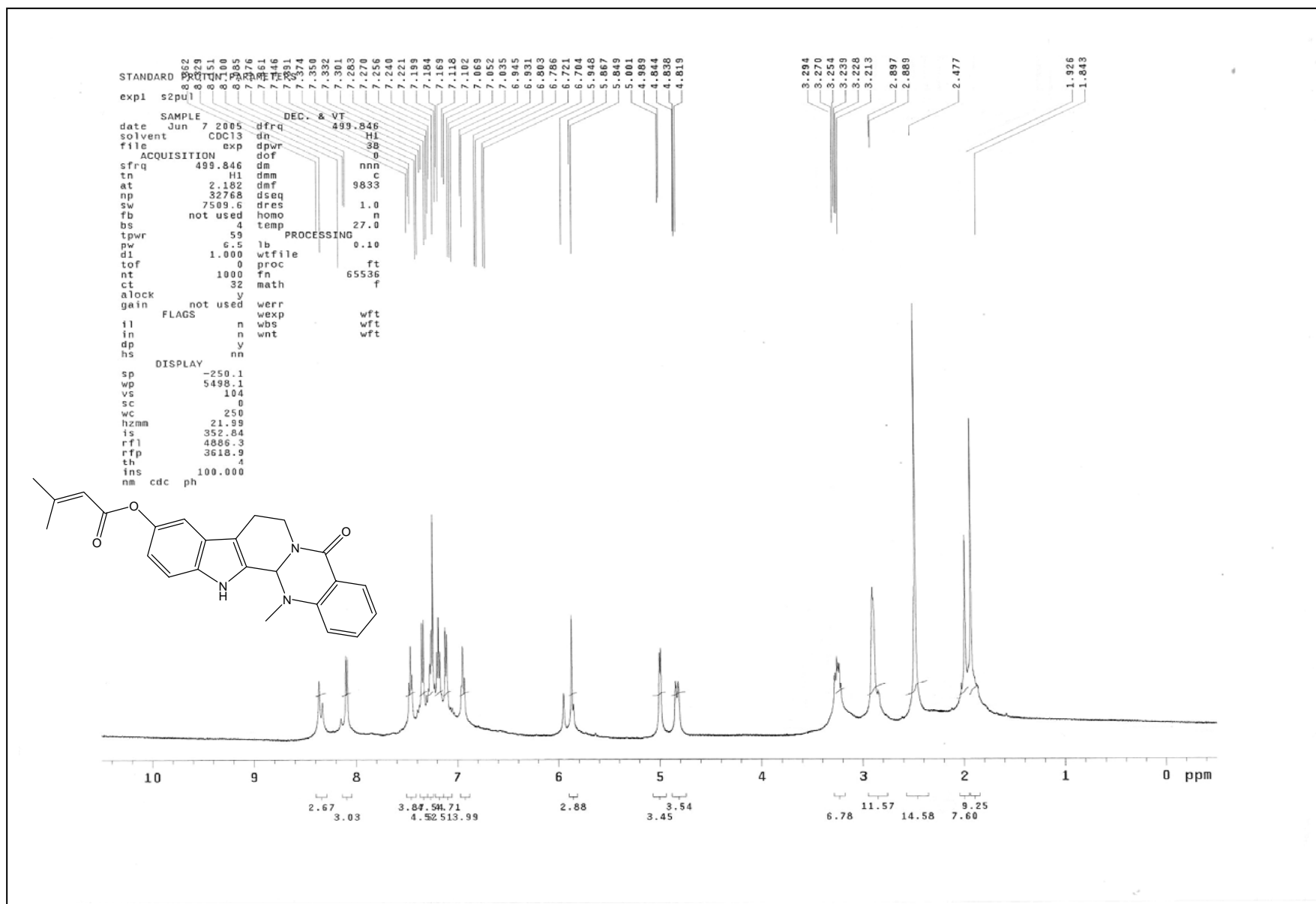
圖 23 化合物 49 之 1 H核磁共振光譜圖
