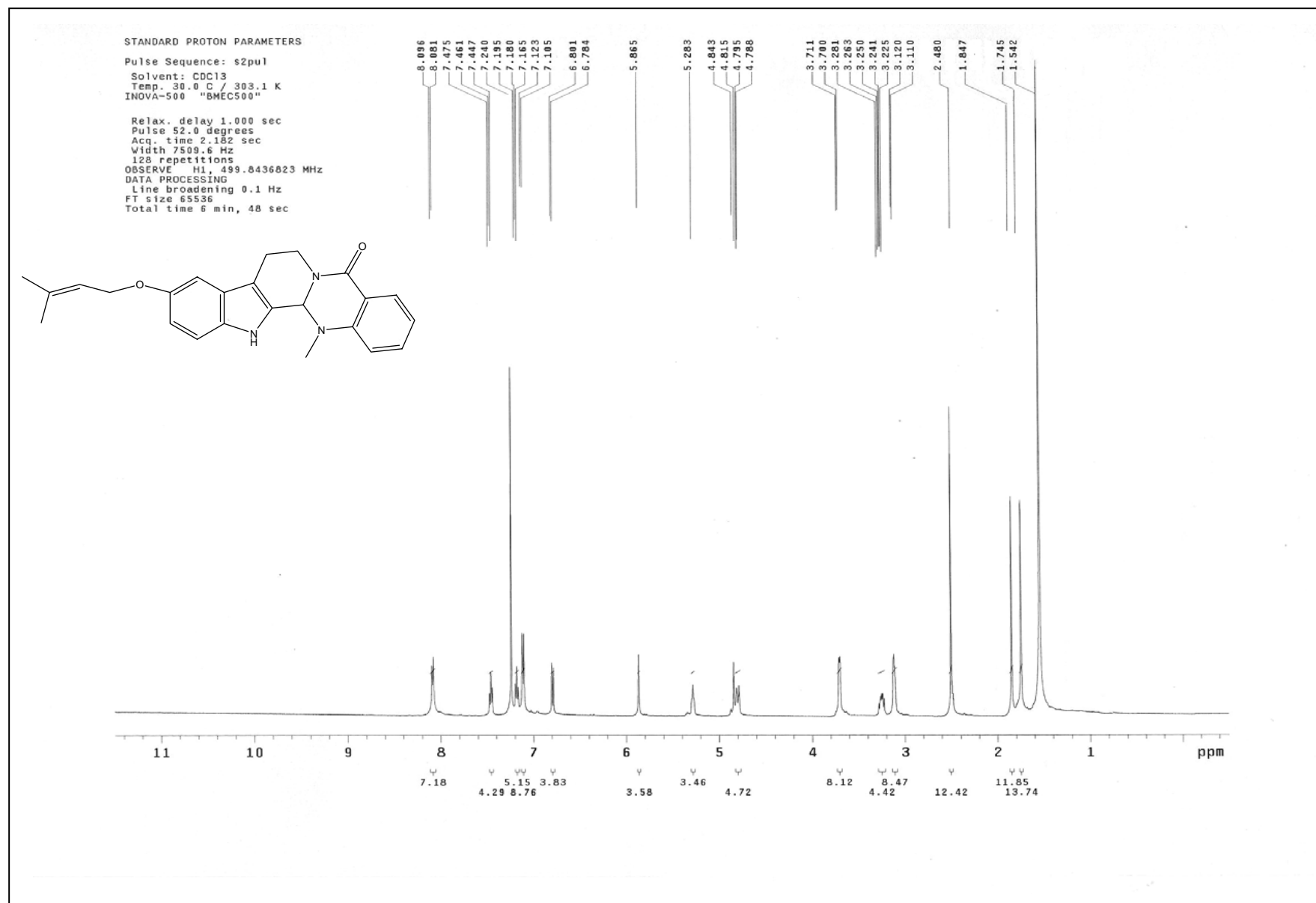
圖 18 化合物 43 之 1 H核磁共振光譜圖
