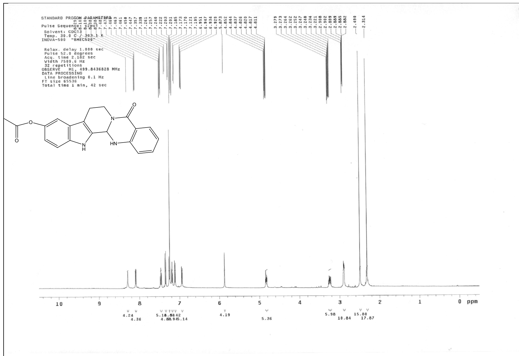
圖 17 化合物 40 之 1 H核磁共振光譜圖
