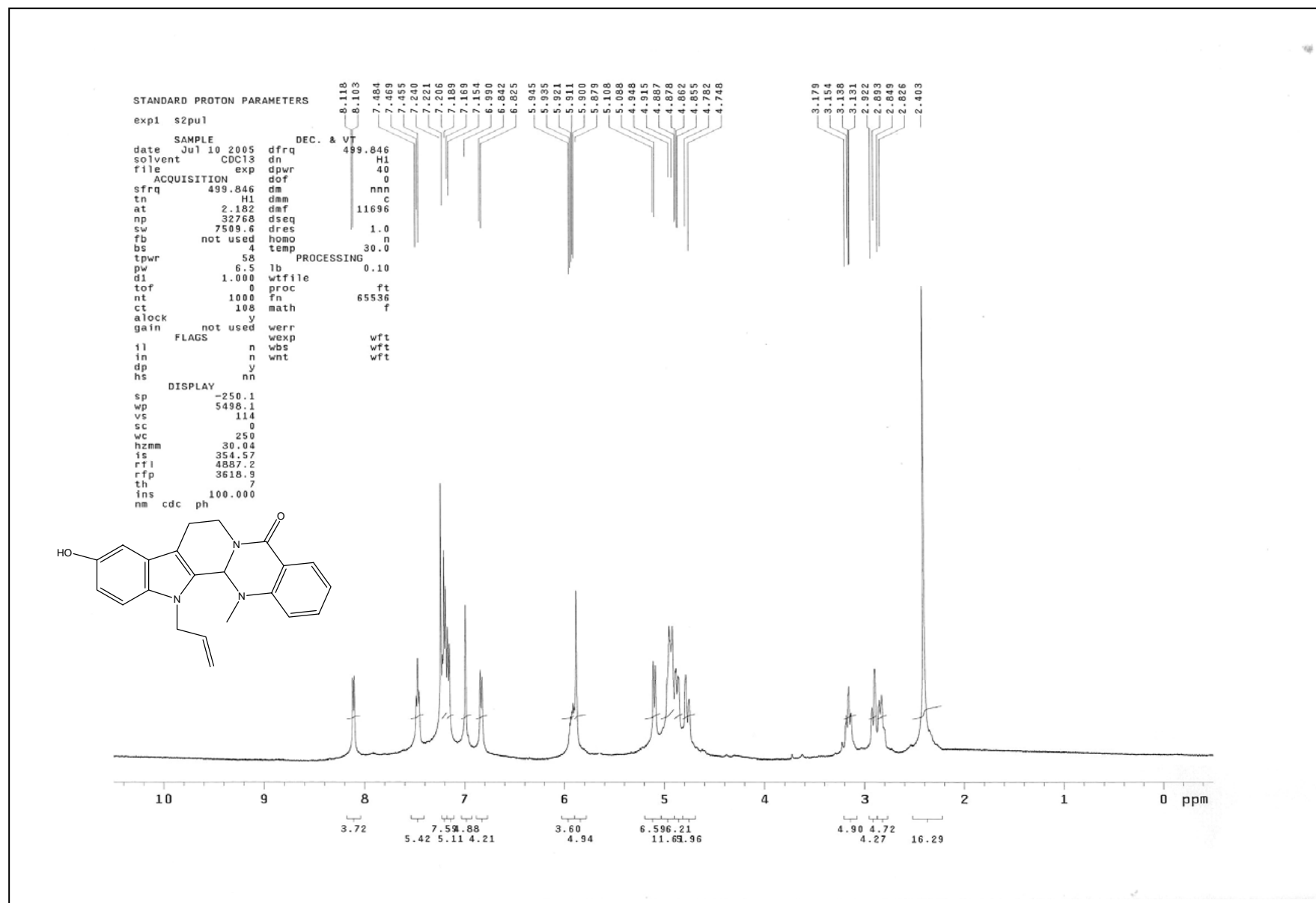
圖 26 化合物 52 之 1 H核磁共振光譜圖
