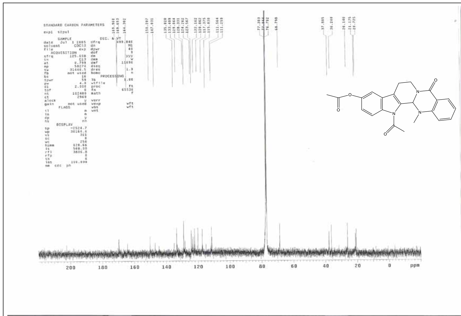
圖 32 化合物 41 之 13 C核磁共振光譜圖
