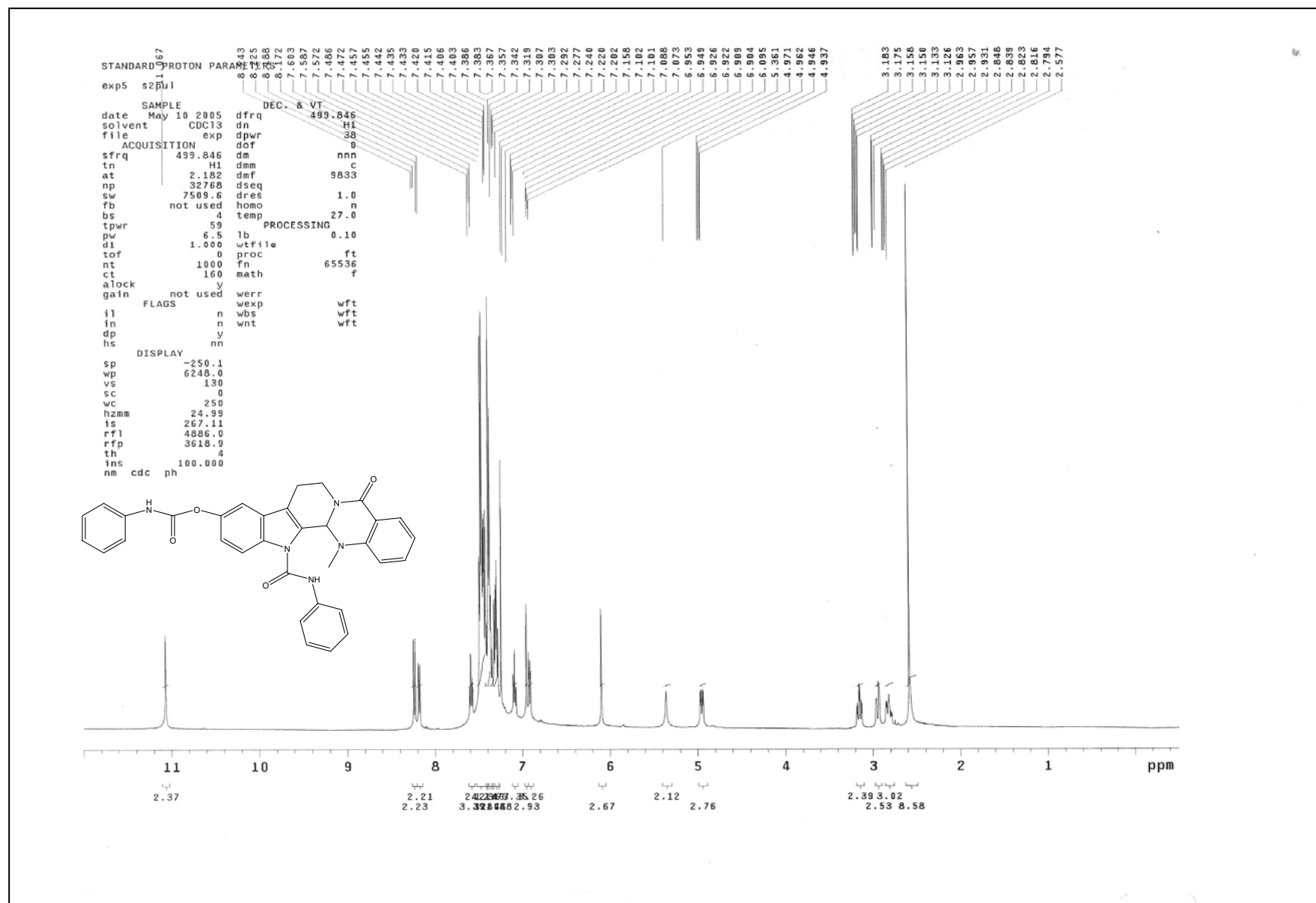
圖 27 化合物 53 之 1 H核磁共振光譜圖
