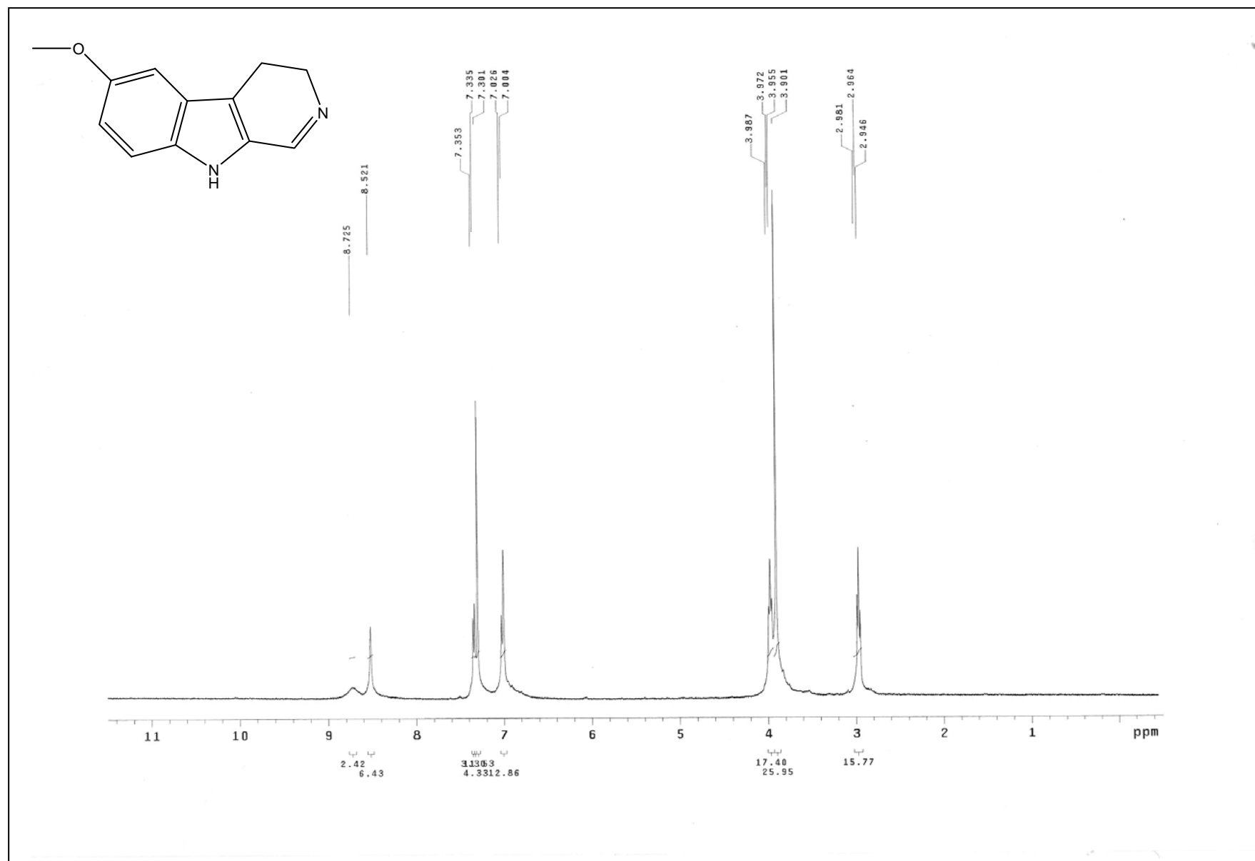
圖 7 化合物 31 之 1 H核磁共振光譜圖
