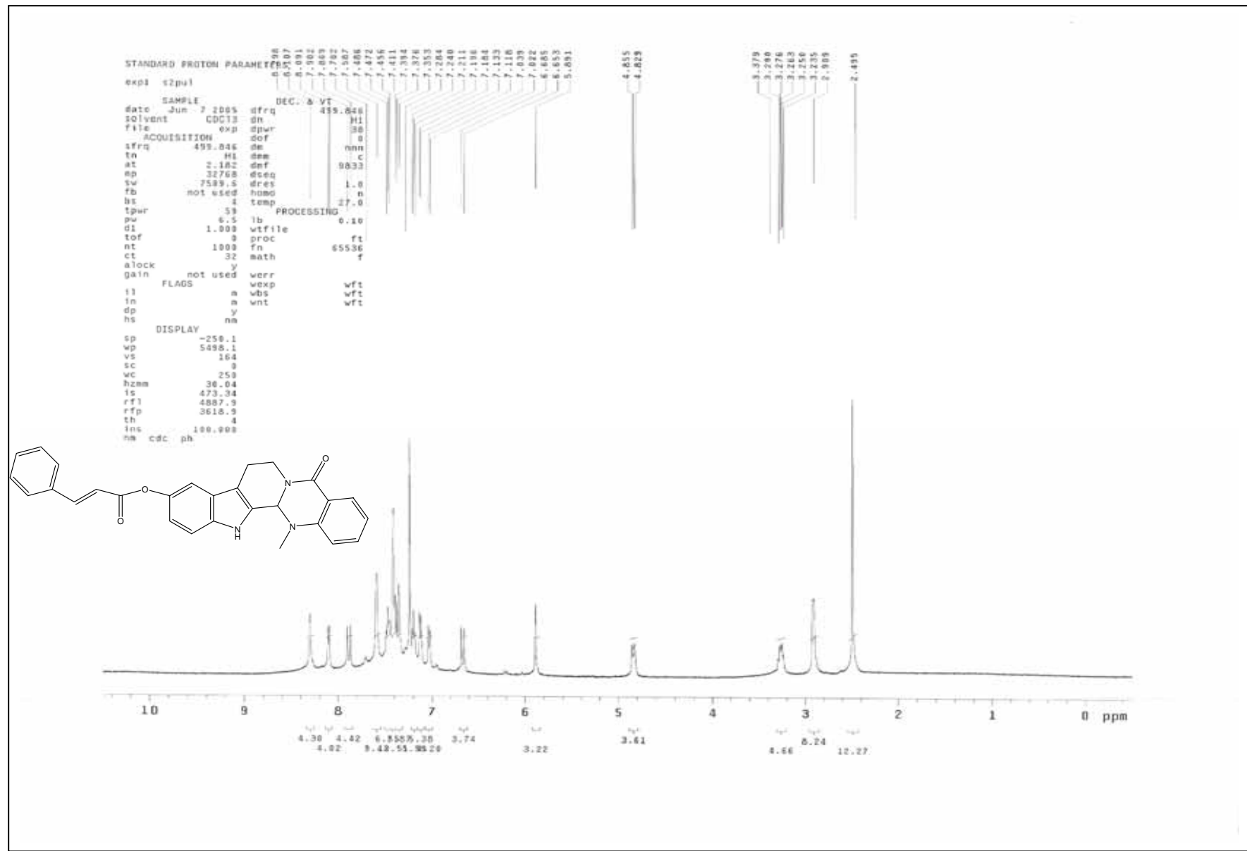
圖 24 化合物 50 之 1 H核磁共振光譜圖
