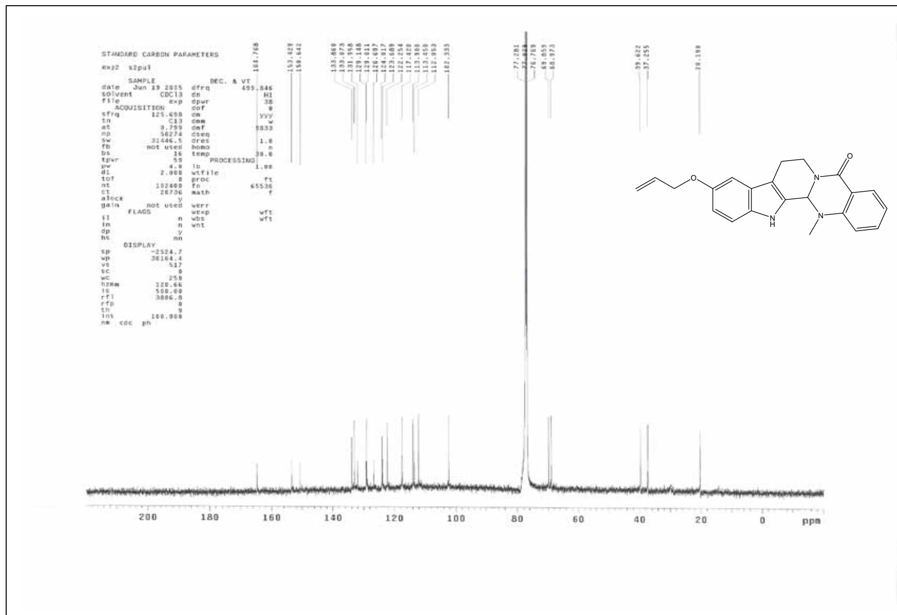
圖 33 化合物 42 之 ^{13}\text{C} 核磁共振光譜圖
