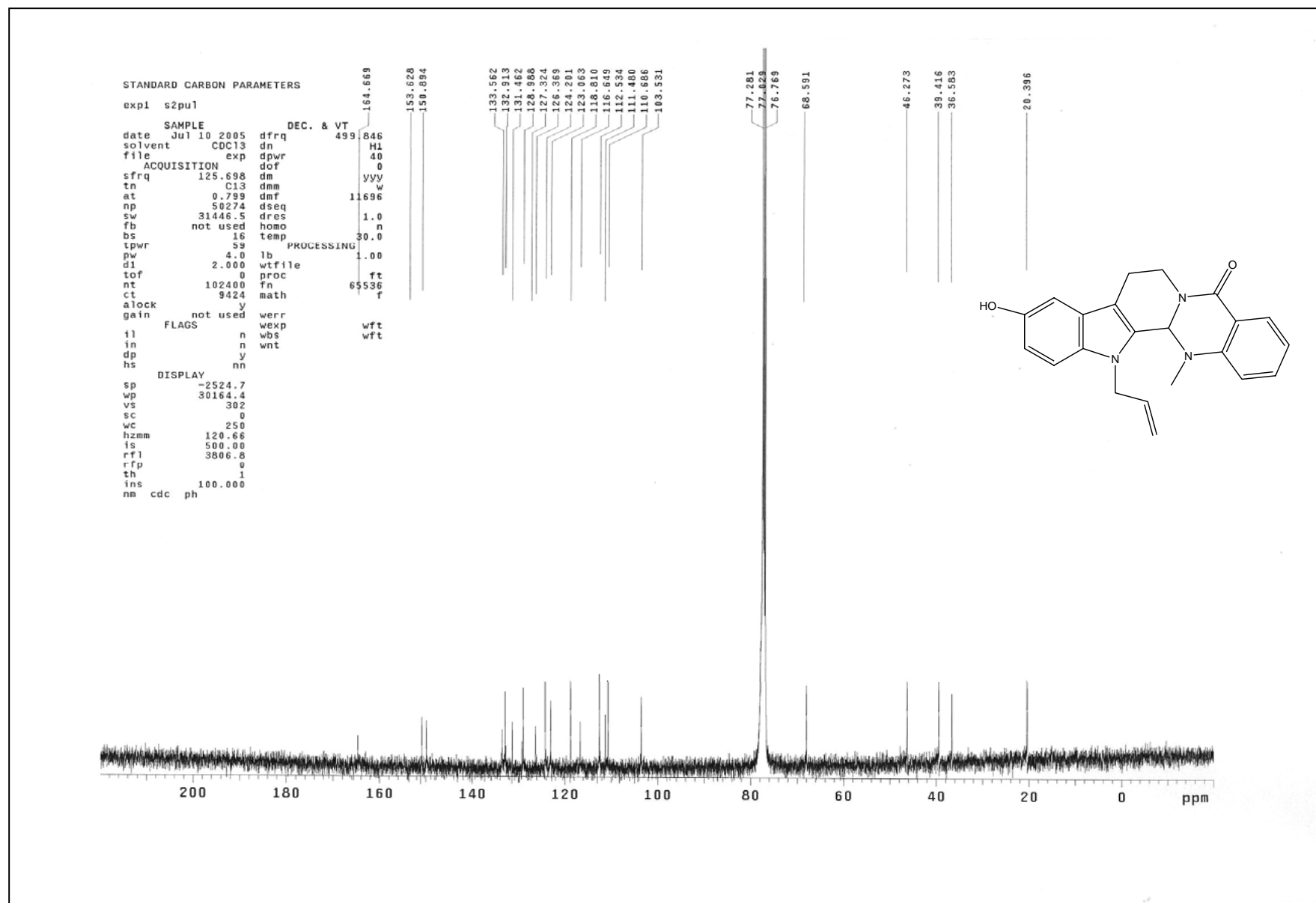
圖 42 化合物 52 之 ^{13}\text{C} 核磁共振光譜圖
