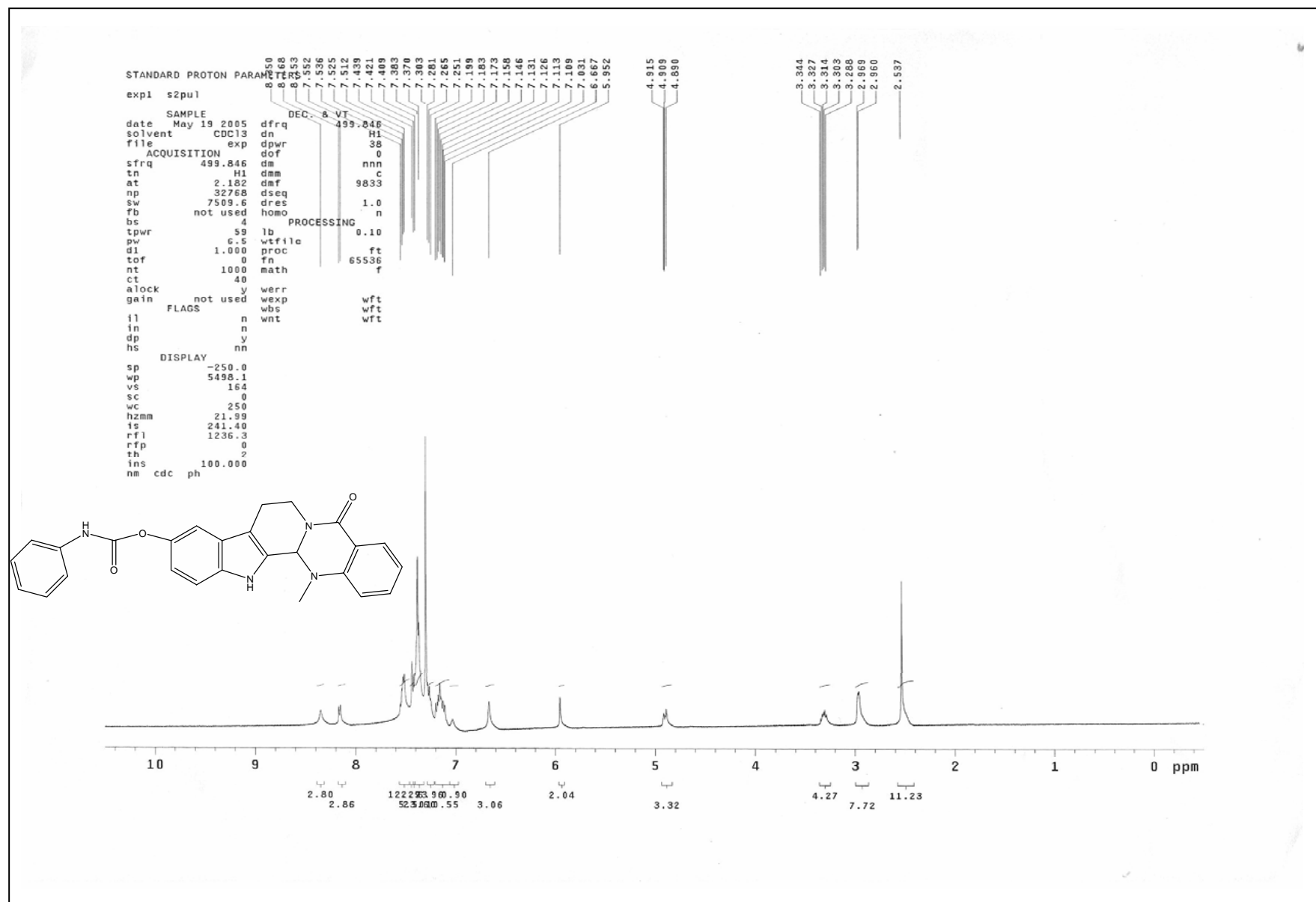
圖 21 化合物 46 之 1 H核磁共振光譜圖
