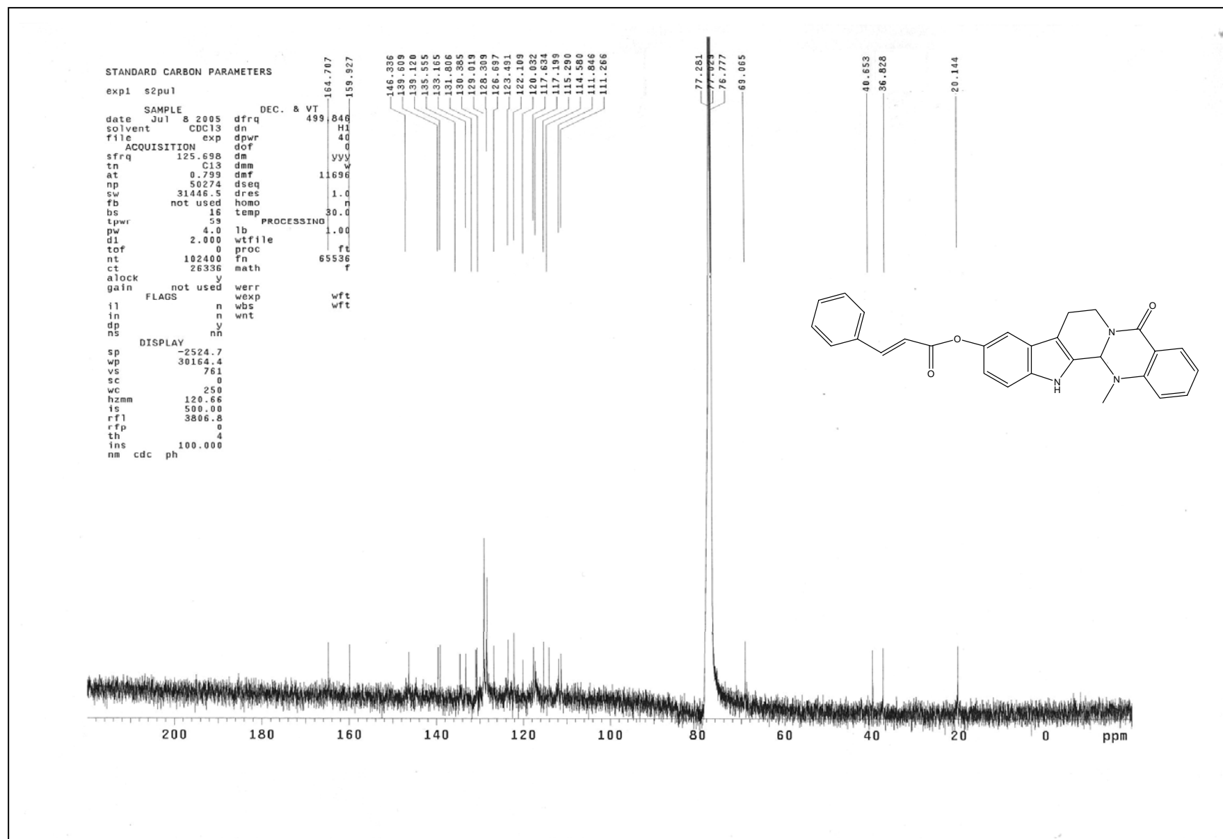
圖 40 化合物 50 之 ^{13}\text{C} 核磁共振光譜圖
