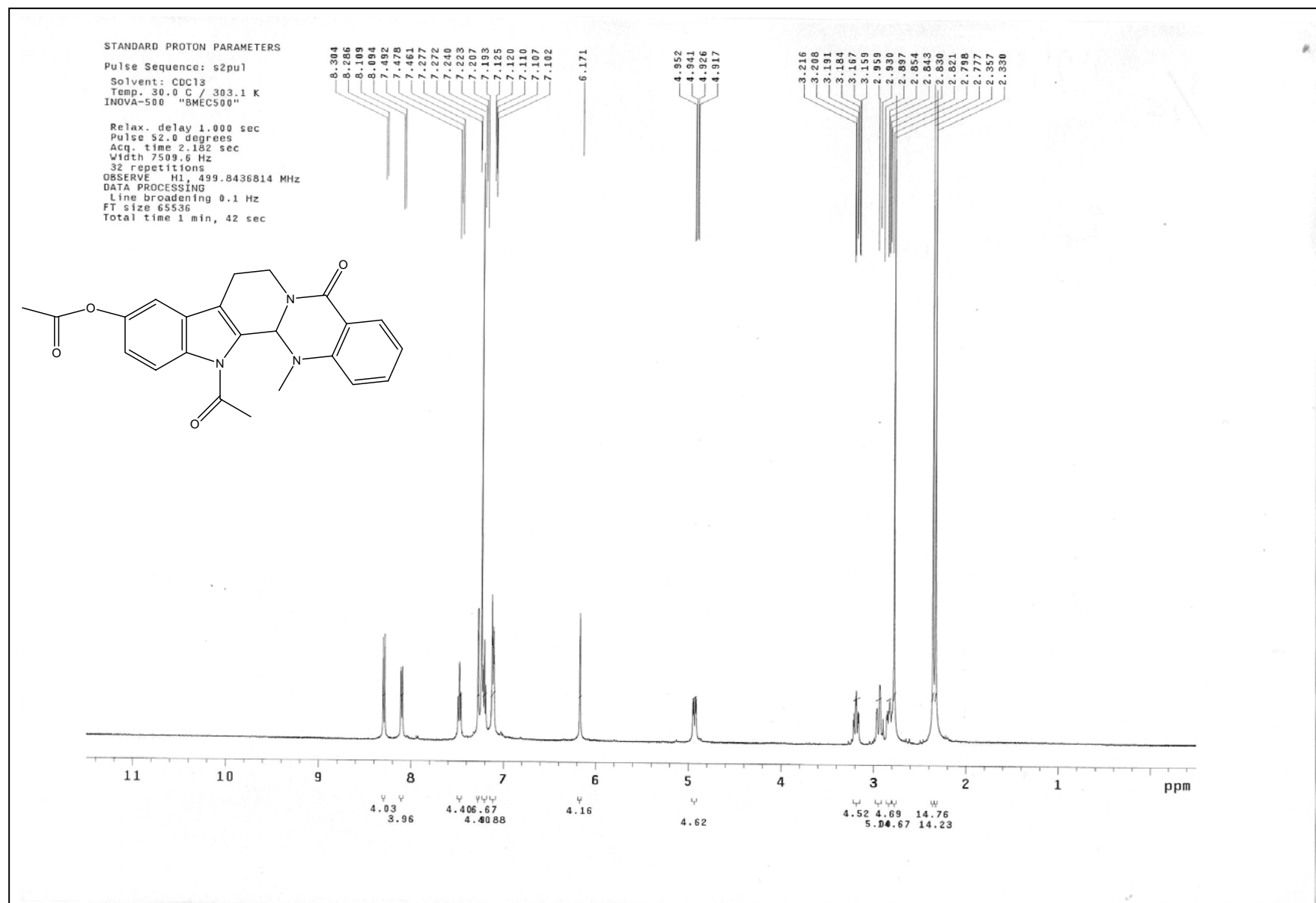
圖 16 化合物 41 之 1 H核磁共振光譜圖
