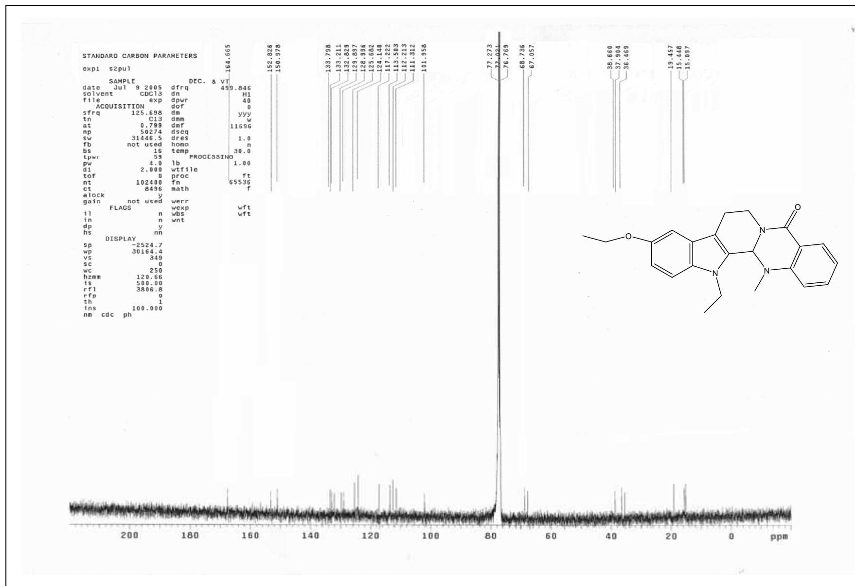
圖 36 化合物之 ^{13}\text{C} 核磁共振光譜圖
