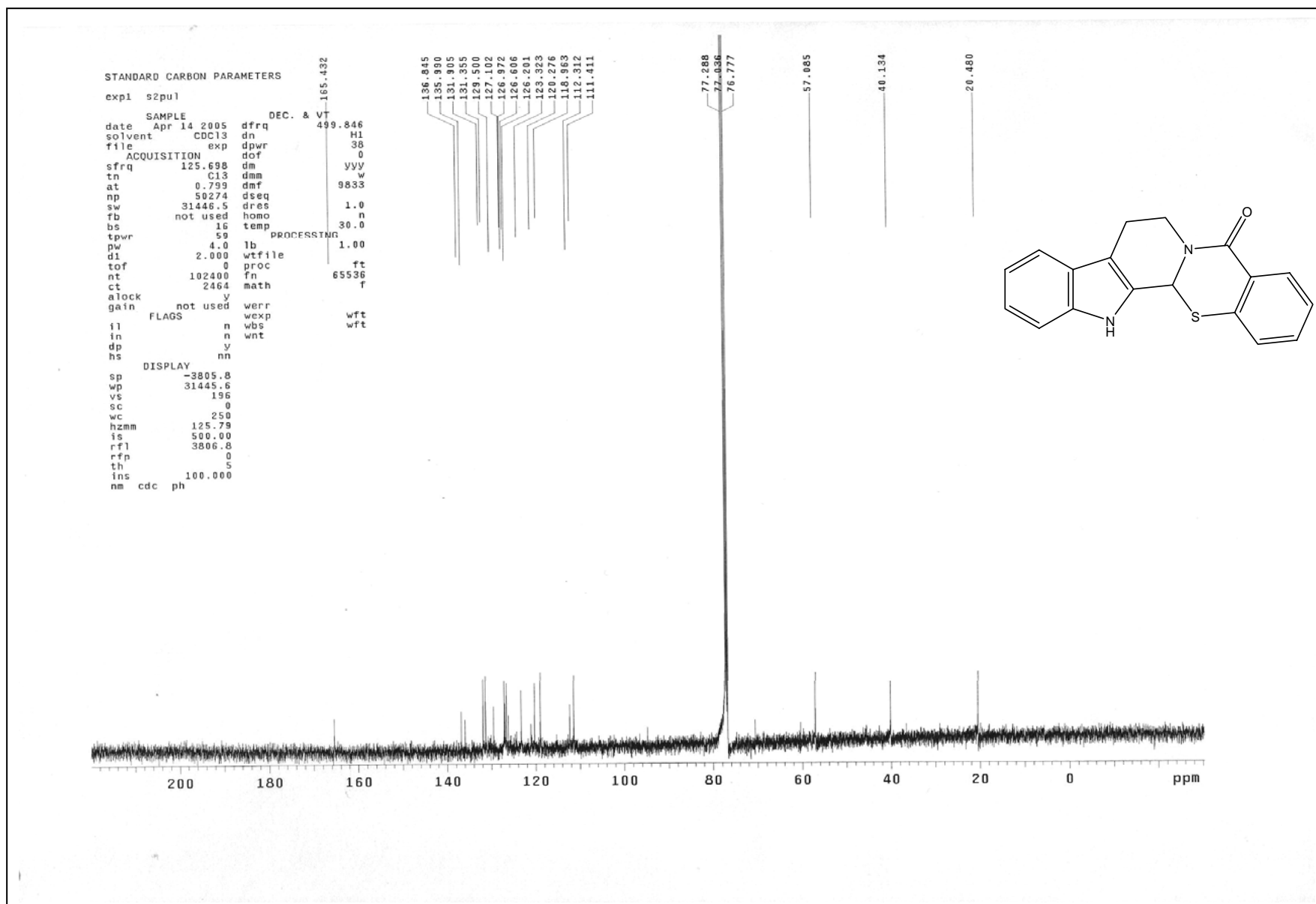
圖 35 化合物 44 之 13 C核磁共振光譜圖
