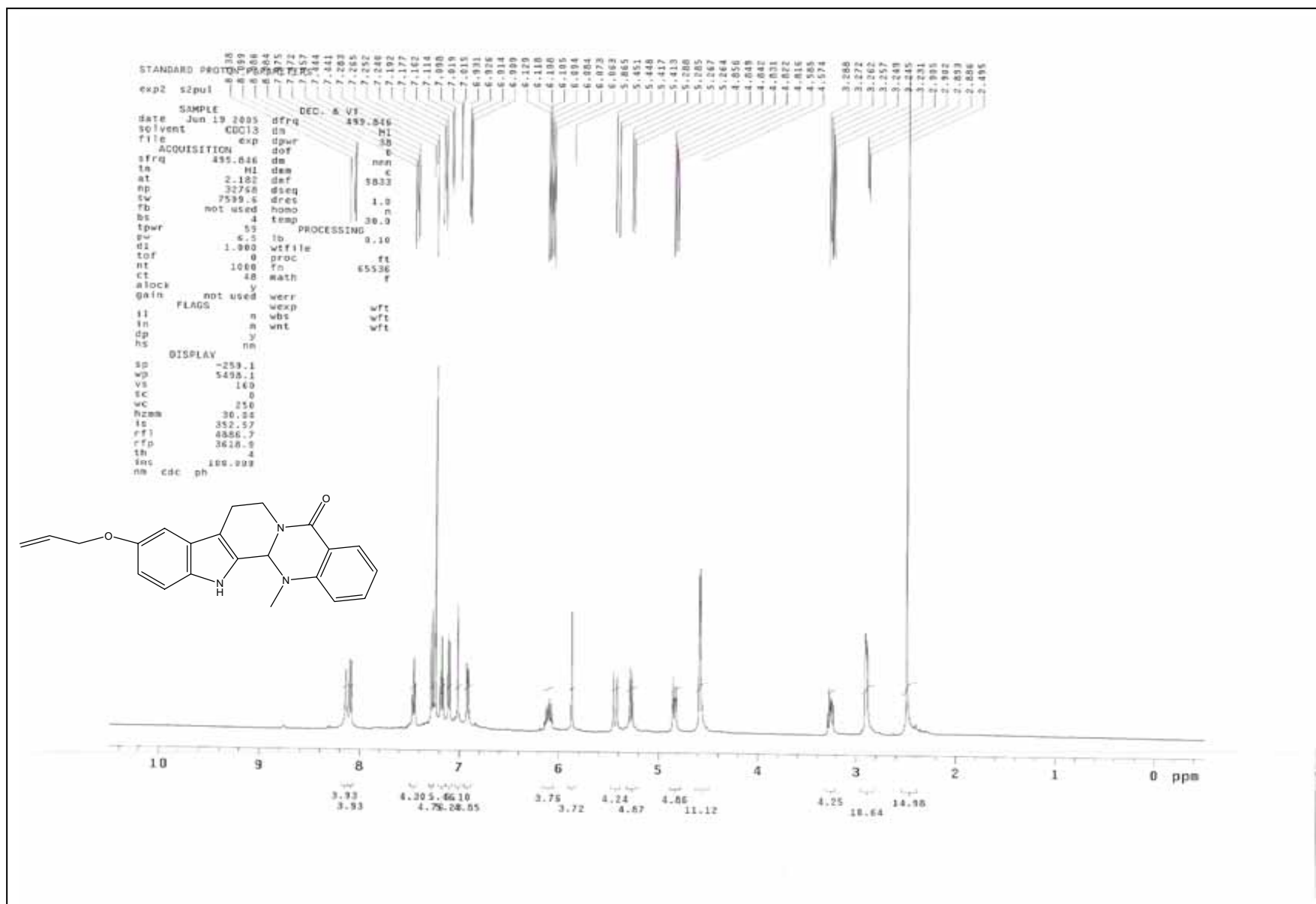
圖 17 化合物 42 之 1 H核磁共振光譜圖
