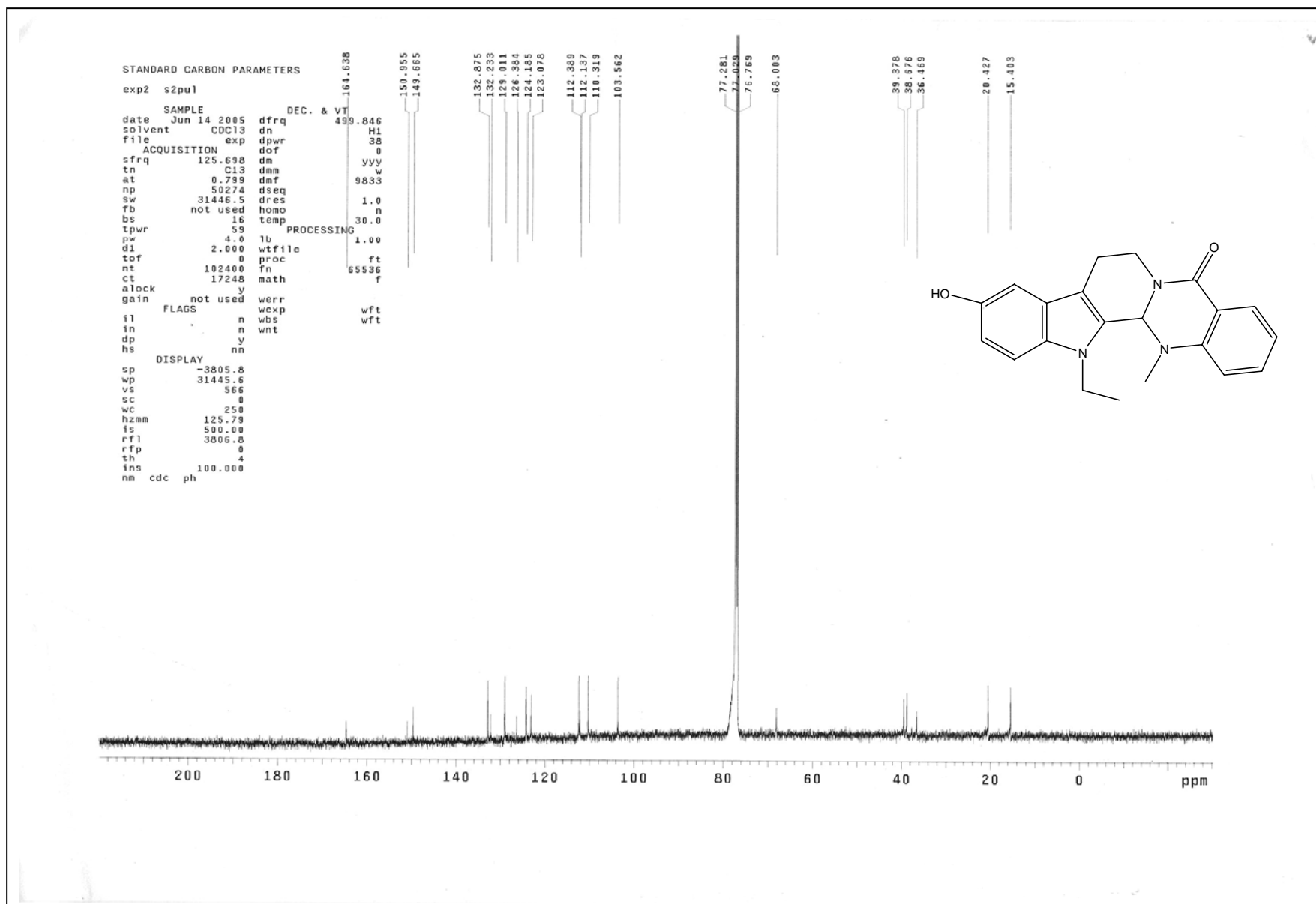
圖 41 化合物 51 之 ^{13}\text{C} 核磁共振光譜圖
