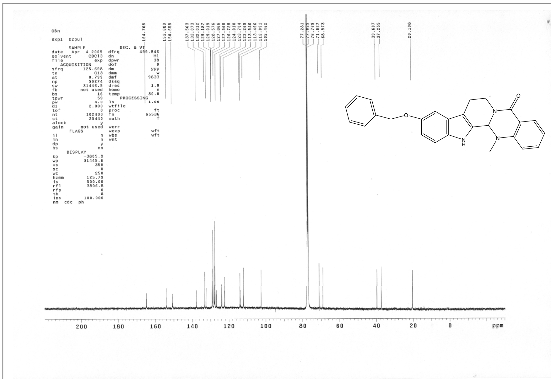
圖 29 化合物 38 之 ^{13}\text{C} 核磁共振光譜圖
