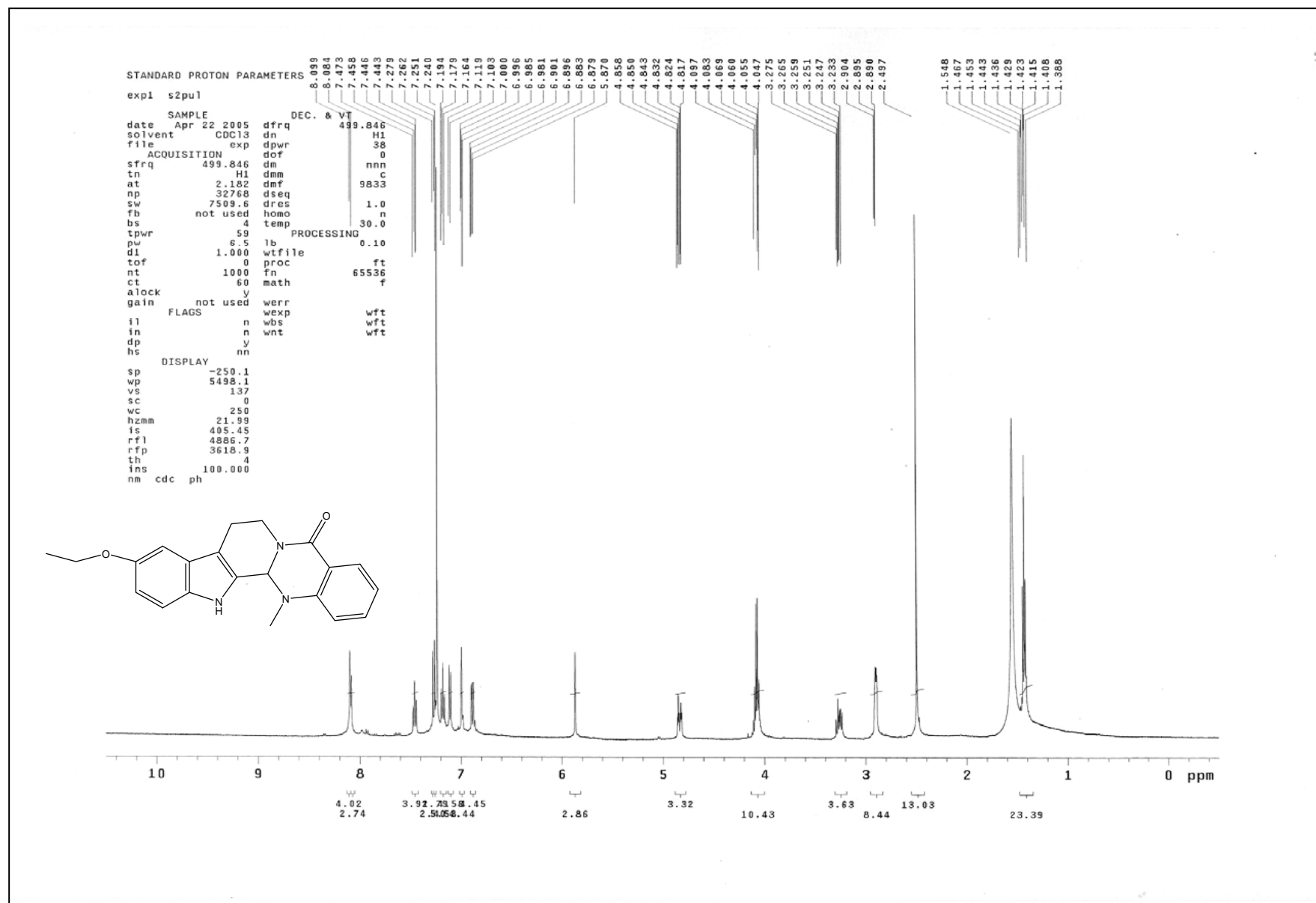
圖 14 化合物 39 之 1 H核磁共振光譜圖
