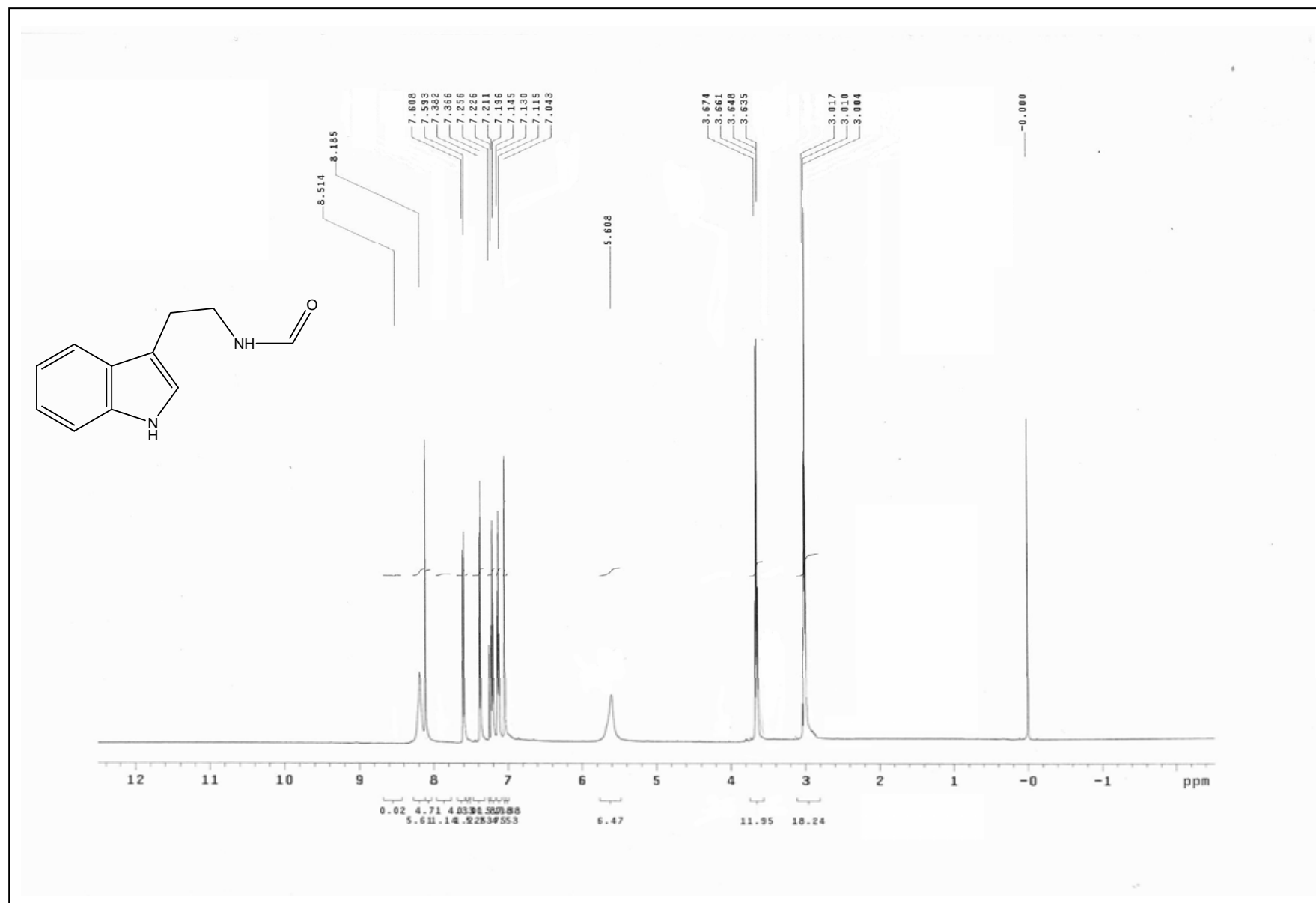
圖 1 化合物 25 之 1 H核磁共振光譜圖
