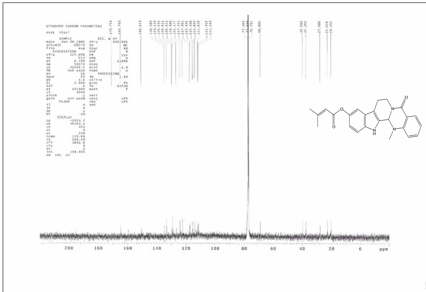
圖 39 化合物 49 之 ^{13}\text{C} 核磁共振光譜圖
