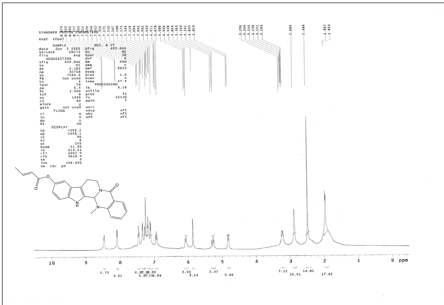
圖 22 化合物 48 之 1 H核磁共振光譜圖
