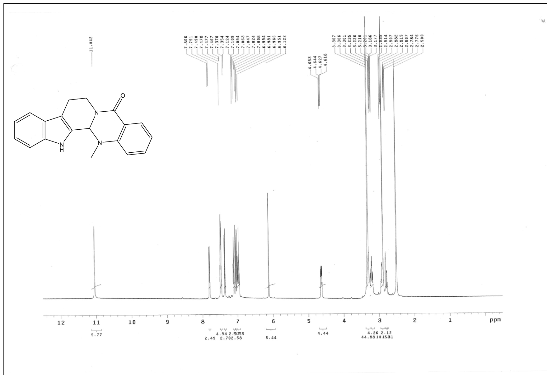
圖 3 化合物 2 之 1 H核磁共振光譜圖
