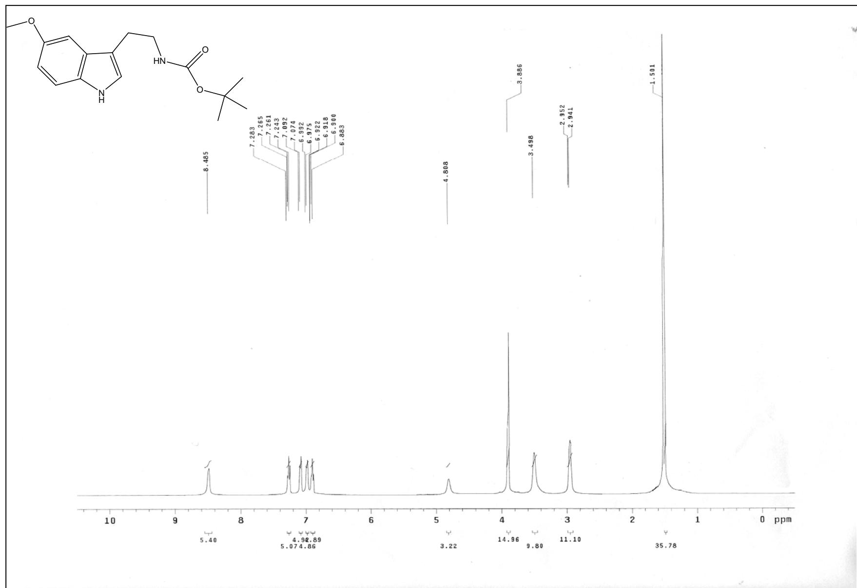
圖 5 化合物 28 之 1 H核磁共振光譜圖
