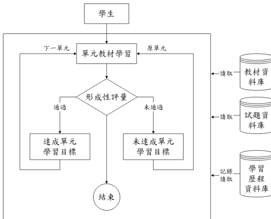
圖 13 適性學習流程圖
