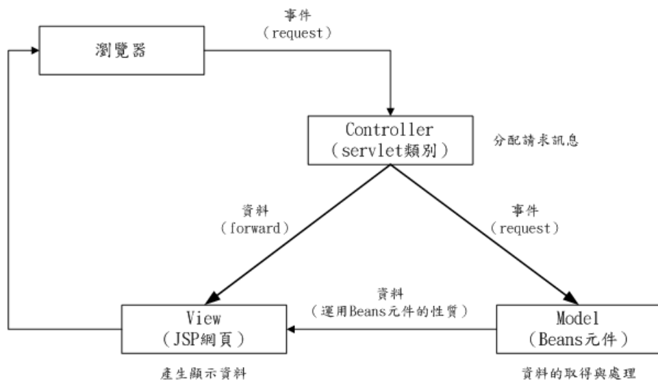
圖 16 MVC 架構圖（資料來源：JSP 動態網頁入門實務）
