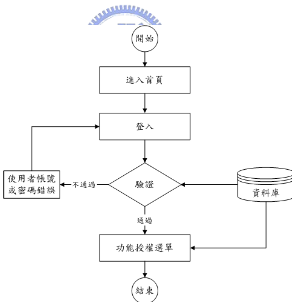
圖 12 系統登入流程圖
