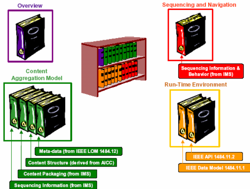
圖 1 SCORM 架構圖 (資料來源：www.adlnet.org)
