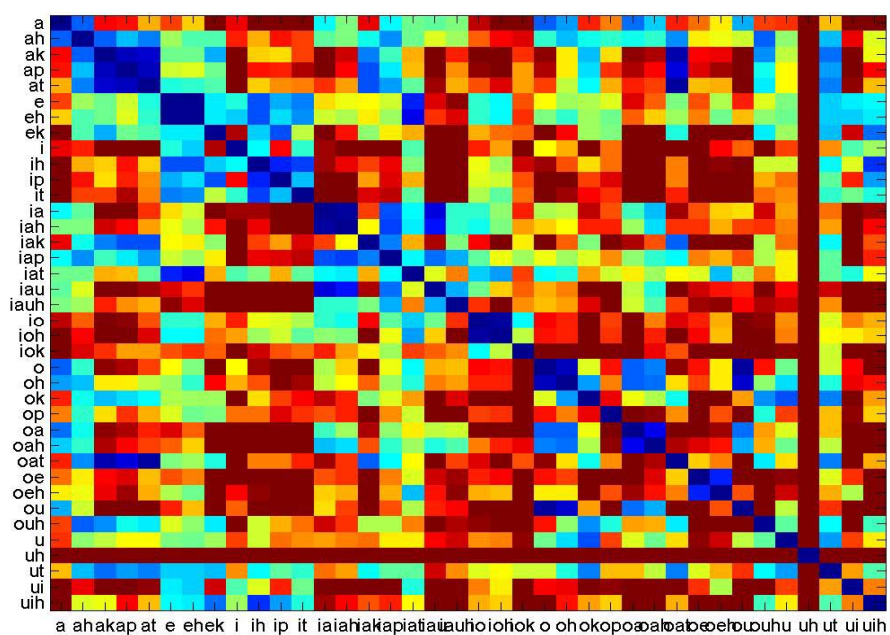
圖五 未根據變調規則修改之前 state3 之間 confusion 的情況，顏色越黑代表 confusion 的情形越嚴重
