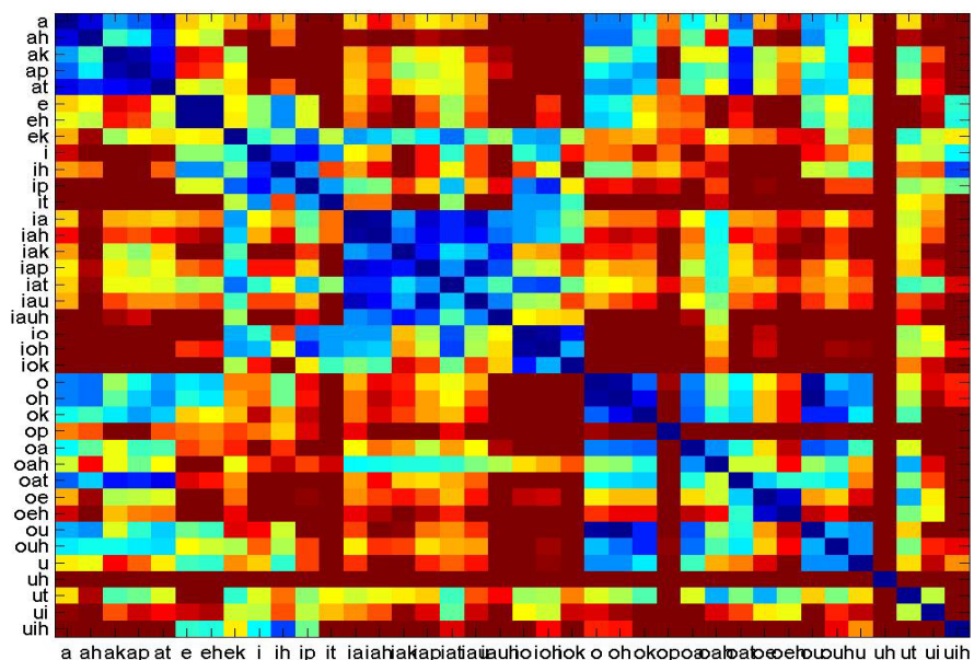
圖三 未根據變調規則修改之前 state2 之間 confusion 的情況, 顏色越黑代表 confusion 的情形越嚴重
