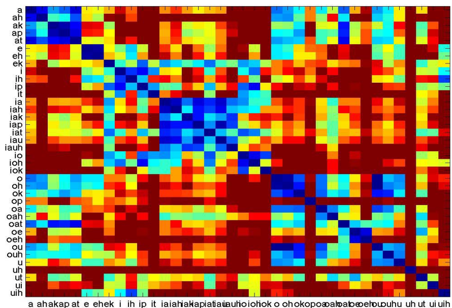
圖四 根據變調規則修改之後 state2 之間 confusion 的情況, 顏色越黑代表 confusion 的情形越嚴重
