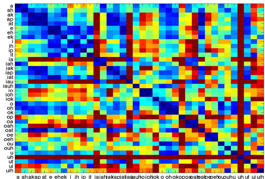
圖七 未根據變調規則修改之前 state4 之間 confusion 的情況，顏色越黑代表 confusion 的情形越嚴重
