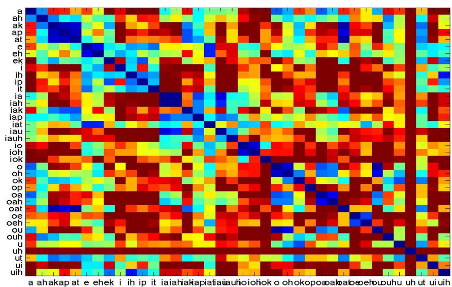
圖六 根據變調規則修改之後 state3 之間 confusion 的情況，顏色越黑代表 confusion 的情形越嚴重
