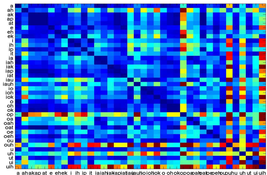
圖十 根據變調規則修改之後 state5 之間 confusion 的情況，顏色越黑代表 confusion 的情形越嚴重
