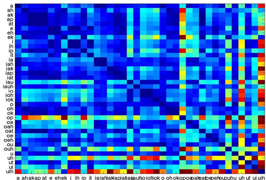
圖九 未根據變調規則修改之前 state5 之間 confusion 的情況，顏色越黑代表 confusion 的情形越嚴重
