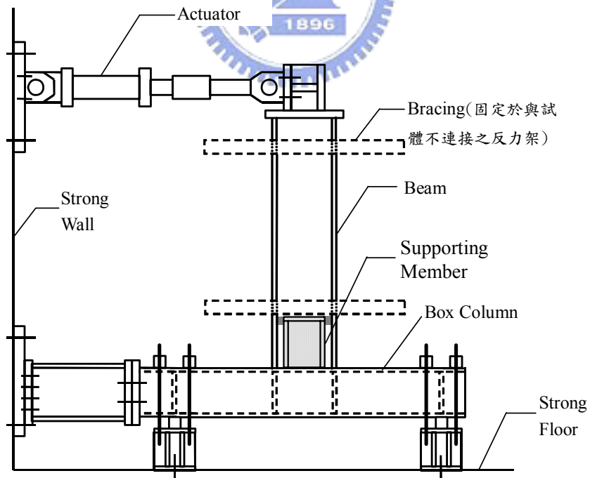
圖 4.9 試驗配置圖
