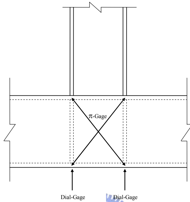
圖 4.10 量測儀器配置圖
