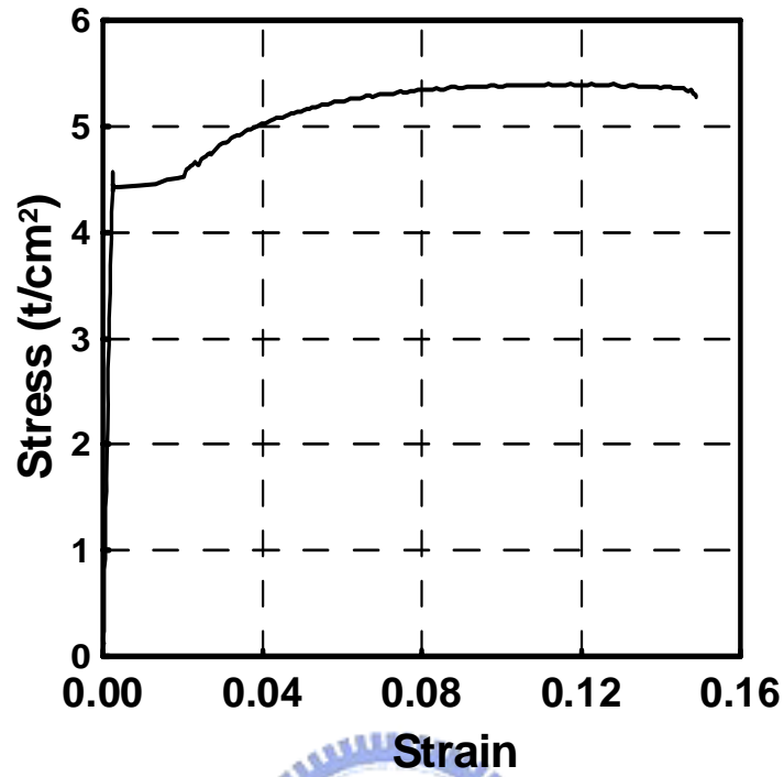
圖 4.8 梁腹板拉力試片應力-應變曲線
