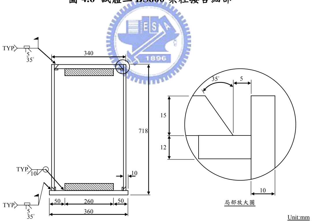
圖 4.7 試體二 BS600 協力桿件接合細部
