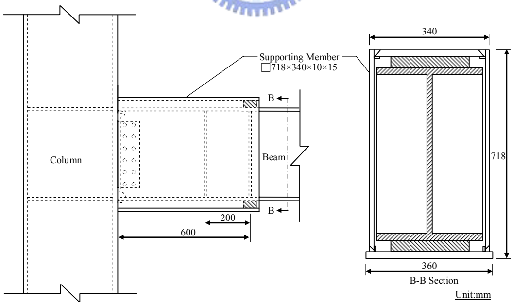
圖 4.5 試體二 BS600 協力桿件配置圖
