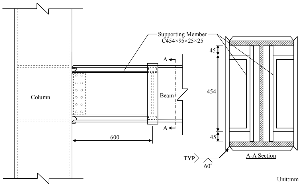
圖 4.2 試體一 CM600 協力桿件配置圖
