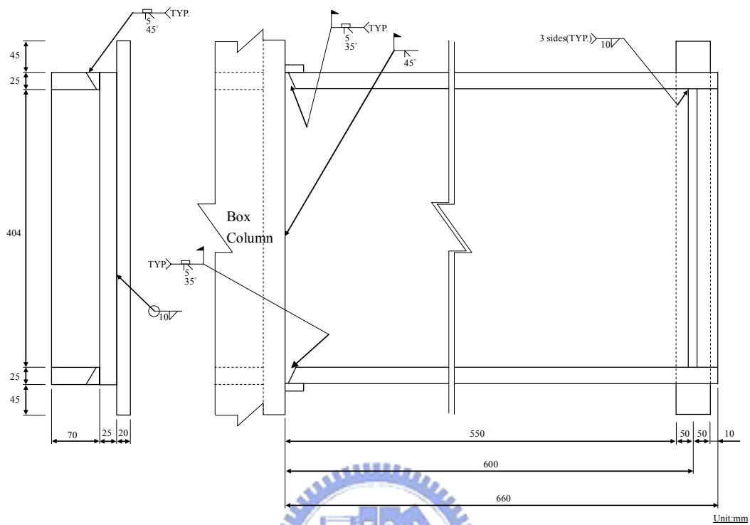
圖 4.4 試體一 CM600 協力桿件接合細部
