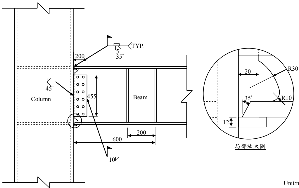
圖 4.6 試體二 BS600 梁柱接合細部
