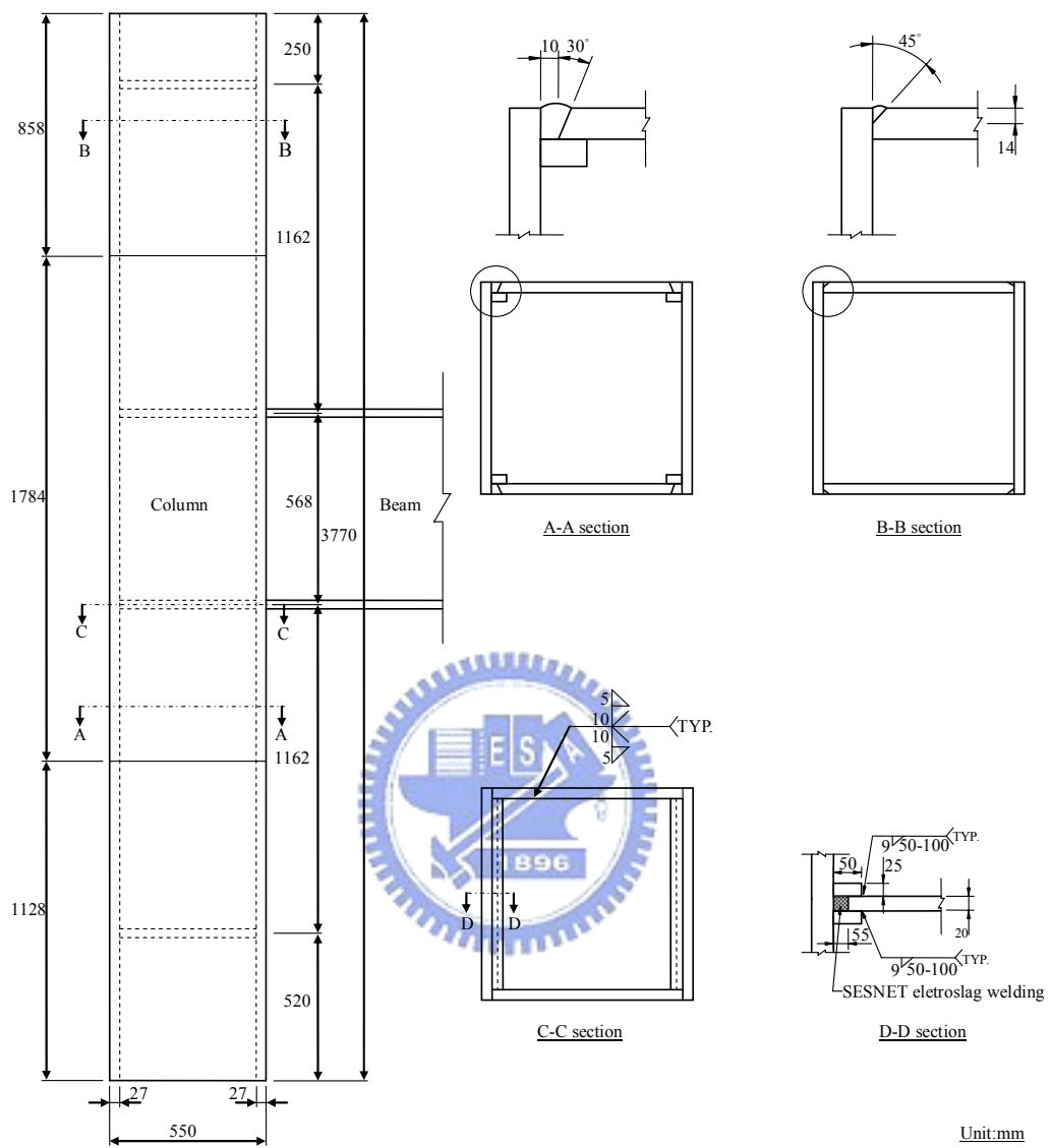
圖 4.1 柱試體接合細部
