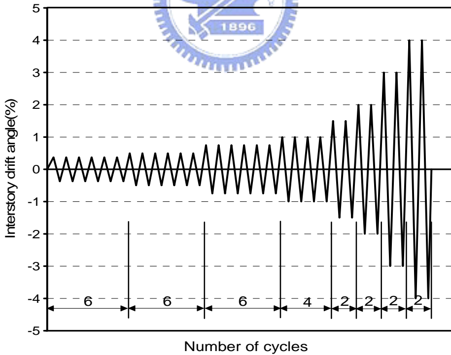
圖 4.11 位移控制歷程圖
