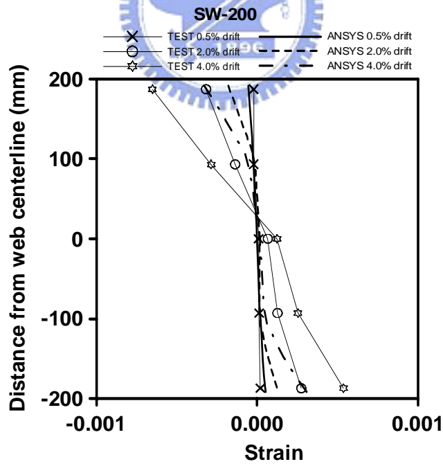
圖 6.6 CM400 於 SW-200 位置模擬與實驗之應變分佈比較
