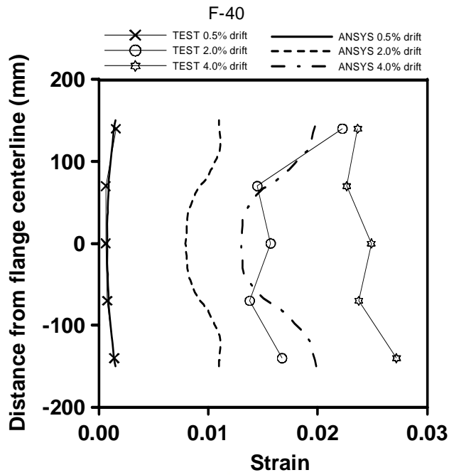
圖 6.3 CM400 於 F-40 位置模擬與實驗之應變分佈比較
