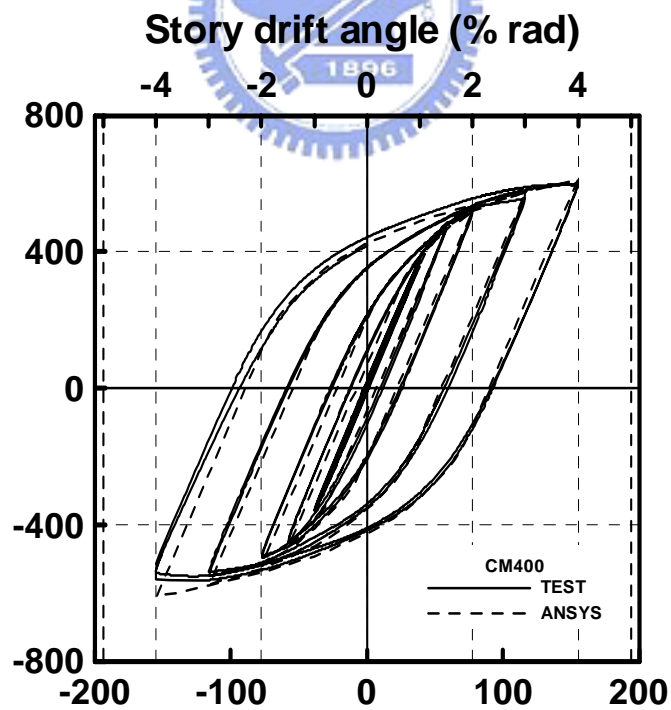
圖 6.2 CM400 模擬與實驗之梁端載重-位移曲線
