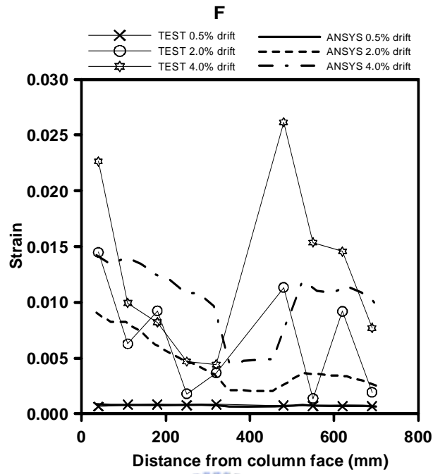
圖 6.5 CM400 於 F 位置模擬與實驗之應變分佈比較
