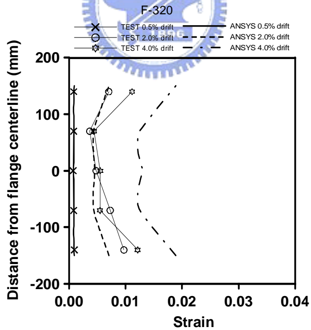
圖 6.4 CM400 於 F-320 位置模擬與實驗之應變分佈比較
