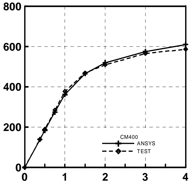
圖 6.1 CM400 模擬與實驗之梁端載重-位移包絡線
