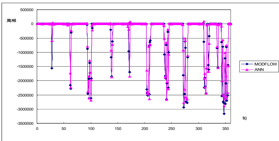
圖附 A.38 案例 2-1(c)模擬 C 湖溢流量
