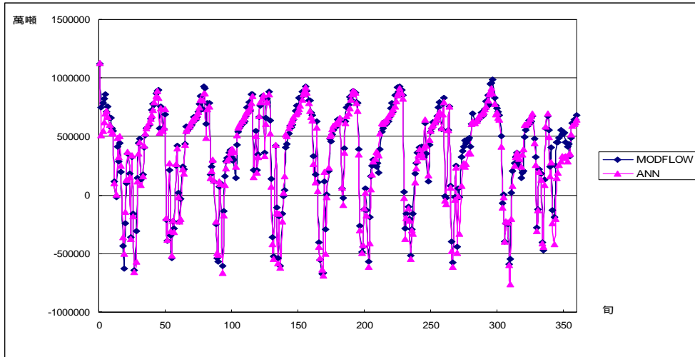
圖附 A.33 案例 2-1(c)模擬 C 湖交換量
