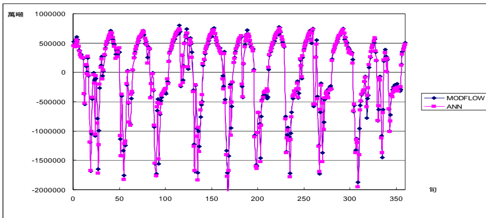
圖附 A.32 案例 2-1(c)模擬 B 湖交換量
