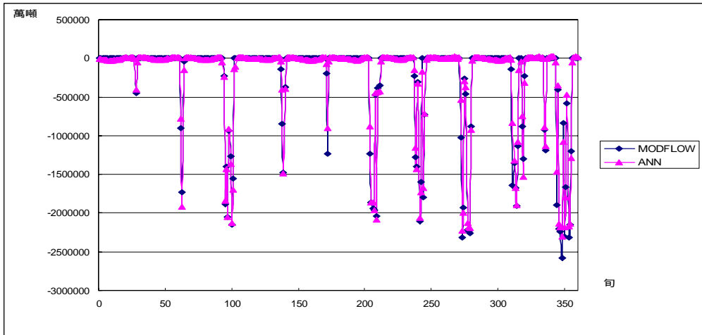
圖附 A.36 案例 2-1(c)模擬 A 湖溢流量
