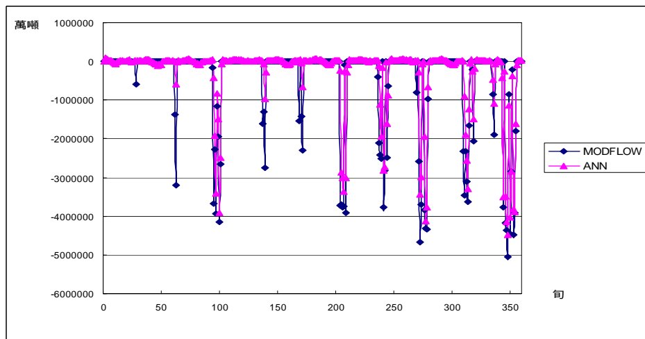
圖附 A.10 案例 1-2 模擬 E 湖溢流量
