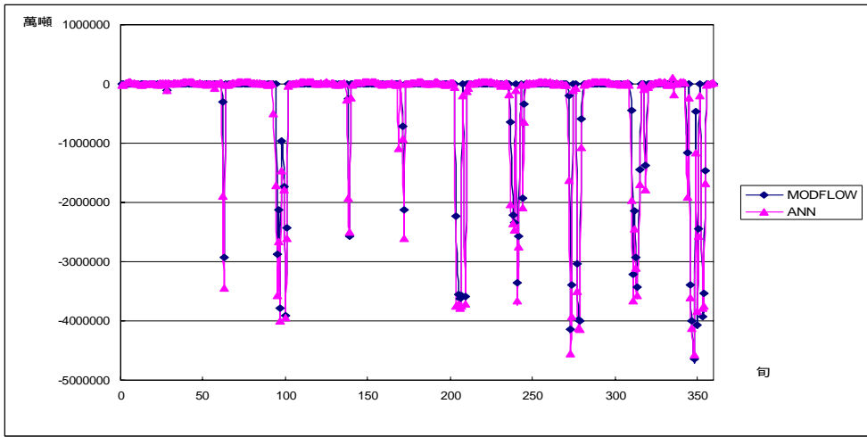
圖附 A.49 案例 2-2 模擬 D 湖溢流量
