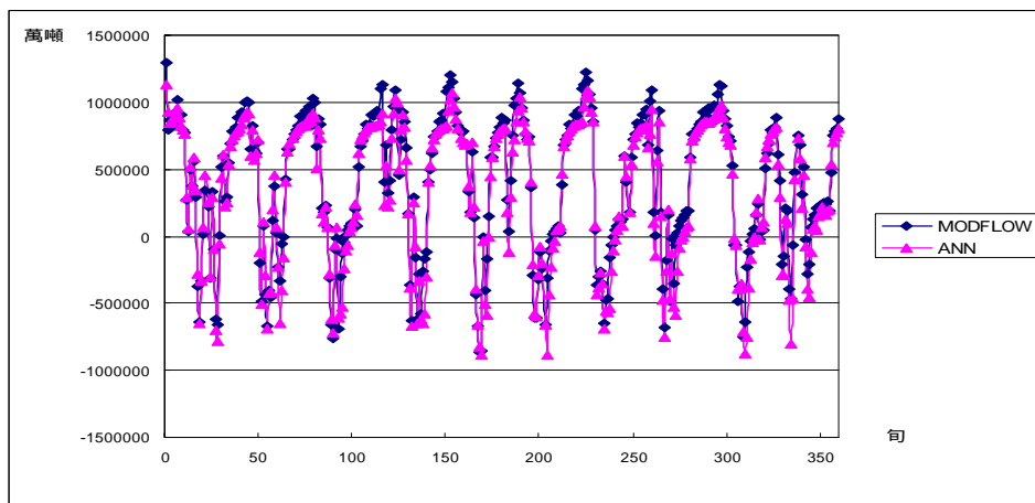
圖附 A.11 案例 2-1(a)模擬 A 湖交換量
