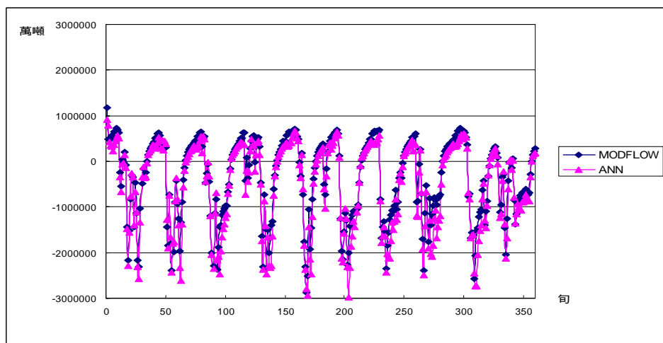
圖附 A.5 案例 1-2 模擬 E 湖交換量
