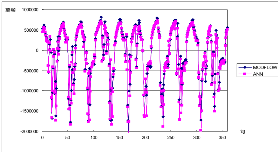
圖附 A.12 案例 2-1(a)模擬 B 湖交換量
