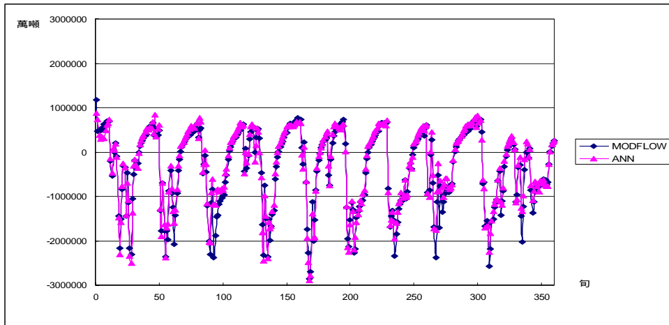
圖附 A.25 案例 2-1(b)模擬 E 湖交換量
