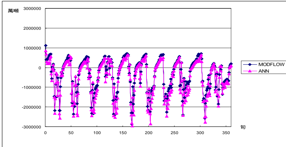
圖附 A.15 案例 2-1(a)模擬 E 湖交換量
