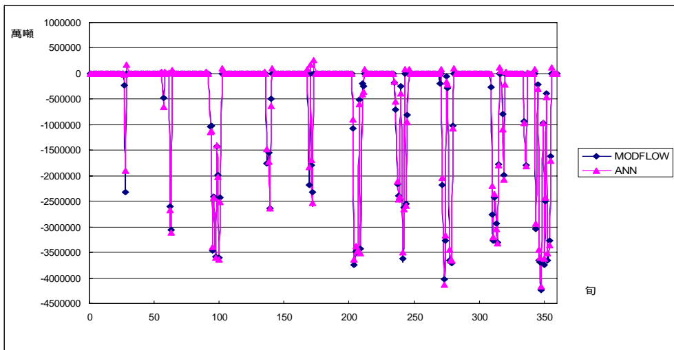
圖附 A.37 案例 2-1(c)模擬 B 湖溢流量
