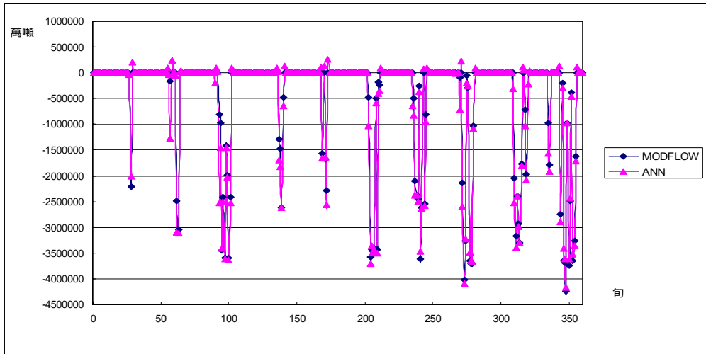
圖附 A.27 案例 2-1(b)模擬 B 湖溢流量
