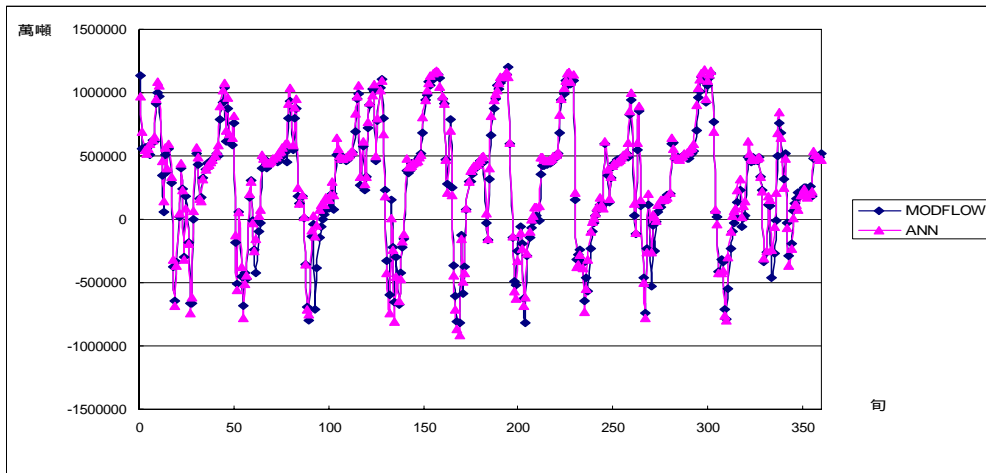
圖附 A.21 案例 2-1(b)模擬 A 湖交換量
