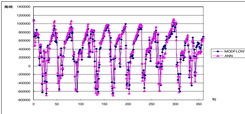
圖附 A.43 案例 2-2 模擬 C 湖交換量
