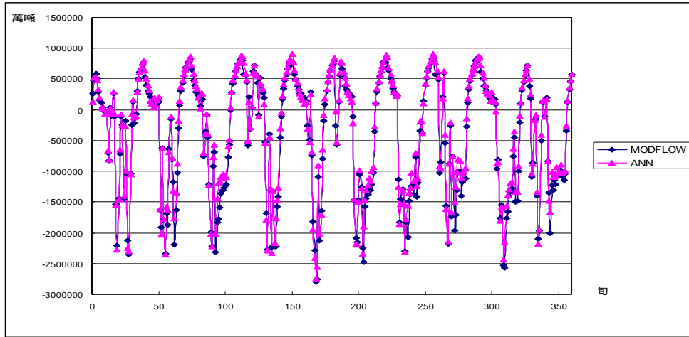
圖附 A.24 案例 2-1(b)模擬 D 湖交換量
