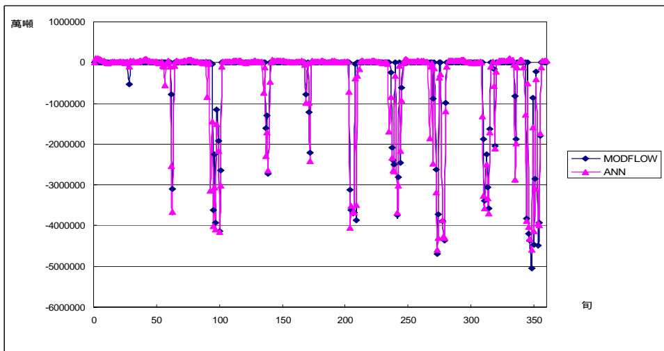
圖附 A.50 案例 2-2 模擬 E 湖溢流量
