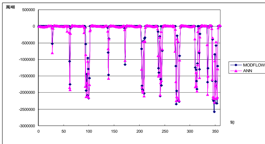
圖附 A.26 案例 2-1(b)模擬 A 湖溢流量
