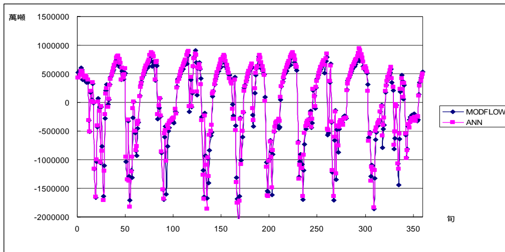
圖附 A.22 案例 2-1(b)模擬 B 湖交換量
