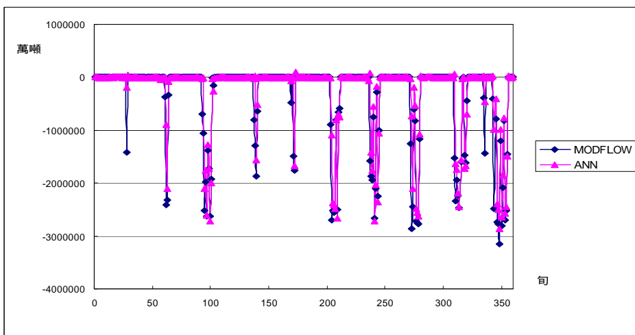
圖附 A.8 案例 1-2 模擬 C 湖溢流量
