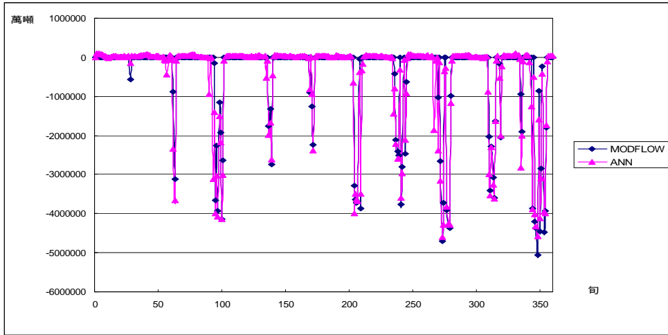
圖附 A.30 案例 2-1(b)模擬 E 湖溢流量
