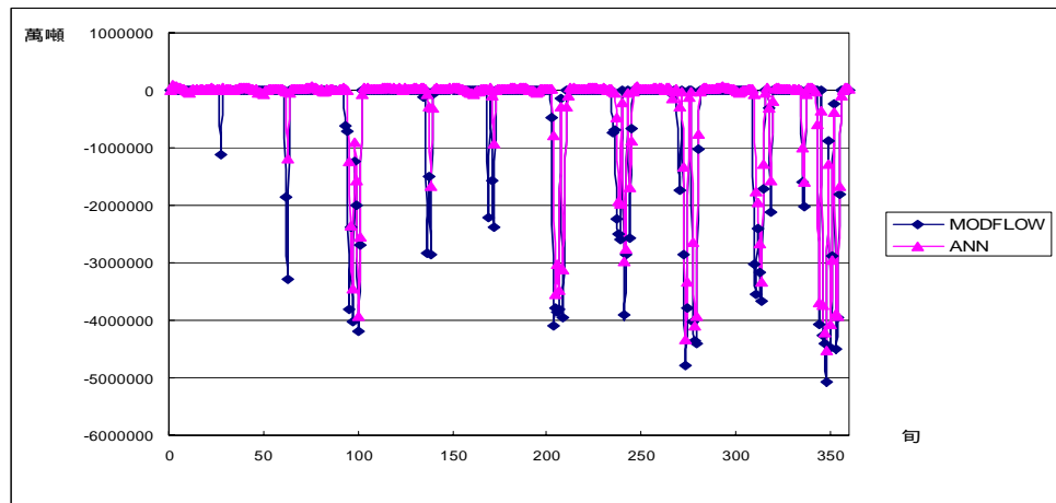
圖附 A.20 案例 2-1(a)模擬 E 湖溢流量
