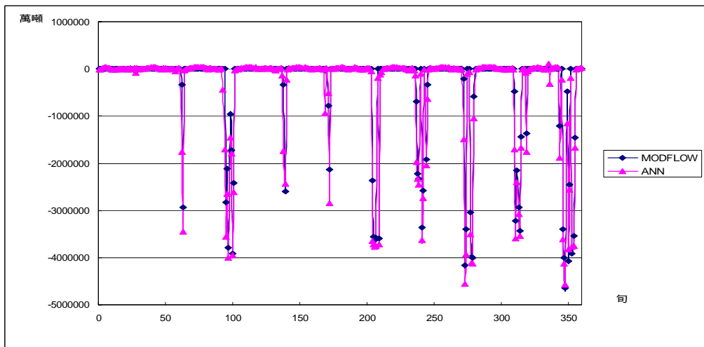
圖附 A.29 案例 2-1(b)模擬 D 湖溢流量
