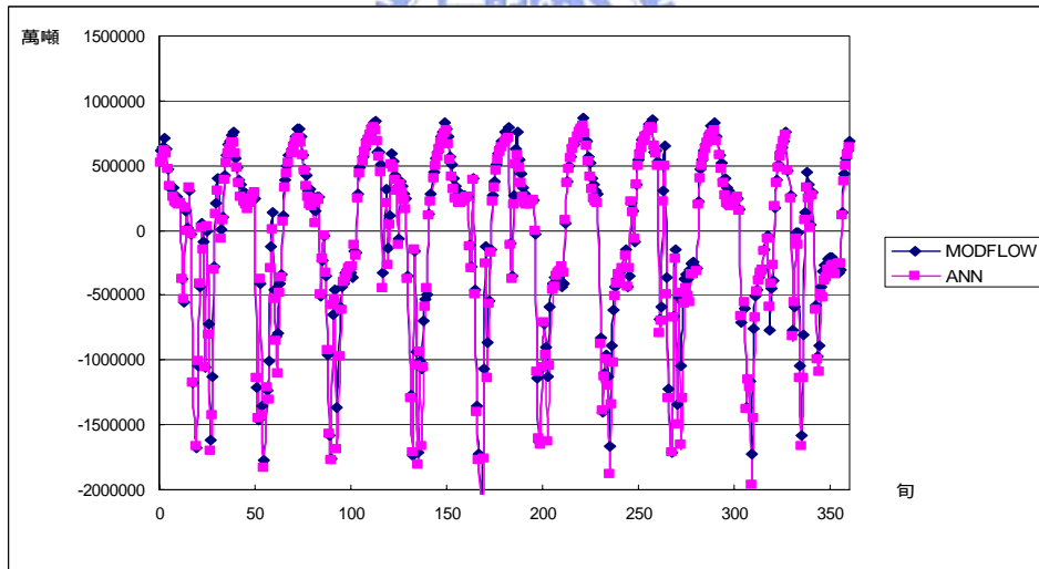
圖附 A.2 案例 1-2 模擬 B 湖交換量
