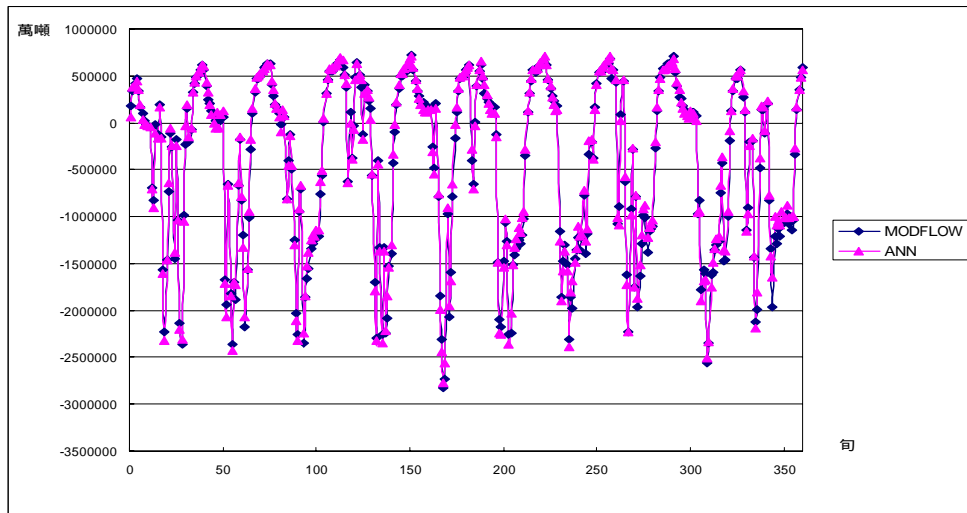
圖附 A.34 案例 2-1(c)模擬 D 湖交換量
