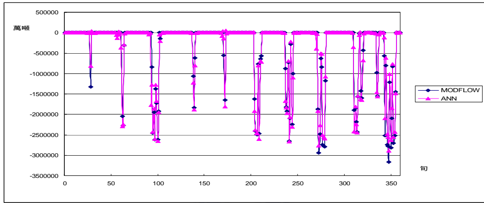
圖附 A.28 案例 2-1(b)模擬 C 湖溢流量
