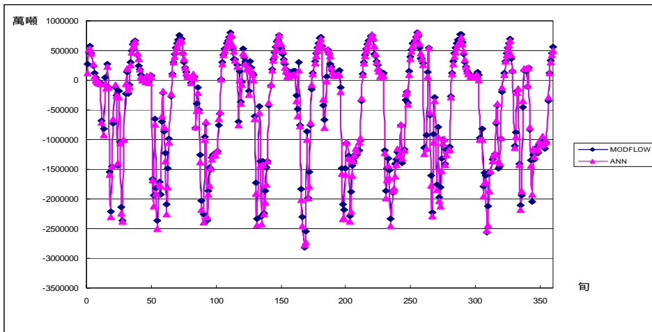
圖附 A.4 案例 1-2 模擬 D 湖交換量
