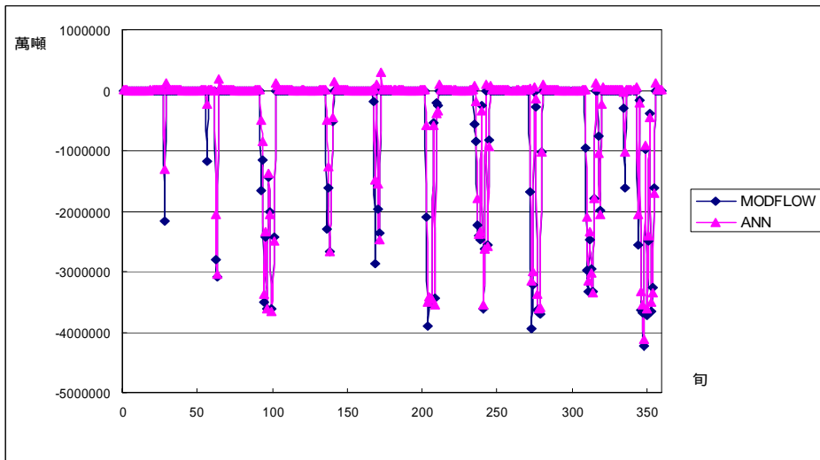
圖附 A.7 案例 1-2 模擬 B 湖溢流量
