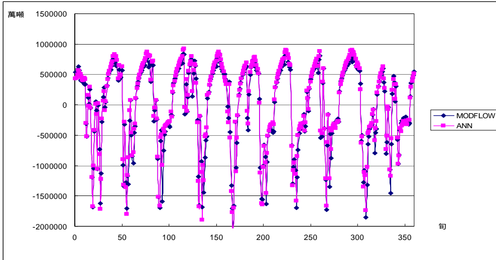
圖附 A.42 案例 2-2 模擬 B 湖交換量
