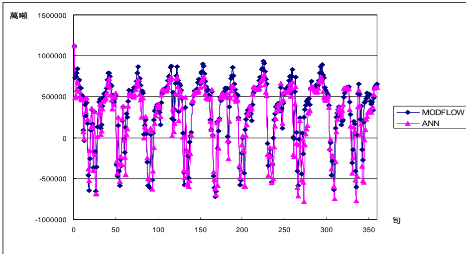
圖附 A.3 案例 1-2 模擬 C 湖交換量
