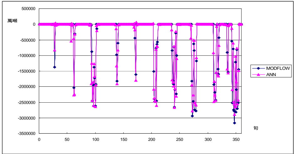
圖附 A.48 案例 2-2 模擬 C 湖溢流量
