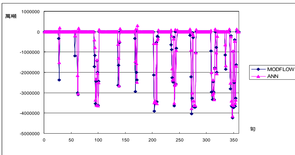
圖附 A.17 案例 2-1(a)模擬 B 湖溢流量
