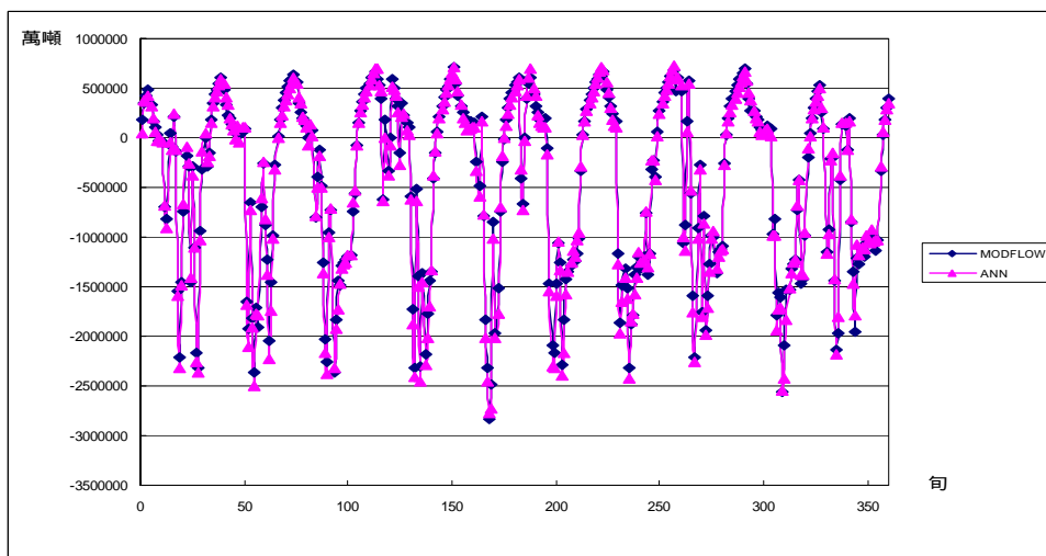
圖附 A.14 案例 2-1(a)模擬 D 湖交換量
