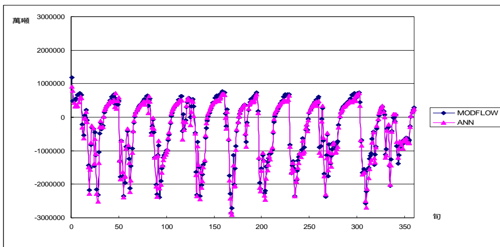
圖附 A.35 案例 2-1(c)模擬 E 湖交換量
