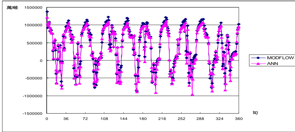
圖附 A.1 案例 1-2 模擬 A 湖交換量
