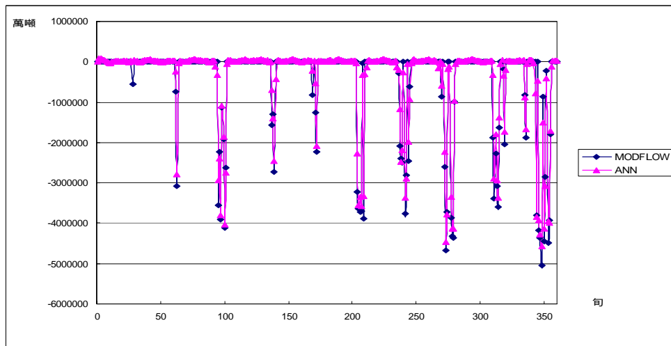
圖附 A.40 案例 2-1(c)模擬 E 湖溢流量
