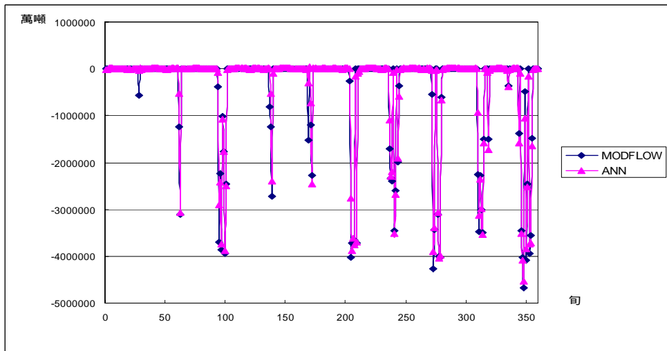
圖附 A.19 案例 2-1(a)模擬 D 湖溢流量
