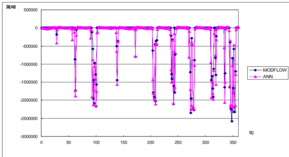
圖附 A.46 案例 2-2 模擬 A 湖溢流量
