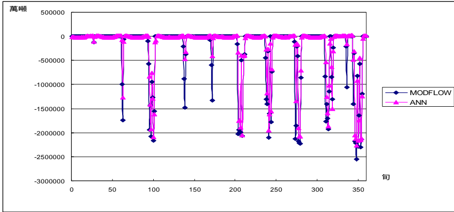
圖附 A.6 案例 1-2 模擬 A 湖溢流量
