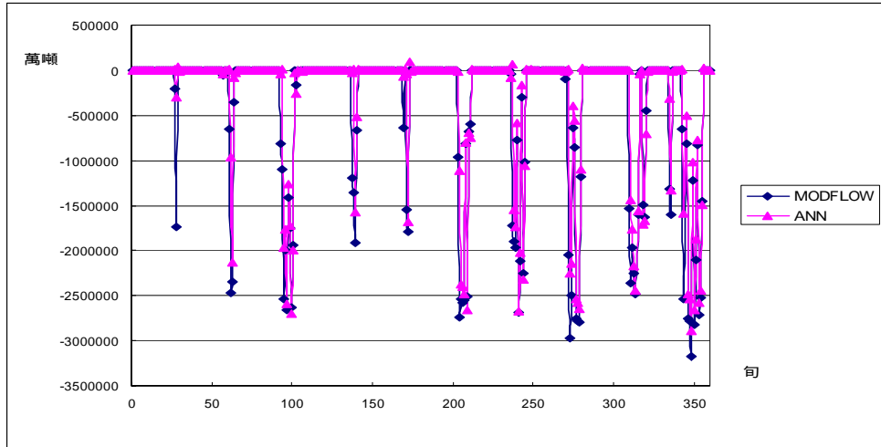
圖附 A.18 案例 2-1(a)模擬 C 湖溢流量
