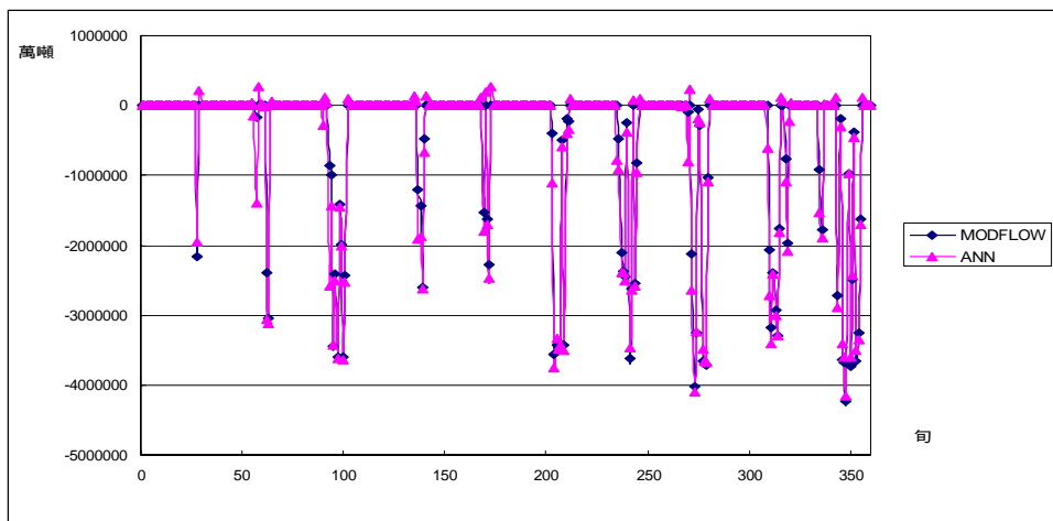
圖附 A.47 案例 2-2 模擬 B 湖溢流量
