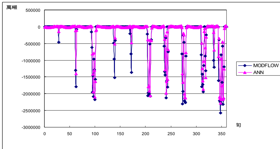
圖附 A.16 案例 2-1(a)模擬 A 湖溢流量
