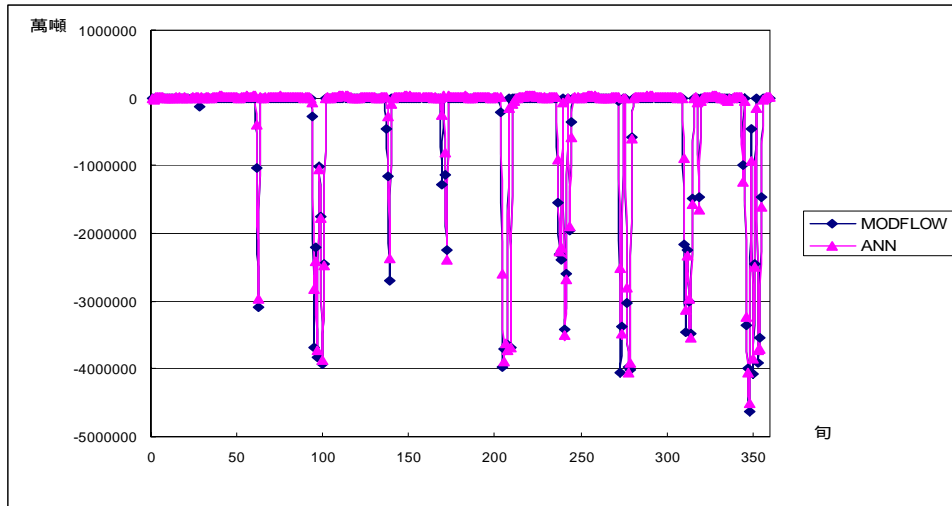
圖附 A.9 案例 1-2 模擬 D 湖溢流量
