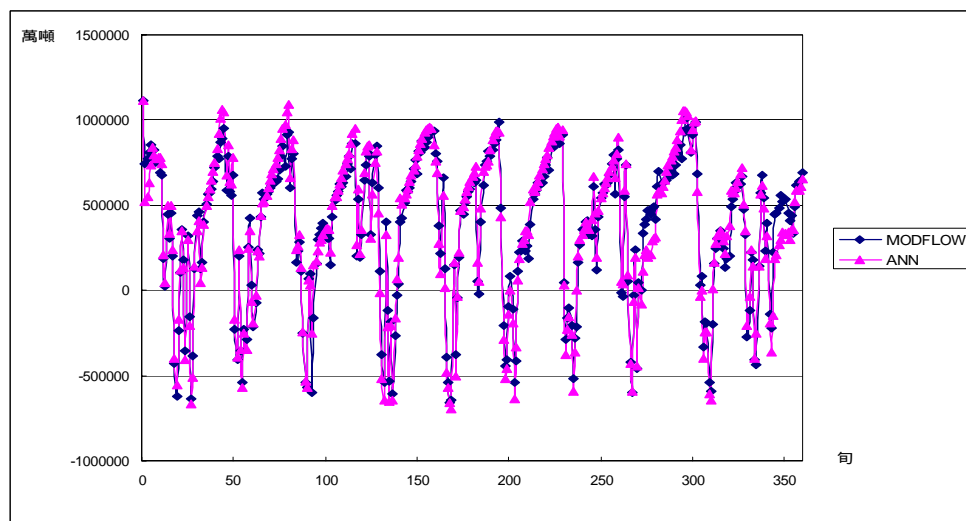
圖附 A.23 案例 2-1(b)模擬 C 湖交換量
